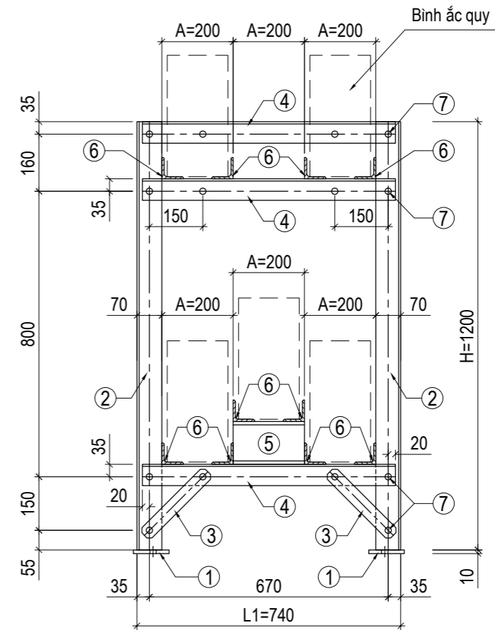
MẶT CẮT 2-2
