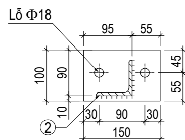
CHI TIẾT BẢN ĐÉ
