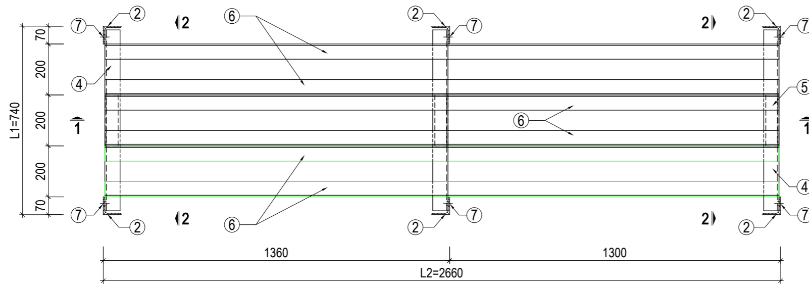
MẶT BẰNG
