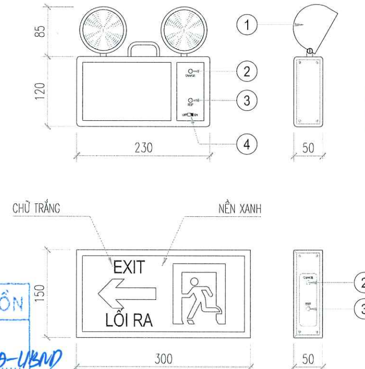
CHI TIẾT KÍCH THƯỚC CÁC LOẠI ĐÈN
