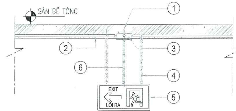
CHI TIẾT LẮP ĐẶT ĐÈN EXIT THOÁT NẠN LOẠI CHỈ MỘT HƯỚNG
