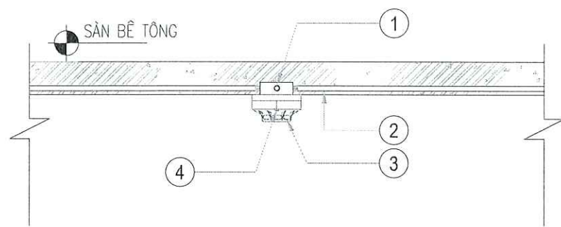
CHI TIẾT LẮP ĐẶT ĐÀU BÁO DƯỚI SÀN BÊ TÔNG
