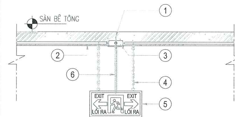
CHI TIẾT LẮP ĐẶT ĐÈN EXIT THOÁT NẠN LOẠI CHỈ HAI HƯỚNG
