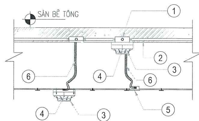
CHI TIẾT LẮP ĐẶT ĐÀU BÁO DƯỚI TRẦN GIẢ
