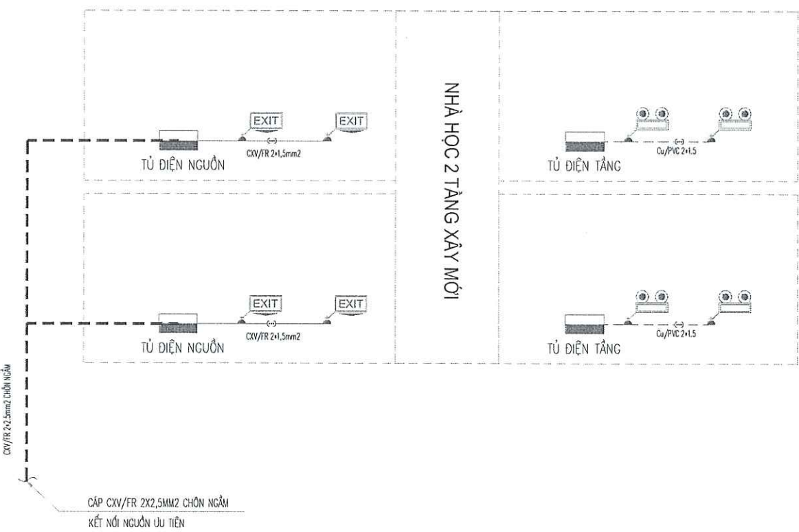
SƠ ĐỒ NGUYÊN LÝ CẤP ĐIỆN ĐÈN EXIT, ĐÈN CHIẾU SÁNG SỰ CỐ
