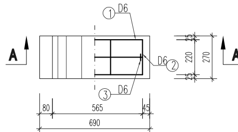
CHI TIẾT ĐẾ CỐNG D500
