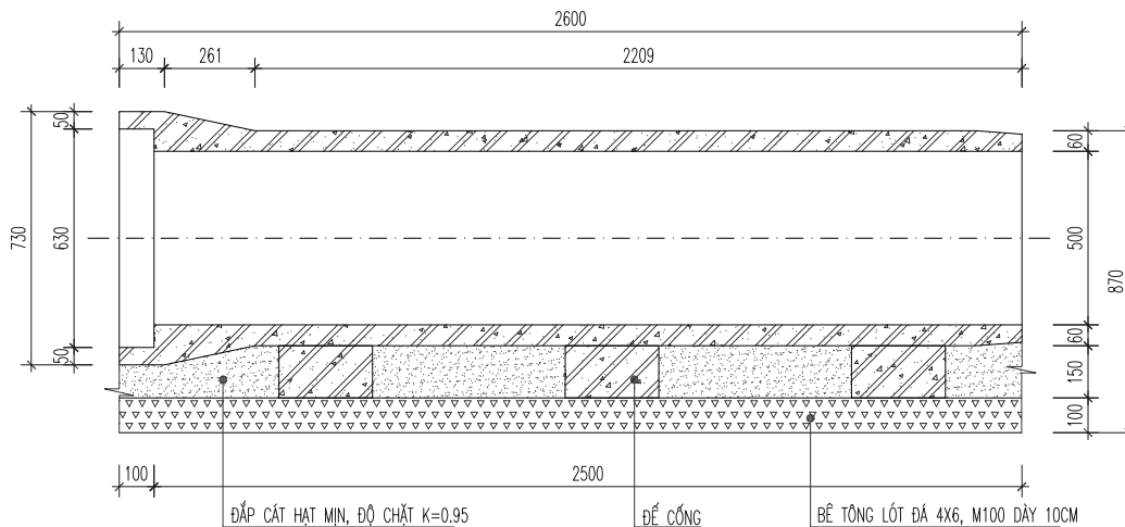
CHI TIẾT CỐNG D500
