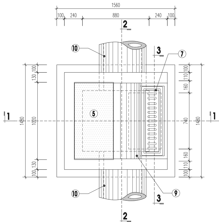
MẶT BẰNG GA
