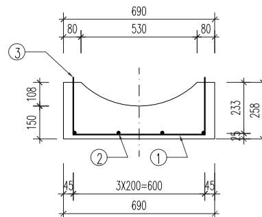
MẶT CẮT A-A
