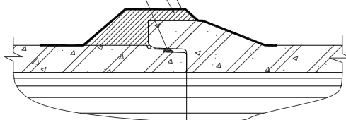
CHI TIẾT MỐI NỐI CỐNG
