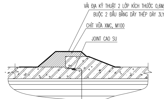
CHI TIẾT MỖI NƠI CỐNG
