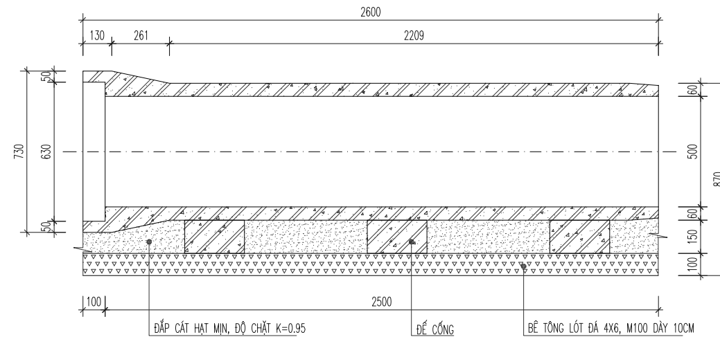
CHI TIẾT CỔNG D500
