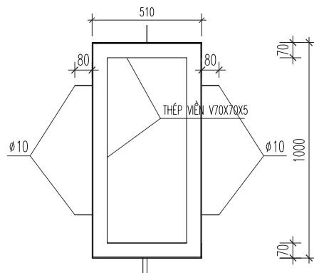
THÉP HÌNH TẤM ĐAN 5
