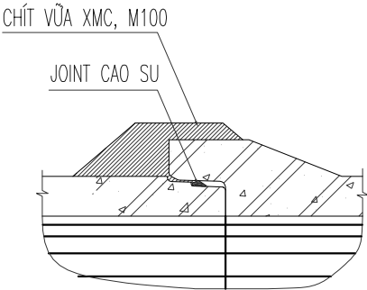
CHI TIẾT MỐI NỐI CỐNG
