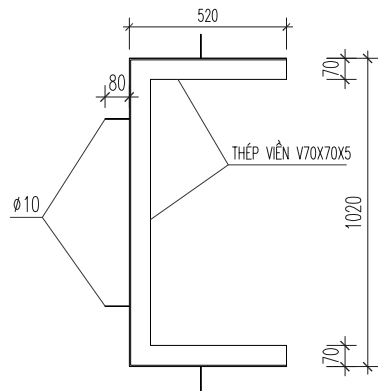
THÉP HÌNH CỔ GA K1
