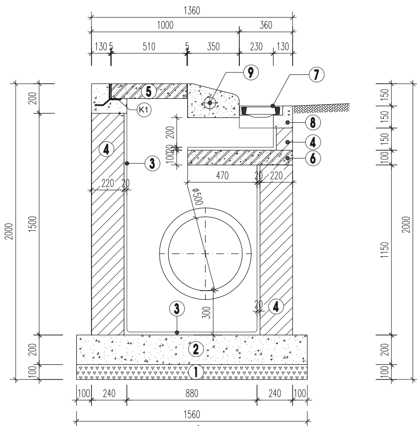
MẶT CẮT 1-1
