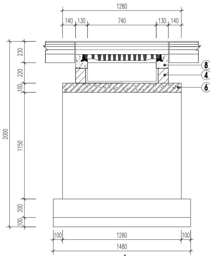
MẶT CẮT 3-3
