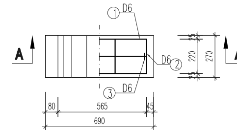
CHI TIẾT ĐỂ CỐNG D500
