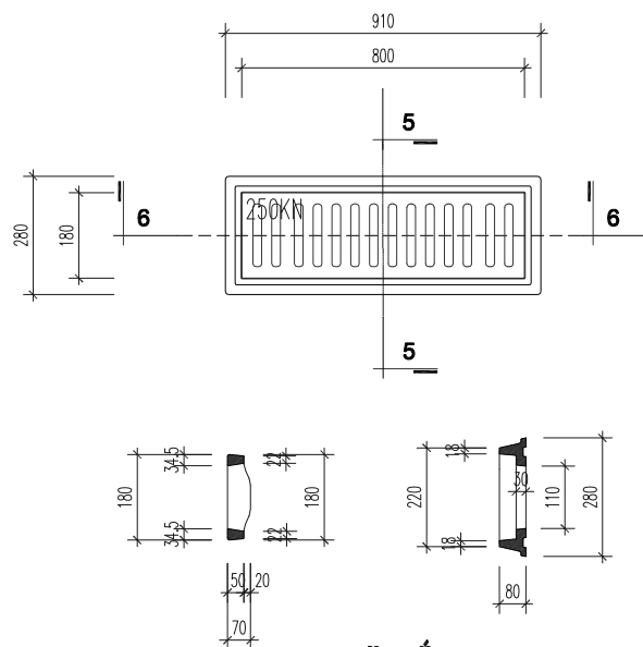
MẶT CẮT 5-5
