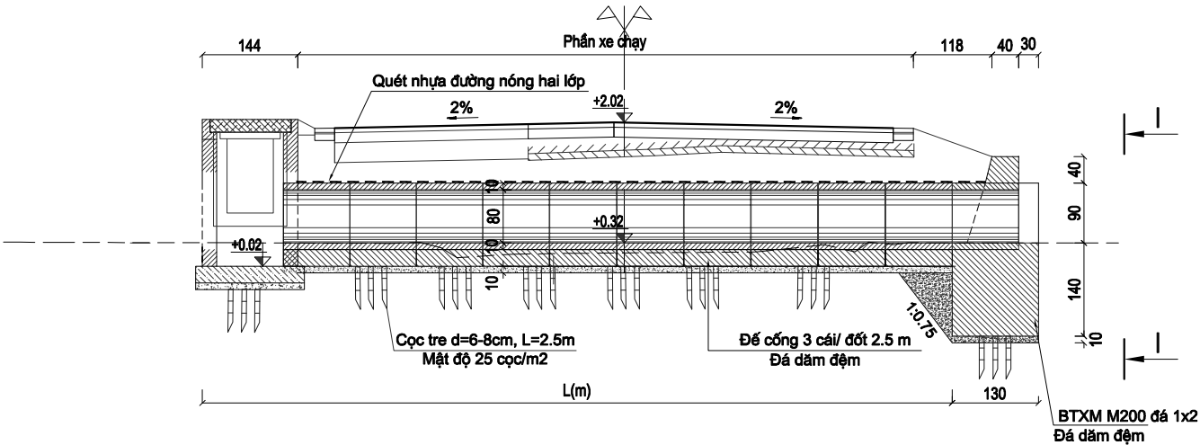
CẮT DỌC CỐNG TRÒN NGANG ĐƯỜNG BTCT D=800
