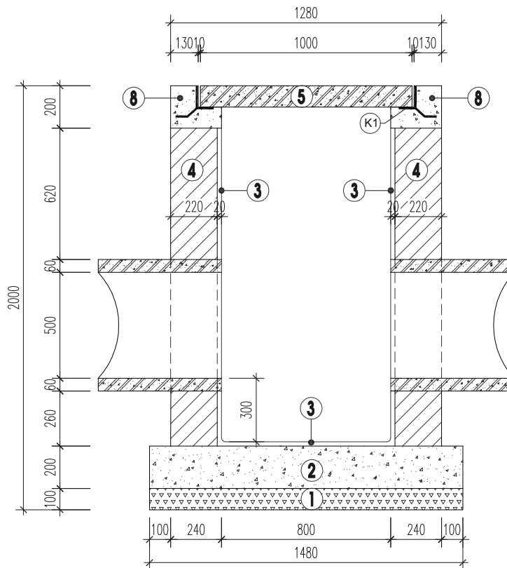
MẶT CẮT 2-2
