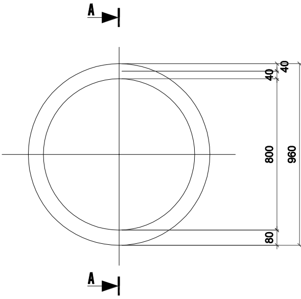
MẶT CẮT I-I (SECTION I-I)
