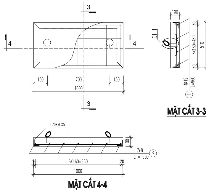
CẤU TẠO TẤM ĐAN 5
