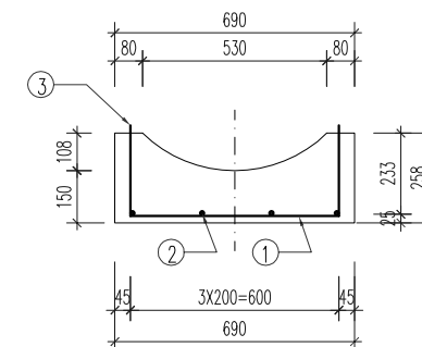
MẮT CẮT A-A
