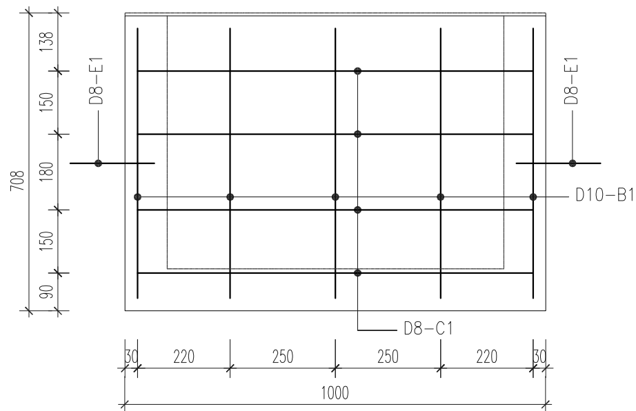
CHI TIẾT HỐ THU LOẠI 2
