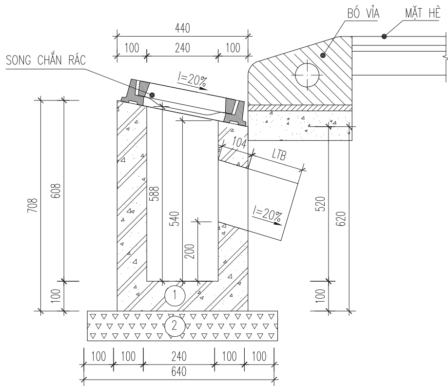
MẶT CẮT A-A
