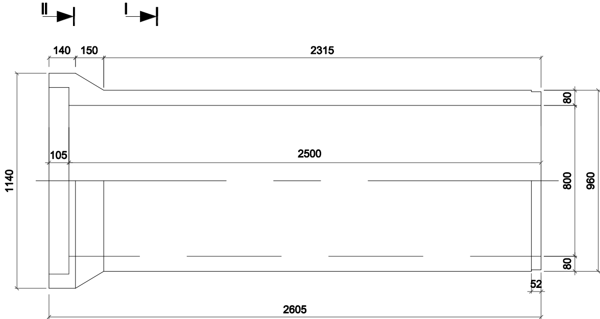
1/2 MẶT CẮT A-A (1/2 SECTION A-A)
