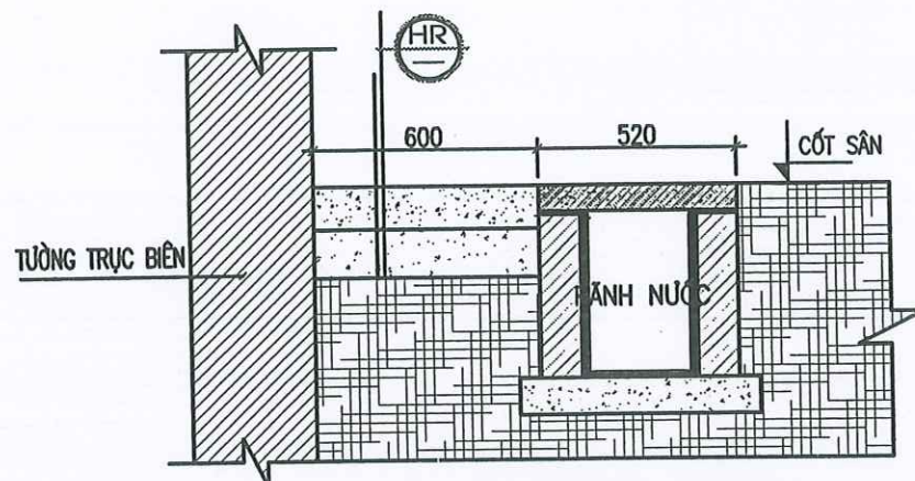
CHI TIẾT HÈ RÃNH QUANH NHÀ (S=34.0M2)
