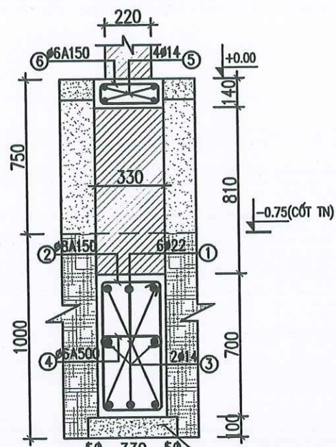
CẮT DẪM MÓNG ĐIỂN HÌNH
