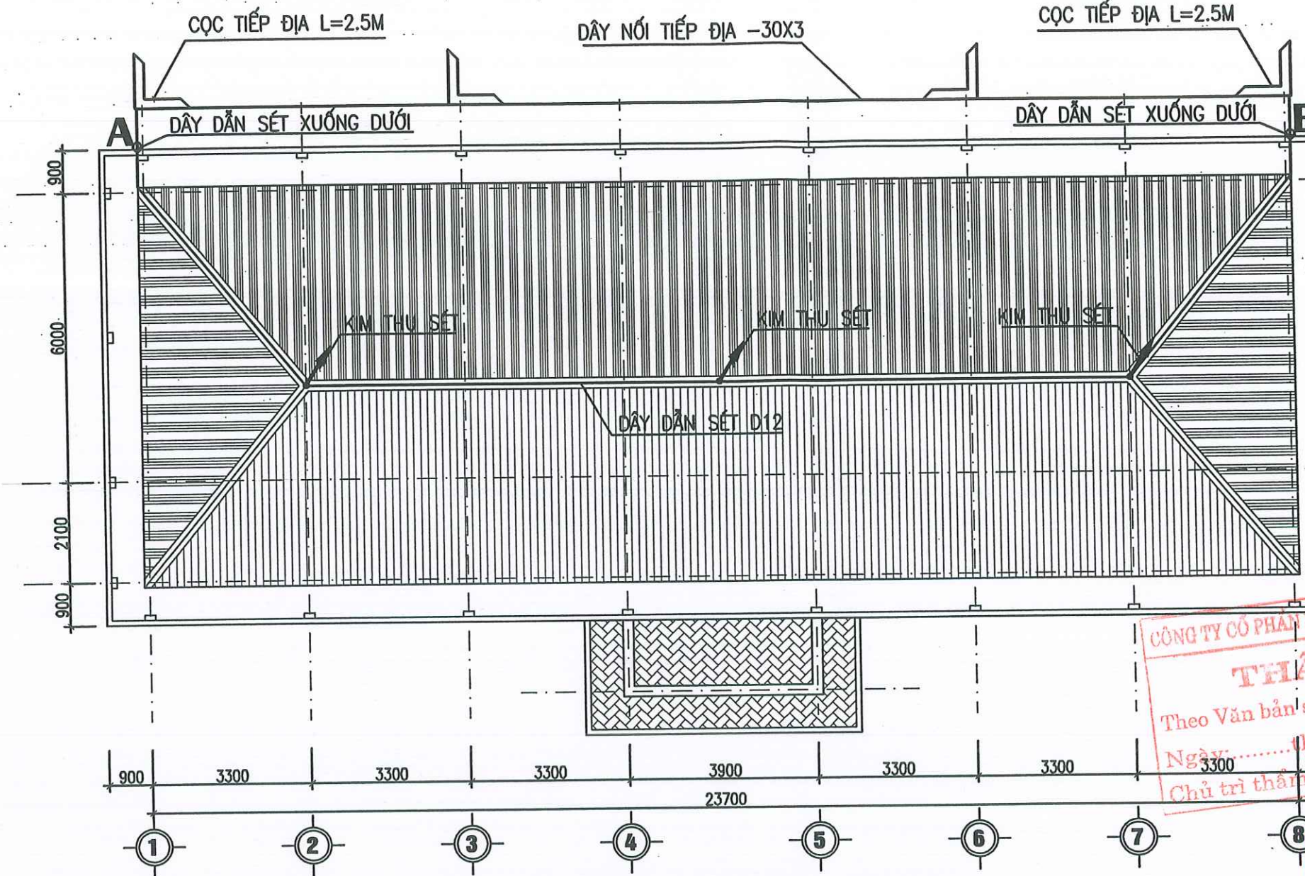
MẶT BẰNG CHỐNG SÉT MÁI
