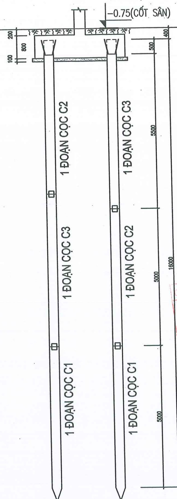
MẶT CẮT QUA ĐÀI CỌC (CỌC ĐẠI TRÀ)
