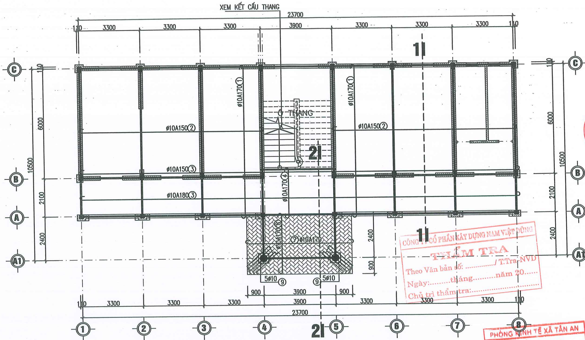
MẶT BẰNG THÉP SÀN MÁI TẦNG 1 (LỚP TRÊN)
