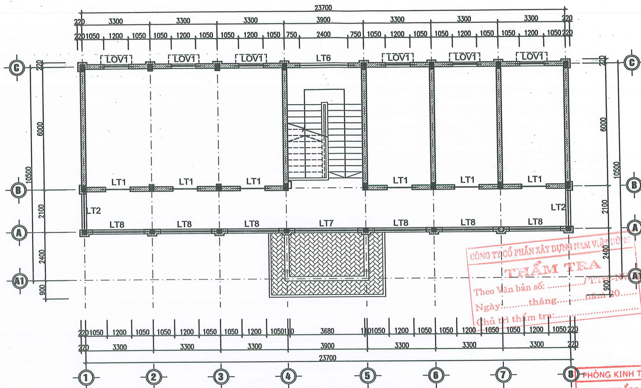
MẶT BẰNG LANH TÔ, Ô VĂNG TẦNG 2
