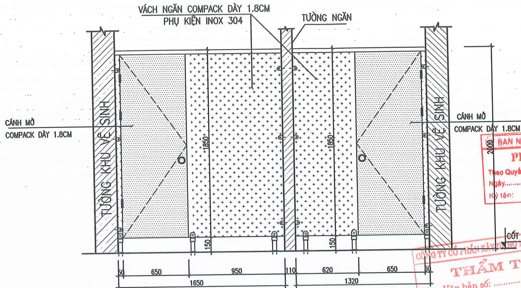
CHI TIẾT VÁCH NGĂN XÍ: 1 CÁI
