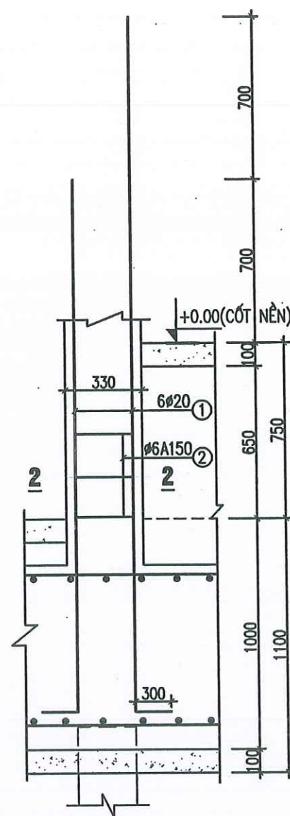
12 CỘT CỘT C2
