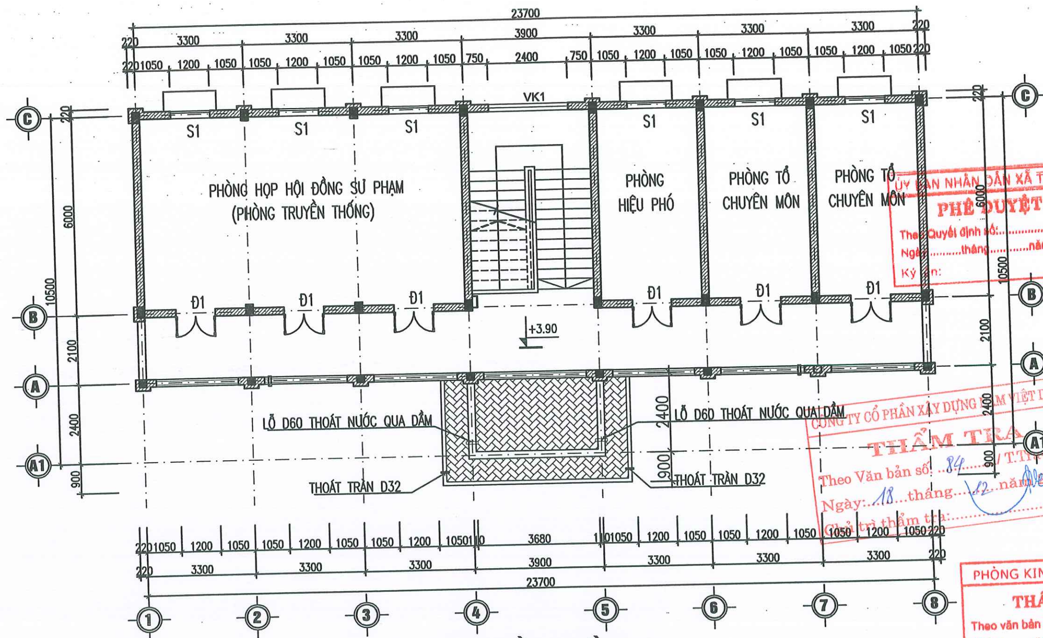
MẶT BẰNG TẦNG 2
