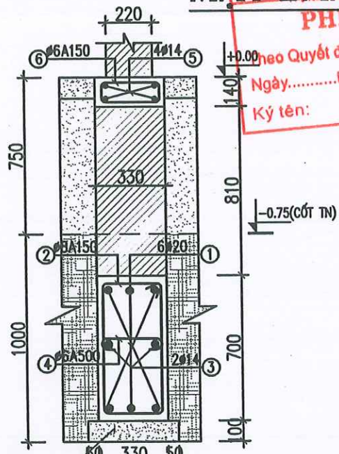
CẮT DẪM MÓNG TRỤC A, A1
