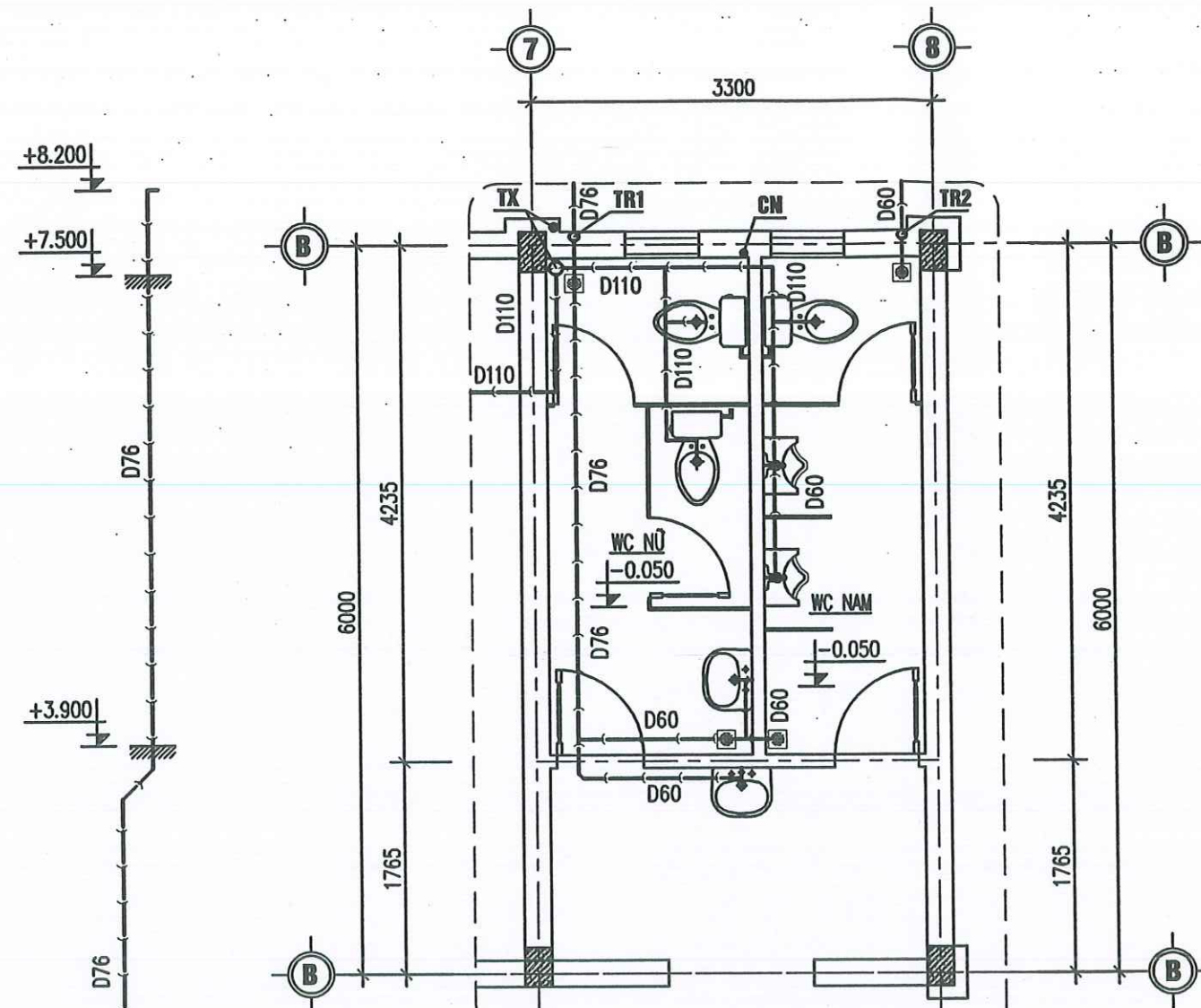
MẶT BẰNG CHI TIẾT THOÁT NƯỚC KHU WC
