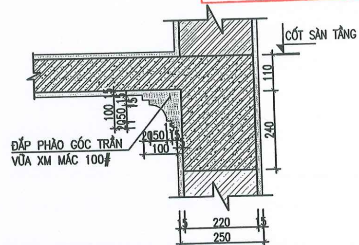
CHI TIẾT ĐẮP PHẪO GÓC TRẦN
