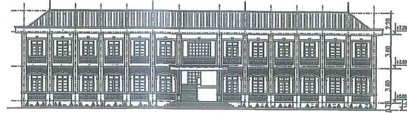
TRIỂN KHAI MẶT ĐÚNG CÔNG TRÌNH ĐẠI DIỆN
