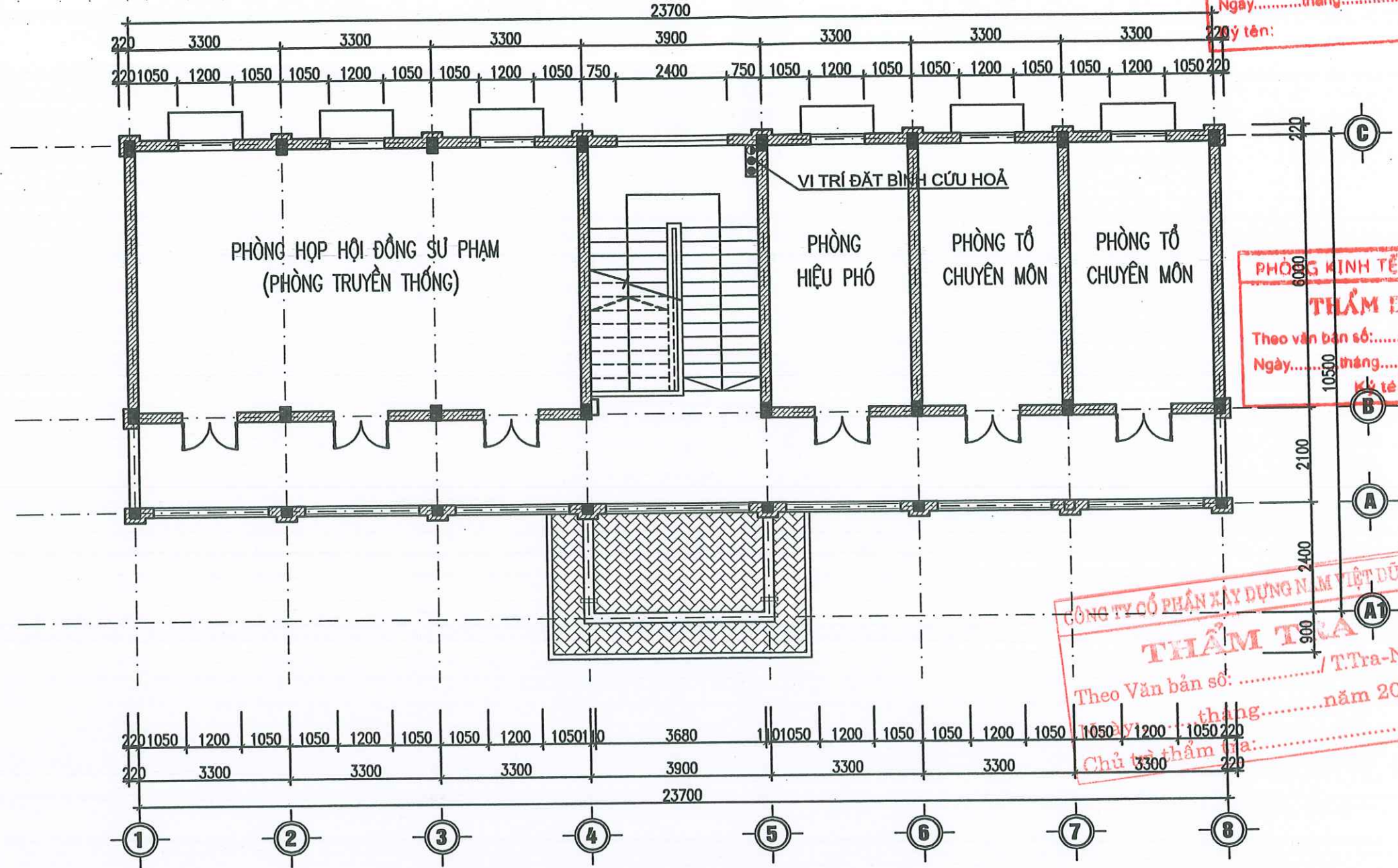
MẶT BẰNG CỨU HỎA TẦNG 2
