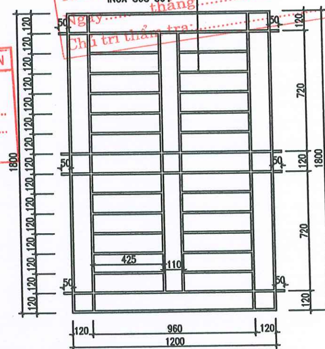
HOA SẮT CỬA SỔ S1: 11 BỘ (26.2M*0.57167KG=14.97KG/BỘ)
