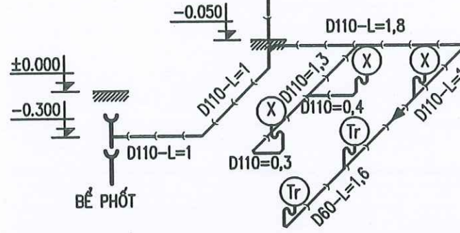
SƠ ĐỒ THOÁT NƯỚC XÍ, TIỂU WC
