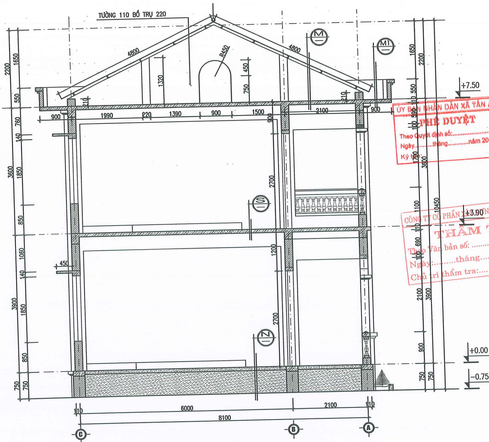
MẶT CẮT A-A
