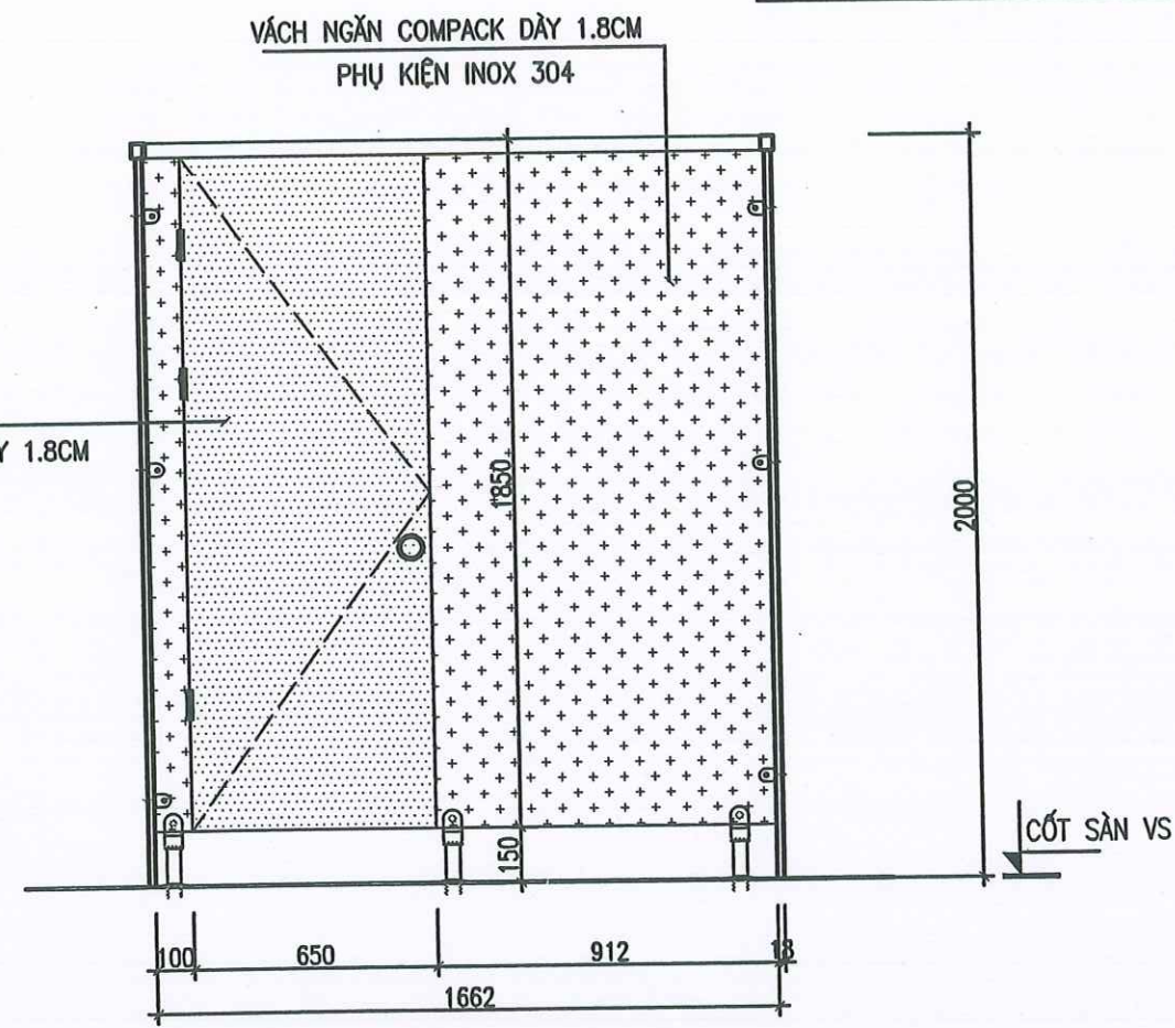
CHI TIẾT VÁCH NGĂN XÍ NỮ: 1 CÁI
