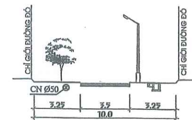
MẶT CẮT 1-1 ĐẠI DIỆN ĐƯỜNG XOM
