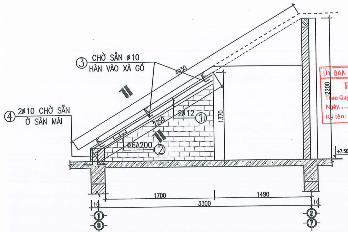
CHI TIẾT 4 TƯỜNG THU HỒI HAI ĐẦU HỒI - SL: 04
