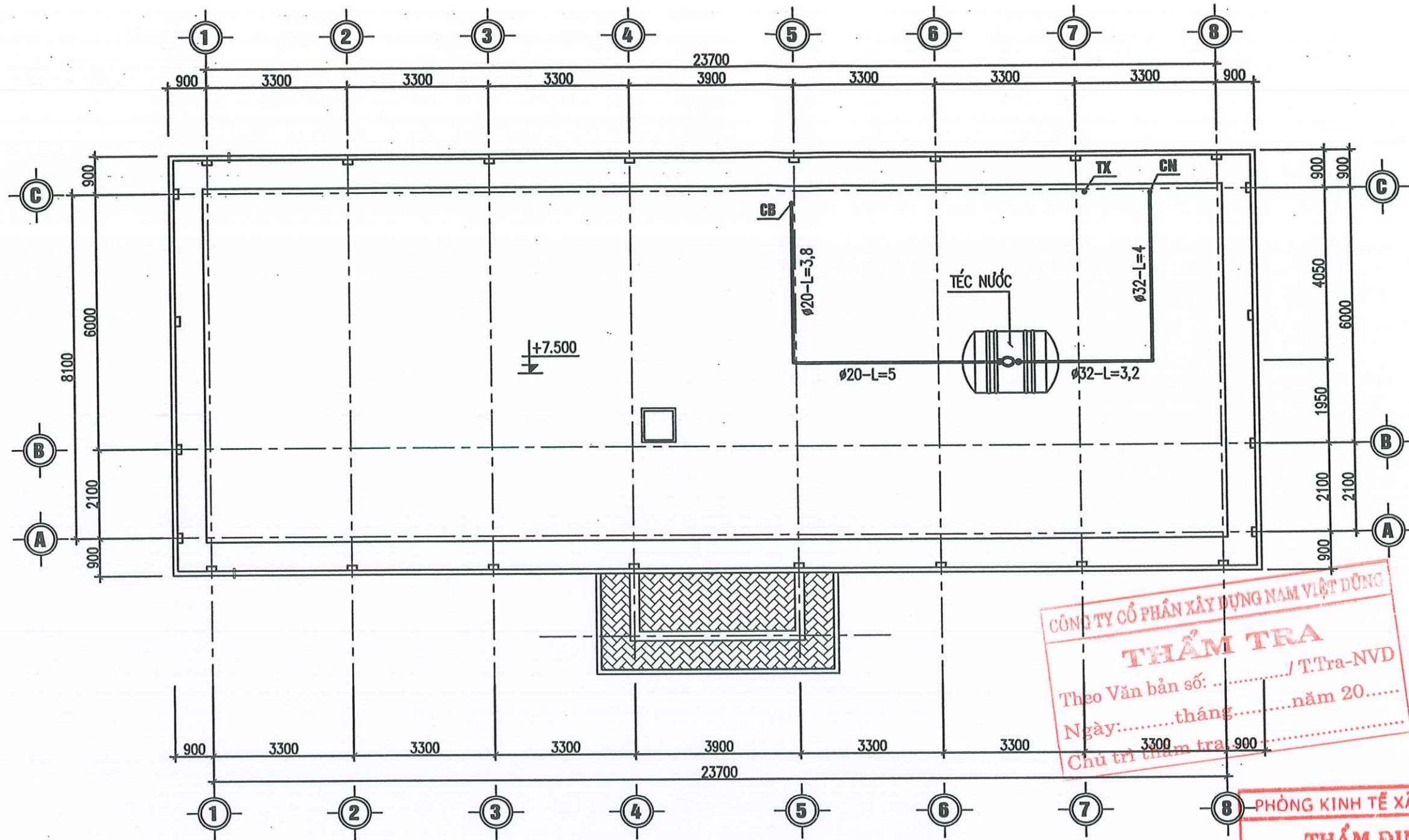
MẶT BẰNG CẤP THOÁT NƯỚC TẦNG ÁP MÁI
