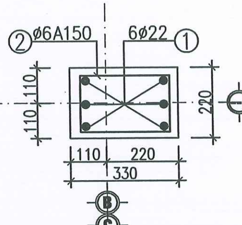
CẮT 2-2
