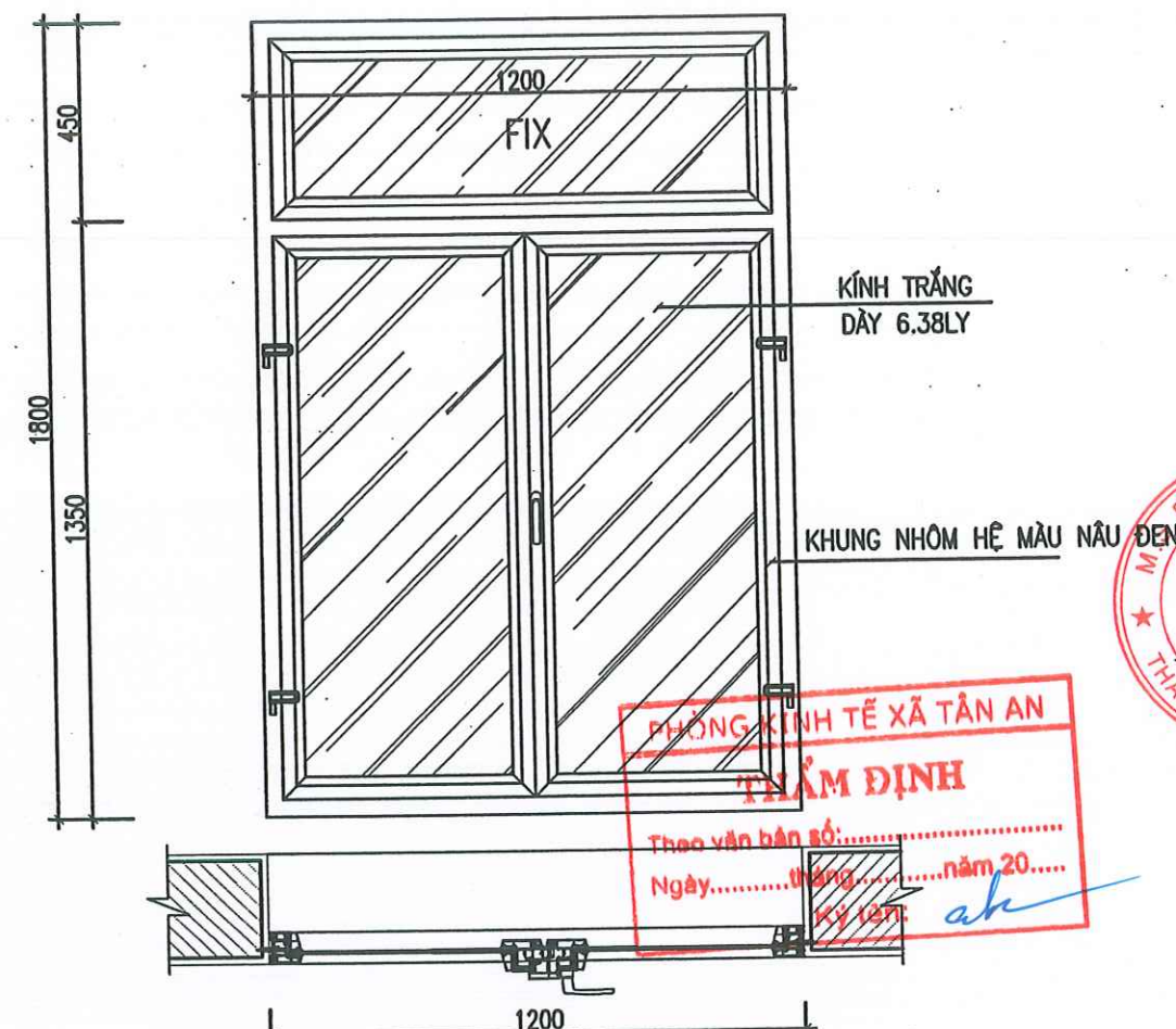
CỬA SỔ S1 (1200X1800) - 11 BỘ CỬA NHÔM HỆ CẢNH MỞ QUAY
