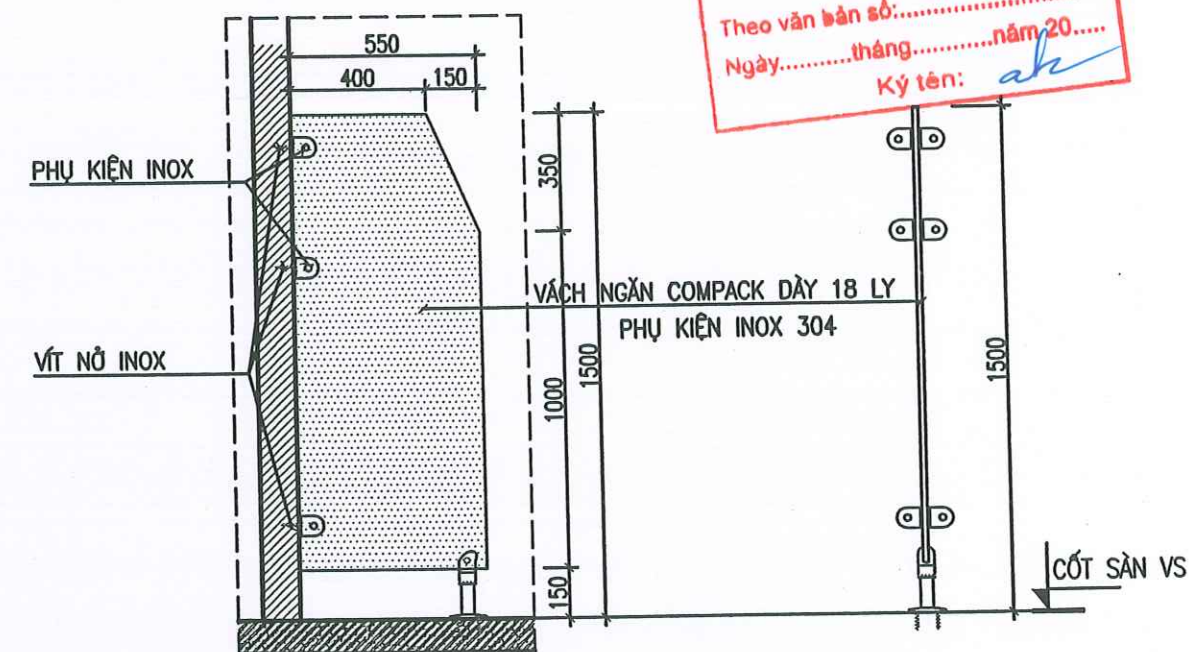
CHI TIẾT VÁCH NGĂN TIỂU NAM: 2 CÁI PHỤ KIỆN INOX 304
