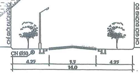
MẶT CẮT 2-2 ĐẠI DIỆN ĐƯỜNG THÔNG
