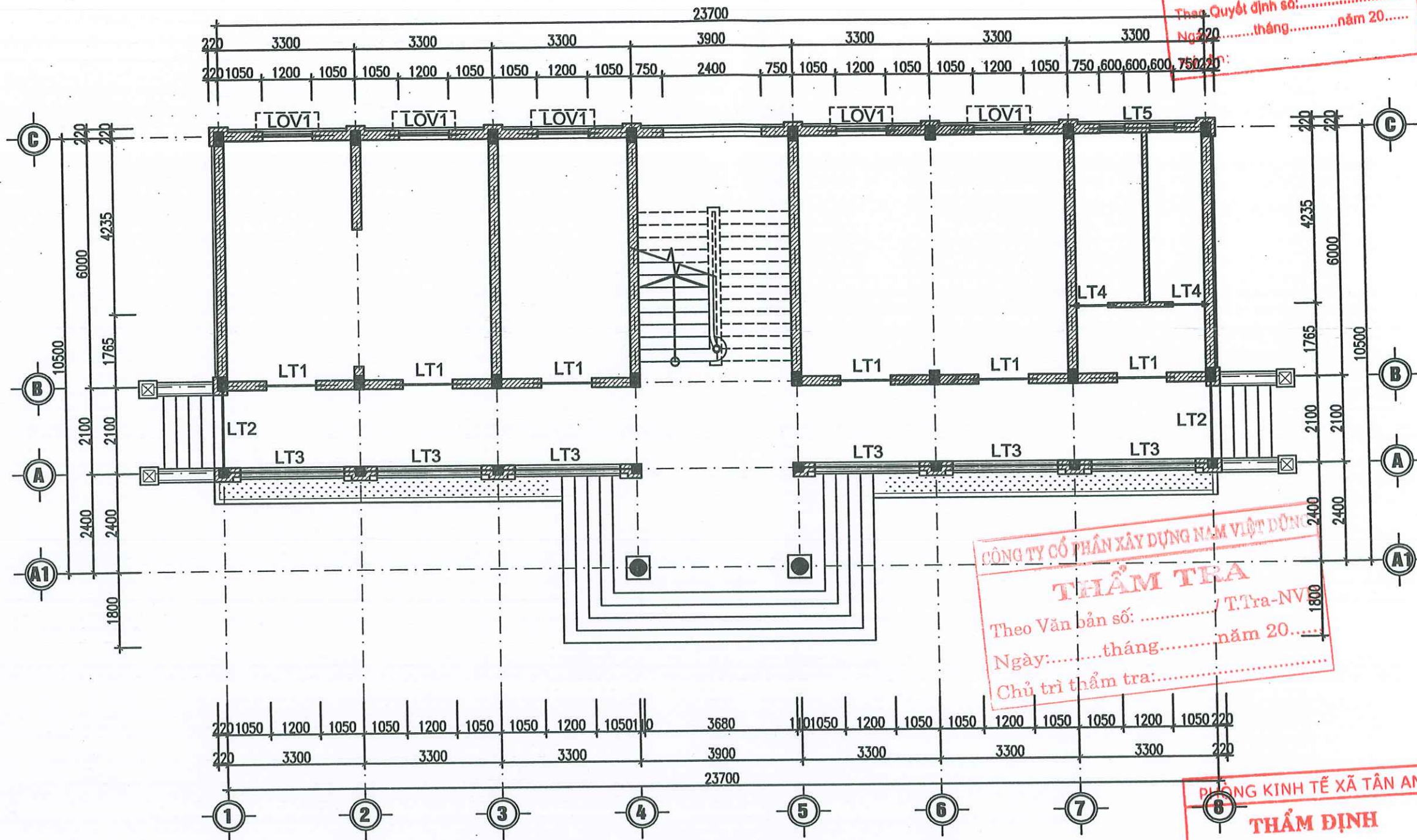
MẶT BẰNG LANH TÔ, Ô VĂNG TẦNG 1
