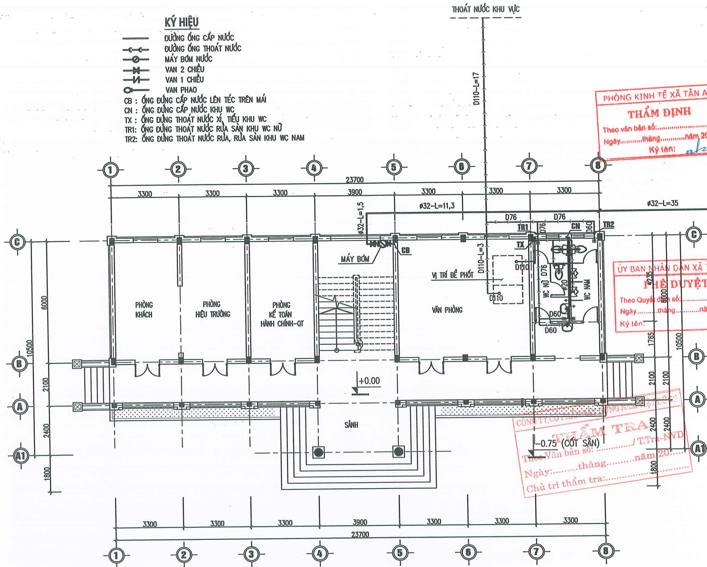
MẶT BẰNG CẤP THOÁT NƯỚC TẦNG 1
