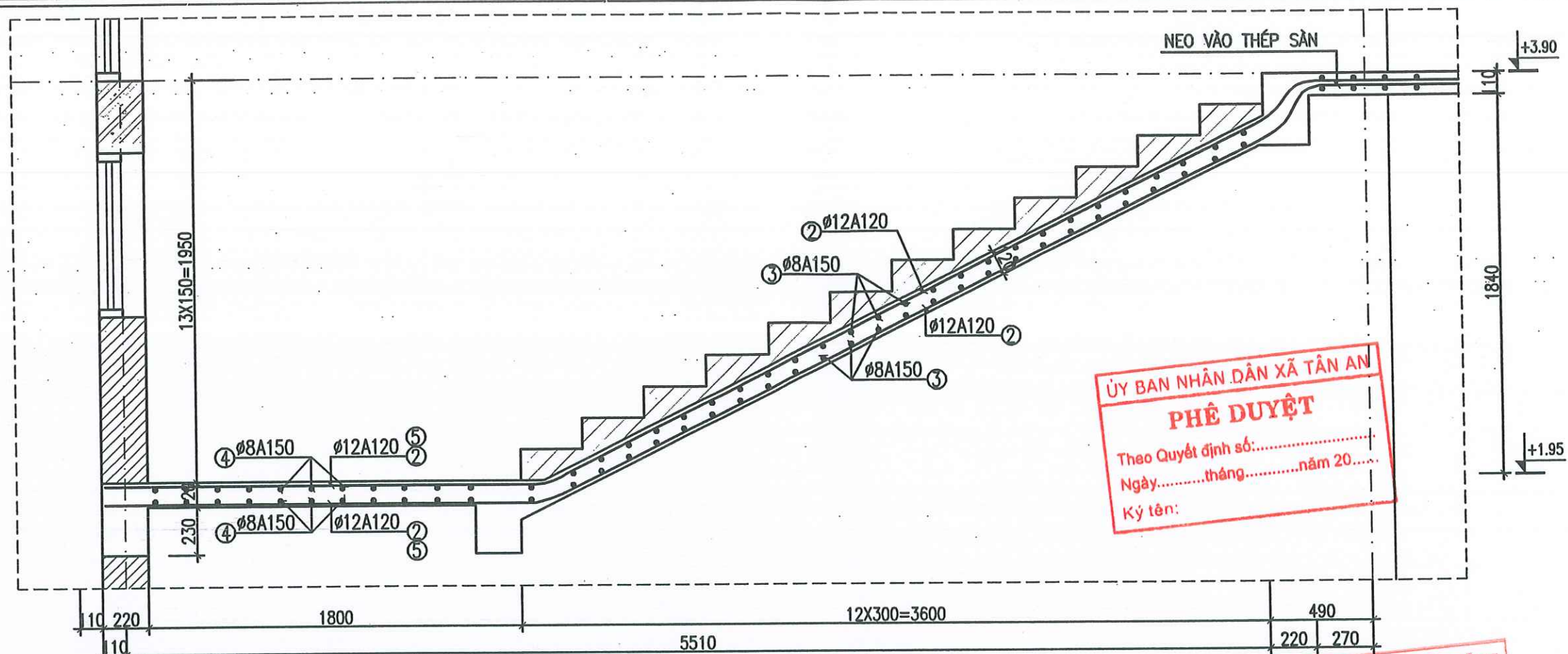
CẮT B-B CHI TIẾT THANG
