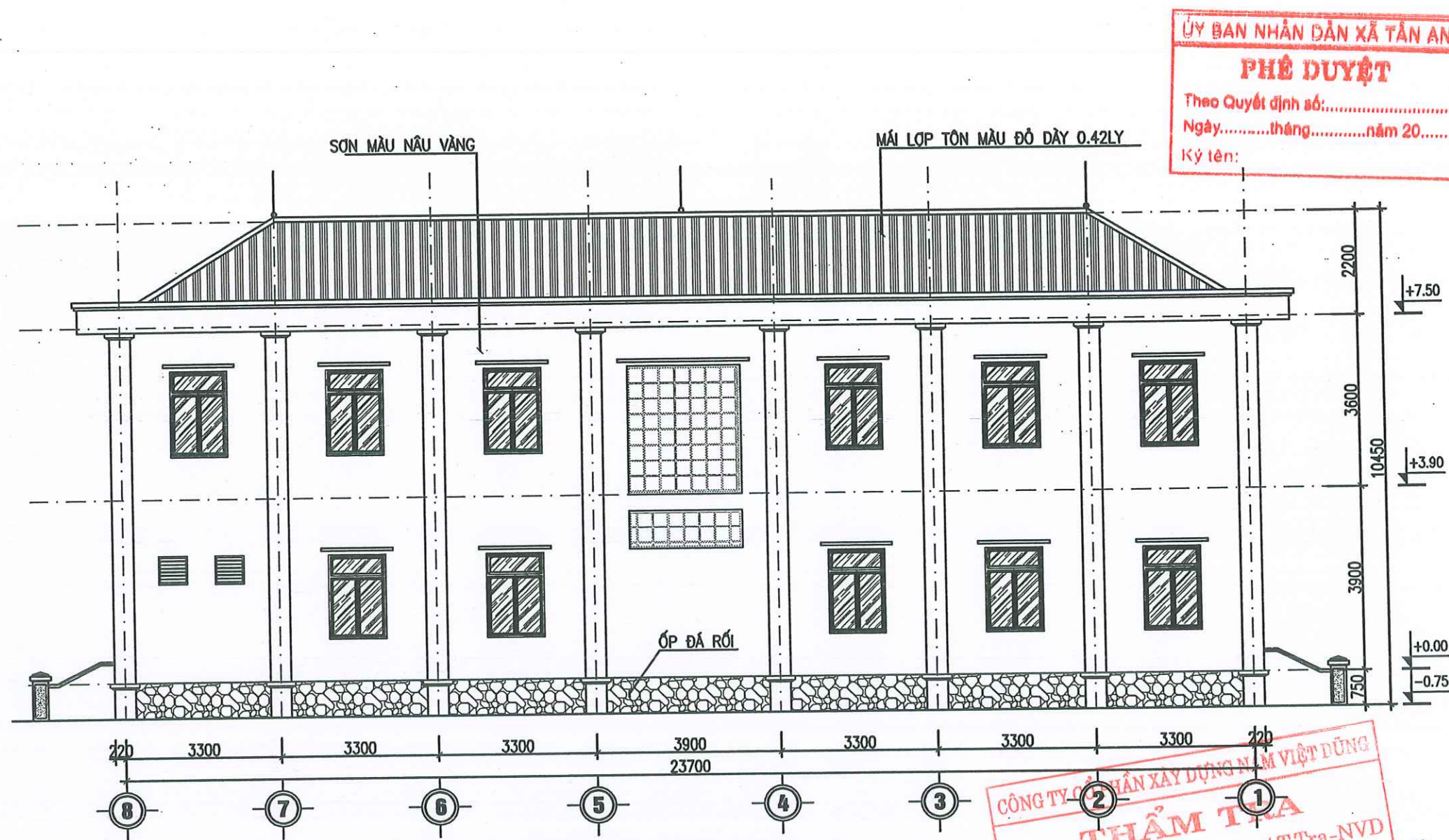
MẶT ĐÚNG TRỤC 8-1
