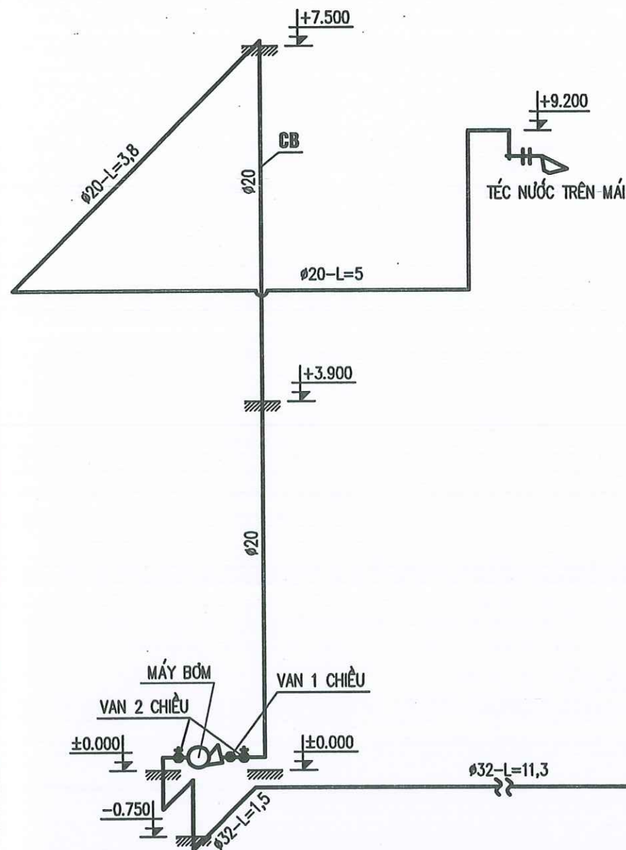
SƠ ĐỒ CẤP NƯỚC LÊN TẾC TRÊN MÁI
