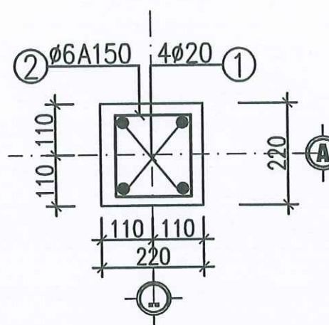
CẮT 1-1
