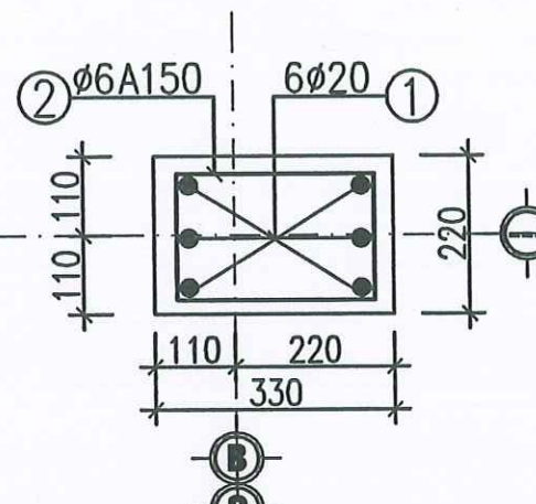
CẮT 2-2
