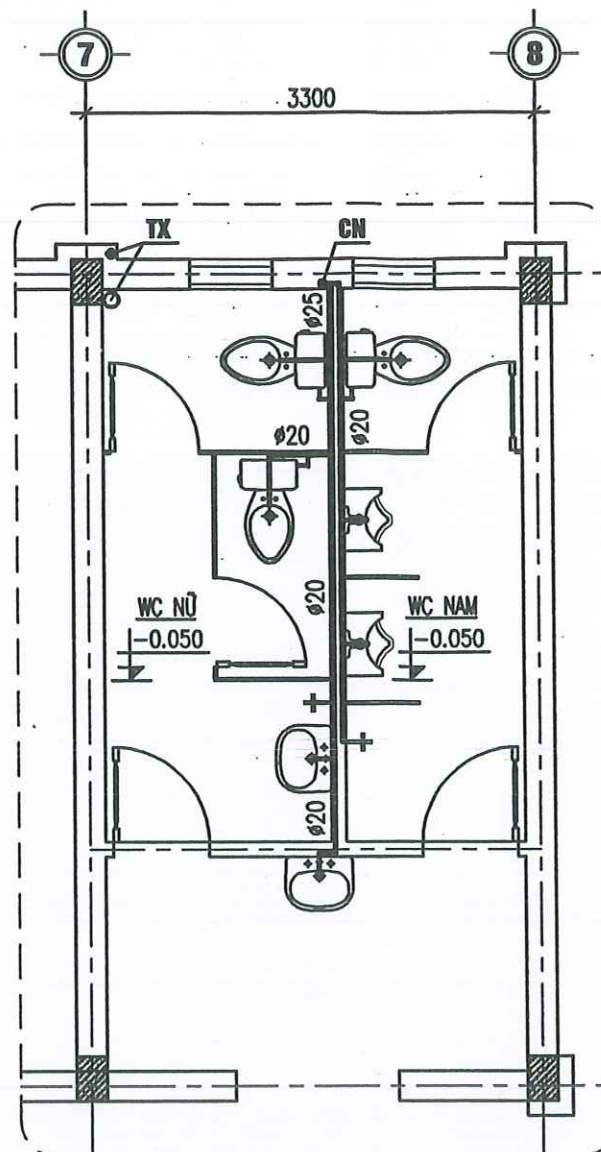
MẶT BẰNG CHI TIẾT CẤP NƯỚC KHU WC
