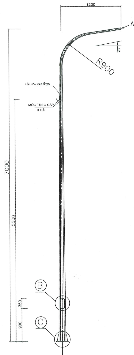
CỘT THÉP BÁT GIÁC CON CÁN ĐƠN CAO 7M
