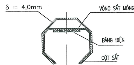
CẮT D-D
