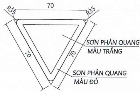
BIỂN SỐ W.208 TỈ LỆ : 1/20 (GIAO NHAU ĐƯỜNG ƯU TIÊN)
