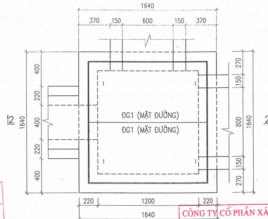
MẶT BẰNG HỒ GA B600 ĐẠN ĐG1 (DƯỚI MẶT ĐƯỜNG) 1 GA: G13
