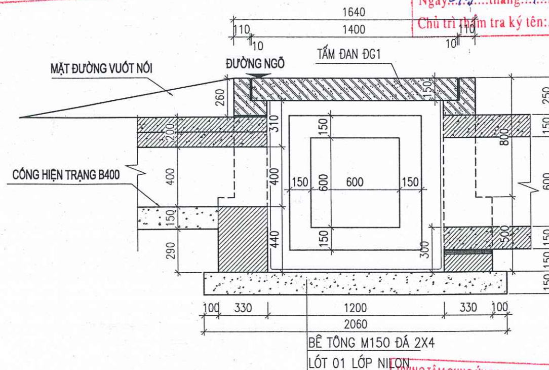
MẶT CẮT 2-2
