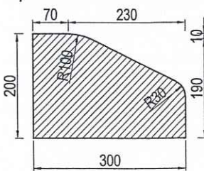
CẤU TẠO VIÊN VỈA 20X30X100
