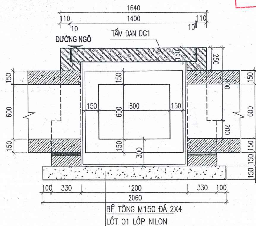
MẶT CẮT 1-1
