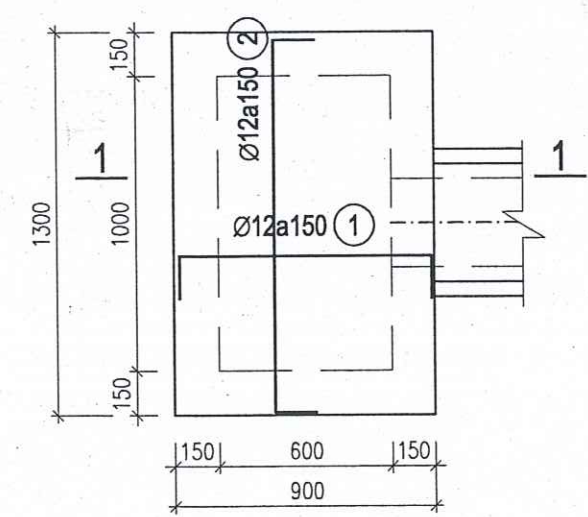
MẶT BẰNG THÉP ĐÁY HỐ THU GT1
