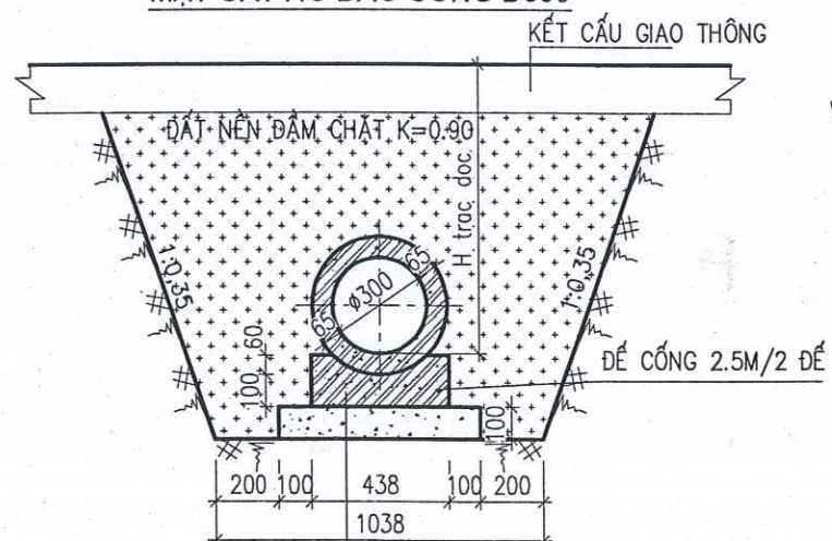
MẶT CẮT HỒ ĐÀO CỐNG D300
