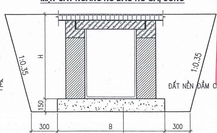
MẶT CẮT NGANG HỒ ĐÀO HỒ GA, CỐNG
