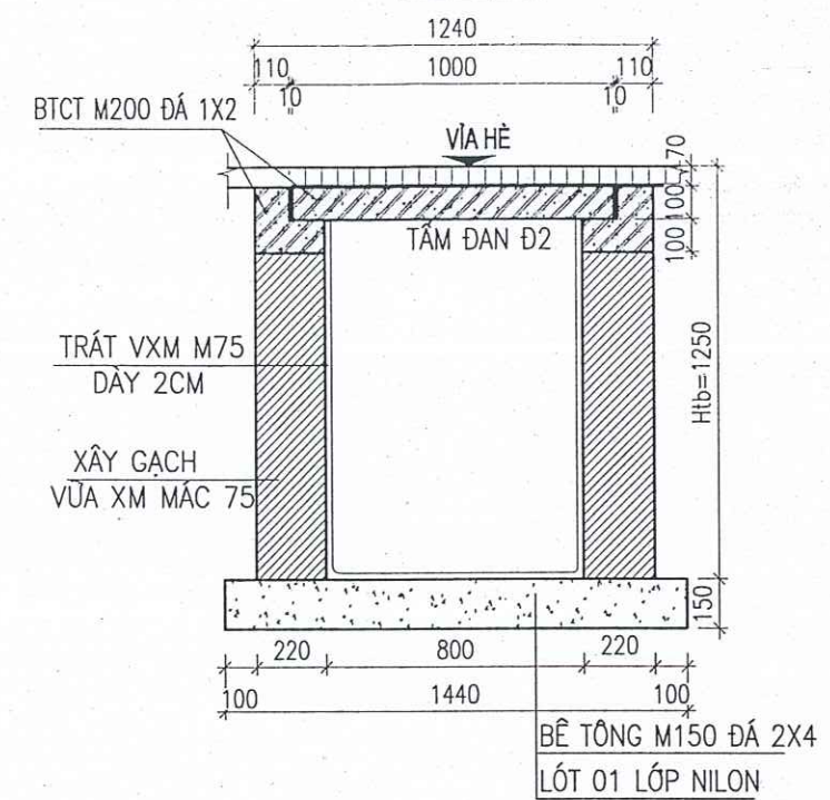
MẶT CẮT NGANG CÔNG B800 (DƯỚI VÍA HÈ)
