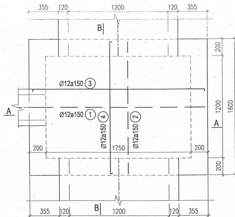
MẶT BẰNG THÉP ĐÁY HỐ GA TỪ G17 ĐẾN G22
