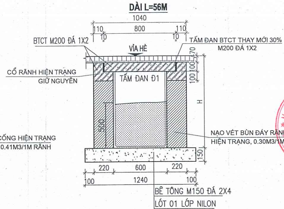
MẶT CẮT NGANG CỐNG B600 HIỆN TRẠNG
