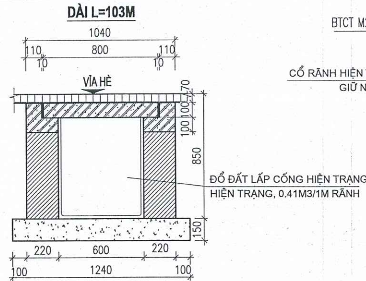
MẶT CẮT NGANG CỐNG HIỆN TRẠNG B600
