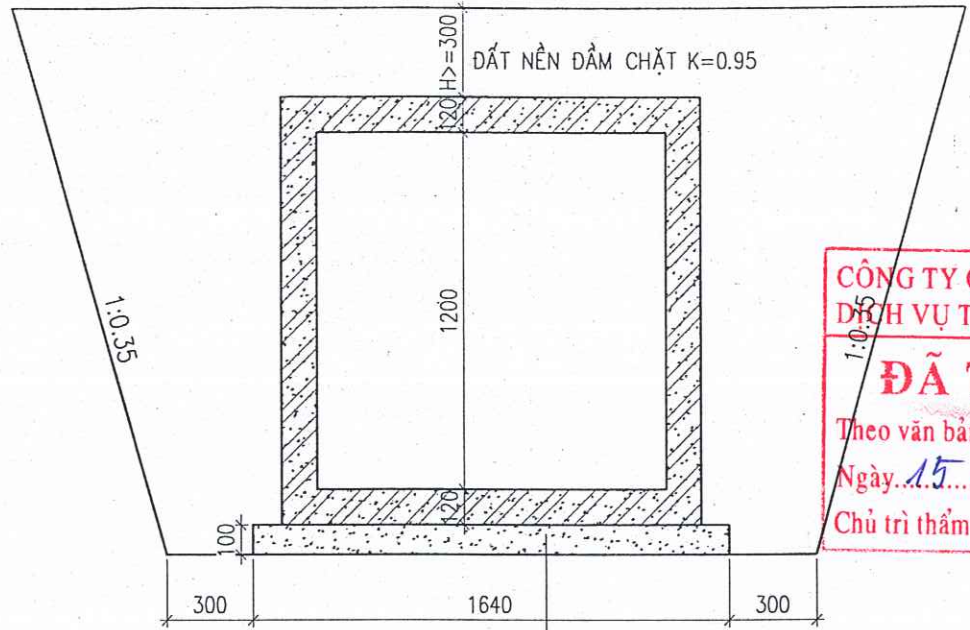
MẶT CẮT HỒ ĐÀO CỐNG BXH=1.2X1.2M (DÀI L = 107M)
