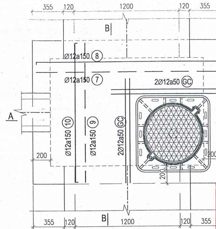
MẶT BẰNG THÉP NẮP HỐ GA TỪ G17 ĐẾN G22
