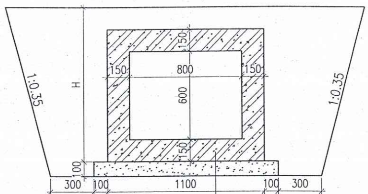
CÔNG HỘP BTCT BXH=0.8X0.6M ĐỒ TẠI CHỖ (DÀI L = 43M)
