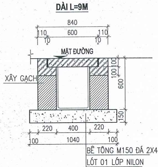
MẶT CẮT NGANG PHÁ DỠ CỐNG B400 (CỐNG HIỆN TRẠNG)
