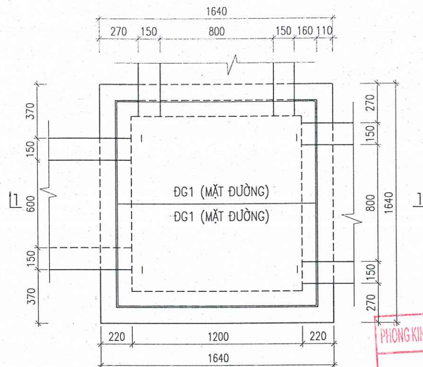
MẶT BẰNG HỒ GA B600 ĐẠN ĐG1 (DƯỚI MẶT ĐƯỜNG) 1 GA: G14
