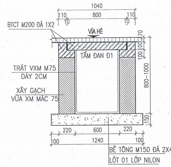
MẶT CẮT NGANG CÔNG B600 (DƯỚI VÍA HÈ)
