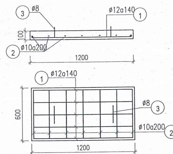
BỐ TRÍ THÉP TẤM ĐAN ĐG2 (DƯỚI HÈ) GIĂNG MIỆNG CÁC LOẠI HỐ GA CÓ KT: 1000X1000
