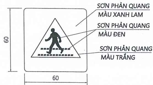
BIỂN SỐ I.423B TỈ LỆ : 1/20 (ĐƯỜNG ĐI BỘ SANG NGANG)
