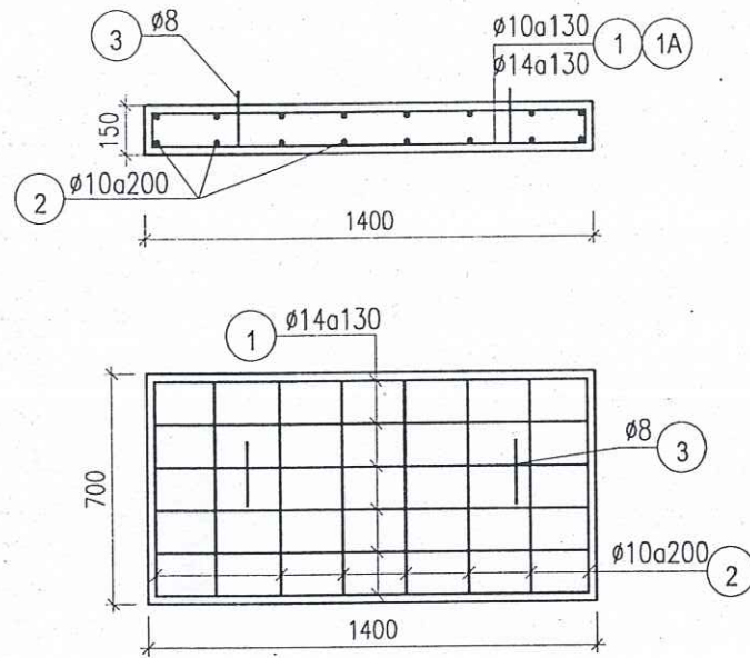
BỐ TRÍ THÉP TẤM ĐAN ĐG1 (DƯỚI MẶT ĐƯỜNG) GIĂNG MIỆNG CÁC LOẠI HỐ GA CÓ KT: 1200X1200
