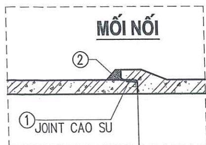
JOINT CAO SU
