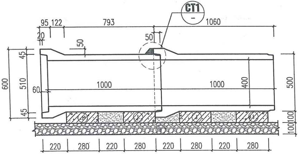
CÁI DỌC TUYẾN CỐNG D400 ĐIỂN HÌNH
