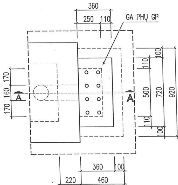
MẶT BẰNG GA
