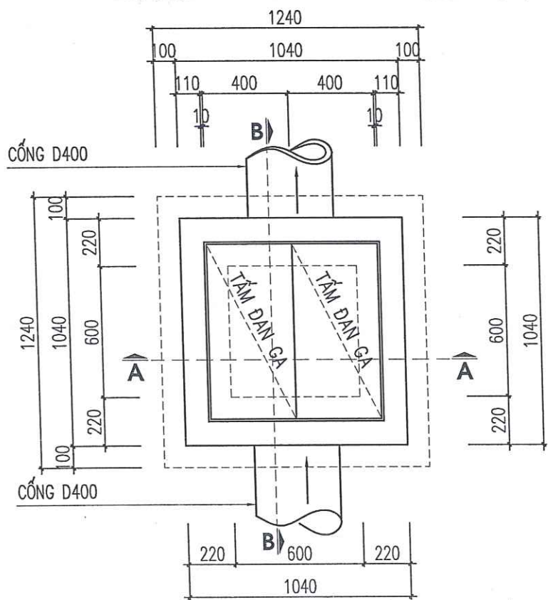
MẶT BẰNG GA
