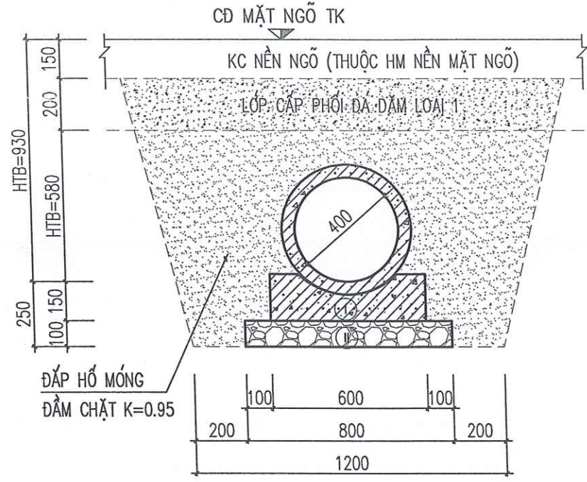
CHI TIẾT LẮP ĐẶT CỐNG D400
