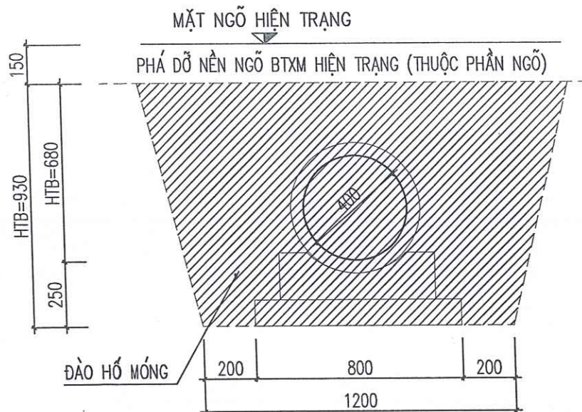
MẶT CẮT HỒ ĐÀO CỐNG D400
