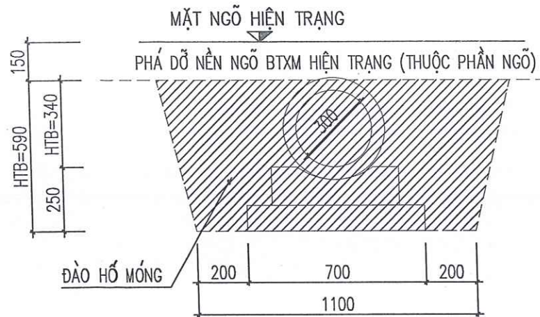
MẶT CẮT HỐ ĐÀO CỐNG D300
