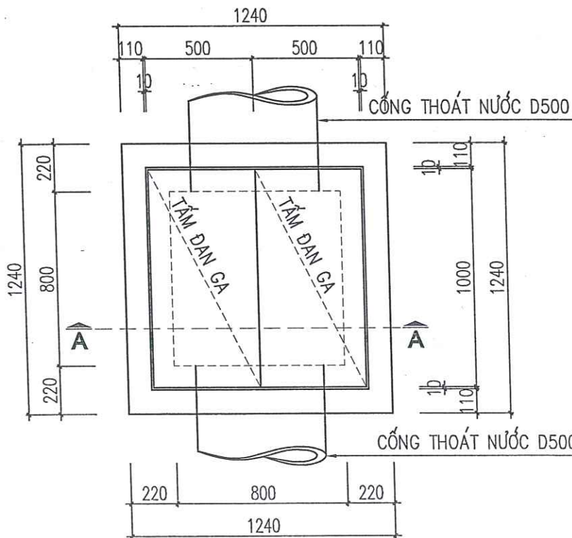
MẶT BẰNG GA (HIỆN TRẠNG)
