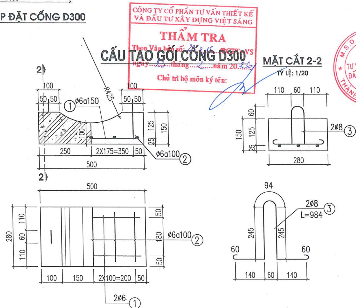
BẢNG THỐNG KÊ VẬT LIỆU CHO 01 GỐI CỔNG D300
