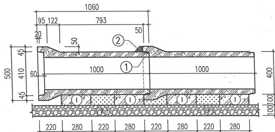
CẮT DỌC TUYẾN CỐNG D300 ĐIỂN HÌNH
