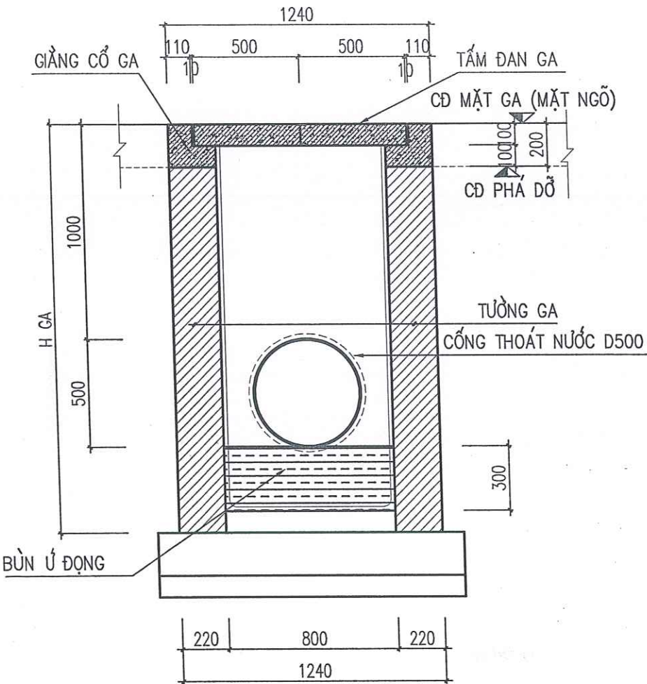
MẶT CẮT A-A
