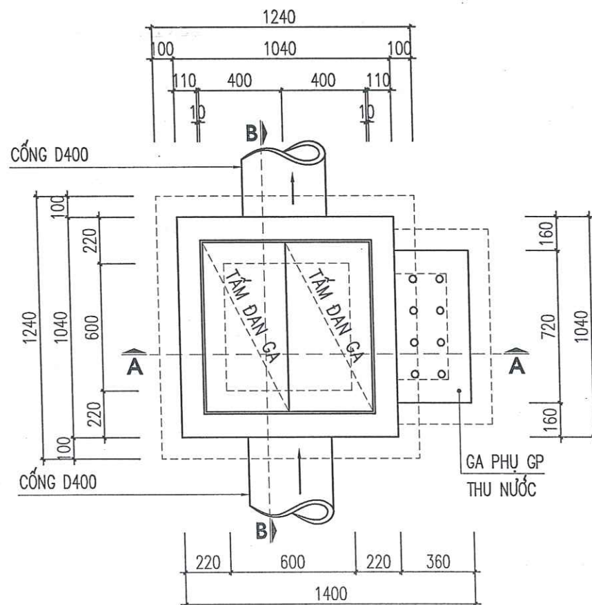
MẶT BẰNG GA
