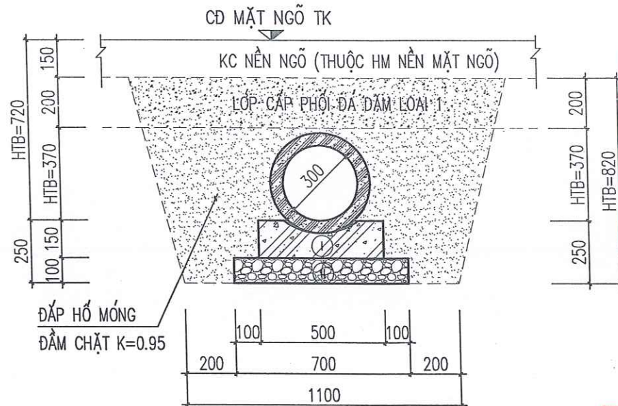
CHI TIẾT LẮP ĐẶT CỐNG D300
