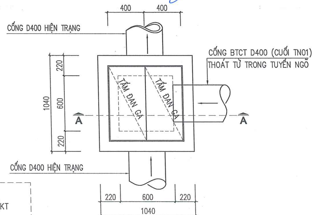
MẶT BẰNG GA (CẢI TẠO)
