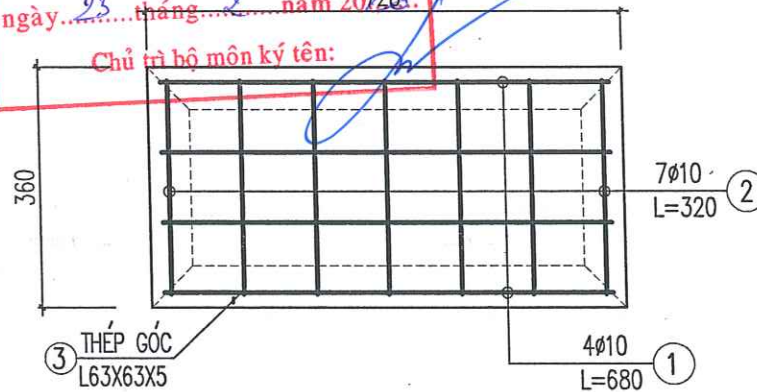
CẦU TẠO CỐT THÉP TẤM ĐAN A
