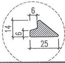
JOINT CAO SU
