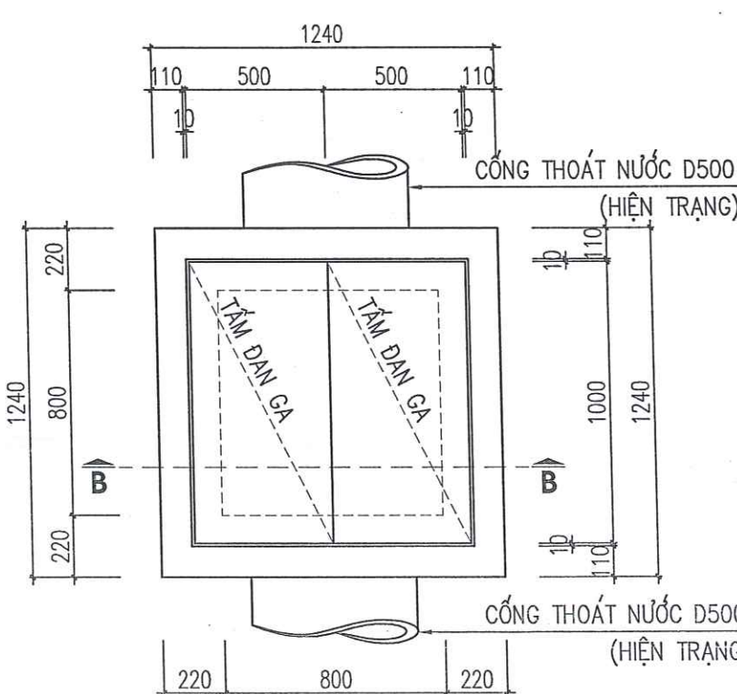
MẶT BẰNG GA (CẢI TẠO)
