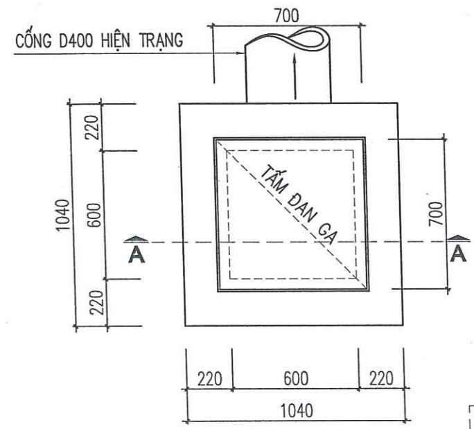
MẶT BẰNG GA (HIỆN TRẠNG)
