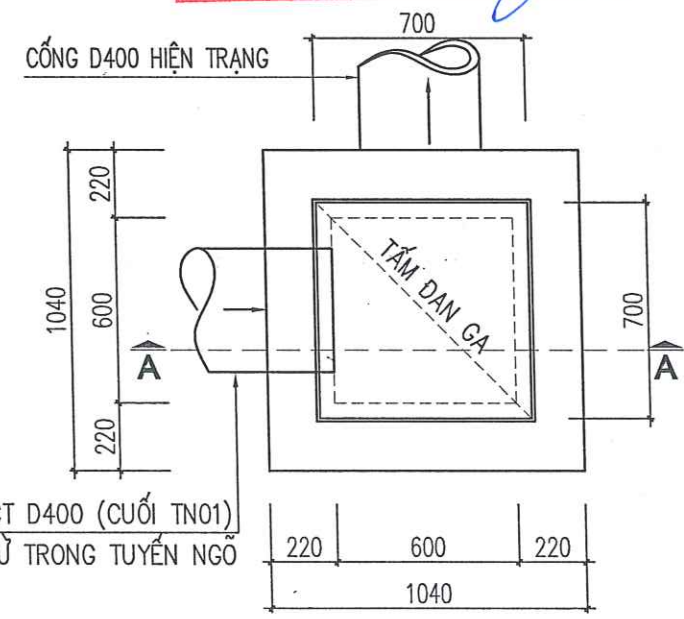
MẶT BẰNG GA (CẢI TẠO)
