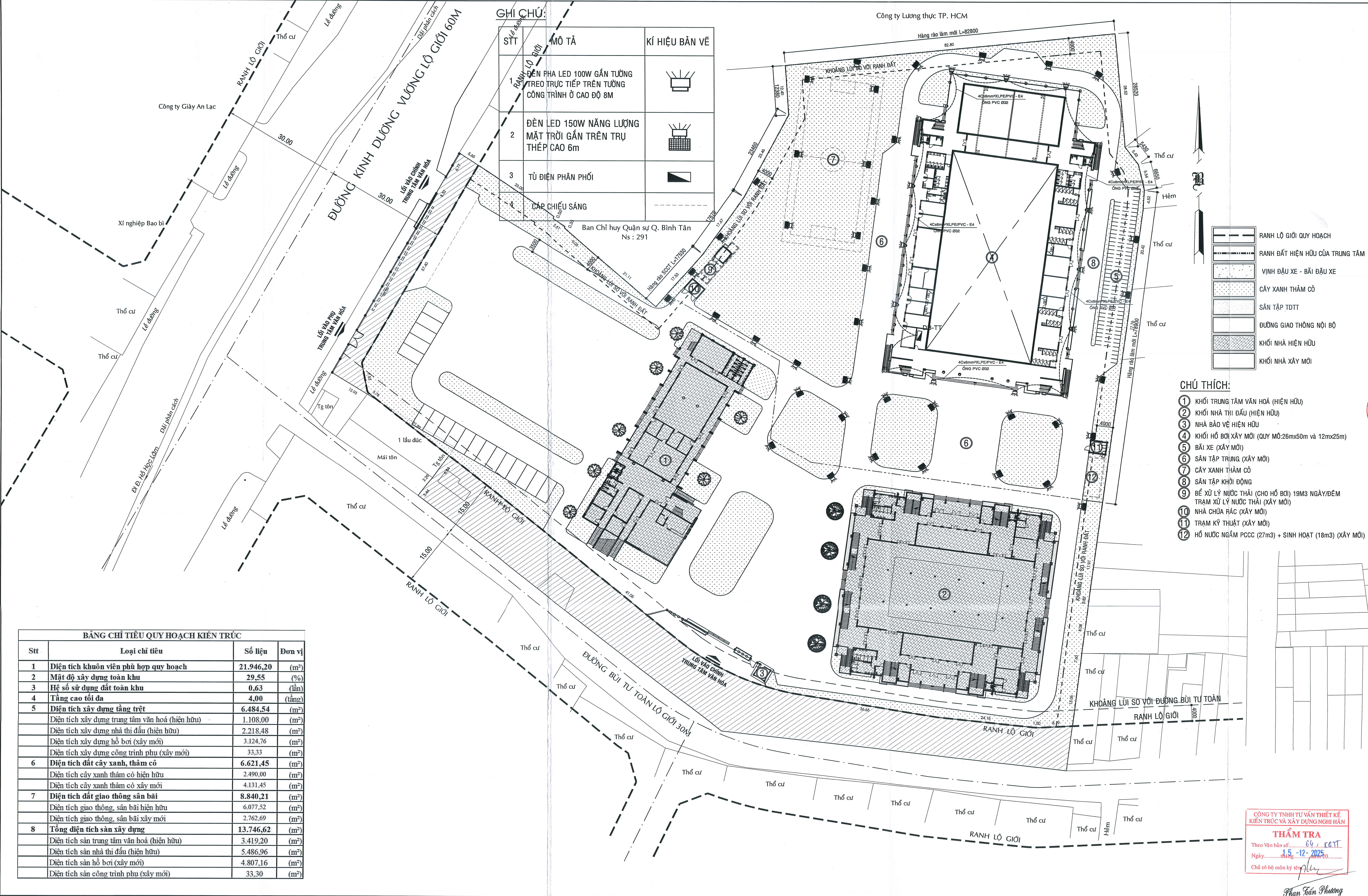
MẶT BẰNG TỔNG THỂ HỒ BƠI TL 1/400
