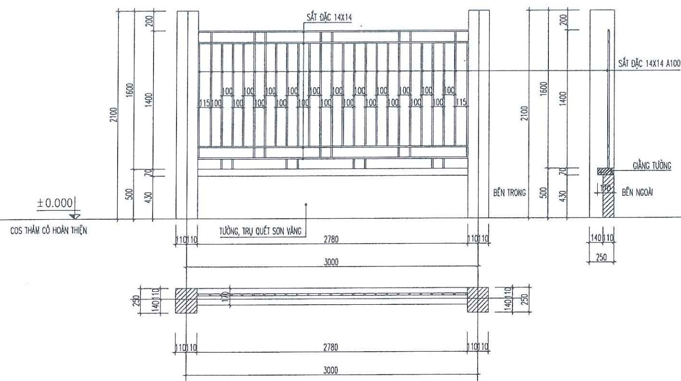
TƯỜNG RÀO THOÁNG ĐOẠN 1-2 BƯỚC 3000
