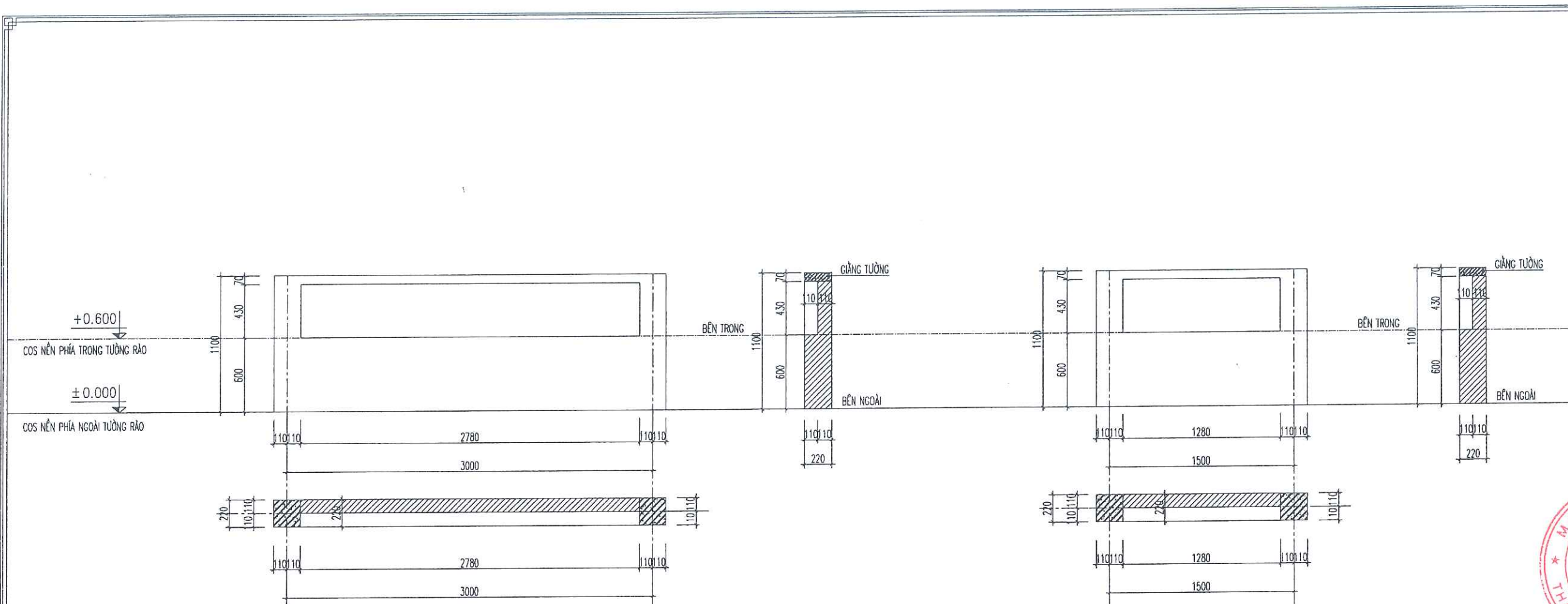
TƯỜNG RÀO ĐOẠN 4-5 BƯỚC 1500 ( SỐ LƯỢNG: 01 CK )
