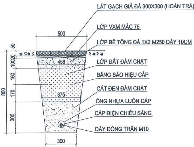
MẶT CẮT Rãnh CÁP TRÊN HỀ (LOẠI 1)
