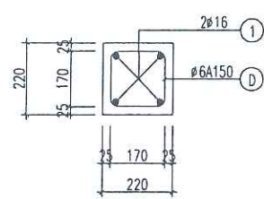
MẶT CẮT 1-1
