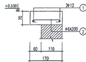
GIẢNG TƯỜNG RÀO LOẠI 1
