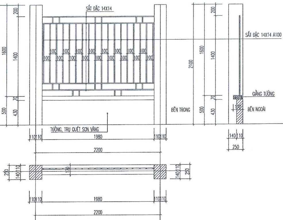
TƯỜNG RÀO THOÁNG ĐOẠN 1-2 BƯỚC 2200
