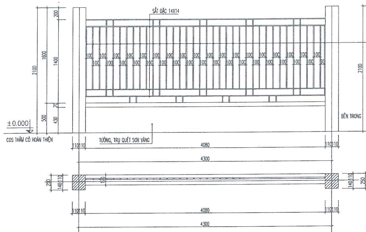
TƯỜNG RÀO THOÁNG ĐOẠN 4-5 BƯỚC 4300
