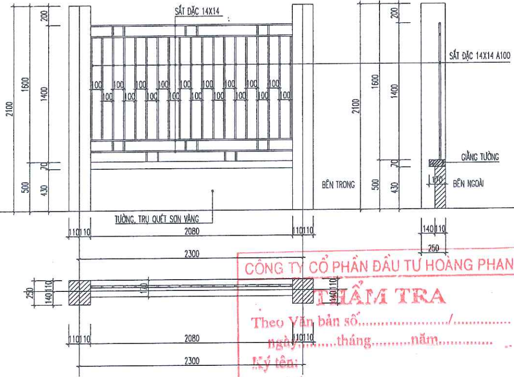
TƯỜNG RÀO THOÁNG ĐOẠN 6-7 BƯỚC 2300
