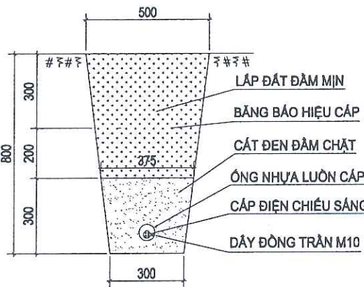
MẶT CẮT Rãnh CÁP NỀN ĐẤT (LOẠI 1)
