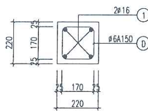
MẶT CẮT 1-1
