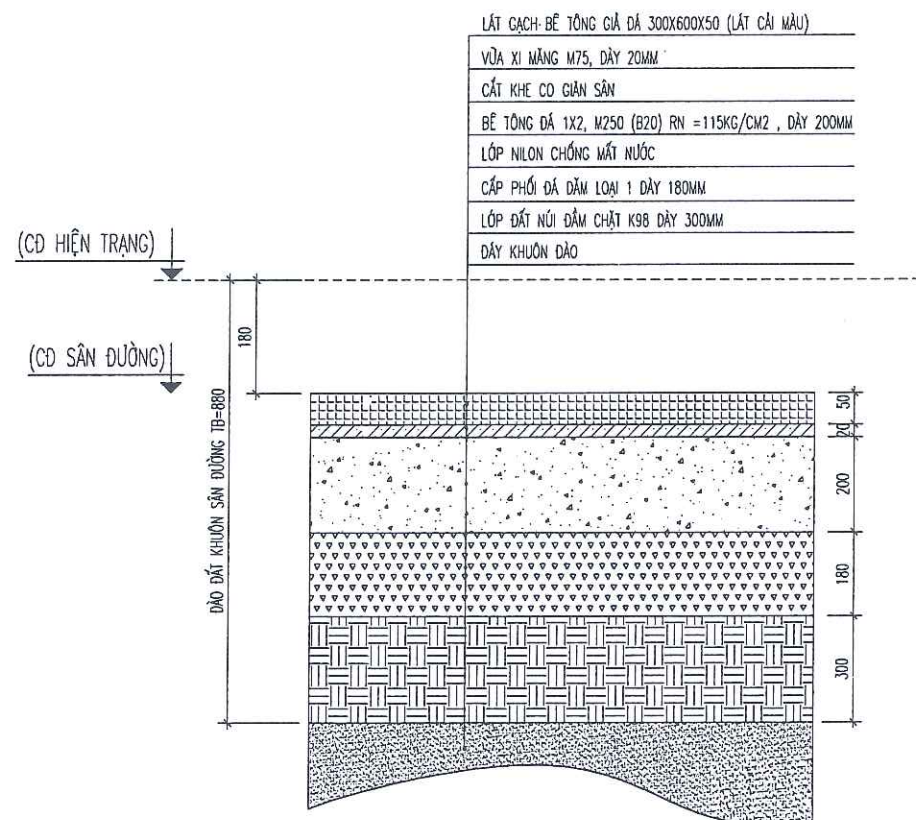
KẾT CẤU NỀN SÂN ĐƯỜNG - Ô A42
