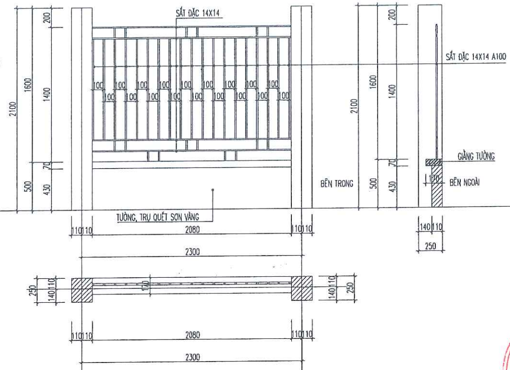
TƯỜNG RÀO THOÁNG ĐOẠN 5-6 BƯỚC 2300
