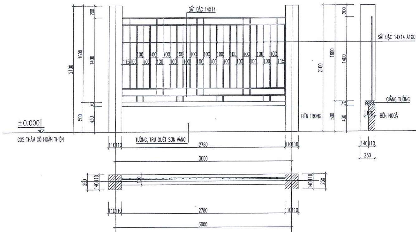
TƯỜNG RÀO THOÁNG ĐOẠN 6-7 BƯỚC 3000
