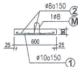
MẶT CẮT 1 - 1
