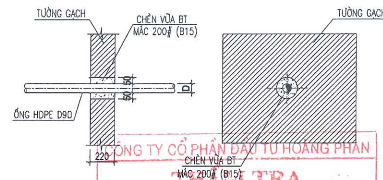
CHI TIẾT ỐNG QUA TƯỜNG
