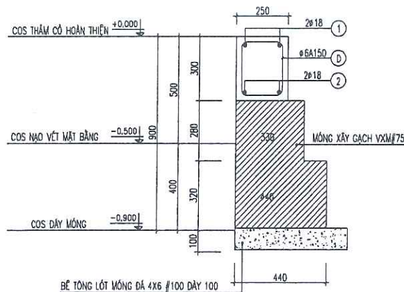
MÓNG TƯỜNG RÀO LOẠI 1
