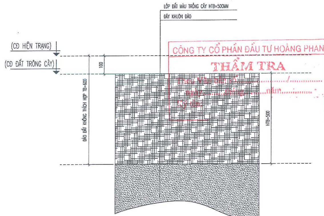
KẾT CẤU ĐẤT TRỒNG CÂY THÂM CỎ - Ô A42
