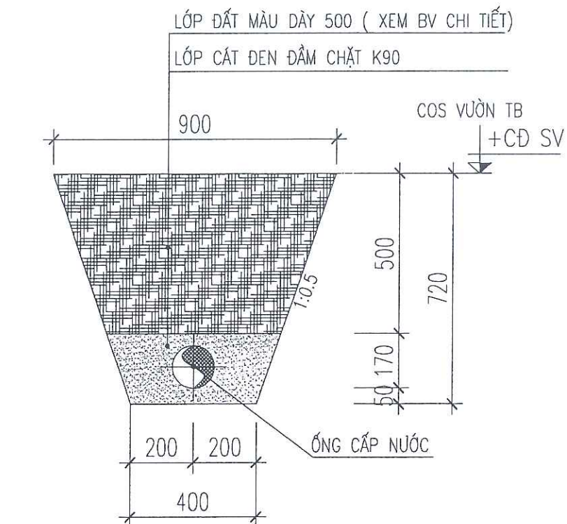
MẶT CẮT NGANG ĐIỂN HÌNH CHÔN ỐNG (SÂN VƯỜN: 57.67M)
