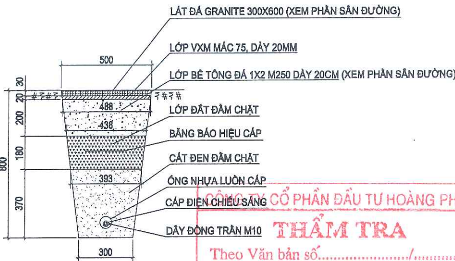
MẶT CẮT Rãnh CÁP TRÊN SÂN ĐƯỜNG (LOẠI 1)
