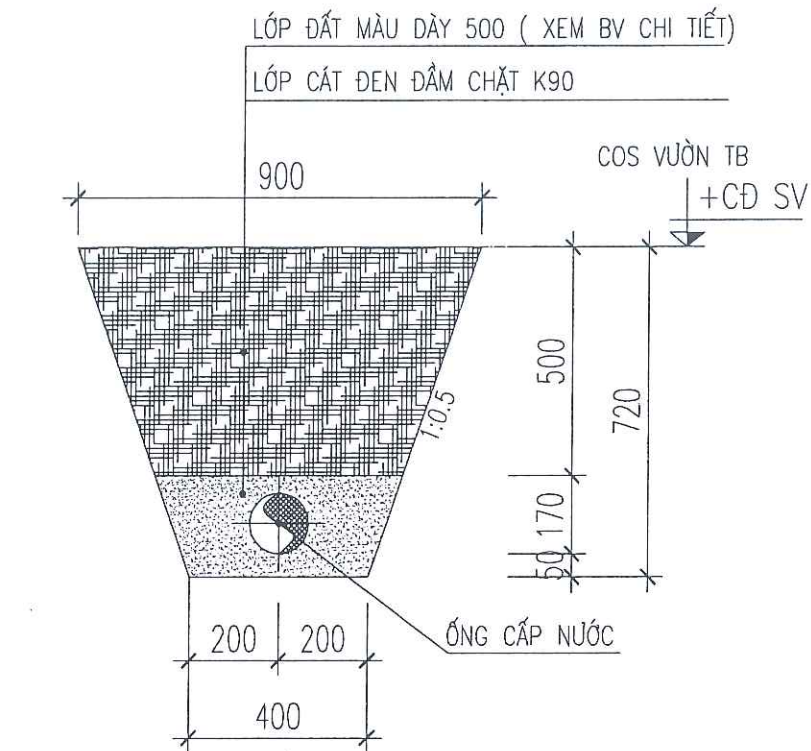
MẶT CẮT NGANG ĐIỂN HÌNH CHÔN ỚNG (SÂN VƯỜN: 59.7M)
