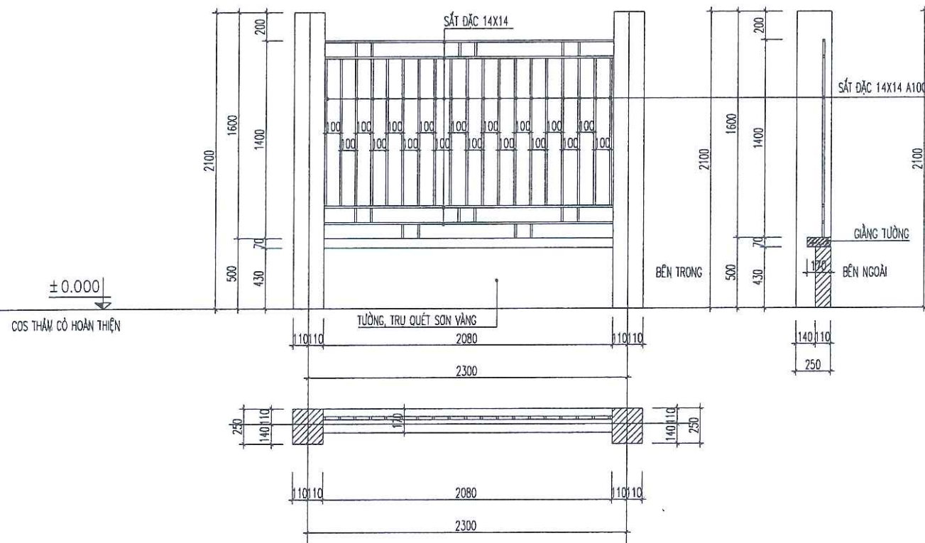
TƯỜNG RÀO THOÁNG ĐOẠN 2-3 BƯỚC 2300
