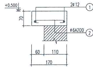
GIẺNG TƯỜNG RÀO
