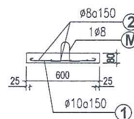
MẶT CẮT 1-1
