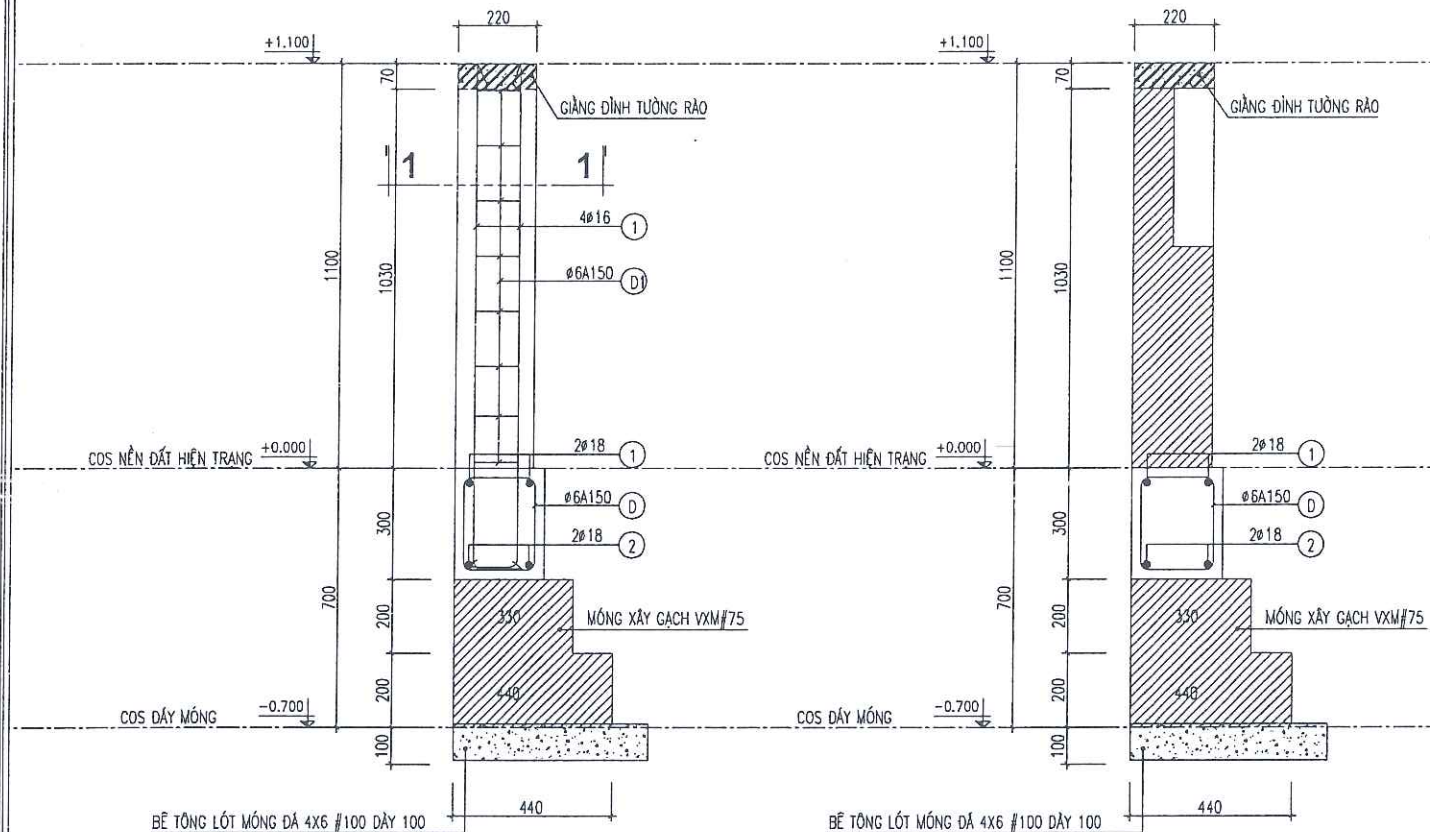
MÓNG TƯỜNG RÀO ĐOẠN 4-5
