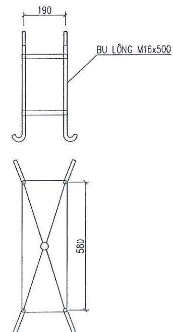
KHUNG MÓNG TỦ
