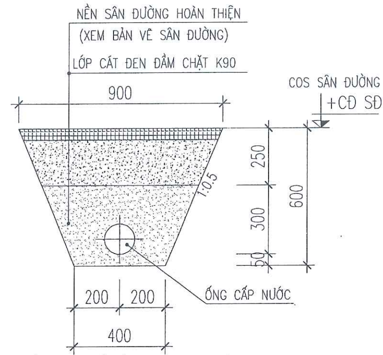
MẶT CẮT NGANG ĐIỂN HÌNH CHÔN ỚNG (SÂN ĐƯỜNG: 16.4M)
