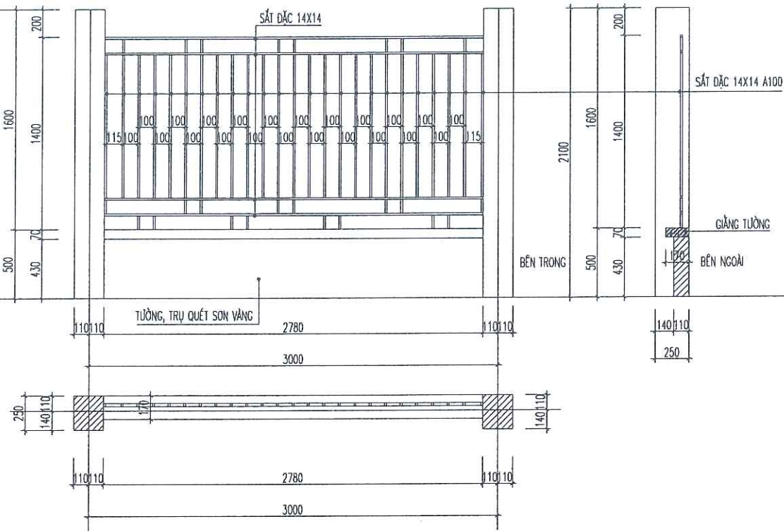
TƯỜNG RÀO THOÁNG ĐOẠN 8-9 BƯỚC 3000 ( SỐ LƯỢNG: 01 CK )
