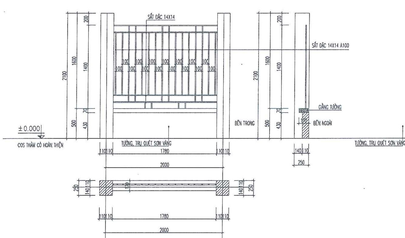
TƯỜNG RÀO THOÁNG ĐOẠN 8-9 BƯỚC 2000 ( SỐ LƯỢNG: 01 CK )
