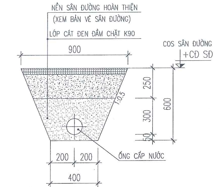
MẶT CẮT NGANG ĐIỂN HÌNH CHÔN ỐNG (SÂN ĐƯỜNG: 8.6M)
