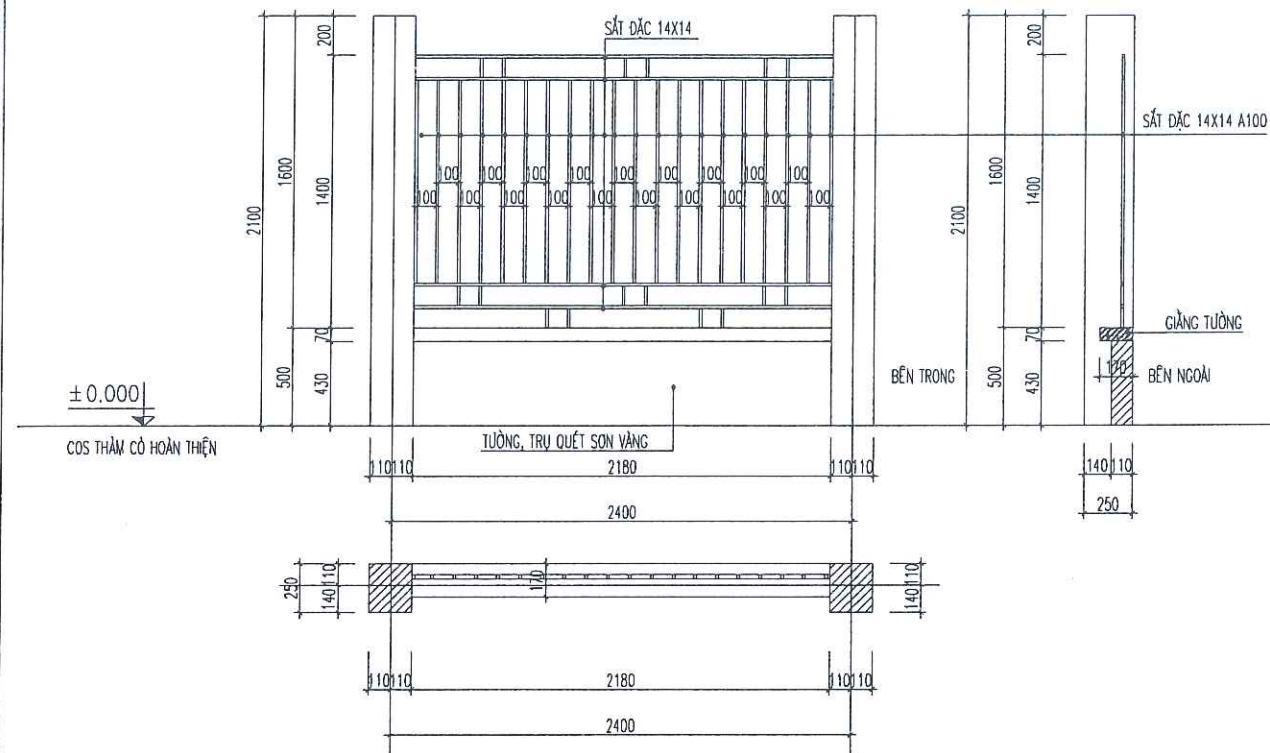
TƯỜNG RÀO THOÁNG ĐOẠN 7-8 BƯỚC 2400 ( SỐ LƯỢNG: 01 CK )
