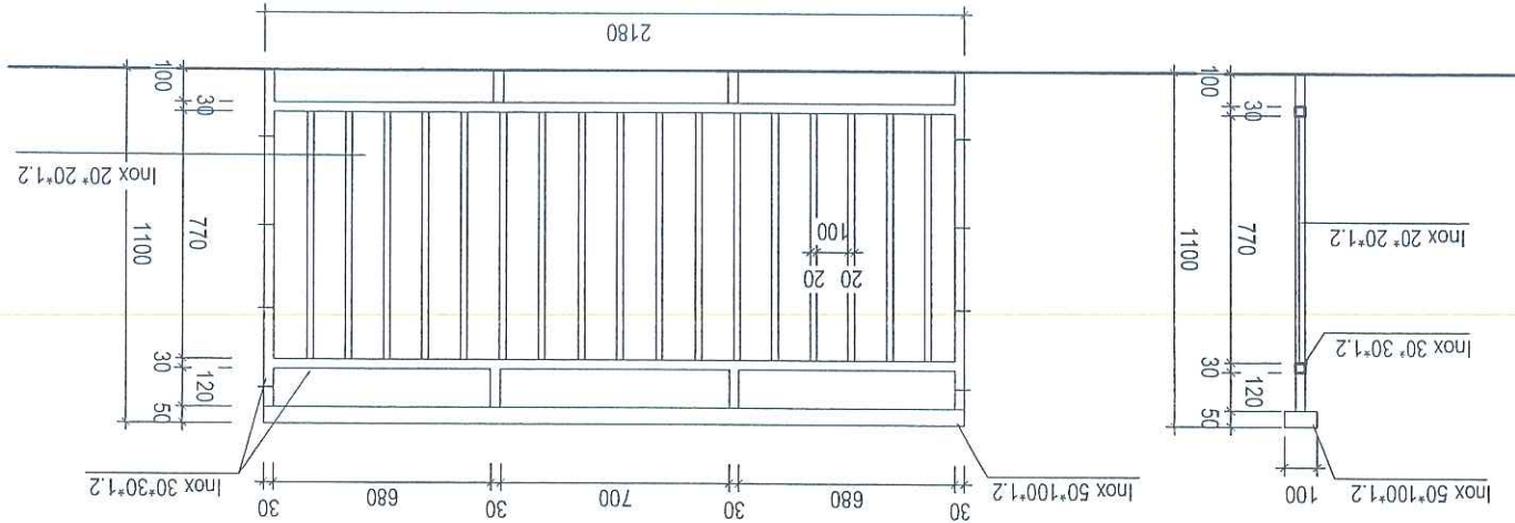
CHI TIẾT LAN CAN LC2 (SL:02CK)
