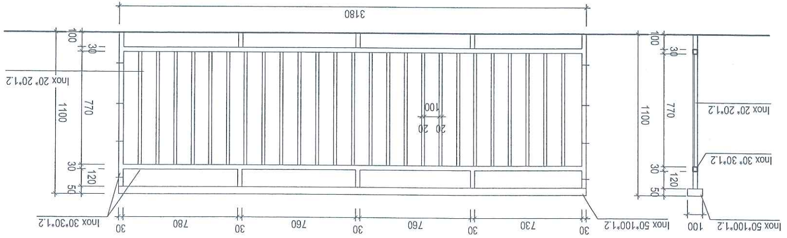
CHI TIẾT LAN CAN LC1 (SL:03CK)
