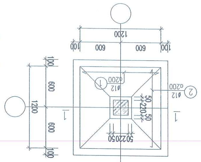
MÔNG M.C1 (SL=04)
