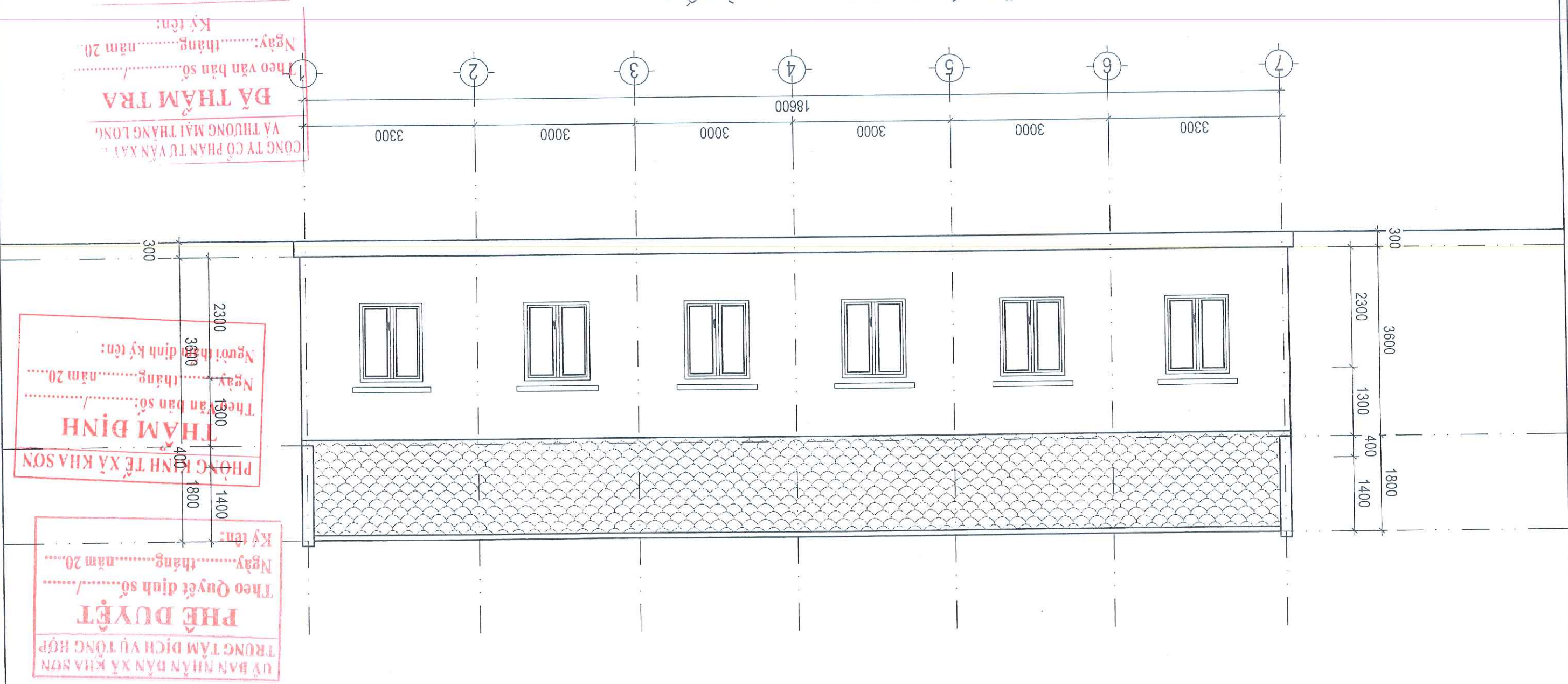
MẶT ĐỪNG TRÚC 8 - 1 NHÀ SỐ 2
