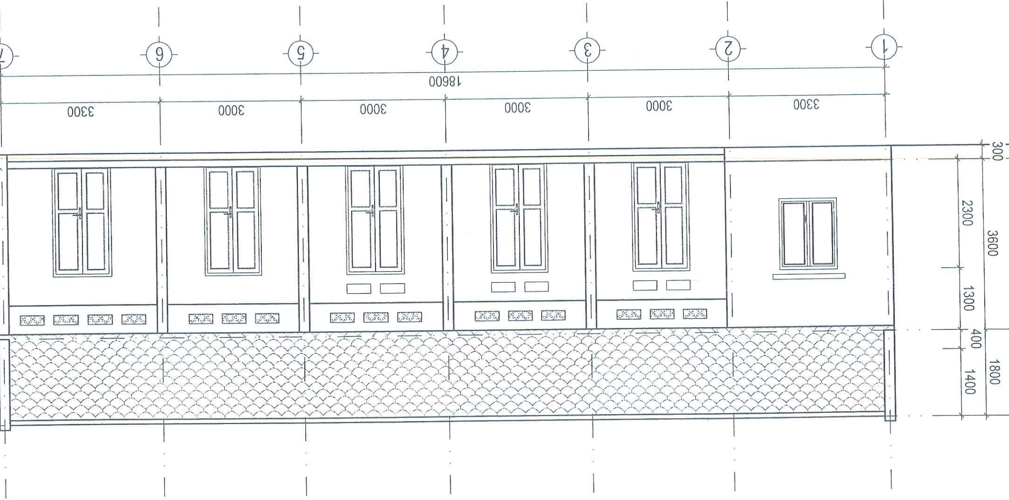
MẶT DƯNG TRÚC 1 - 8 NHÀ SỐ 2
