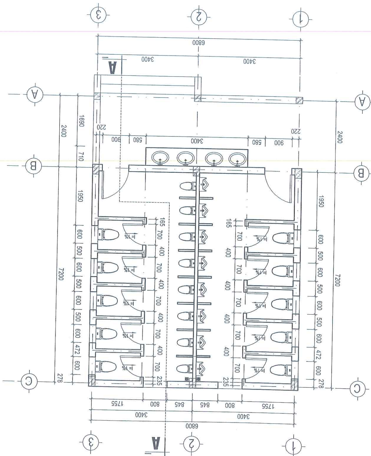
MẶT BẰNG TẦNG 1 NHÀ WC
