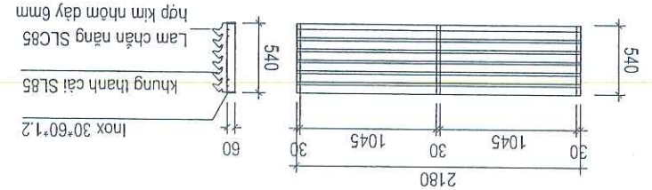
CHẠN NẶNG CN2 (SL:02CK)
