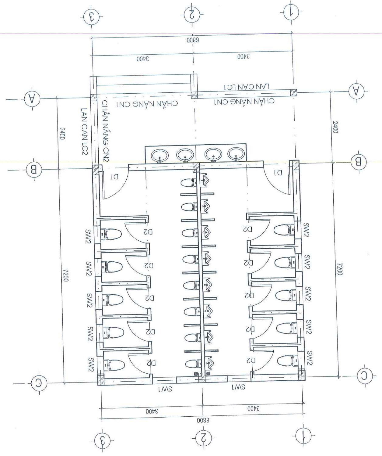
MẶT BẰNG CỦA TẦNG 1 NHÀ WC
