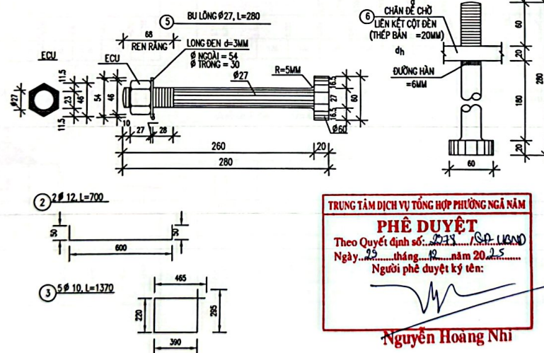
CHI TIẾT HÀN BU LÔNG $27 VÀO CHÂN ĐỂ CHỜ LIÊN KẾT CỘT ĐÈN
