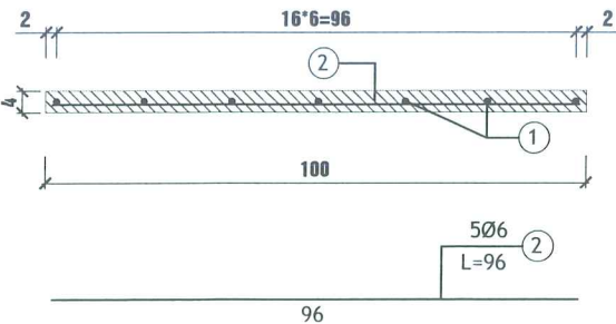
CẮT DỌC BẢN RÃNH B600 ĐÚC SẴN (TL:1/10)
