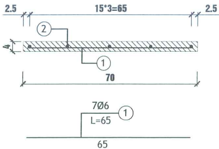
CẮT NGANG BẢN RÃNH B600 ĐÚC SẴN (TL:1/10)
