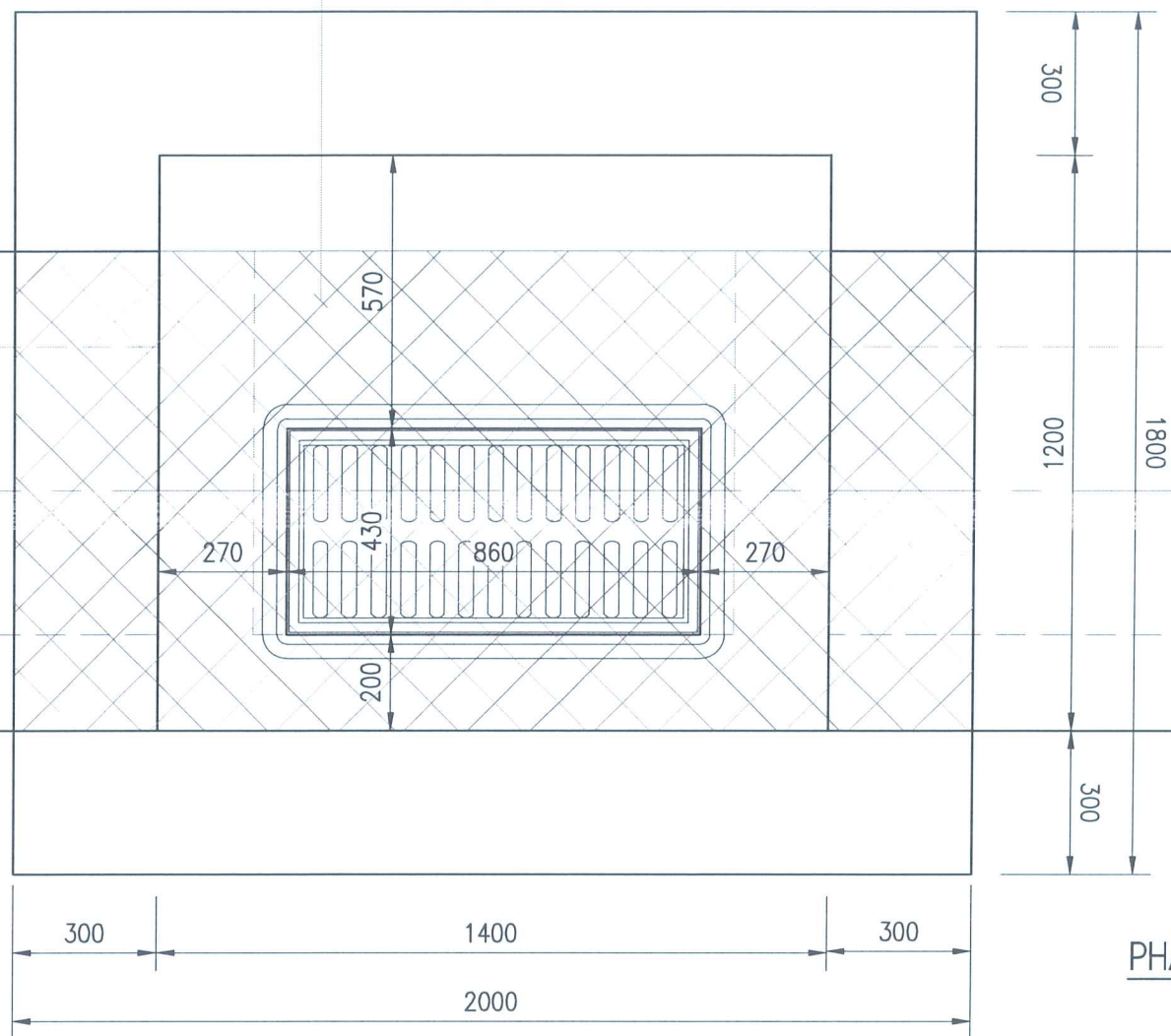
MẶT BẰNG HỒ ĐÀO GA LOẠI 1,2,3
