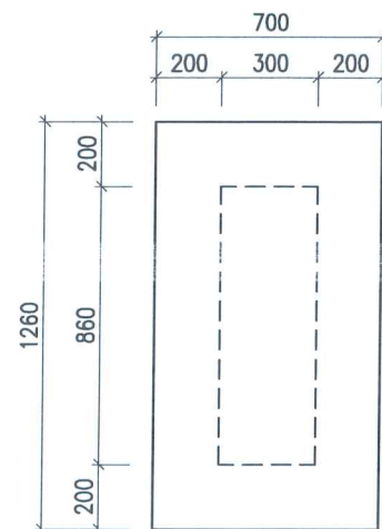
MẶT BẰNG ĐÁY
