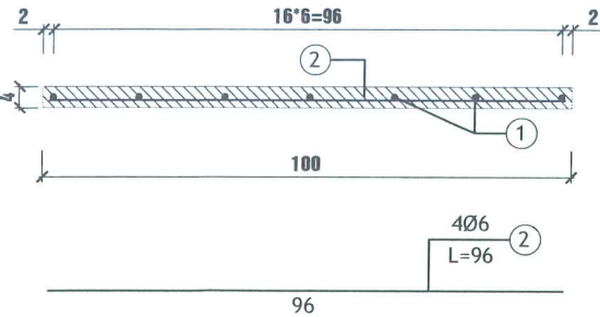
CẮT DỌC BẢN RÃNH B400 ĐÚC SẴN (TL:1/10)
