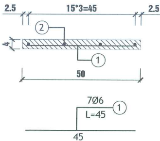
CẮT NGANG BẢN RÃNH B400 ĐÚC SẴN (TL:1/10)
