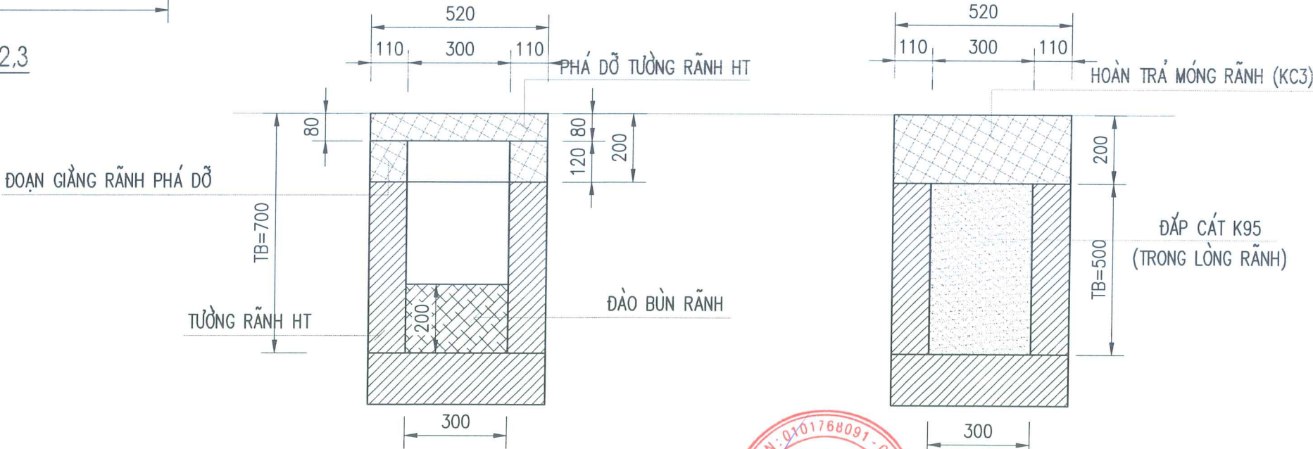
PHÁ DỠ ĐẠN RÃNH HIỆN TRẠNG
