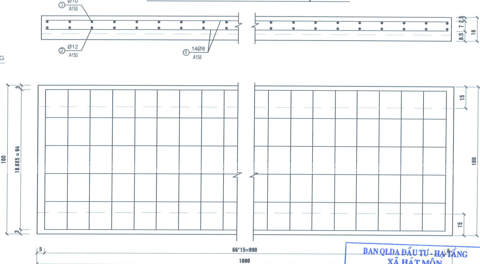
CHI TIẾT TẦM ĐAN R NH ĐỔ TRỰC TIẾP
