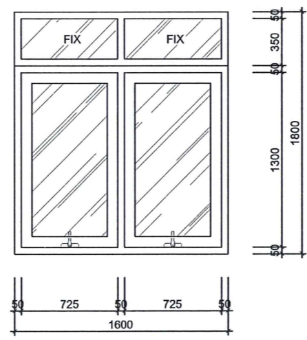
CHI TIẾT CỬA KÍNH CS3 KIỂM TRA KỊCH THUỘC THỰC TẾ TRƯỚC KHI THI CÔNG PHỤ KIỆN: KÍNH LONG ĐỒNG BÒ
