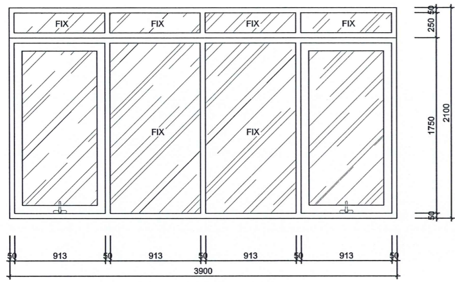
CHI TIẾT CỬA KÍNH CS1 KIỂM TRA KỊCH THUỘC THỰC TẾ TRƯỚC KHI THI CÔNG PHỤ KIỆN: KÍNH LONG ĐỒNG BÒ
