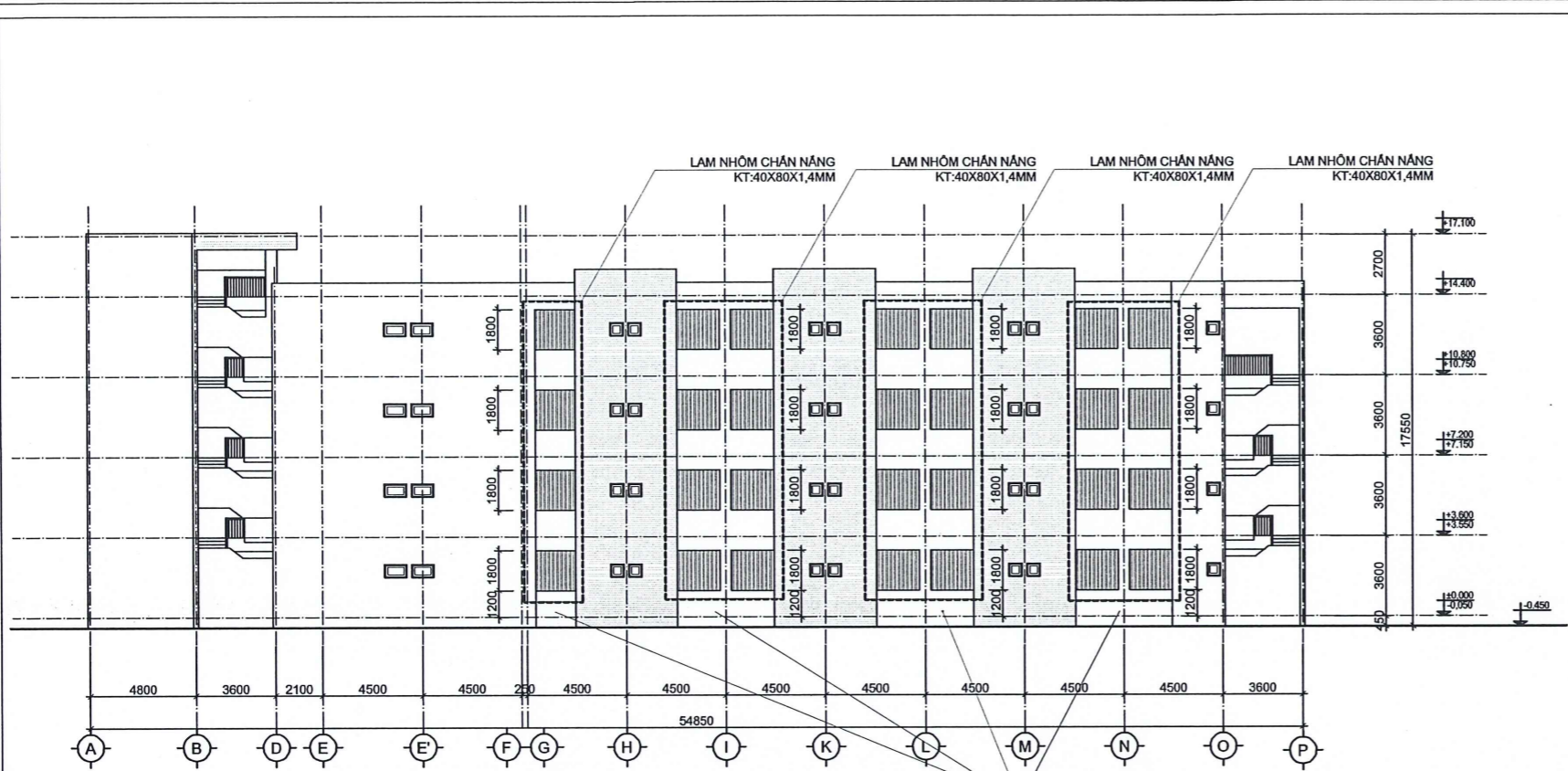
MẶT ĐỨNG TRỤC A-P
