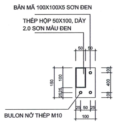
LIÊN KẾT THÉP HỘP 50X100 VỚI NỀN BÊ TÔNG
