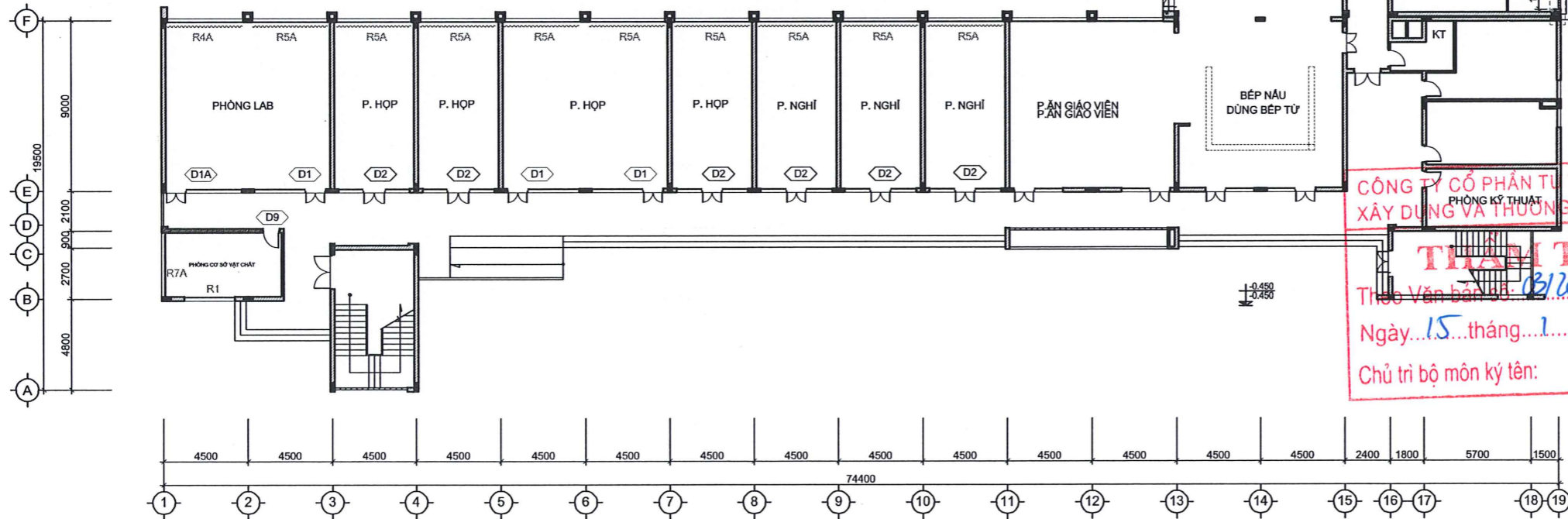
MẶT BẰNG RÈM, DECAL + CỬA TẦNG 1
