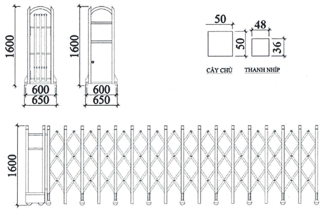
CHI TIẾT CÔNG XÉP TỰ ĐỘNG
