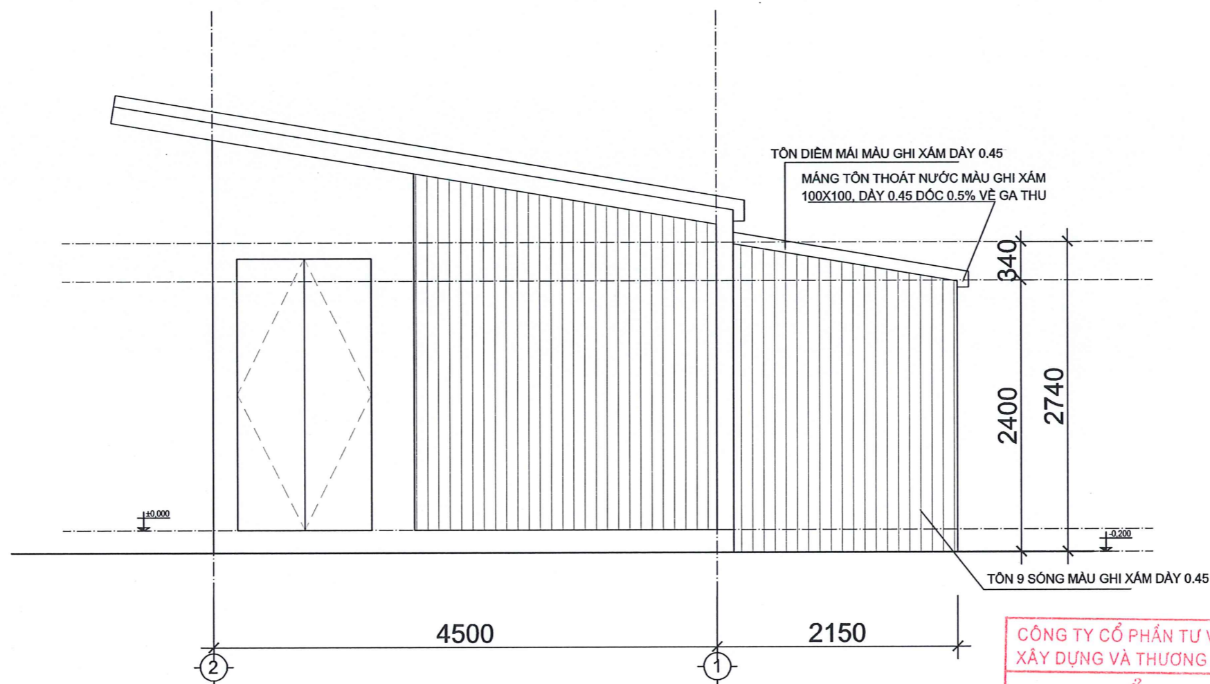
MẶT ĐỨNG TRỤC 2-1
