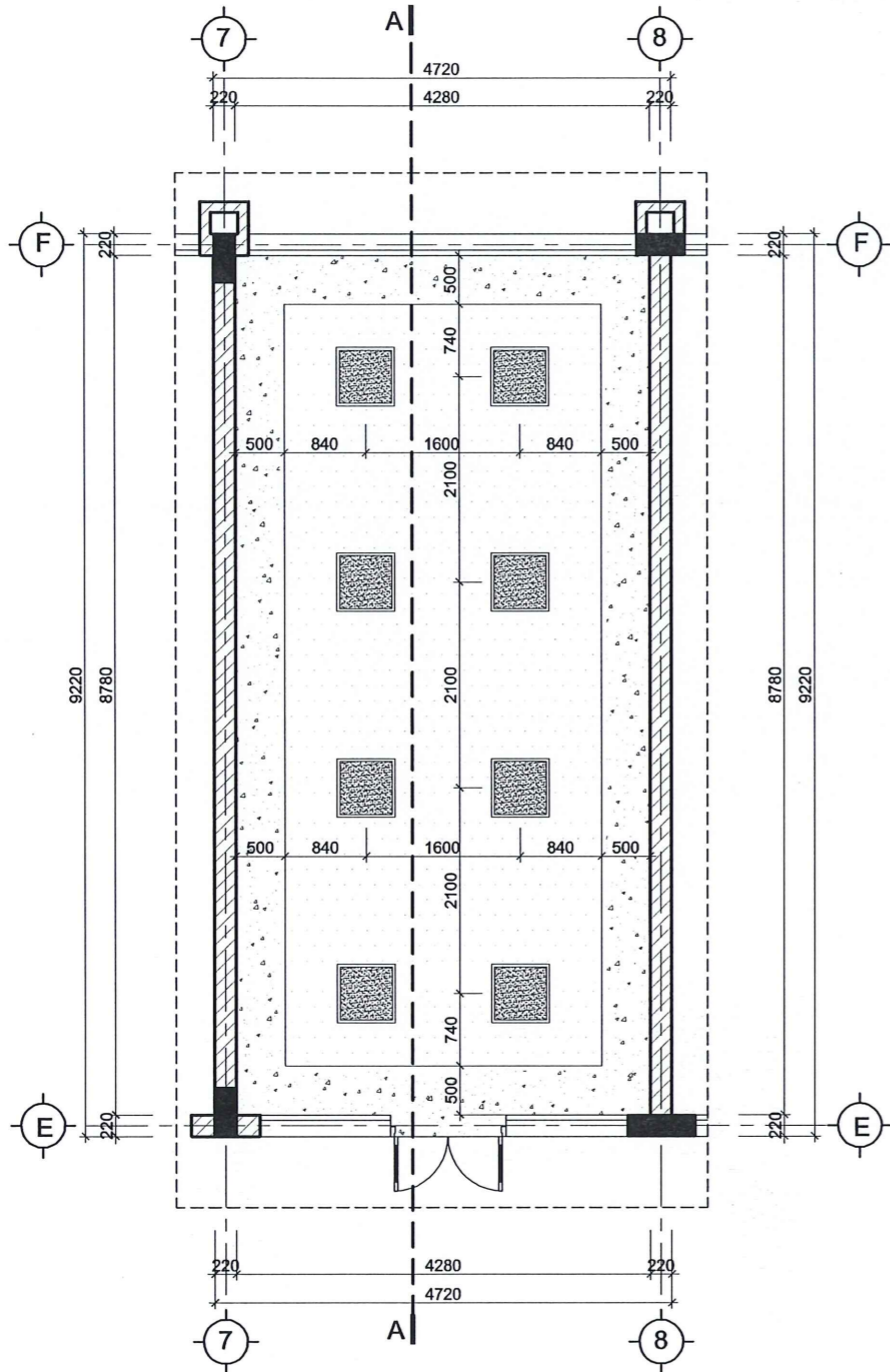
CHI TIẾT TRẦN ĐIỀN HÌNH 02
