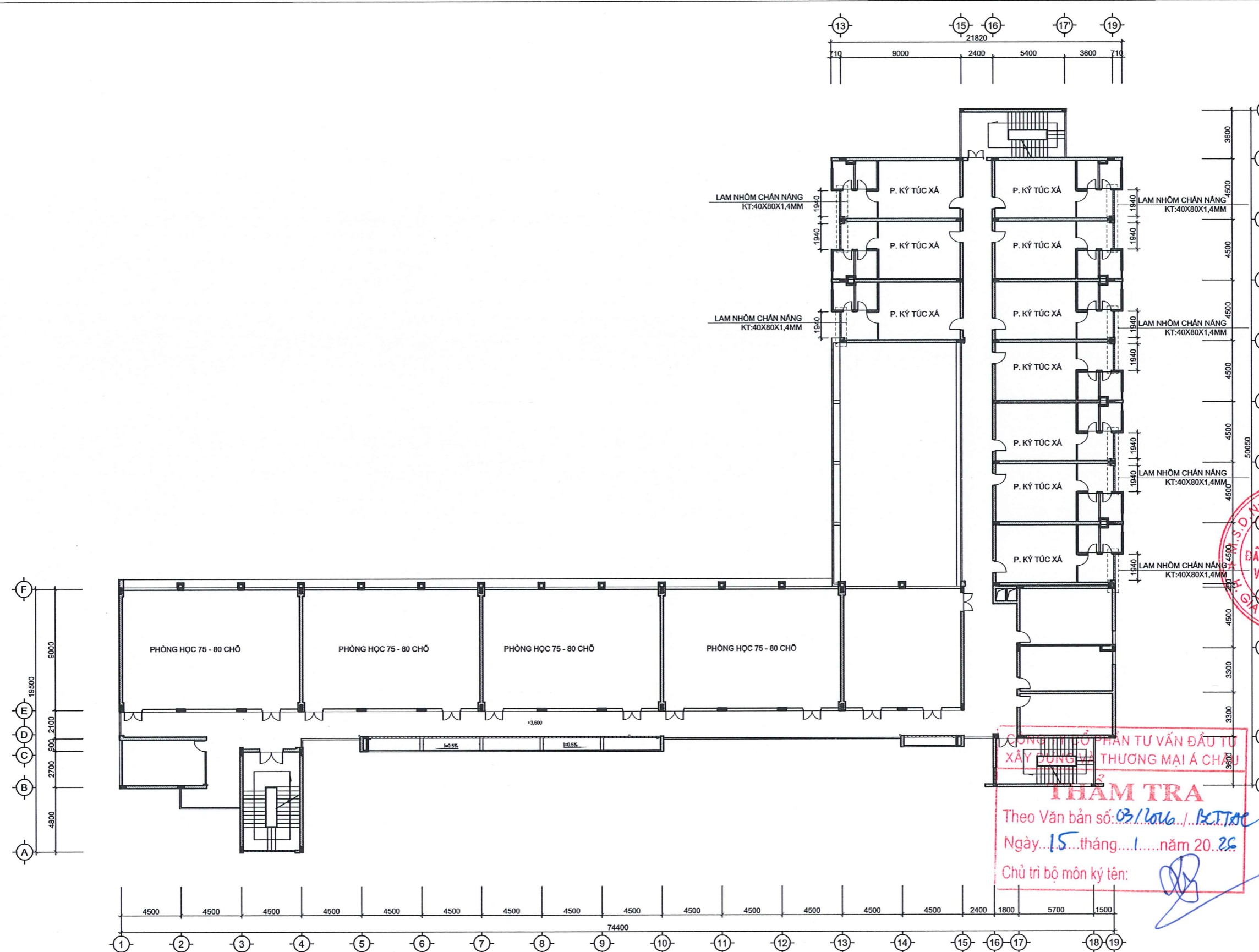
MẶT BẰNG RÈM, LAM NHÔM TẦNG 2
