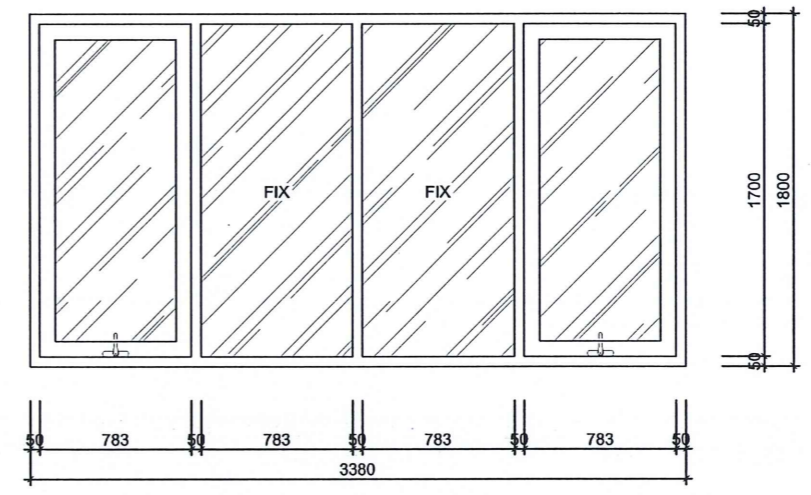
CHI TIẾT CỬA KÍNH CS7 KIỂM TRA KỊCH THUỘC THỰC TẾ TRƯỚC KHI THI CÔNG PHỤ KIỆN: KÍNH LONG ĐỒNG BÒ
