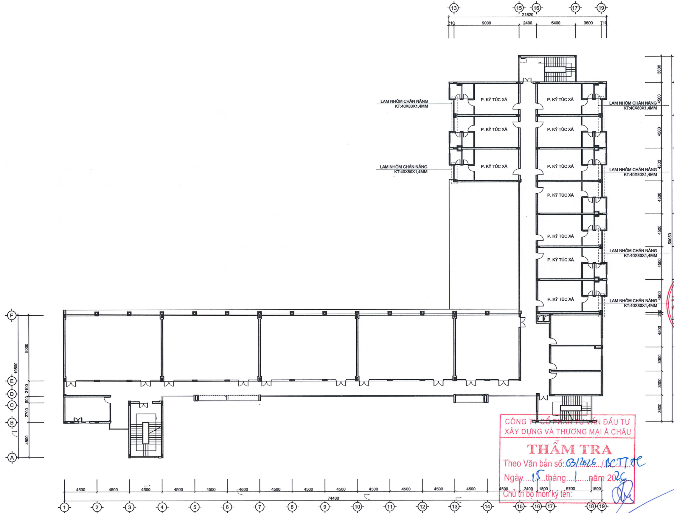
MẶT BẰNG RÈM, LAM NHÔM TẦNG 4
