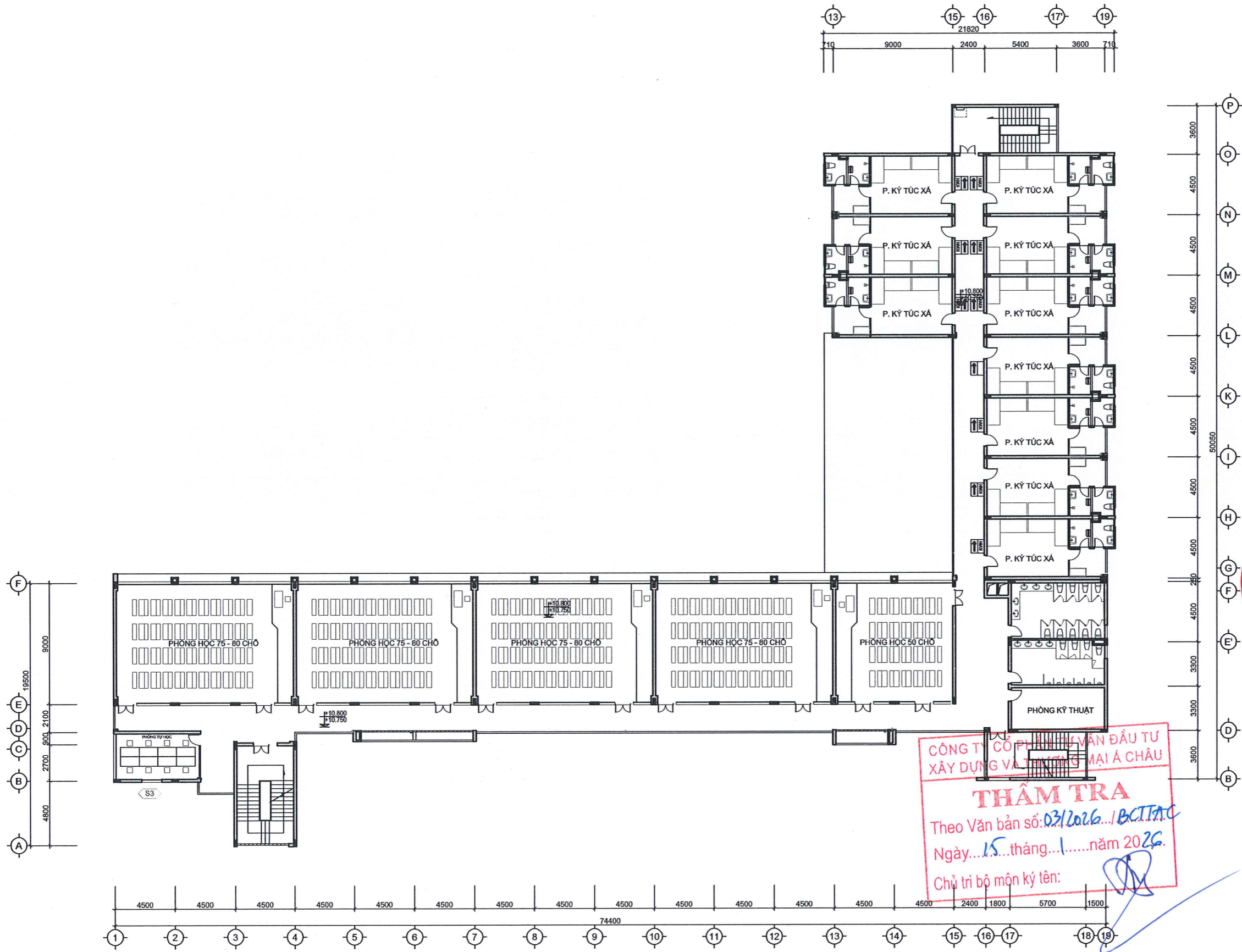
MẶT BẰNG BỐ TRÍ NỘI THẤT TẦNG 4
