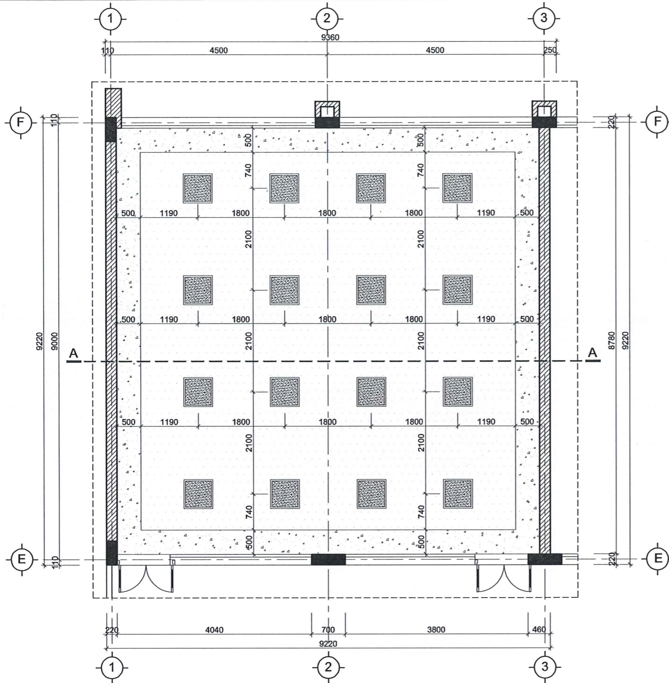
CHI TIẾT TRẦN ĐIỀN HÌNH 01
