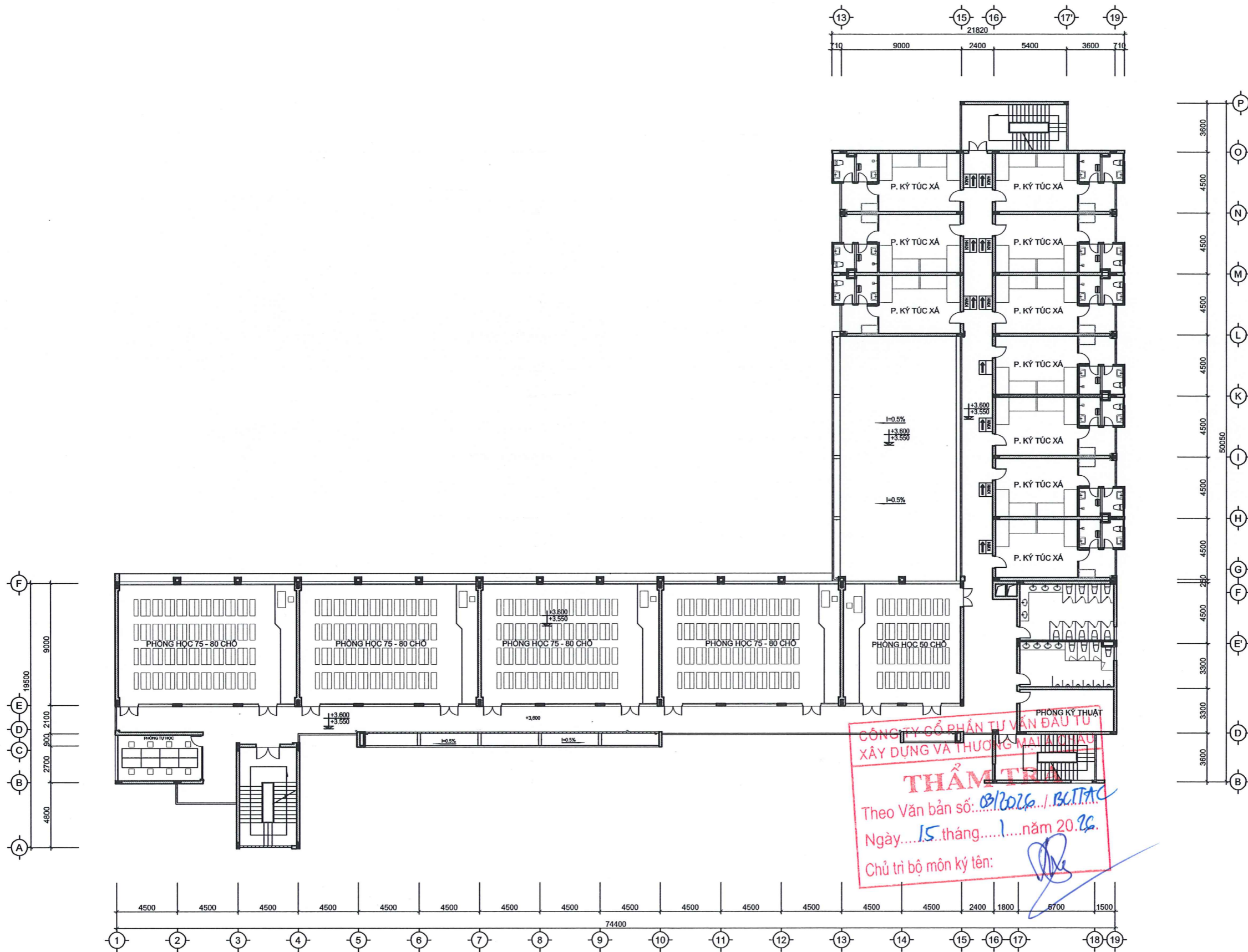
MẶT BẰNG BỐ TRÍ NỘI THẤT TẦNG 2
