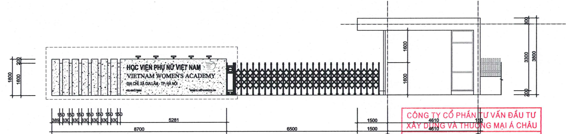
MẶT ĐỨNG CÔNG XÉP TỰ ĐỘNG
