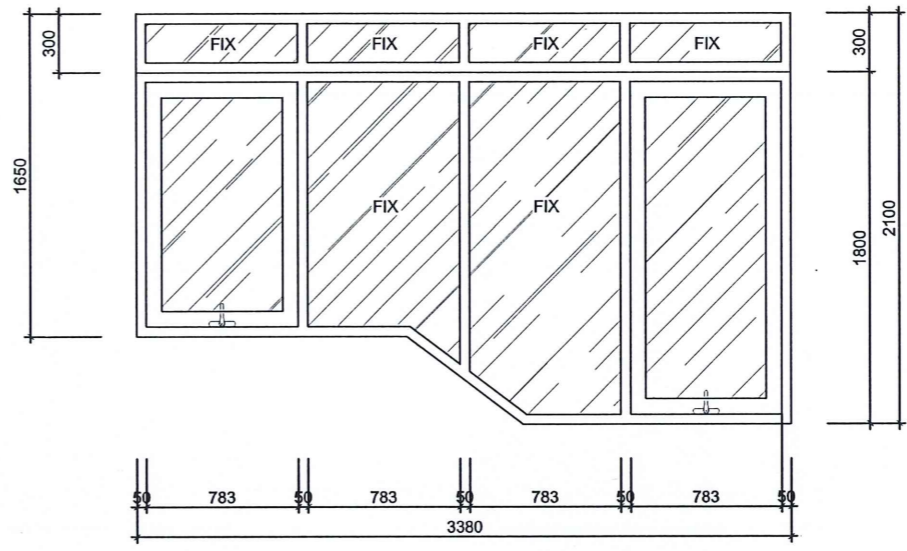
CHI TIẾT CỬA KÍNH CS2 KIỂM TRA KÍCH THƯỚC THỰC TẾ TRƯỚC KHI THI CÔNG PHỤ KIỆN: KIM LONG ĐỒNG BÒ
