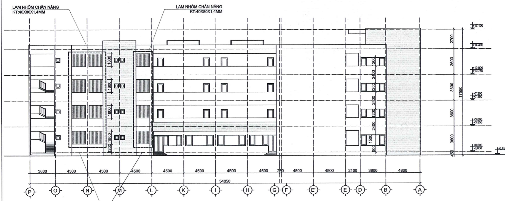
MẶT ĐỨNG TRỤC P-A
