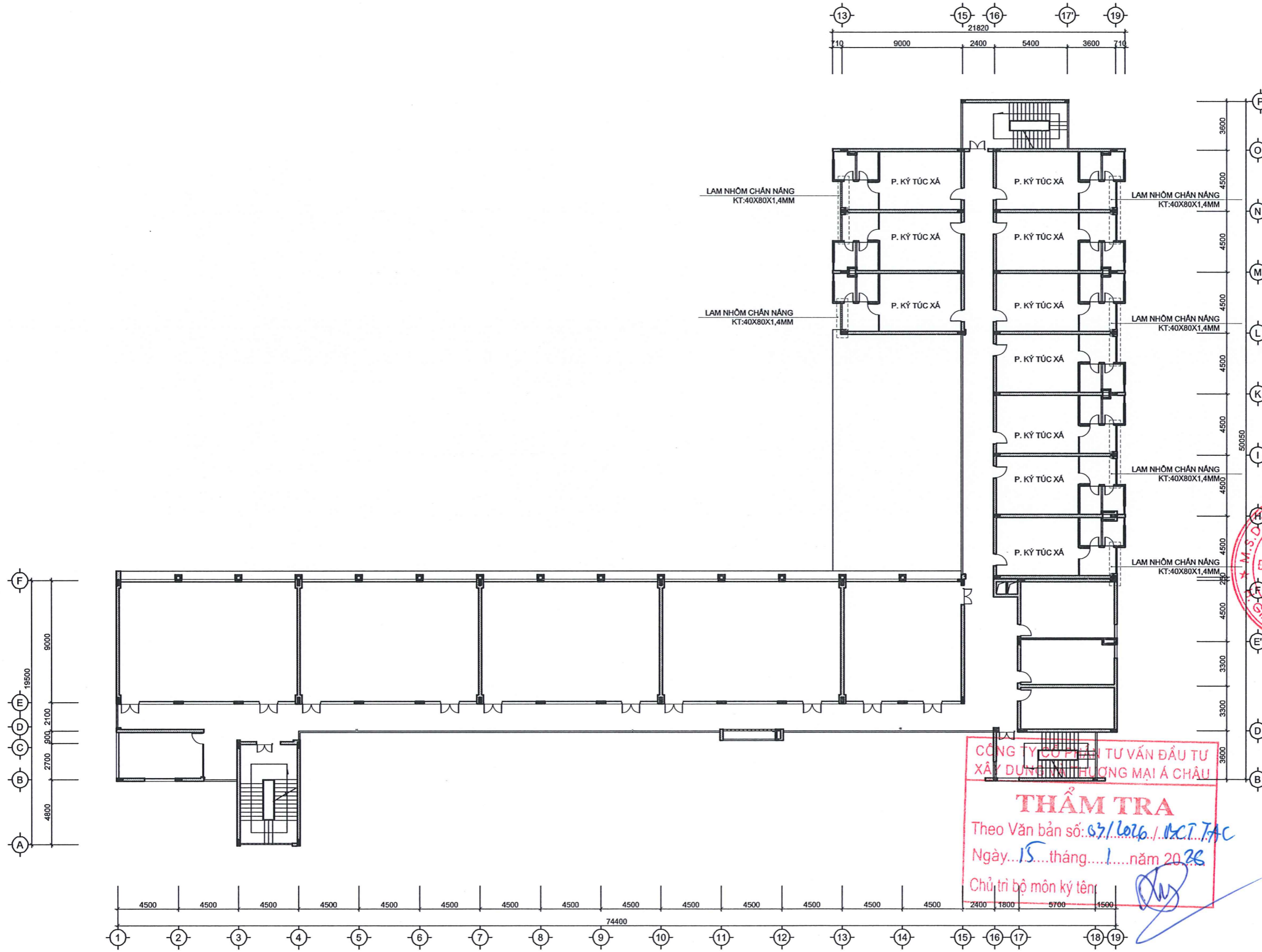
MẶT BẰNG RÈM, LAM NHÔM TẦNG 3
