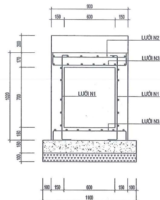
BỐ TRÍ THÉP CỐNG
