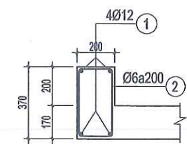
GỜ CHÂN BÁNH XE
