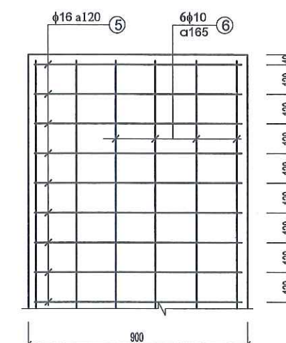
LƯỚI N3 (2 TẦM)
