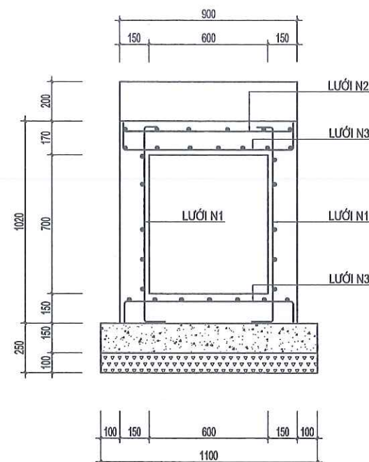
BỐ TRÍ THÉP CÔNG
