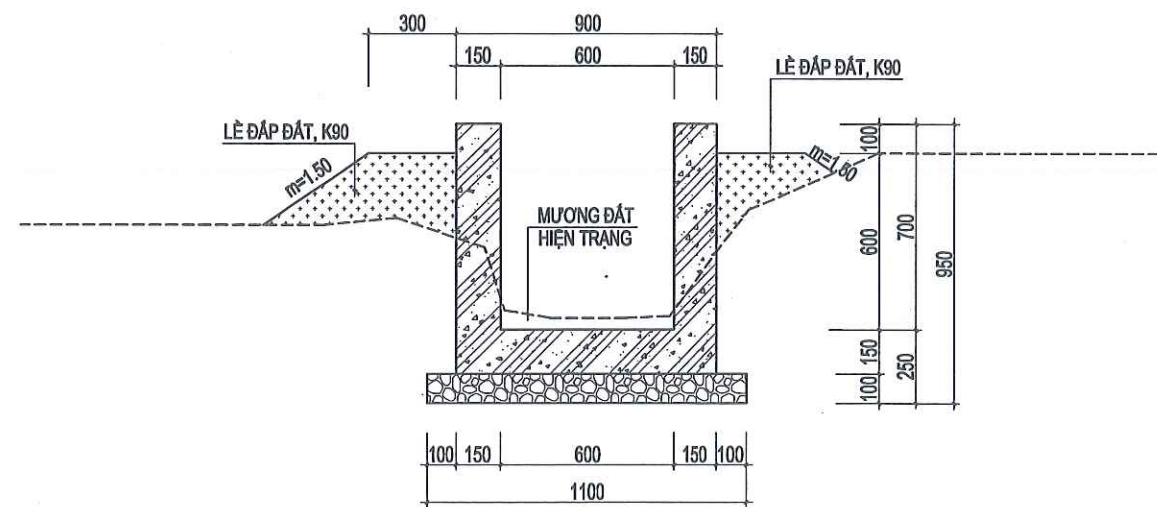
MẶT CẮT HOÀN THIỆN
