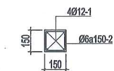
CẮT NGANG 1-1
