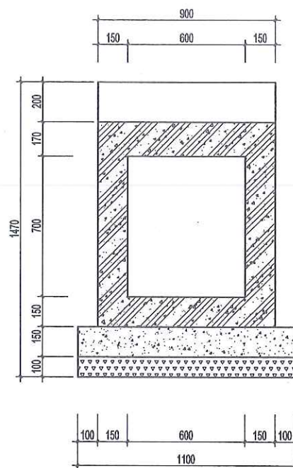
MẶT CẮT NGANG CỐNG HỘP
