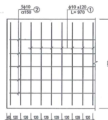
LUỚI N1 (2 TẦM)
