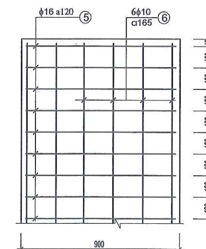
LUỚI N3 (2 TẦM)
