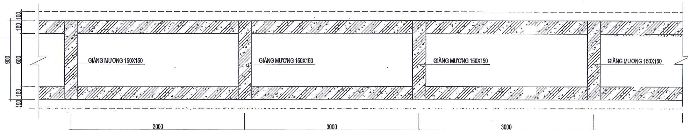
MẶT BẰNG ĐOẠN MƯƠNG ĐIỀN HÌNH
