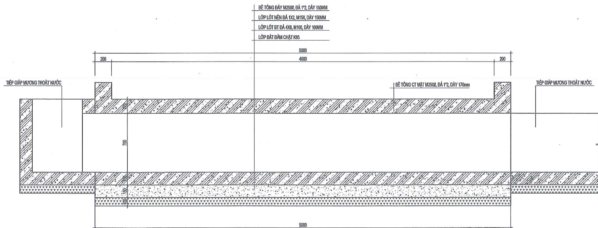
MẶT CẮT DỌC CÔNG HỘP C1, C2
