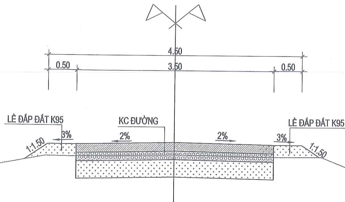
MẶT CẮT NGANG ĐẠI DIỆN (TỪ KM0 +915.29- KM1+484.01)
