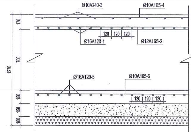
BỐ TRÍ THÉP CÔNG
