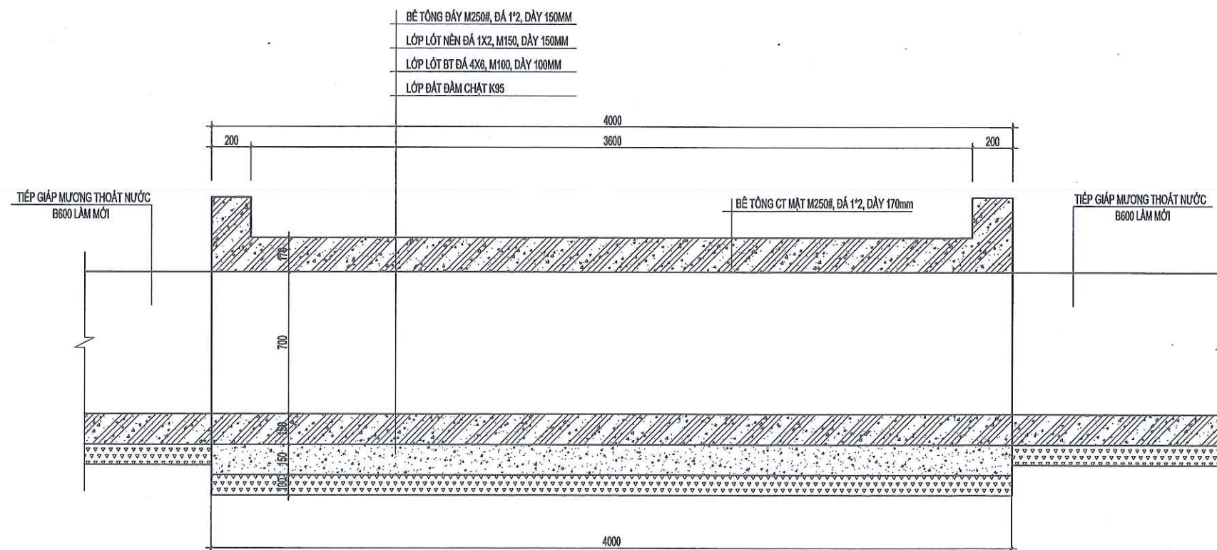
MẶT CẮT DỌC CÔNG HỘ
