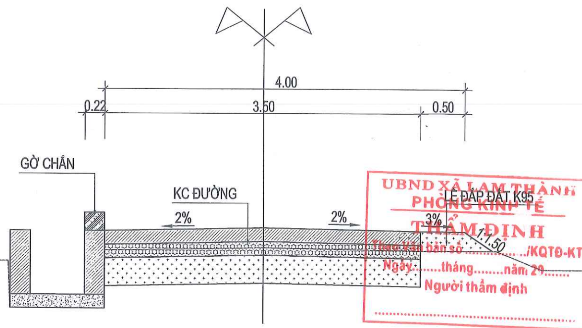
MẶT CẮT NGANG ĐẠI DIỆN (TỪ KM0- KM0+908.97)
