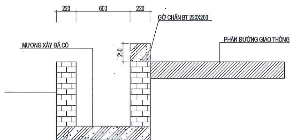
ĐỒ GỖ CHẤN BT SÁT MƯƠNG (TỪ CỌC KM0 - ĐẾN CỌC P4 DÀI 908M)
