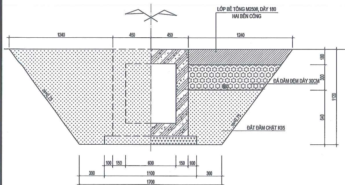
1/2 MẶT CẮT ĐÀO, ĐÁP
