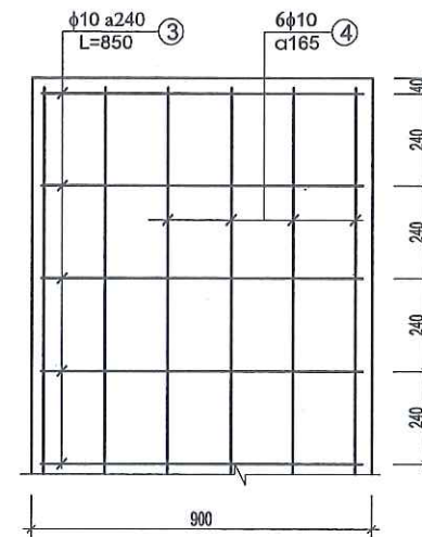
LƯỚI N2 (1 TẤM)
