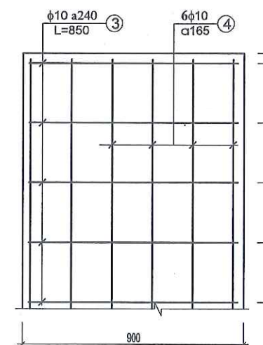
LUỚI N2 (1 TẦM)
