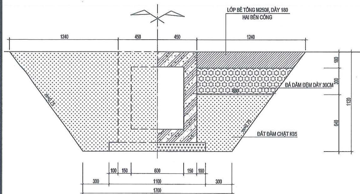
1/2 MẶT CẮT ĐÀO, ĐẬP
