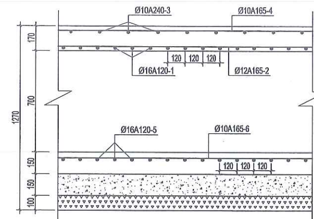
BỐ TRÍ THÉP CỐNG
