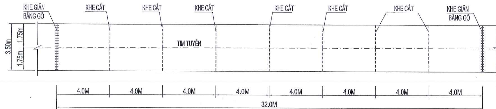
BỐ TRÍ KHE CẮT ĐIỀN HÌNH ĐƯỜNG 3.5m
