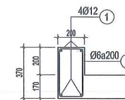
GỜ CHẤN BÁNH XE
