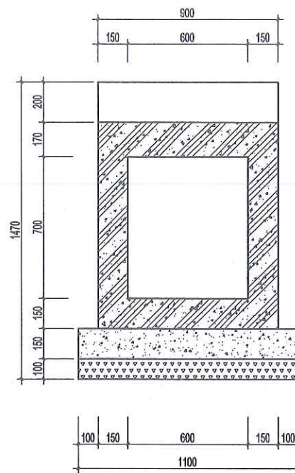
MẶT CẮT NGANG CÔNG HỢP
