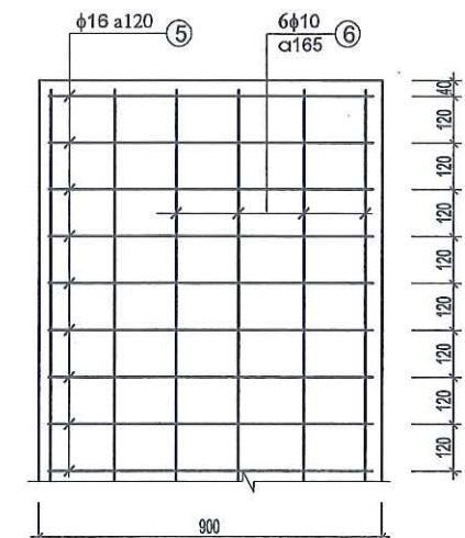
LƯỚI N3 (2 TẦM)
