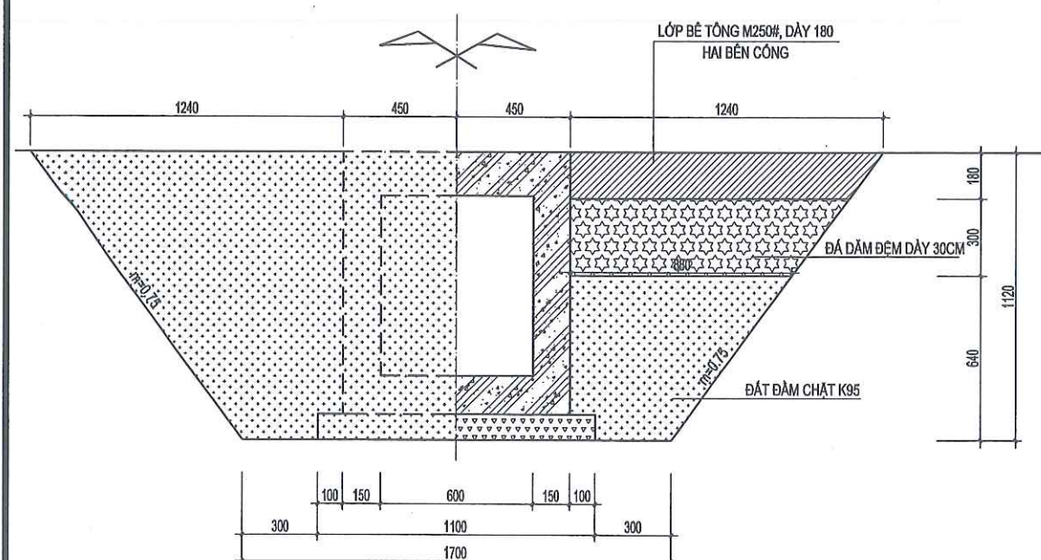
1/2 MẶT CẮT ĐÀO, ĐẬP
