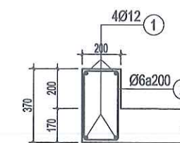
GỜ CHÂN BÁNH XE
