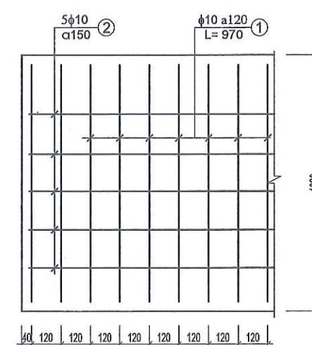
LƯỚI N1 (2 TẦM)
