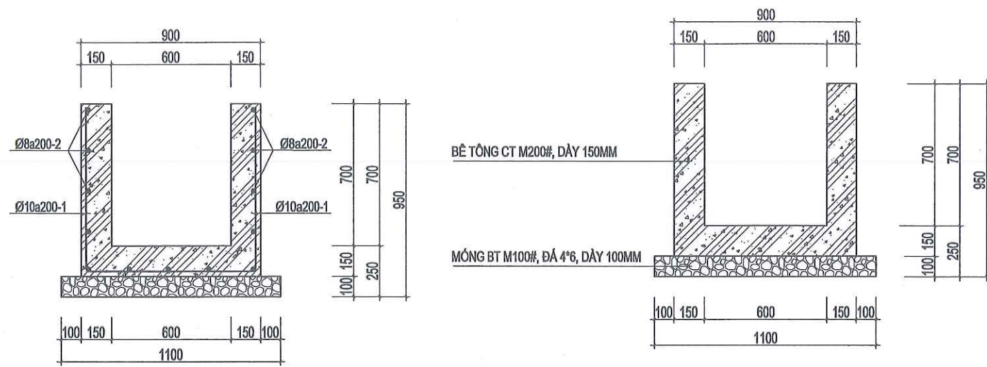
BỐ TRÍ THÉP MƯƠNG
