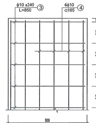
LƯỚI N2 (1 TẦM)
