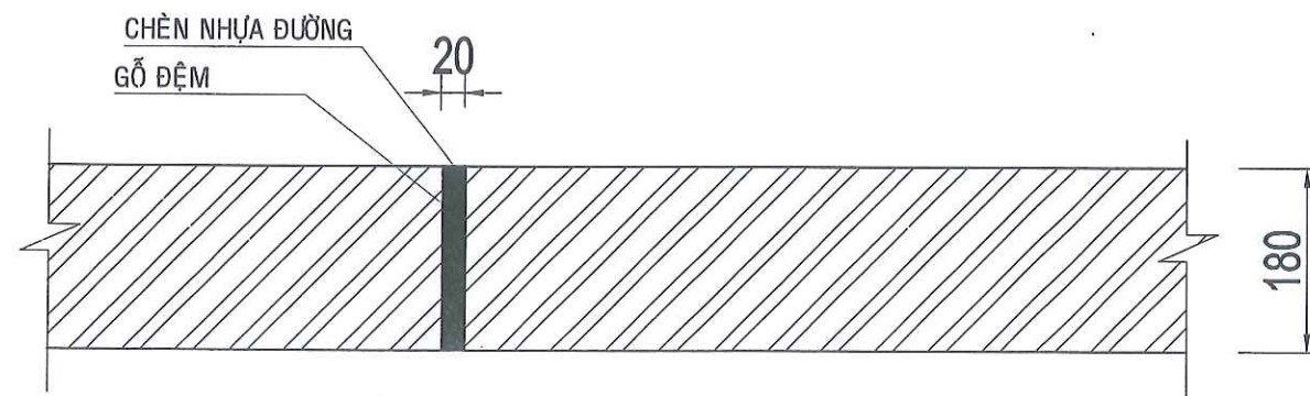
CHI TIẾT KHE DẪN BẰNG GỖ
