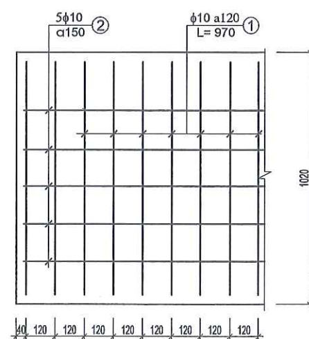
LƯỚI N1 (2 TẤM)
