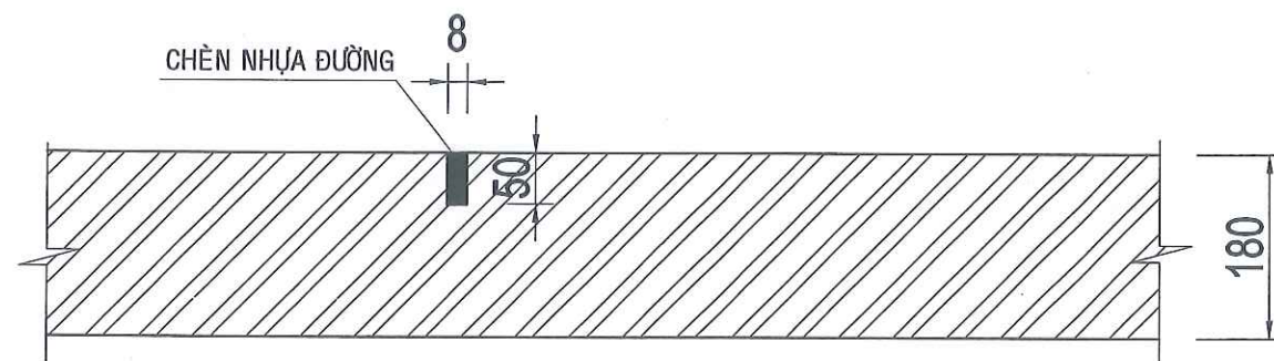
CHI TIẾT KHE CẮT
