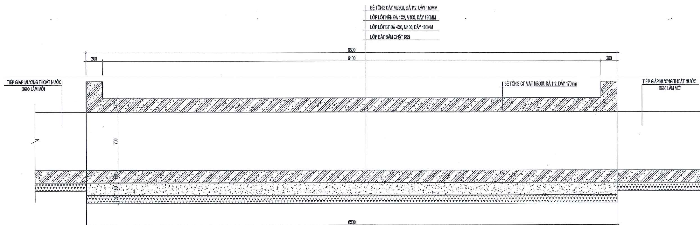
MẶT CẮT DỌC CỐNG HỘP
