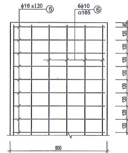
LƯỚI N3 (2 TẤM)
