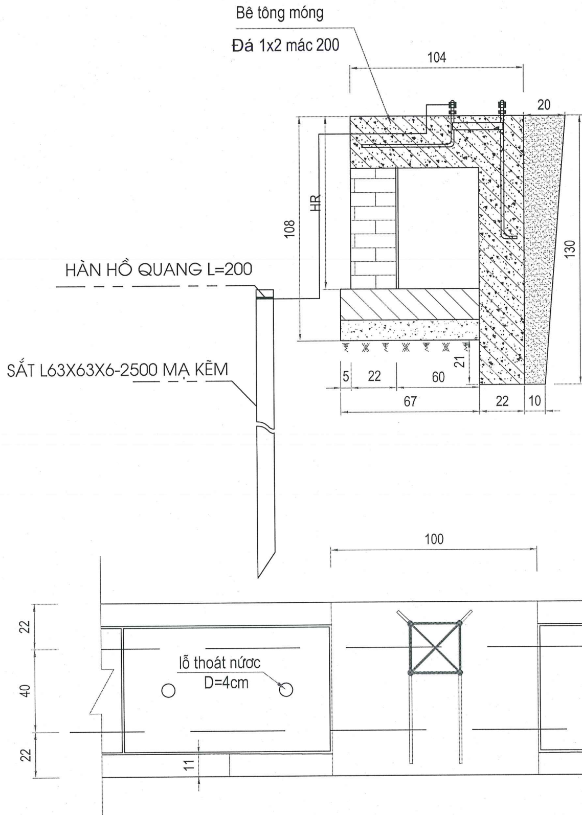
MẶT BẰNG RÃNH TẠI VỊ TRÍ CỘT CHIẾU SÁNG (TL 1/25)
