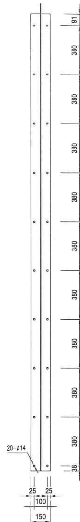
HƯỚNG NHÌN 1
