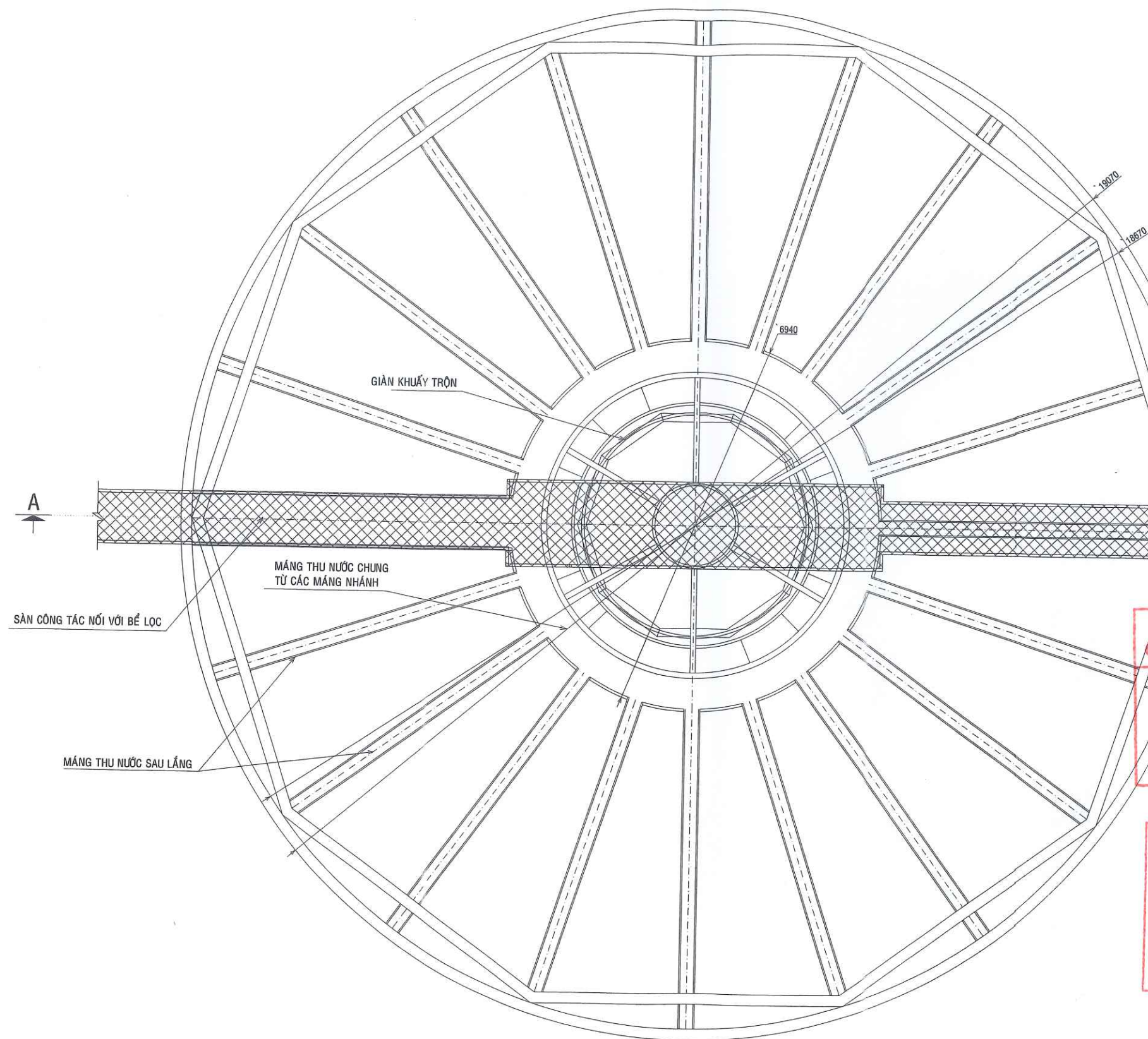
MẶT BẰNG BỂ LẮNG ACCELATOR B
