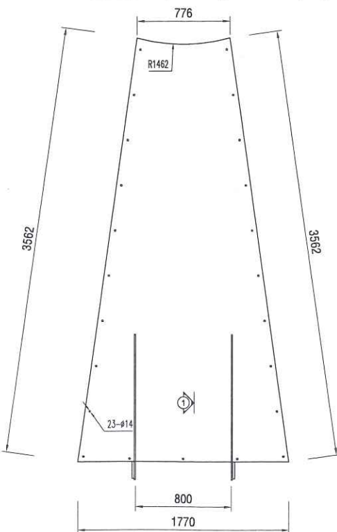
CHI TIẾT 1c Vật liệu: thép CT3 dày 6mm sơn Epoxy
