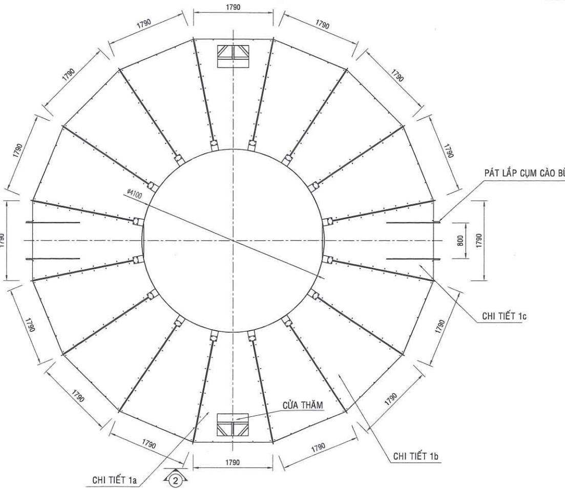
MẶT BẰNG
