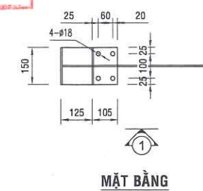
CHI TIẾT 5 TẤM THÉP CT3 DÀY 8MM (UỖN CÔNG R=2050MM) Vật liệu: thép CT3 dày 8mm sơn Epoxy
