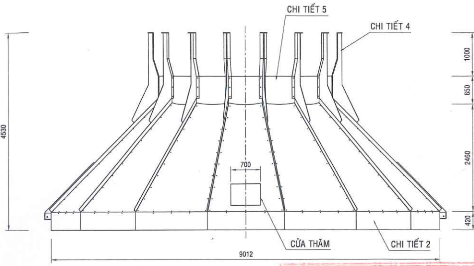
HƯỚNG NHÌN 2
