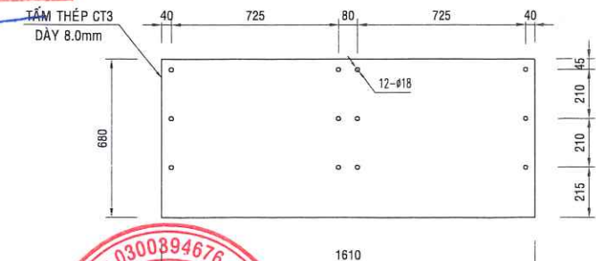
CHI TIẾT 5 TẤM THÉP CT3 DÀY 8MM (UỖN CÔNG R=2050MM) Vật liệu: thép CT3 dày 8mm sơn Epoxy
