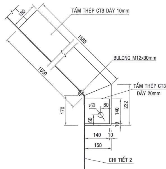
HƯỚNG NHÌN 1
