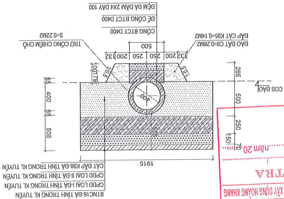
MẶT CÁT NGANG CÔNG D400
