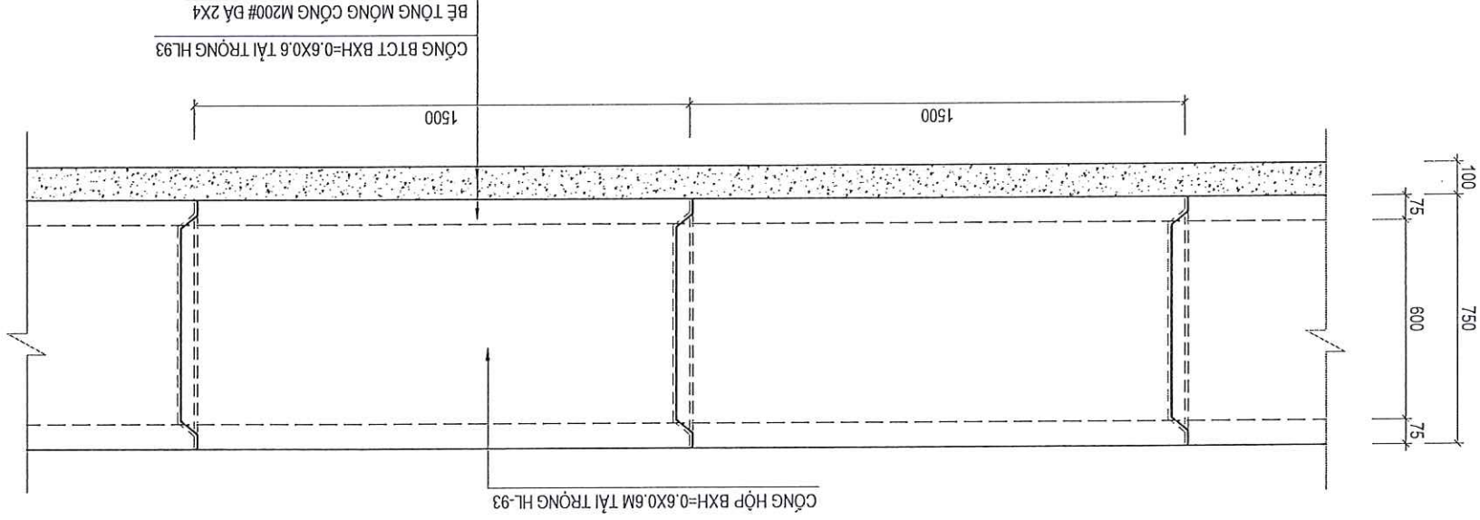
MẶT CẮT DỌC LẬP ĐẶT CÔNG HỘP BXH: 600X600
