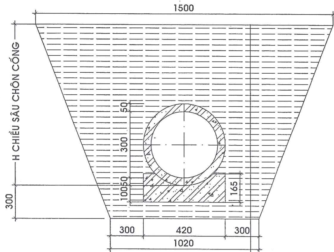
MẶT CẮT RĂNG ĐẶT CỐNG BTCT D300
