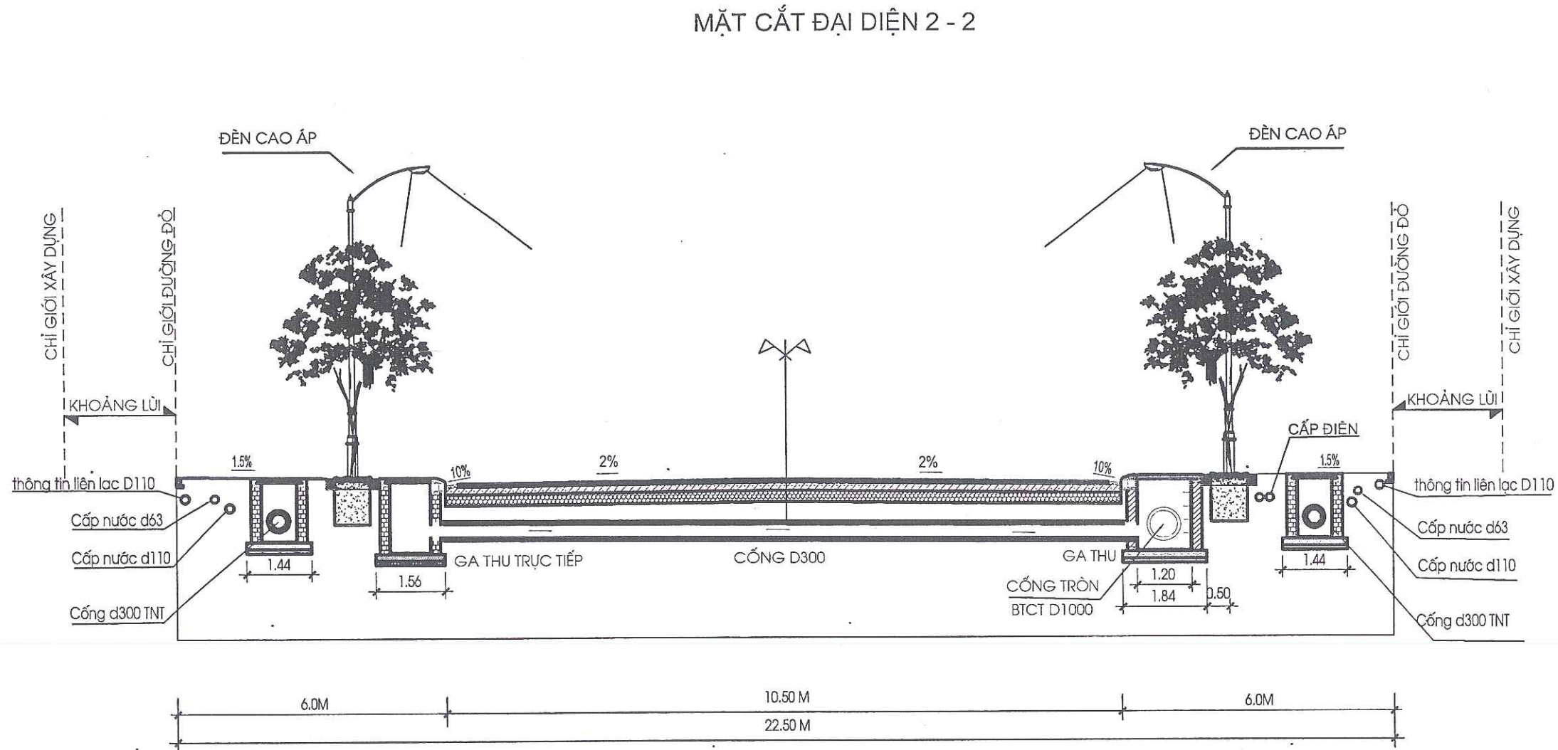
KẾT CẤU MẶT ĐƯỜNG MẶT CẮT 2-2
