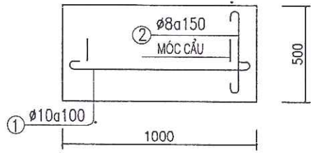
MẶT BẰNG TẦM ĐÀN A (2CK)
