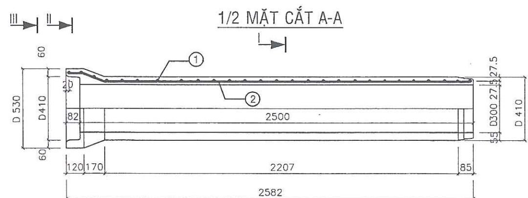
1/2 CHÍNH DIỆN
