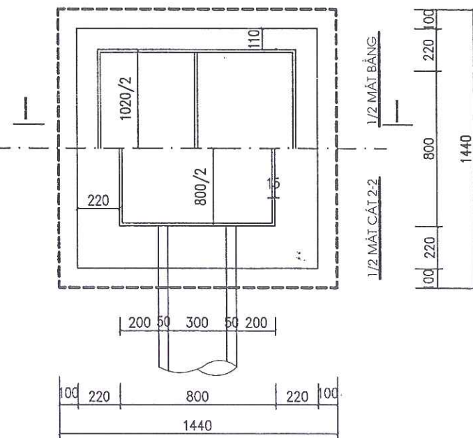
MẶT BẰNG HỐ GA LOẠI 1
