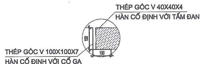
CHI TIẾT 1
