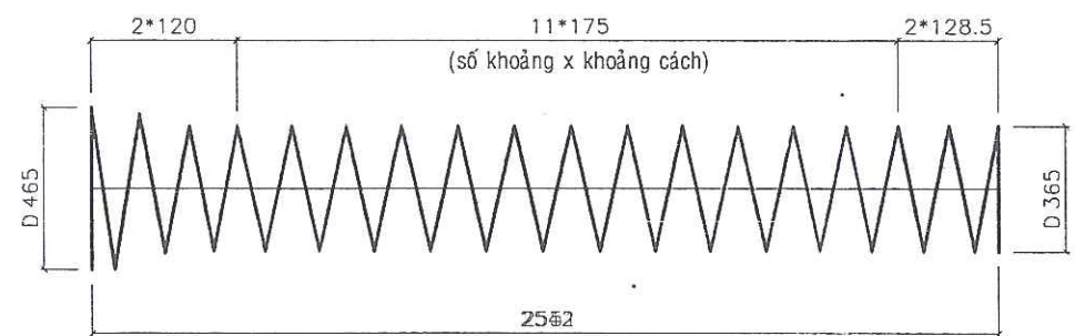
CỐT THÉP SỐ 1
