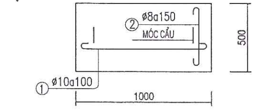
MẶT BẰNG TẤM ĐAN A (18CK)
