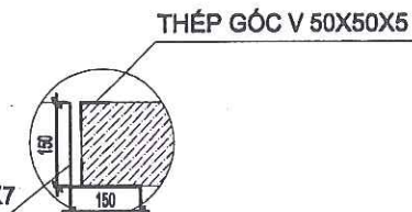
CHI TIẾT 1
