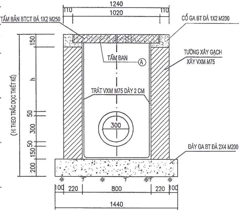
MẶT CẮT 1-1
