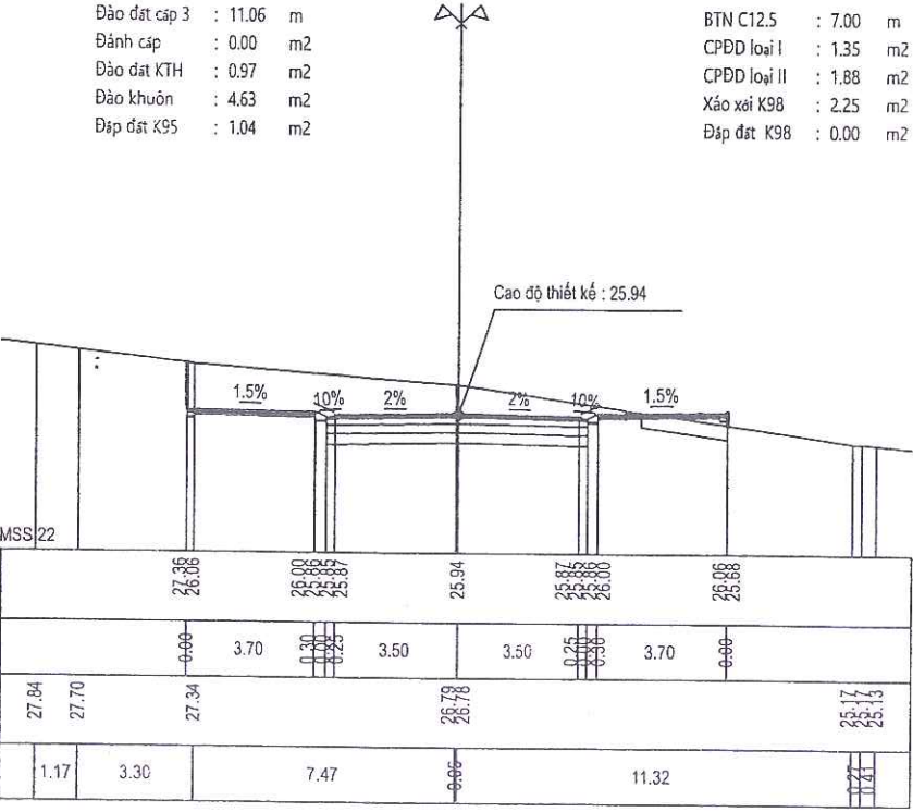
Cọc 17 Km 0 + 304.85
