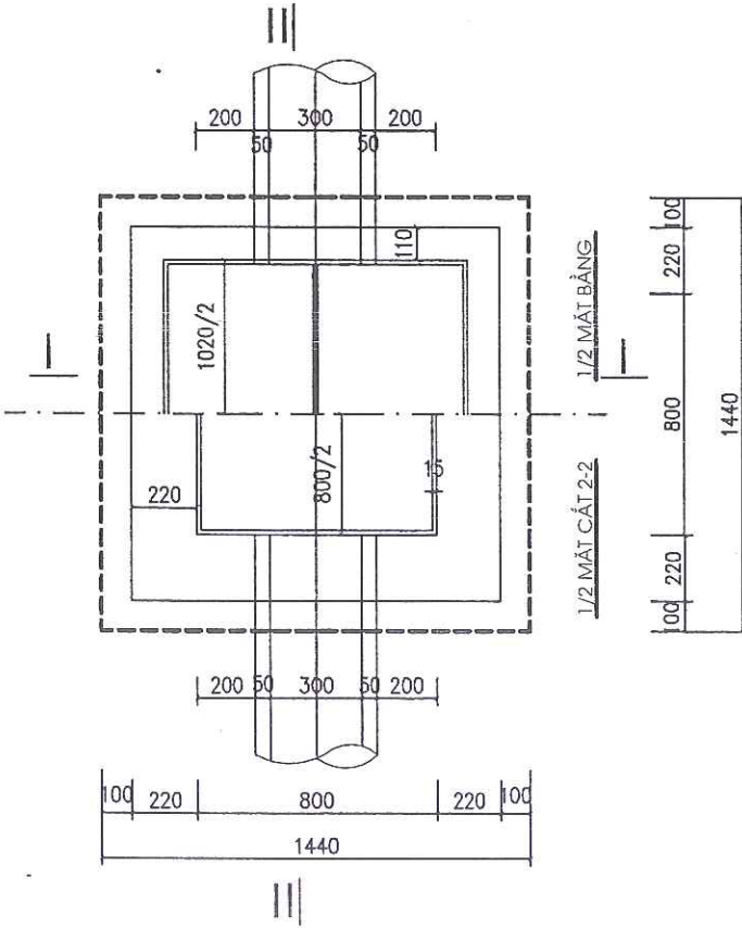
MẶT BẰNG HỒ GA LOẠI 2
