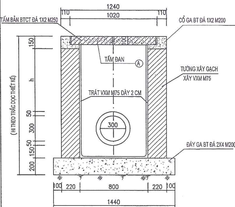
MẶT CẮT 1-1
