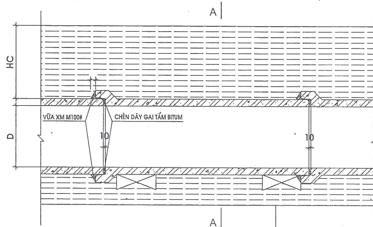
CẮT DỌC TUYẾN CỐNG
