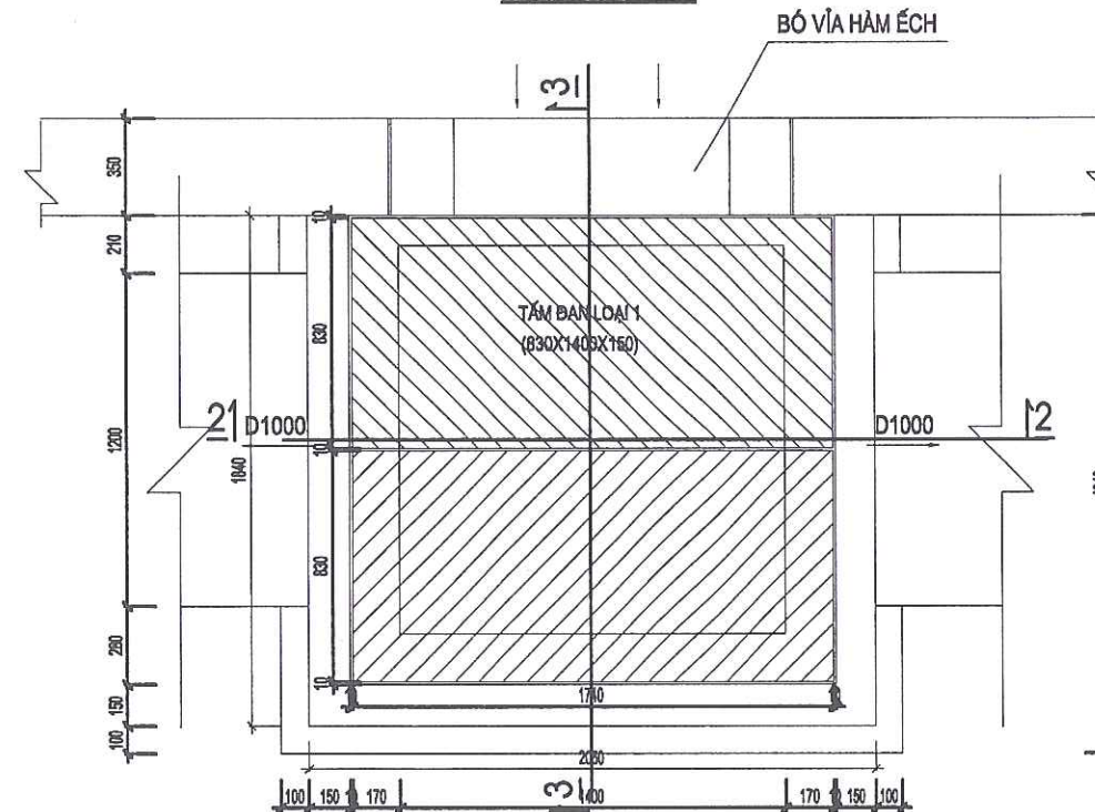
MẶT BẰNG GA
