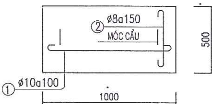
MẶT BẰNG TẤM ĐAN A (18CK)
