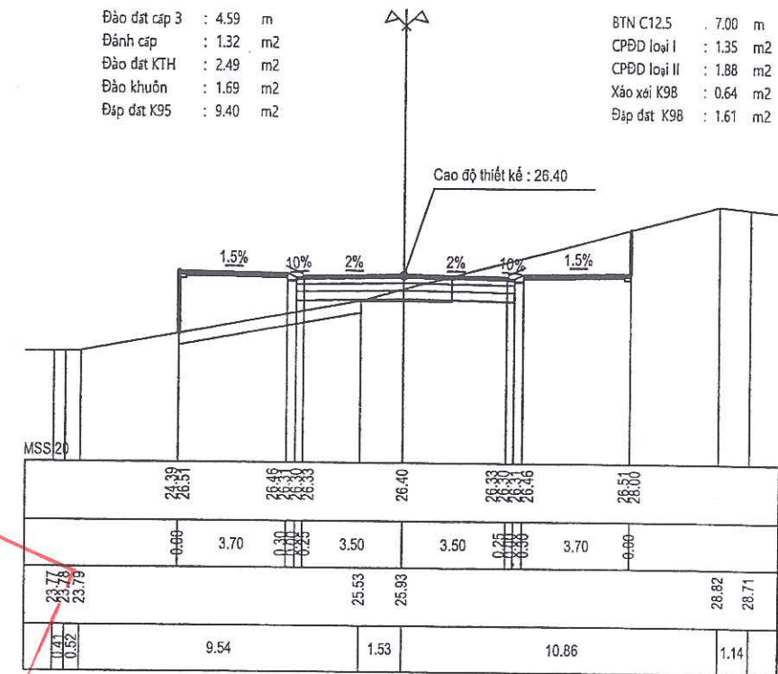
Cọc 8 Km 0 + 131.81
