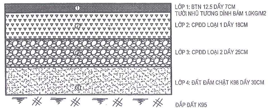
KẾT CẤU MẶT ĐƯỜNG MẶT CẮT 2-2
