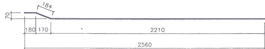
CỐT THÉP SỐ 2
