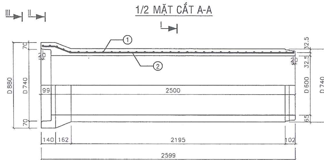
1/2 CHÍNH DIỆN
