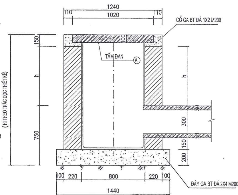
MẶT CẮT II-II
