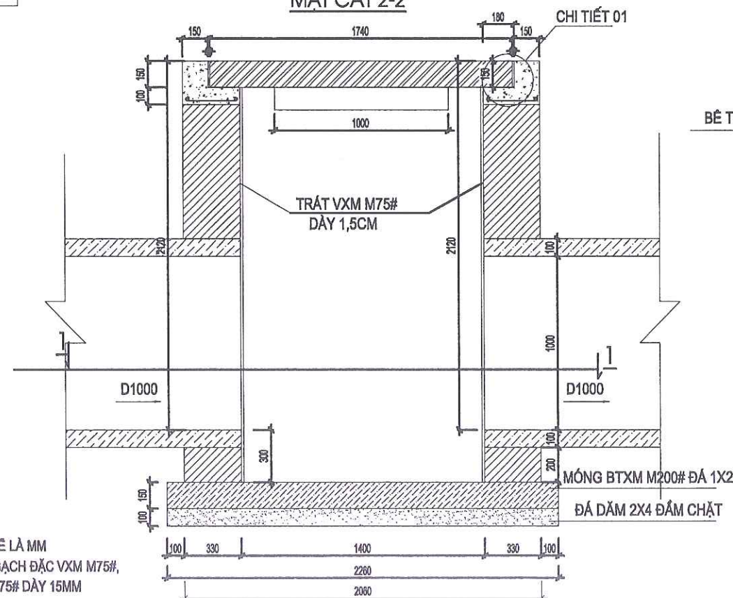
MẶT CẮT 2-2
