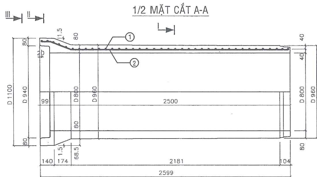
1/2 CHÍNH DIỆN
