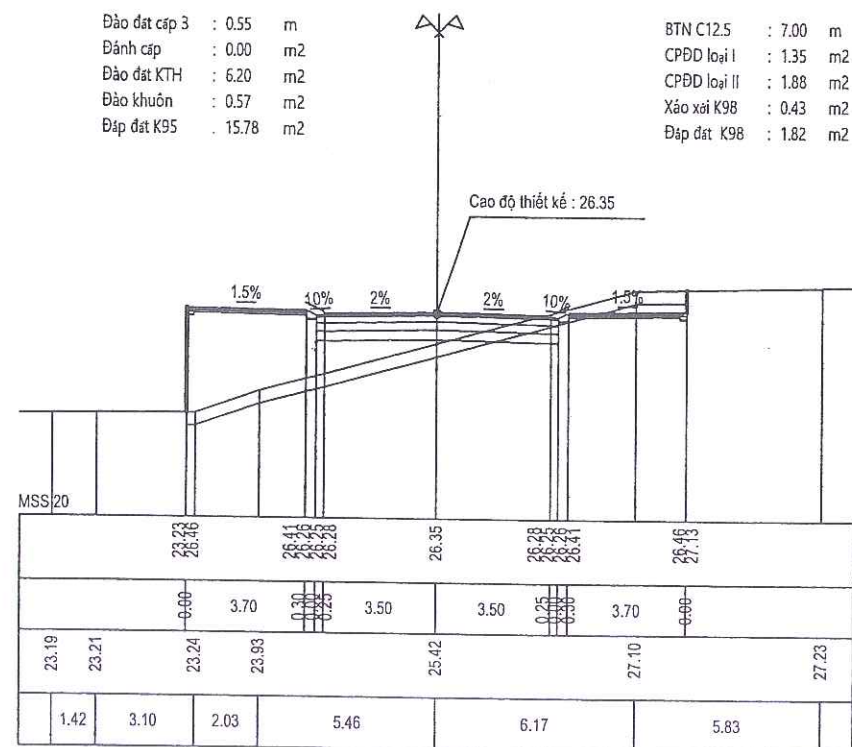
Cọc 9 Km 0 + 150.00
