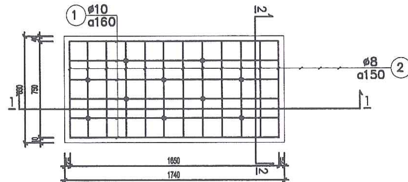
CHI TIẾT TẤM ĐẠN LOẠI 1 ( 1740X830X150)
