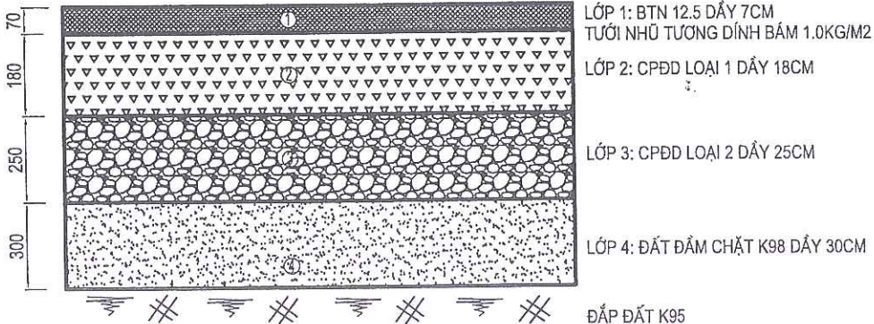
A CẦU MẶT ĐƯỜNG MẶT CẮT 3A-3A
