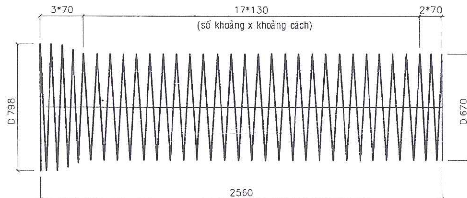
CỐT THÉP SỐ 1
