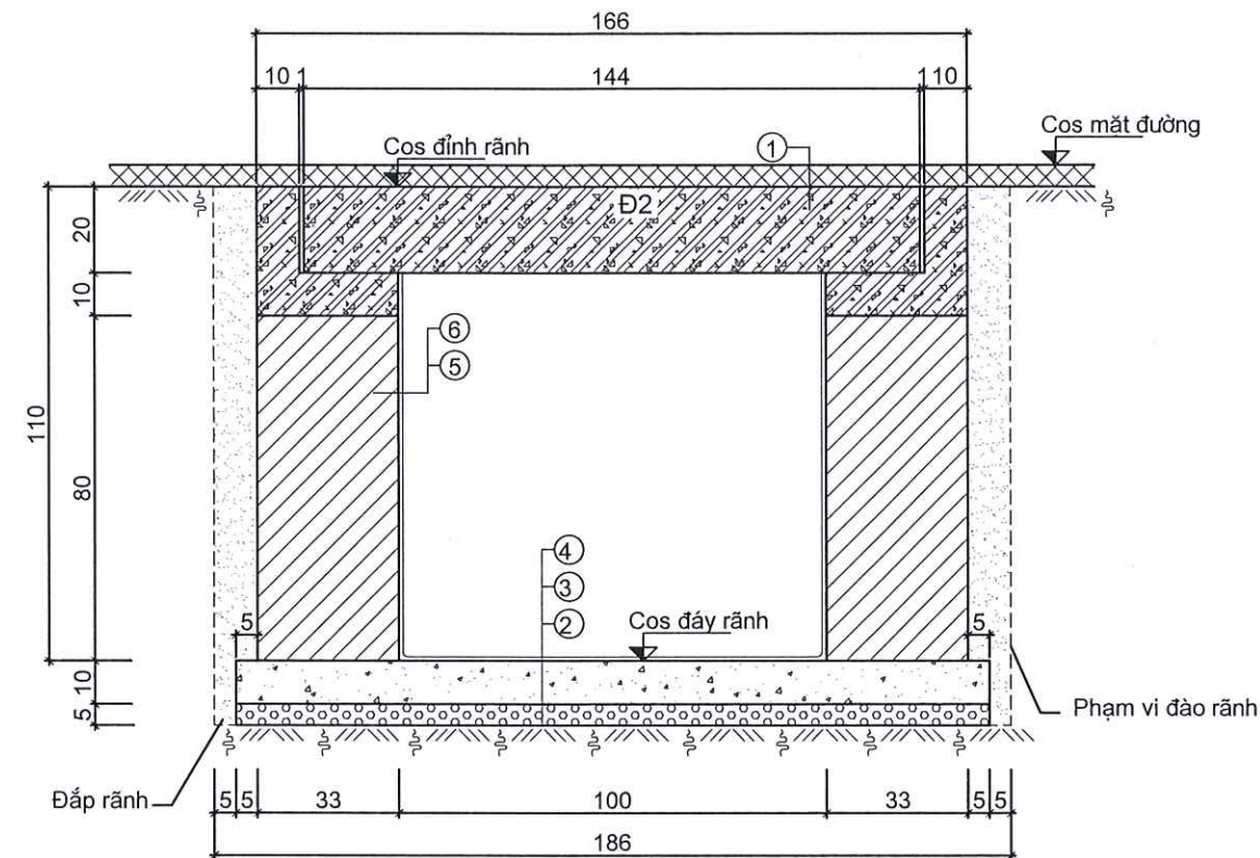
MẶT CẮT 5 - 5
