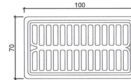
TẦM CHẴN RÁC COMPOSIT 1000X700X70MM (TẢI TRỌNG \geq 12.5T ; SL=03CK)
