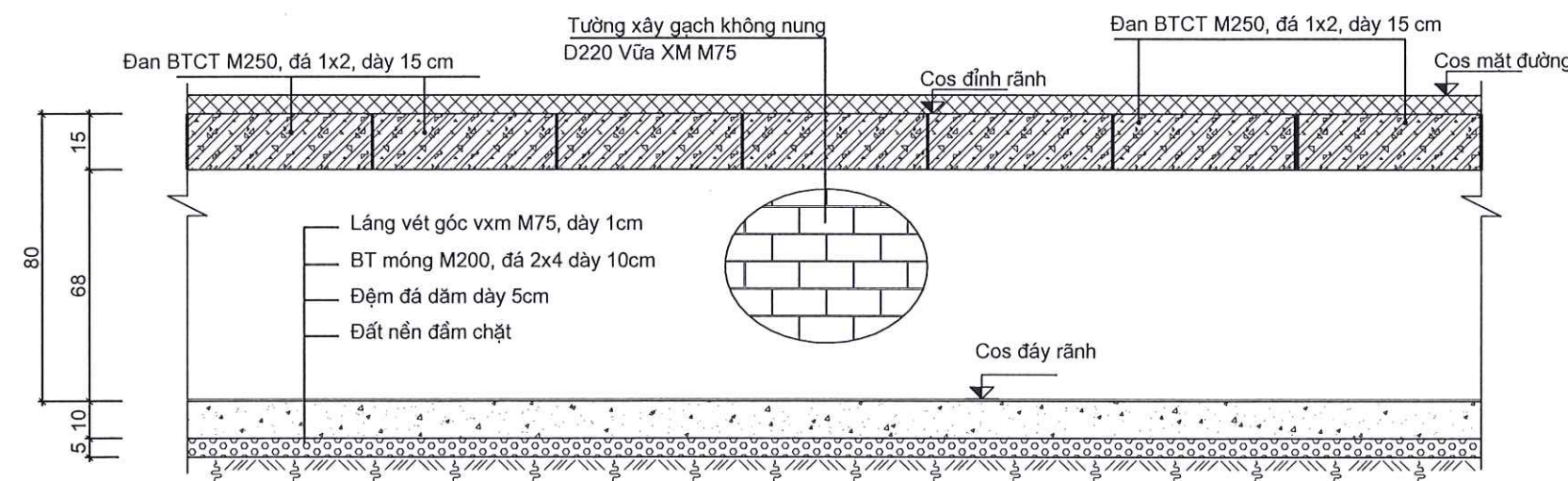
MẶT CẮT 1-1
