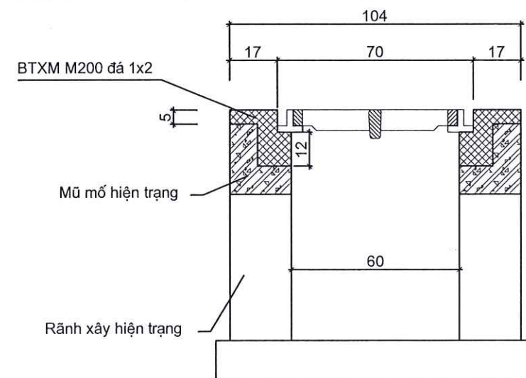
CẮT NGANG GA DẶT TẤM CHẮN RÁC THU NƯỚC (SL=03CK)
