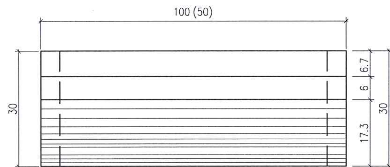
MẶT BẰNG VIÊN VỈA
