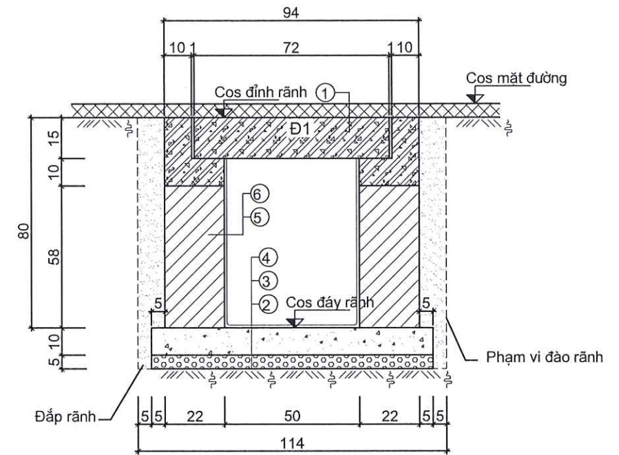
MẶT CẮT 2-2
