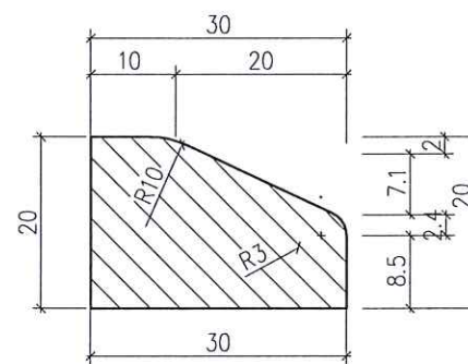
CẮT NGANG VIÊN VỈA
