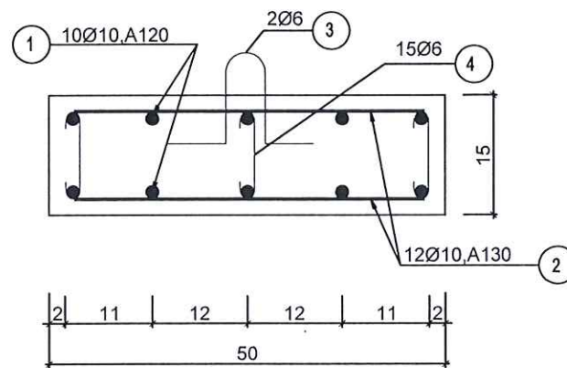
CHI TIẾT TẤM ĐAN D1 (SL=303CK)
