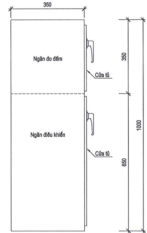
MẶT BÊN TỦ
