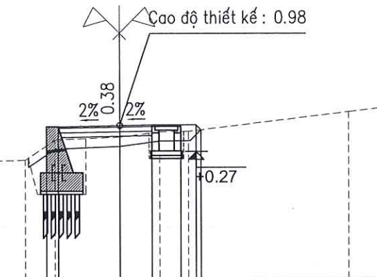
Cọc TC1 Km 0 + 102.24
