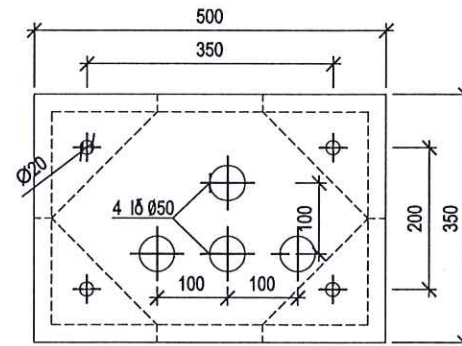
MẶT ĐÁY TỦ
