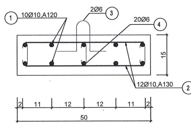
CHI TIẾT TẤM ĐAN D3 (SL= 05CK)
