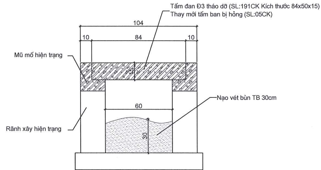
CẮT NGANG HIỆN TRẠNG RÃNH CẢI TẠO TUYẾN NHÁNH (L=95,5M)
