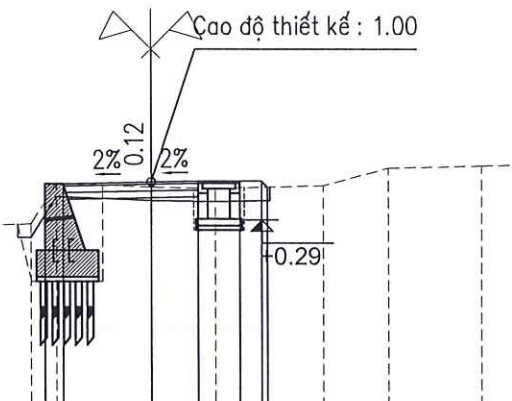
Cọc P1 Km 0 + 94.09
