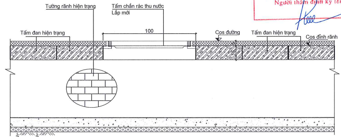
CẮT ĐỌC GA THU NƯỚC (SL=03CK)
