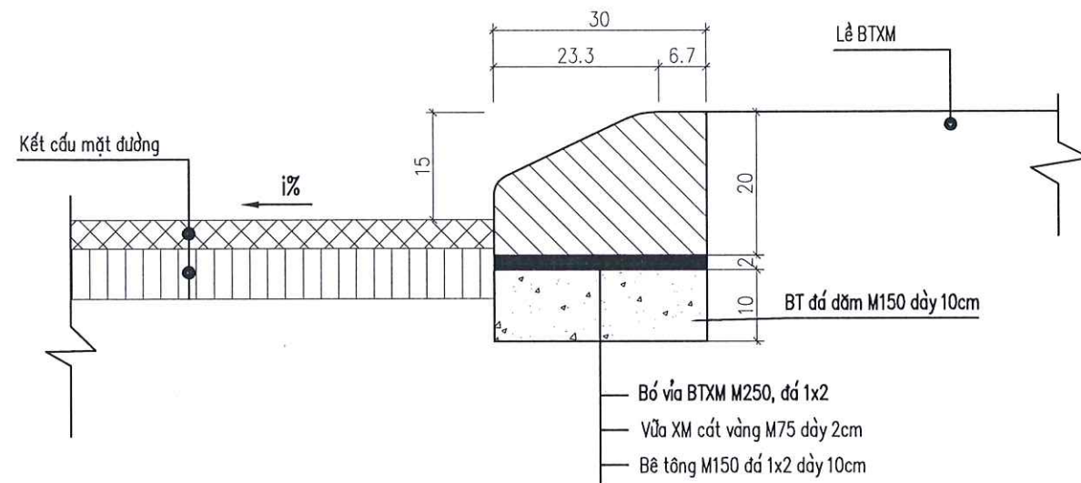
CHI TIẾT BÓ VỈA (L=193.0M)
