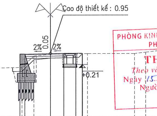
Cọc 8 Km 0 + 127.02
