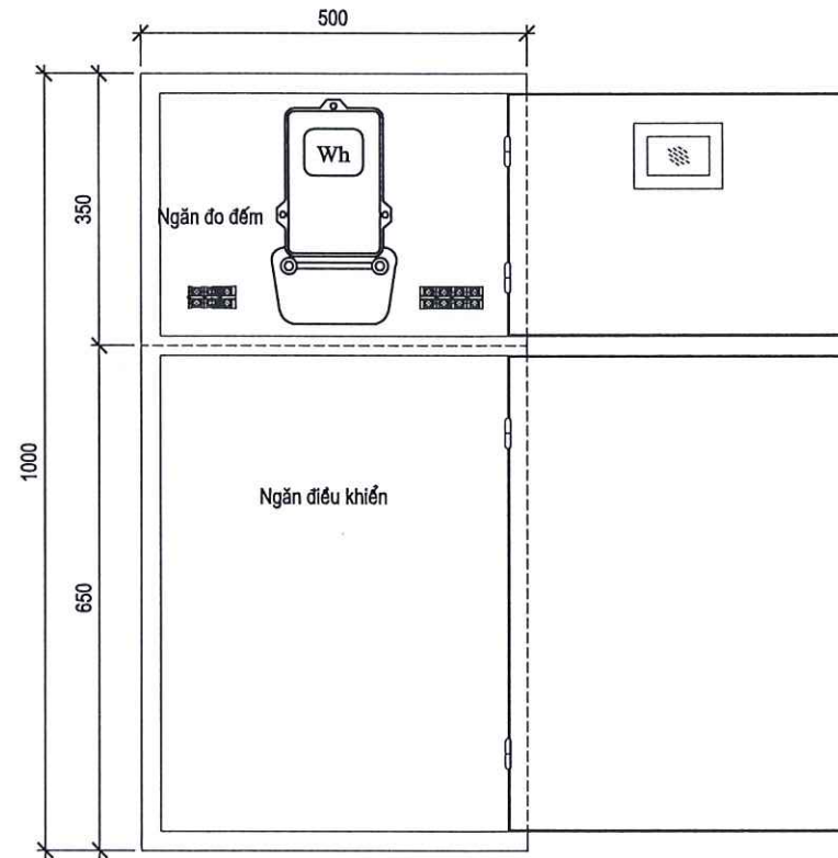
KHAI TRIỂN MẶT TRƯỚC
