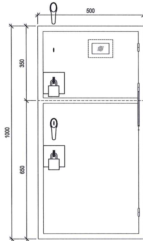
MẶT TRƯỚC TỦ
