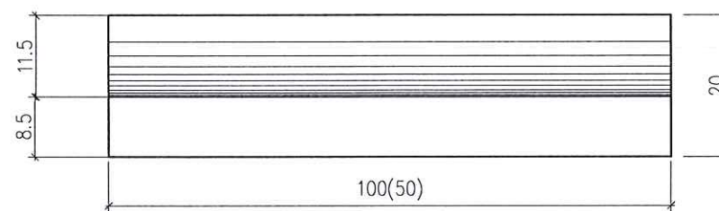
MẶT ĐỨNG VIÊN VỈA
