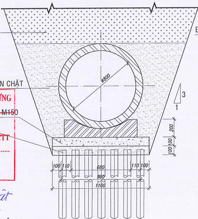
MÓNG CỐNG Ø800 DƯỚI ĐƯỜNG
