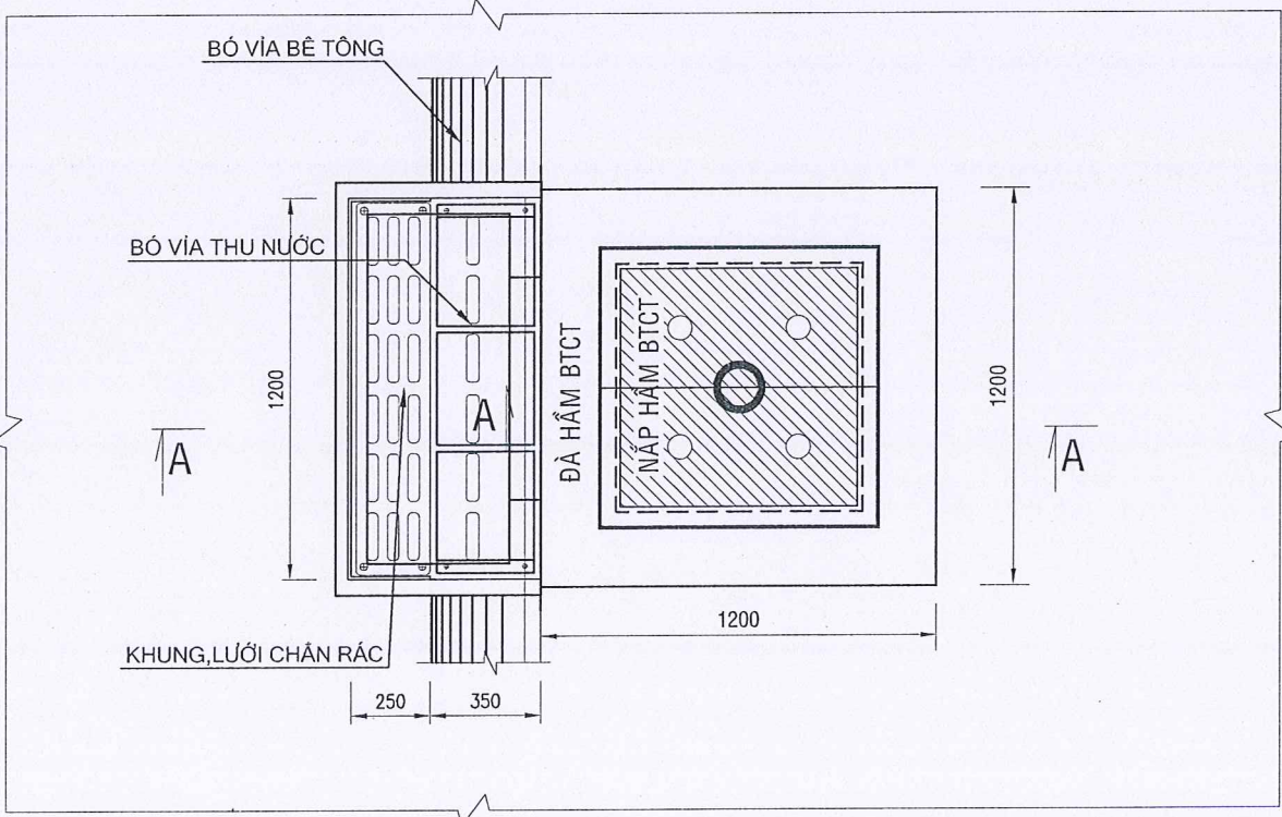
MẶT BẰNG HẦM GA <TL 1/25>
