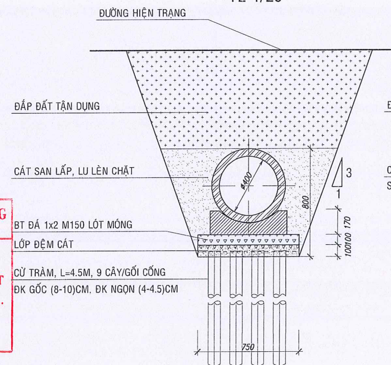
MẶT CẮT NGANG CỐNG 1-1 TL 1/25
