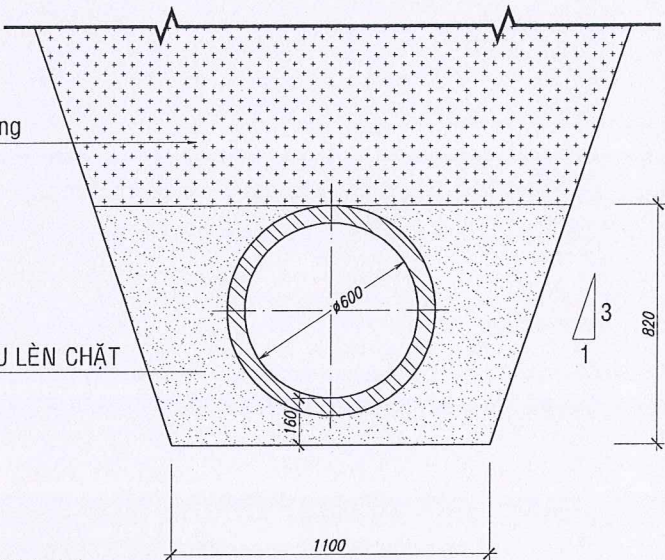
MẶT CẮT 2-2 TL 1/25
