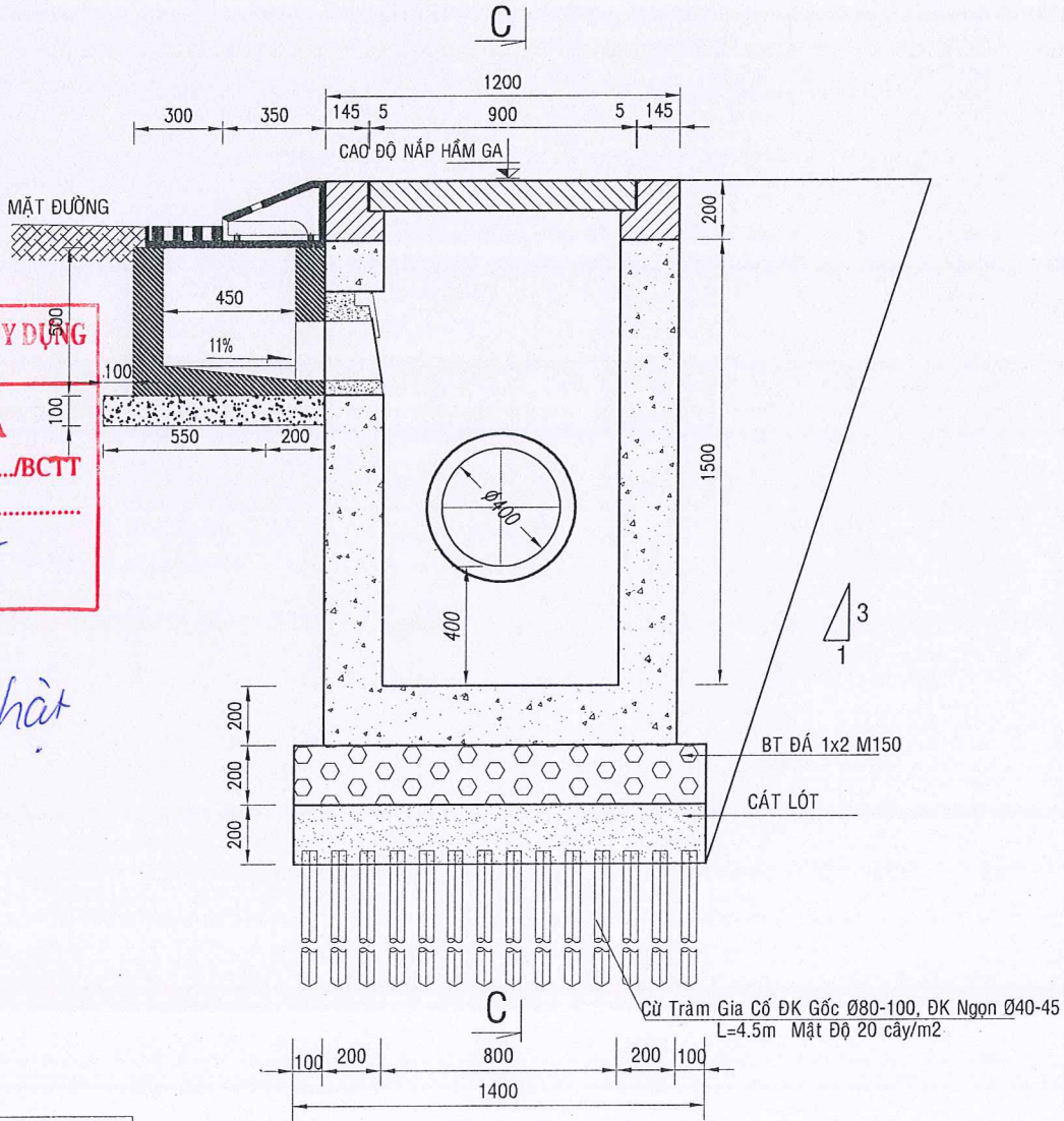
MẶT CẮT A-A
