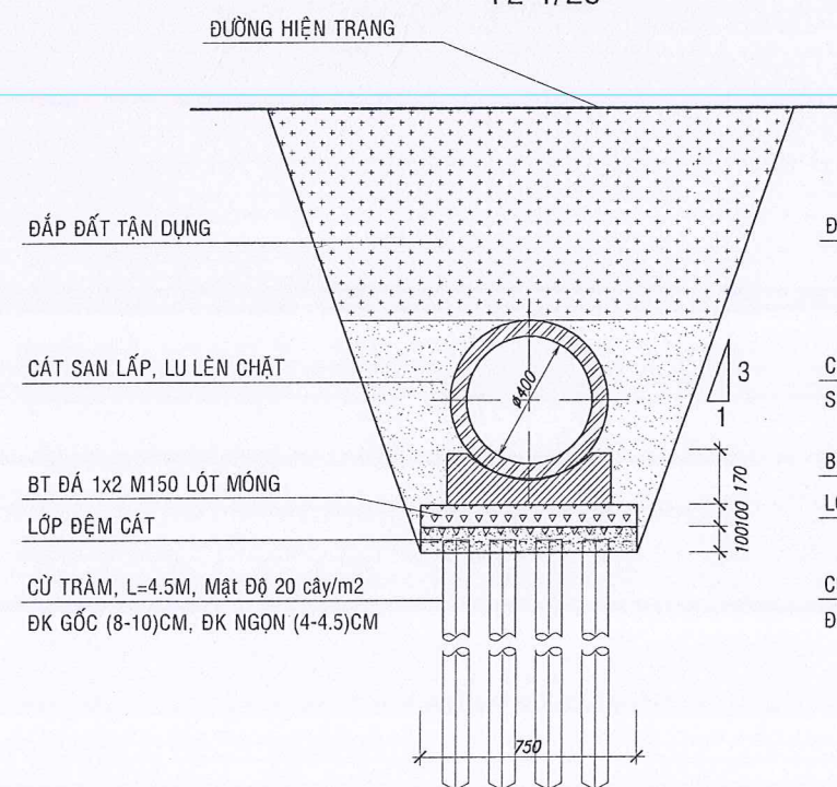
MẶT CẮT NGANG CỐNG 3-3 TL 1/25
