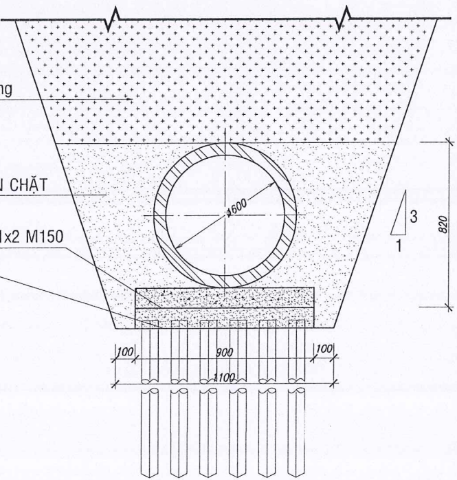
MẶT CẮT 2-2 TL 1/25
