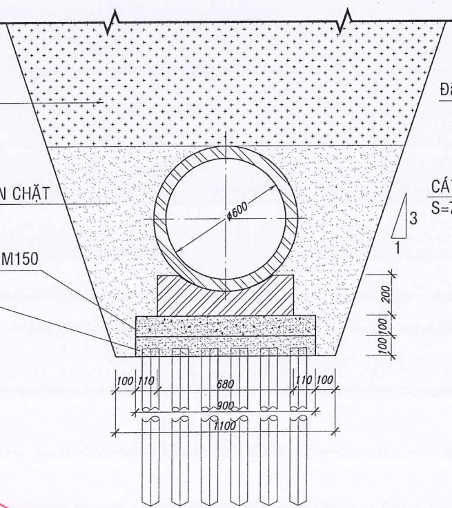
MẶT CẮT 1-1 TL 1/25
