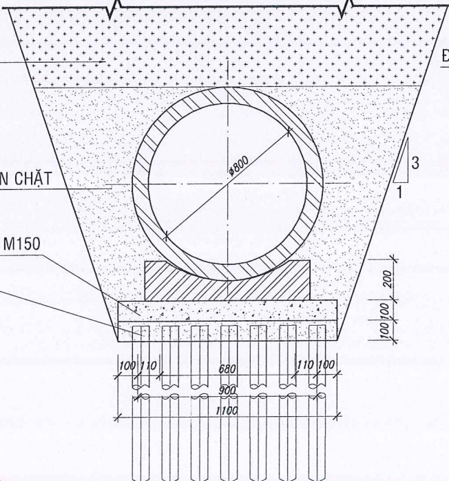
MẶT CẮT 1-1
