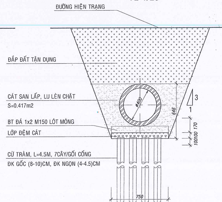
MẶT CẮT NGANG CỐNG 4-4 TL 1/25
