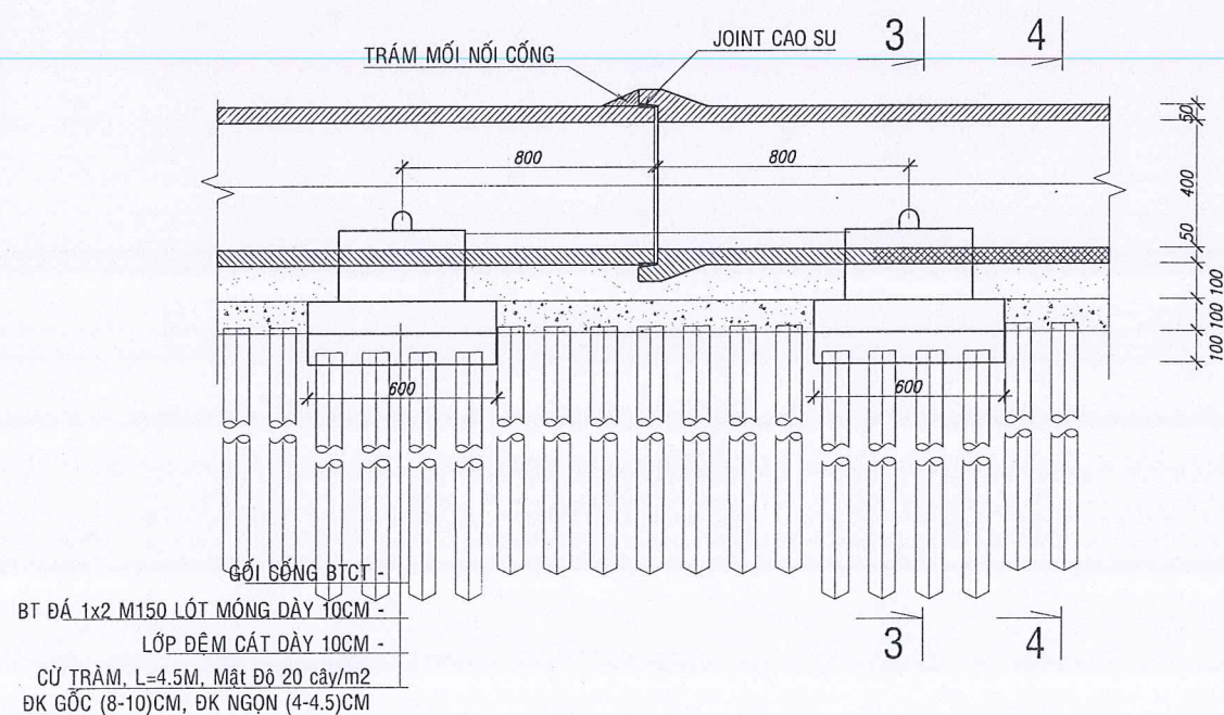
MẶT CẮT DỌC MỘT ĐOẠN CỐNG Ø400 BẰNG ĐƯỜNG TL 1/25
