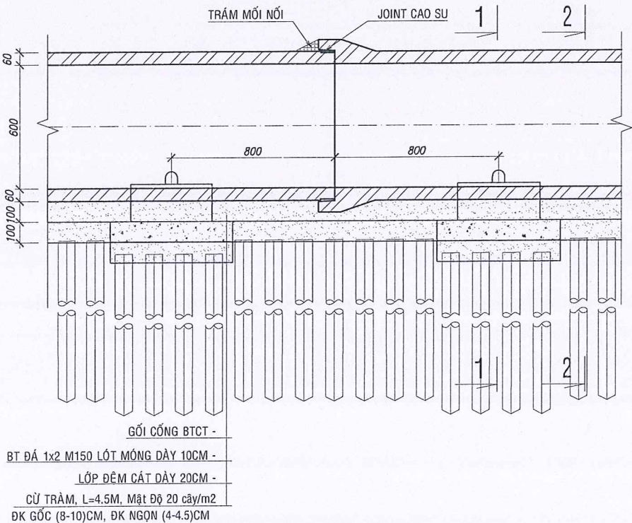
MẶT CẮT DỌC MỘT ĐOẠN CỐNG Ø600 TL 1/25
