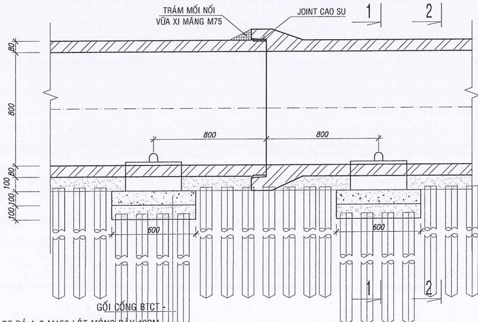
MẶT CẮT DỌC MỘT ĐOẠN CỐNG Ø800
