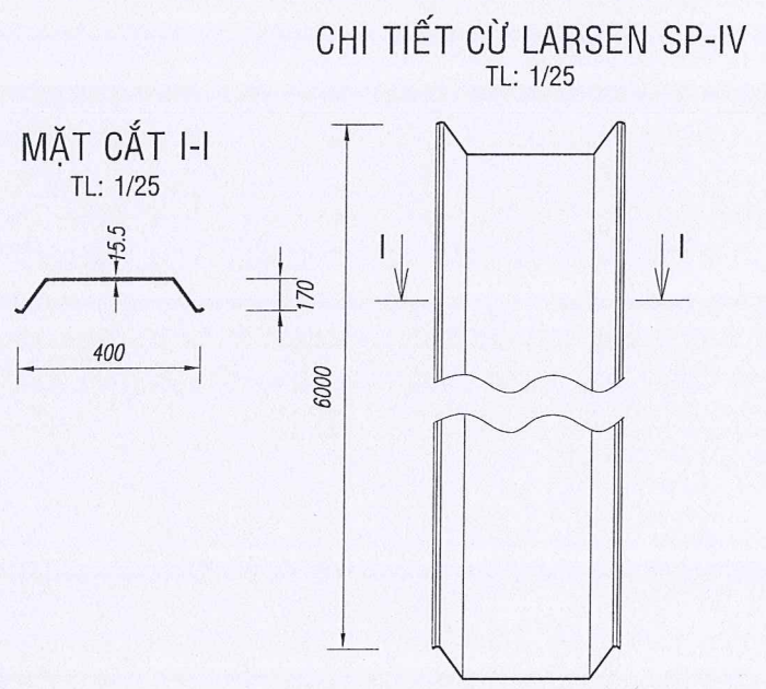
MẶT ĐỨNG CỬ LARSEN
