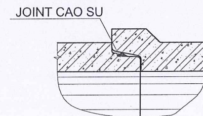
MỐI NỐI
