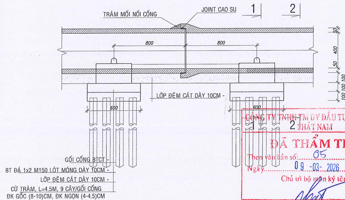
MẶT CẮT DỌC MỘT ĐOẠN CỐNG Ø400 VỈA HÈ TL 1/25
