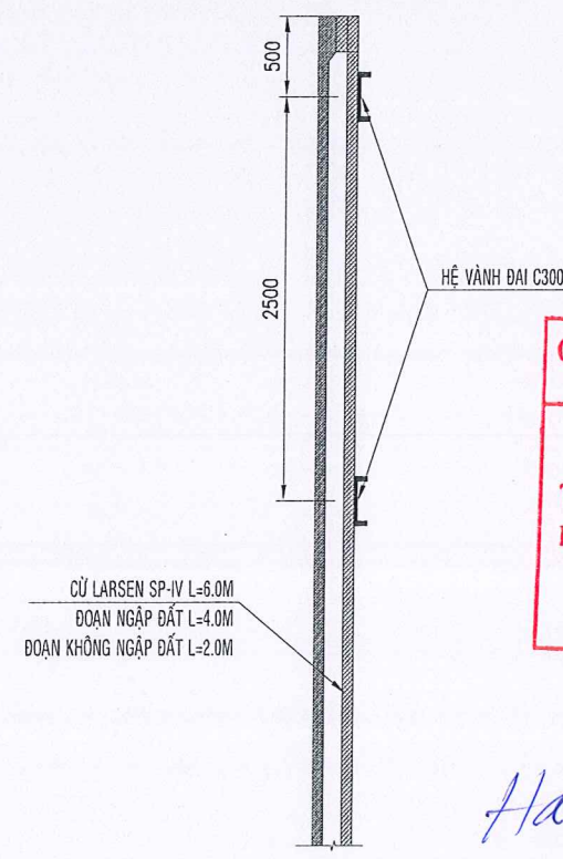
MẶT ĐỨNG CỬ LARSEN
