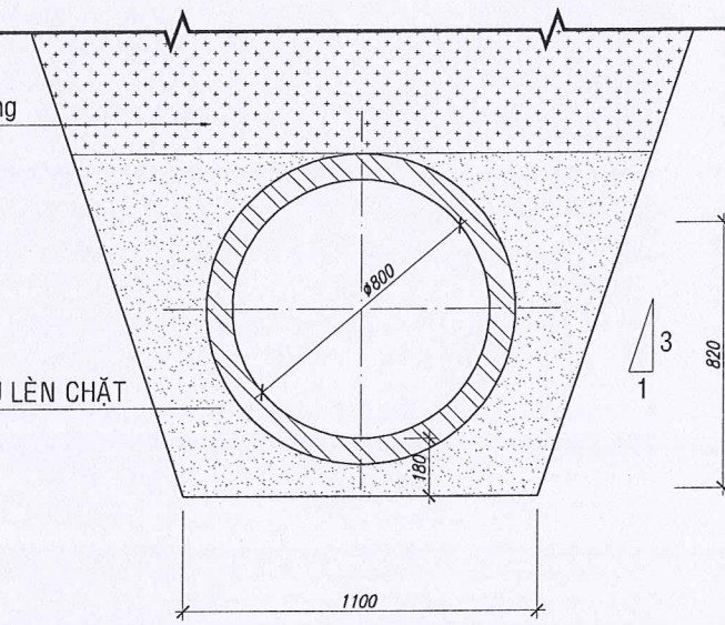
MẶT CẮT 2-2
