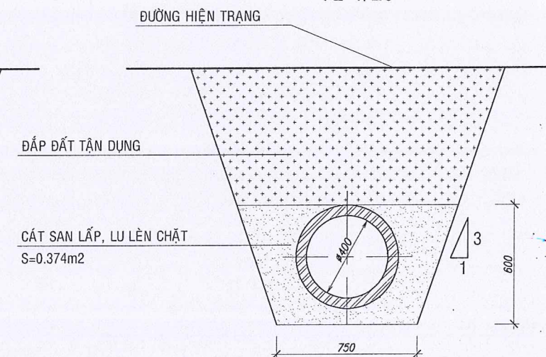
MẶT CẮT NGANG CỐNG 2-2 TL 1/25
