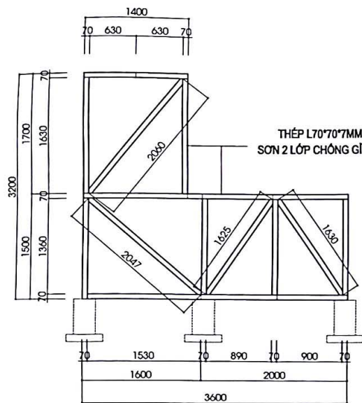
MẶT ĐỨNG 1
