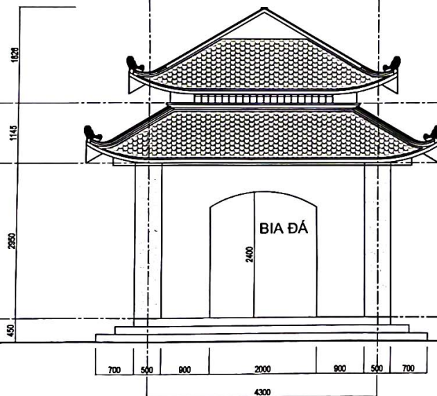
MẶT ĐỨNG
