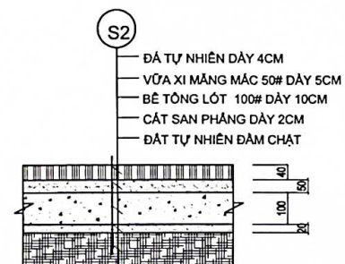
MẶT CẮT KẾT CẤU SÀN LÁT ĐÁ TỰ NHIÊN
