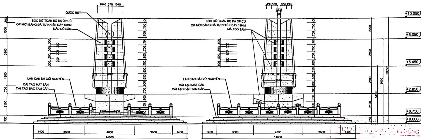
MẶT ĐỨNG TRƯỚC
