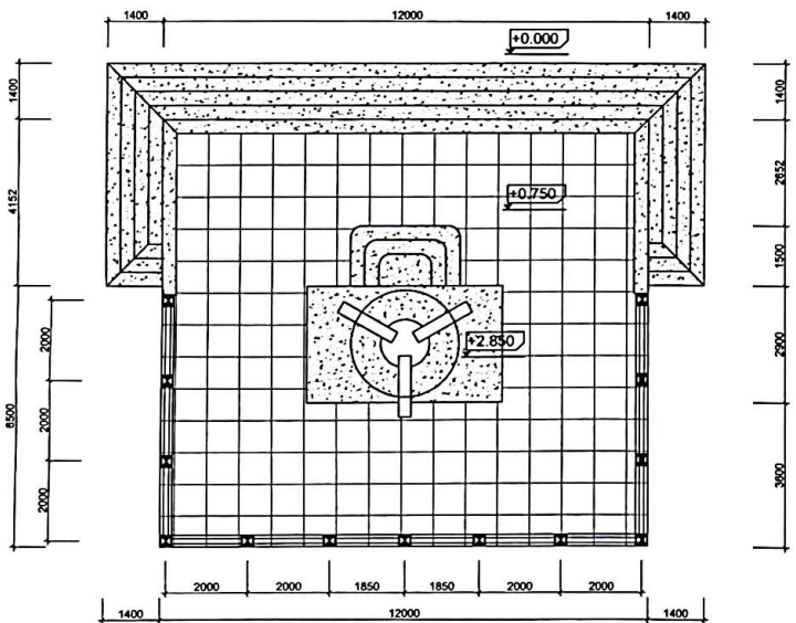
MẶT BẰNG
