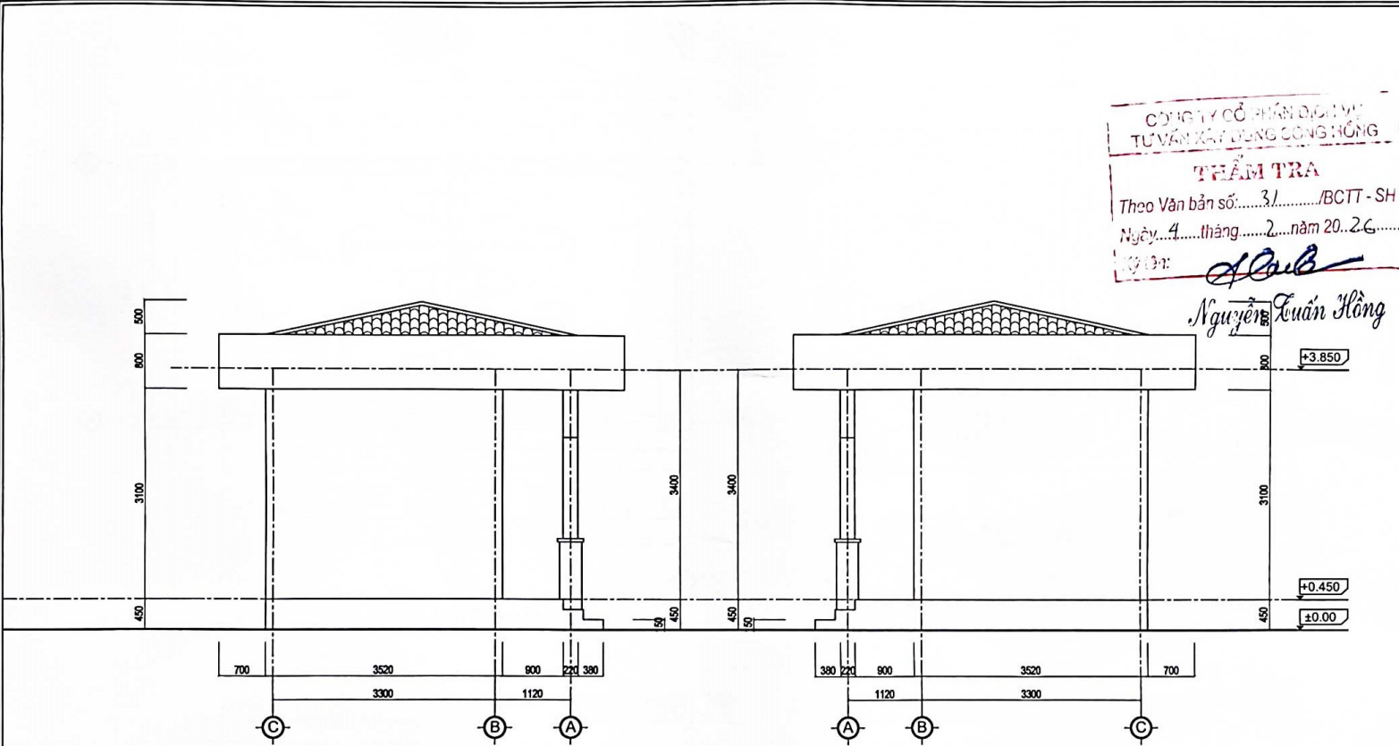
MẶT ĐỨNG TRỤC C-A
