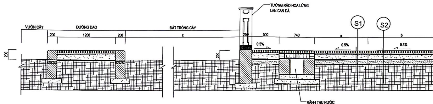
MẶT CẮT 1-1
