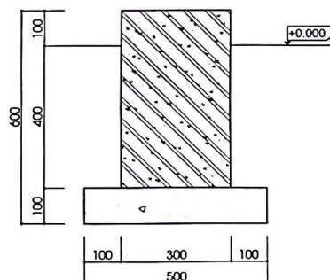
CHÂN BÊ TÔNG ĐỠ (6 CỘT)
