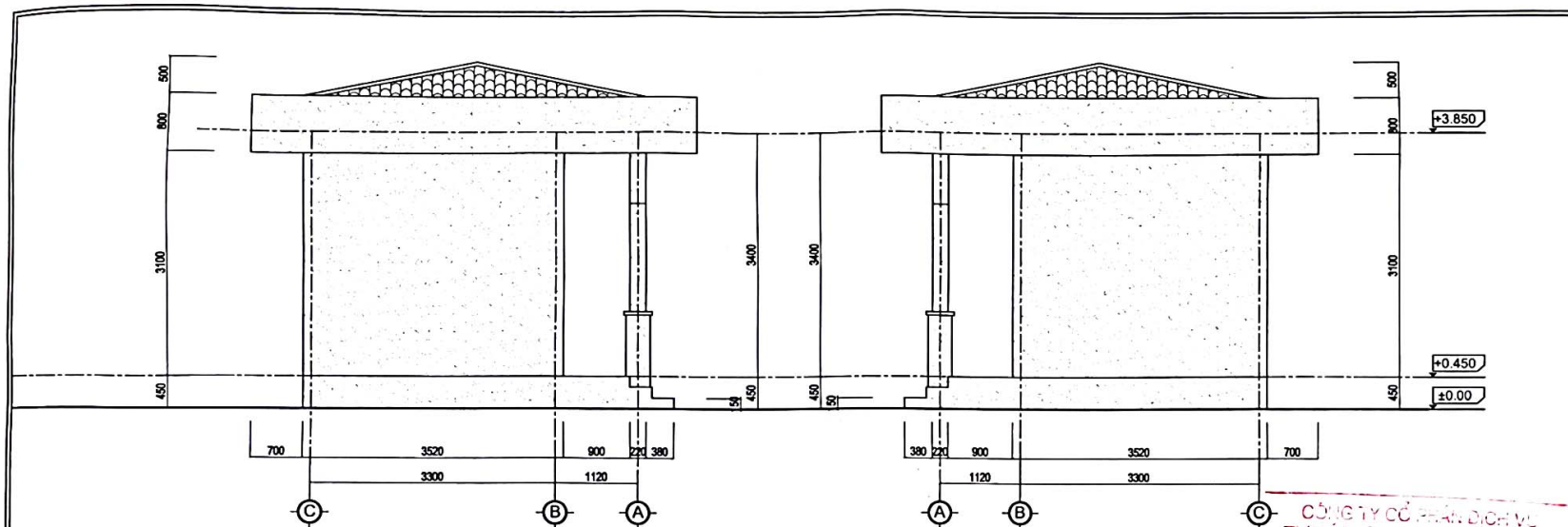
MẶT ĐỨNG TRỰC C-A
