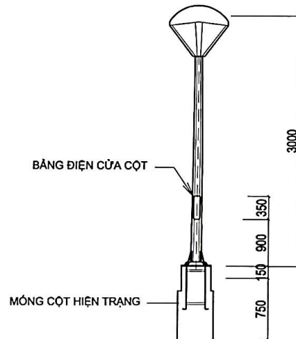
CỘT ĐÈN CHIẾU SÁNG
