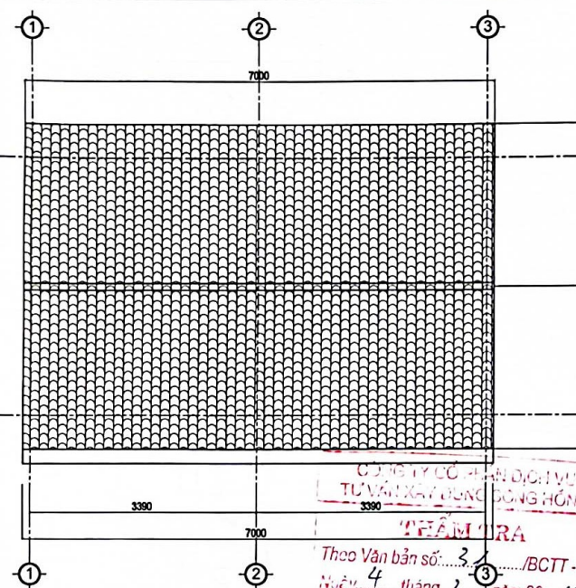
MẶT BẰNG Mái
