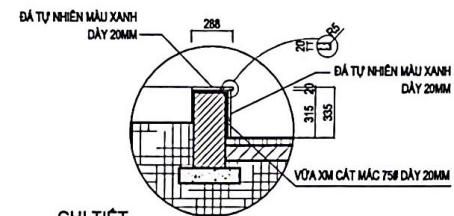
CHI TIẾT
