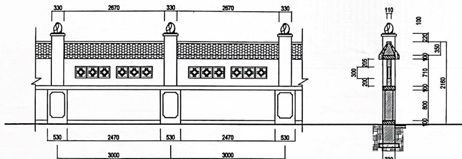
CHI TIẾT HÀNG RÀO KHUÂN VIÊN
