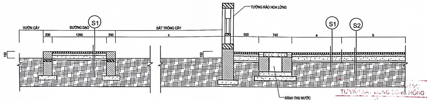
MẶT CẮT 1-1
