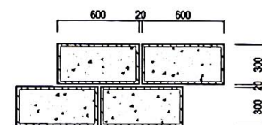
QUY CÁCH LÁT NỀN
