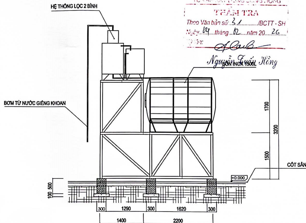
HỆ THỐNG LỌC, BỒN INOX, GIÁ ĐỠ
