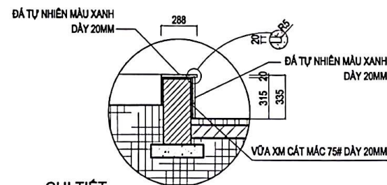
CHI TIẾT
