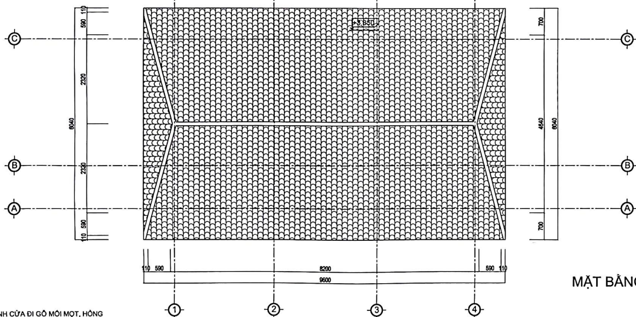
MẶT BẰNG
