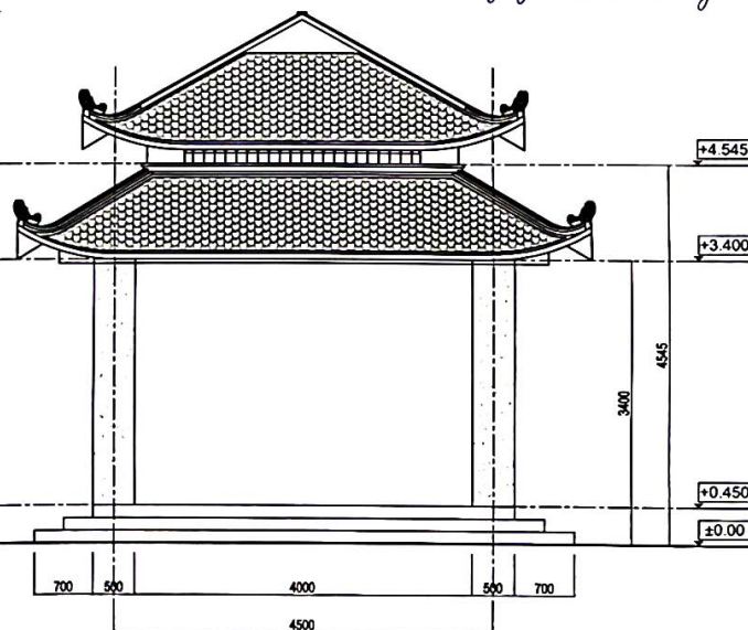
MẶT ĐỨNG
