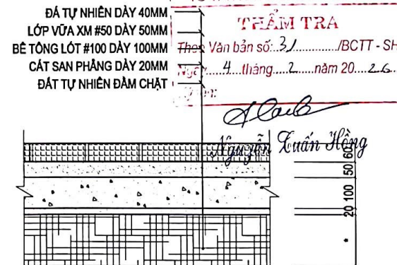
MẶT CẮT SÀN LÁT GẠCH BLOCK HIỆN TRẠNG CAO ĐỘ TRUNG BÌNH 79.20
