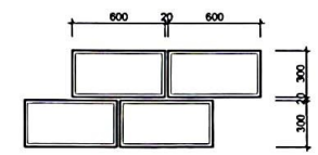
QUY CÁCH LÁT NỀN KỶ ĐÀI
