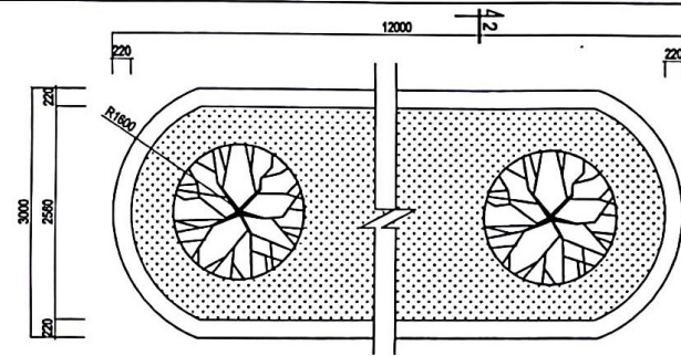
MẶT BẰNG
