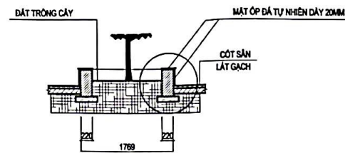
MẶT CẮT 3-3
