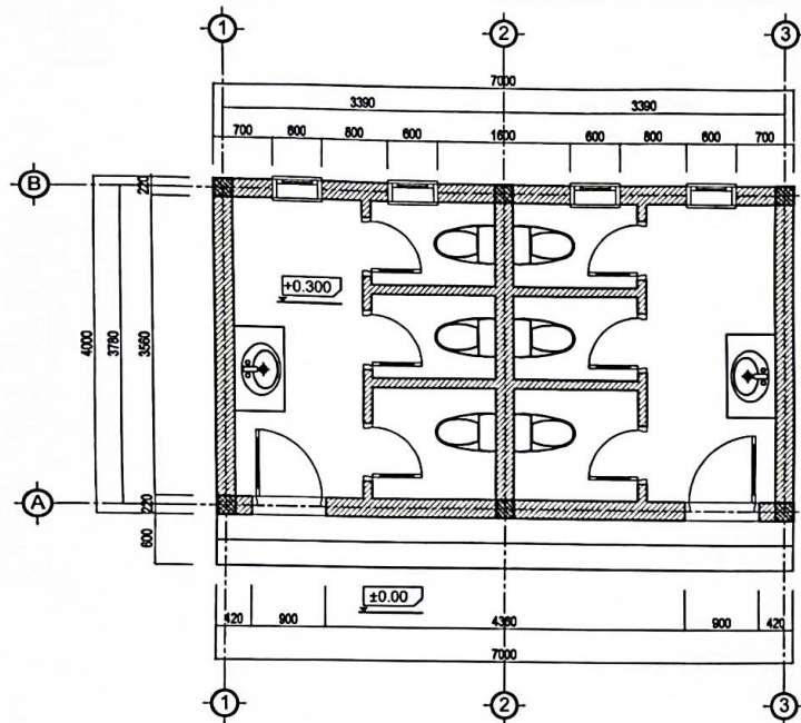
MẶT BẰNG
