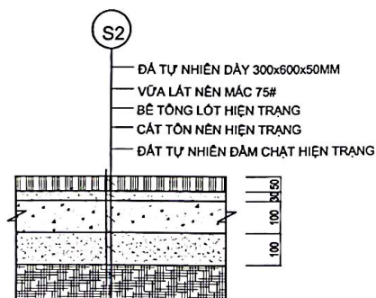
MẶT CẮT KẾT CẤU SÂN S2: 1025M2 (TẬN DỤNG BÊ TÔNG LÓT NỀN CŨ)
