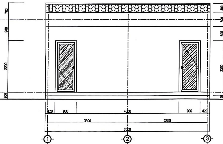
MẶT ĐỨNG TRỰC 1-3
