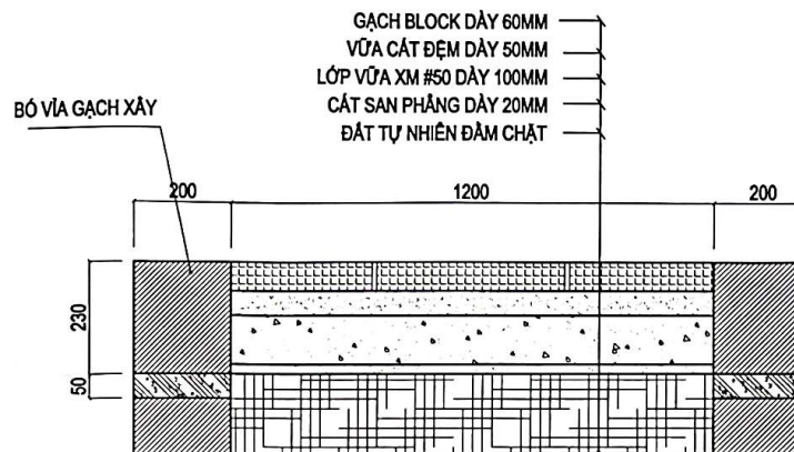
MẶT CẮT ĐƯỜNG ĐẠO LÁT GẠCH BLOCK HIỆN TRẠNG CAO ĐỘ TRUNG BÌNH 78.50
