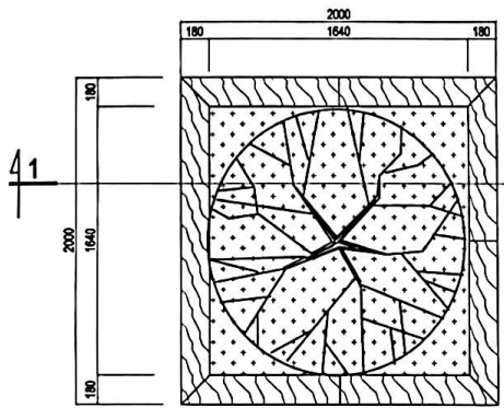
MẶT BẰNG
