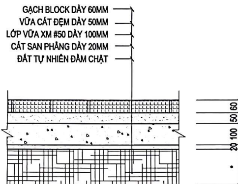
MẶT CẮT SÀN LÁT GẠCH BLOCK HIỆN TRẠNG CAO ĐỘ TRUNG BÌNH 79.00
