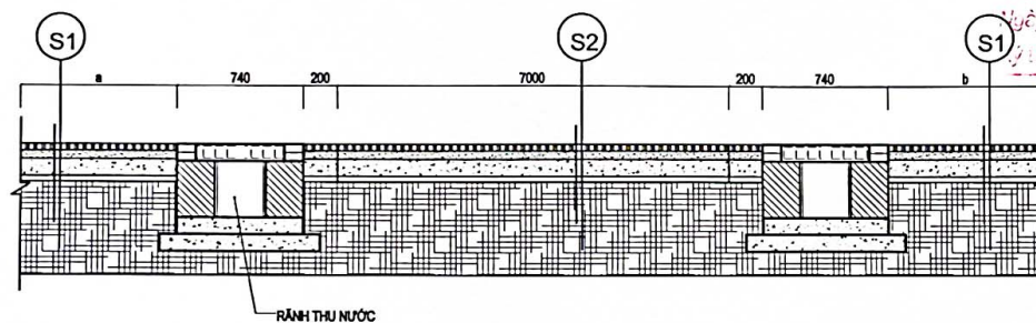
MẶT CẮT 2-2
