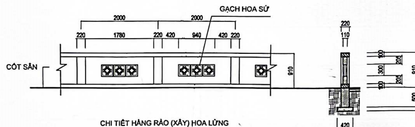
CHI TIẾT HÀNG RÀO (XÂY) HOA LỬNG
