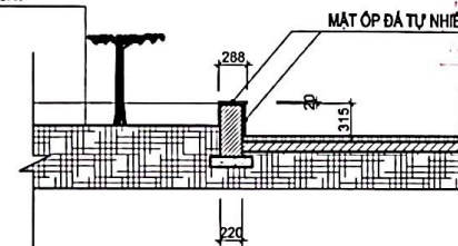
MẶT CẮT 1-1
