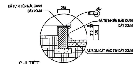
CHI TIẾT
