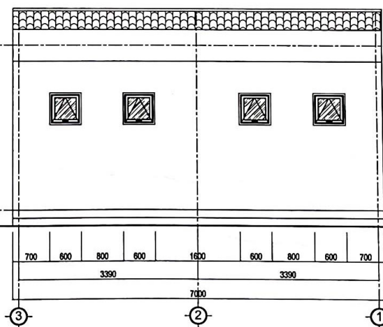
MẶT ĐỨNG TRỰC 3-1
