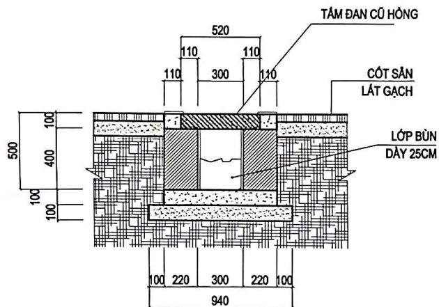
MẶT CẮT RÃNH THOÁT NƯỚC HIỆN TRẠNG
