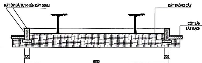
MẶT CẮT 1-1
