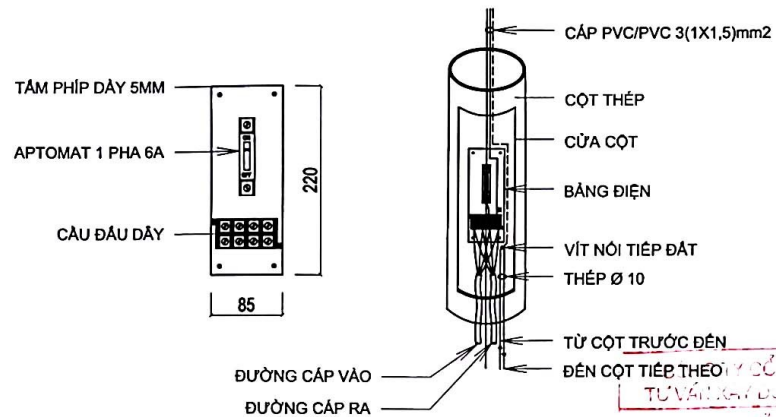
BẢNG ĐIỆN CỬA CỘT ĐÈN CHIẾU SÁNG
