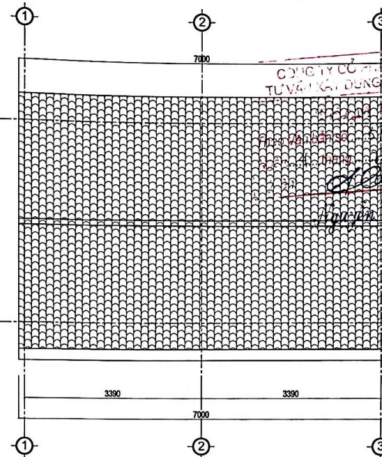
MẶT BẰNG MÁI
