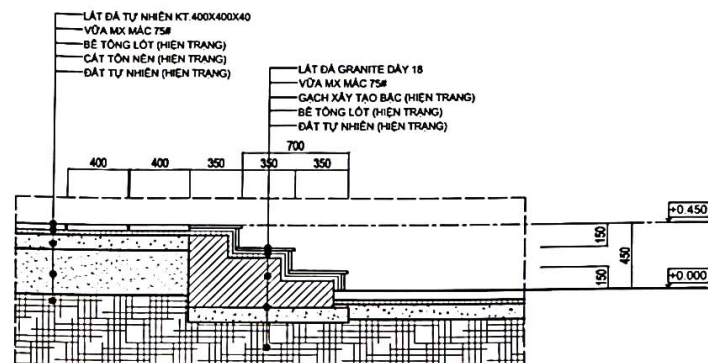
CHI TIẾT
