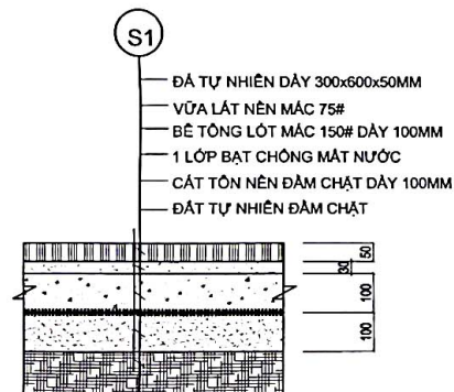
MẶT CẮT KẾT CẤU SÂN S1: 3561M2
