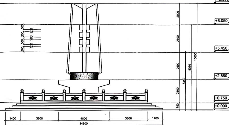
MẶT ĐỨNG SAU
