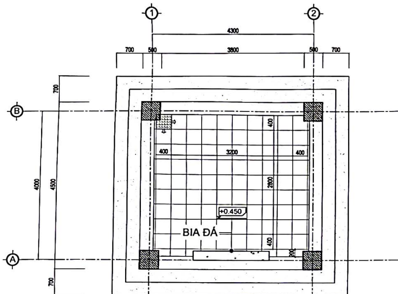
MẶT BẰNG
