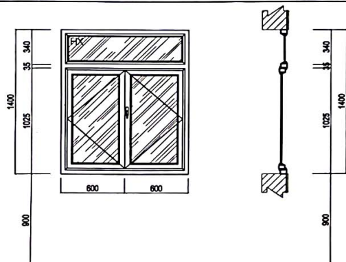
CHI TIẾT CỬA SỔ
