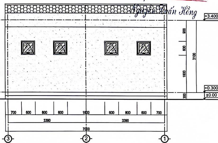
MẶT ĐỨNG TRỰC 3-1
