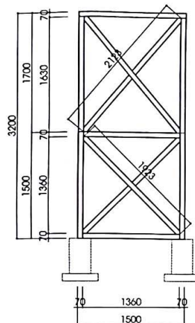
MẶT ĐỨNG 2
