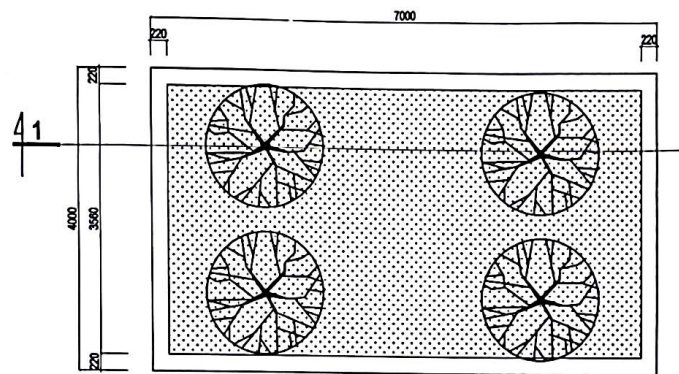
MẶT BẰNG
