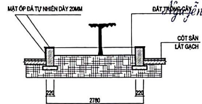
MẶT CẮT 2-2
