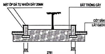
MẶT CẮT 2-2
