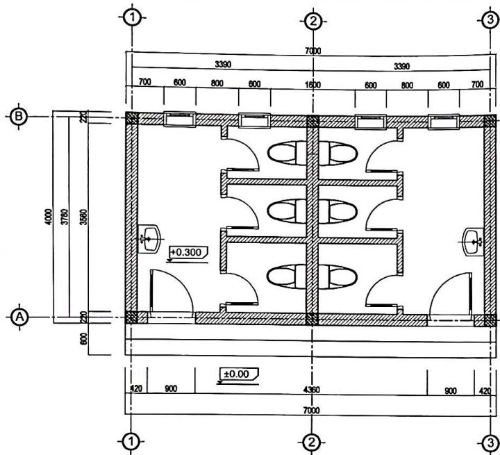
MẶT BẰNG
