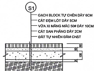
MẶT CẮT KẾT CẤU SÀN LÁT GẠCH BLOCK TỰ CHÈN
