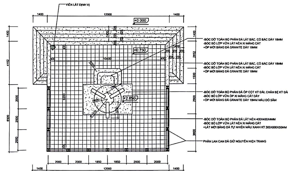
MẶT BẰNG
