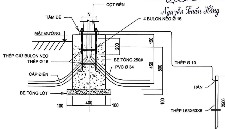
CHI TIẾT CHÂN CỘT ĐÈN 02 BỘ LÂM MỚI
