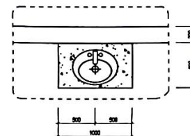
MẶT BẰNG BÀN ĐÁ (SL=02CK)
