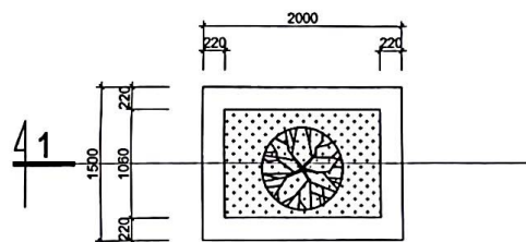
MẶT BẰNG
