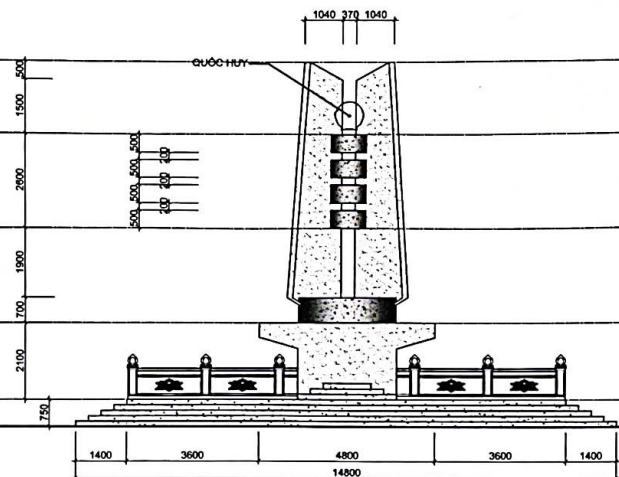
MẶT ĐỨNG TRƯỚC
