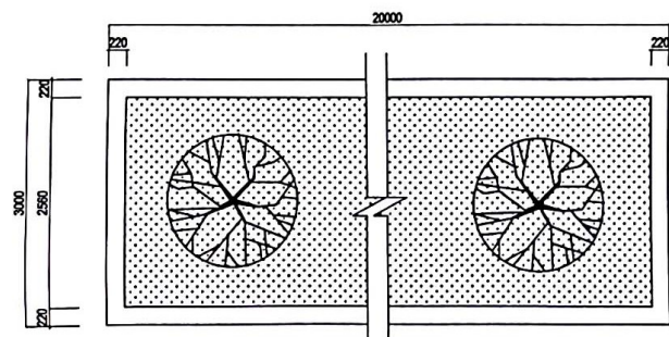
MẶT BẰNG
