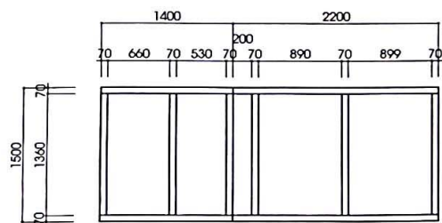
MẶT BẰNG
