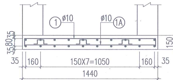
MẶT CẮT: 2-2
