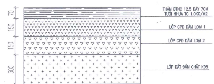
KẾT CẤU NỀN MẶT ĐƯỜNG LOẠI 3 – KC3
