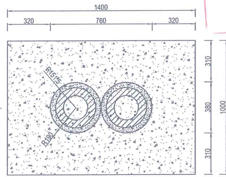
MẶT BẰNG MÓNG
