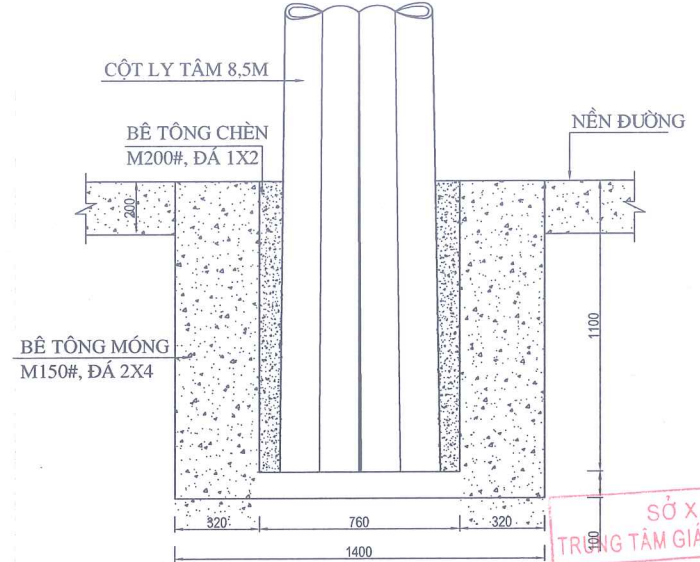
MẶT ĐỨNG MÓNG
