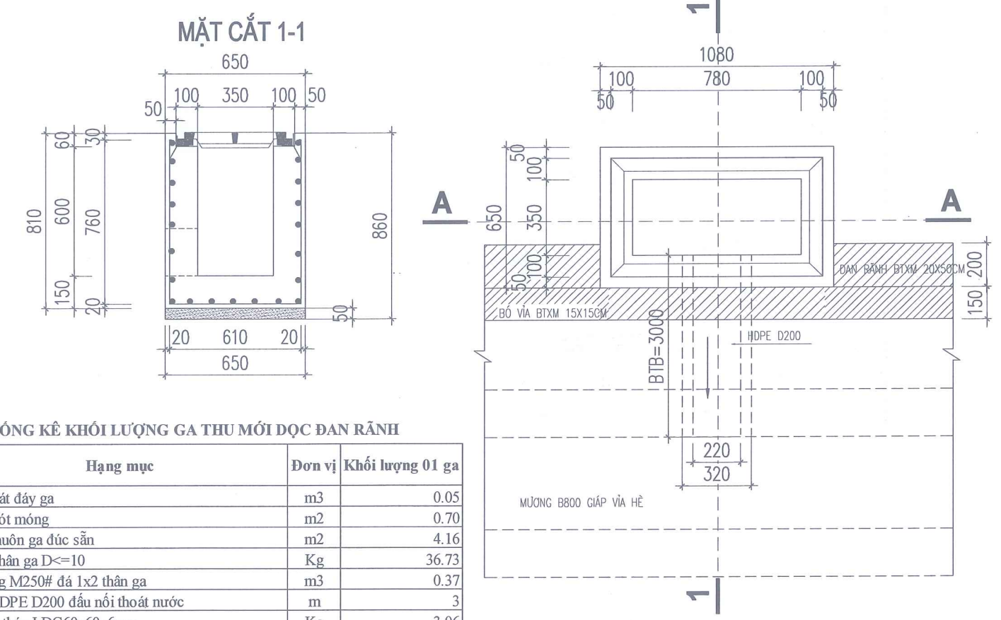
MẶT BẰNG GA THU NƯỚC DỌC HÈ-GS1
