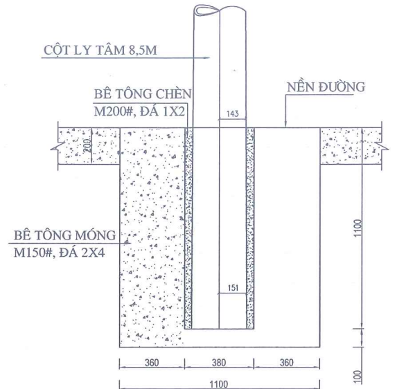
MẶT ĐỨNG MÓNG
