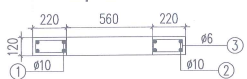
MẶT CẮT 1-1
