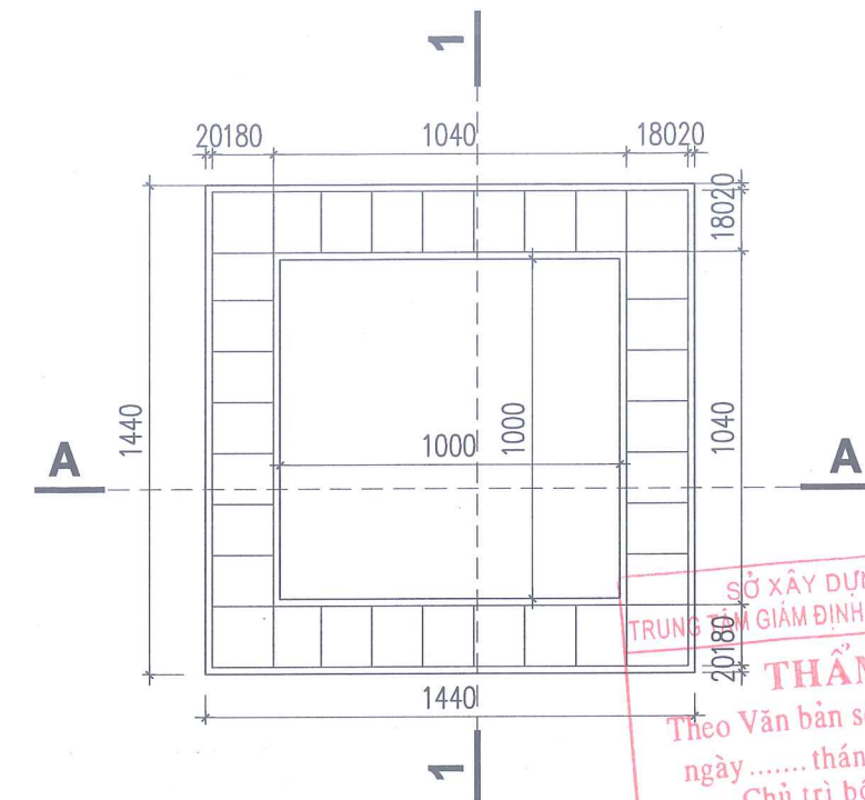
MẶT BẰNG CỐT THÉP GIẰNG GA 15X22CM
