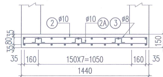
MẶT CẮT: 2-2
