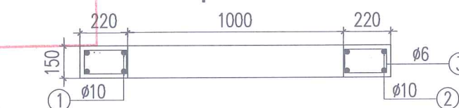
MẶT CẮT 1-1
