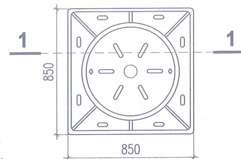
CHI TIẾT NẮP GA COMPOSITE
