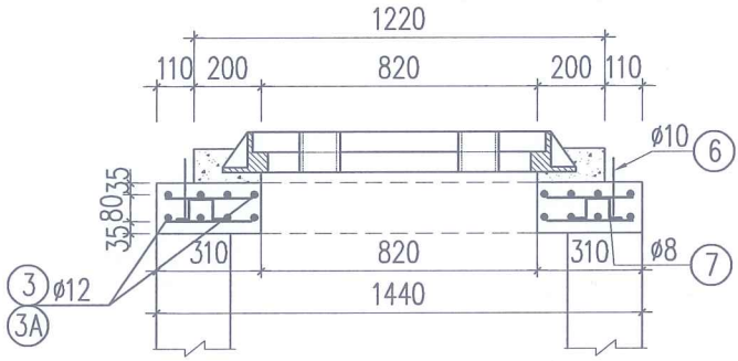
MẶT CẮT: 2-2
