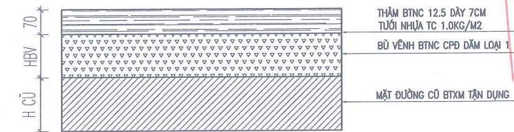
KẾT CẤU NỀN MẶT ĐƯỜNG LOẠI 2 – KC2
