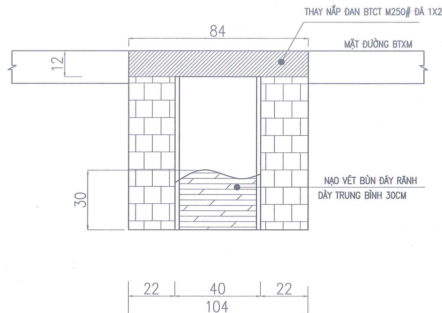
MẶT CẮT NGANG RÃNH B400
