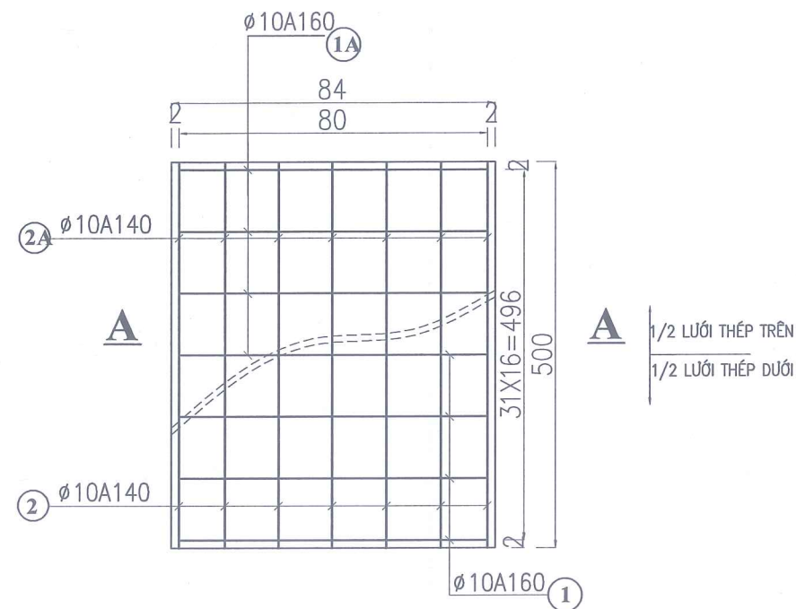
BỐ TRÍ THÉP TẤM ĐAN RÃNH B400 ĐƠN NGUYÊN 5M/CK
