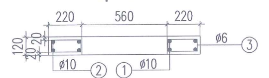
MẶT CẮT 1-1
