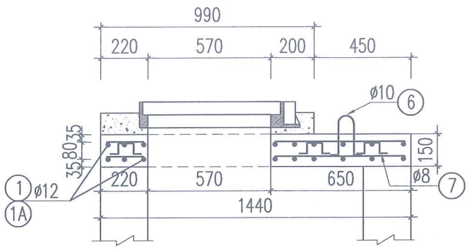
MẶT CẮT: 1-1
