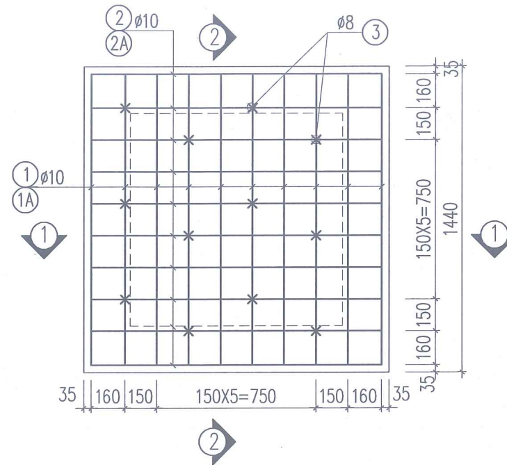
MẶT BẰNG CỐT THÉP BẢN ĐÁY (CỐT THÉP LƯỚI TRÊN + LƯỚI DƯỚI)
