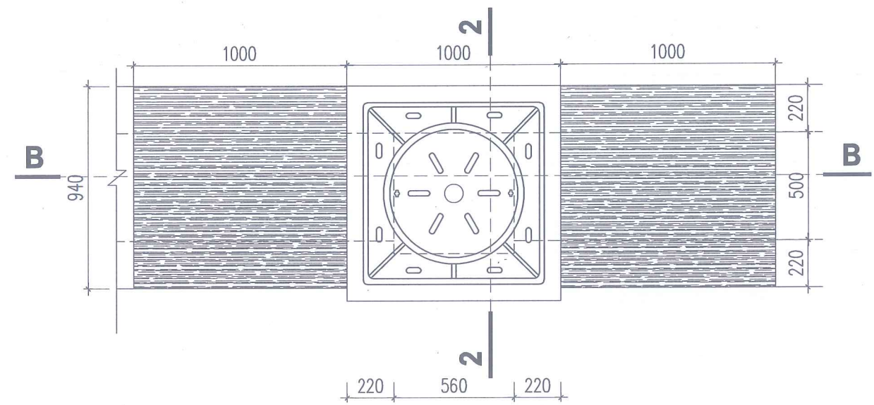
MẶT BẰNG HỐ GA TRÊN RĂNG CŨ B500-GB5
