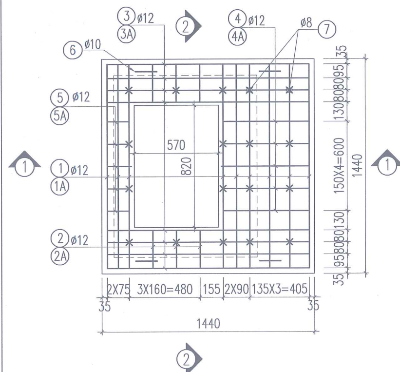
MẶT BẰNG CỐT THÉP TẤM ĐAN (CỐT THÉP LƯỚI TRÊN + LƯỚI DƯỚI)
