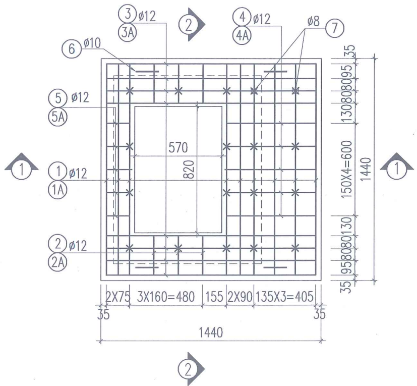
MẶT BẰNG CỐT THÉP TẦM ĐÀN (CỐT THÉP LƯỚI TRÊN + LƯỚI DƯỚI)
