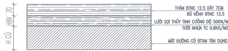
KẾT CẤU NỀN MẶT ĐƯỜNG LOẠI 1 – KC1
