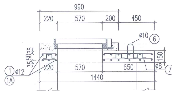
MẶT CẮT: 1-1
