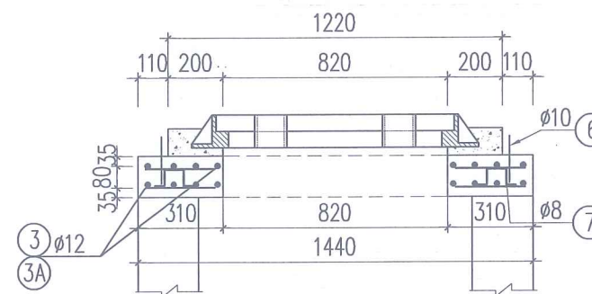
MẶT CẮT: 2-2
