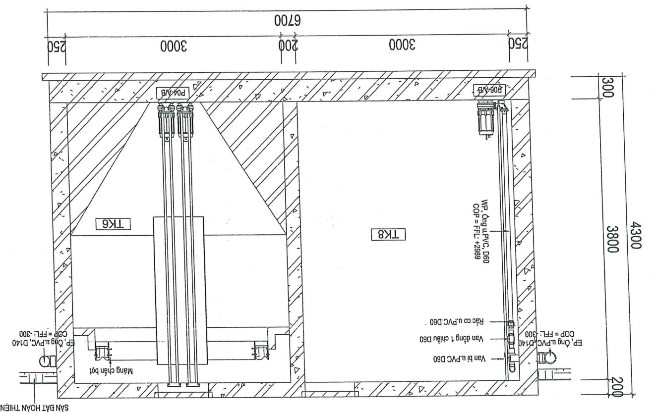
MẶT CẮT 9-9
