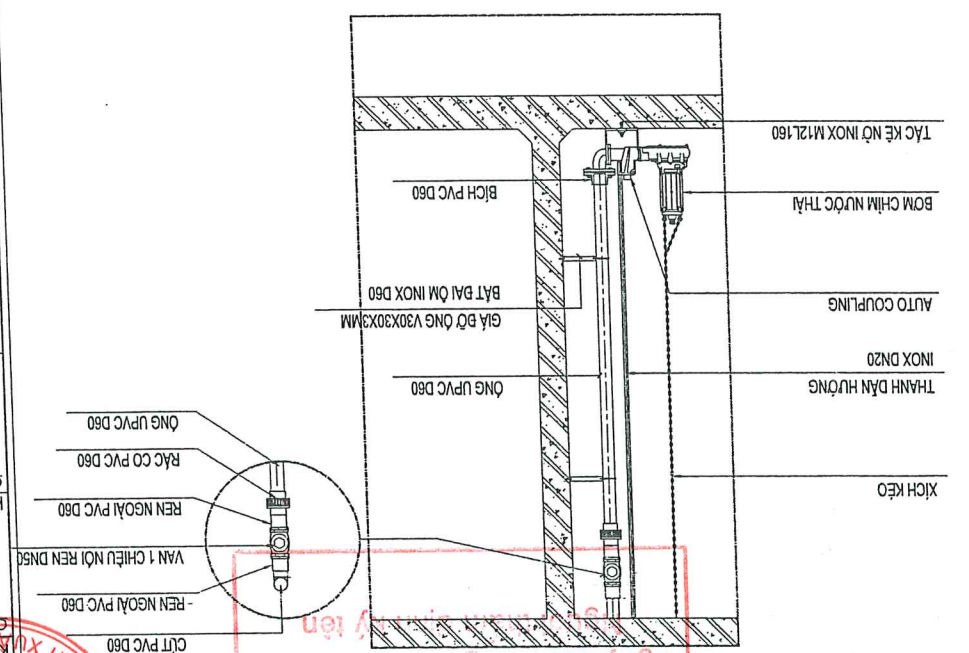
CHI TIẾT LẬP ĐẶT BƠM CHÌM BỂ ĐIỀU HÒA, BỂ HIỆU KHÍ, BỂ LẠNG
