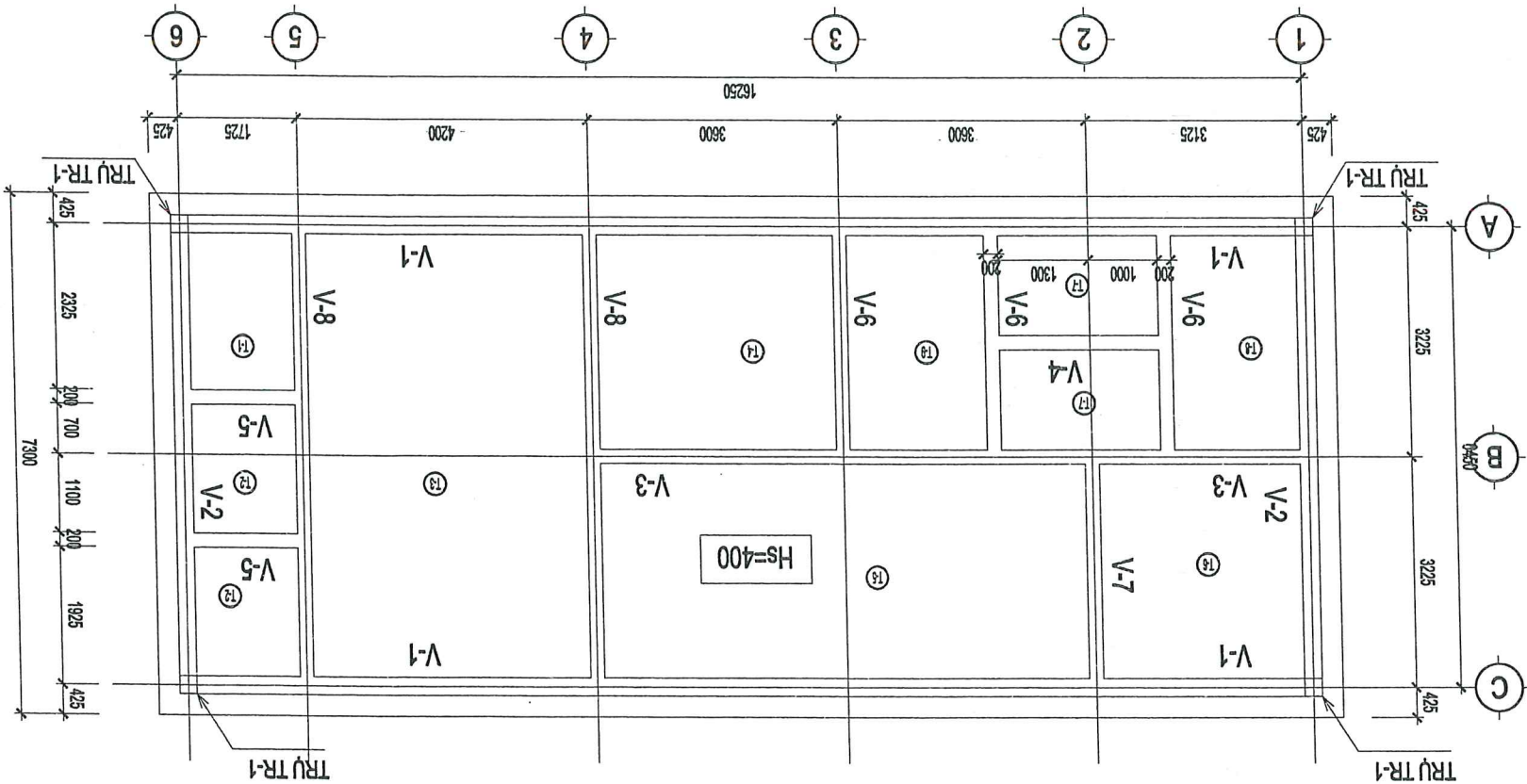
MẶT BẰNG BỐ TRÍ DÂY TRÀM XLNT CAO ĐỘ -3.800
