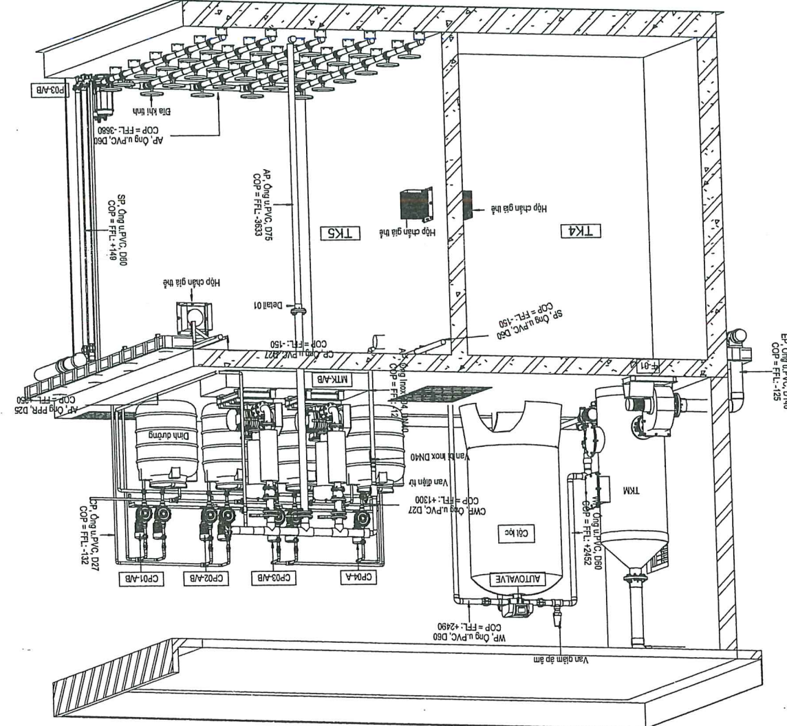
3D VIEW MẶT CẮT 6-6
