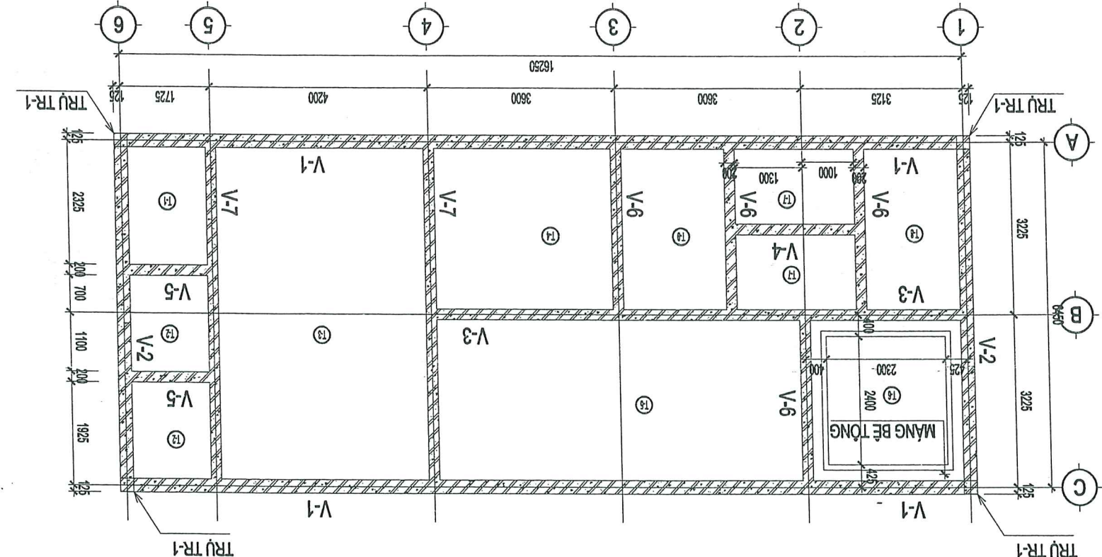
MẶT BẰNG BỐ TRÍ DÂY TRÀM XLNT CAO ĐỘ -0.650
