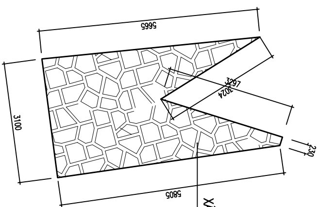
MẶT BẰNG NỀN HỒ LĂNG SỐ 1 VỊ TRÍ SỐ 1 (S= 13.5M 2 )
