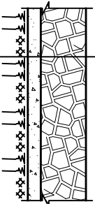
CẦU TẠO NỀN HỒ LĂNG SỐ 1 VỊ TRÍ SỐ 3 (S= 33.5M 2 )
