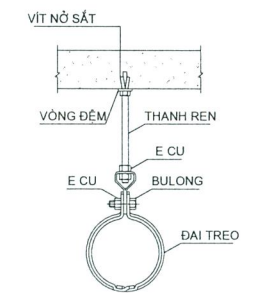
GIÁ TREO ỚNG CHỮA CHÁY CHO ỚNG D25 ~ D50
