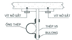
GIÁ TREO ỚNG CHỮA CHÁY CHO ỚNG D50 ~ D80
