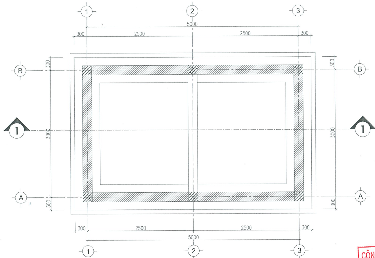
MẶT BẰNG ĐÁY BỂ
