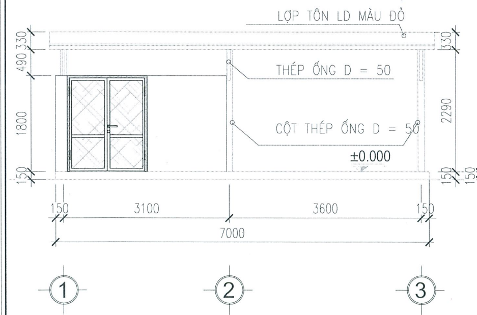
MẶT ĐỨNG MÁI CHE
