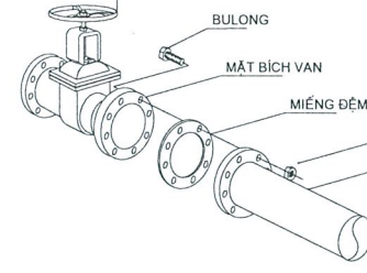
NỐI ỚNG VỚI MẶT BÍCH VAN
