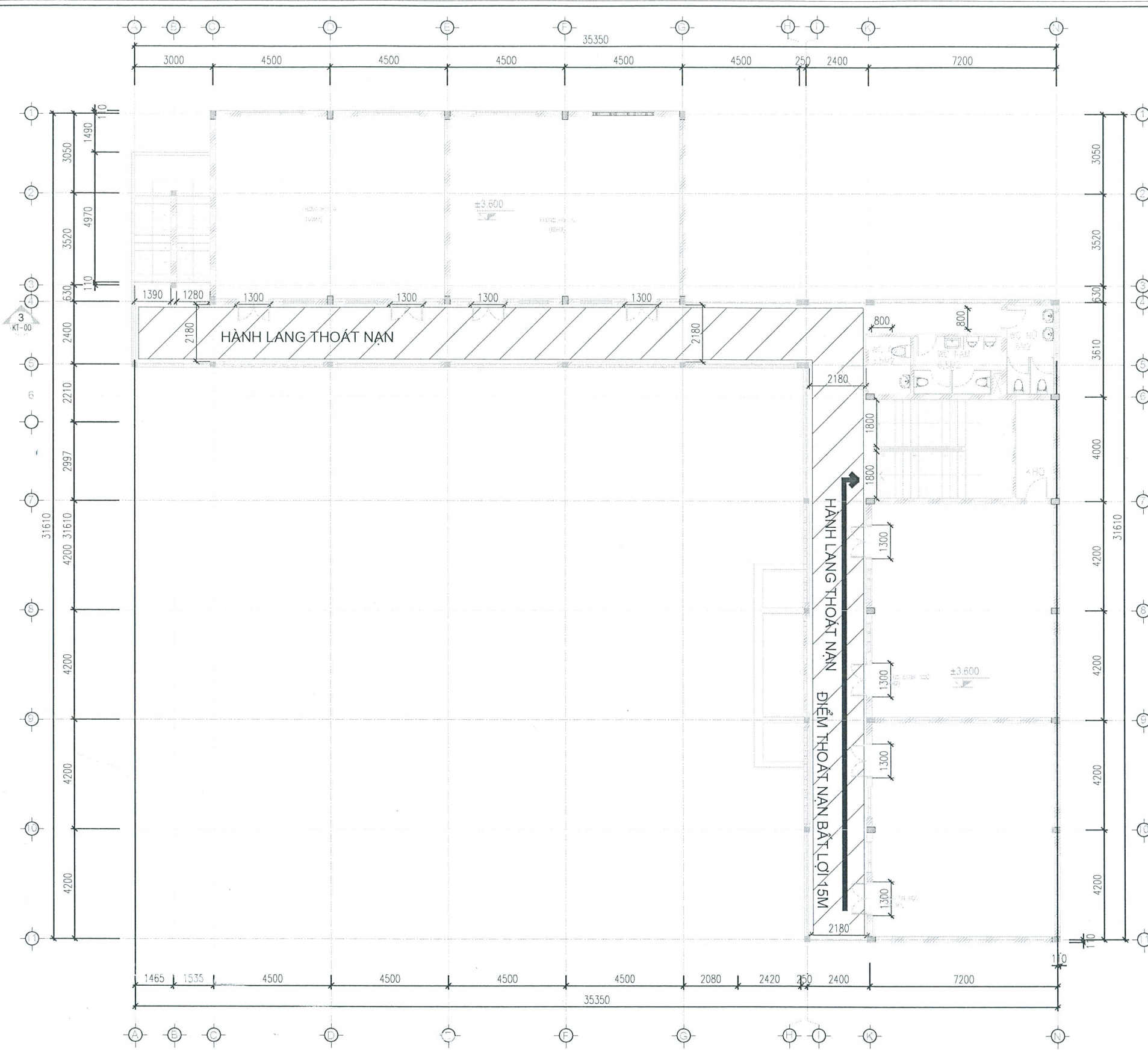
MẶT BẰNG TẦNG 2
