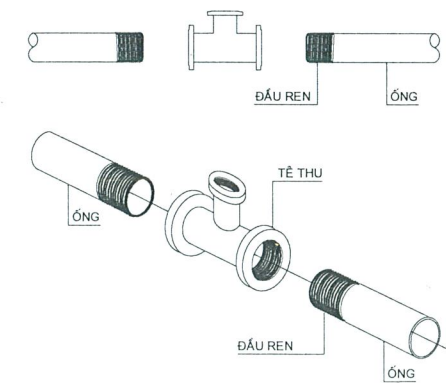
ỚNG NỐI VỚI PHỤ KIỆN BẰNG REN
