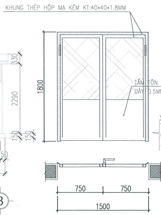
CHI TIẾT CỬA PHÒNG BƠM PCCC
