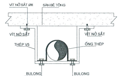
GIÁ TREO ỚNG CHỮA CHÁY CHO ỚNG D80 ~ D125
