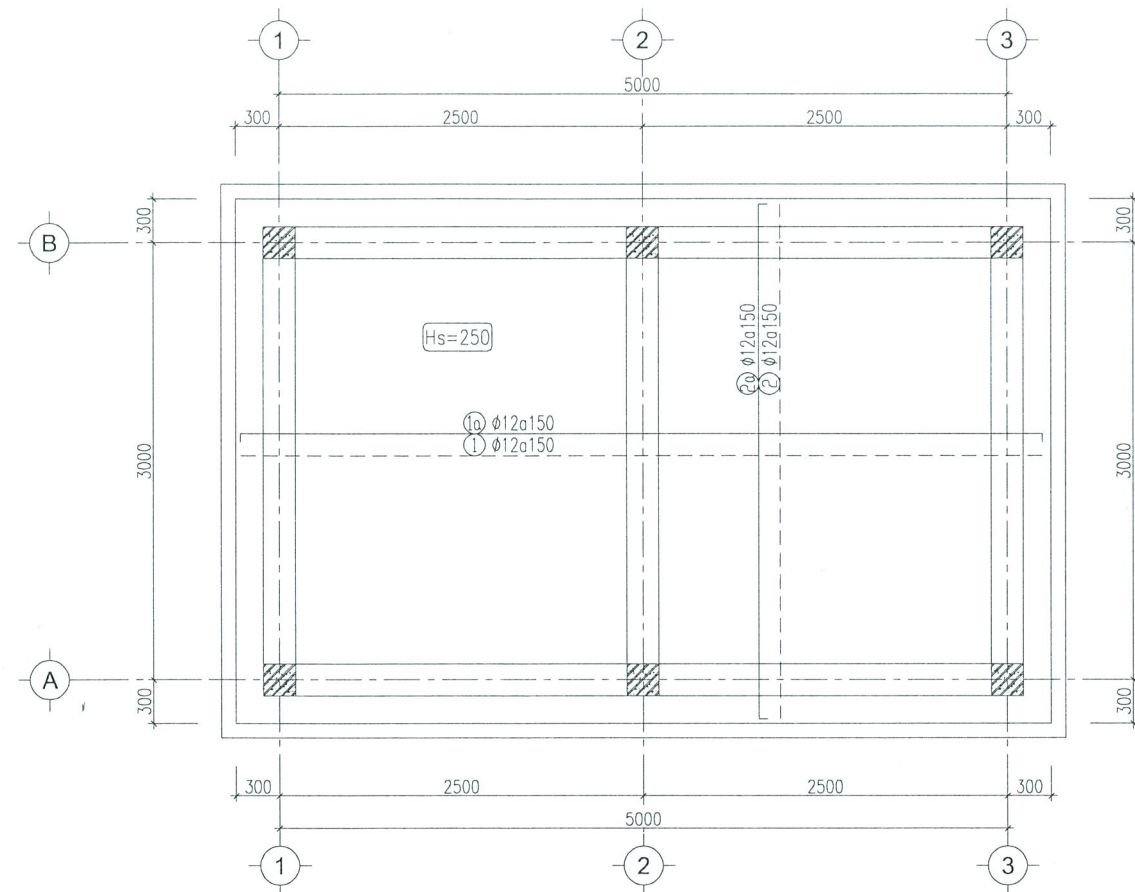
MẶT BẰNG THÉP ĐÁY BÊ
