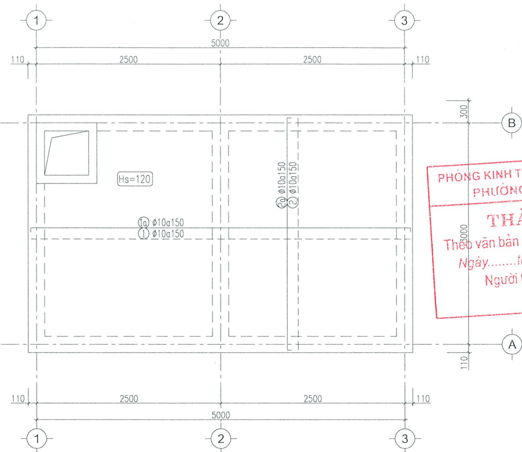
MẶT BẰNG THÉP NẮP BÊ
