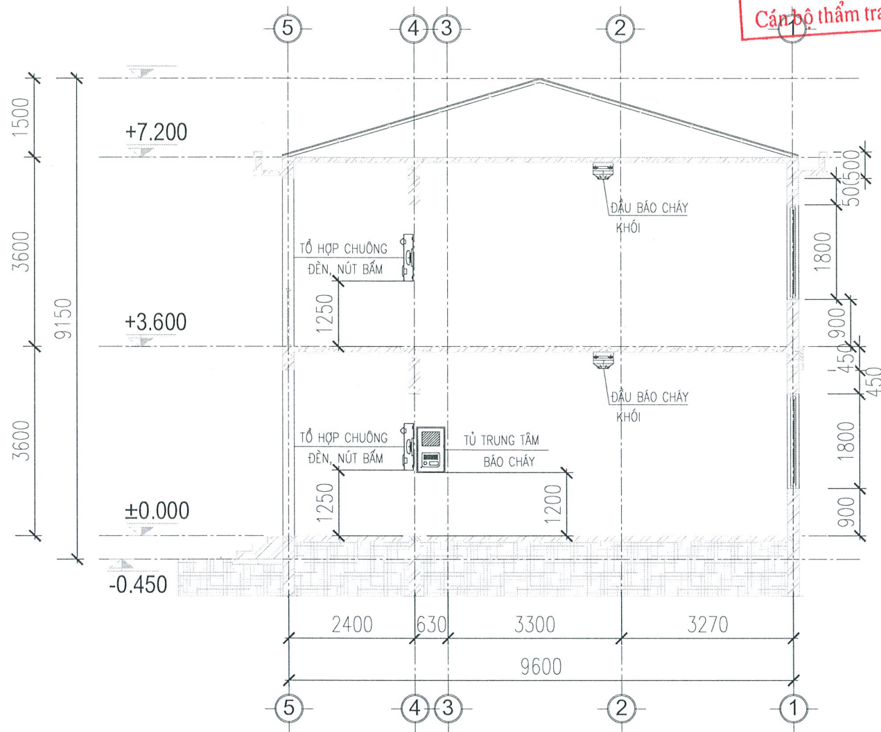
MẶT CẮT 3-3
