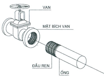
ỐNG NỐI VỚI VAN BẰNG REN
