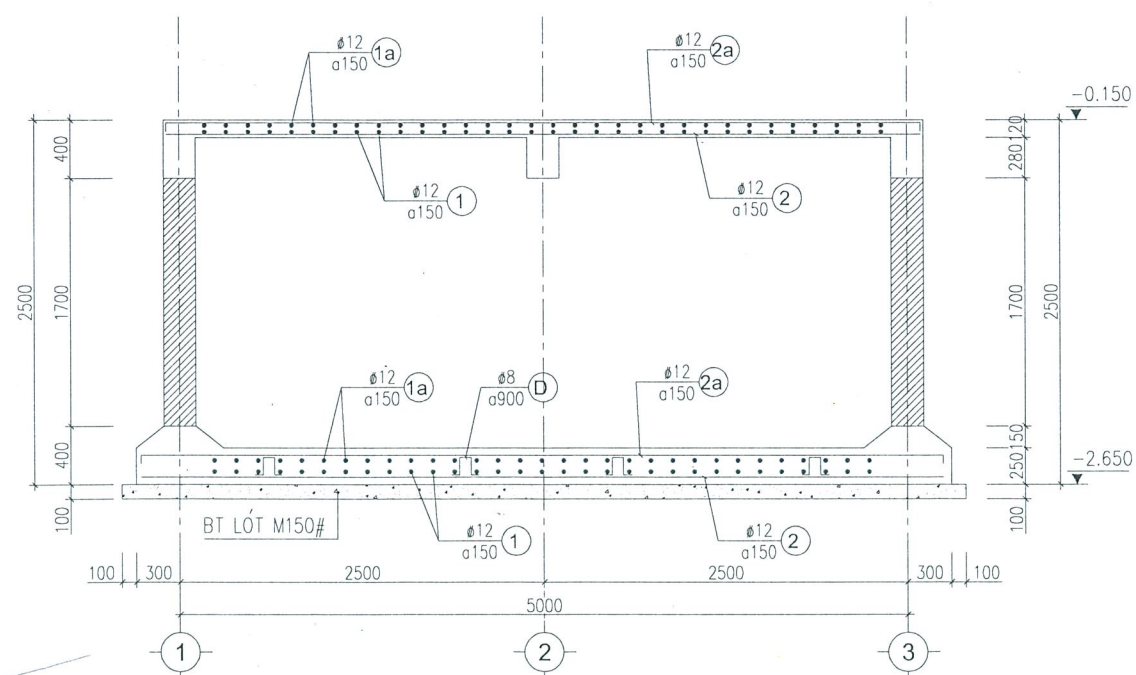
MẶT CẮT 1-1
