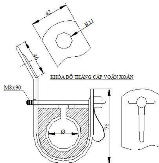
Hình ảnh minh họa khóa đờ
