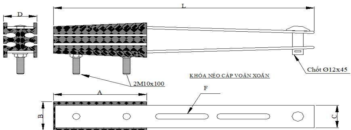
Hình 31 Hình ảnh minh họa khóa néo
