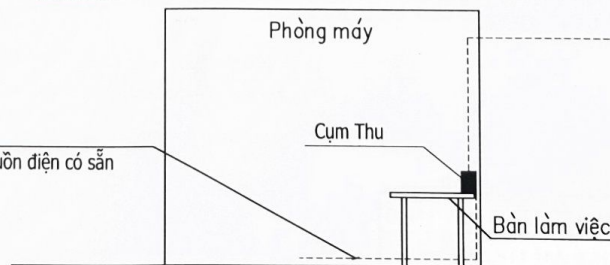
MẶT ĐÚNG BỐ TRÍ LOA TRÊN CỘT BTS
