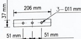
Sơ đồ kích thước chung
