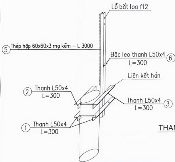
THANH SỐ 1: L50X4 300 (2CK)
