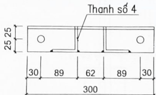
THANH SỐ 3 L50X4 300 (1CK)
