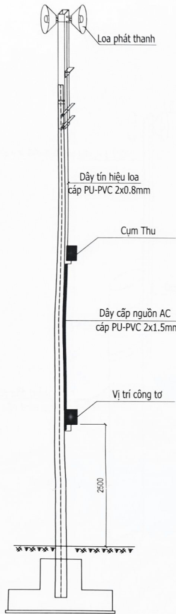
MẶT ĐÚNG BỐ TRÍ LOA TRÊN CỘT ĐIỆN
