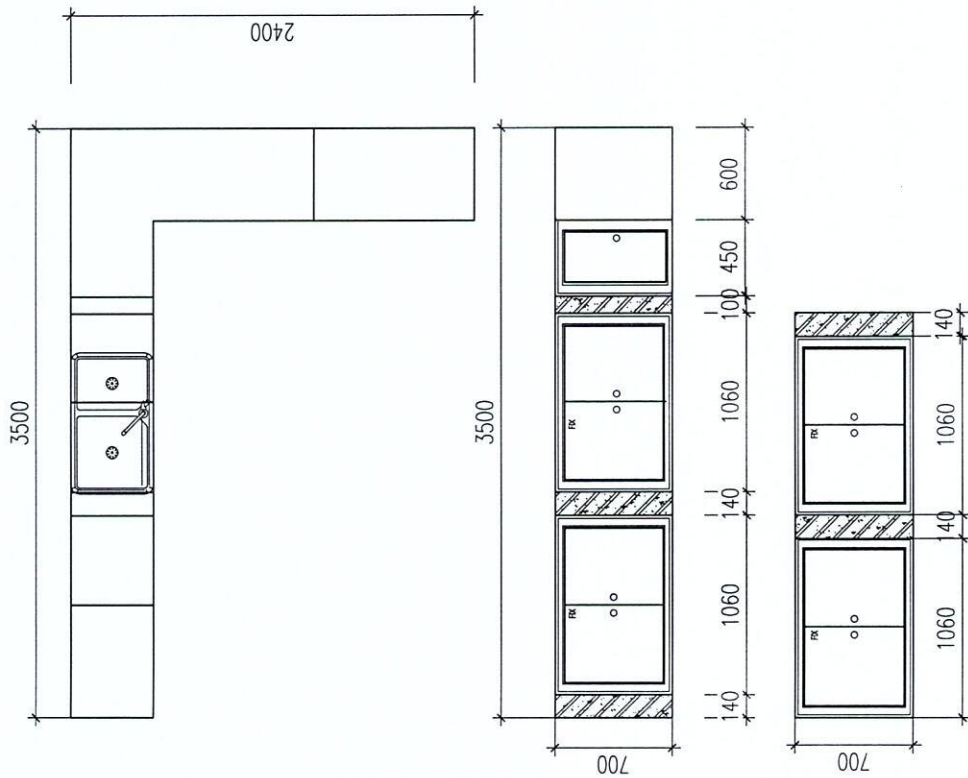
TỦ CHẠM BẾP DƯỚI
