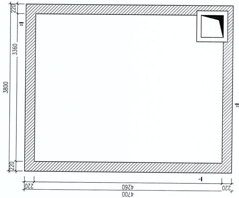
MẶT BẰNG BỂ NƯỚC
