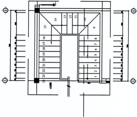
MẶT BẰNG THANG TẦNG 1 LÊN TẦNG 2
