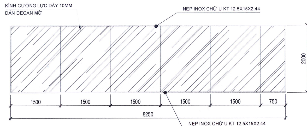
CHI TIẾT VÁCH KÍNH VK1 KT 8250X2000 TL:1/50
