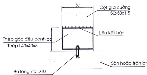
MẶT CẮT 2-2
