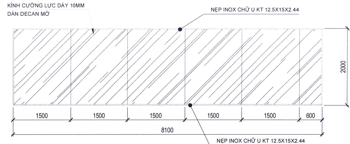
CHI TIẾT VÁCH KÍNH VK2 KT 8100X2000 TL:1/50
