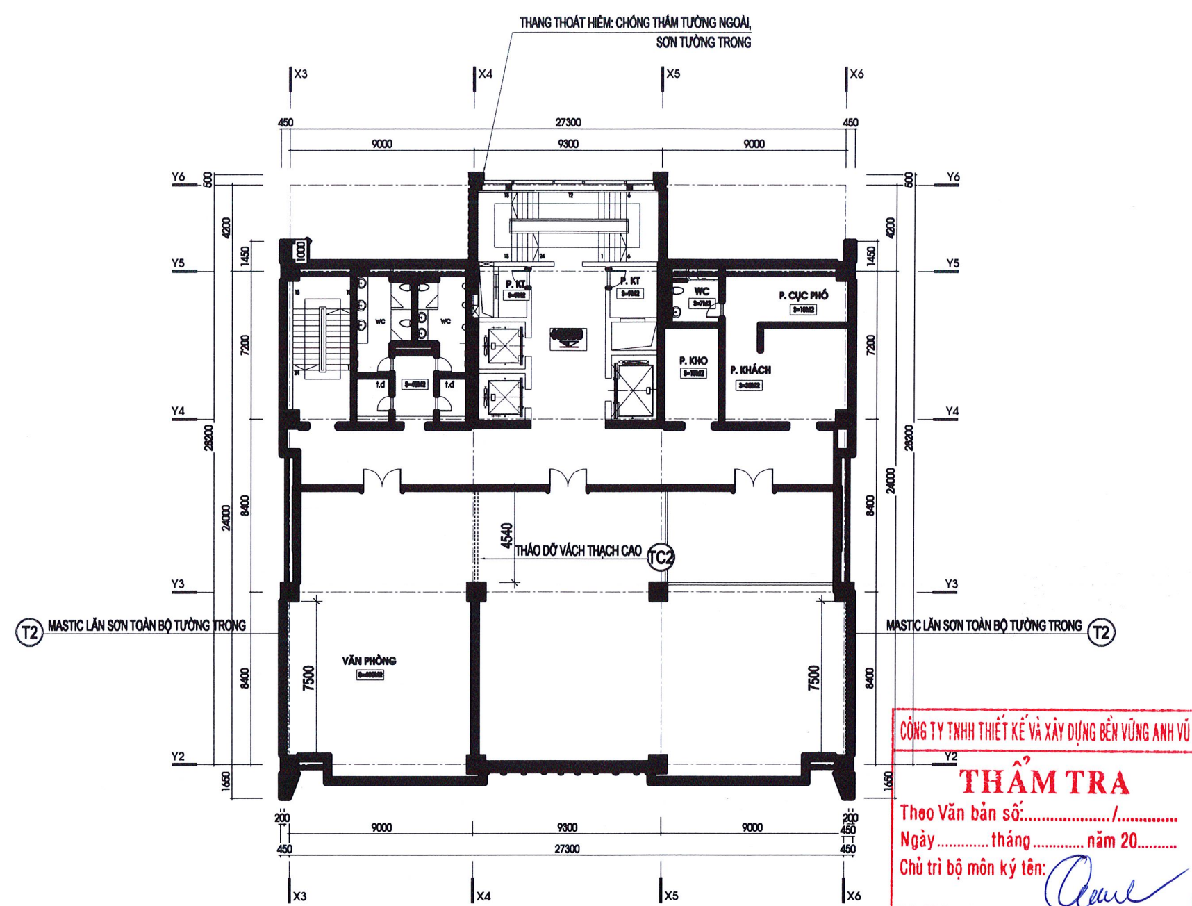
MẶT BẰNG TẦNG 8 - CẢI TẠO TL:1/100
