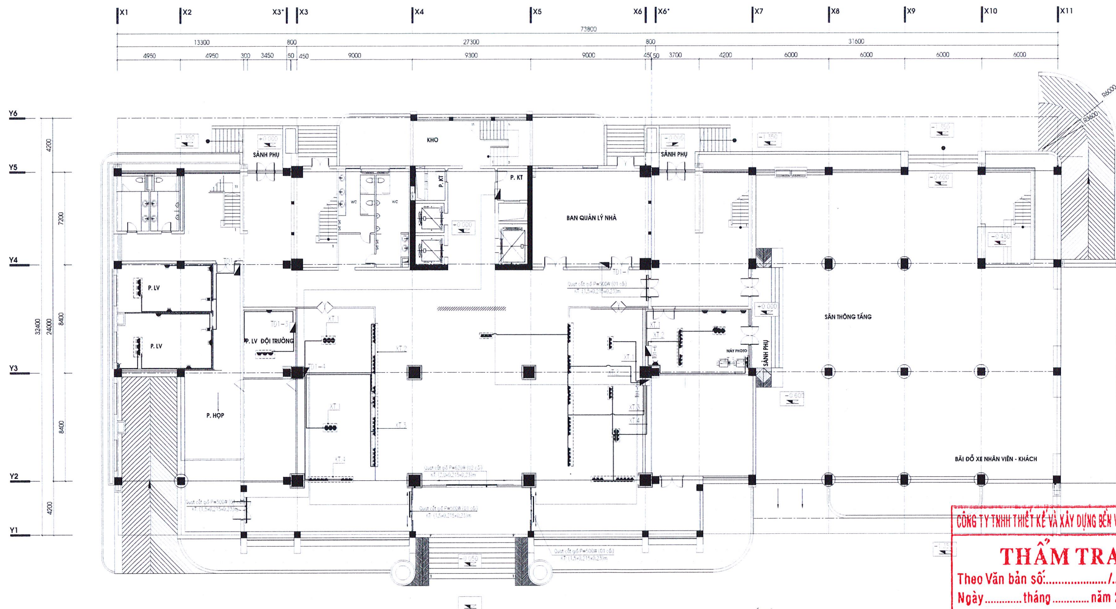
MẶT BẰNG BỐ TRÍ Ồ CẨM TẦNG 1 - CẢI TẠO
