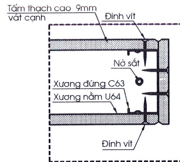
CHI TIẾT ĐẦU VÁCH
