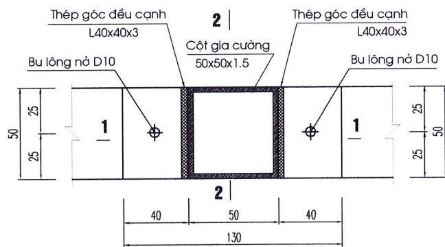
CHI TIẾT LIÊN KẾT THÉP GIA CƯỜNG VỚI NỀN VÀ TRẦN BT
