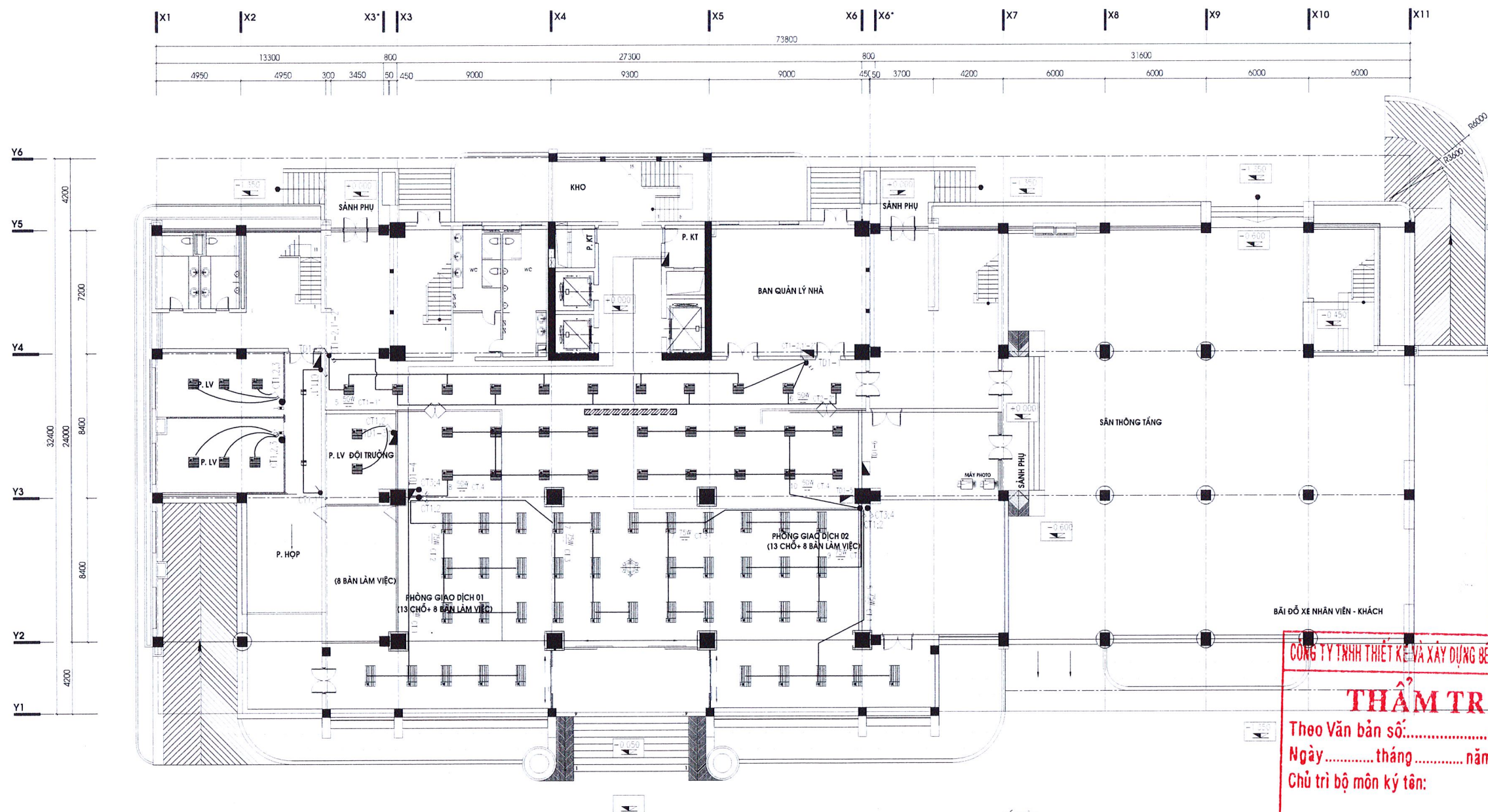
MẶT BẰNG BỐ TRÍ CHIẾU SÁNG TẦNG 1 - CẢI TẠO
