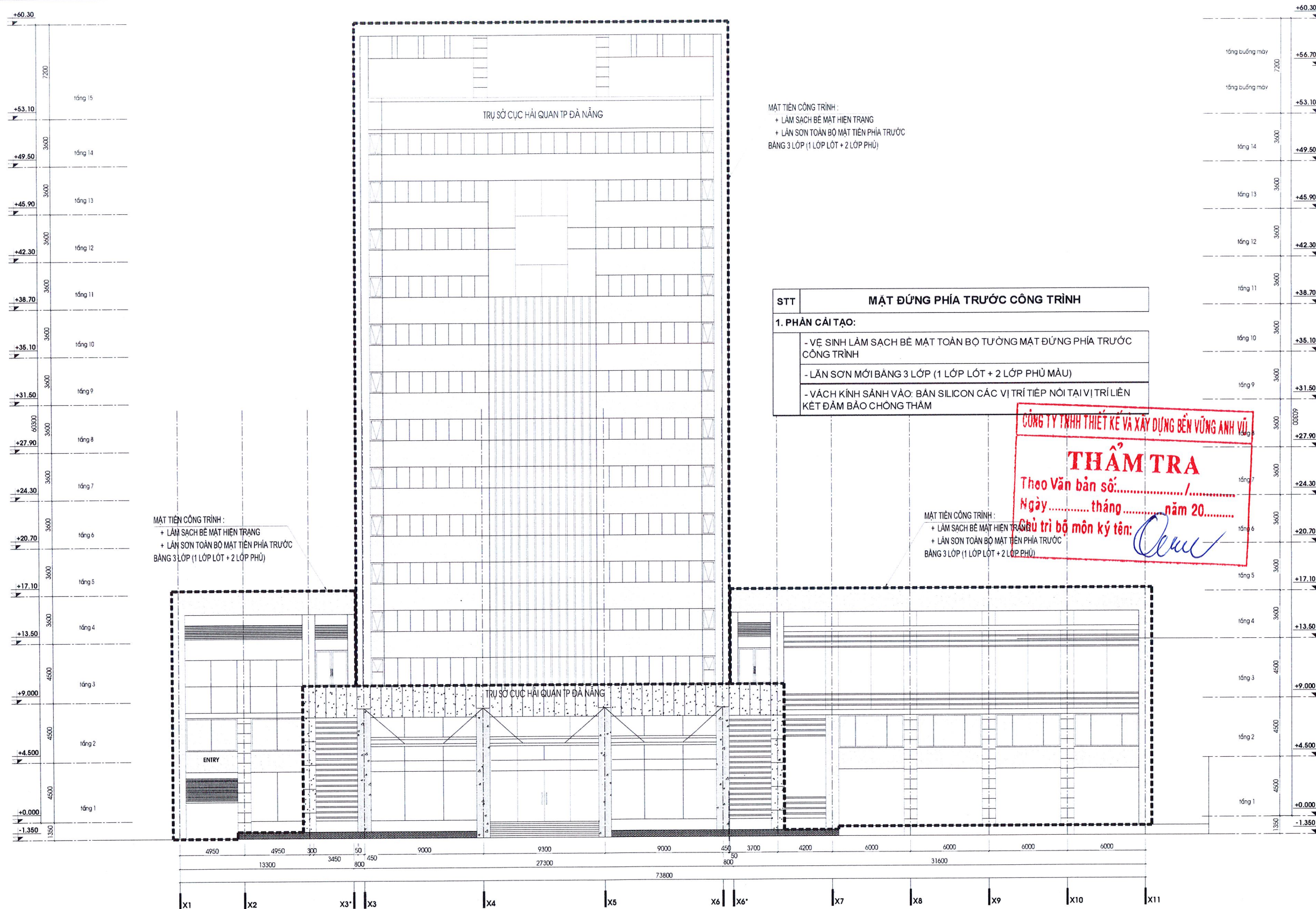
MẶT ĐỪNG TRỤC X1-X11 - CẢI TẠO TL:1/100
