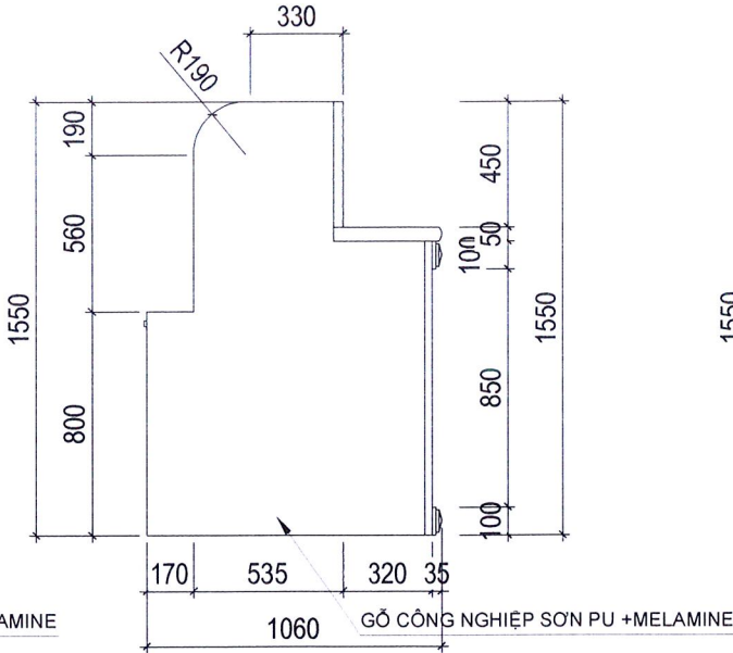
MẶT BÊN
