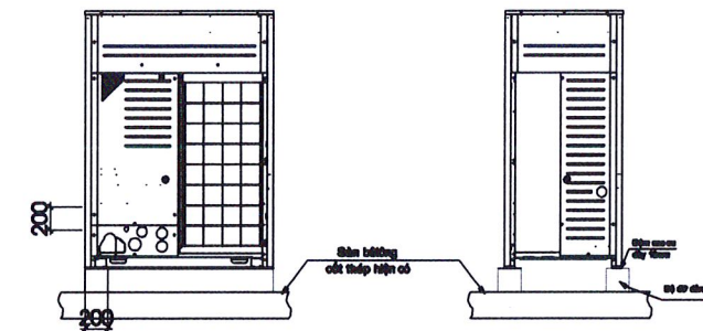
CHI TIẾT LẮP ĐẶT DÀN NÓNG VRF
