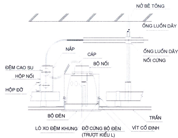
CHI TIẾT LẮP ĐÈN DOWNLIGHT ÂM TRẦN
