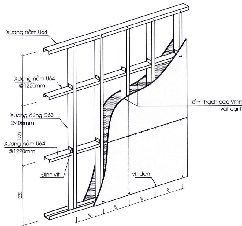
HỆ KHUNG THẠCH CAO ĐIỂN HÌNH
