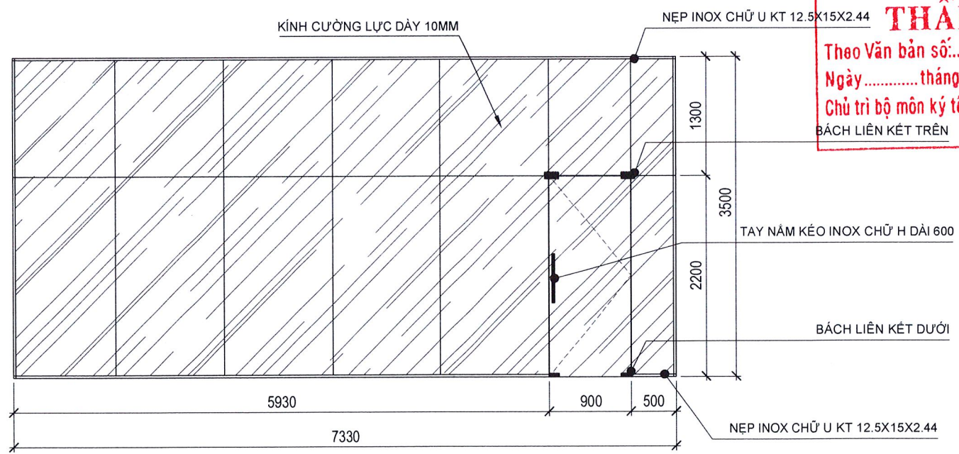
CỬA ĐI D1 900X2200 TL:1/50
