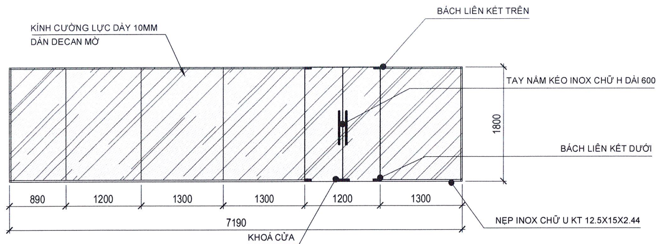
CHI TIẾT VÁCH KÍNH V5 KT 7190X1800 TL:1/50
