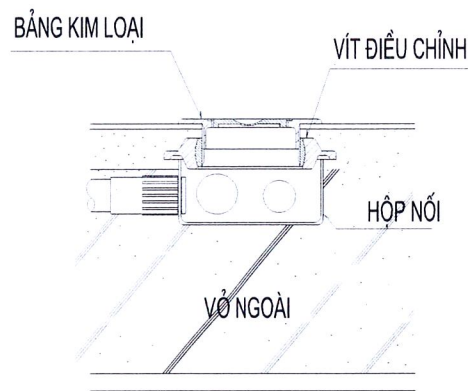
CHI TIẾT LẮP HỘP ĐẦU DÂY ÂM TRẦN
