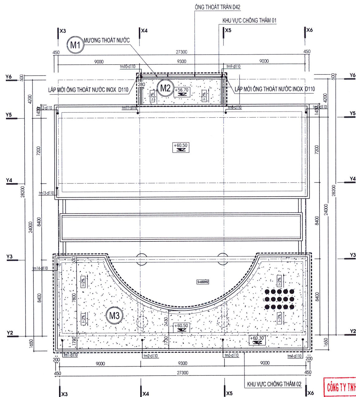
MẶT BẰNG TẦNG 15 - CẢI TẠO
