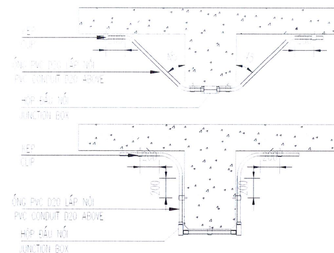
CHI TIẾT LẮP ĐẶT ỨNG PVC VƯỢT DẦM INSTALLATION DETAIL OF PVC CONDUIT
