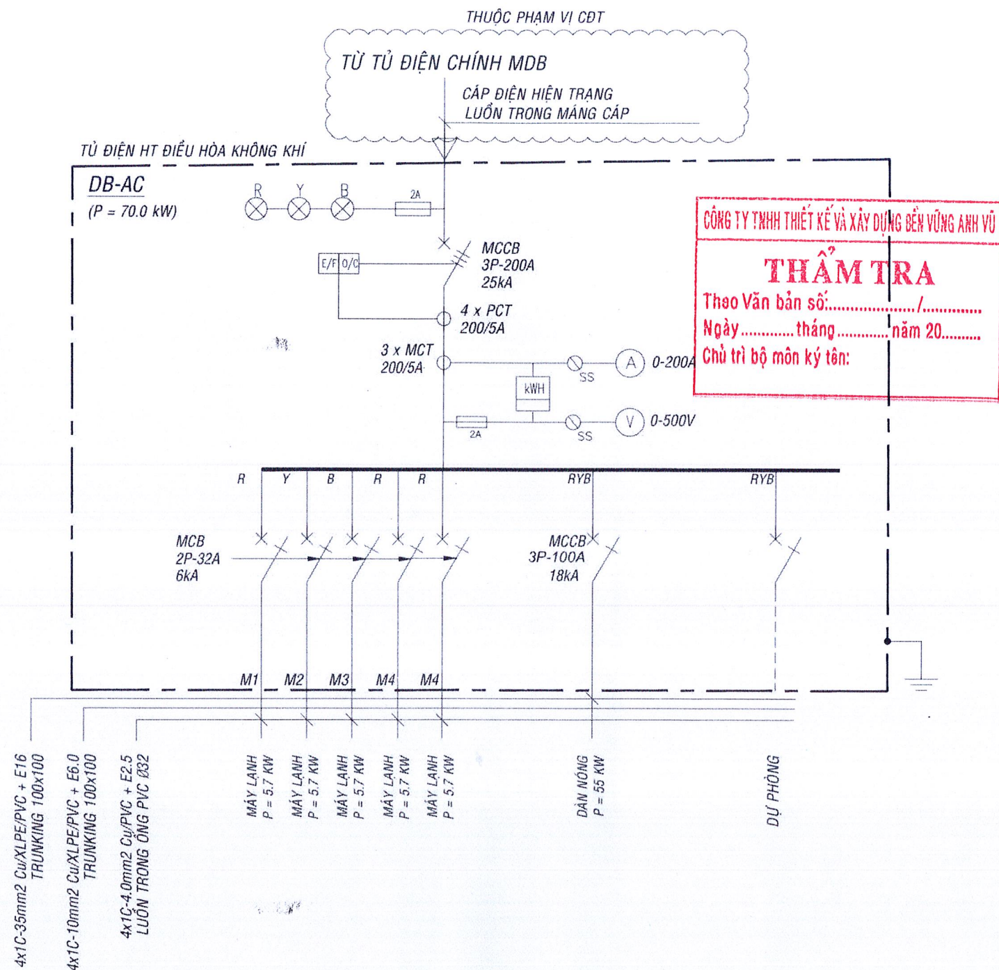
SƠ ĐỒ NGUYÊN LÝ TỦ ĐIỆN DB-AC
