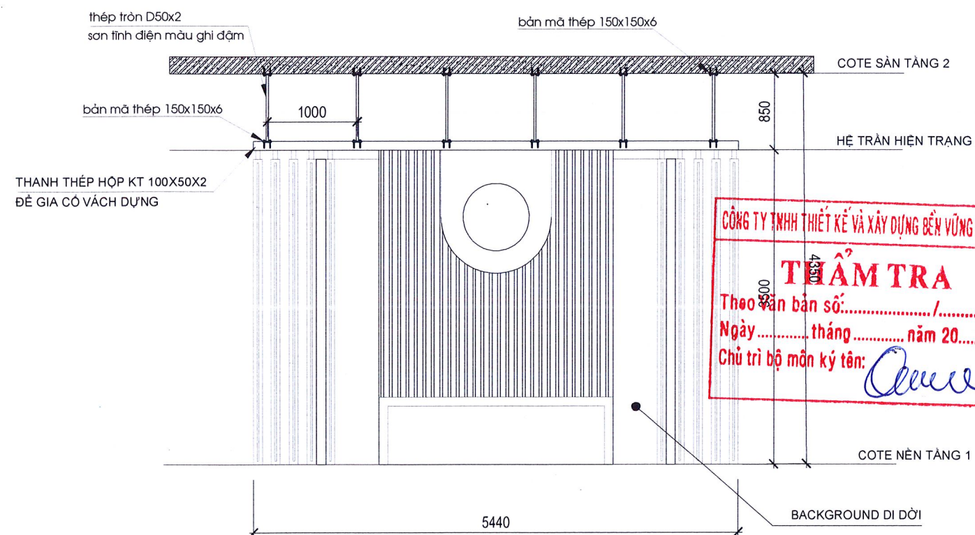
CHI TIẾT VÁCH BACKGROUND DI DỜI TL:1/50
