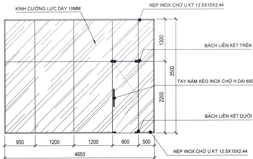
CHI TIẾT VÁCH KÍNH V4 KT 4650X3500 TL:1/50
