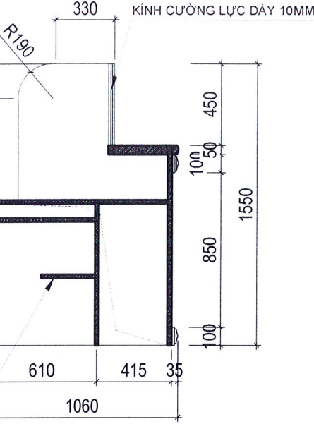
MẶT CẮT
