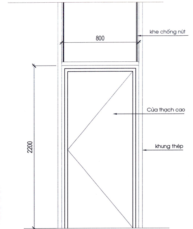
CHI TIẾT LẮP ĐẶT VỊ TRÍ CỬA THẠCH CAO
