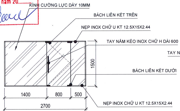
CHI TIẾT VÁCH KÍNH V7 KT 2700X1500 TL:1/50
