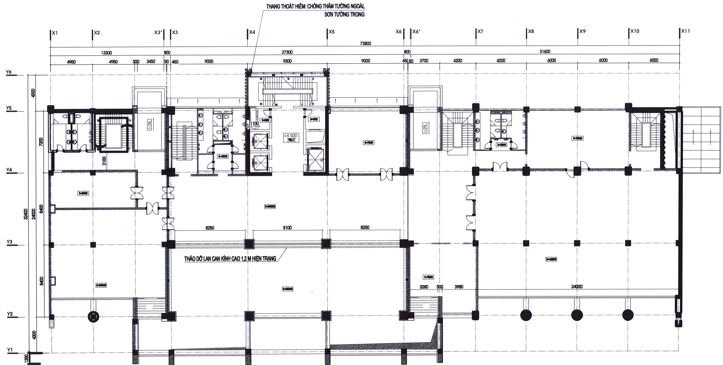
MẶT BẰNG TẦNG 2 HIỆN TRẠNG - THẢO DỖ
