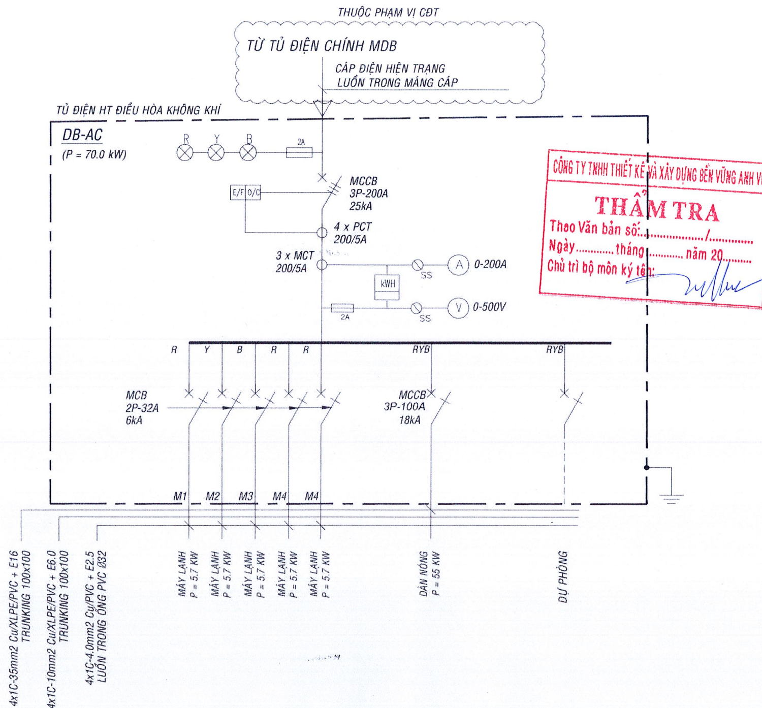
SƠ ĐỒ NGUYÊN LÝ TỦ ĐIỆN DB-AC
