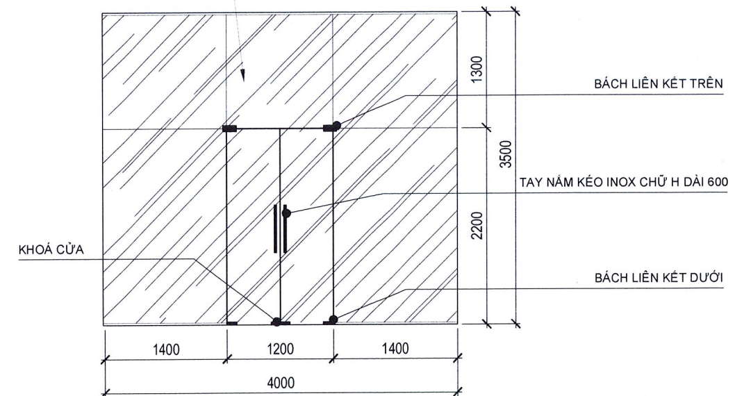
CHI TIẾT VÁCH KÍNH ĐIỂN HÌNH TL:1/50
