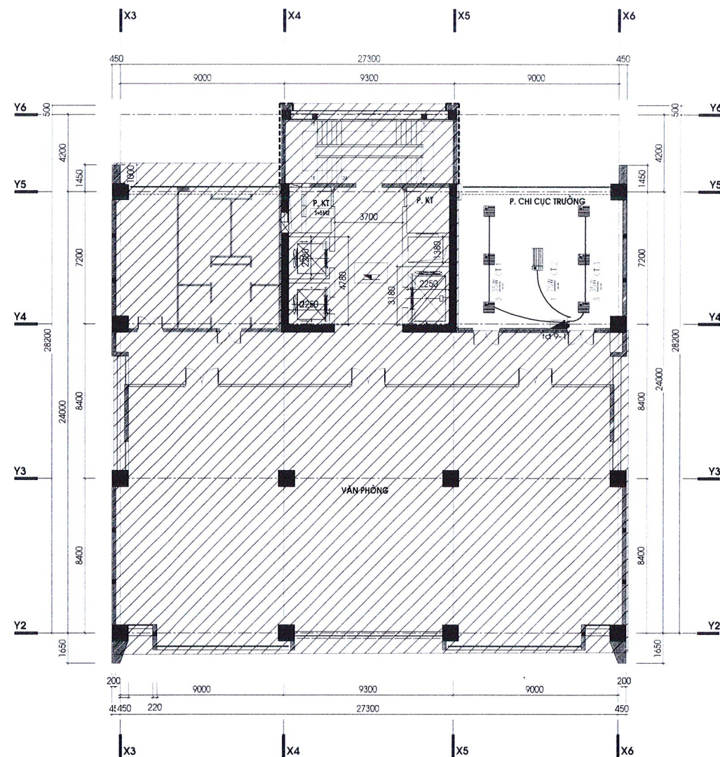
MẶT BẰNG BỐ TRÍ CHIẾU SÁNG TẦNG 9 - CẢI TẠO
