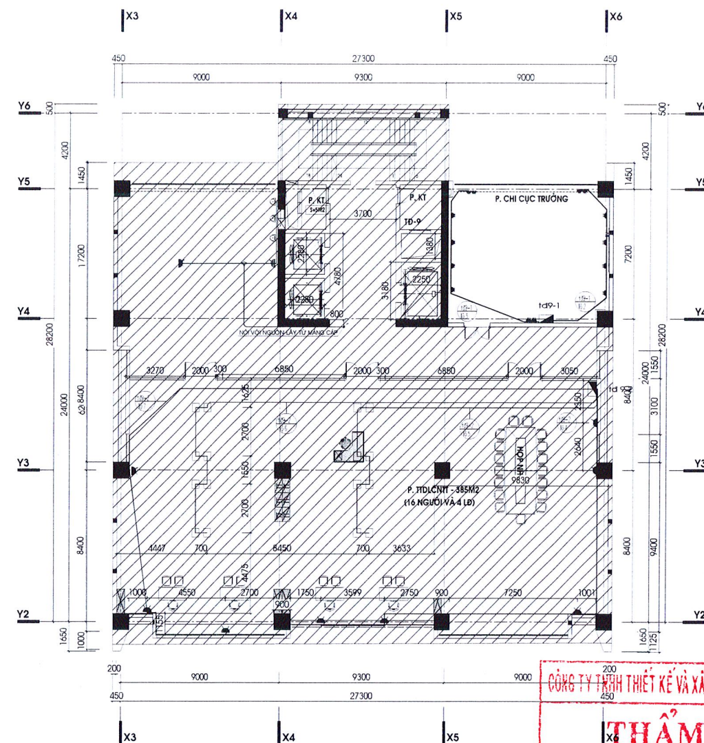
MẶT BẰNG BỐ TRÍ Ồ CẨM TẦNG 9 - CẢI TẠO
