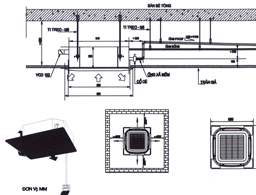
CHI TIẾT LẮP ĐẶT MÁY CASSETTE
