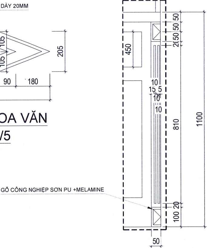
CHI TIẾT CHÂN TỦ
