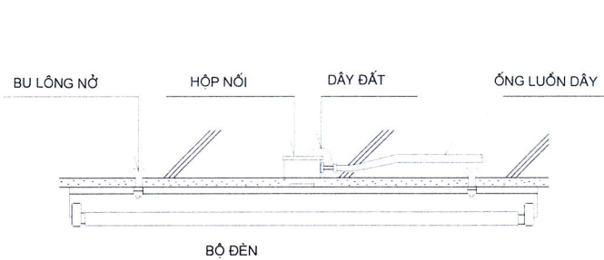
CHI TIẾT LẮP BỘ ĐÈN GẮN TRẦN
