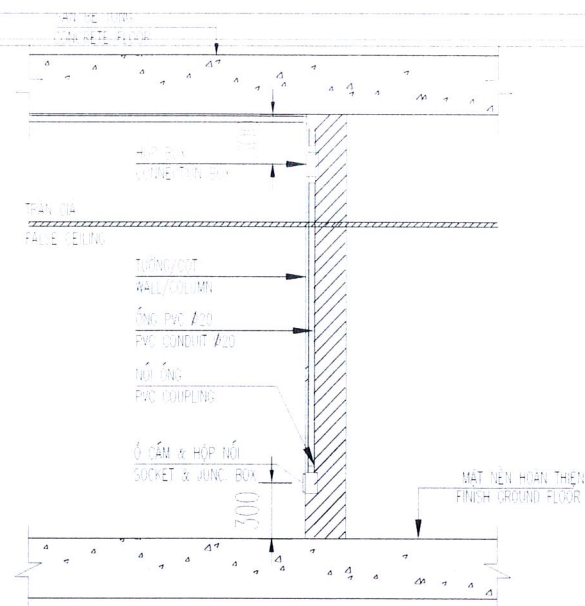
CHI TIẾT LẮP ĐẶT Ổ CẮM ĐIỆN ẨM TƯỜNG INSTALLATION DETAIL OF SOCKET
