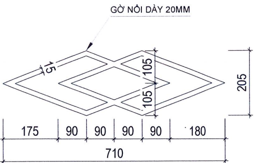
CHI TIẾT HOA VĂN TL:1/5
