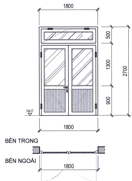
CHI TIẾT CỬA D2 (SL:02) TL:1/25
