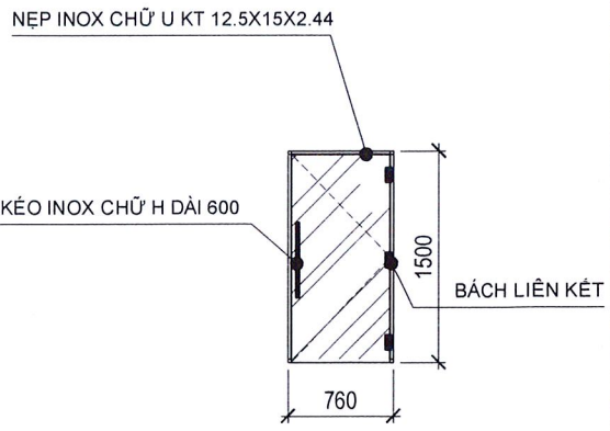
CHI TIẾT CỬA ĐI D4 KT 780X1500 TL:1/50
