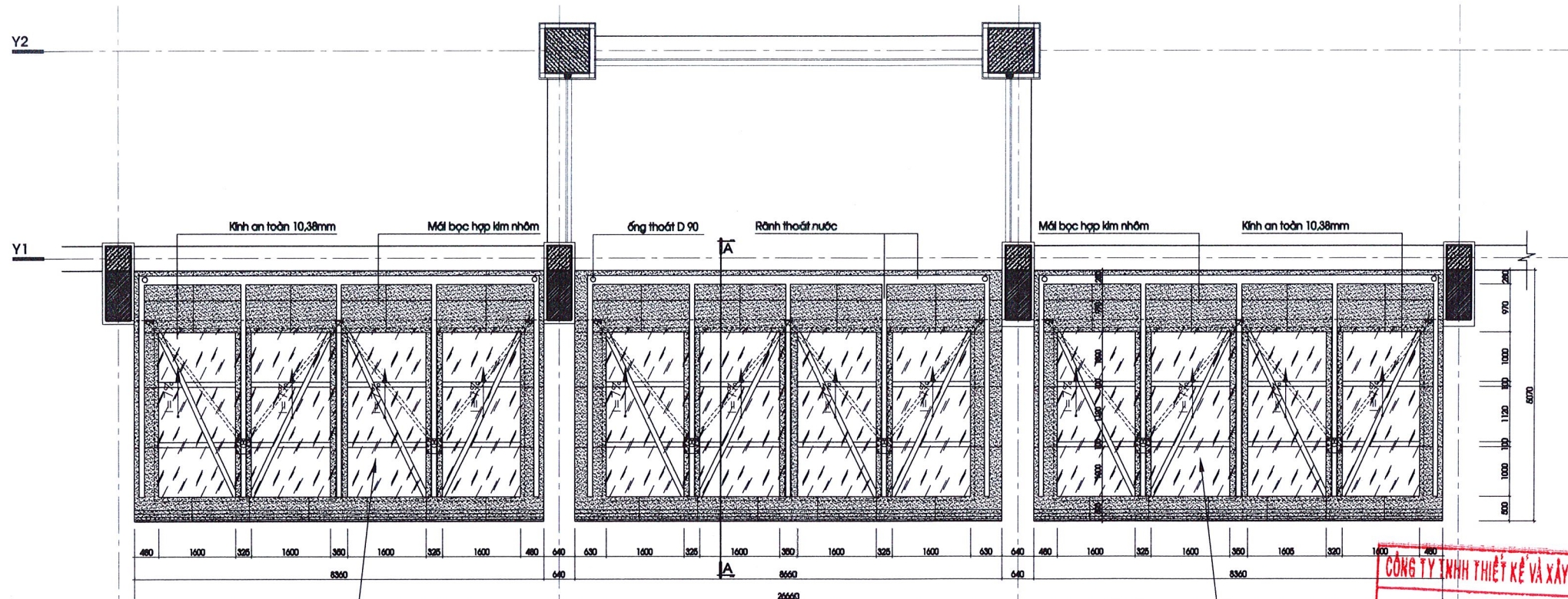
MẶT BẰNG MÁI SẴNH TRỤC X3-X6 TL:1/50
