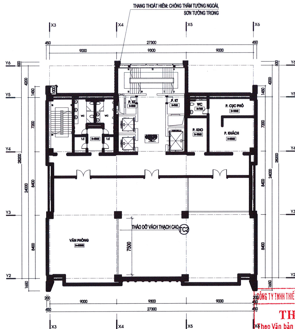
MẶT BẰNG TẦNG 6 - CẢI TẠO TL:1/100
