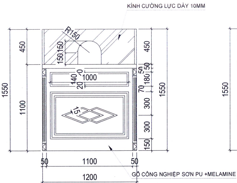
MẶT ĐỨNG TRƯỚC TL:1/10
