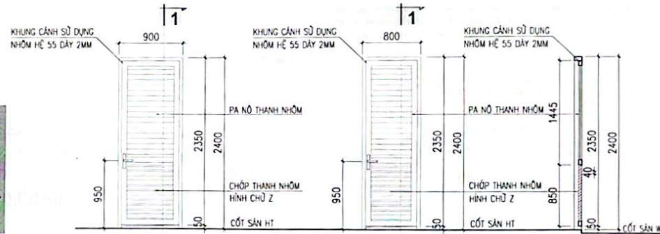
CỬA WC D4A2 (THAY MỚI)
