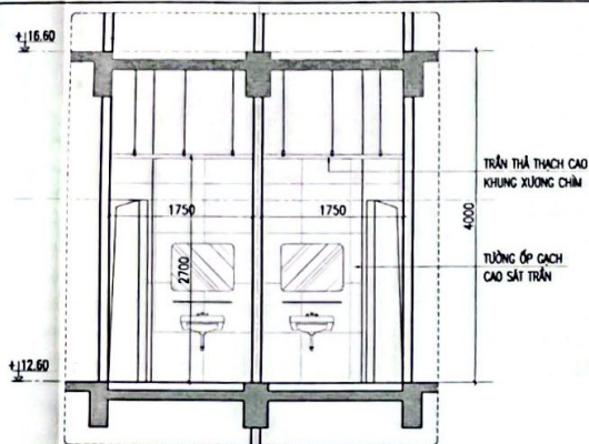
X12 CẮT 1-1
