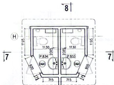
M.BẰNG WC P.833 & P.834
