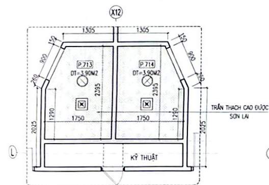
M.BẦNG TRẦN WC P.713 & P.714
