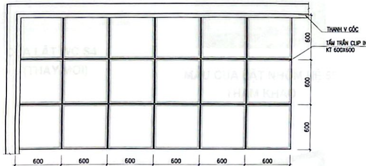
CHI TIẾT MẶT BẰNG
