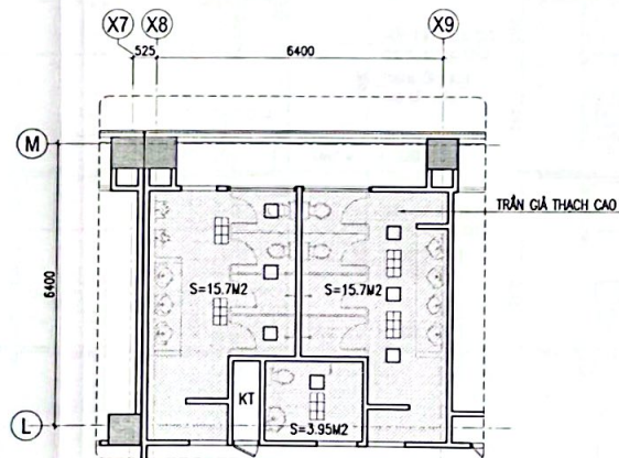
MẶT BẰNG KHU VỆ SINH WC - 01 TẦNG 3 - HIỆN TRẠNG
