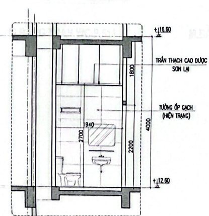
K CẮT 6-6
