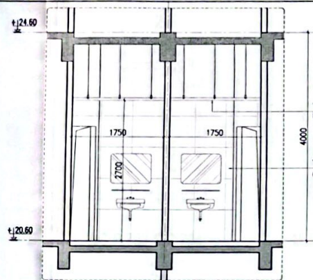
X12 CẮT 1-1
