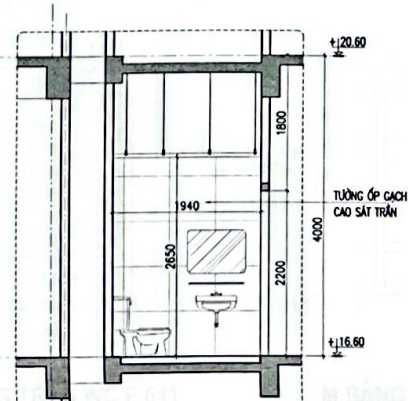
CẮT 6-6
