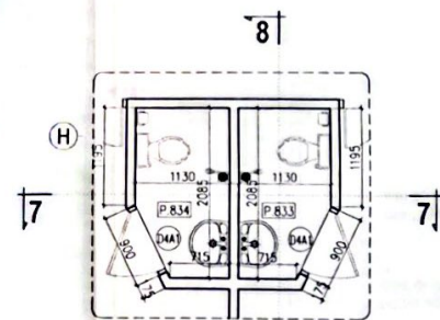
M.BẰNG WC P.833 & P.834
