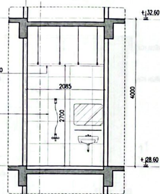
CẮT 8-8
