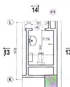
M.BẦNG WC P.716
