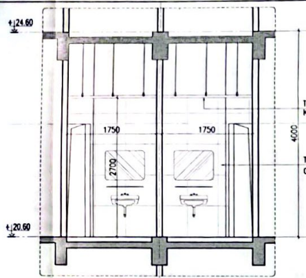
CẮT 1-1
