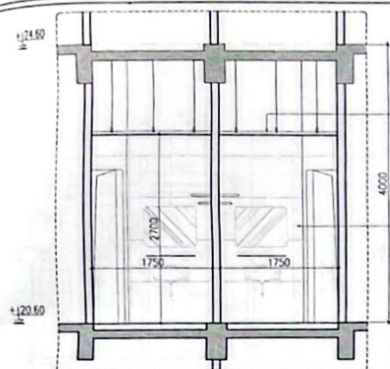
X12 CẮT 1-1
