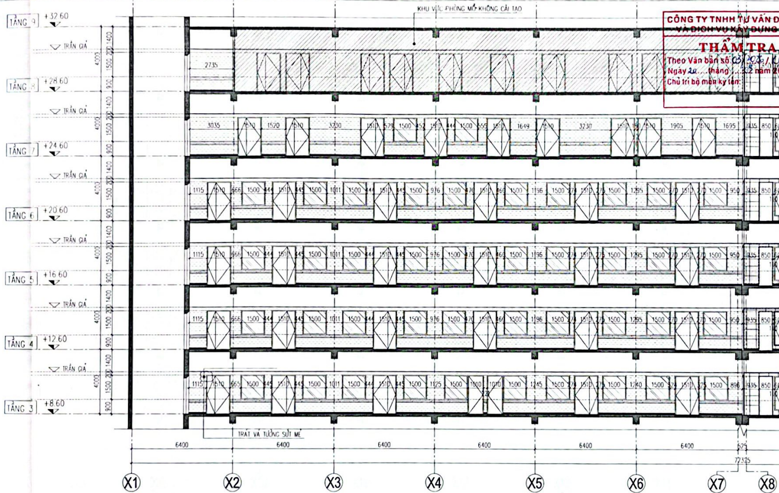
MẶT CẮT CẢI TẠO B-B (P1)
