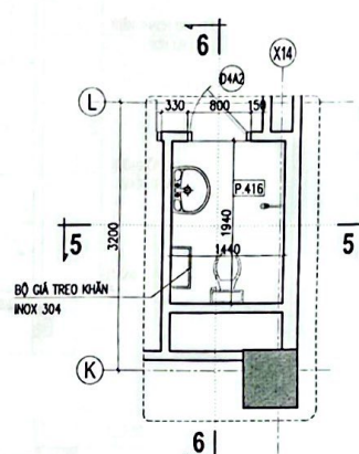
M.BẢNG WC P.416
