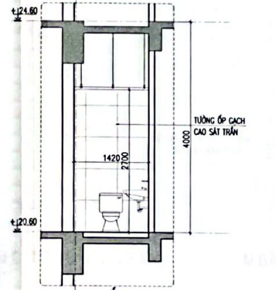
CẮT 5-5
