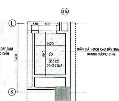
M.BẰNG TRẦN WC P.512
