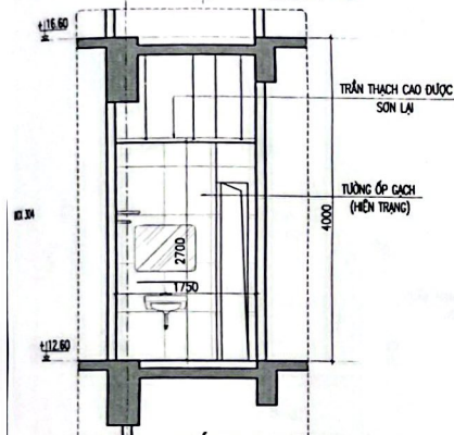
X13 CẮT 3-3
