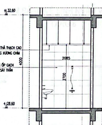
CẮT 12-12
