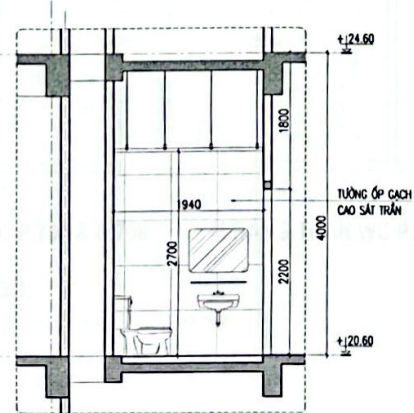
K CẮT 6-6
