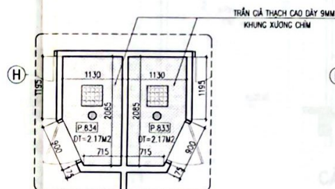
M.BẰNG TRẦN WC P.833 & P.834
