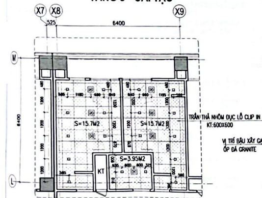
MẶT BẰNG TRẦN KHU VỆ SINH WC - 01 CẢI TẠO
