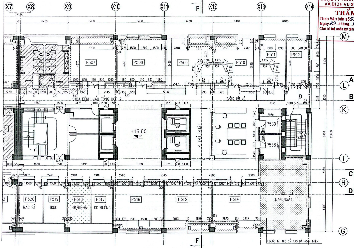
MẶT BẰNG HIỆN TRẠNG TƯỜNG & TRẦN TẦNG 5 (P2)
