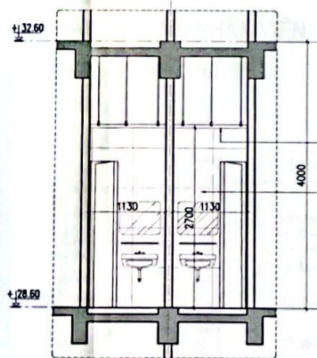
CẮT 11-11
