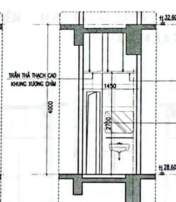
CẮT 13-13
