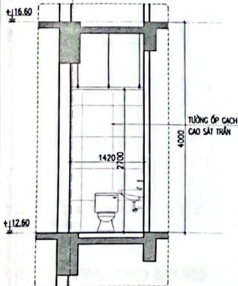
X14 CẮT 5-5
