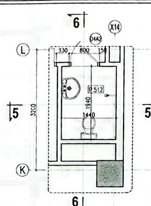
M.BẰNG WC P.512
