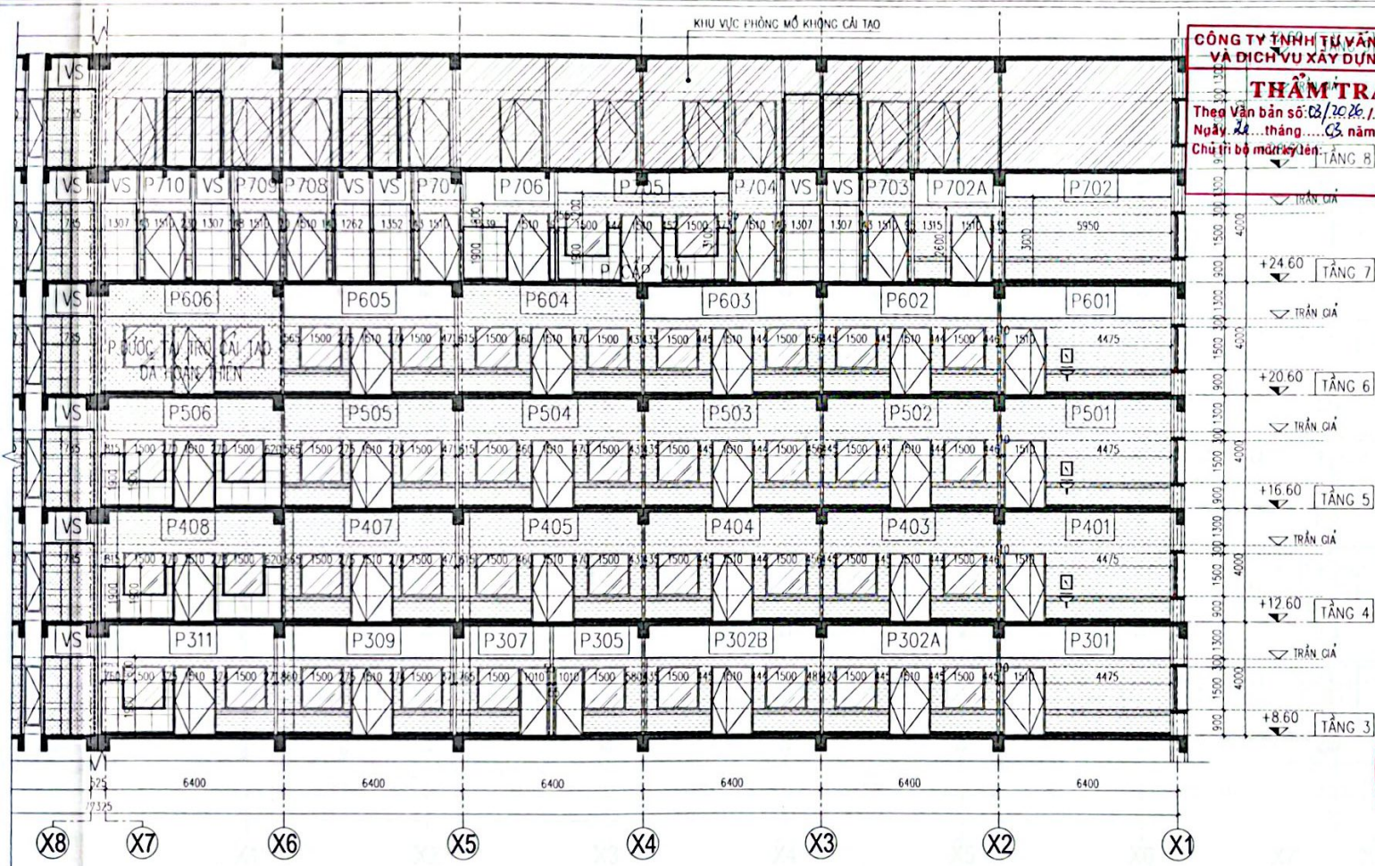
MẶT CẮT CẢI TẠO A-A (P2)
