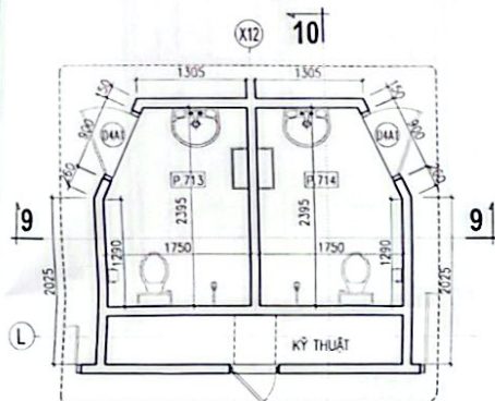
M.BẦNG WC P.713 & P.714
