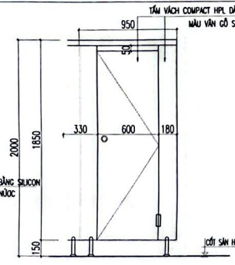
VÁCH NGĂN VN - 1 (KHOANG XÍ)
