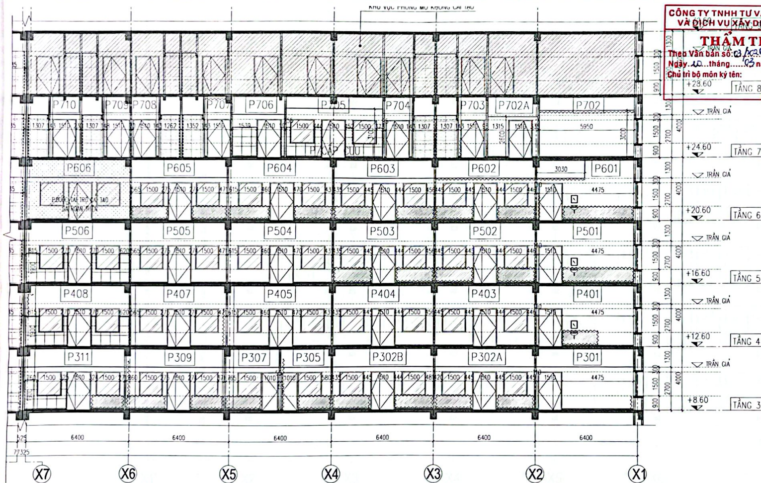
MẶT CẮT HIỆN TRẠNG A-A (P2)
