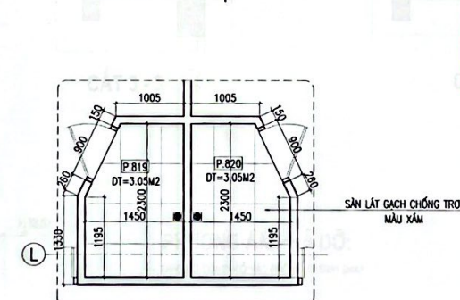
M.BẰNG LÁT SÀN WC P.819 & P.820
