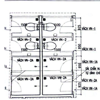
MẶT BẰNG ĐỊNH VỊ VÁCH NGĂN VỆ SINH WC - 01 (TẦNG 3)
