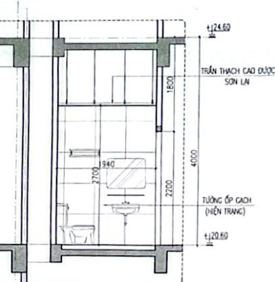
K CẮT 14-14
