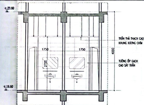
CẮT 1-1
