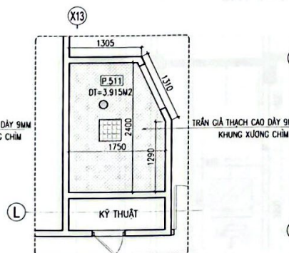
M.BẰNG TRẦN WC P.511
