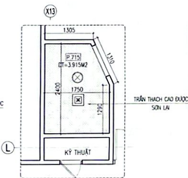
M.BẦNG TRẦN WC P.715
