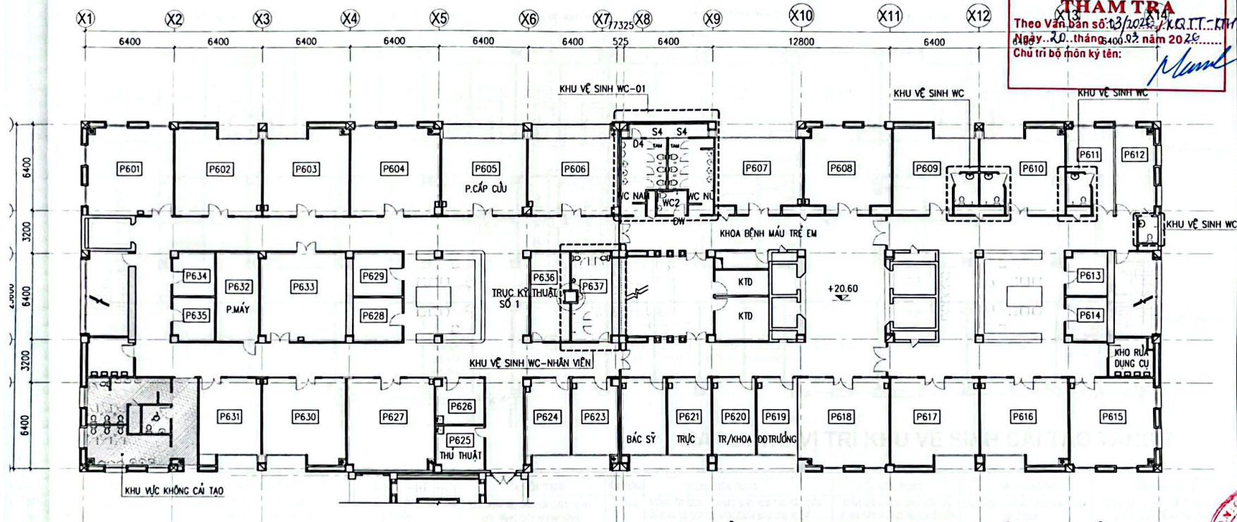
MẶT BẰNG VỊ TRÍ KHU VỆ SINH CẢI TẠO TẦNG 6
