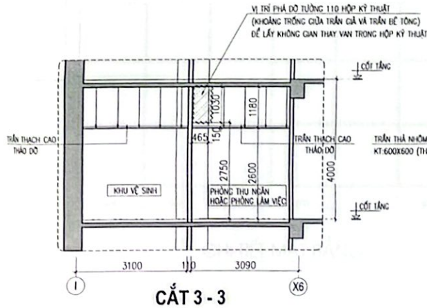
VỊ TRÍ TƯỜNG PHÁ DỠ TRỤC KỸ THUẬT TẦNG 4,5,6,7,8
