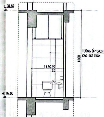
CẮT 5-5
