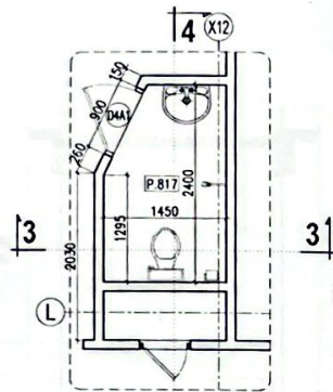
M.BẰNG WC P.817
