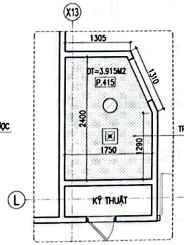
M.BẢNG TRẦN WC P.415
