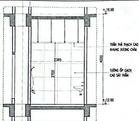
L CẮT 2-2
