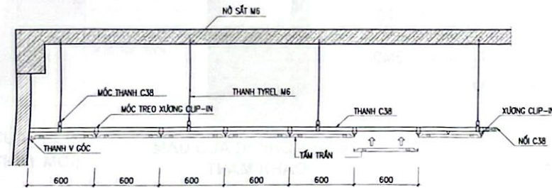
CHI TIẾT MẶT CẮT
