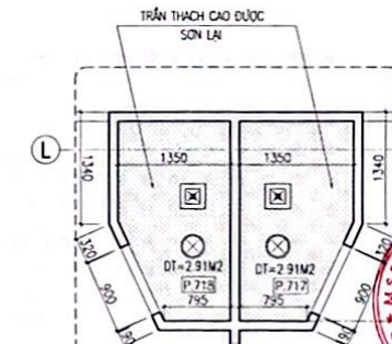
M.BẰNG TRẦN WC P.717 & P.718
