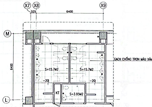
MẶT BẰNG KHU VỆ SINH WC - 01 TẦNG (4 - 8) - HIỆN TRẠNG
