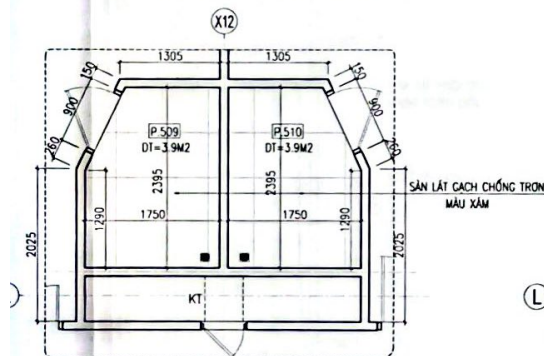
M.BẰNG WC P.509 & P.510
