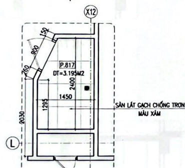
M.BẰNG LÁT SÀN WC P.817
