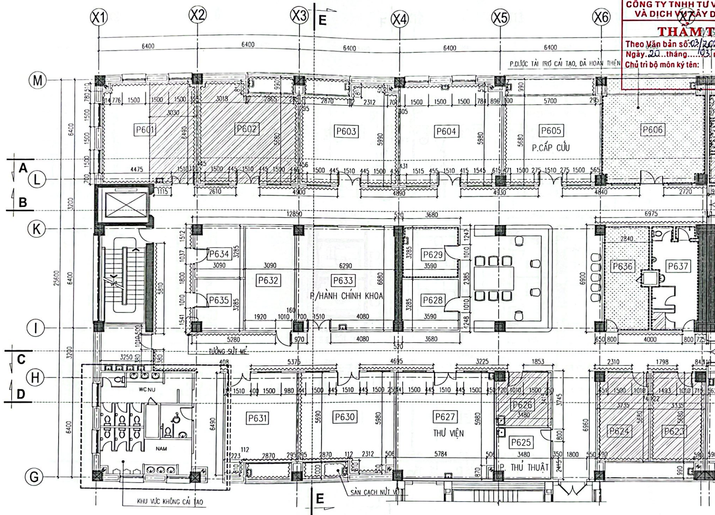
MẶT BẰNG HIỆN TRẠNG TƯỜNG & TRẦN TẦNG 6 (P1)
