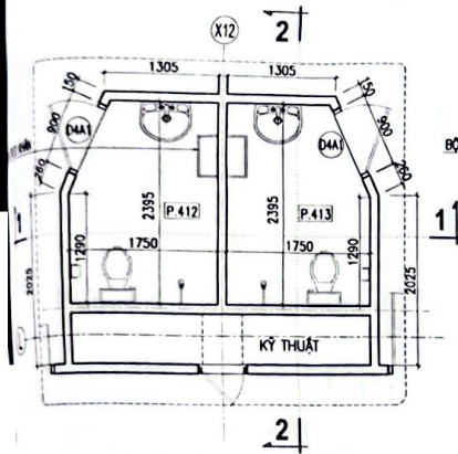
M.BẢNG WC P.412 & P.413
