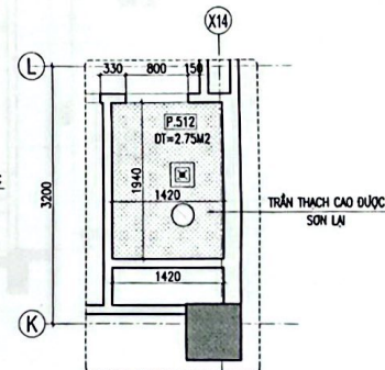
M.BẢNG TRẦN WC P.512
