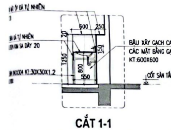
BÀN ĐÁ 1
