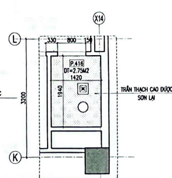
M.BẢNG TRẦN WC P.416
