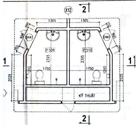
M.BẰNG WC P.509 & P.510
