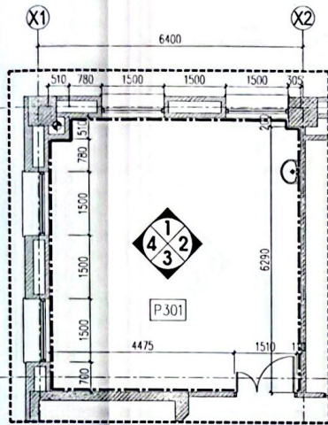
MẶT BẰNG PHÒNG ĐIỂN HÌNH HIỆN TRẠNG CHƯA ỐP GẠCH (CÓ TRẦN GIẢ)
