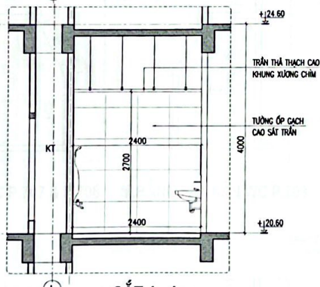
L CẮT 4-4
