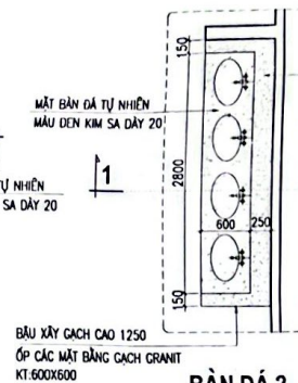
BÀN ĐÁ 2
