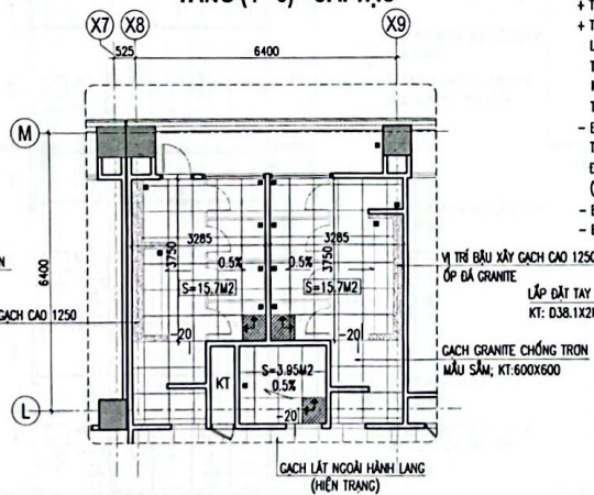
MẶT BẰNG LÁT SÀN KHU VỆ SINH WC - 01 CẢI TẠO
