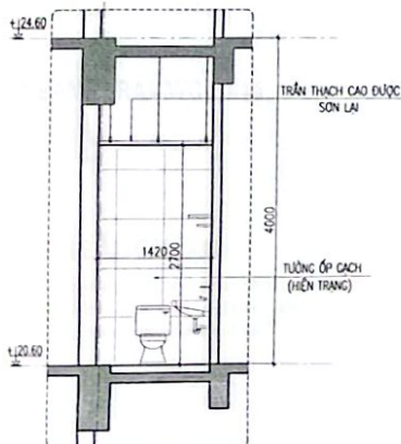
X14 CẮT 13-13
