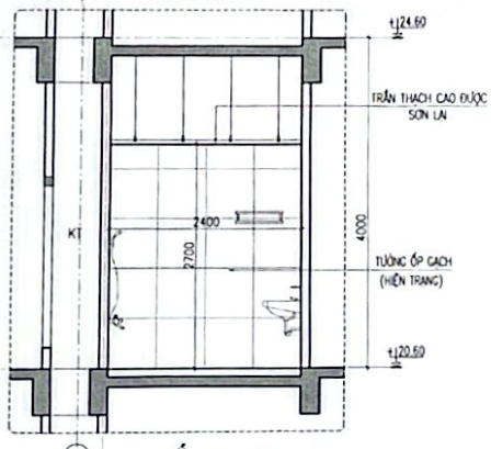
L CẮT 12-12
