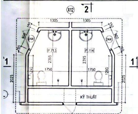
M. BẢNG WC P.713 & P.714
