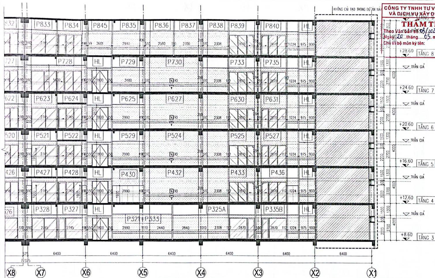
MẶT CẮT CẢI TẠO H-H (P2)
