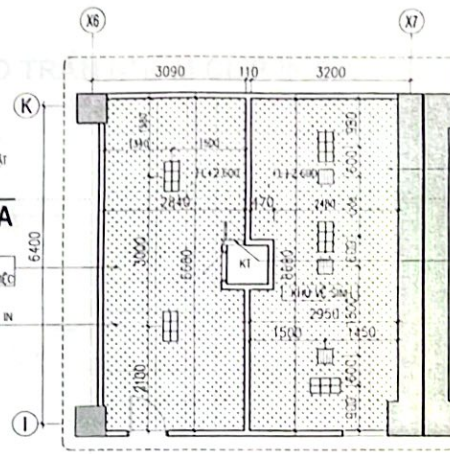
M.BẰNG TRẦN VỆ SINH NHÂN VIÊN TẦNG 4,5,6,7,8 (LÀM MỚI)
