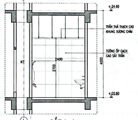
CẮT 4-4
