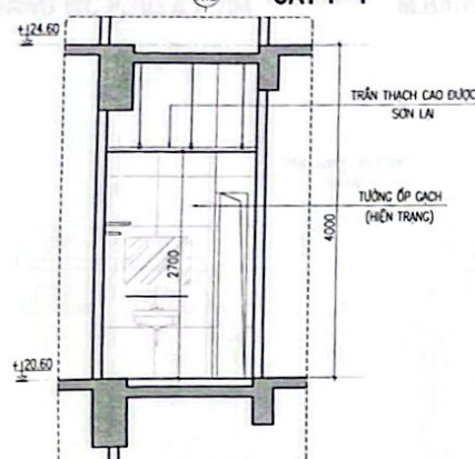
X13 CẮT 3-3
