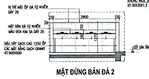
BÀN ĐÁ 2
