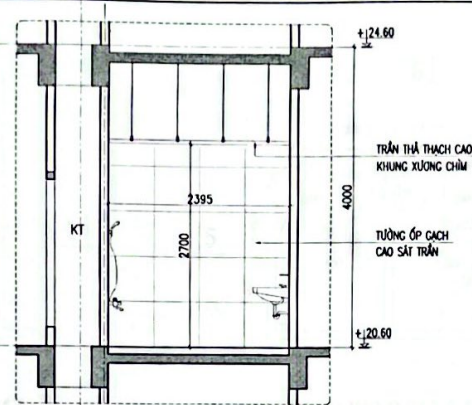
CẮT 2-2
