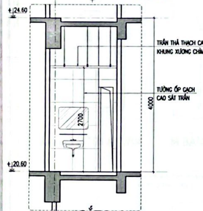
X13 CẮT 3-3
