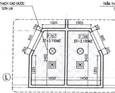
M.BẰNG TRẦN WC P.707 & P.708
