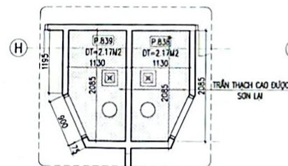
M.BẰNG LÁT TRẦN P.838 & P.839
