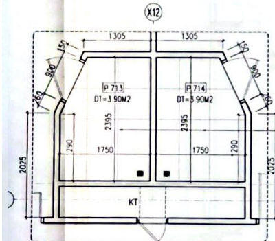
M. BẢNG LÁT SÀN WC P.713 & P.714
