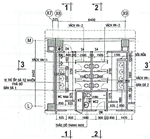
MẶT BẰNG KHU VỆ SINH WC - 01 TẦNG (4 - 8) - HIỆN TRẠNG
