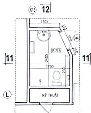
M.BẦNG WC P.715
