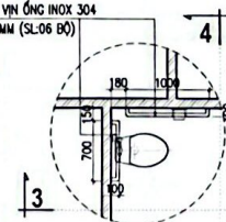
CHI TIẾT CT-1
