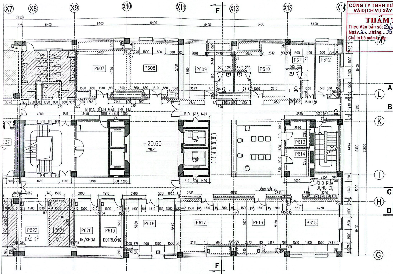
MẶT BẰNG HIỆN TRẠNG TƯỜNG & TRẦN TẦNG 6 (P2)
