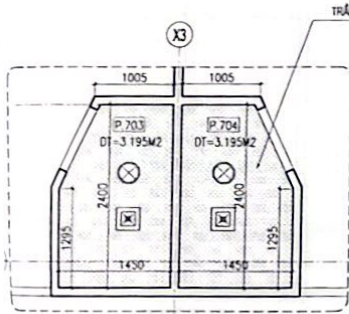
M.BẰNG TRẦN WC P.703 & P.704
