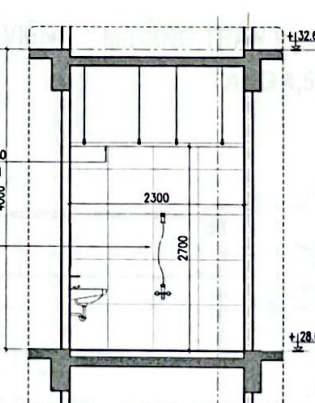
CẮT 14-14
