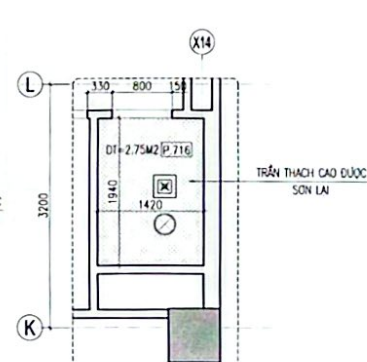
M.BẦNG TRẦN WC P.716
