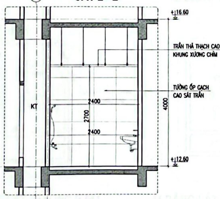
L CẮT 4-4
