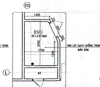
M.BẰNG WC P.511
