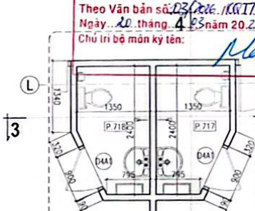
M.BẰNG WC P.717 & P.718
