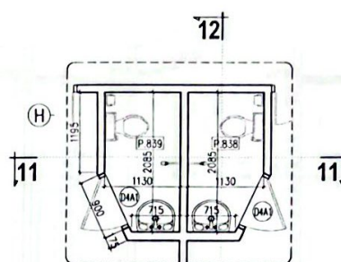
M.BẰNG WC P.838 & P.839
