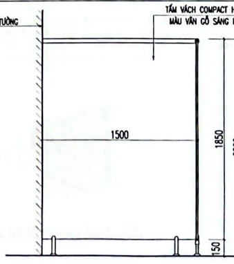
VÁCH NGĂN VN - 2 (KHOANG XÍ)
