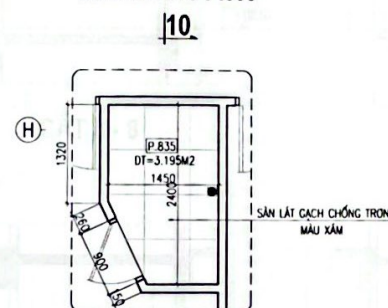
M.BẰNG LÁT SÀN WC P.835
