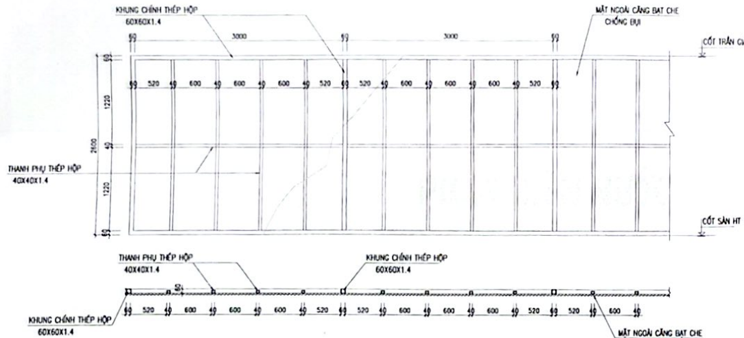
CHI TIẾT HỆ KHUNG CHE BẠT (ĐIỂN HÌNH)
