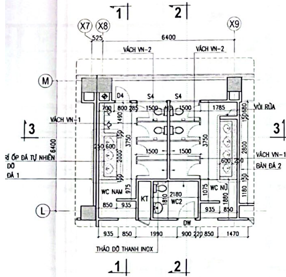
MẶT BẰNG KHU VỆ SINH WC - 01 TẦNG 3 - HIỆN TRẠNG
