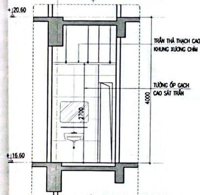
CẮT 3-3
