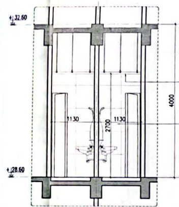
CẮT 7-7
