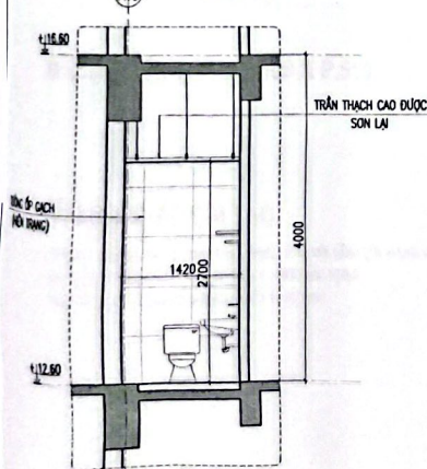
X14 CẮT 5-5
