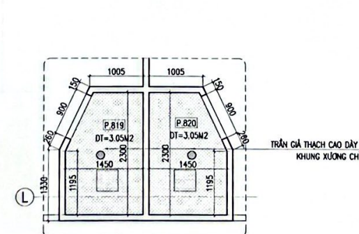
M.BẰNG TRẦN P.819 & P.820
