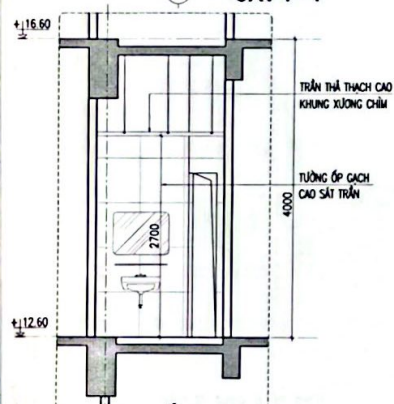
X13 CẮT 3-3
