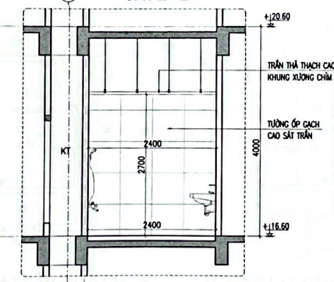
CẮT 4-4
