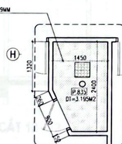
M.BẰNG TRẦN WC P.835
