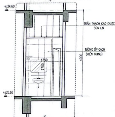
X13 CẮT 11-11
