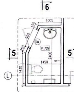
M.BẰNG WC P.709
