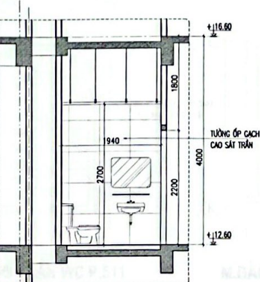
K CẮT 6-6
