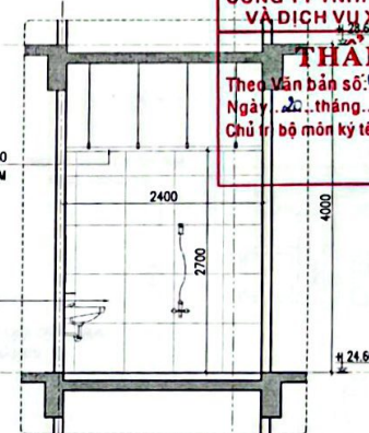
CẮT 10-10
