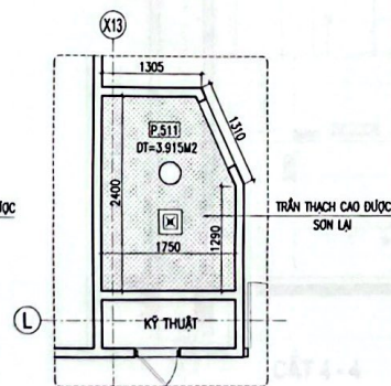
M.BẢNG TRẦN WC P.511
