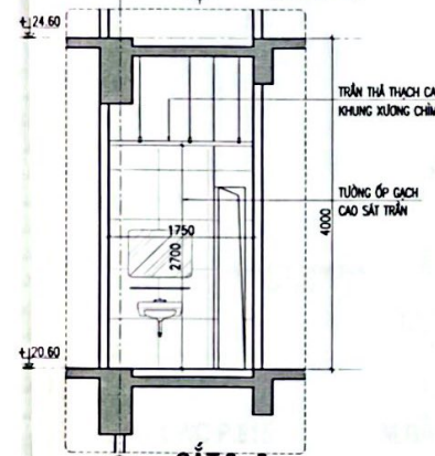
CẮT 3-3
