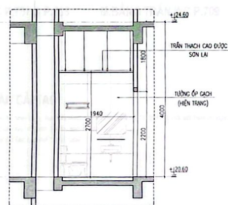
K CẮT 6-6
