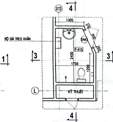
M.BẢNG WC P.415
