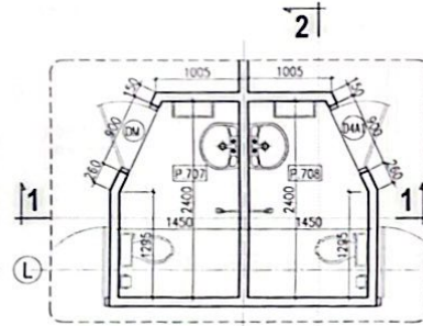
M.BẰNG WC P.707 & P.708
