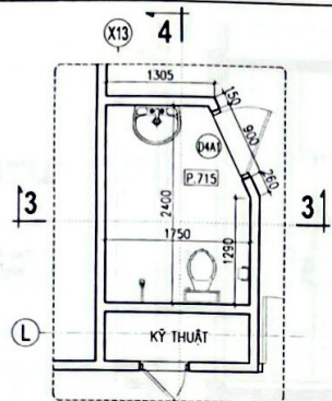
M. BẢNG WC P.715
