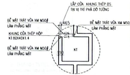
TRỤC KỸ THUẬT SỐ 1 SAU KHI LẮP CỬA DS CÁCH CỐT SÀN HOÀN THIỆN +2.750 (KHOẢNG TRỐNG GIỮA TRẦN GẢ VÀ TRẦN BÊ TÔNG)
