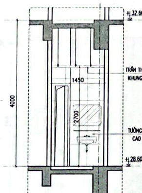
CẮT 9-9
