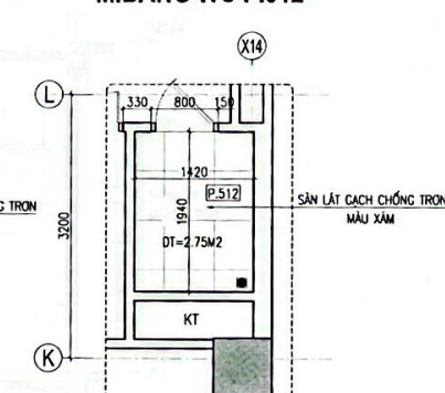
M.BẰNG LÁT SÀN WC P.512
