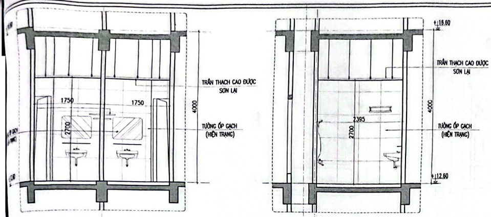
X12 CẮT 1-1
