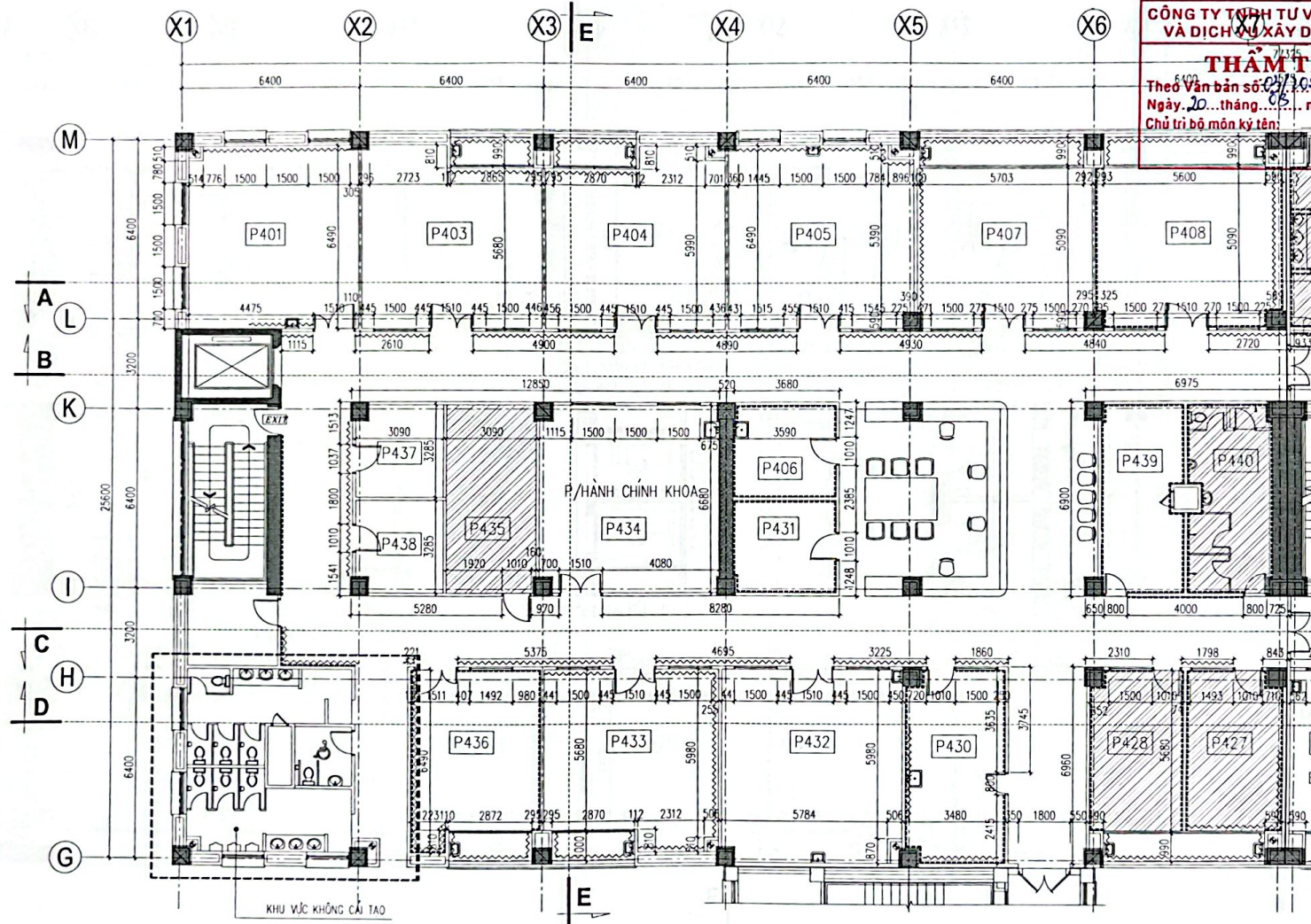
MẶT BẰNG HIỆN TRẠNG TƯỜNG & TRẦN TẦNG 4 (P1)
