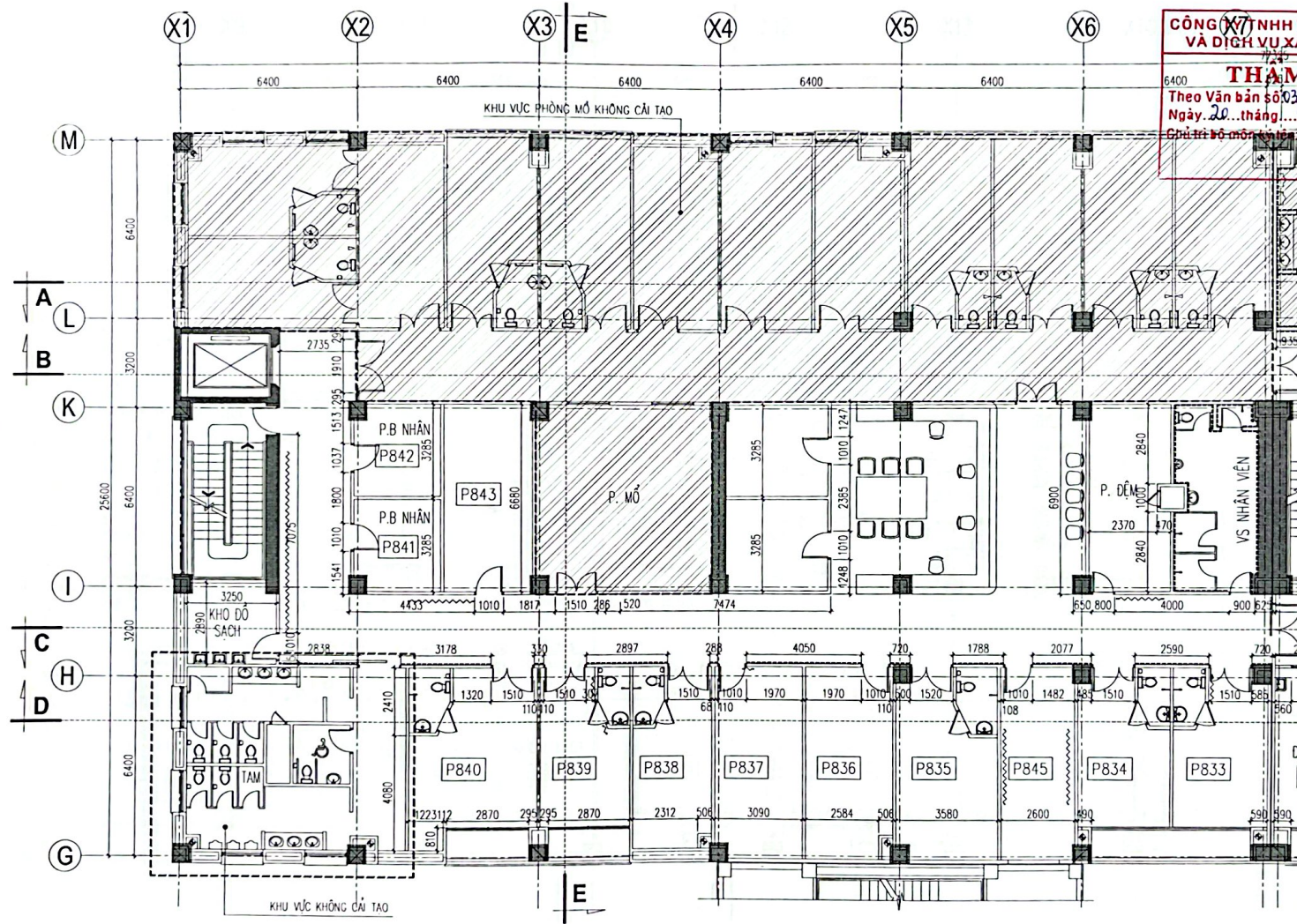
MẶT BẰNG HIỆN TRẠNG TƯỜNG & TRẦN TẦNG 8 (P1)
