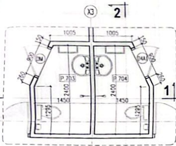
M.BẰNG WC P.703 & P.704
