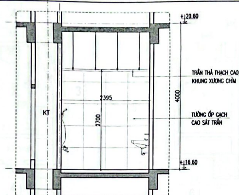
CẮT 2-2
