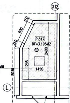
M.BẰNG TRẦN WC P.817
