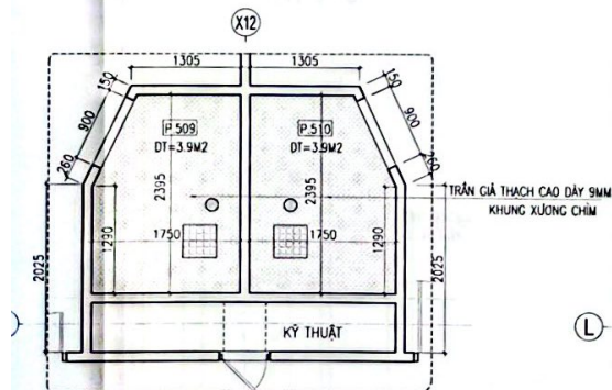
M.BẰNG TRẦN WC P.509 & P.510
