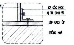
CHI TIẾT KE GÓC
