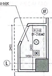
M.BẰNG TRẦN WC P.710
