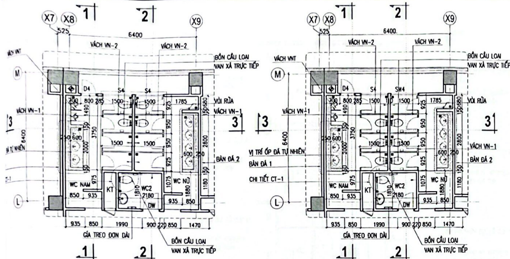
MẶT BẰNG KHU VỆ SINH WC - 01 TẦNG 3 - CẢI TẠO
