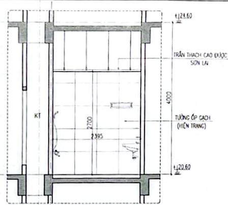
L CẮT 10-10
