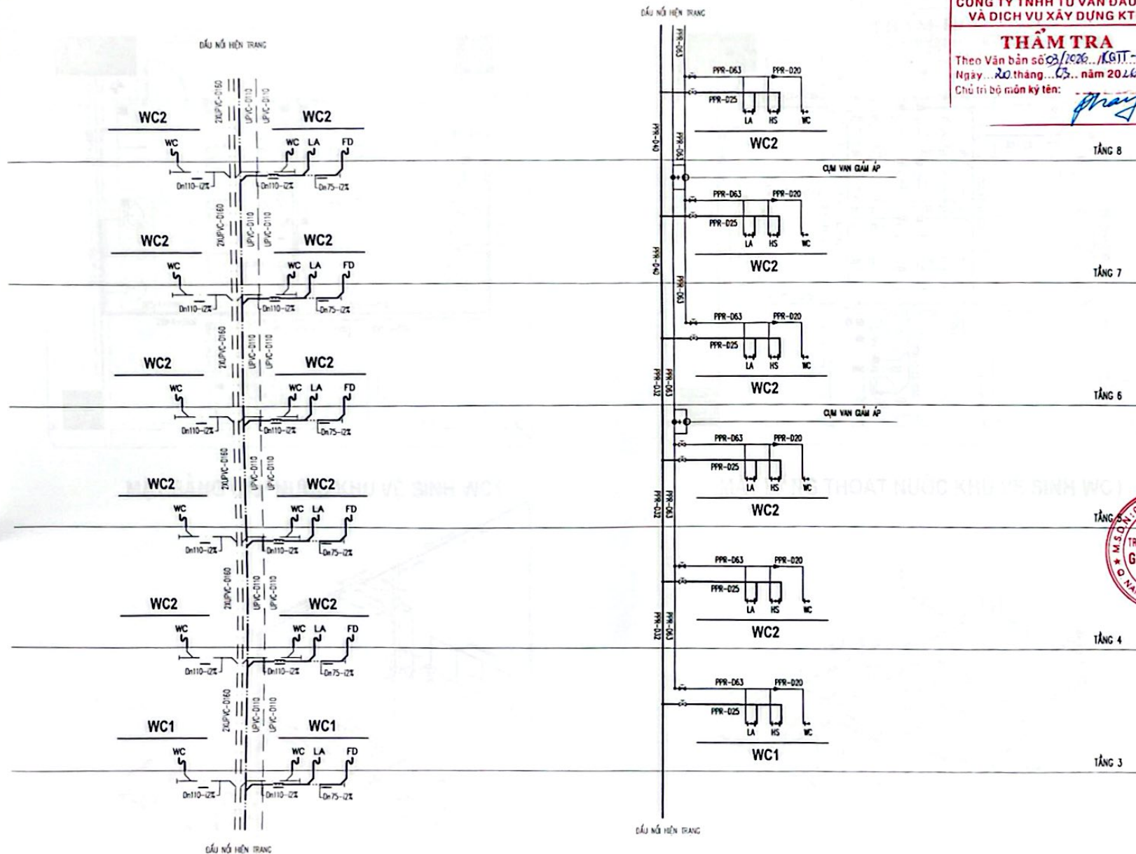
SƠ ĐỒ CẤP THOÁT NƯỚC VỆ SINH CHUNG
