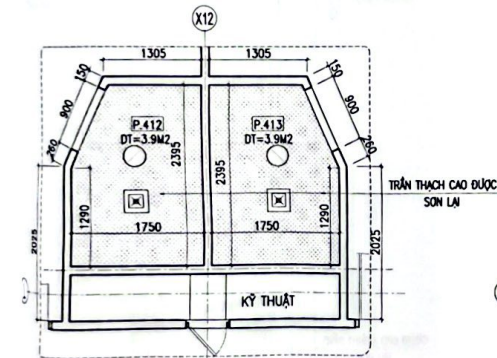
M.BẢNG TRẦN WC P.412 & P.413
