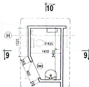
M.BẰNG WC P.835
