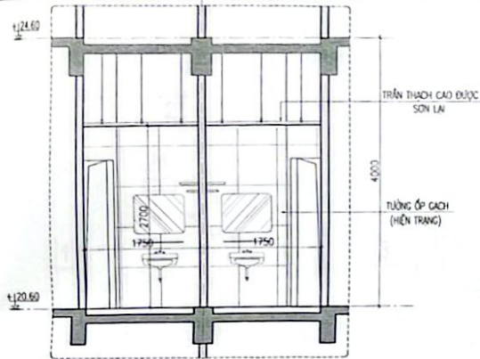
X12 CẮT 9-9
