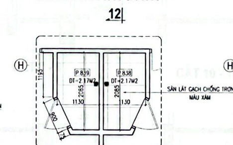
M.BẰNG WC P.838 & P.839
