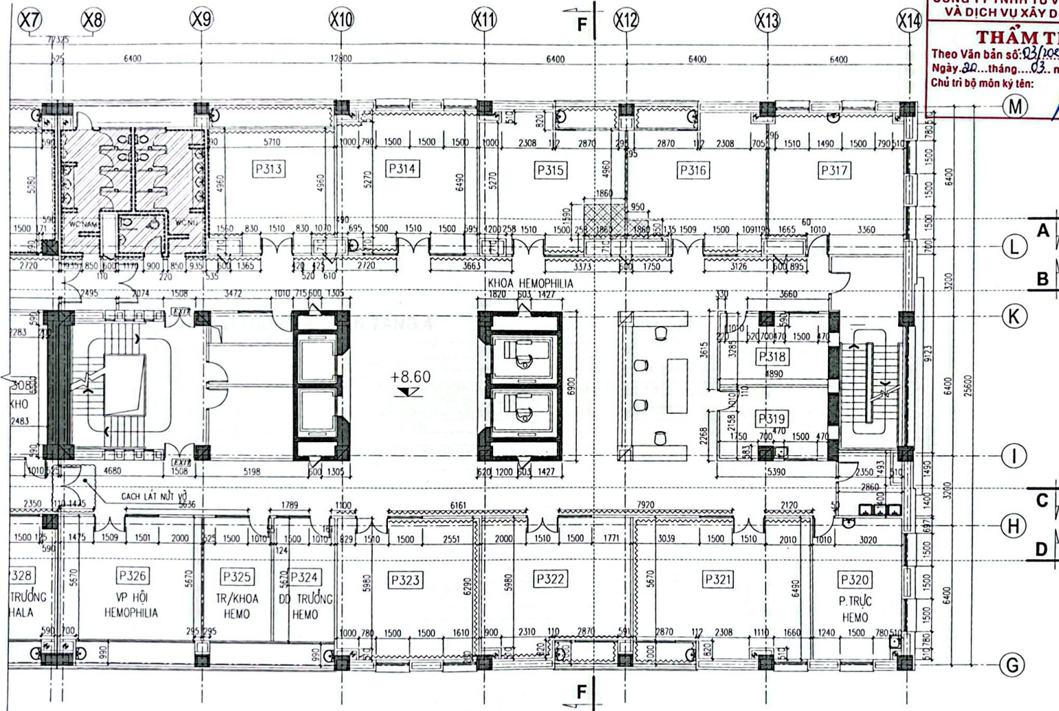
MẶT BẰNG HIỆN TRẠNG TƯỜNG & TRẦN TẦNG 3 (P2)
