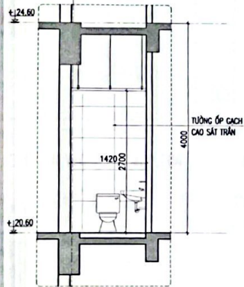
X14 CẮT 5-5
