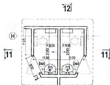
M.BẰNG WC P.838 & P.839
