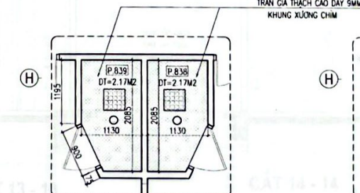
M.BẰNG LÁT TRẦN P.838 & P.839
