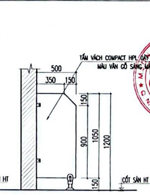
VÁCH NGĂN VTN
