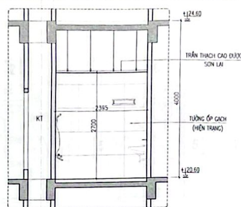
L CẮT 2-2
