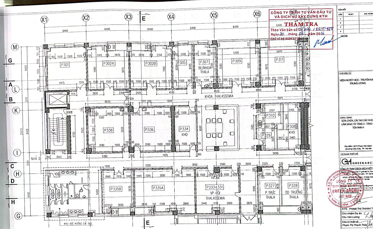
MẶT BẰNG CẢI TẠO TƯỜNG TẦNG 3 (P1)
