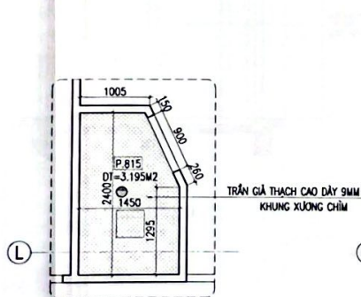
M.BẰNG TRẦN WC P.815
