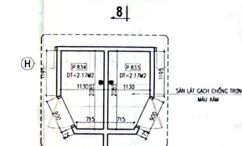
M.BẰNG WC P.833 & P.834
