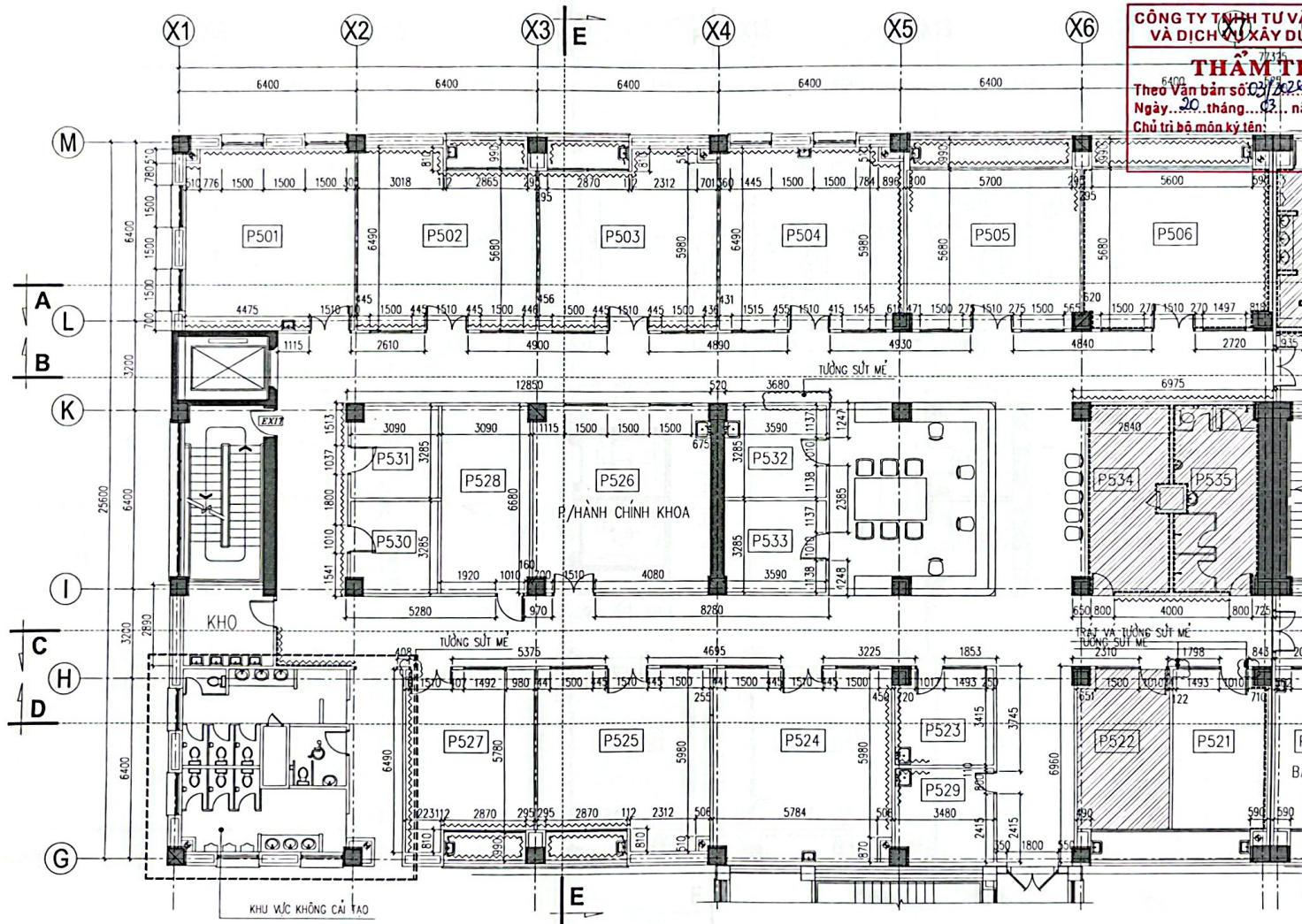
MẶT BẰNG HIỆN TRẠNG TƯỜNG & TRẦN TẦNG 5 (P1)
