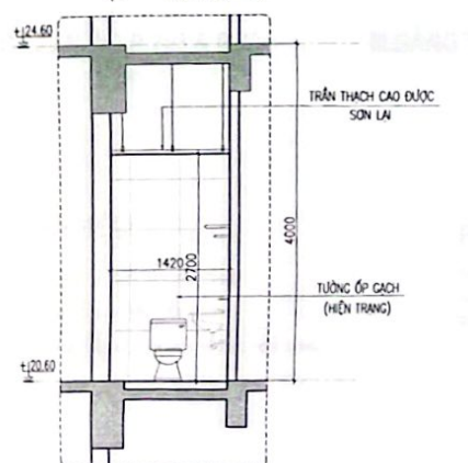
X14 CẮT 5-5
