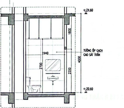
CẮT 6-6
