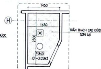
M.BẰNG TRẦN WC P.840
