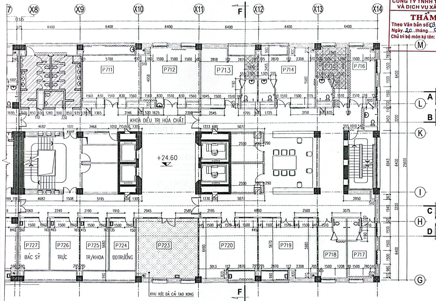
MẶT BẰNG HIỆN TRẠNG TƯỜNG & TRẦN TẦNG 7 (P2)
