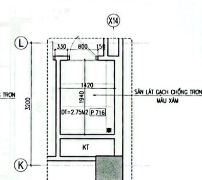
M. BẢNG LÁT SÀN WC P.716
