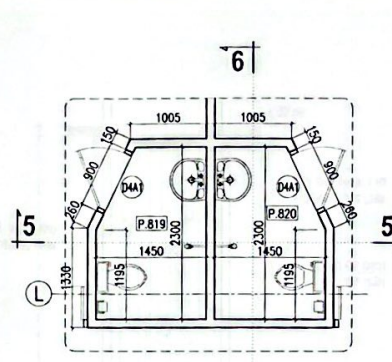
M.BẰNG WC P.819 & P.820
