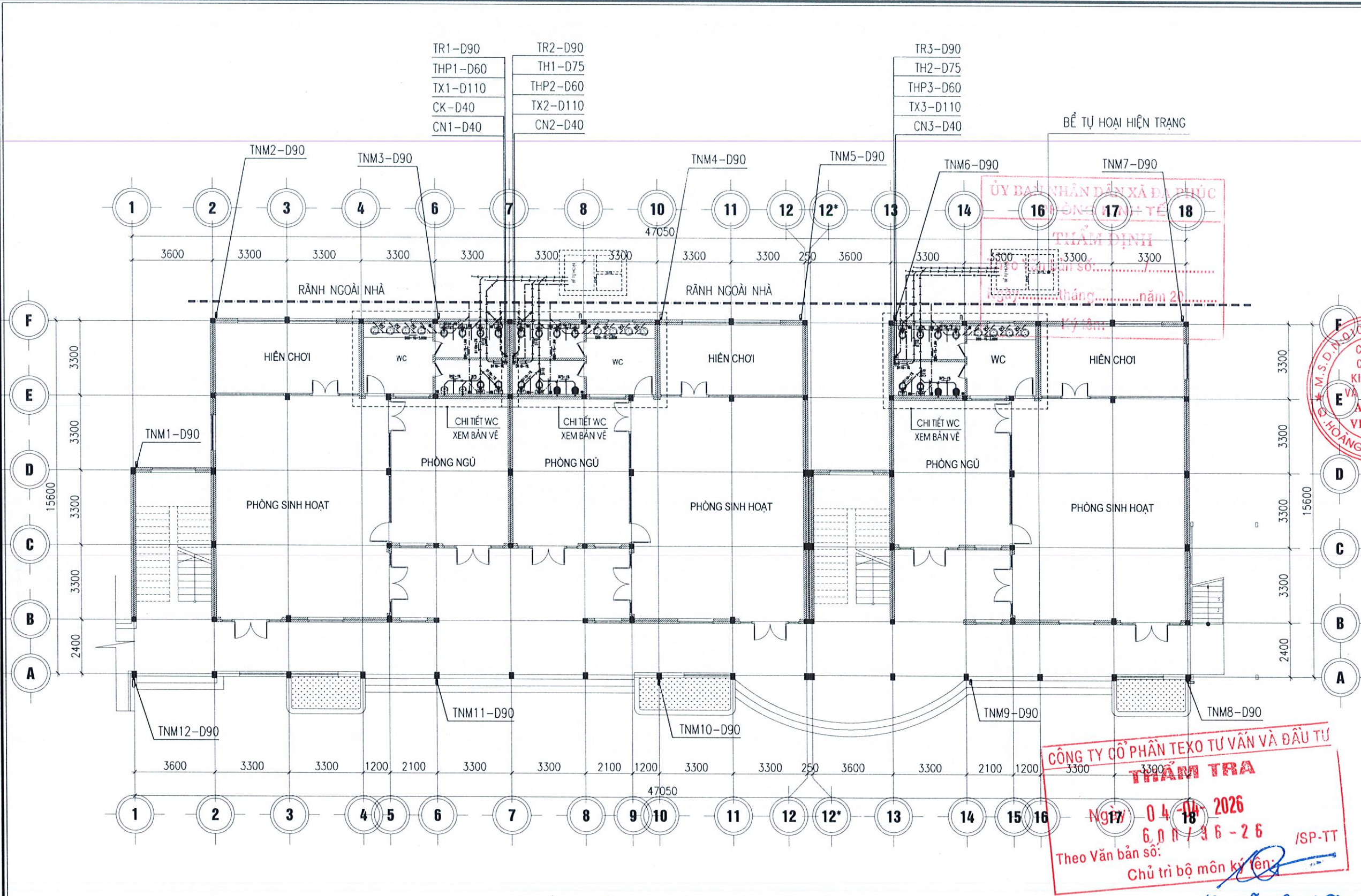
MẶT BẰNG CẢI TẠO CẤP THOÁT NƯỚC TẦNG 1
