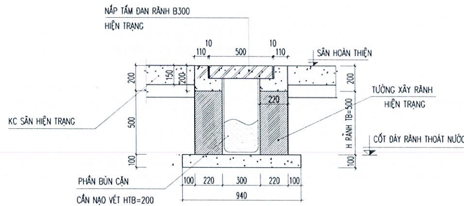
MẶT CẮT RĂNG B300 HIỆN TRẠNG CẢI TẠO
