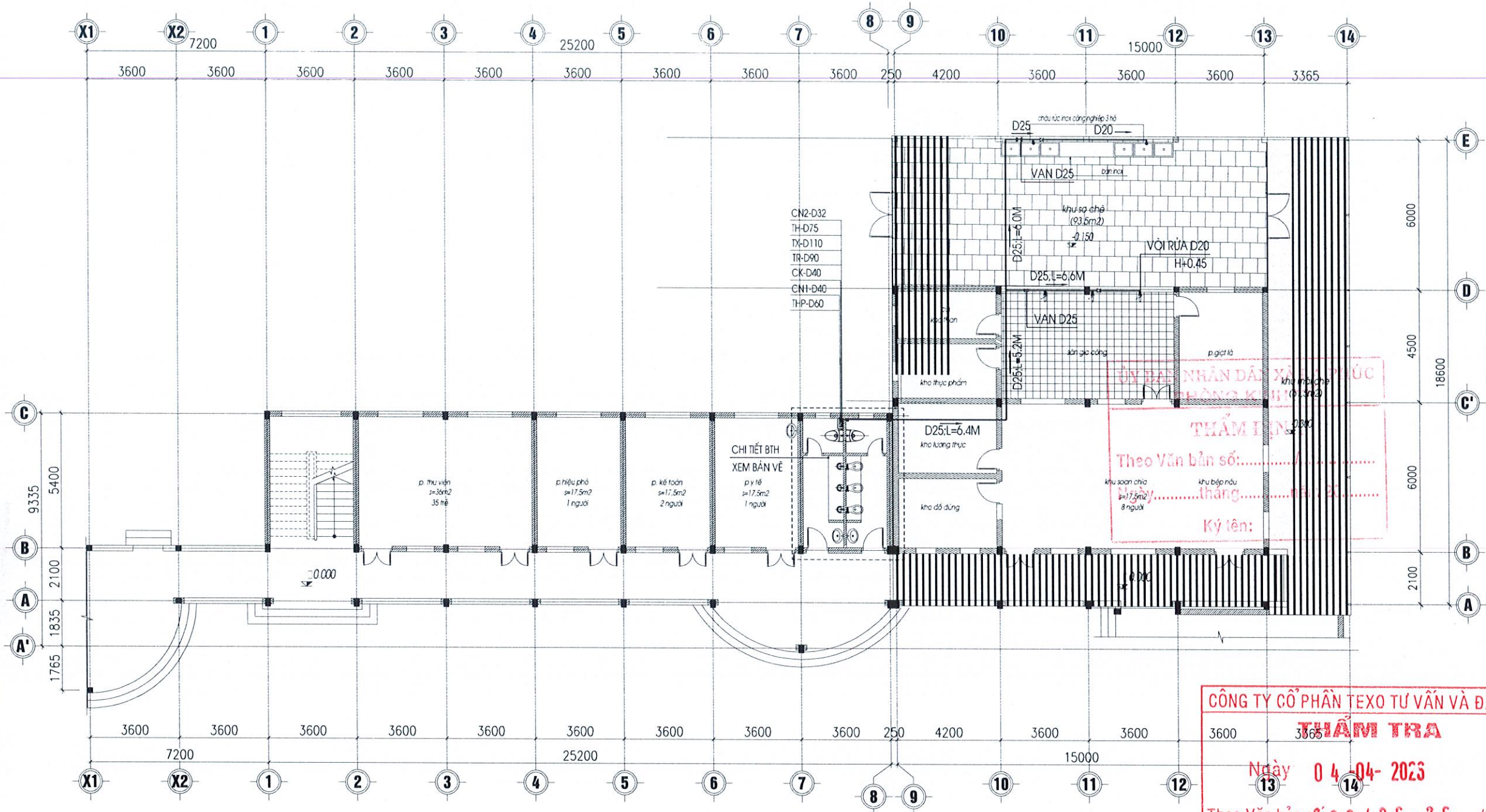
MẶT BẰNG CẢI TẠO CẤP THOÁT NƯỚC TẦNG 1
