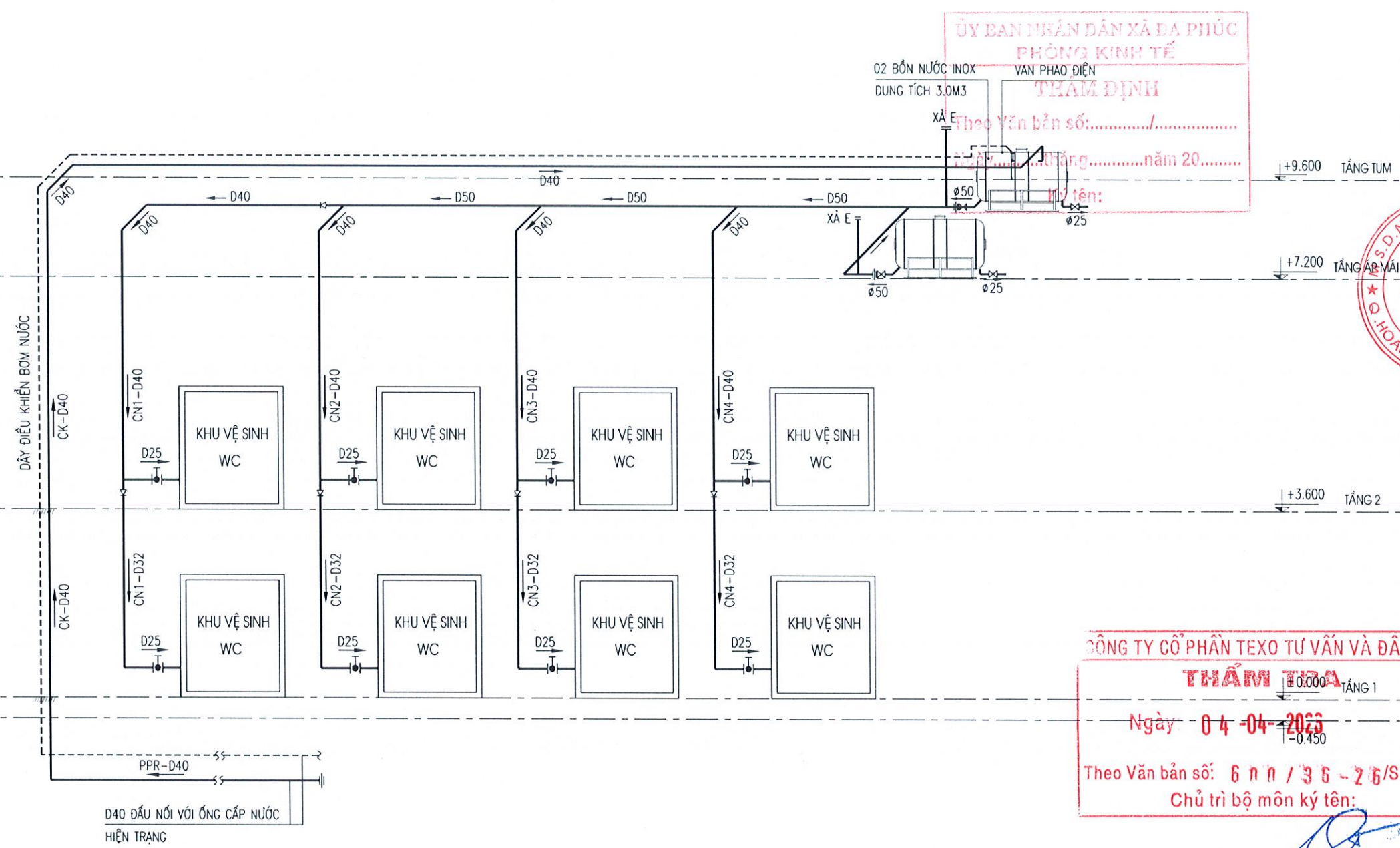
SƠ ĐỒ NGUYÊN LÝ CẤP NƯỚC SINH HOẠT
