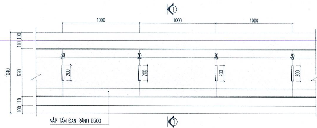
MẶT BẰNG RĂNG THOÁT NƯỚC B300 (KHỐI LƯỢNG: L=263,0 M)
