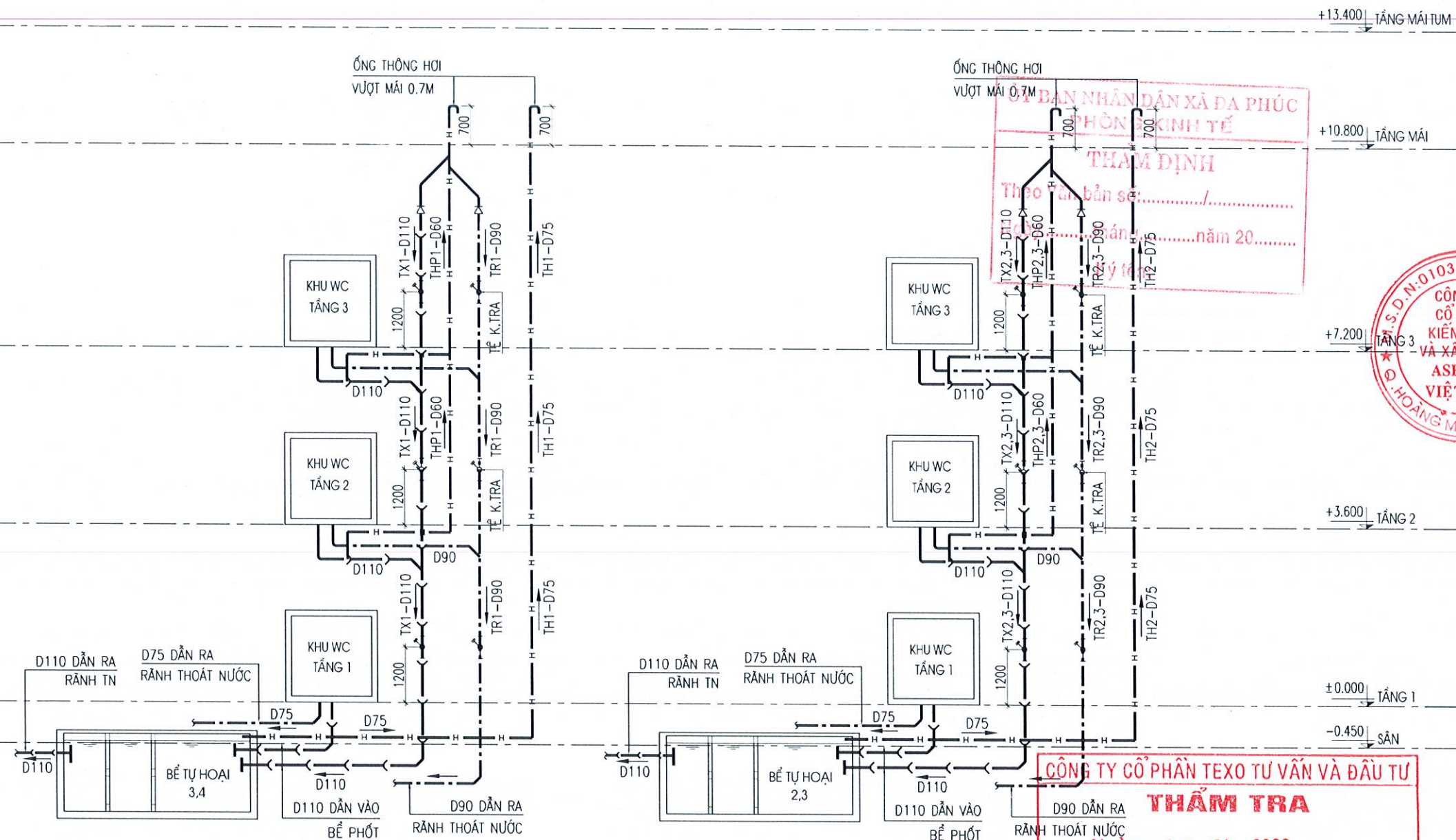
SƠ ĐỒ NGUYÊN LÝ THOÁT NƯỚC SINH HOẠT
