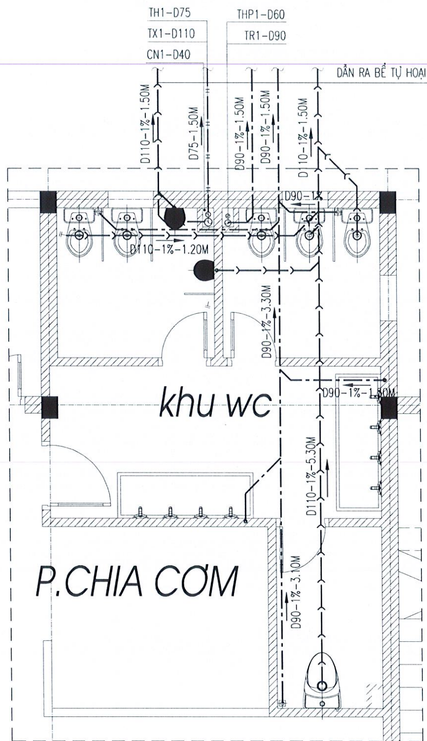
MẶT BẰNG CẤP NƯỚC KHU WC TẦNG 1
