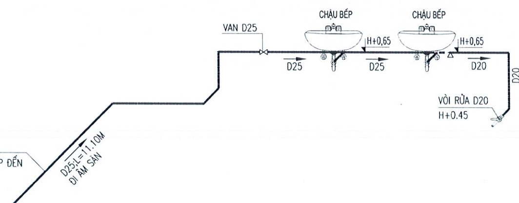
SƠ ĐỒ KHÔNG GIAN CẤP NƯỚC KHU BẾP
