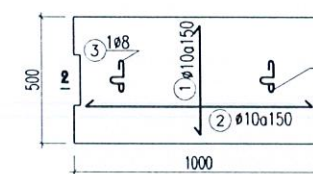
BỐ TRÍ THÉP TẮM ĐAN RĂNG B300 THAY MỚI
