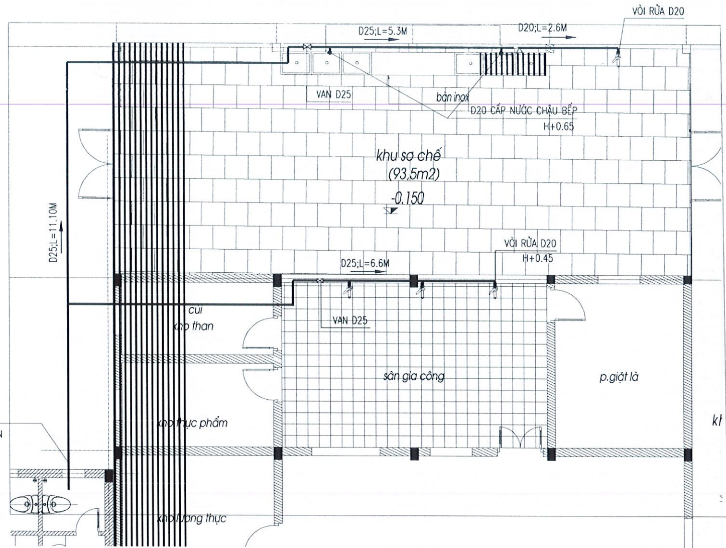
MẶT BẰNG CẤP NƯỚC KHU BẾP
