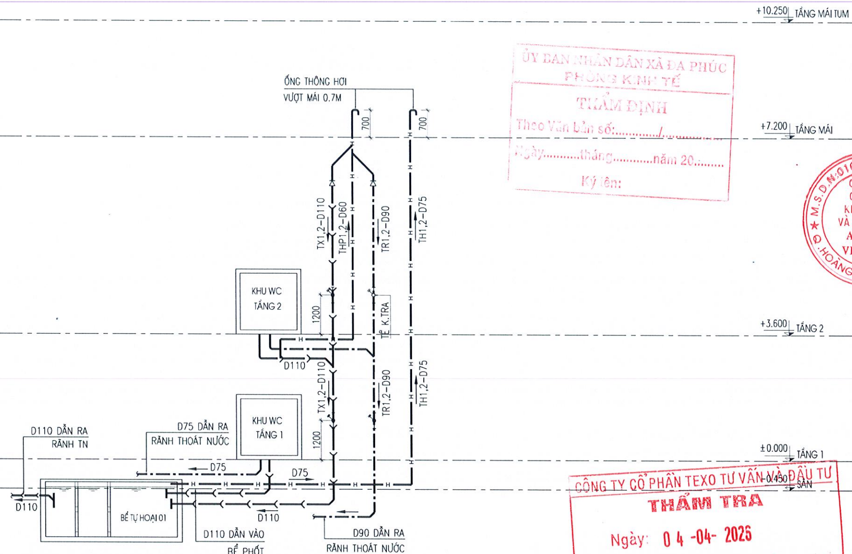
SƠ ĐỒ NGUYÊN LÝ THOÁT NƯỚC SINH HOẠT
