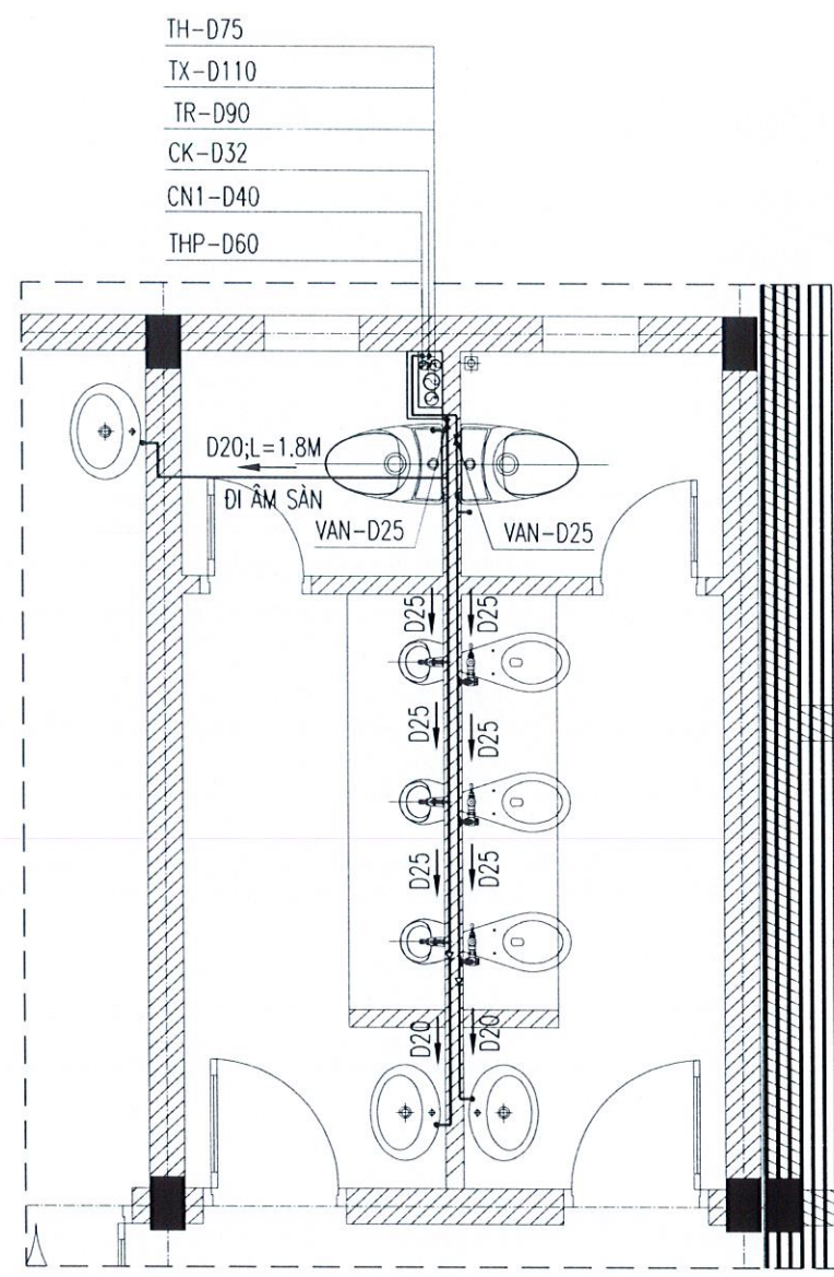
MẶT BẰNG CẤP NƯỚC KHU WC TẦNG 1
