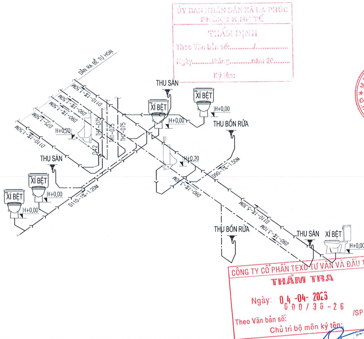
SƠ ĐỒ KHÔNG GIAN CẤP NƯỚC WC TẦNG 1
