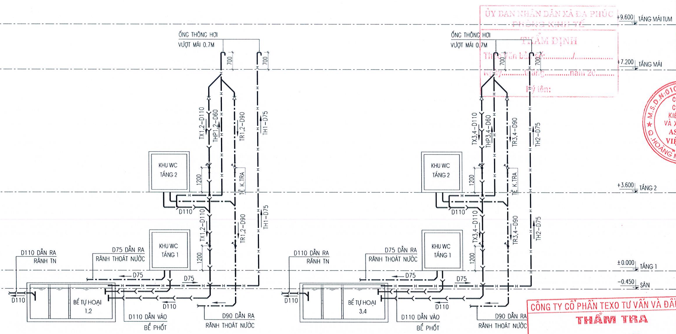
SƠ ĐỒ NGUYÊN LÝ THOÁT NƯỚC SINH HOẠT
