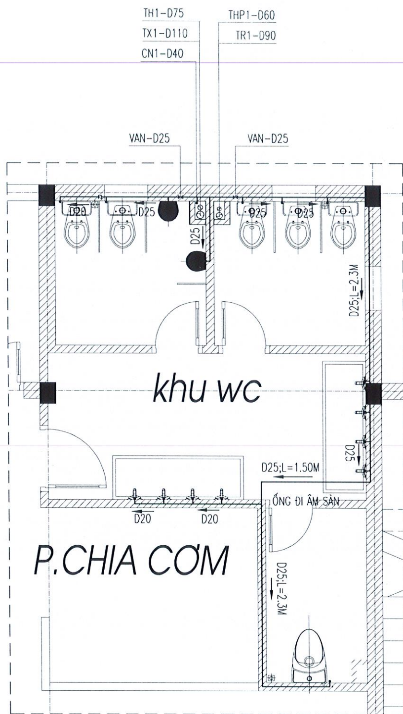
MẶT BẰNG CẤP NƯỚC KHU WC TẦNG 2
