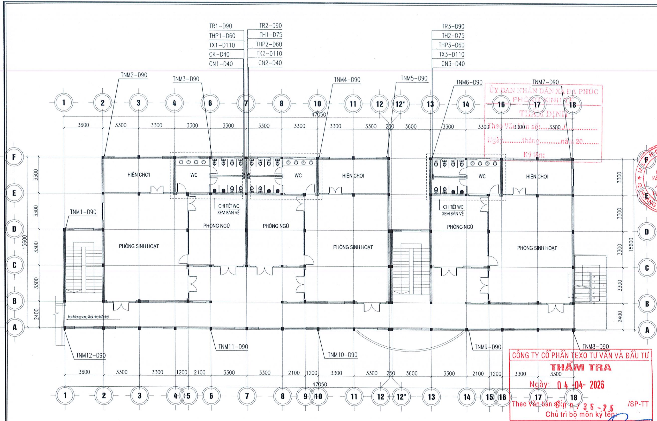
MẶT BẰNG CẢI TẠO CẤP THOÁT NƯỚC TẦNG 2
