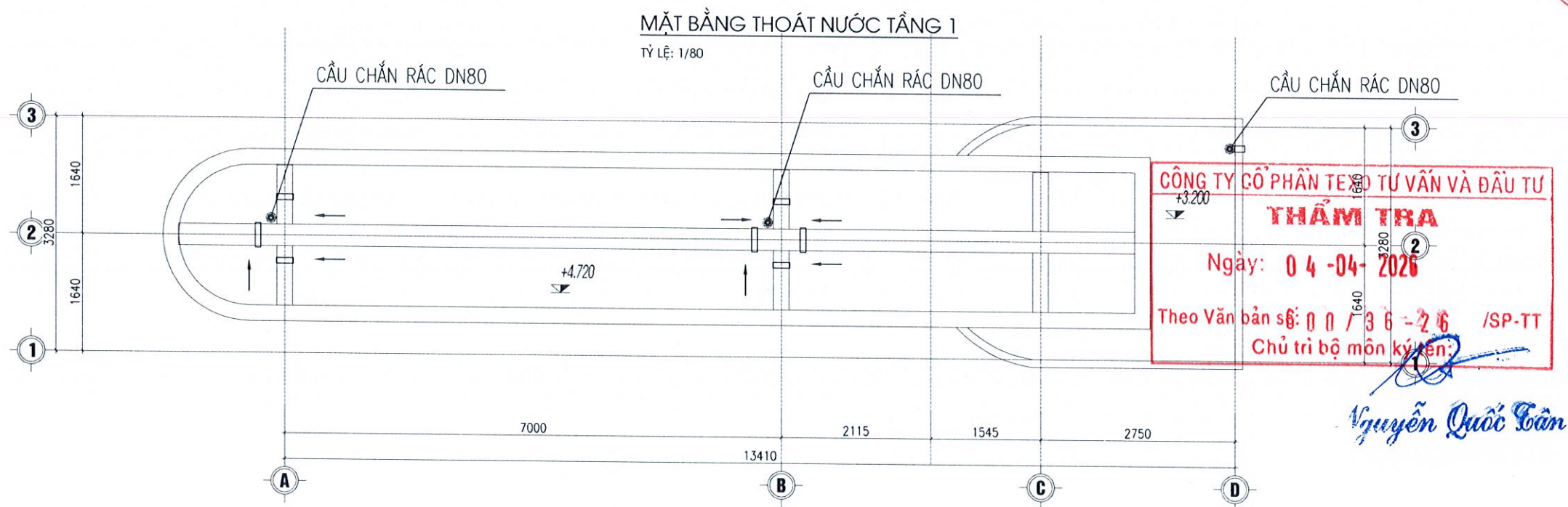
MẶT BẰNG THOÁT NƯỚC MÁI TỶ LỆ: 1/80
