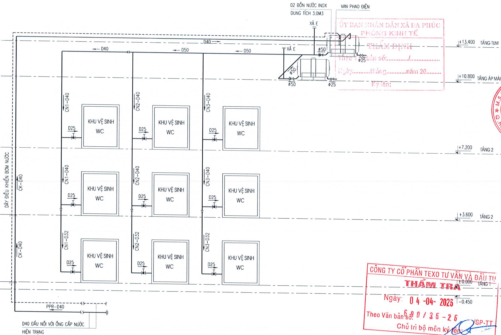
SƠ ĐỒ NGUYÊN LÝ CẤP NƯỚC SINH HOẠT
