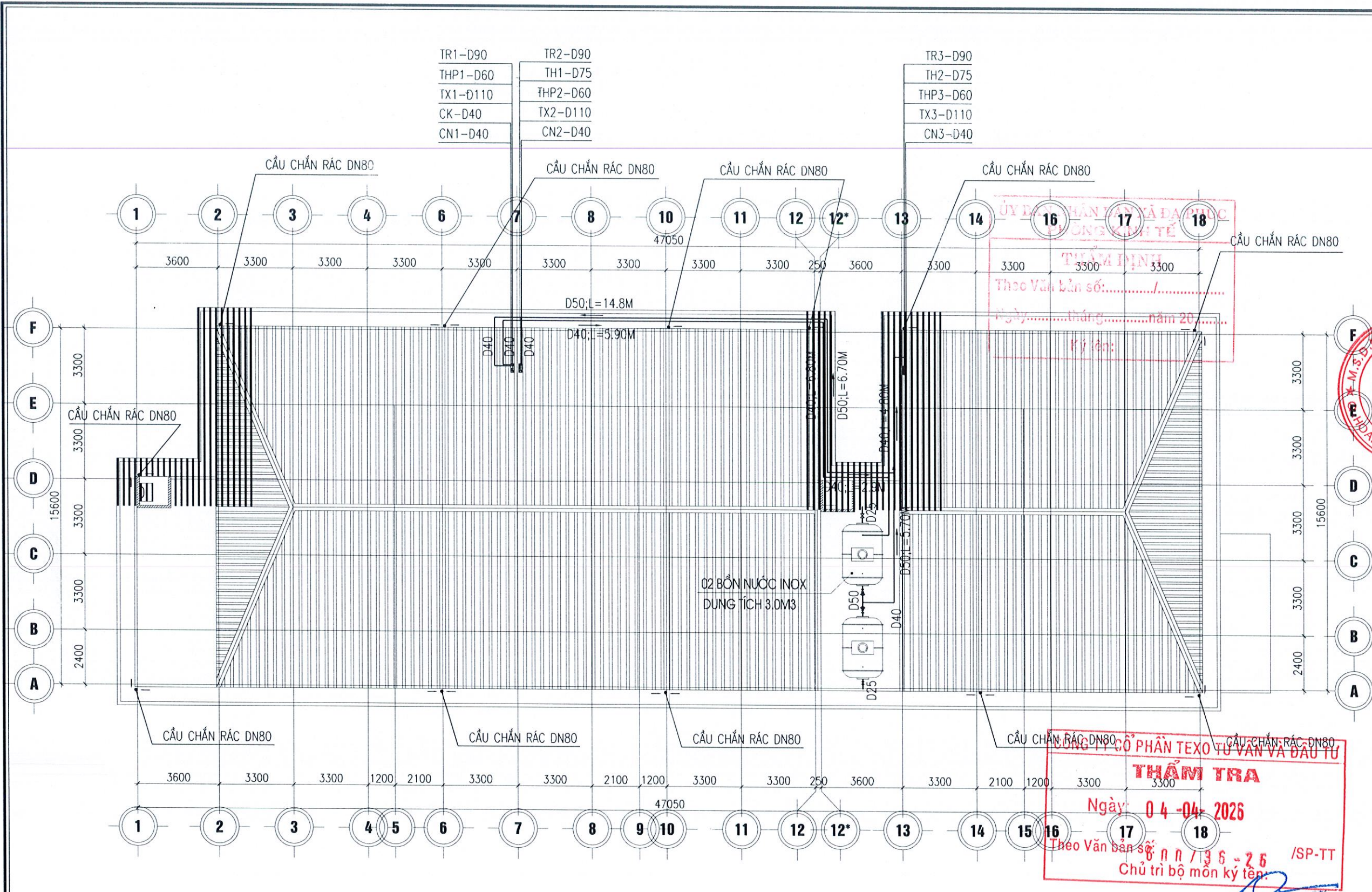
MẶT BẰNG CẢI TẠO CẤP THOÁT NƯỚC TẦNG MÁI
