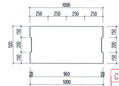
TẮM ĐAN RĂNG B300 THAY MỚI
