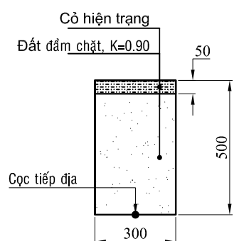
MẶT CẮT: CO01
