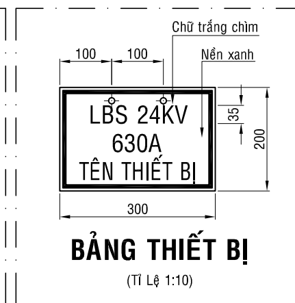
BẢNG BÁO NGUY HIỂM (Tỉ Lệ 1:10)
