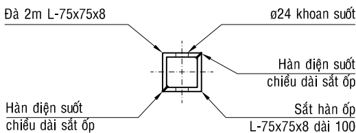
MẶT CẮT X-X
