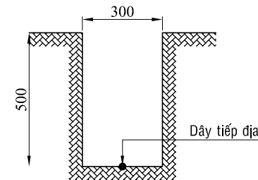
RÃNH TIẾP ĐỊA (TL 1:20)
