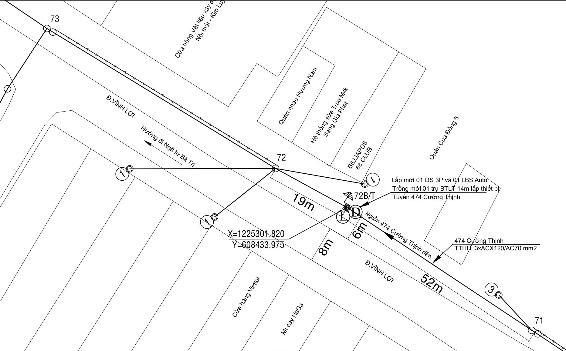
TRỤ 72 TUYẾN 474 CƯỜNG THỊNH (Hiện hữu)
