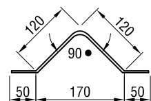
CHI TIẾT A - SẮT DẸP 50x5 (TỈ LỆ 1:10)
