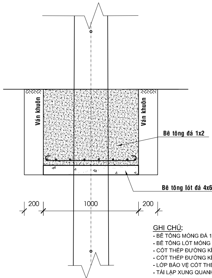
MẶT CẮT 1-1
