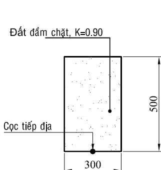
MẶT CẮT: DA01
