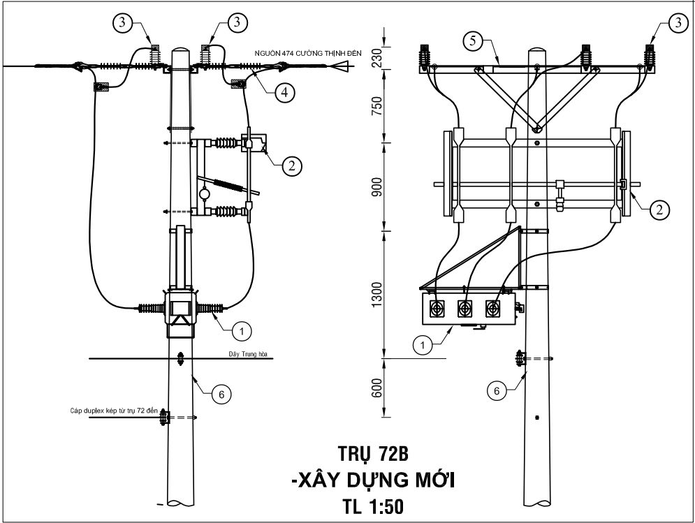
TRỤ 72B TUYẾN 474 CƯỜNG THỊNH (xây dựng mới tại vị trí cột hiện có của dân)
