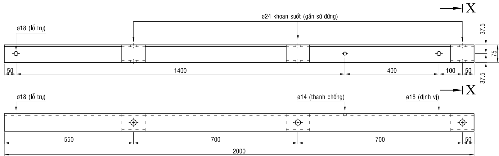
ĐÀ A - SẮT L-75x75x8 DÀI 2m (Tỉ lệ 1:10)
