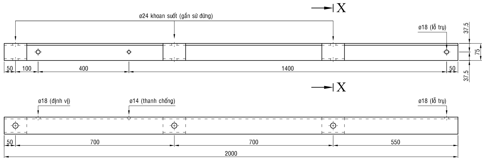
ĐÀ A - SẮT L-75x75x8 DÀI 2m (Tỉ lệ 1:10)
