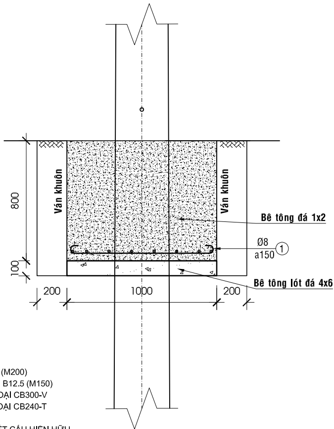
MẶT CẮT 2-2
