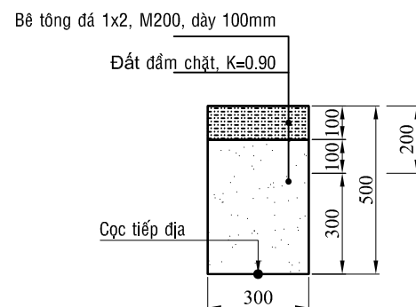
MẶT CẮT: BV01
