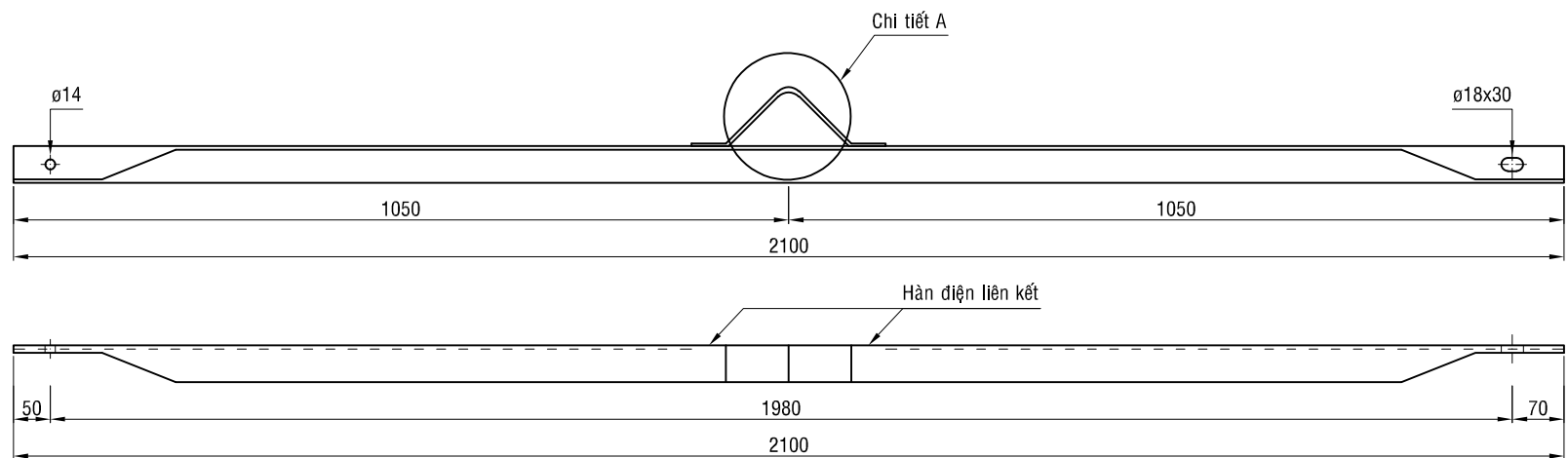
THANH CHỐNG - SẮT L-50x50x5 DÀI 2,1m (Tỉ lệ 1:10)
