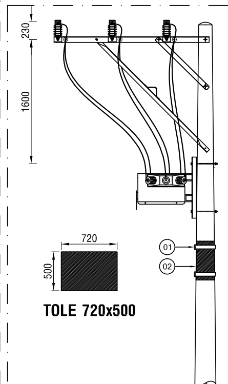
CHI TIẾT TẮM CHỐNG ĐỘNG VẬT XÂM NHẬP
