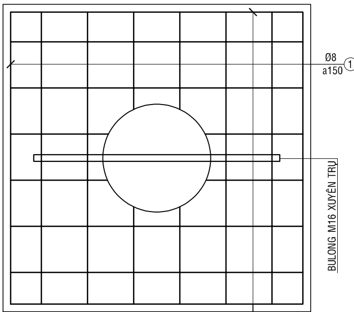
MẶT BẰNG BỐ TRÍ THÉP
