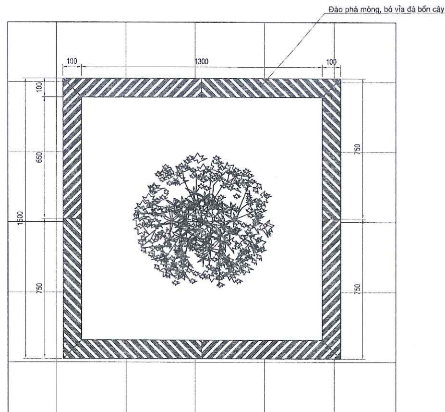
MẶT BẰNG HIỆN TRẠNG HỒ TRỒNG CÂY LOẠI 4 (TỶ LỆ 1/15)
