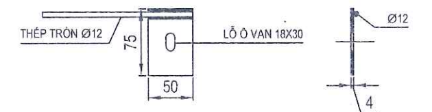
HÌNH A: TAI BẮT TIẾP ĐỊA D=4MM
