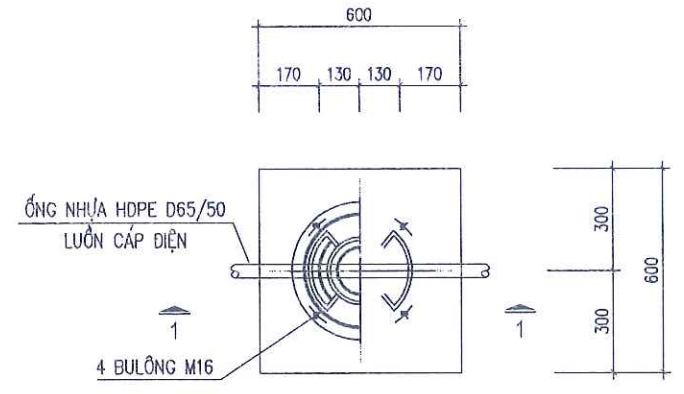
MÓNG CỘT ĐÈN CHIẾU SÁNG
