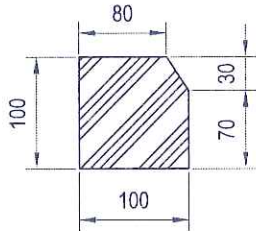
MẶT CẮT 1-1 (TỶ LỆ 1/15)
