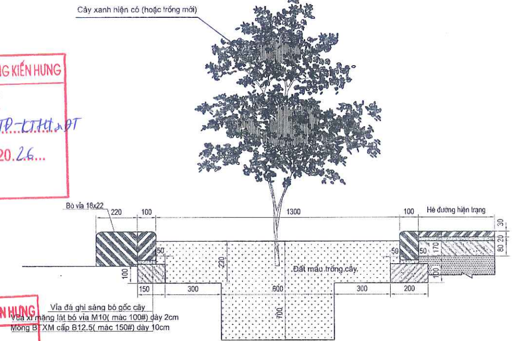
CẮT NGANG CẢI TẠO HỒ TRỒNG CÂY LOẠI 5
