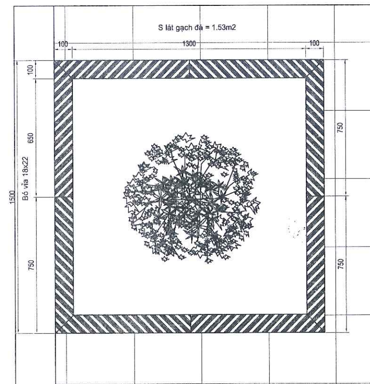
CHI TIẾT SỬA CHỮA SCB5
