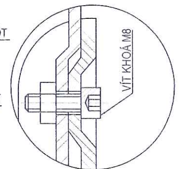
CHI TIẾT B
