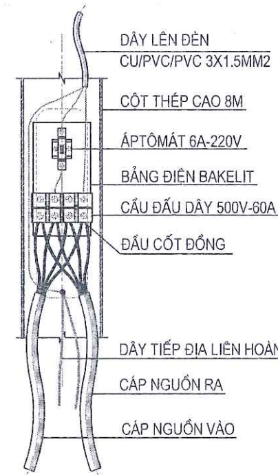
BẢNG ĐIỆN CỬA CỘT
