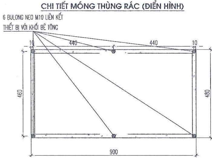
MẶT BẰNG
