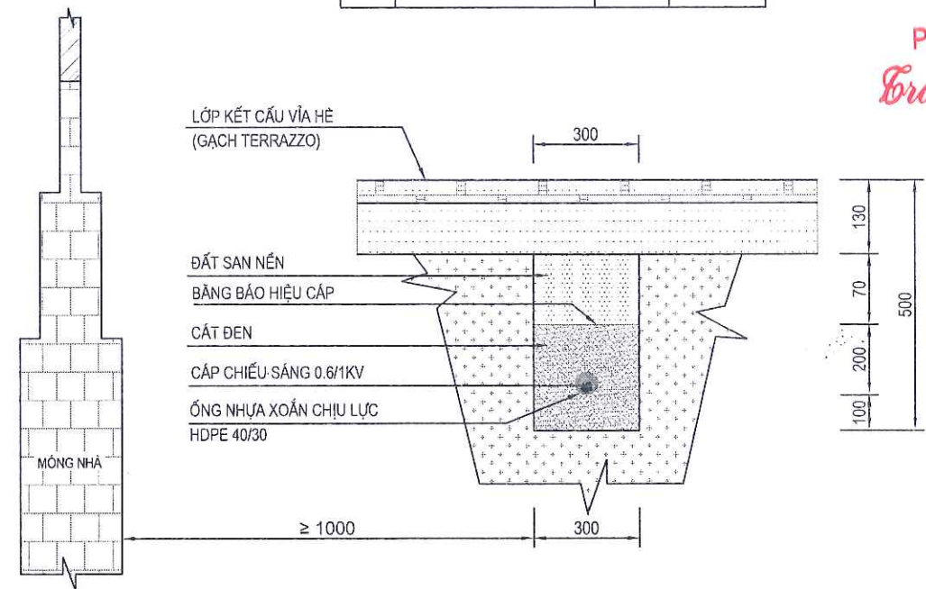
CÁP ĐI SONG SONG MÔNG NHÀ
