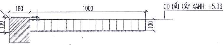
MẶT CẮT 2-2
