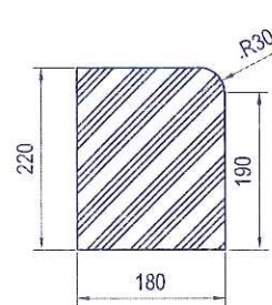
MẶT CẮT 1-1 (TỶ LỆ 1/10)
