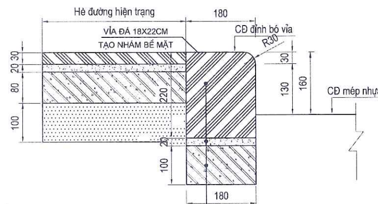
CHI TIẾT VỈA ĐÁ SỬA CHỮA SC6 (TỶ LỆ 1/10)
