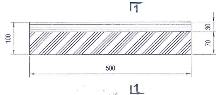
VỈA ĐÁ ĐƯỜNG DẠO LOẠI B1 KÍCH THƯỚC 10X10X50CM (TỶ LỆ 1/15)
