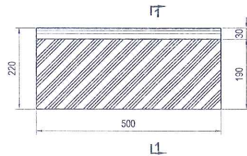
VỈA ĐÁ LOẠI A1 KÍCH THƯỚC 18X22X50CM (TỶ LỆ 1/10)
