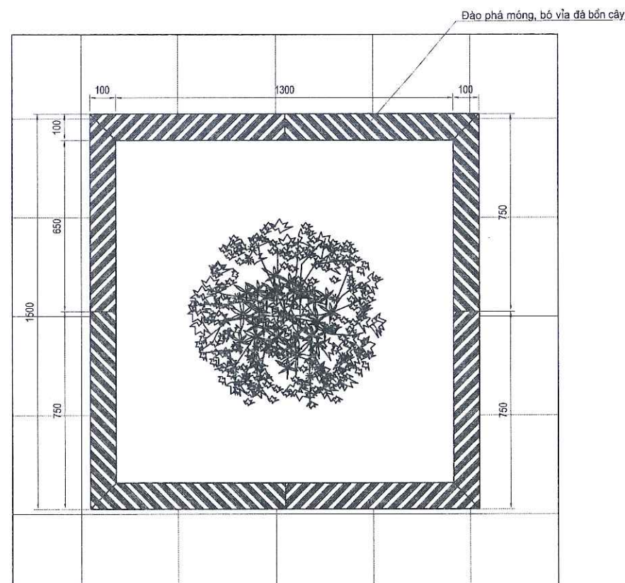
MẶT BẰNG HIỆN TRẠNG HỐ TRỒNG CÂY LOẠI 4 (TỶ LỆ 1/15)
