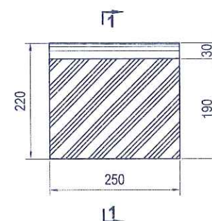
VỈA ĐÁ LOẠI A2 KÍCH THƯỚC 18X22X25CM (TỶ LỆ 1/10)
