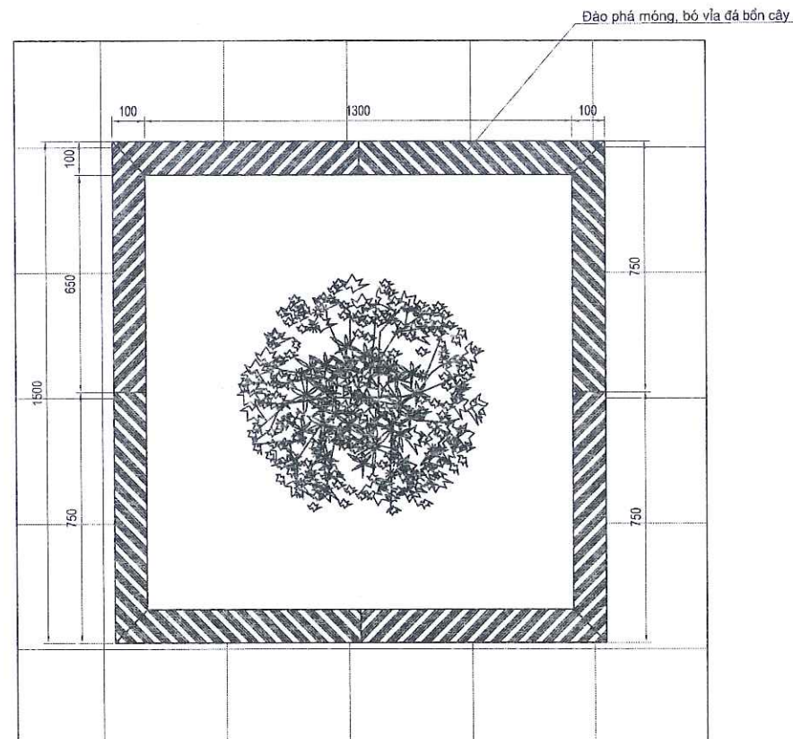
MẶT BẰNG HIỆN TRẠNG HỒ TRỒNG CÂY LOẠI 4 (TỶ LỆ 1/15)
