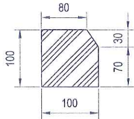
MẶT CẮT 1-1 (TỶ LỆ 1/15)
