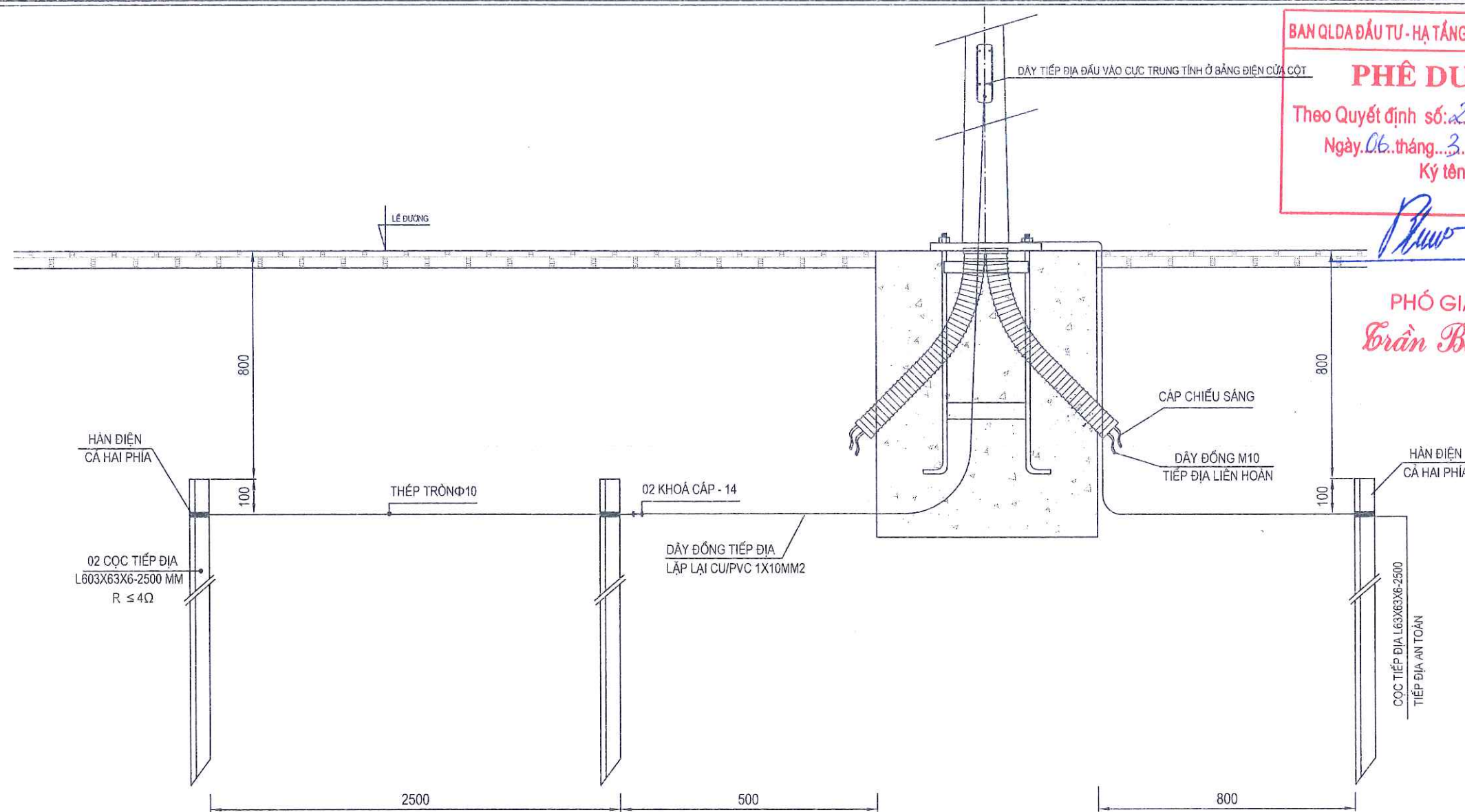
CHI TIẾT TIẾP ĐỊA LẬP LẠI RC-2
