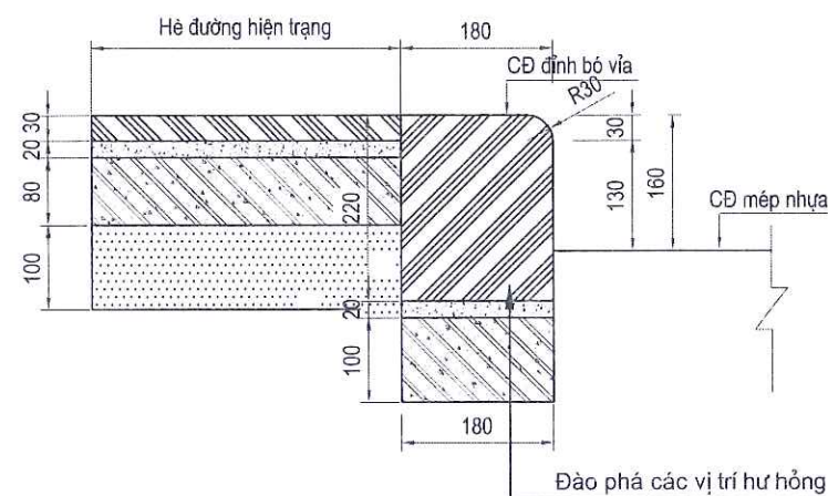
CHI TIẾT VỈA ĐÁ HIỆN TRẠNG SC6 (TỶ LỆ 1/10)
