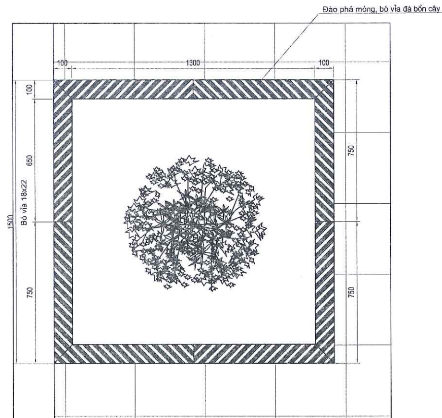
MẶT BẰNG HIỆN TRẠNG HỒ TRỒNG CÂY LOẠI 5 (TỶ LỆ 1/15)
