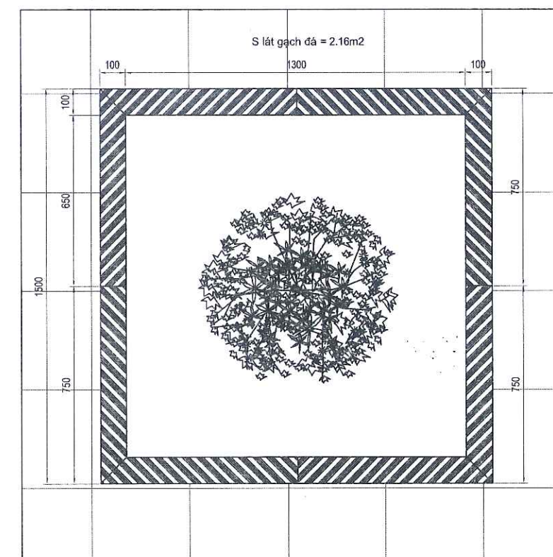
CHI TIẾT SỬA CHỮA SCB4
