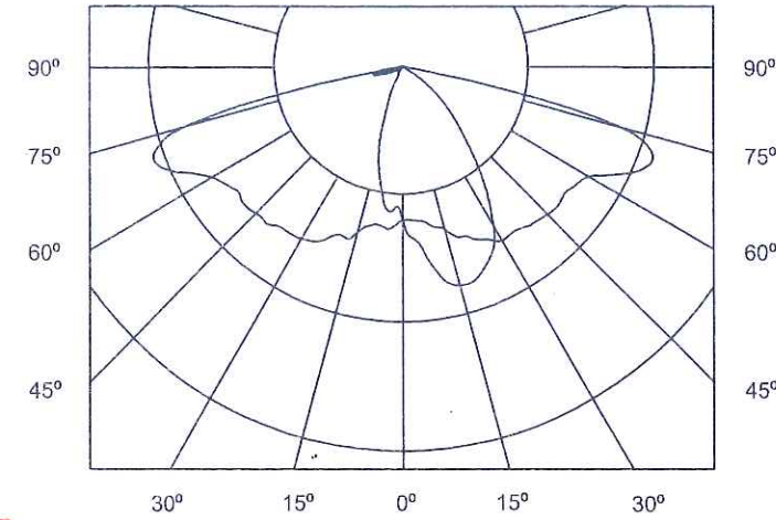
BIỂU ĐỒ TIẾT GIẢM CÔNG SUẤT CỦA BỘ ĐÈN (DIM)
