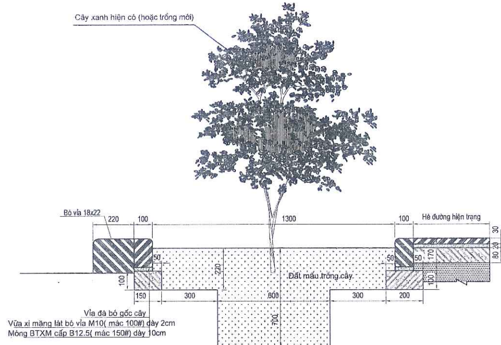
CẮT NGANG HIỆN TRẠNG HỒ TRỒNG CÂY LOẠI 5
