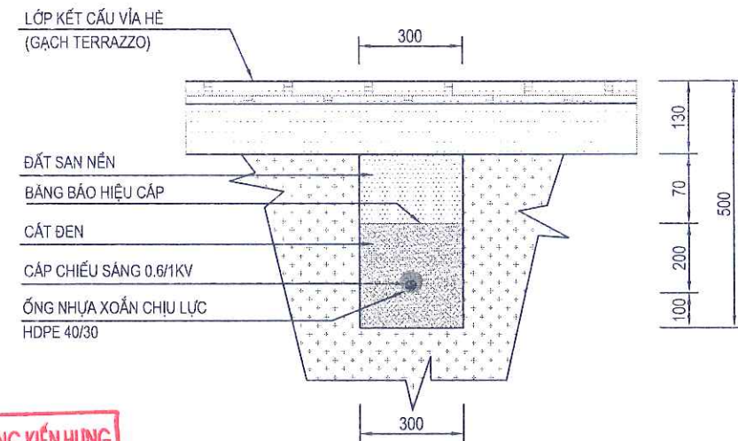
MẶT CẮT HÀO ĐI CÁP CHIẾU SÁNG TRÊN VỈA HÈ HIỆN CÓ HC-6.2
