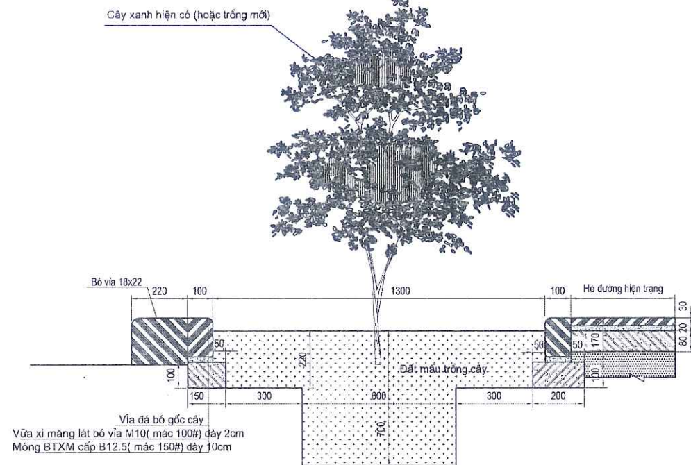
CẮT NGANG HIỆN TRẠNG HỒ TRỒNG CÂY LOẠI 5
