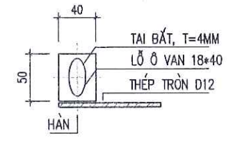
YÊU CẦU KỸ THUẬT CỘT ĐÈN TRANG TRÍ
