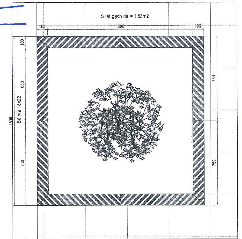
CHI TIẾT SỬA CHỮA SCB5
