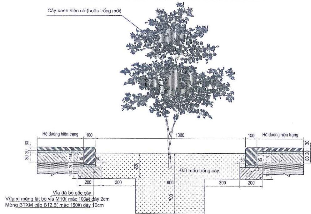
CẮT NGANG HIỆN TRẠNG HỒ TRỒNG CÂY LOẠI 4
