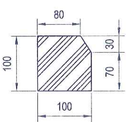
MẶT CẮT 1-1 (TỶ LỆ 1/15)
