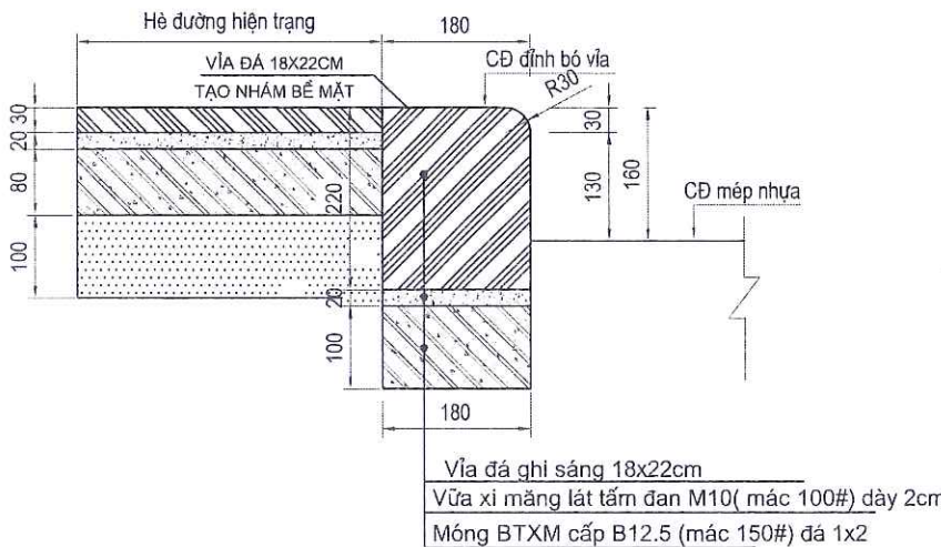
CHI TIẾT VỈA ĐÁ SỬA CHỮA SC6 (TỶ LỆ 1/10)
