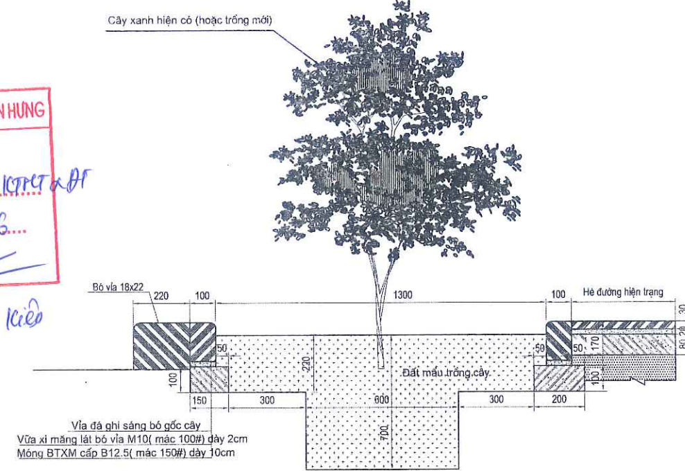
CẮT NGANG CẢI TẠO HỒ TRỒNG CÂY LOẠI 5
