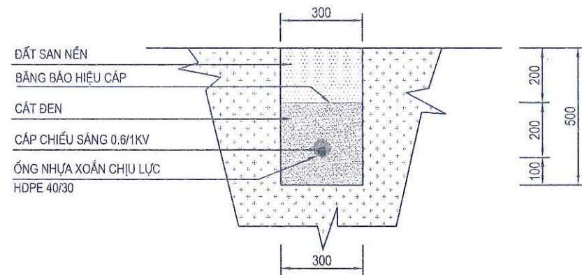
MẶT CẮT HÀO ĐI CÁP CHIẾU SÁNG TRÊN NỀN ĐẤT HC-6.1
