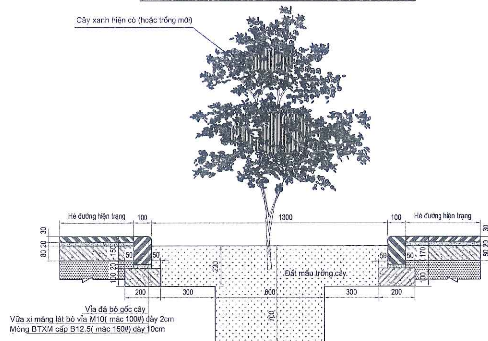
CẮT NGANG HIỆN TRẠNG HỔ TRỒNG CÂY LOẠI 4
