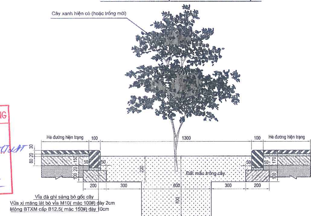
CẮT NGANG CẢI TẠO HỒ TRỒNG CÂY LOẠI 4
