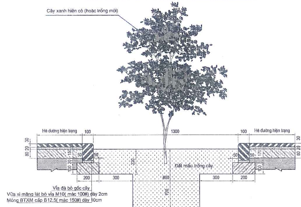
CẮT NGANG HIỆN TRẠNG HỒ TRỒNG CÂY LOẠI 4
