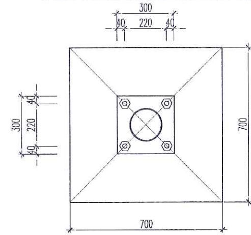
MẶT BẰNG(ĐIỂN HÌNH)
