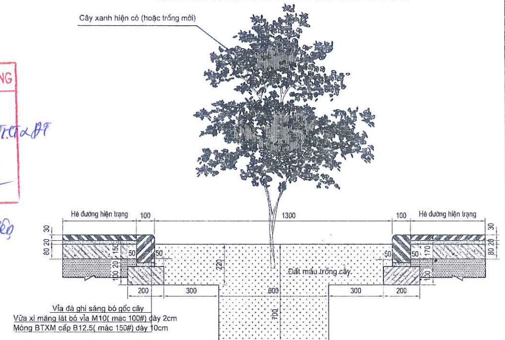
CẮT NGANG CẢI TẠO HỒ TRỒNG CÂY LOẠI 4
