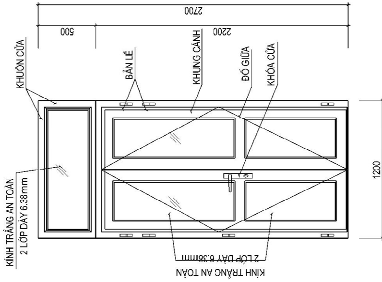
CHI TIẾT CỬA ĐI Đ1 (12BỘ)
