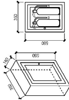
CHI TIẾT HỘP ĐUNG BÌNH CỨU HOẢ (01 BỘ)
