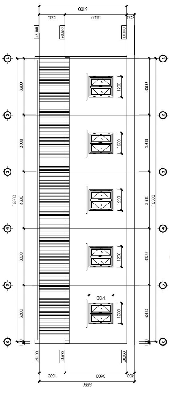
MẶT ĐỨNG TRỤC 6-1
