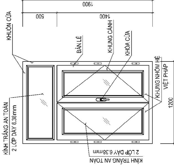
CHI TIẾT CỬA SỔ S1 (10BỘ)
