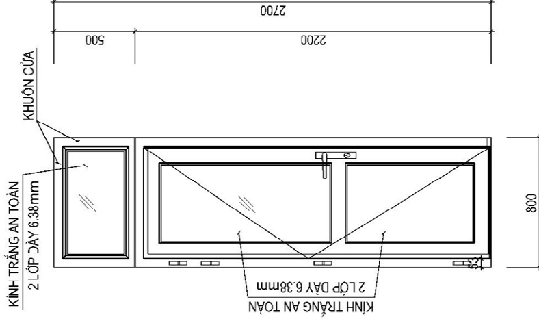
CHI TIẾT CỬA ĐI Đ2 (06BỘ)
