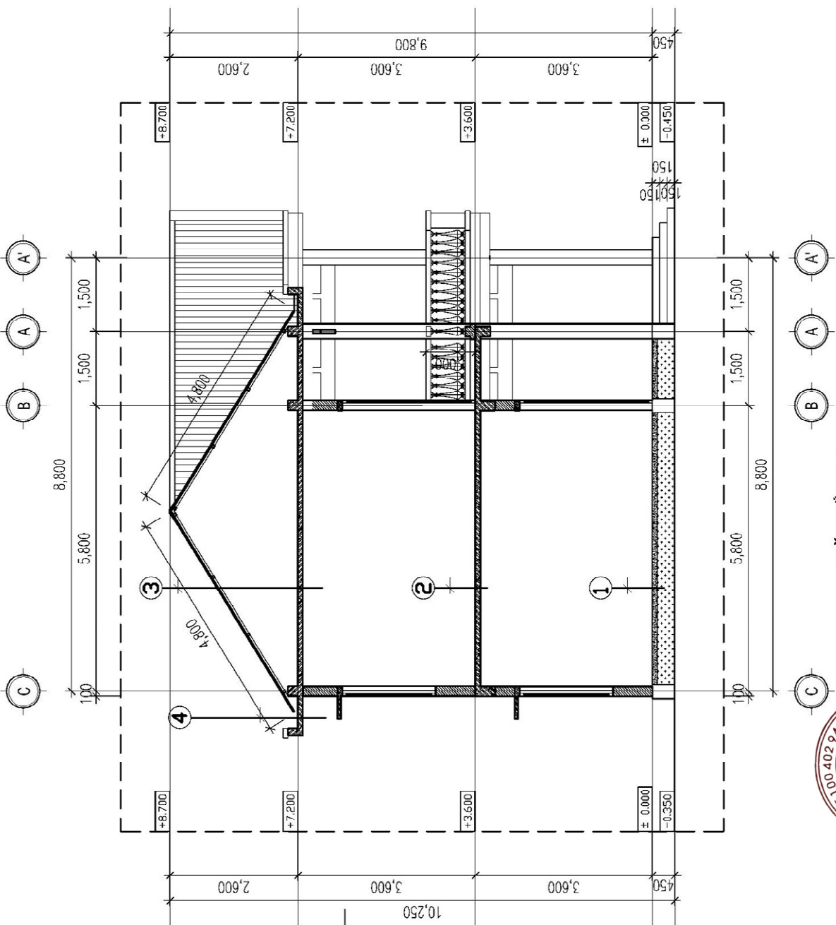
MẶT CẮT 1-1
