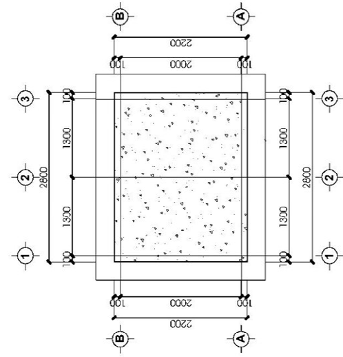
MẶT BẰNG BỂ
