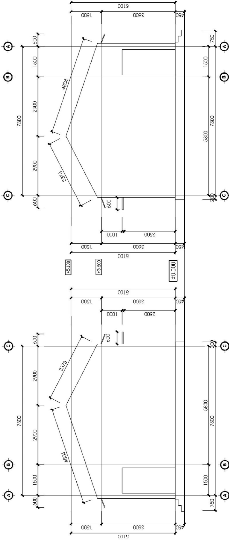
MẶT ĐỨNG TRỤC C-A HIỆN TRẠNG
