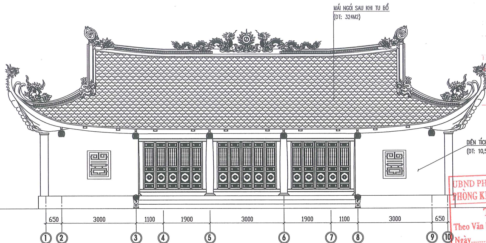
MẶT ĐÚNG TRỰC 1-10
