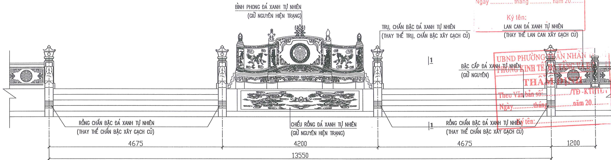
MẶT ĐỨNG BẠC CẤP SÂN CHIẾU RỒNG TU BỔ, TÔN TẠO
