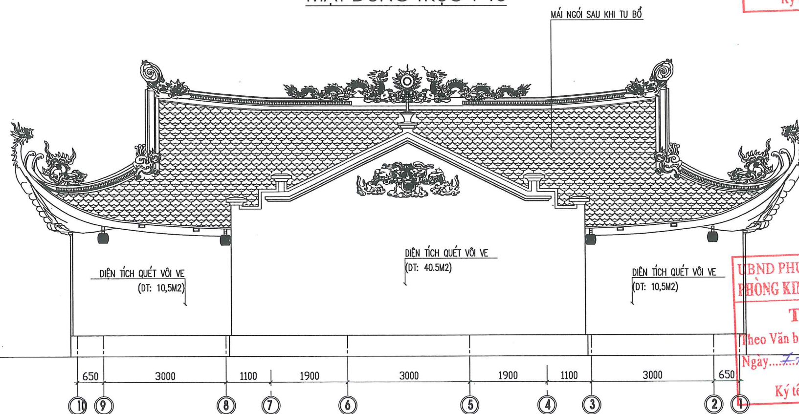
MẶT ĐÚNG TRỰC 10-1
