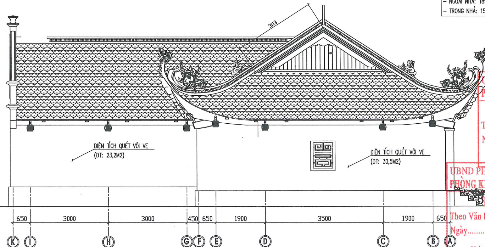
MẶT ĐÚNG TRỰC K-A
