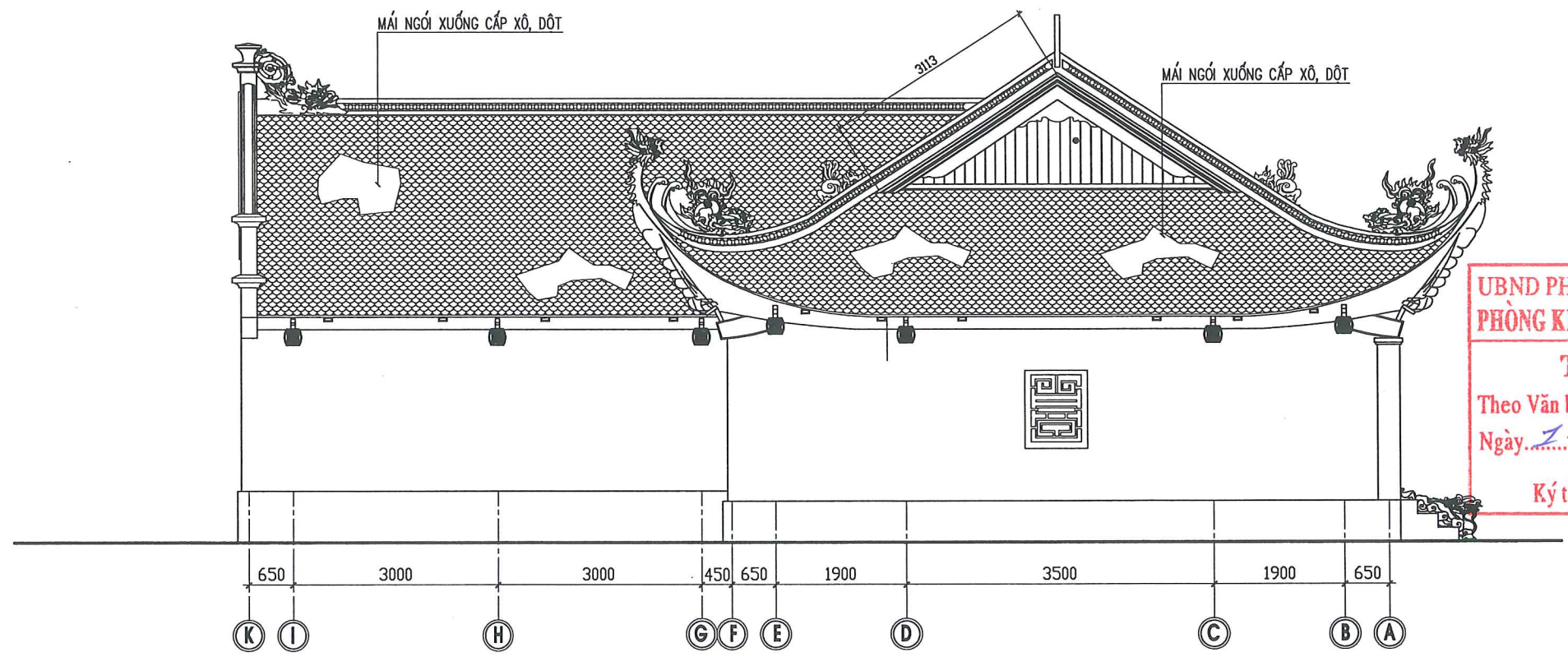
MẶT ĐỨNG TRỰC K-A
