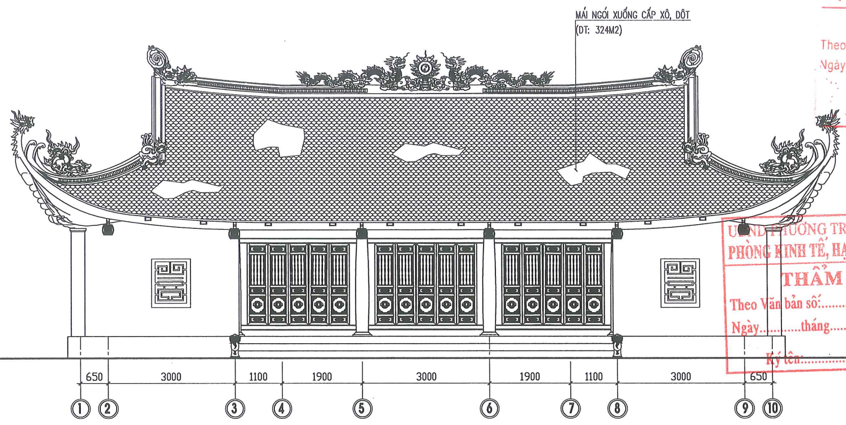
MẶT ĐÚNG TRỰC 1-10
