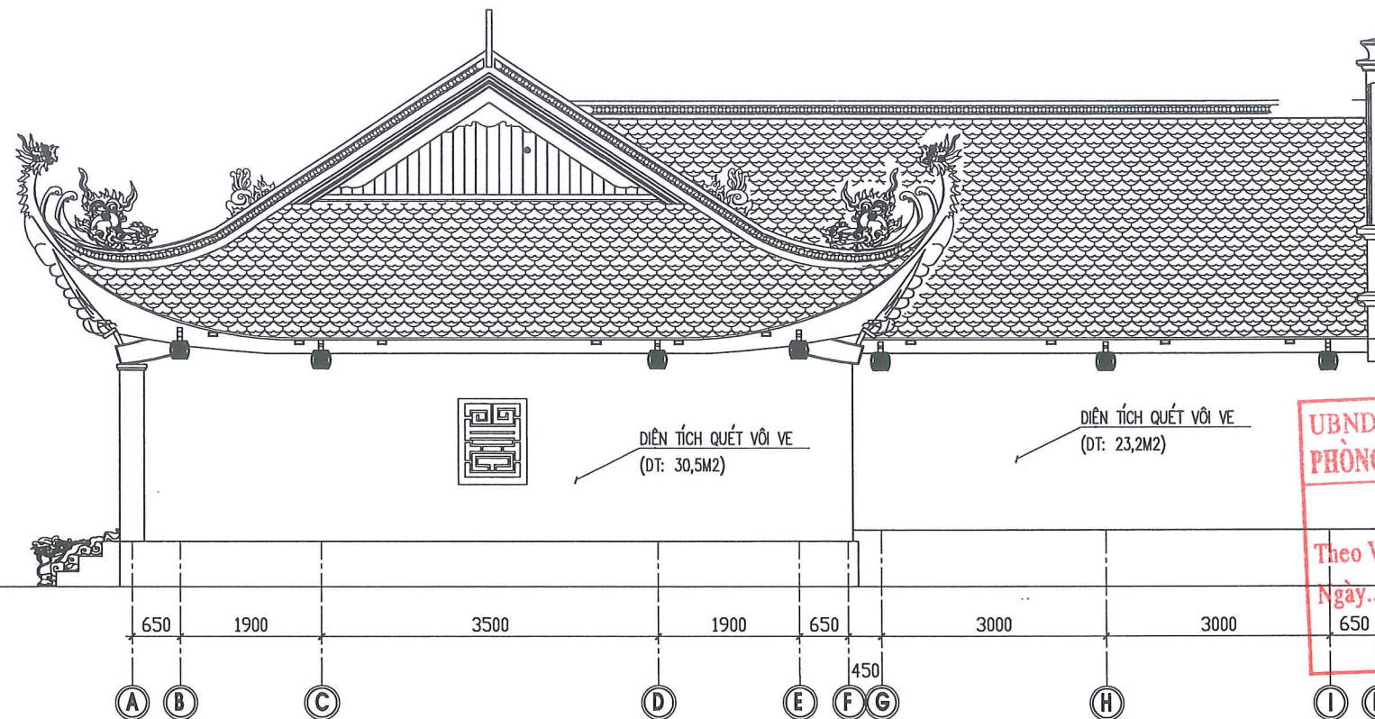
MẶT ĐÚNG TRỰC A-K
