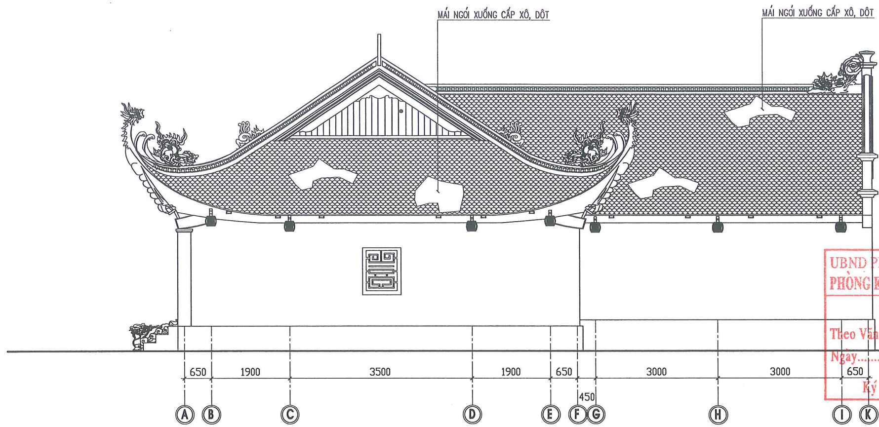
MẶT ĐỨNG TRỰC A-K
