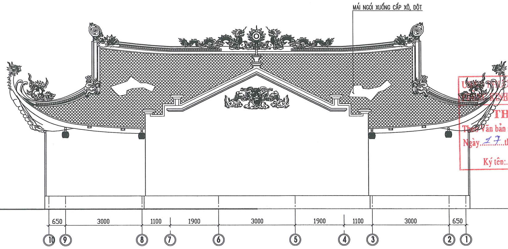
MẶT ĐÚNG CHÍNH DIỆN (TRỤC 1-10; 10-1)
