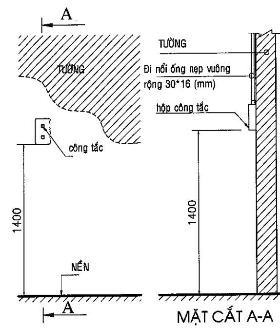
CT. LẮP ĐẶT CÔNG TẮC ĐÈN
