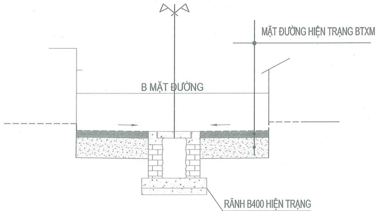
MẶT ĐƯỜNG CẢI TẠO ÁP DỤNG TỪ DDT4-CỌC D4
