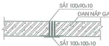
CHI TIẾT B
