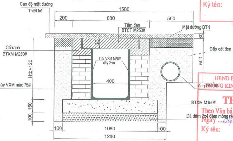
MẶT CẮT ĐÀO ĐẮP RÃNH
