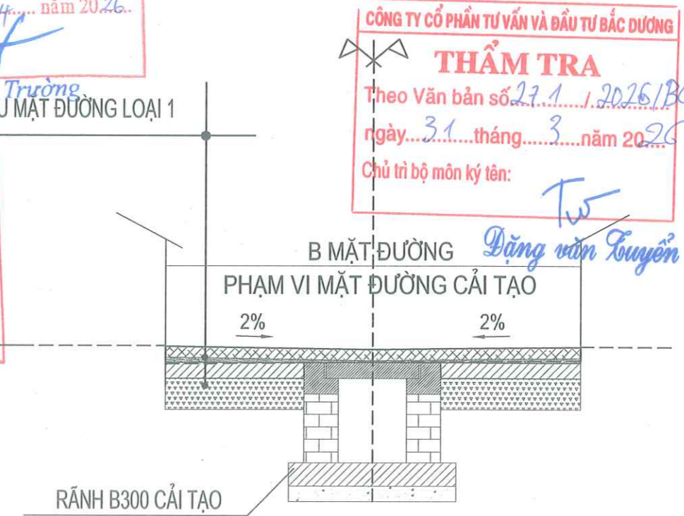
MẶT ĐƯỜNG CẢI TẠO
