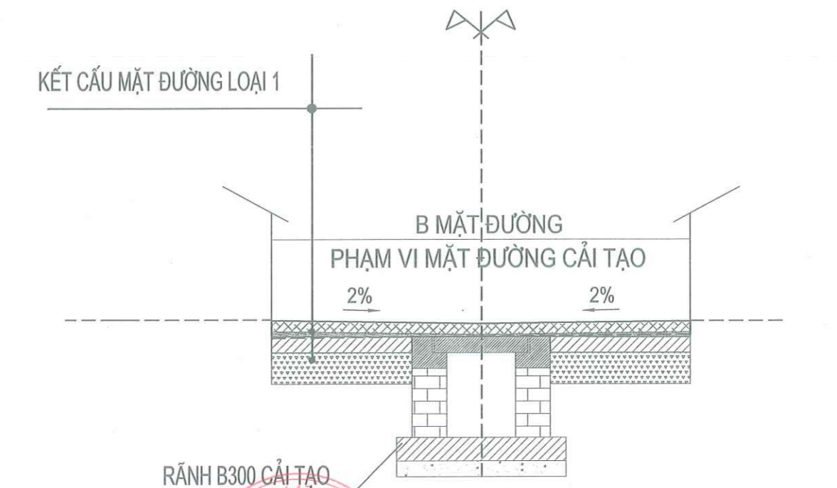
MẶT ĐƯỜNG CẢI TẠO ÁP DỤNG TỪ D4-CỌC CT4
