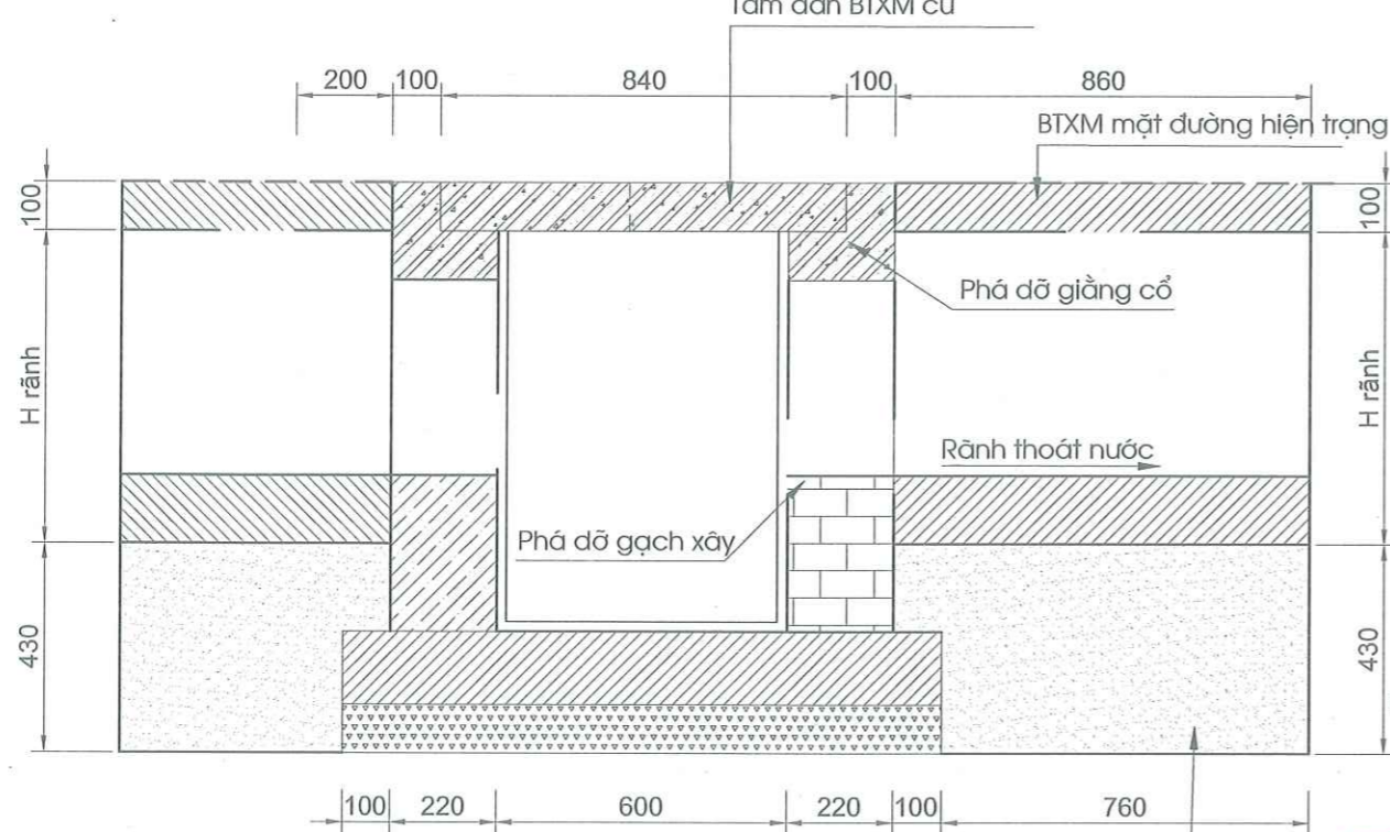
MẶT CẮT A-A ( HỐ GA HIỆN TRẠNG ) TL: 1/25
