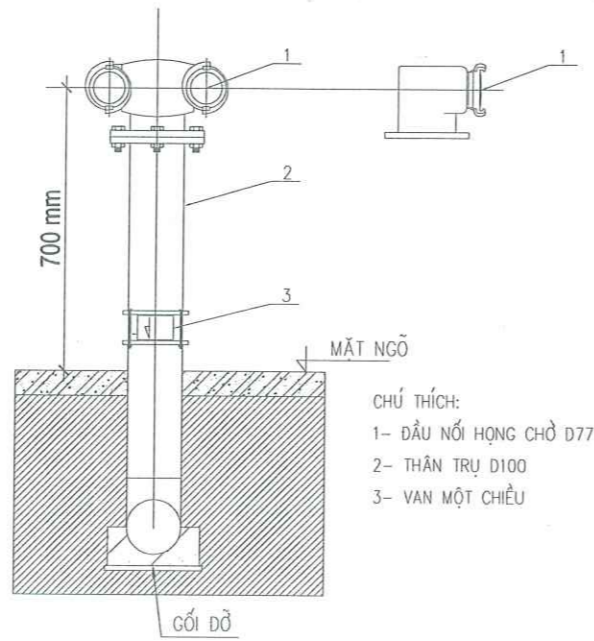
CHI TIẾT HỌNG LẤY NƯỚC O2
