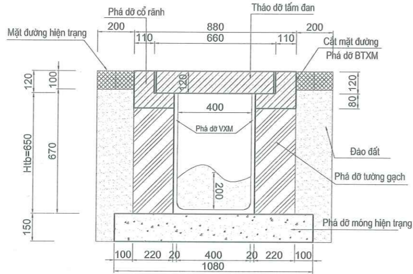
KHOẢNG LƯỢNG PHÁ DỠ 1M RÃNH THOÁT NƯỚC B400
