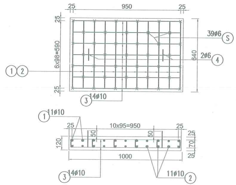
CHI TIẾT TẮM ĐAN RÃNH
