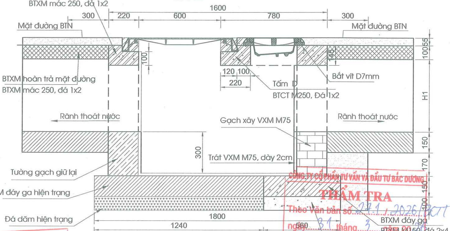
MẶT CẮT A-A TL: 1/25
