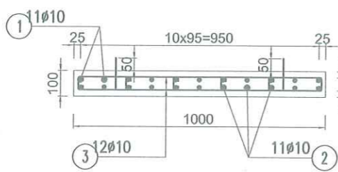
CHI TIẾT CỔ RÃNH
