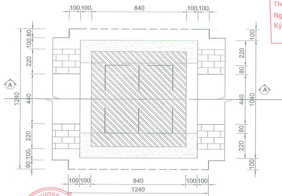
MẶT BẰNG HỐ GA HIỆN TRẠNG TL: 1/25
