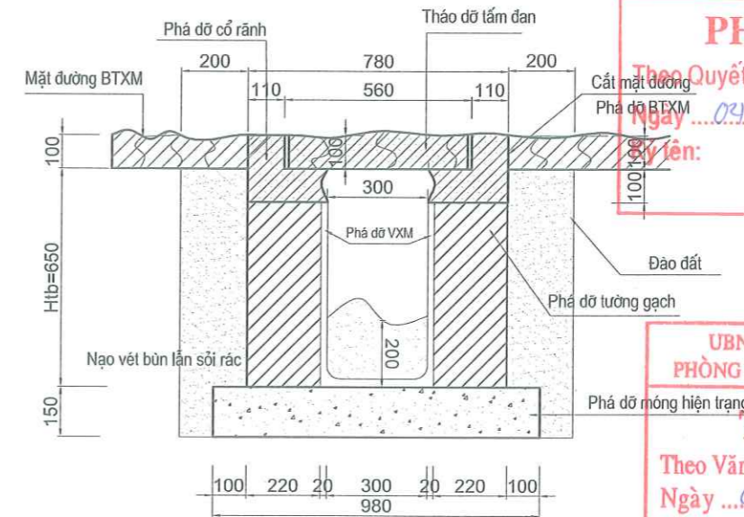
KHOẢNG LƯỢNG PHÁ DỠ 1M RÃNH THOÁT NƯỚC B300
