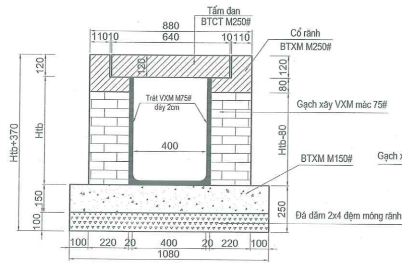
CHI TIẾT TẮM ĐAN RÃNH
