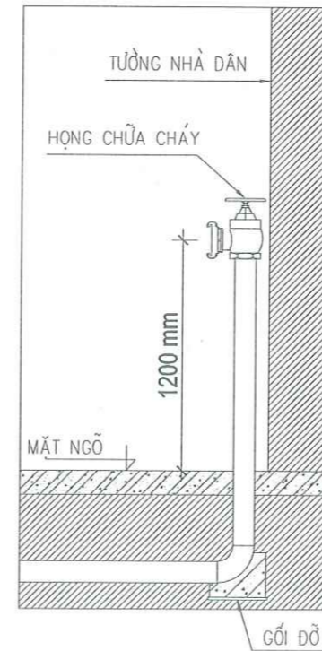
MẶT CẮT HỌNG CHỮA CHÁY
