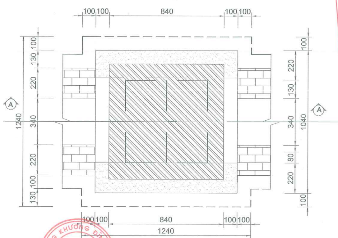
MẶT BẰNG HỐ GA HIỆN TRẠNG TL: 1/25
