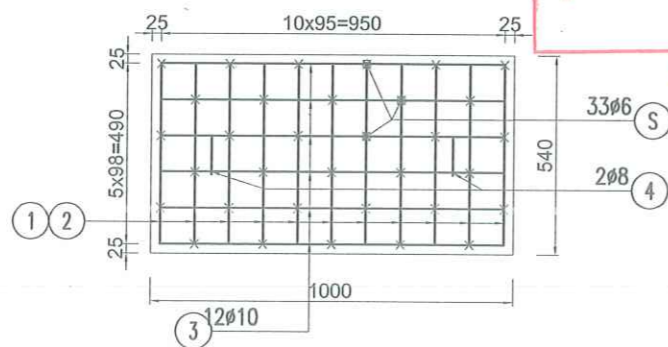
CHI TIẾT TẤM ĐƠN RÃNH
