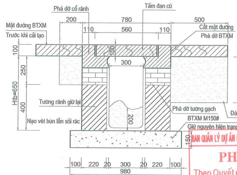
CHI TIẾT TẤM ĐƠN RÃNH
