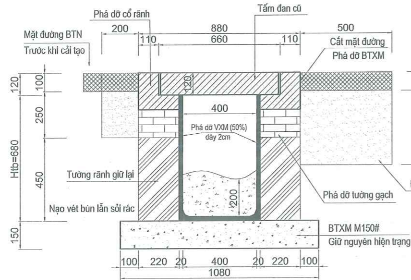
CHI TIẾT RÃNH THOÁT NƯỚC HIỆN TRẠNG
