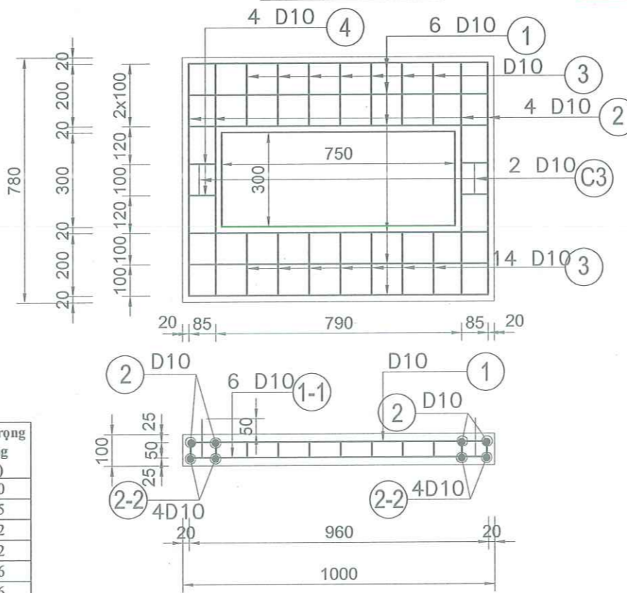
CHI TIẾT TẦM ĐƠN D
