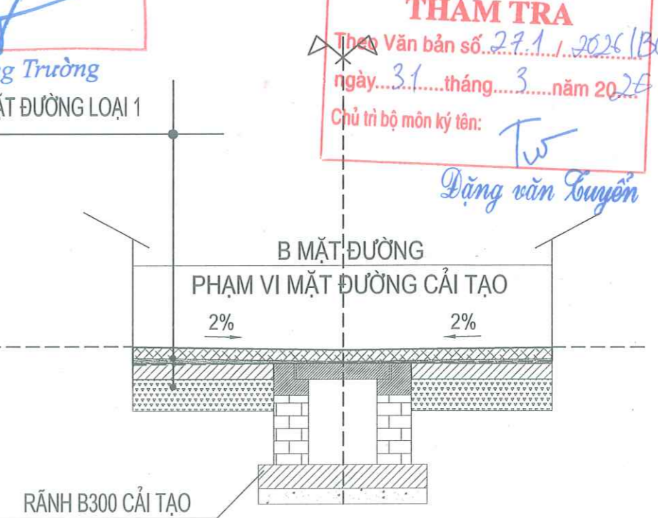
MẶT ĐƯỜNG CẢI TẠO
