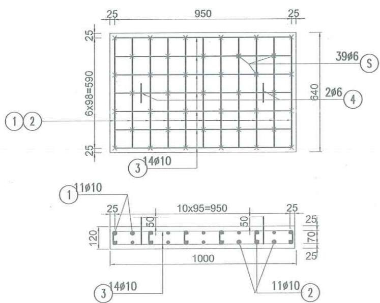
CHI TIẾT TẤM ĐAN RÃNH
