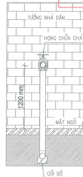
MẶT DỪNG HỌNG CHỮA CHÁY
