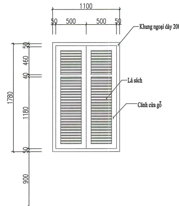
CHI TIẾT CỬA S2
