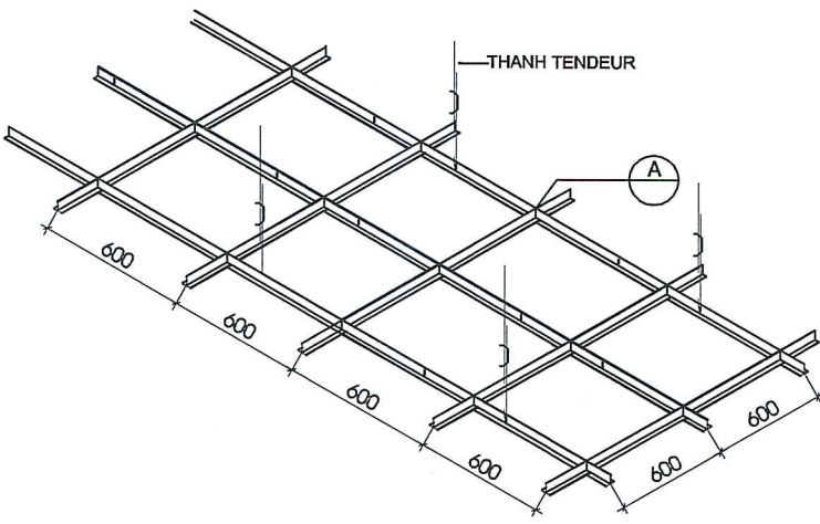
HƯỚNG DẪN LẮP ĐẶT HỆ KHUNG TRẦN NỔI ALPHA VĨNH TƯỜNG
