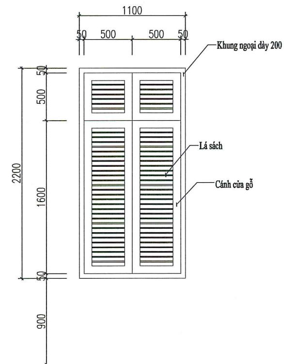
CHI TIẾT CỬA S1
