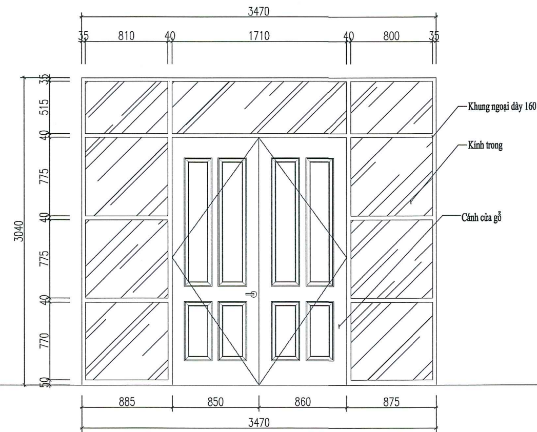
CHI TIẾT CỬA Đ1
