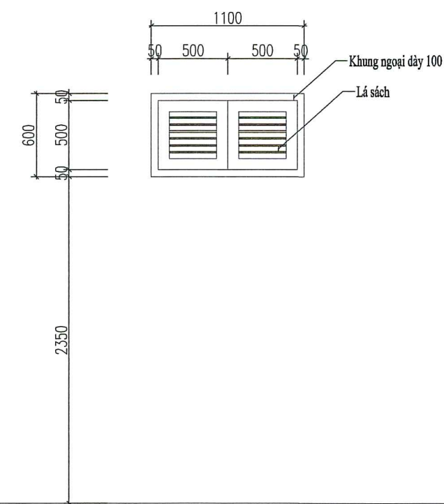
CHI TIẾT CỬA L1
