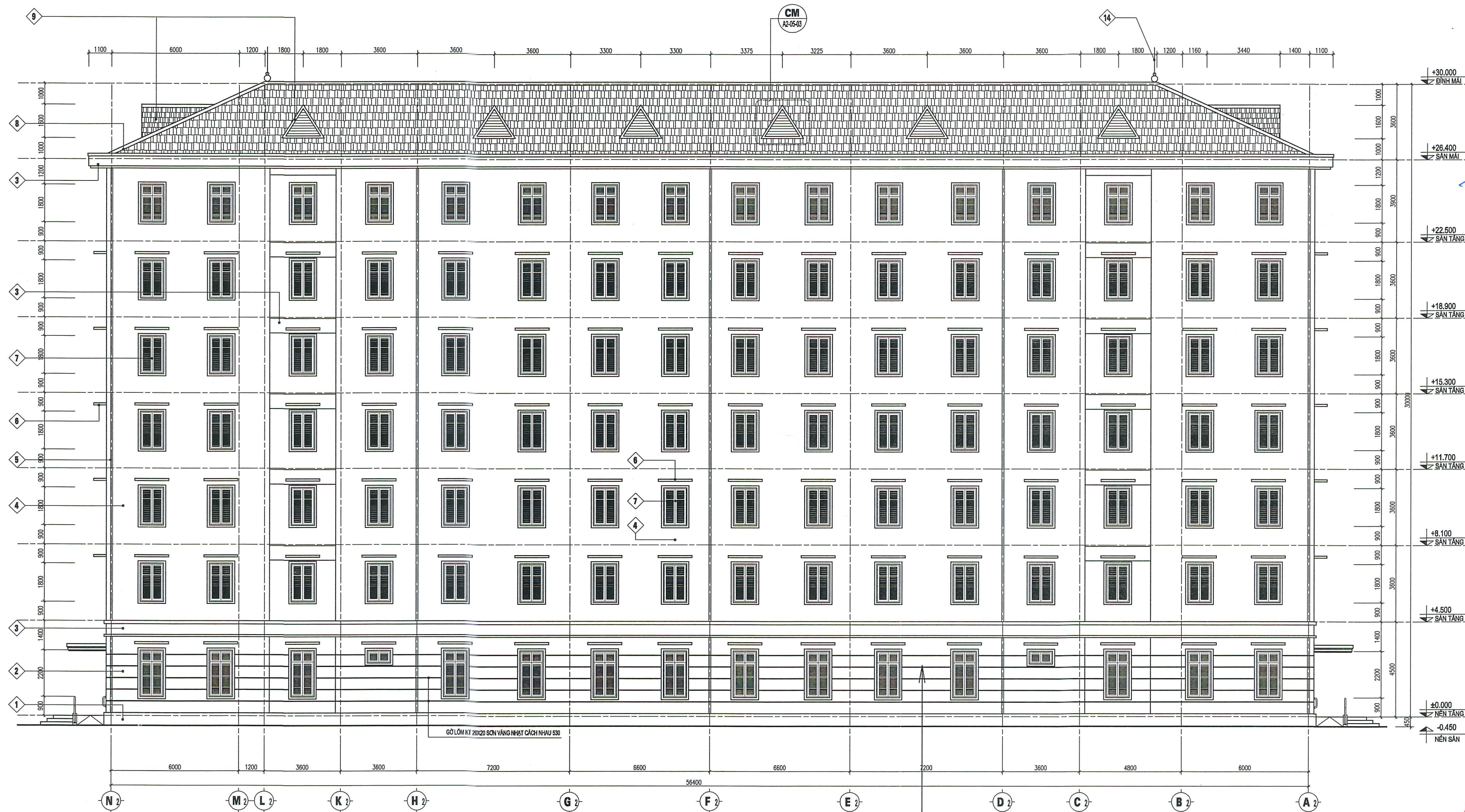
MẶT ĐỨNG HT TRỤC N-A TỶ LỆ 1:100
