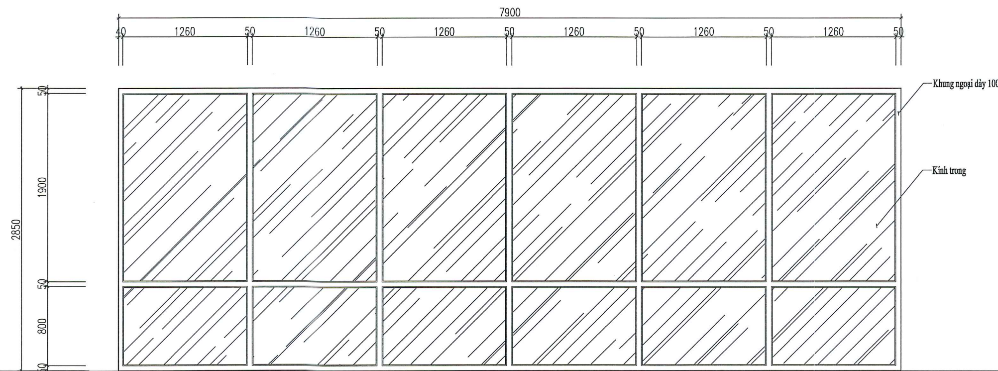
CHI TIẾT CỬA VK1
