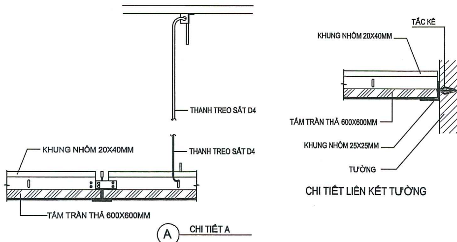
HƯỚNG DẪN LẮP ĐẶT HỆ KHUNG TRẦN NỔI ALPHA VĨNH TƯỜNG
