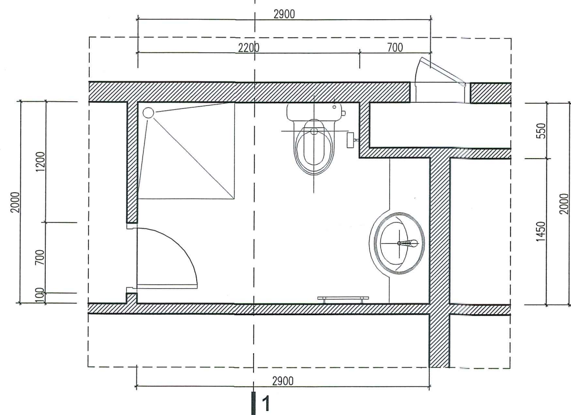
MẶT BẰNG CHI TIẾT VỆ SINH (ĐIỂN HÌNH 2; SL: 1 CÁI)
