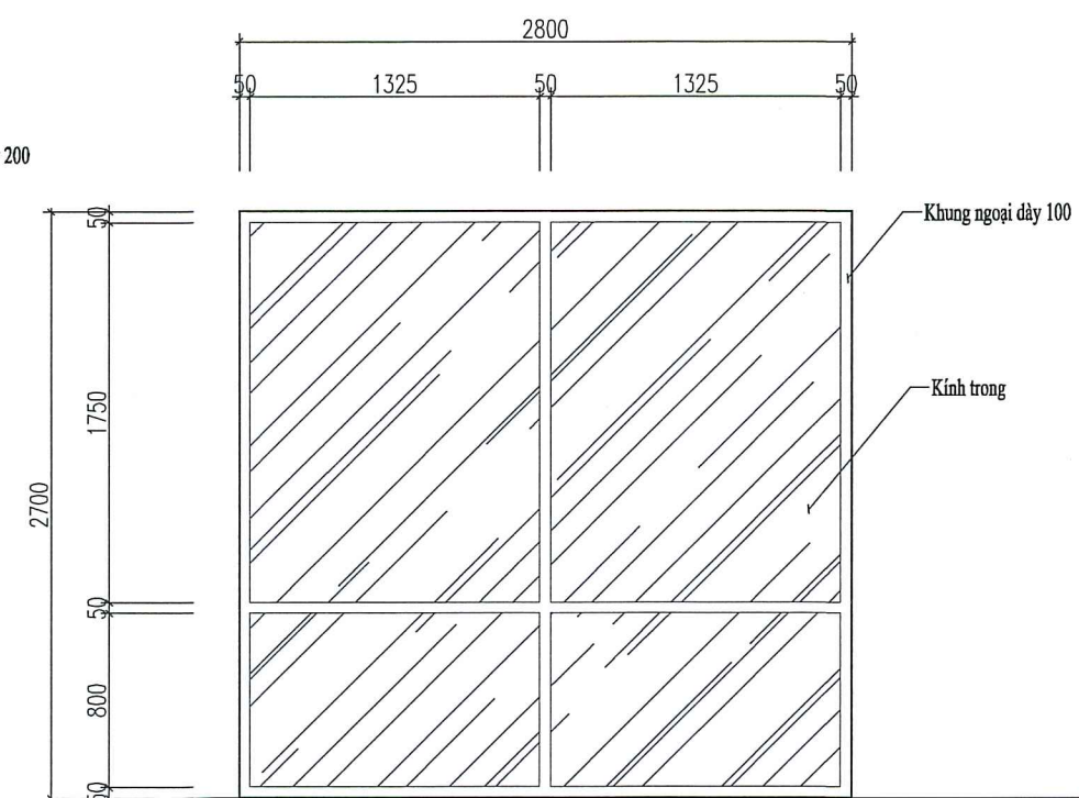
CHI TIẾT CỬA VK2
