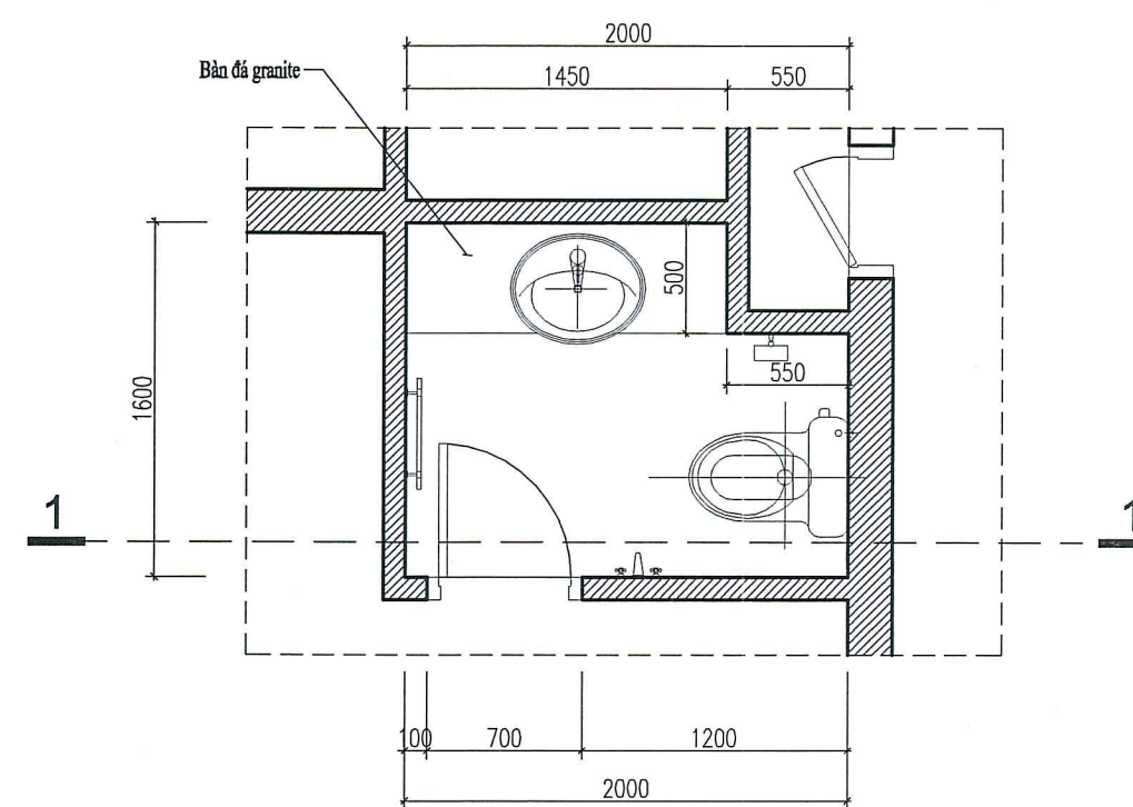
MẶT BẰNG CHI TIẾT VỆ SINH (ĐIỂN HÌNH 1; SL 17 CÁI)
