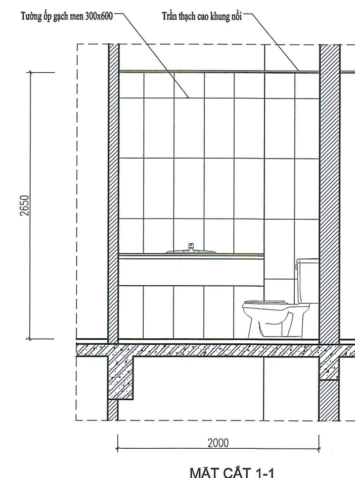
MẶT CẮT 1-1
