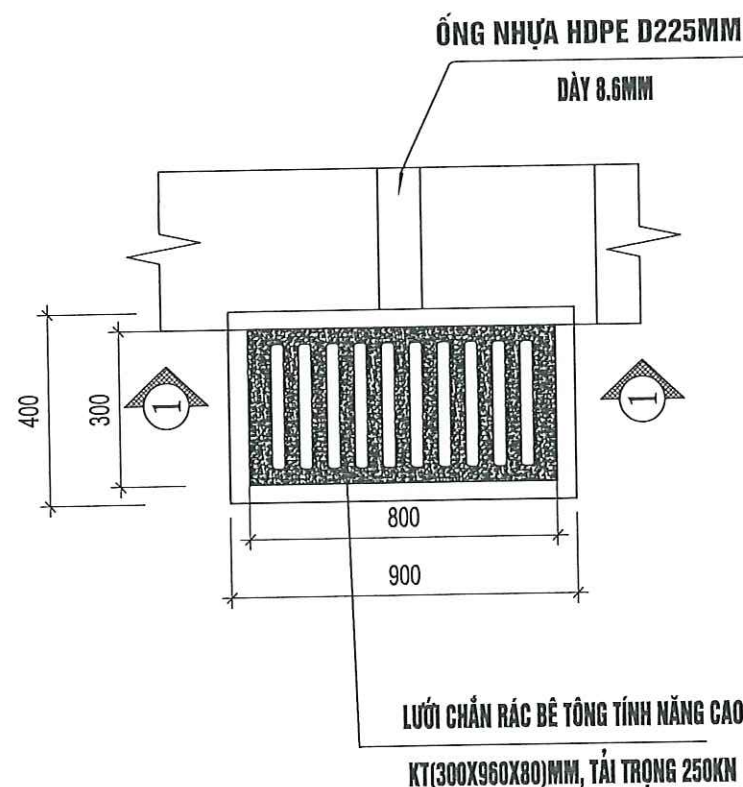
MẶT BẰNG HỒ THU
