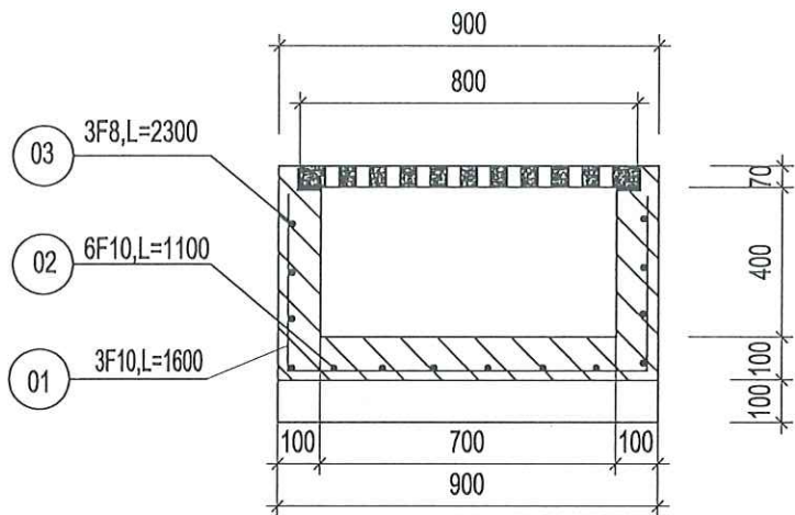
MẶT CẮT 1 - 1
