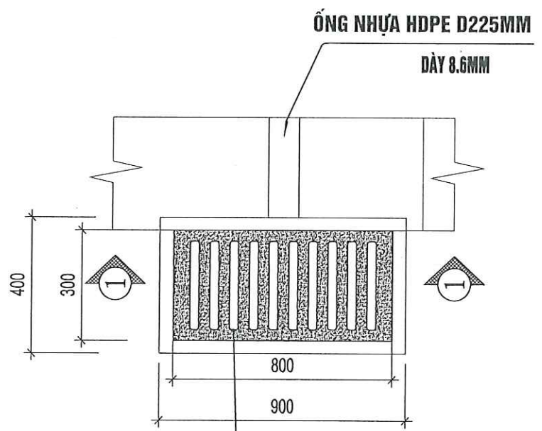
MẶT BẰNG HỒ THU
