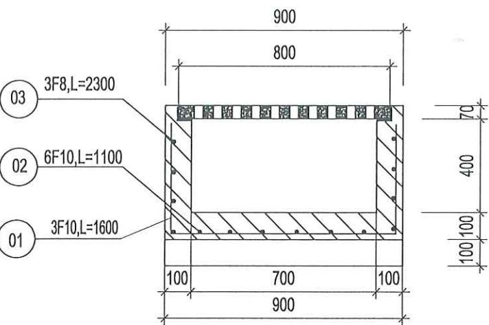
MẶT CẮT 1 - 1
