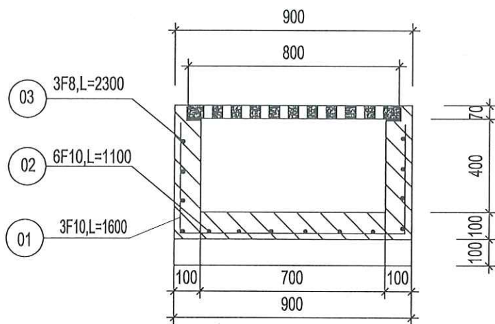
MẶT CẮT 1 - 1
