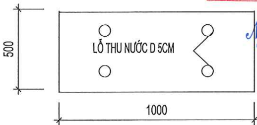
MẶT BẰNG ĐẠN MƯƠNG
