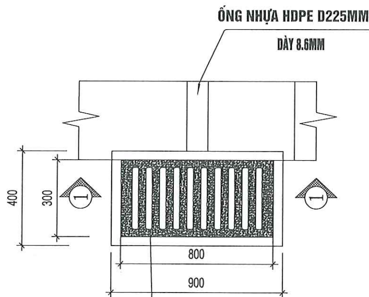
MẶT BẰNG HỒ THU
