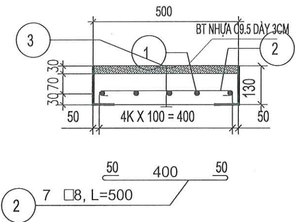
CẮT NGANG
