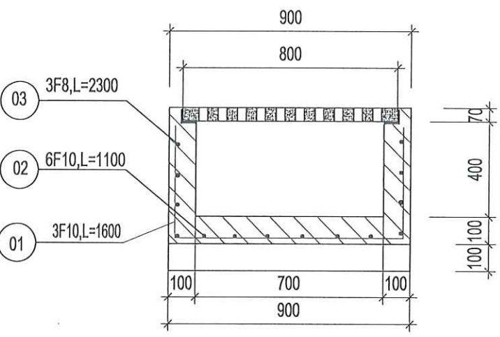
MẶT CẮT 1 - 1
