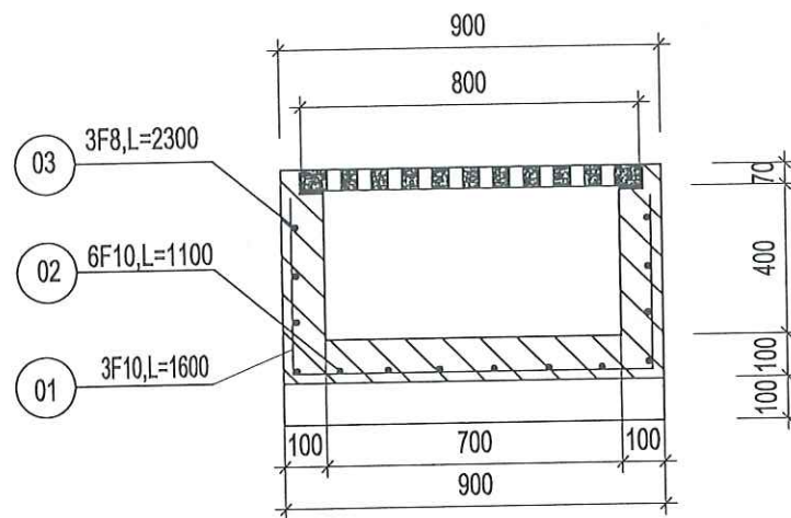
MẶT CẮT 1 - 1
