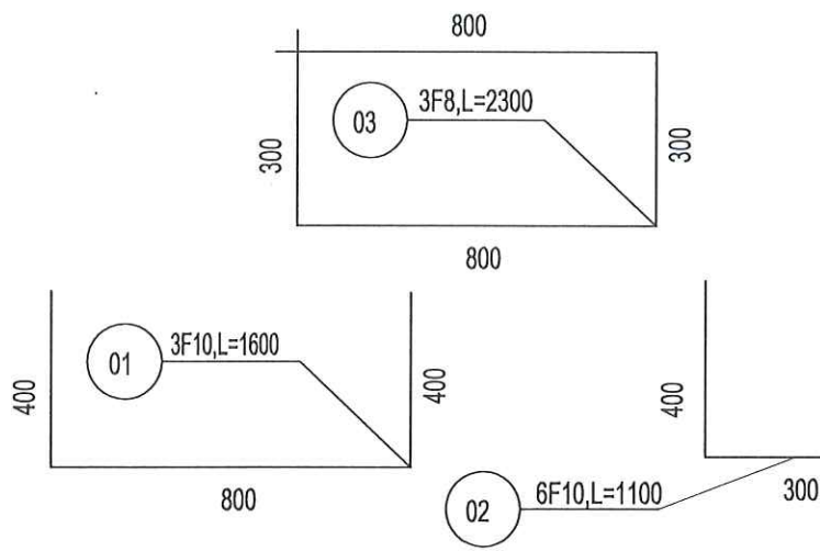
CỐT THÉP HỒ THU NƯỚC
