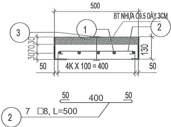
CẮT NGANG
