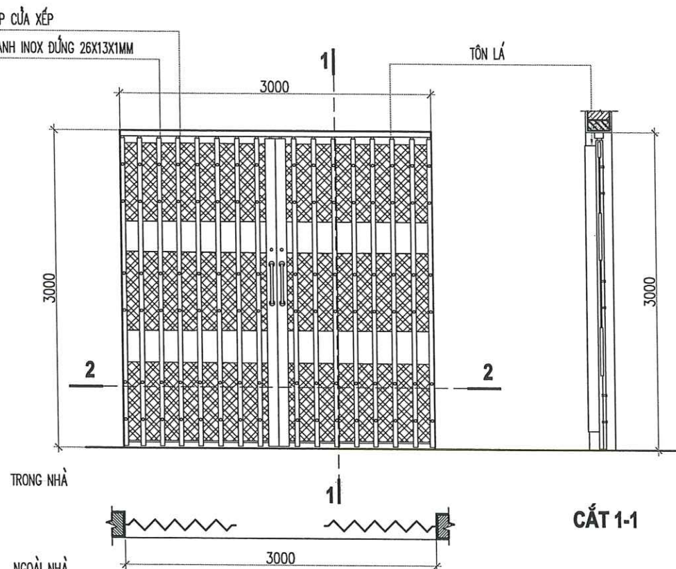
CHI TIẾT CỬA Đ2 (TỶ LỆ : 1/50)
