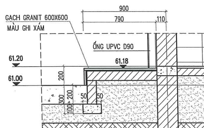
CHI TIẾT BO NỀN
