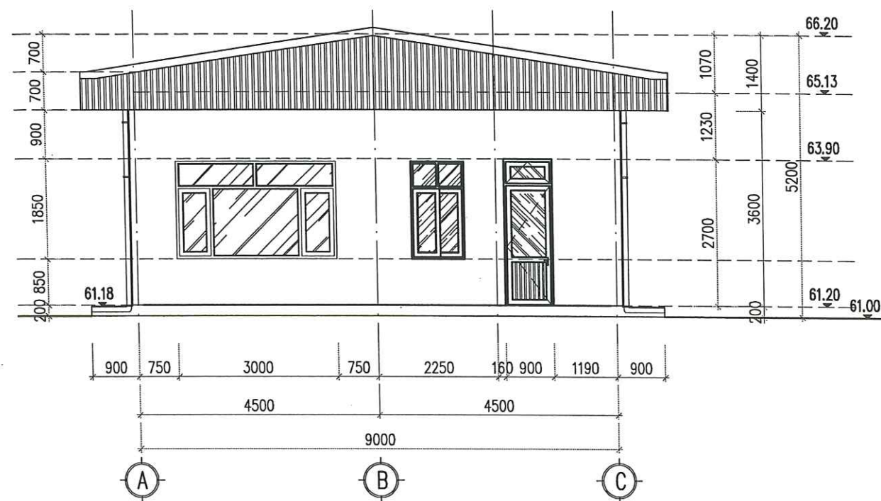
MẶT ĐỨNG TRỰC A-C
