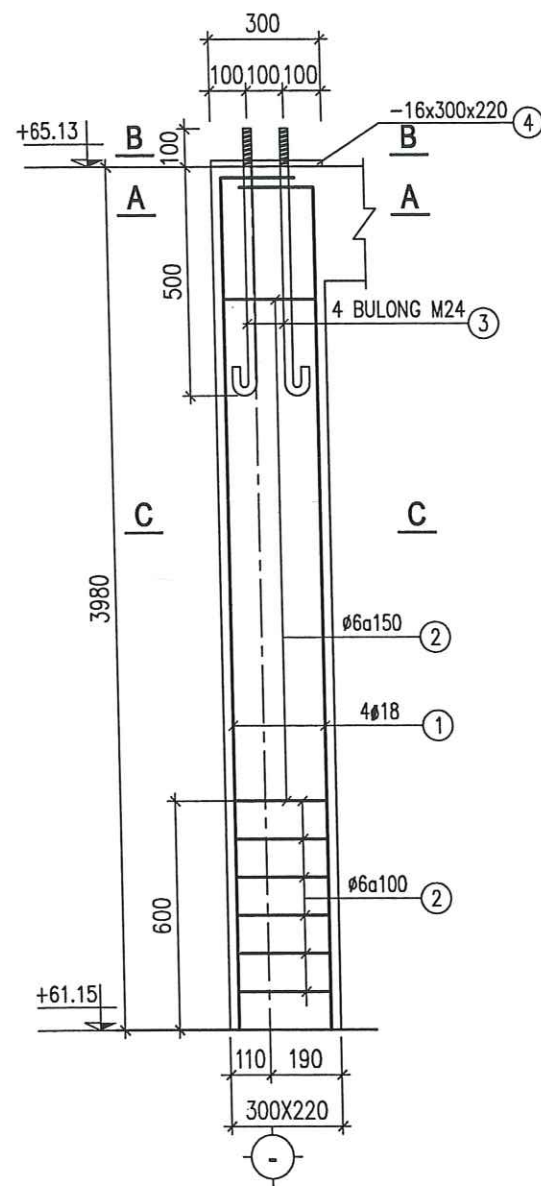
CỘT C1 (SL:06) TỶ LỆ: 1/25
