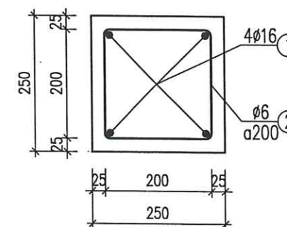
MẶT CẮT A-A TỶ LỆ: 1/10
