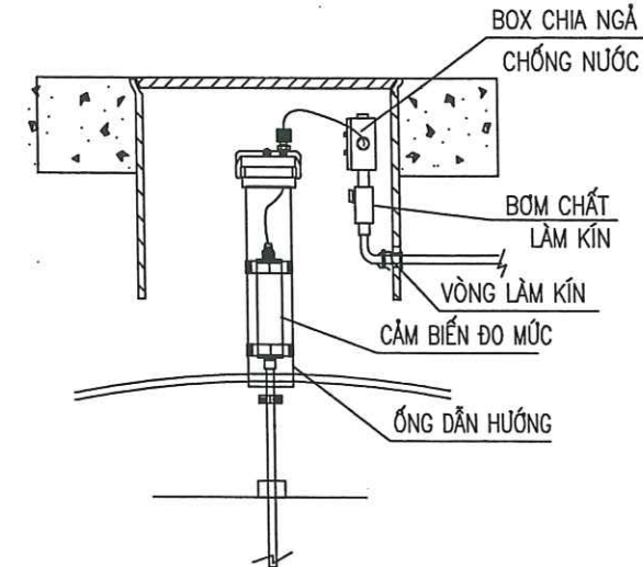
CTLĐ CẢM BIẾN ĐO BỒN TỰ ĐỘNG
