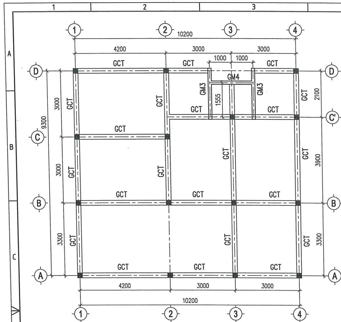
MẶT BẰNG GIẺNG CHỐNG THẨM TỶ LỆ: 1/100
