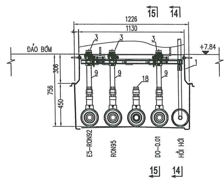
MẶT CẮT 13-13 TỶ LỆ 1:25
