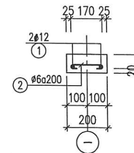
LANH TÔ LT-02 (L=6000, SL:01)
