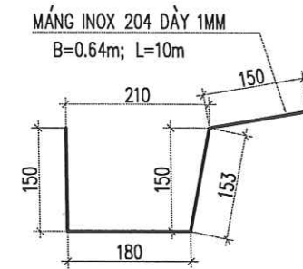
CHI TIẾT MĂNG NƯỚC (SL: 02 CÁI)
