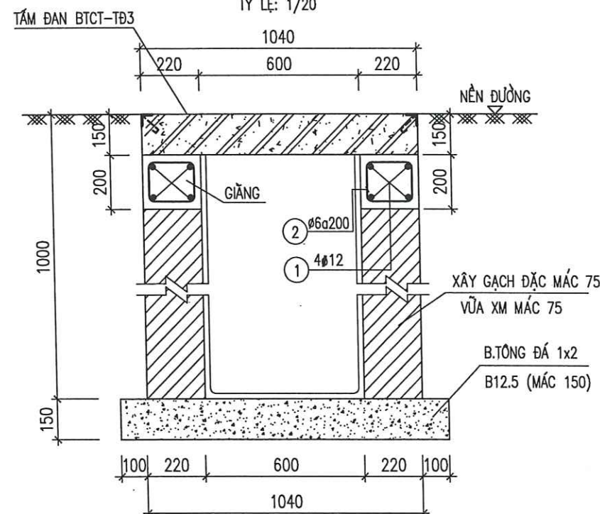
MẶT CẮT 1-1 TỶ LỆ 1/20
