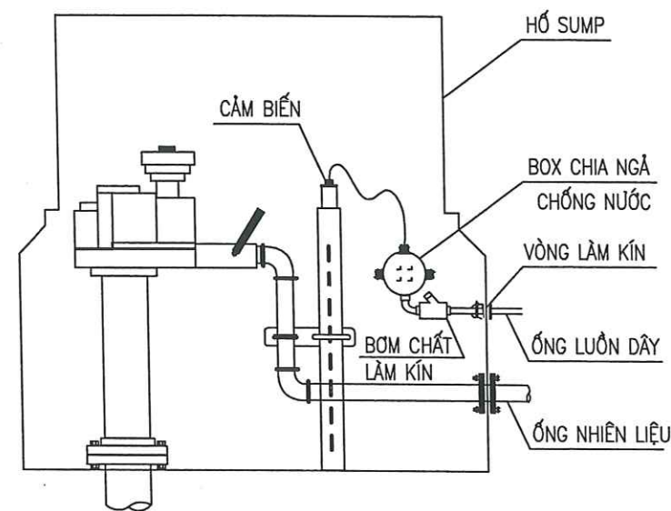
CTLĐ CẢM BIẾN HỒ SUMP CỎ BỂ
