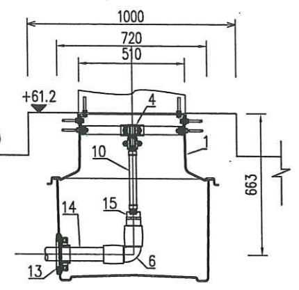
MẶT CẮT 15-15 TẠI ĐIỂM CUỐI
