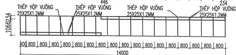
KHUNG ALUMEX XANH, TRẮNG (TỶ LỆ : 1/100)
