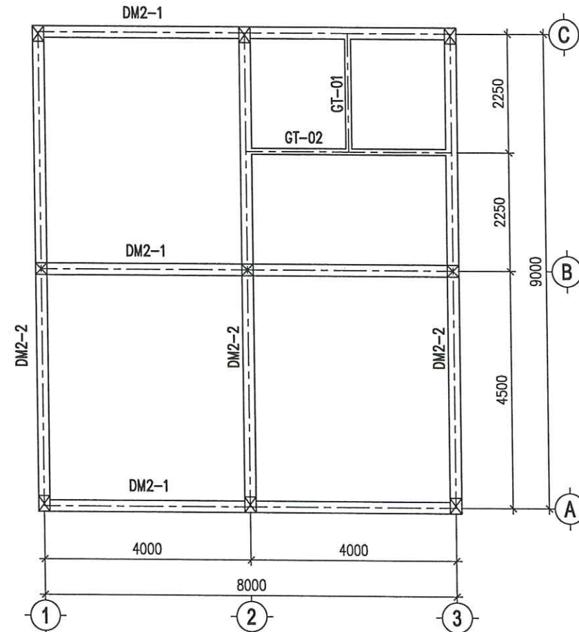
MẶT BẰNG KẾT CẤU COS +65.03 TỶ LỆ: 1/100
