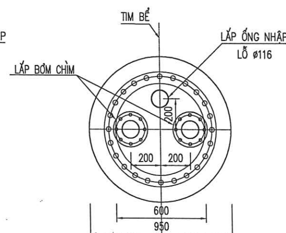
KHOÉT LỖ NẮP ĐẦM BỂ DO-0.001S
