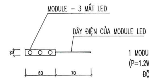
CHI TIẾT 1 MODULE LED TỶ LỆ : 1/2
