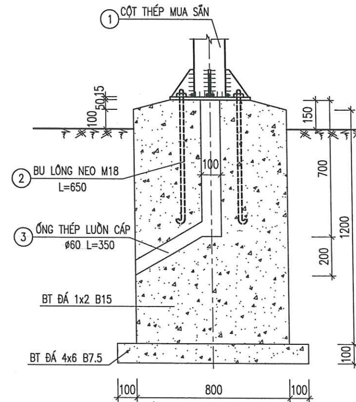
MẶT CẮT 1-1
