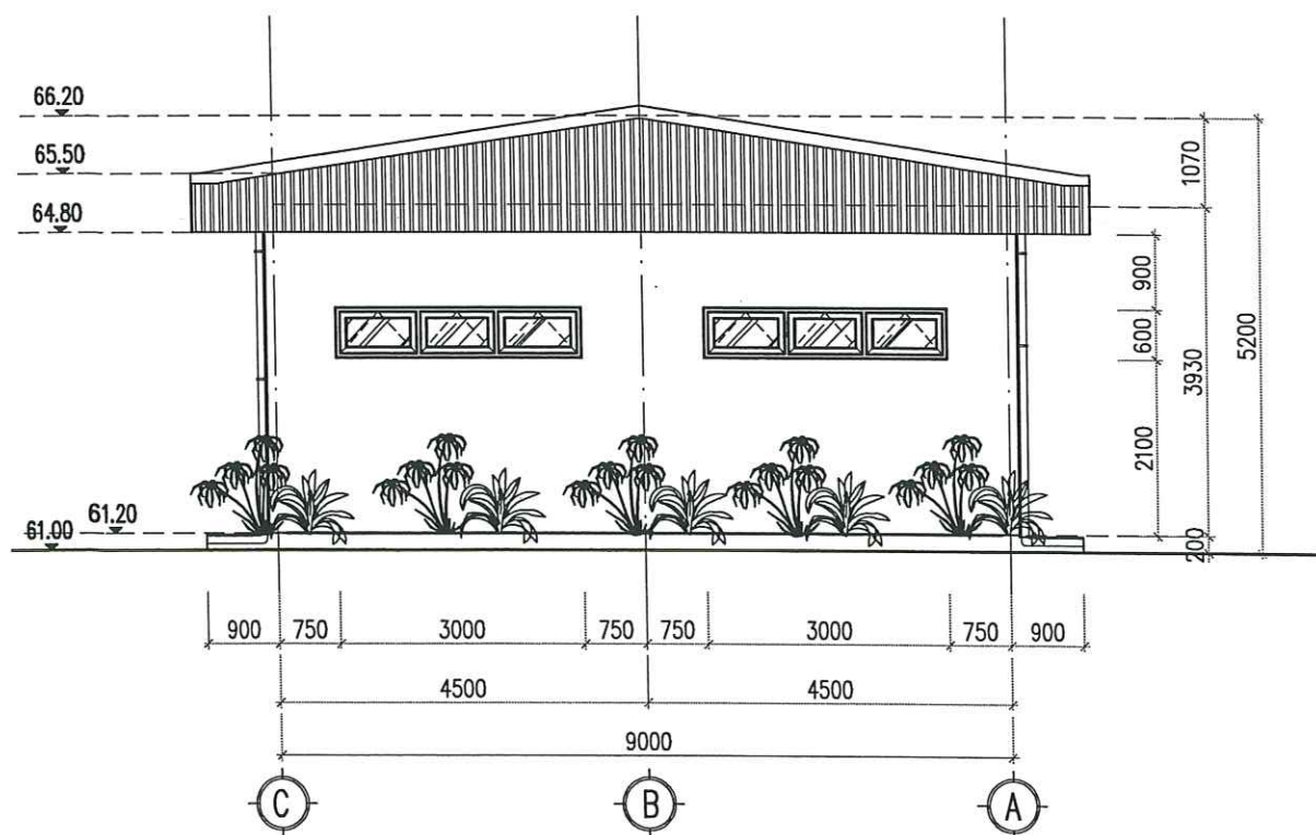
MẶT ĐỨNG TRỰC C-A
