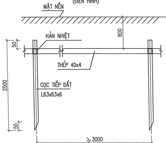
CHI TIẾT CỌC TIẾP ĐẤT - LIÊN KẾT (ĐIỂN HÌNH)
