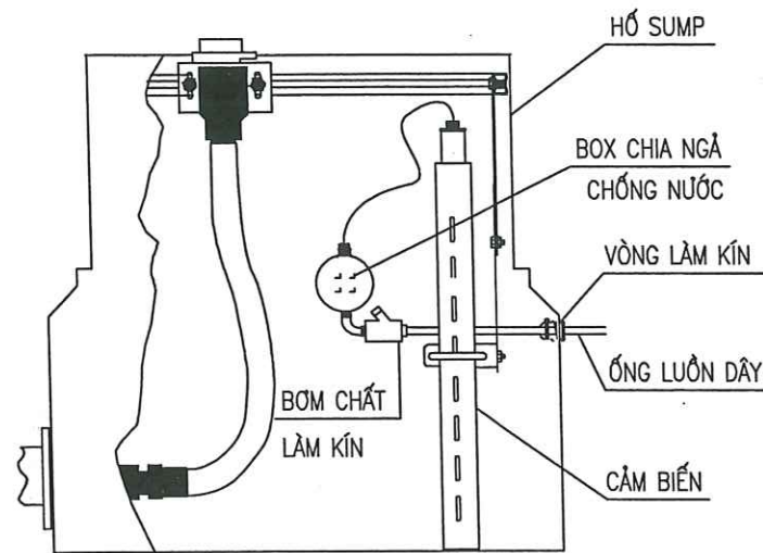
CTLĐ CẢM BIẾN CHÂN CỘT BƠM
