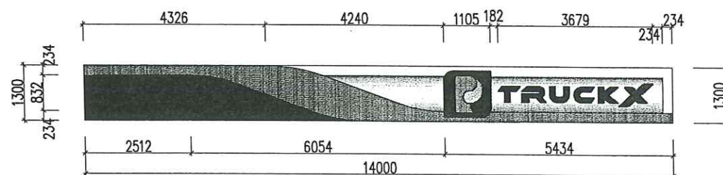
CHI TIẾT DIỂM MÁI TRỤC 1-2 (DM1) TỶ LỆ : 1/100
