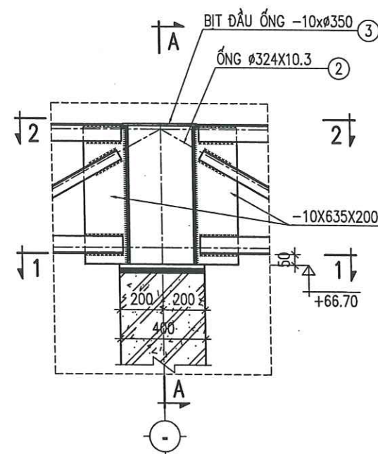
MẶT CẮT A-A TỶ LỆ: 1/25
