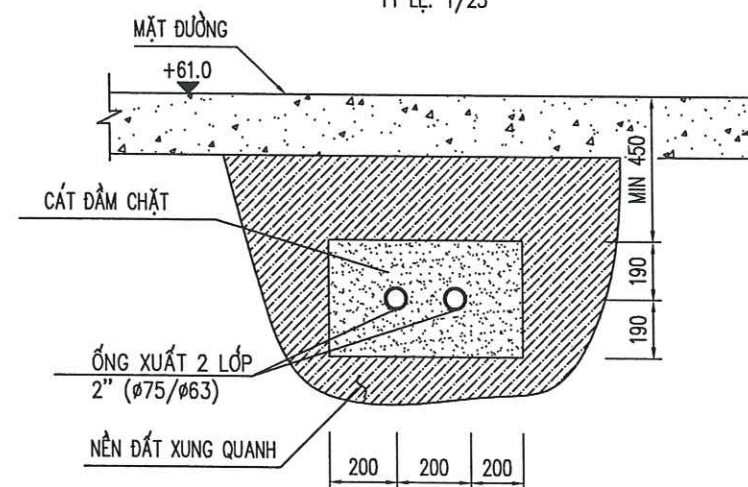
MẶT CẮT 5-5
