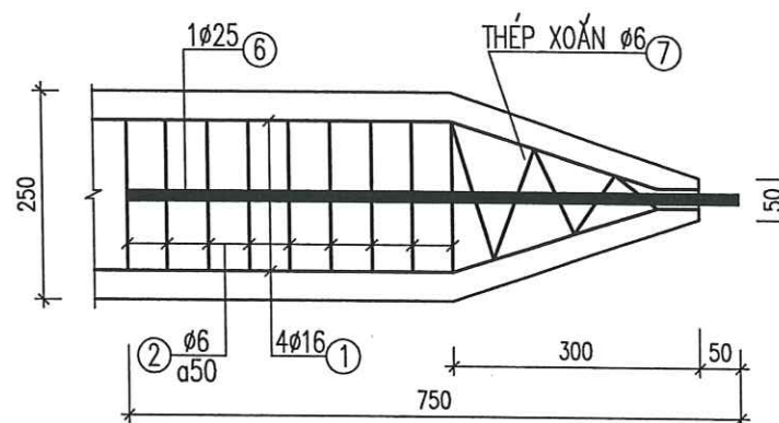
CHI TIẾT B TỶ LỆ: 1/10
