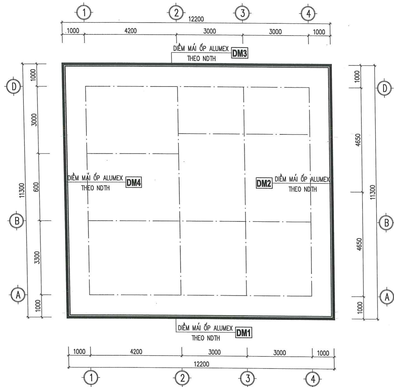
MẶT BẰNG DIỀM MÁI TỶ LỆ: 1/100
