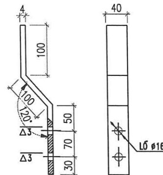
MÁ DƯỚI KẸP KIỂM TRA
