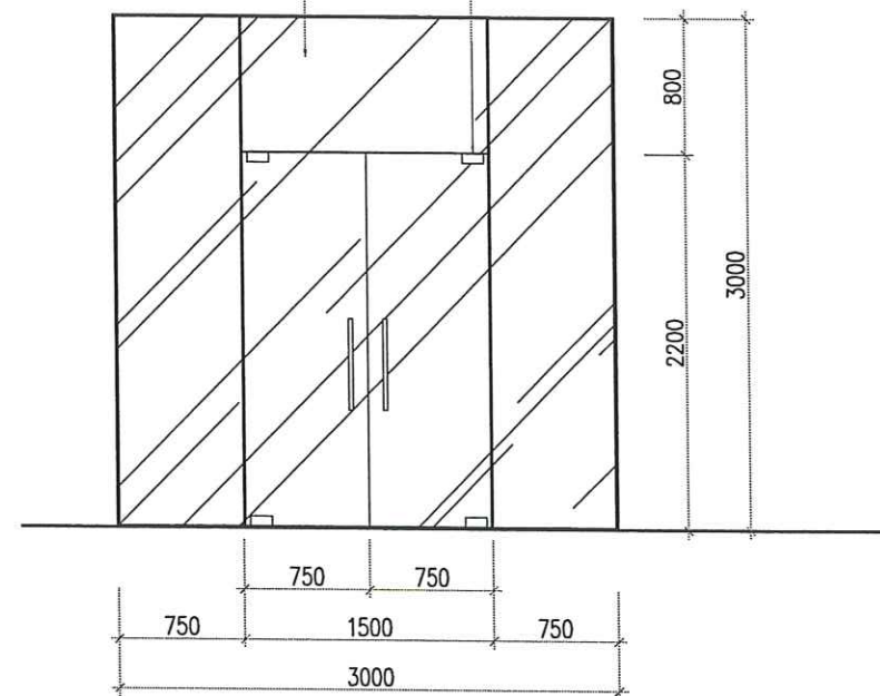
VÁCH KÍNH Đ-VK1 (TỶ LỆ: 1/50)
