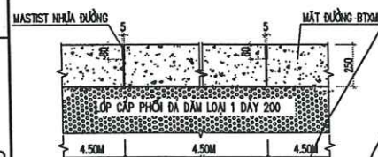
CẤU TẠO KHE CO XÊ KHỎ
