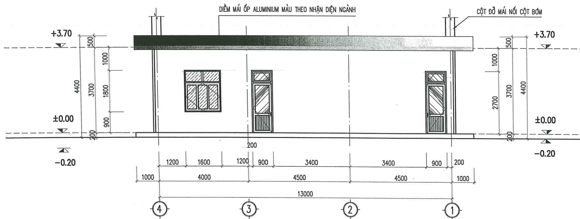
MẶT ĐỨNG TRỰC 4-1
