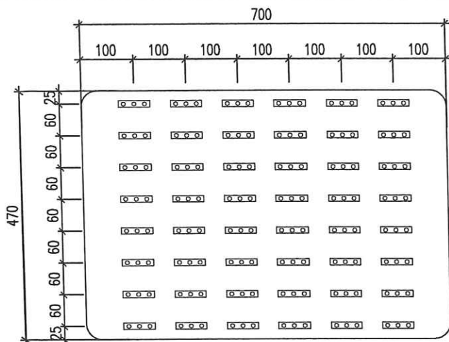
BỐ TRÍ LED BÊN TRONG ICON MẶT HÀNG TỶ LỆ: 1/10
