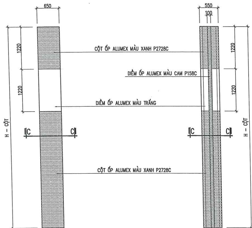
CHI TIẾT CỘT MÁI CHE CỘT BƠM
