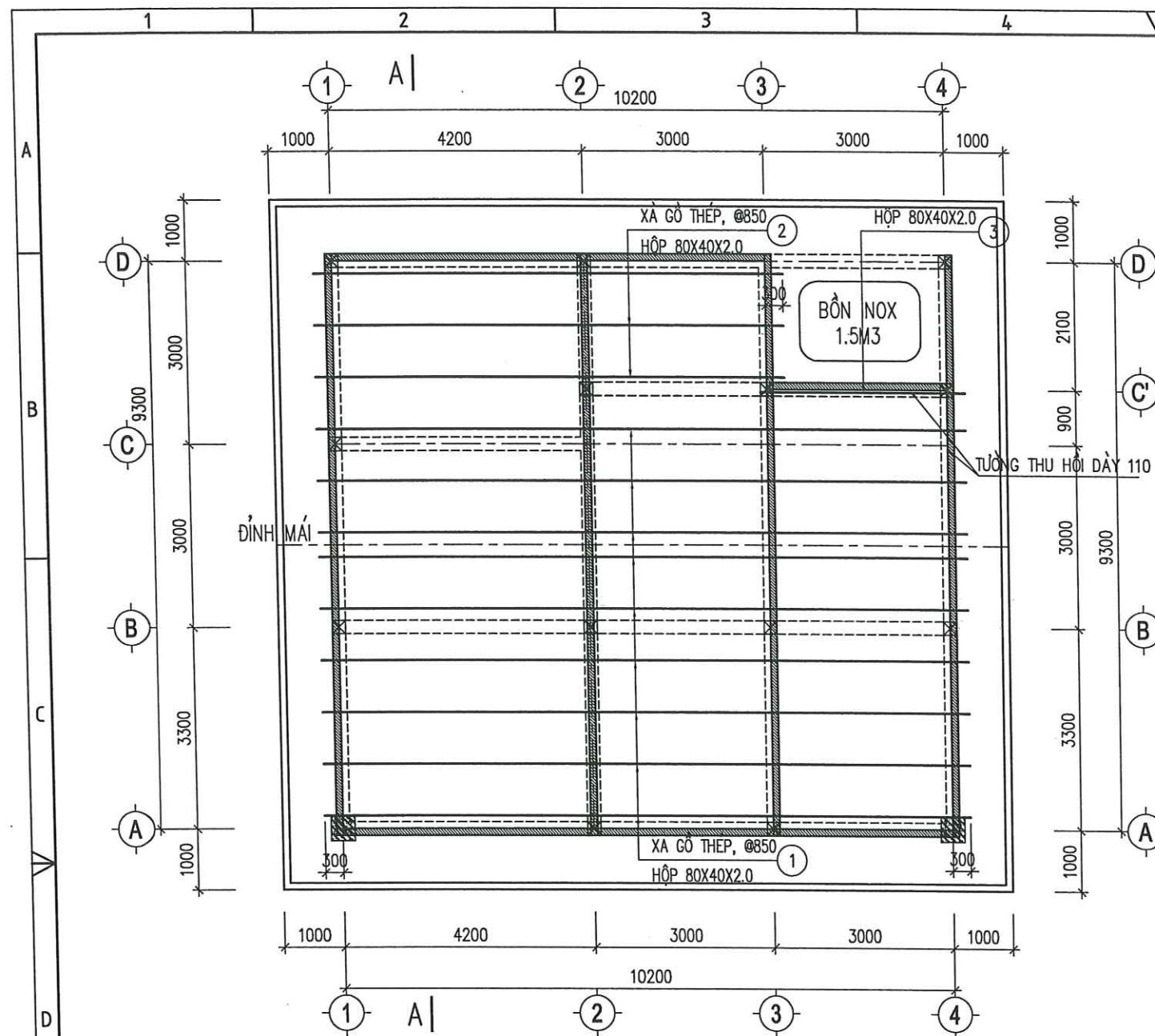
MẶT BẰNG BỐ TRÍ XÀ GỖ MÁI TỶ LỆ: 1/100
