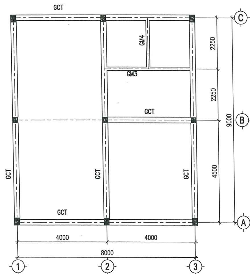
MẶT BẰNG GIẰNG CHỐNG THẨM TỶ LỆ: 1/100
