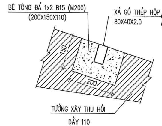
CHI TIẾT CON KÊ XÀ GỖ
