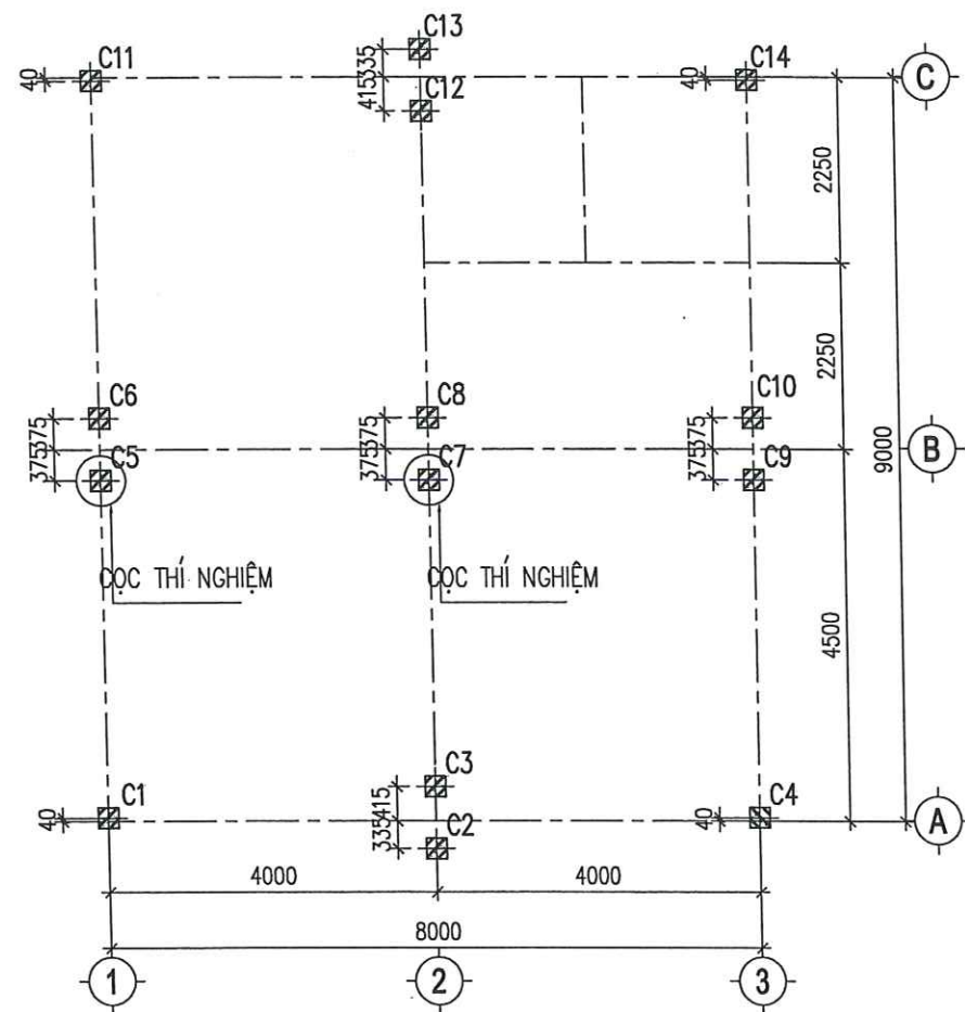
MẶT BẰNG BỐ TRÍ CỌC TỶ LỆ: 1/100
