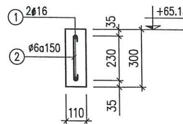
GT-01 (L=2,415M; SL:01) TỶ LỆ: 1/20
