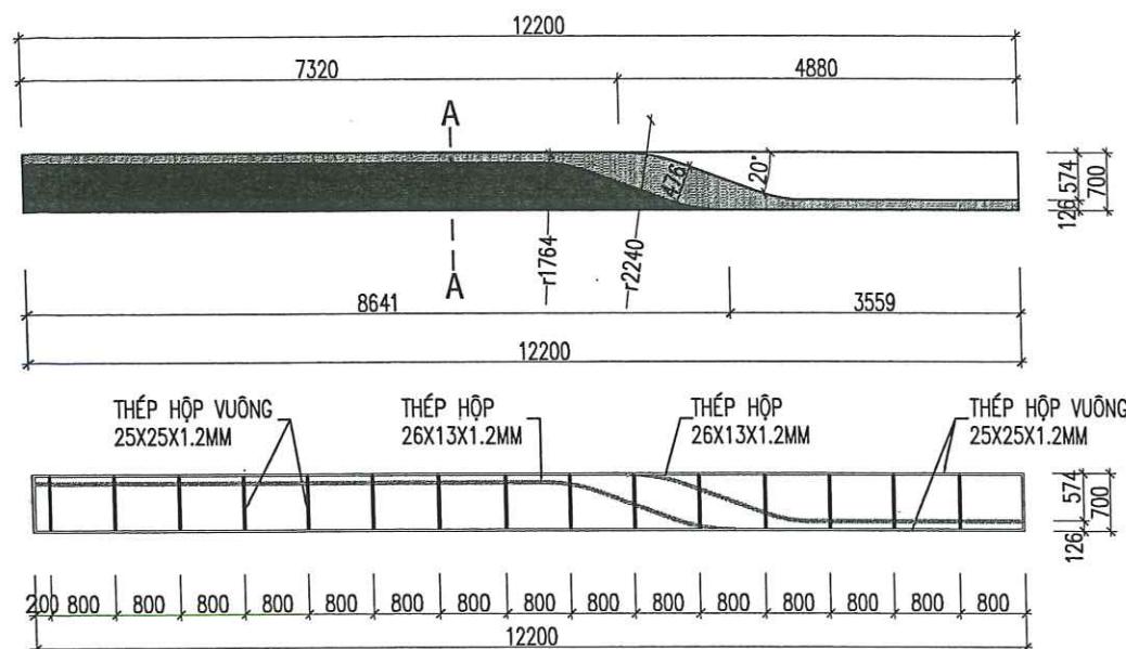
CHI TIẾT DIỂM MÁI TRỤC 1-4 (DM1) VÀ TRỤC 4-1 (DM3) TỶ LỆ : 1/100
