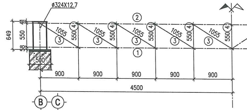
SƠ ĐỒ HÌNH HỌC DÀN D3 TỶ LỆ: 1/50
