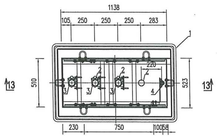
CHI TIẾT HỒ CỘT BƠM 6 VỎI 40-70L/P
