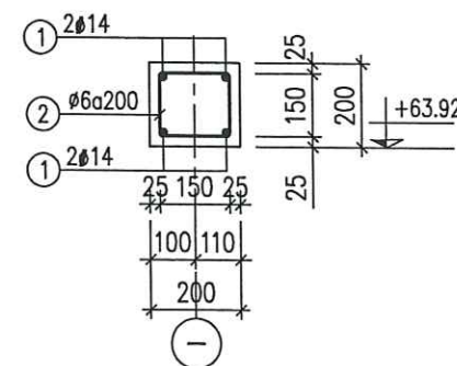
LANH TÔ LT-D2 (L=4290, SL:01)
