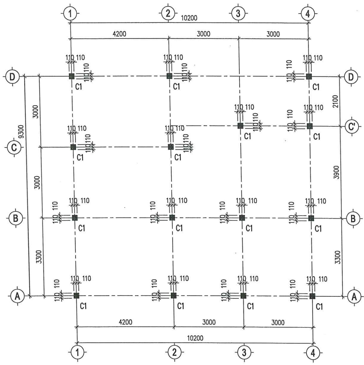
MẶT BẰNG ĐỊNH VỊ CỘT TỶ LỆ: 1/100
