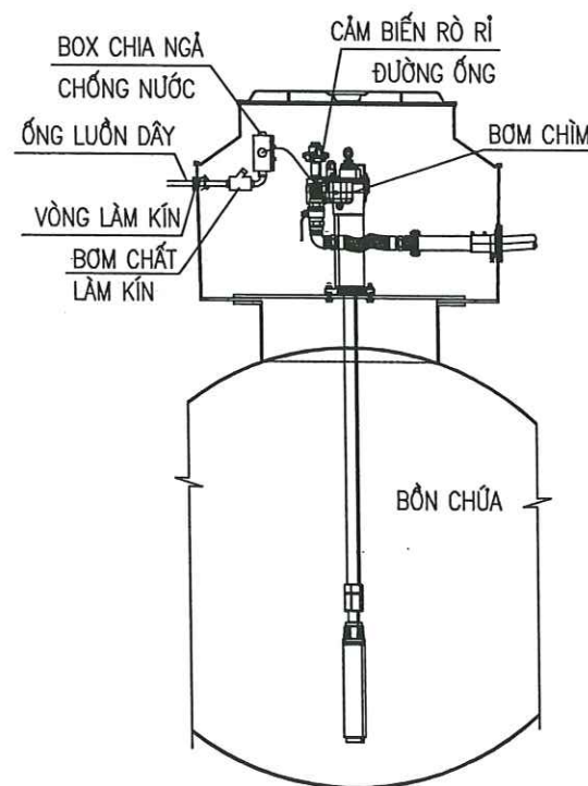
CTLĐ CẢM BIẾN RÒ RỈ ĐƯỜNG ỐNG
