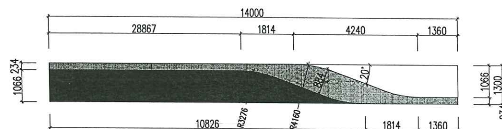
CHI TIẾT DIỂM MÁI 2-1 (DM3) TỶ LỆ : 1/100
