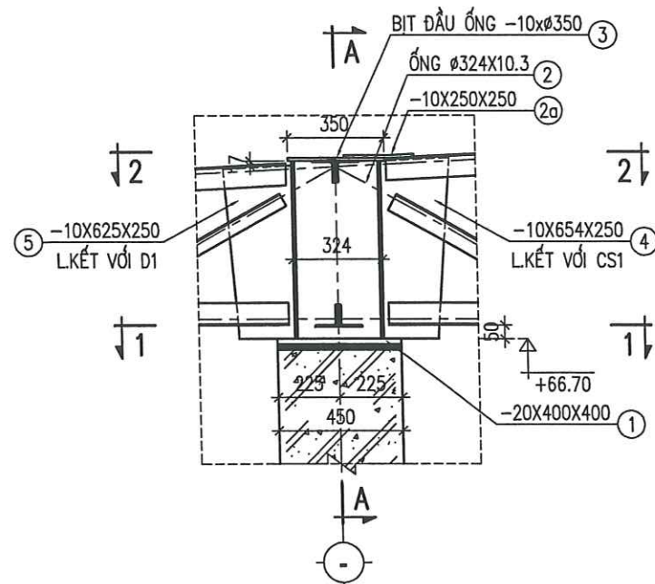
CHI TIẾT ĐẦU CỘT TỶ LỆ: 1/25
