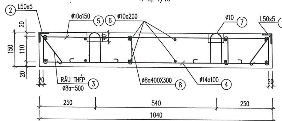
MẶT CẮT A-A TỶ LỆ 1/10
