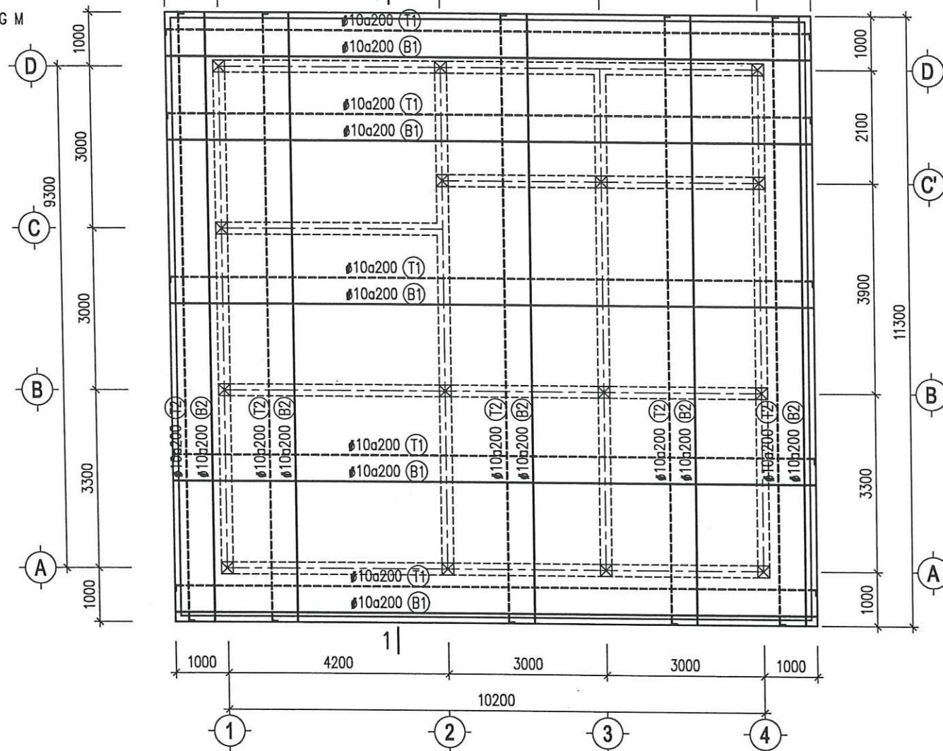
MẶT BẰNG BỐ TRÍ CỐT THÉP MÁI TỶ LỆ: 1/100
