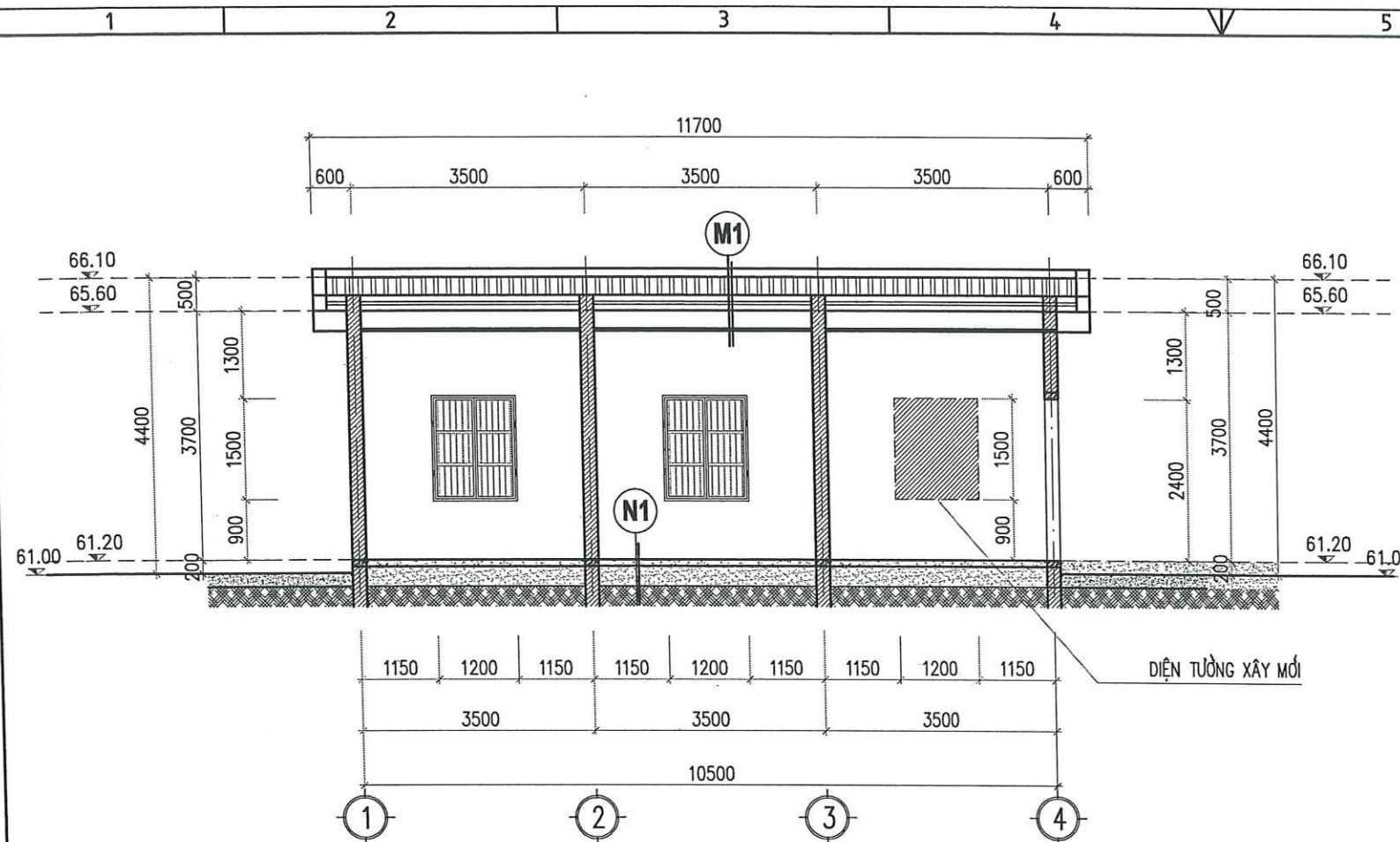
MẶT CẮT B - B
