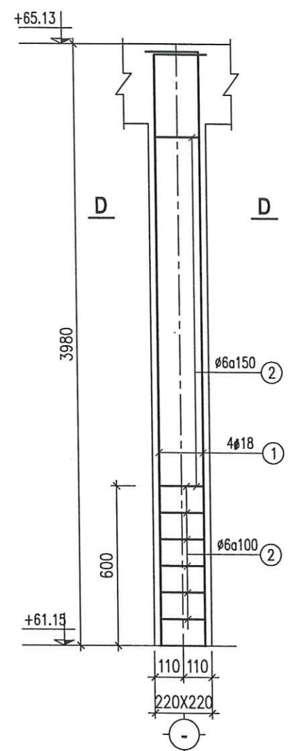
CỘT C2 (SL:03) TỶ LỆ: 1/25
