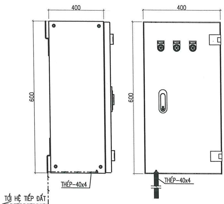
CHI TIẾT LIÊN KẾT TIẾP ĐẤT - TỦ ĐIỆN (ĐIỂN HÌNH)
