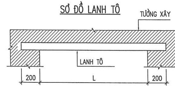
LANH TÔ LT-S1 (L=2000, SL:03)
