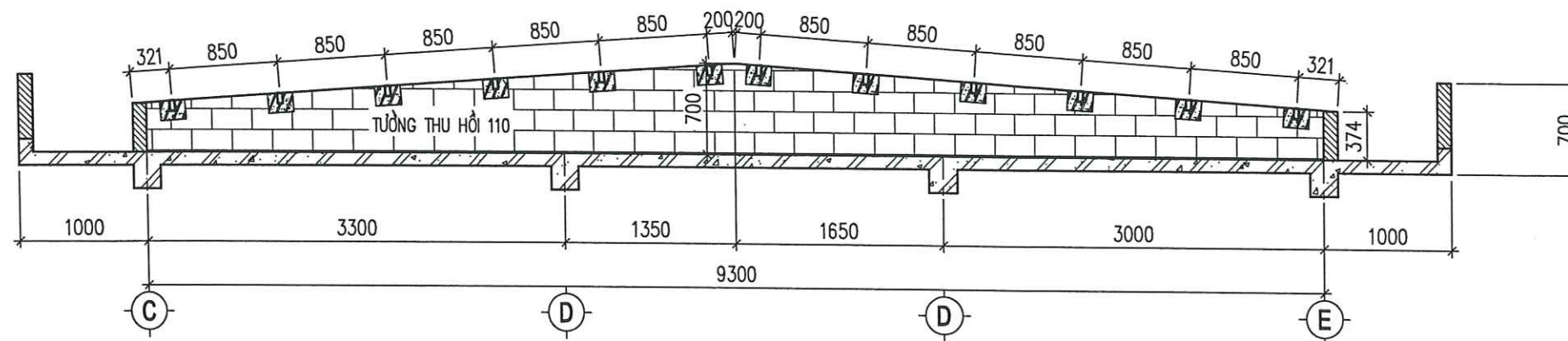
MẶT CẮT A-A TỶ LỆ: 1/25
