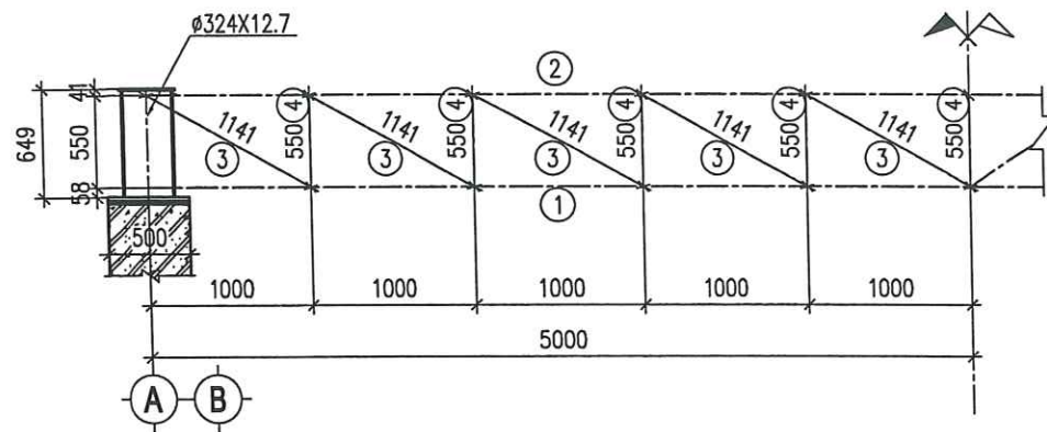
SƠ ĐỒ HÌNH HỌC DÀN D2 TỶ LỆ: 1/50
