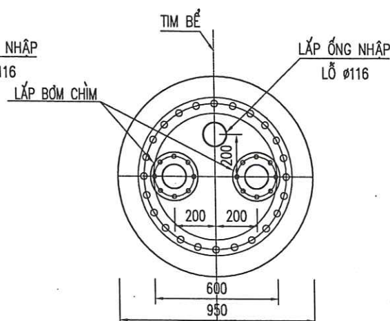
KHOÉT LỖ NẮP ĐẦM BỂ DO-0.05S
