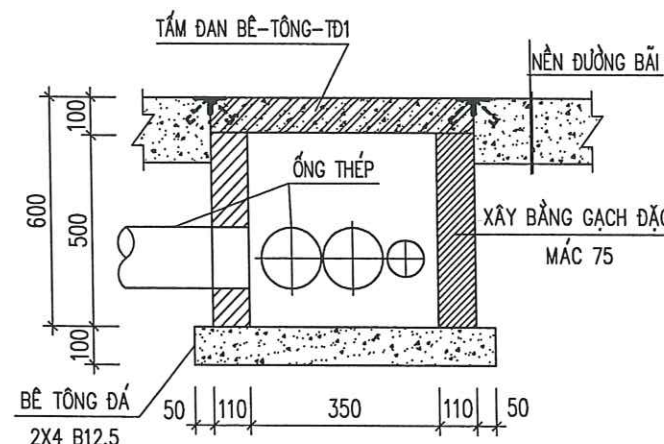
CẮT 1-1
