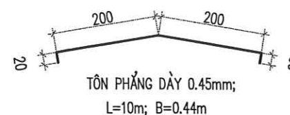
CHI TIẾT TÔN ỨP NÓC (SL: 01 CÁI)
