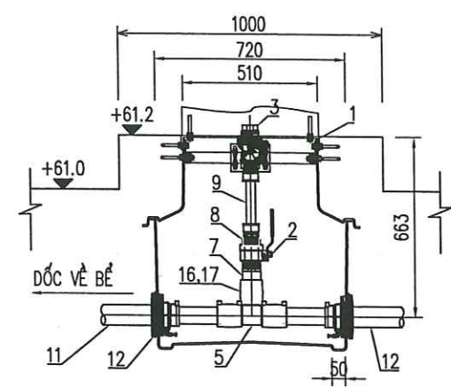
MẶT CẮT 15-15 TẠI ĐIỂM CHUYỂN TIẾP
