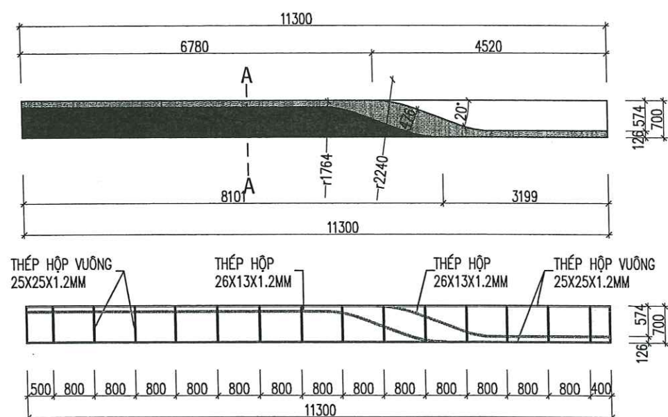
CHI TIẾT DIỂM MÁI TRỤC D-A (DM4) TỶ LỆ : 1/100
