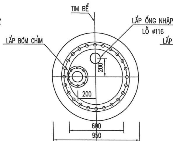
KHOÉT LỖ NẮP ĐẦM BỂ RON95
