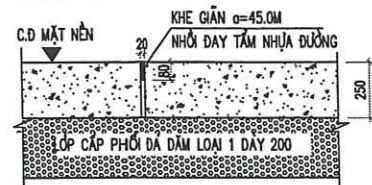
CẤU TẠO KHE DẪN
