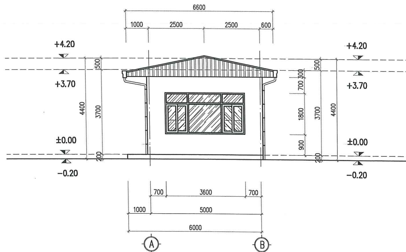
MẶT ĐỨNG TRỤC A - B
