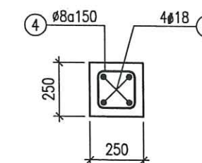
MẶT CẮT B-B TỶ LỆ: 1/25
