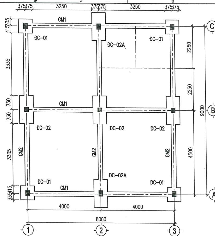
MẶT BẰNG MÓNG TỶ LỆ: 1/100
