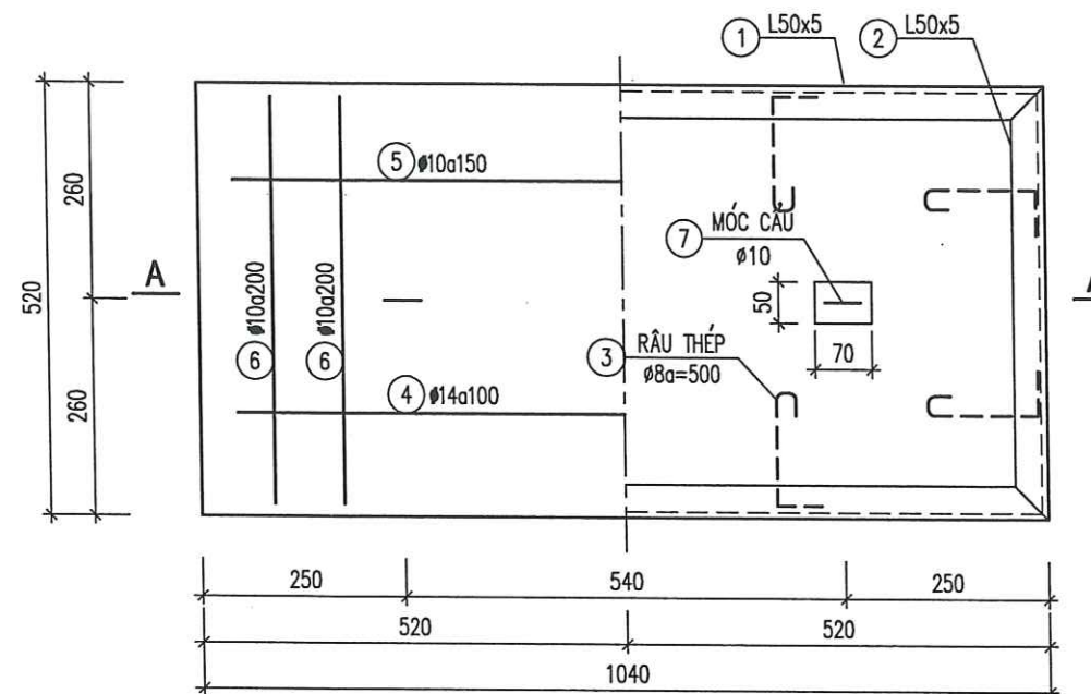
TẤM ĐAN TĐ1 TỶ LỆ 1/10 (1040x520x150)
