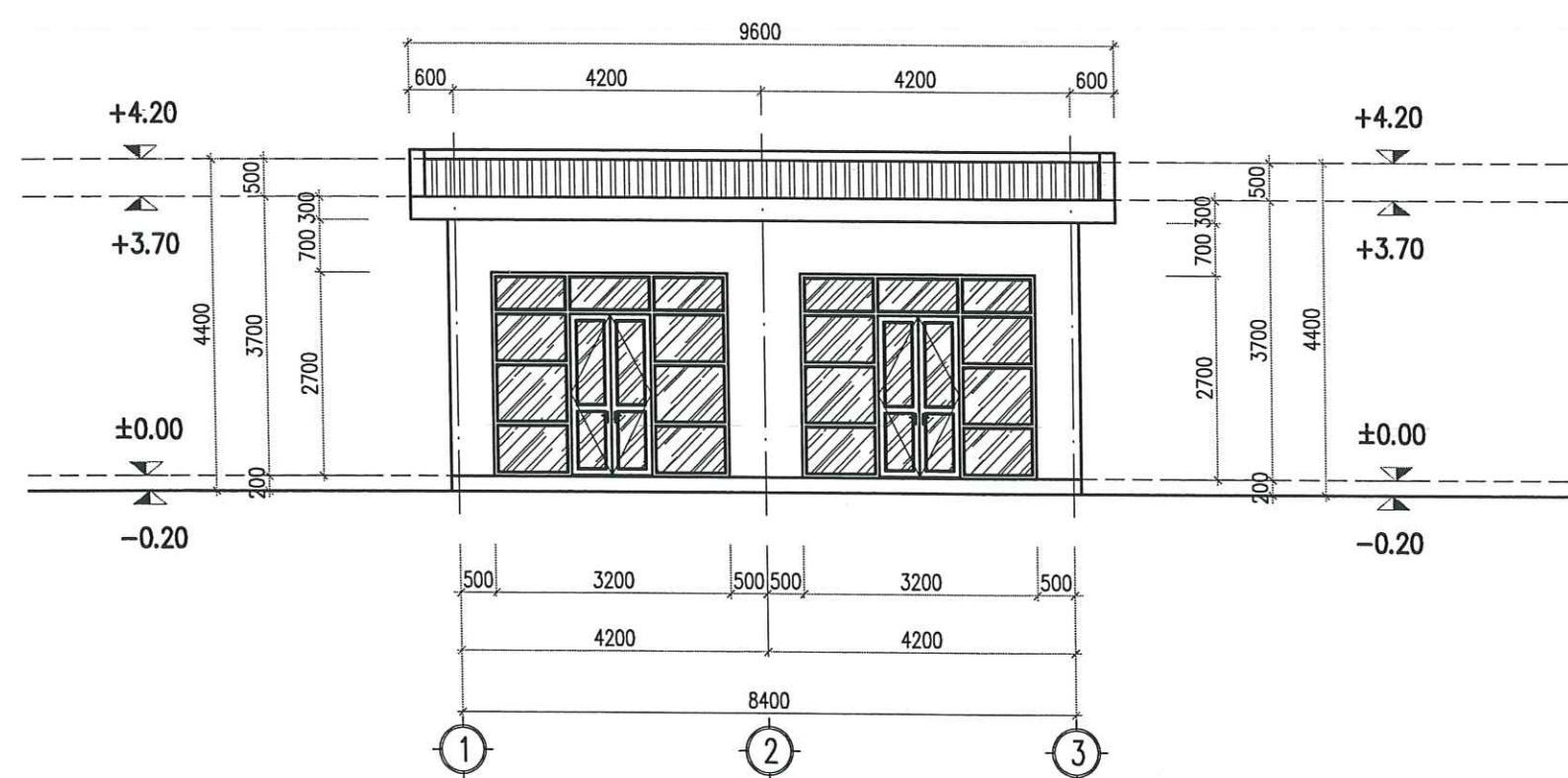
MẶT ĐỨNG TRỤC 1-3
