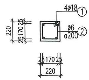
MẶT CẮT 1-1 TỶ LỆ: 1/10
