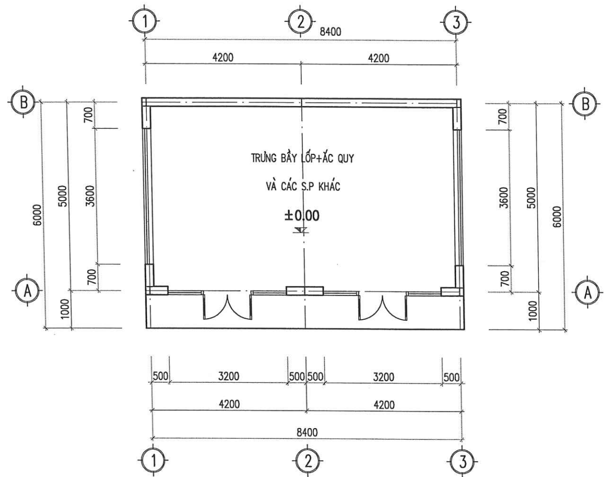
MẶT BẰNG NHÀ TRƯNG BÀY
