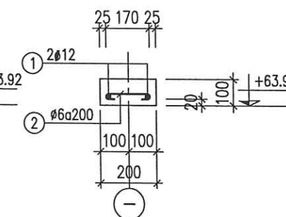
LANH TÔ LT-D2 (L=4290, SL:01)
