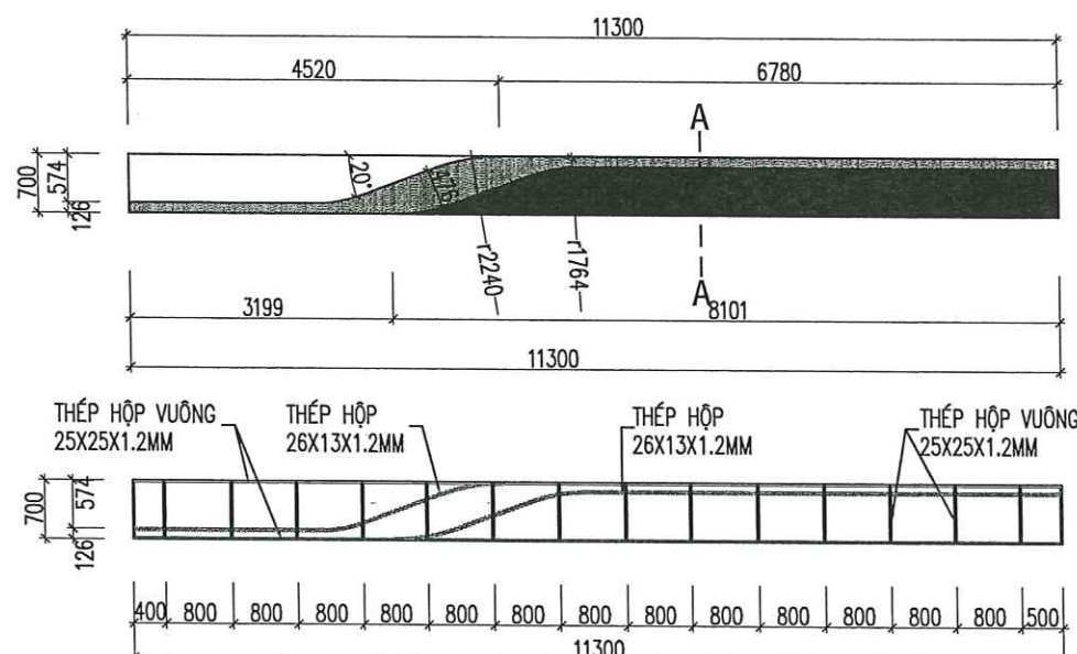
CHI TIẾT DIỂM MÁI TRỤC A-D (DM2) TỶ LỆ : 1/100
