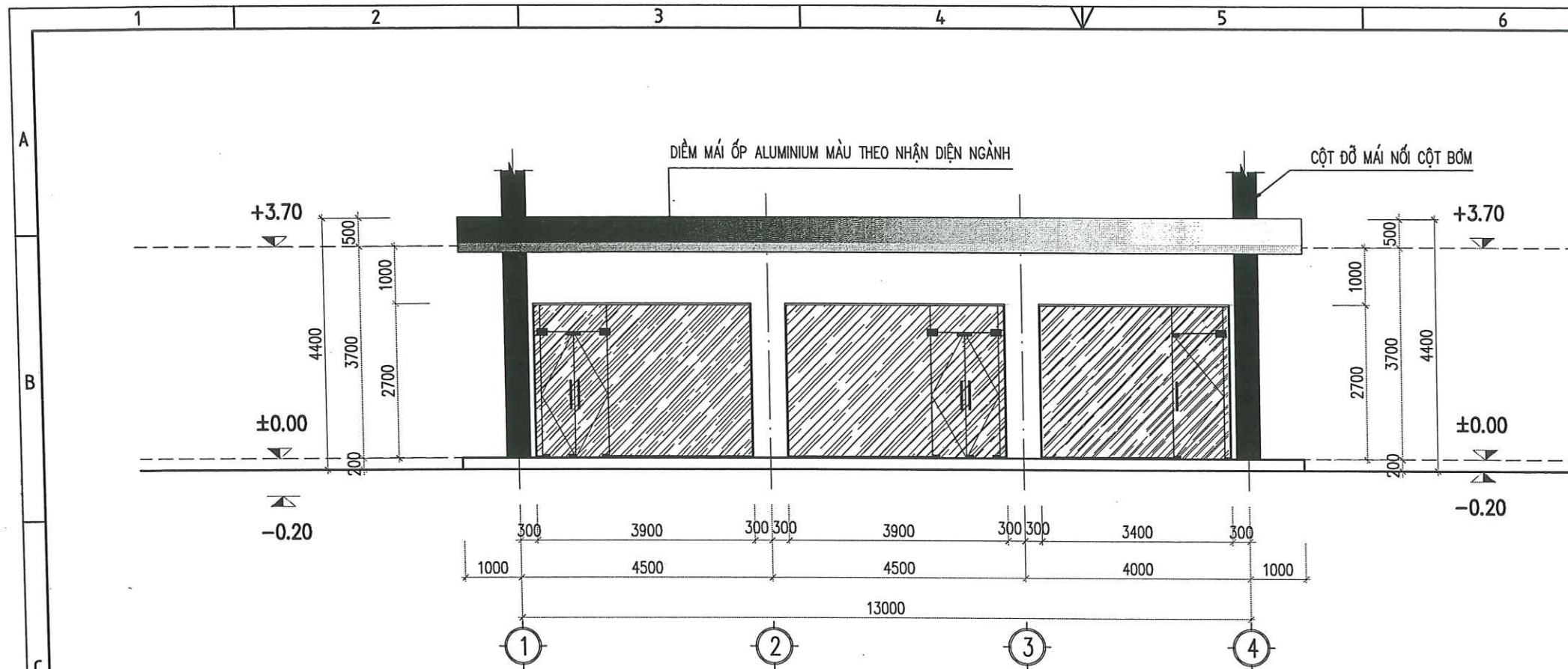
MẶT ĐỨNG TRỰC 1-4
