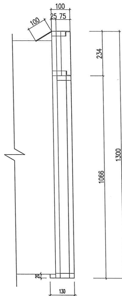
MẶT CẮT A-A (TỶ LỆ : 1/10)
