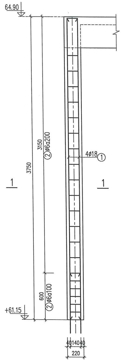
CHI TIẾT CỘT C1 (SL:15) TỶ LỆ: 1/25
