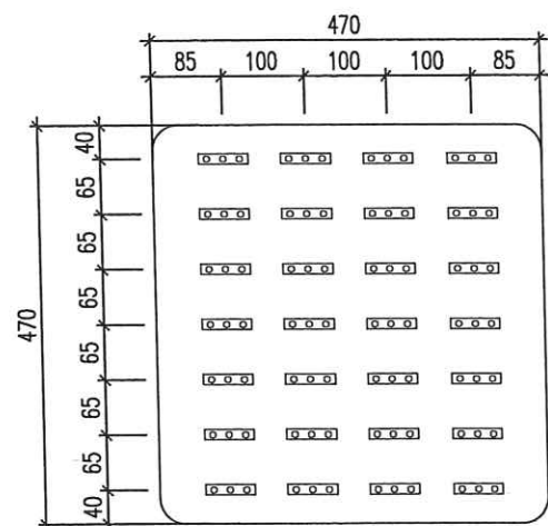
BỐ TRÍ LED BÊN TRONG ICON TIỆN ÍCH TỶ LỆ: 1/10
