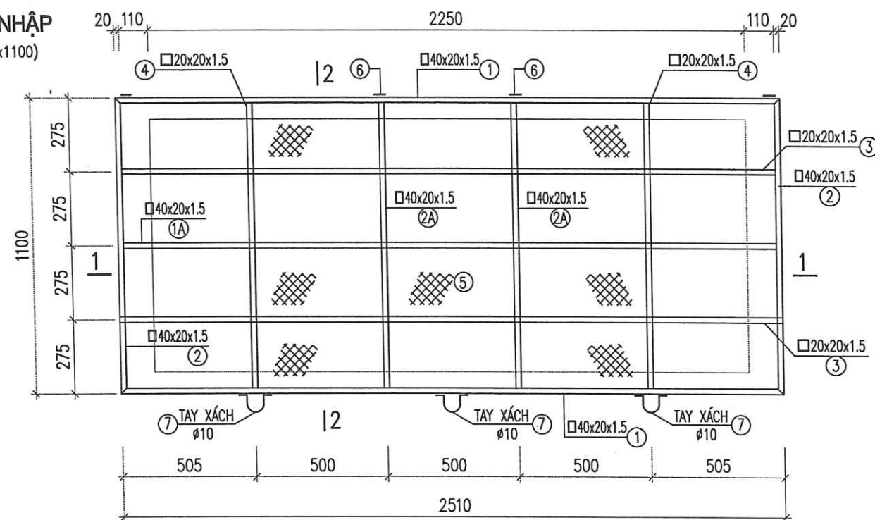
CẮT CẮT 1-1 TỶ LỆ: 1/20 2510 INOX 304 S=0.8MM 2a 40x20x1.5 1a 40x20x1.5 2a 40x20x1.5 2 40x20x1.5 20x20x1.5 4 CD NỀN KHU BÊ H=250-500 745 100 50 110 2250 110 50 2510 NỀN BÊ TÔNG ĐÁ 1X2 B12.5 1 LỚP LỐT NYLON ĐẦM CHẶT LỚP CÁT DƯỚI ĐÁY
