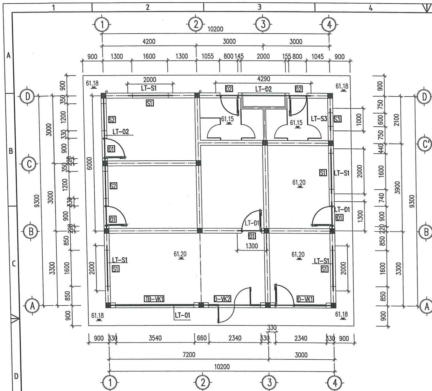
MẶT BẰNG BỐ TRÍ LANH TÔ TỶ LỆ: 1/100
