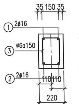
DẦM DM2-1 (L=8,22M; SL:03) TỶ LỆ: 1/20
