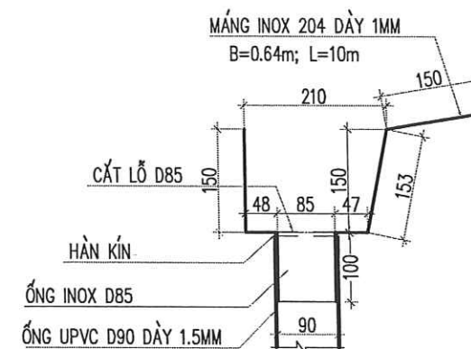
CHI TIẾT LIÊN KẾT MĂNG NƯỚC VỚI ỐNG UPVC D90
