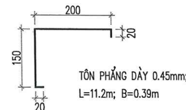
CHI TIẾT TÔN ỨP NÓC BIÊN (SL: 02 CÁI)
