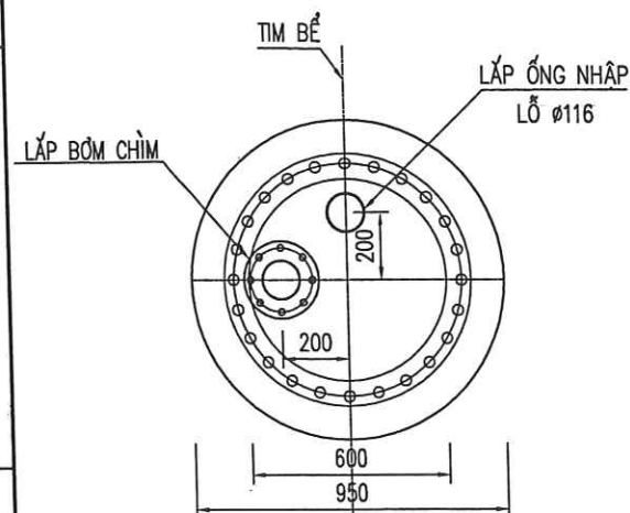
KHOÉT LỖ NẮP ĐẦM BỂ E5-RON92
