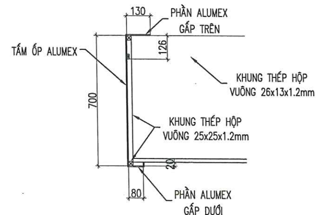
MẶT CẮT A-A TỶ LỆ : 1/20
