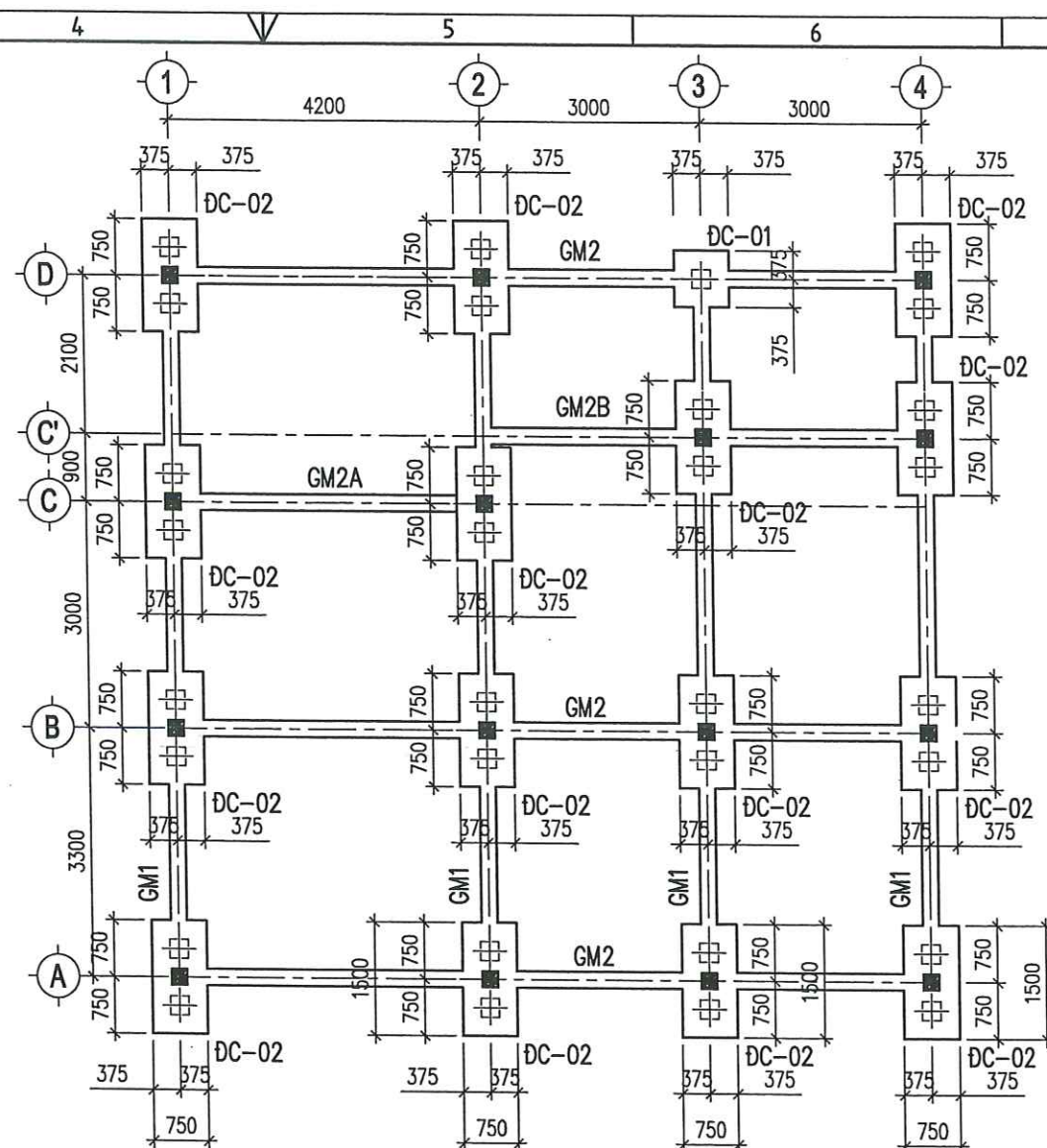
MẶT BẰNG MÓNG TỶ LỆ: 1/100
