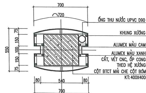
MẶT CẮT C-C
