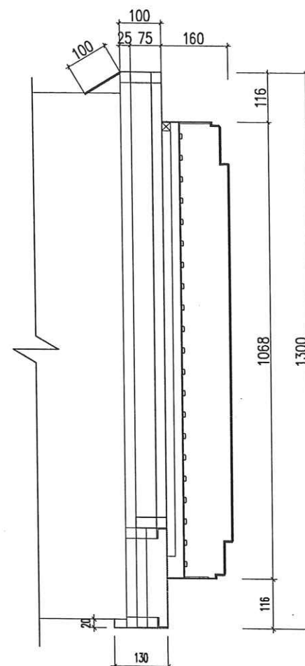
MẶT CẮT B-B (TỶ LỆ : 1/10)
