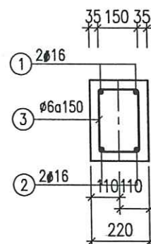
DẦM DM2-2 (L=9,22M; SL:03) TỶ LỆ: 1/20
