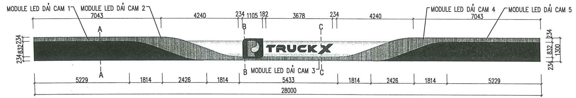
CHI TIẾT DIỀM MÁI TRỤC A-C (DM2) VÀ C-A (DM4) TỶ LỆ : 1/100
