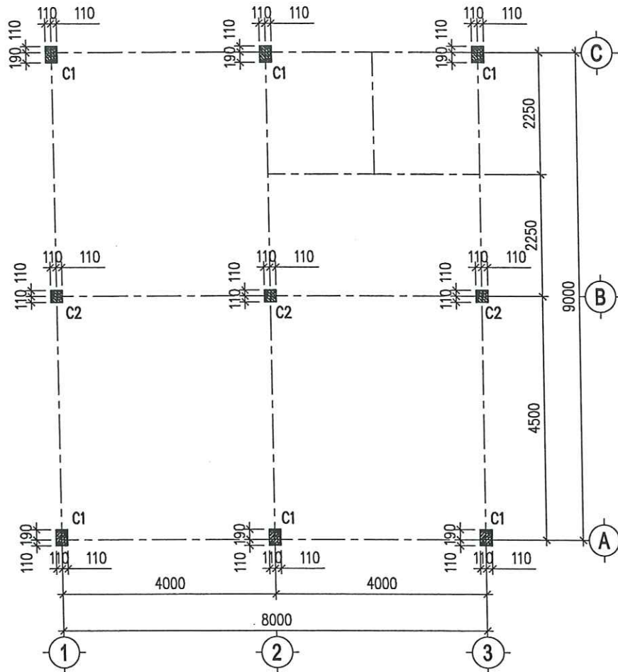
MẶT BẰNG ĐỊNH VỊ CỘT TỶ LỆ: 1/100
