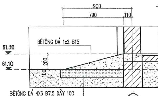
CHI TIẾT ĐƯỜNG DỐC TL:1/25
