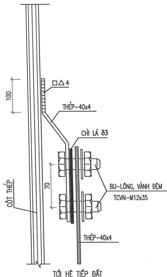
KẸP KIỂM TRA KZ-2 KẾT NỐI CỘT THÉP TỚI HỆ TIẾP ĐẤT (ĐIỂN HÌNH)
