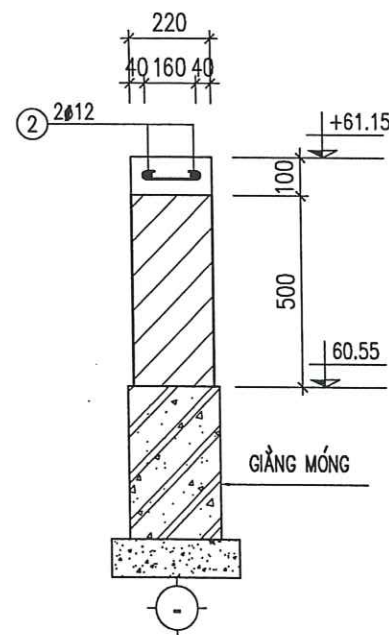
GIẺNG CHỐNG THẨM GCT (L=72M) TỶ LỆ: 1/20
