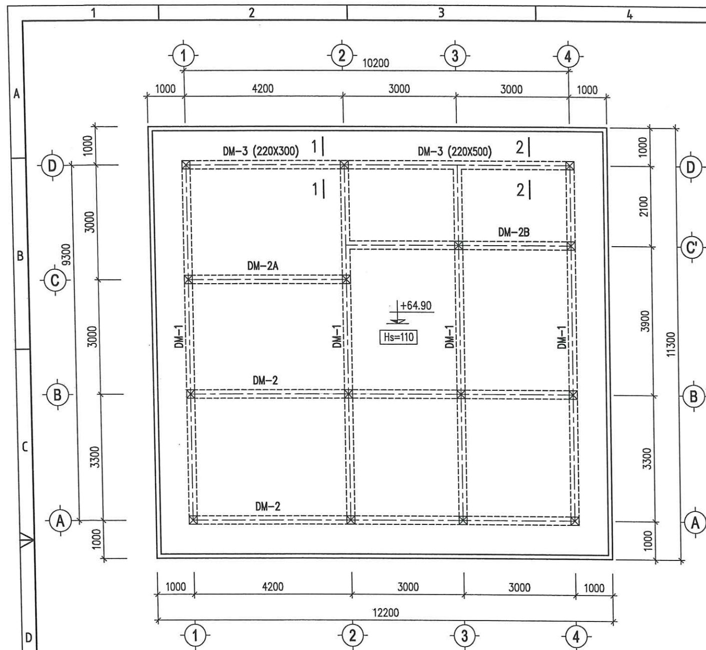
MẶT BẰNG KẾT CẤU TỶ LỆ: 1/100
