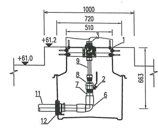
MẶT CẮT 15-15 TẠI ĐIỂM CUỐI
