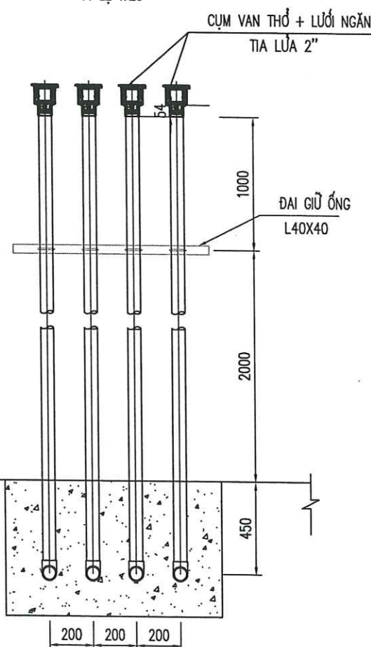
MẶT CẮT 7-7
