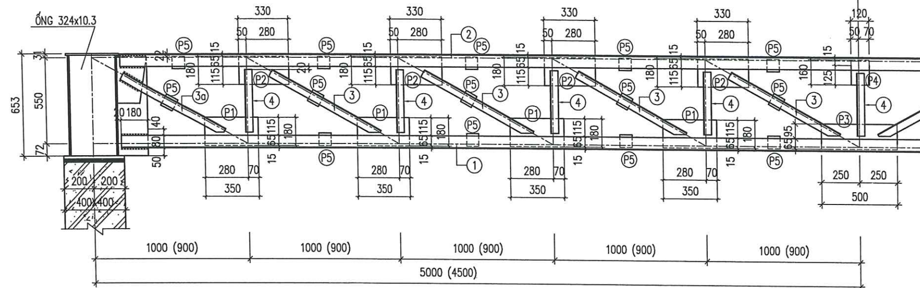
CHI TIẾT DẦM D2 (SL:02) CHI TIẾT DẦM D3 (SL:02) TỶ LỆ: 1/25
