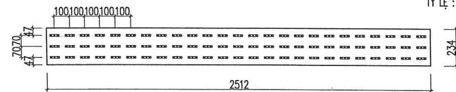
BỐ TRÍ CÁC MODULE LED TẠI DẢI CAM 1 TỶ LỆ : 1/20
