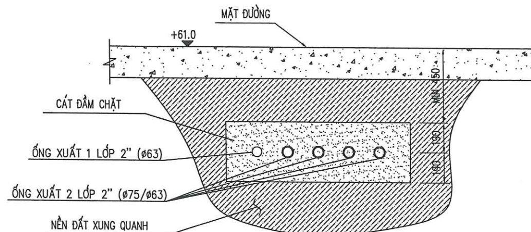
MẶT CẮT 5-5
