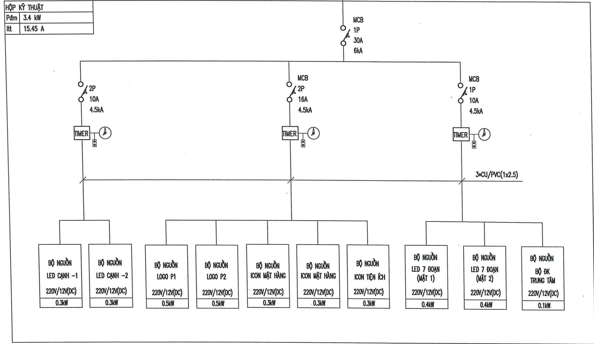
SƠ ĐỒ NGUYÊN LÝ CẤP NGUỒN BÊN TRONG TRỤ BIỂN BÁO GIÁ LOẠI CAO CẤP H=8.6M
