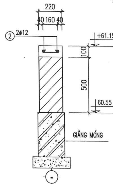
GIẰNG CHỐNG THẨM GCT (L=72M) TỶ LỆ: 1/20
