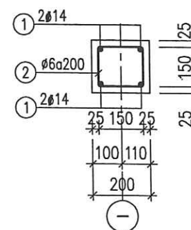
LANH TÔ LT-02 (L=6000, SL:01)
