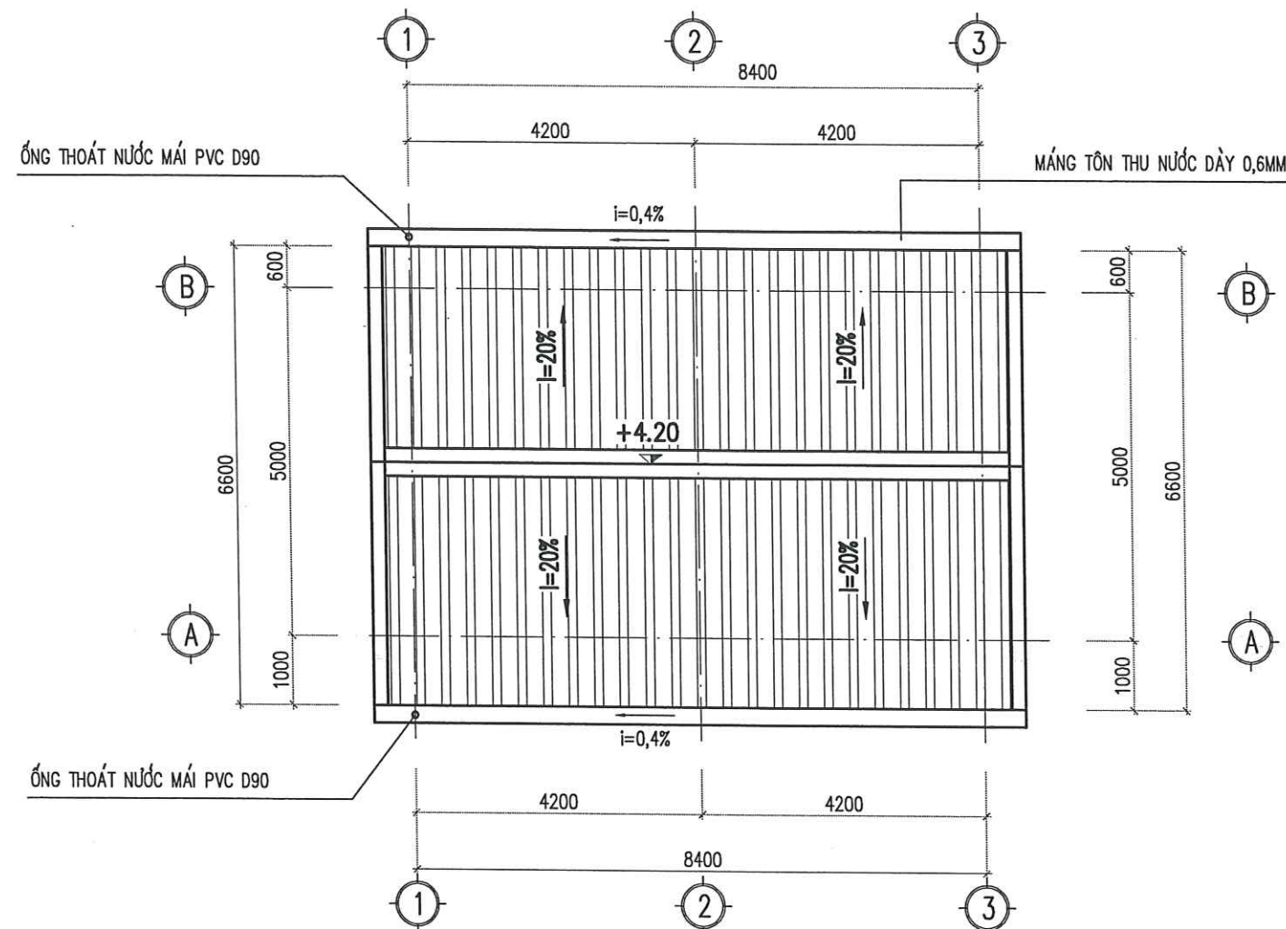
MẶT BẰNG MÁI NHÀ TRƯNG BÀY
