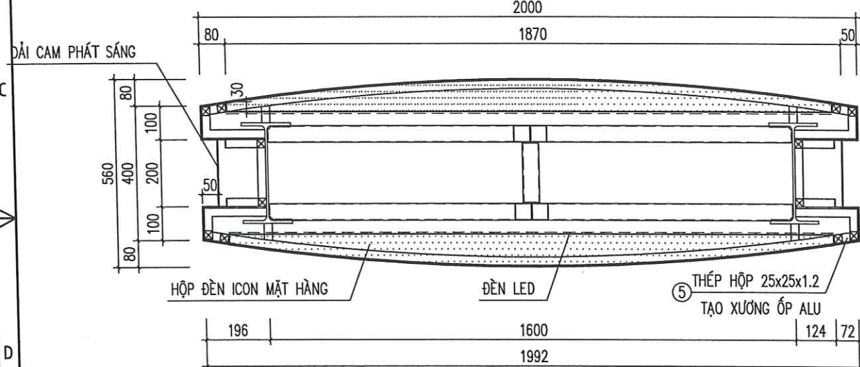
MẶT CẮT B-B
