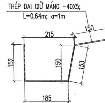
CHI TIẾT ĐAI GIỮ MĂNG NƯỚC (SL: 22 CÁI)
