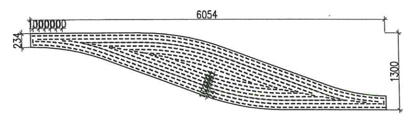
BỐ TRÍ CÁC MODULE LED TẠI DẢI CAM 2 TỶ LỆ : 1/50
