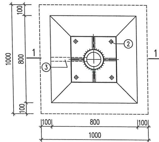
MẶT BẰNG MÓNG
