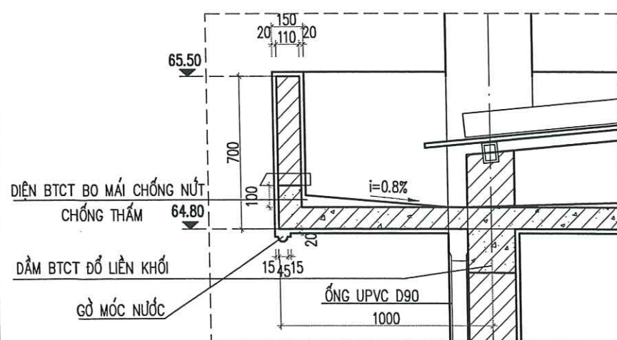
CHI TIẾT SÊ NÔ
