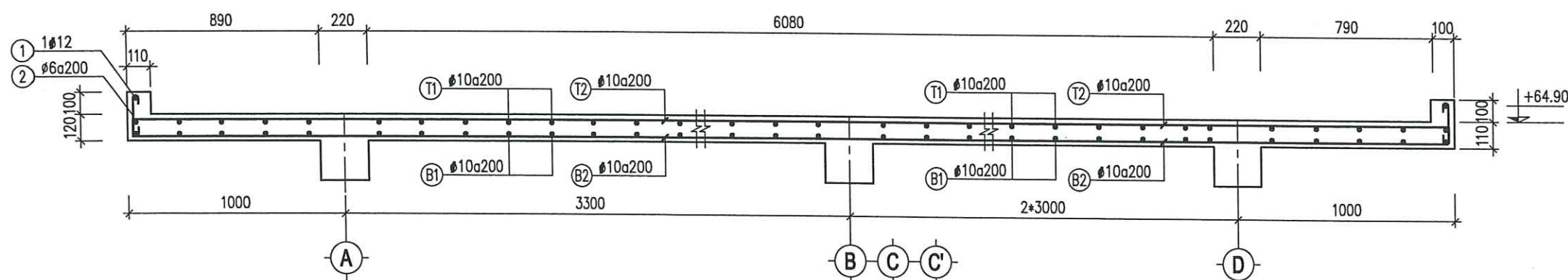
MẶT CẮT 1-1 TỶ LỆ: 1/100
