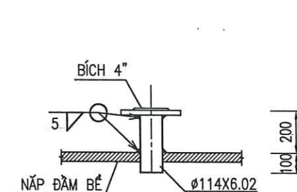
CỔ LỖ ĐO TỰ ĐỘNG
