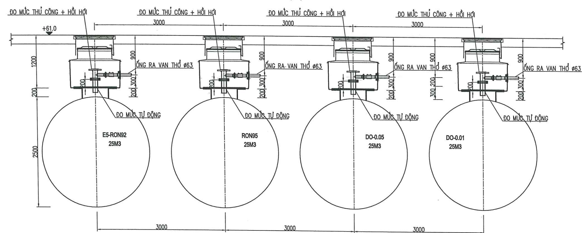
MẶT CẮT 2-2 TỶ LỆ: 1/50
