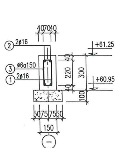
DẦM GM3 (L=2.32 M; SL:02) DẦM GM4 (L=2.07 M; SL:01)
