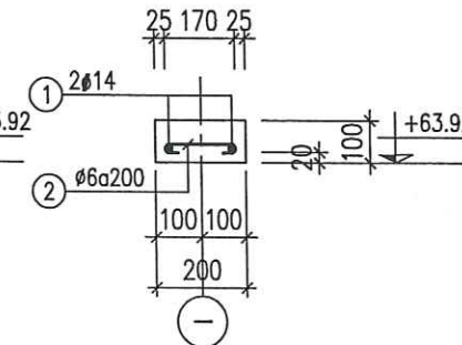
LANH TÔ LT-D1 (L=1300, SL:02)
