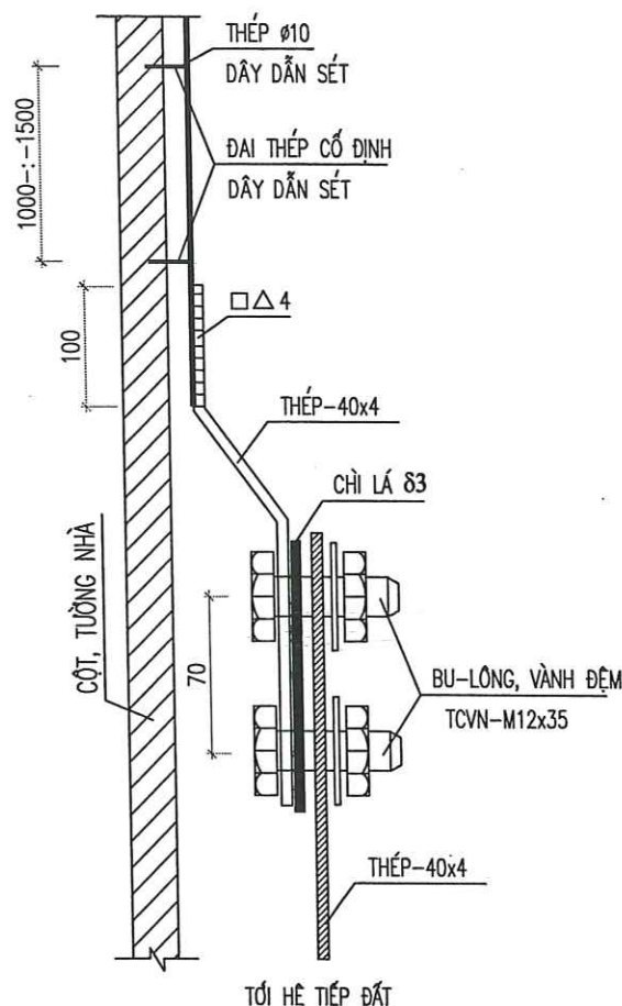
KẸP KIỂM TRA KZ-1 KẾT NỐI TƯỜNG, CỘT NHÀ TỚI HỆ TIẾP ĐẤT (ĐIỂN HÌNH)
