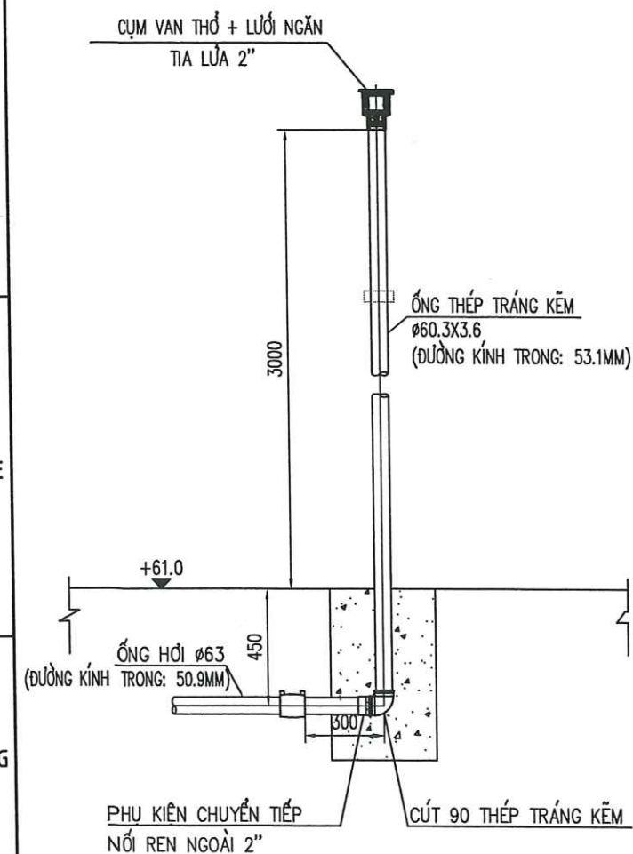
MẶT CẮT 6-6
