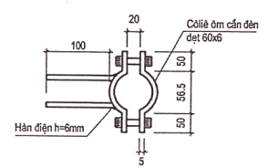
TAY BẮT CẢN ĐÈN
