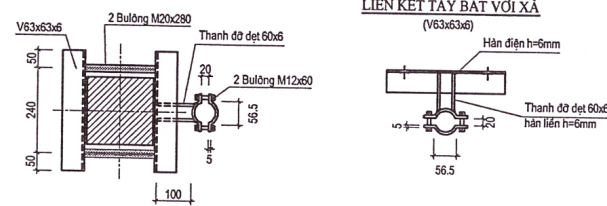
TAY BẮT CẢN ĐÈN
