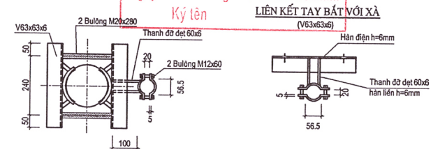
TAY BẮT CẢN ĐÈN
