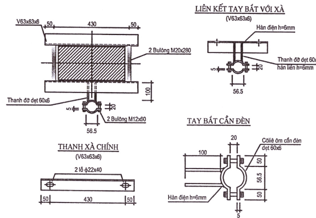
BẢNG KÊ VẬT LIỆU CHO 1 BỘ XÀ BÁT CÁN ĐÈN TRÊN CỘT VUÔNG ĐÔI MẶT PHẪNG NGANG (XÀ TRÊN + XÀ DƯỚI)
