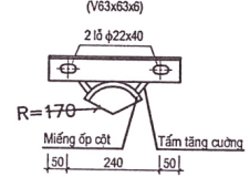
THANH XÀ CHÍNH (V63x63x6)
