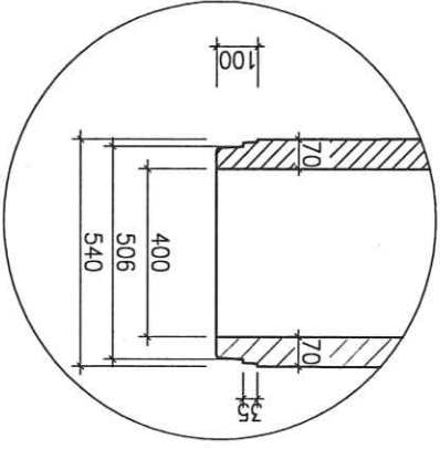
CHI TIẾT B
