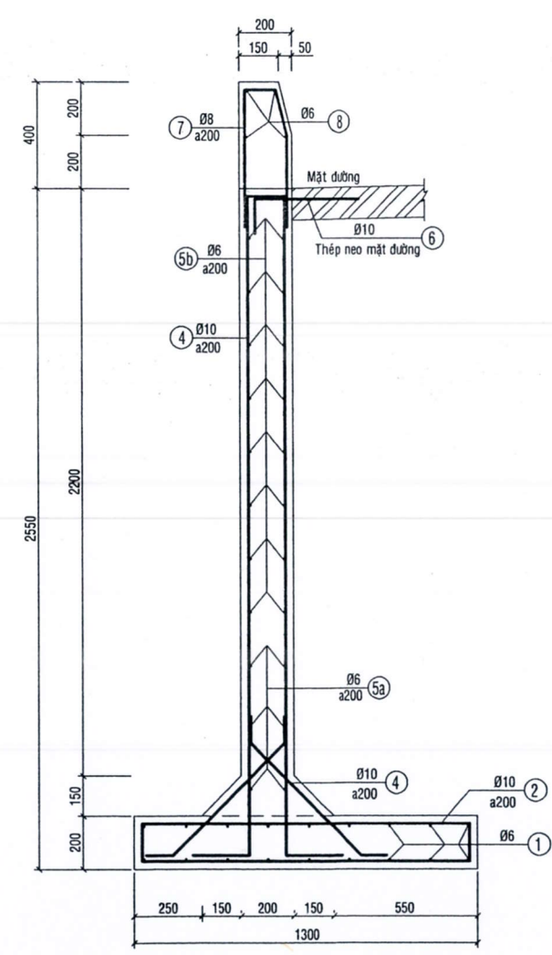
MẶT CẮT A-A TL: 1:25
