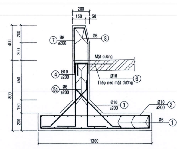
MẶT CẮT B-B TL: 1:25
