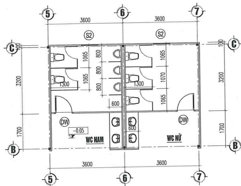
MẶT BẰNG NHÀ VỆ SINH
