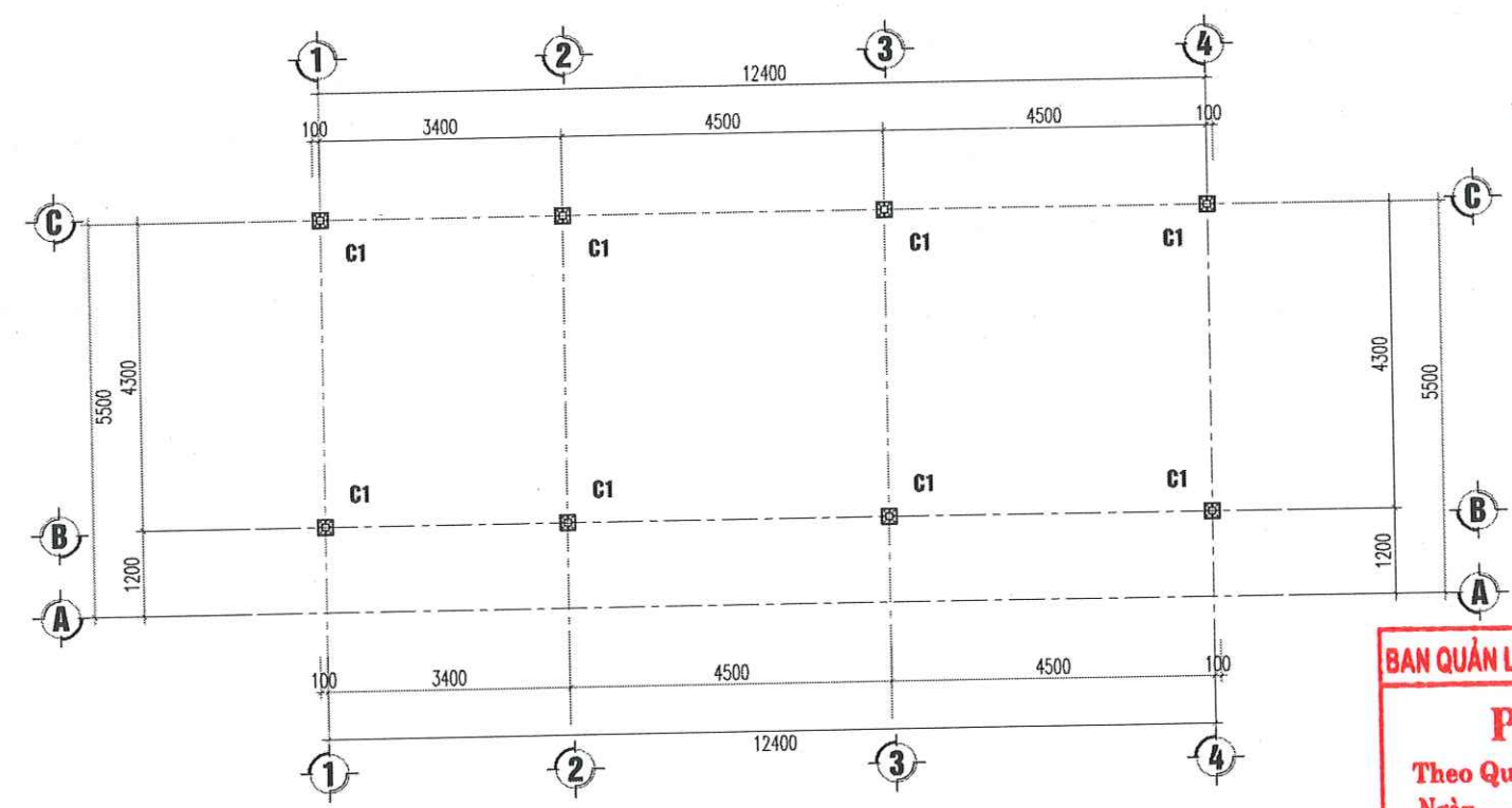
MẶT BẰNG ĐỊNH VỊ CỘT NHÀ B
