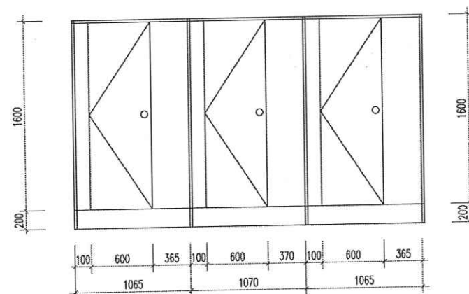
MẶT ĐÚNG VÁCH NGĂN WC NỮ
