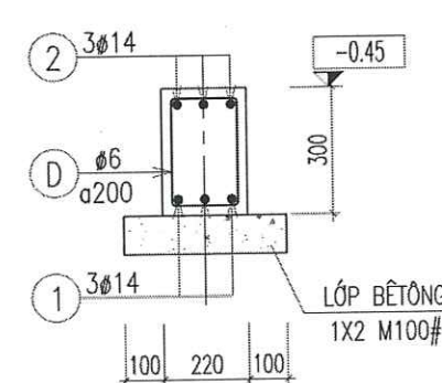
DẦM GM2 (SL= 06, L= 6.42M)
