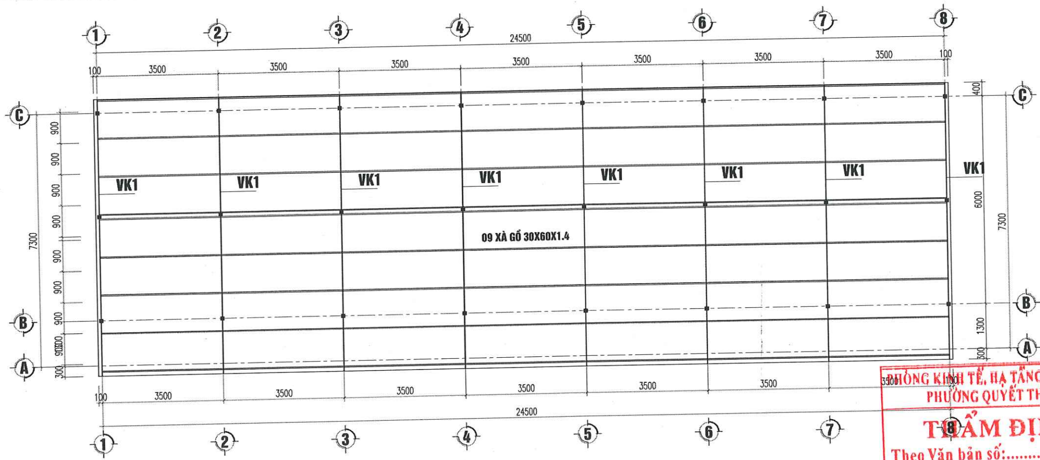
MẶT BẰNG VÌ KÈO+ XÀ GỖ NHÀ C
