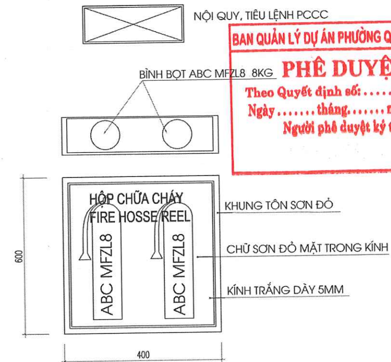
CHI TIẾT BÌNH CHỮA CHÁY TẠI CHỖ
