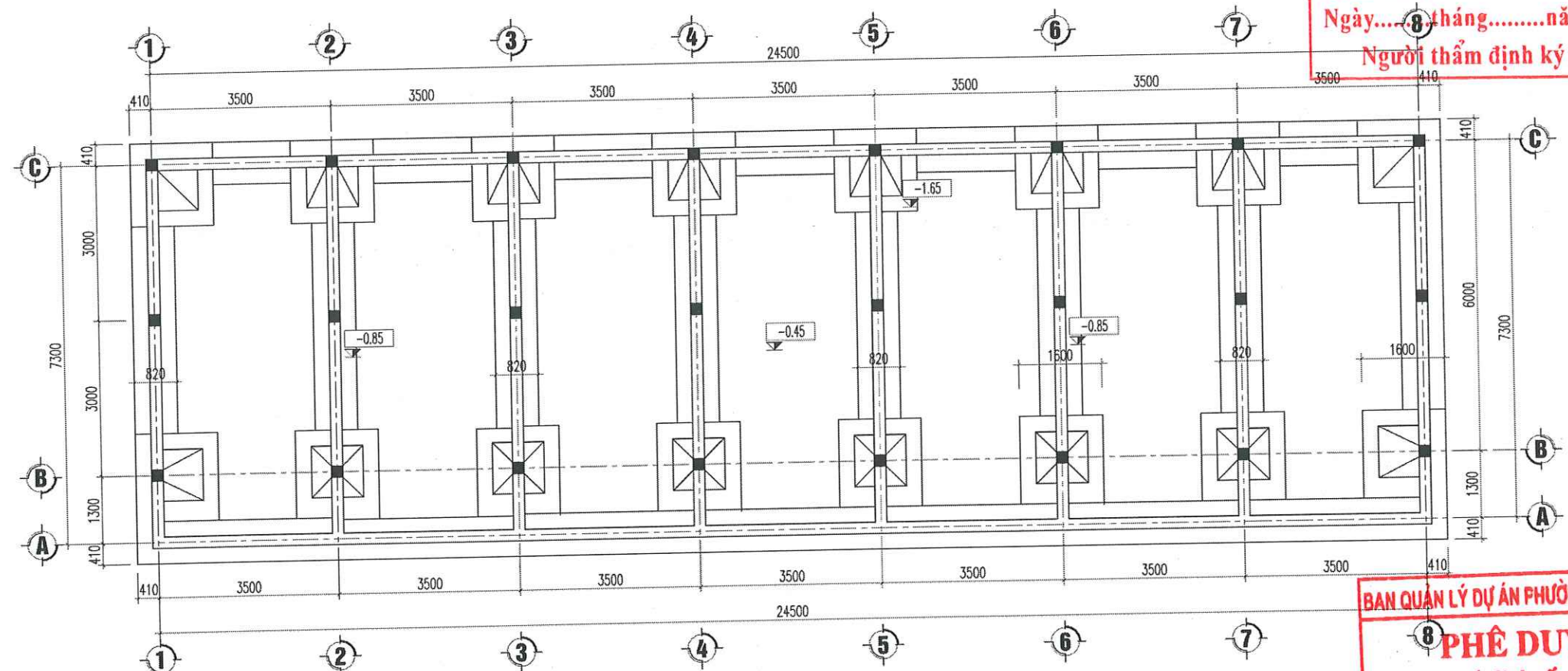
MẶT BẰNG ĐỊNH HƯỚNG ĐÀO MÓNG NHÀ C
