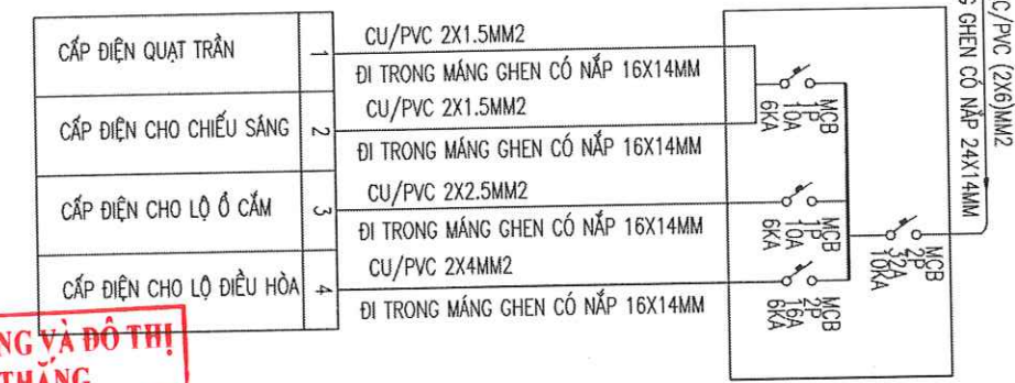
SƠ ĐỒ BẢNG ĐIỆN BD3
