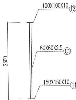
CỘT NHÀ BẢO VỆ
