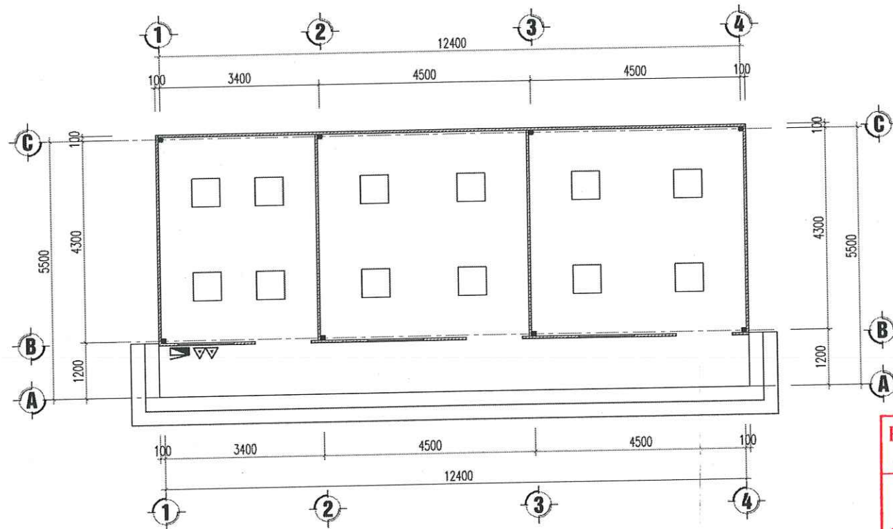
MẶT BẰNG PCCC TẠI CHỖ
