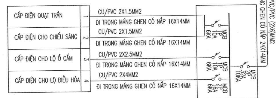
SƠ ĐỒ BẢNG ĐIỆN BD1-5
