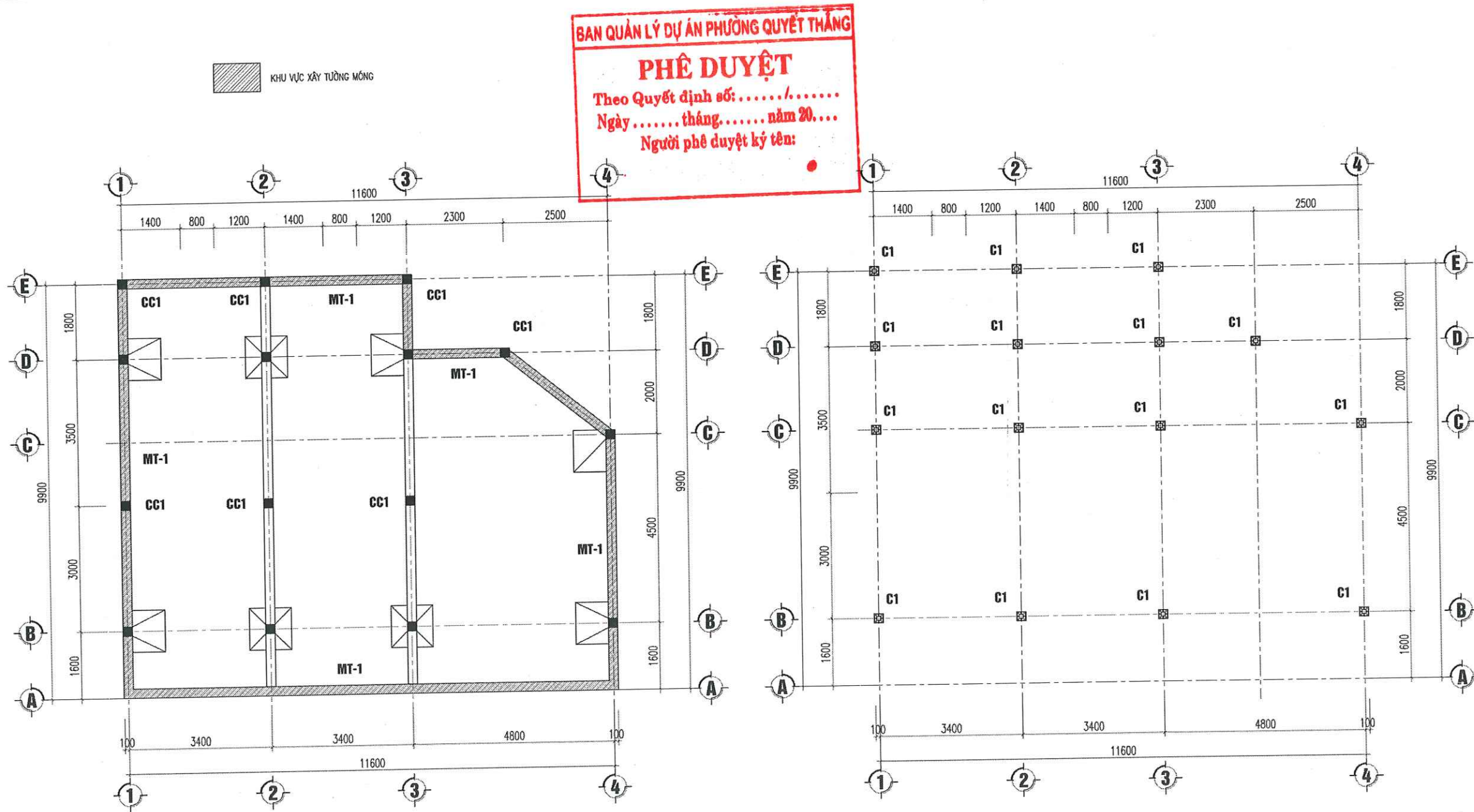
MẶT BẰNG ĐỊNH VỊ CỘT NHÀ A
