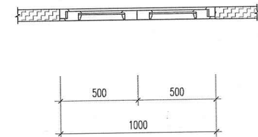
CẮT 2 - 2
