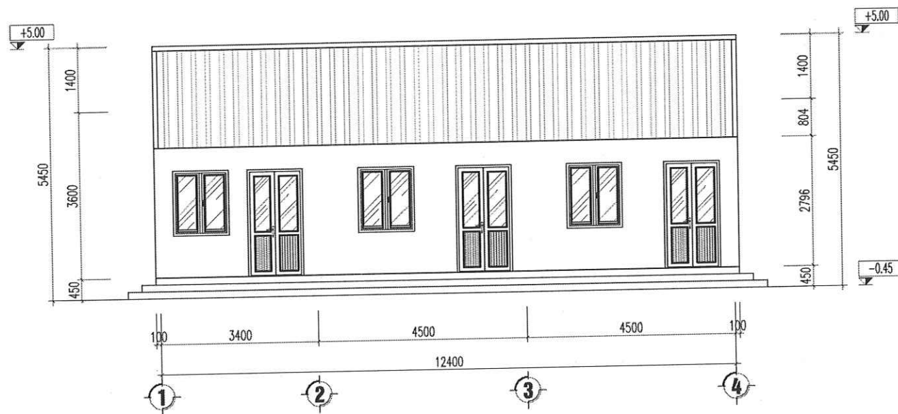
MẶT ĐỨNG TRỰC 1-4
