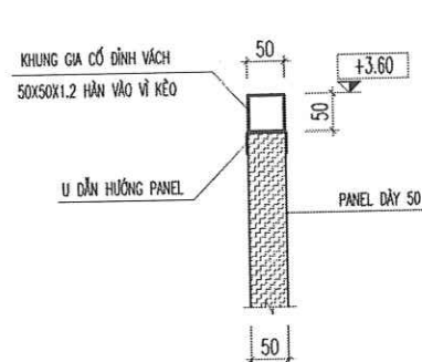
CHI TIẾT ĐÍNH VÁCH PANEL
