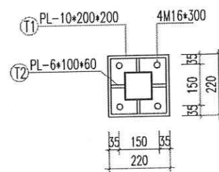
CẮT 1-1
