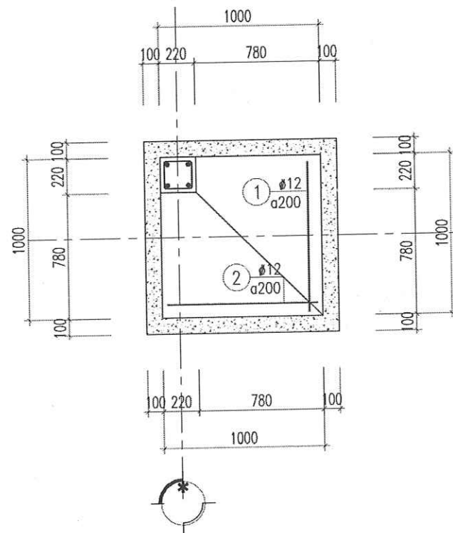
CHI TIẾT MÓNG DM3 (SỐ LƯỢNG= 02)
