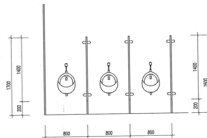
MẶT ĐÚNG VÁCH NGĂN TIỂU
