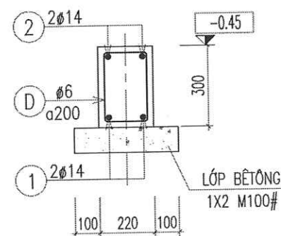
DẦM GM1 (SL= 02, L= 12.62M)
