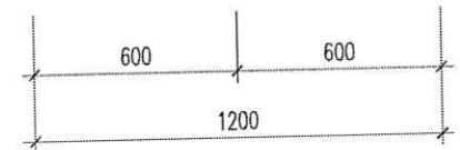
CẮT 2 - 2
