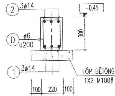
DẦM GM2 (SL= 04, L= 5.61M)
