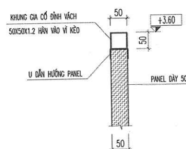
CHI TIẾT ĐỈNH VÁCH PANEL
