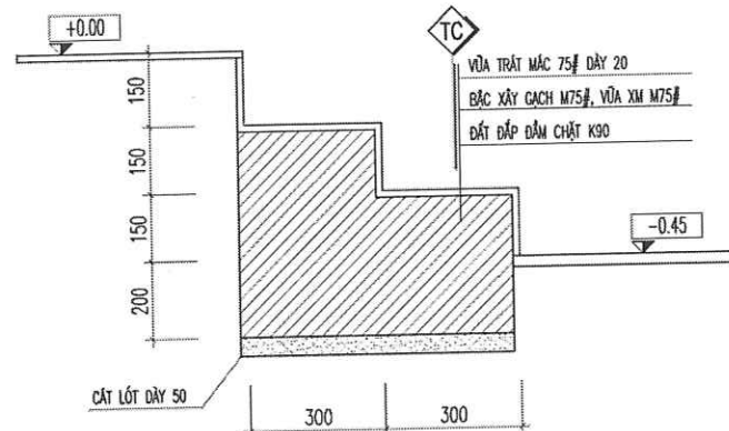
MẶT CẮT TAM CẤP (L= 24.7M)
