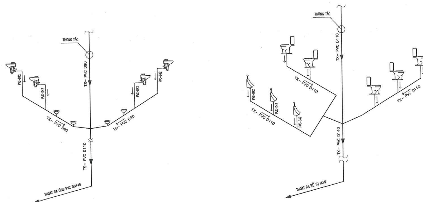
SƠ ĐỒ NGUYÊN LÝ THOÁT NƯỚC
