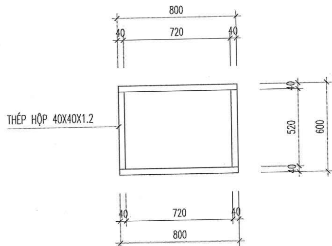
MẶT BẰNG KHUNG ĐỖ BÀN ĐÁ (SL= 02 BỘ)
