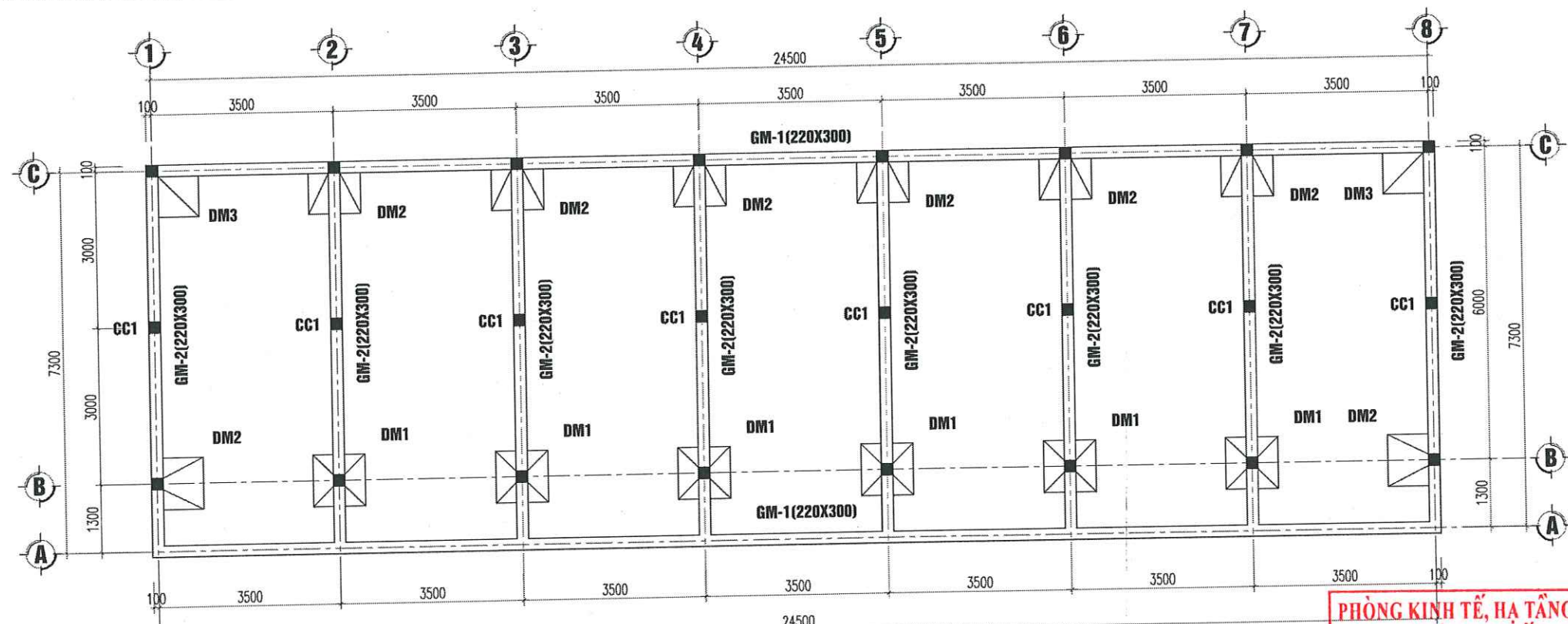
MẶT BẰNG MÓNG NHÀ C
