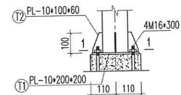
CHI TIẾT CHÂN CỘT C1
