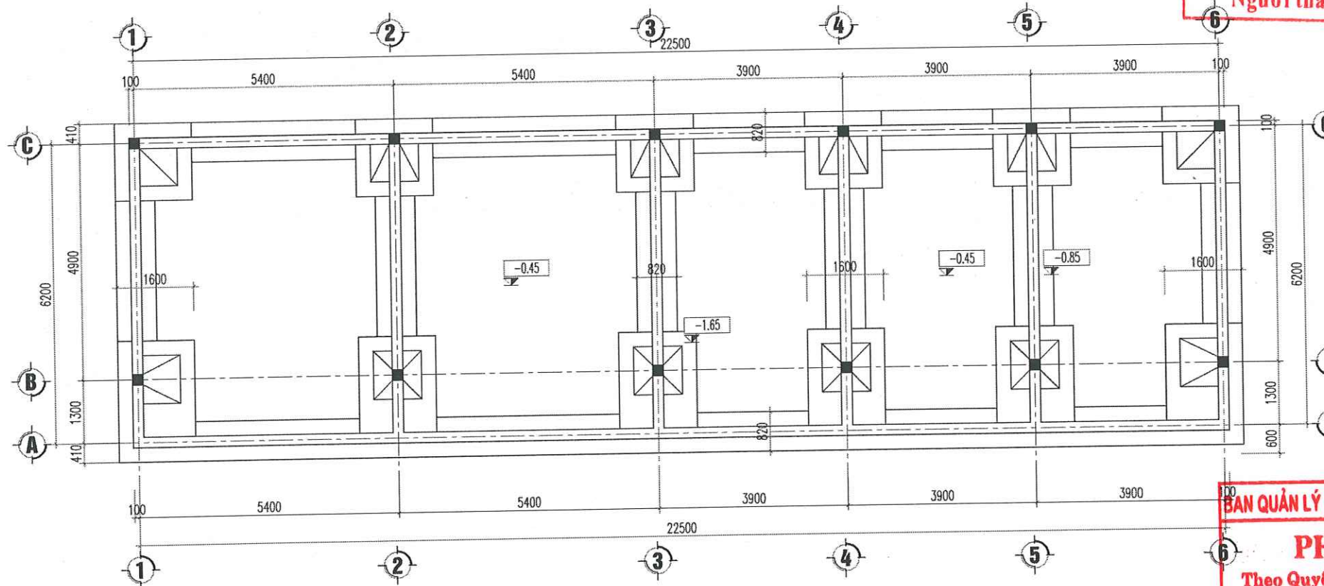
MẶT BẰNG ĐỊNH HƯỚNG ĐÀO MÓNG NHÀ E
