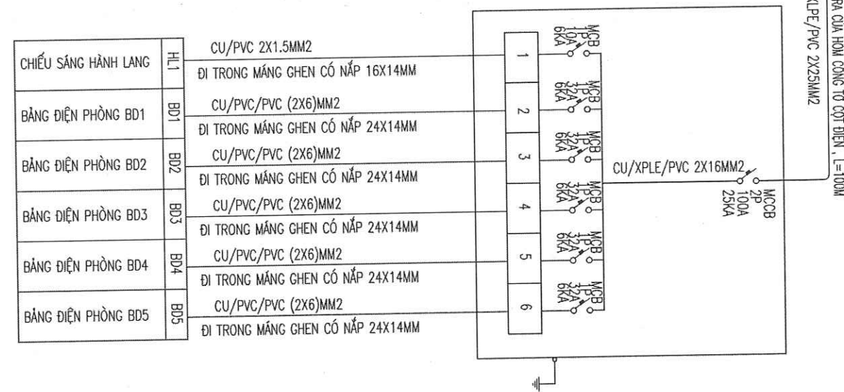
SƠ ĐỒ TỬ ĐIỆN TỔNG
