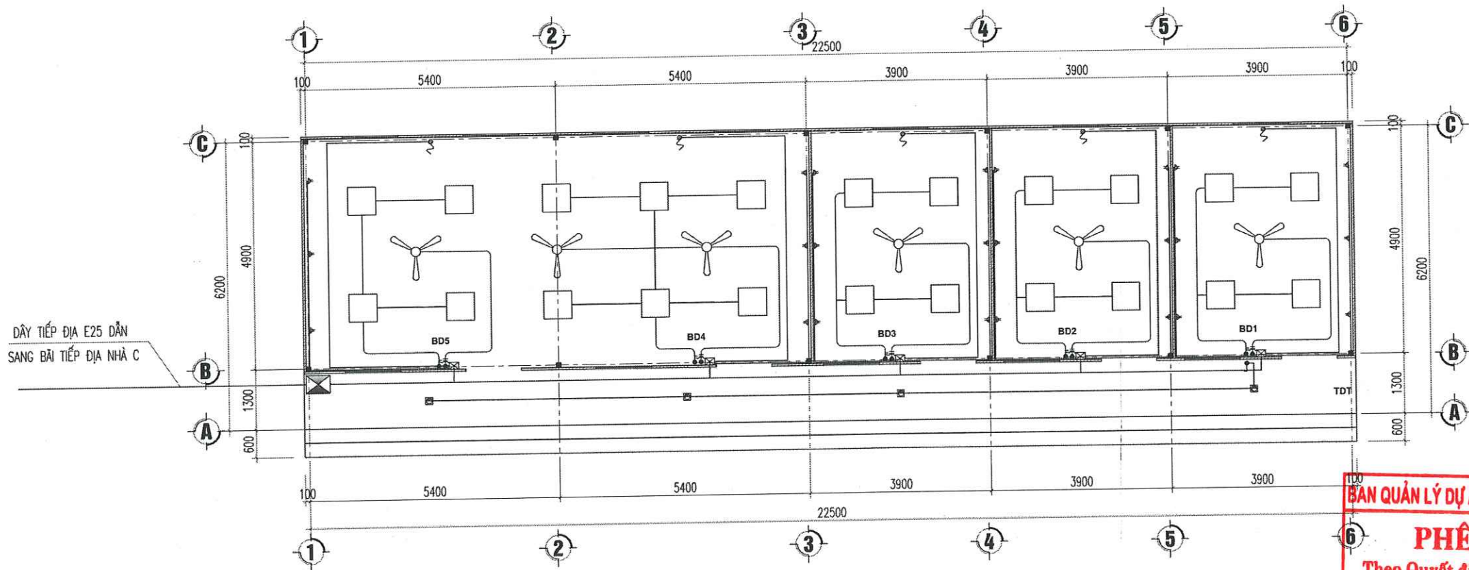
MẶT BẰNG CẤP ĐIỆN NHÀ E
