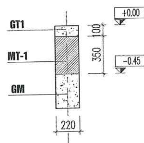
MẶT CẮT MT1 (L=56.02M)
