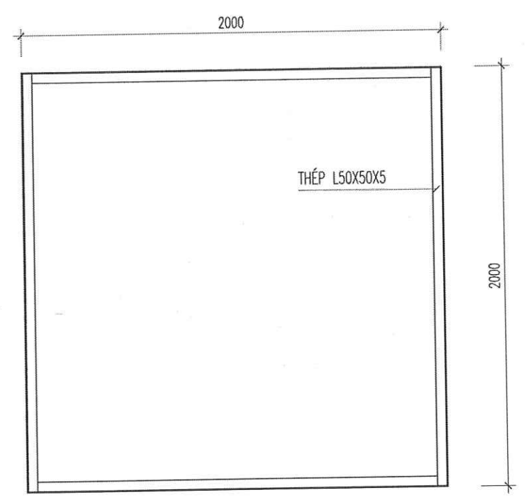
CHÂN KHUNG ĐỒ TẾC NƯỚC
