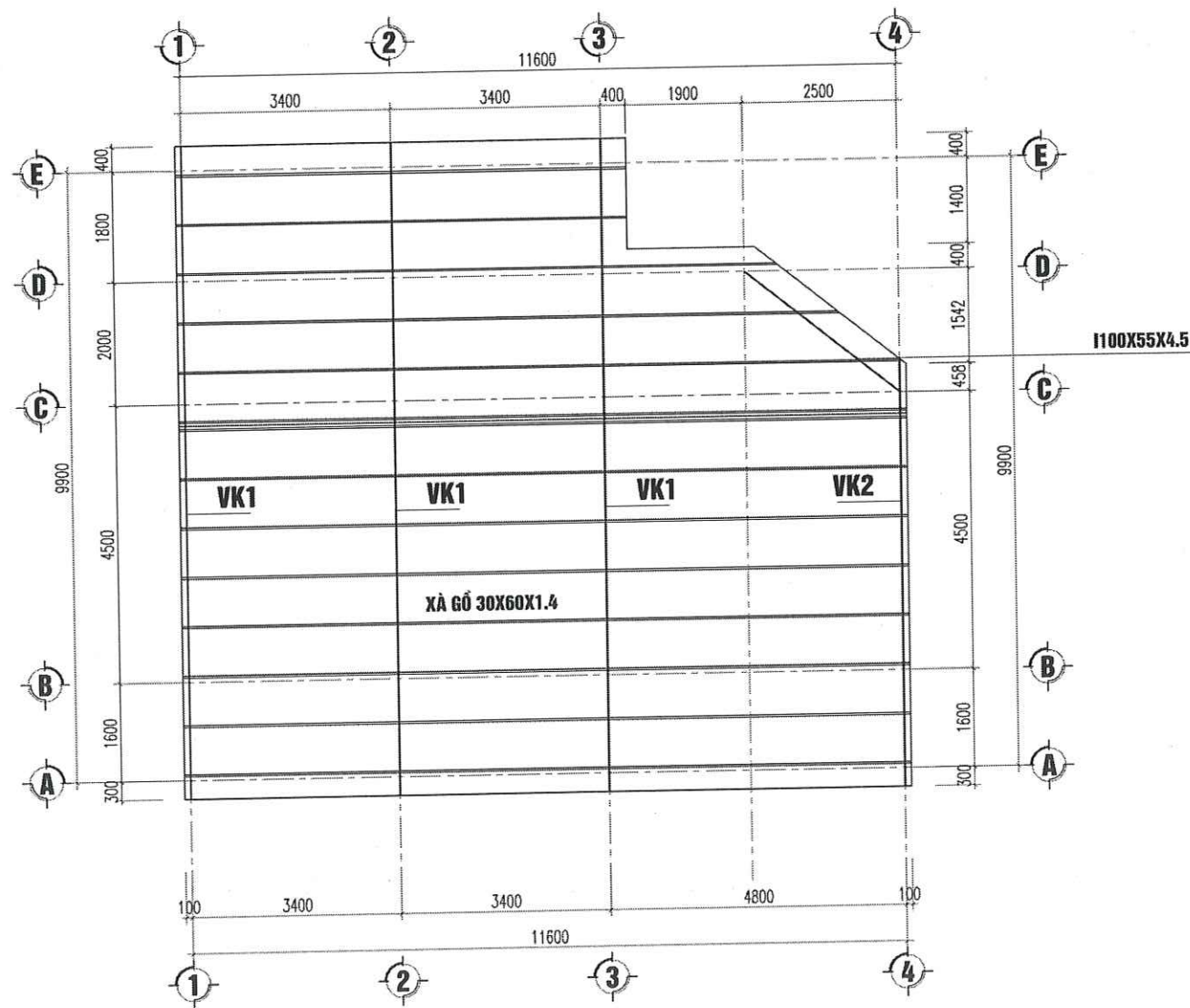
MẶT BẰNG VÌ KÈO+ XÀ GỖ NHÀ A
