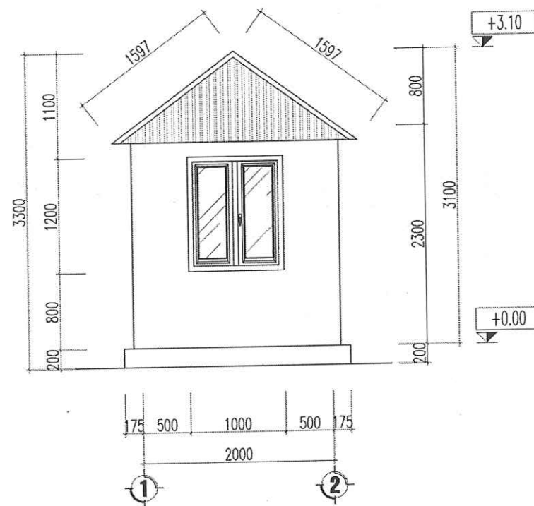
MẶT ĐỨNG 1-2
