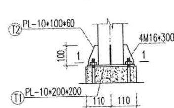
CHI TIẾT CHÂN CỘT C1
