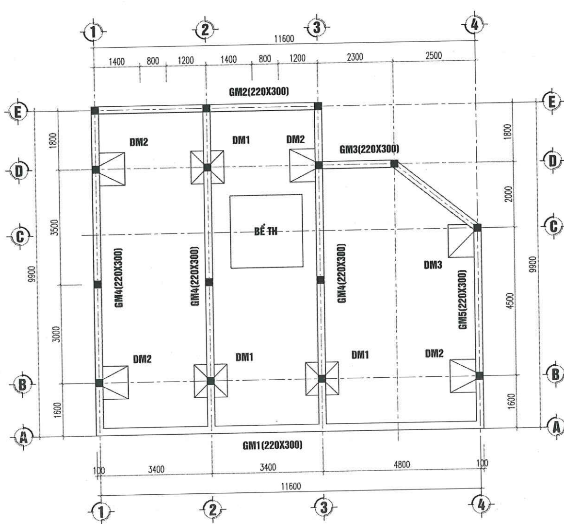
MẶT BẰNG MÓNG NHÀ A
