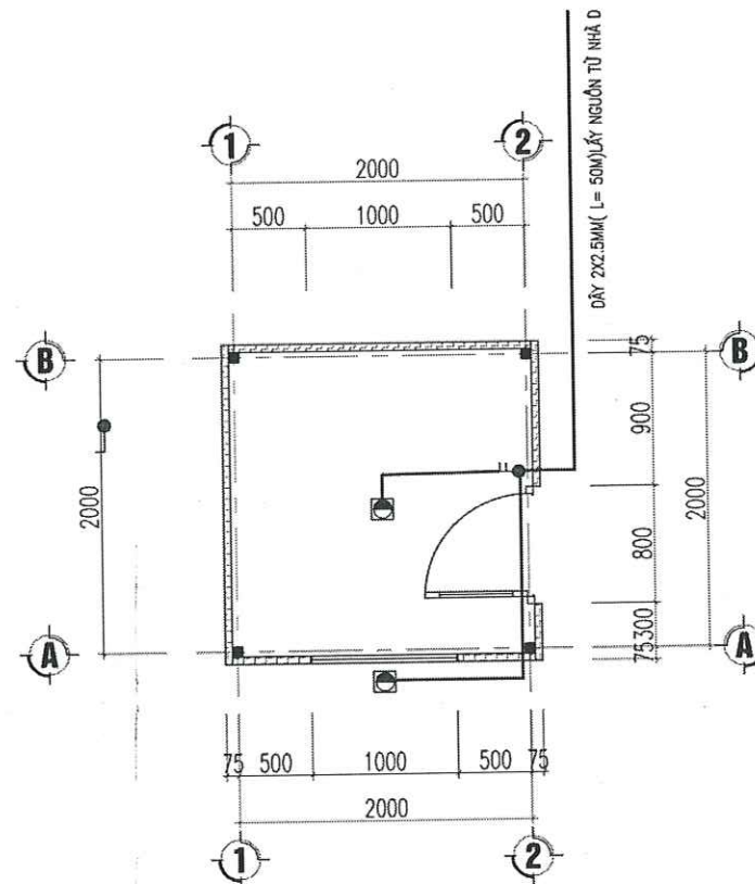
MẶT BẰNG ĐIỆN NHÀ BẢO VỆ
