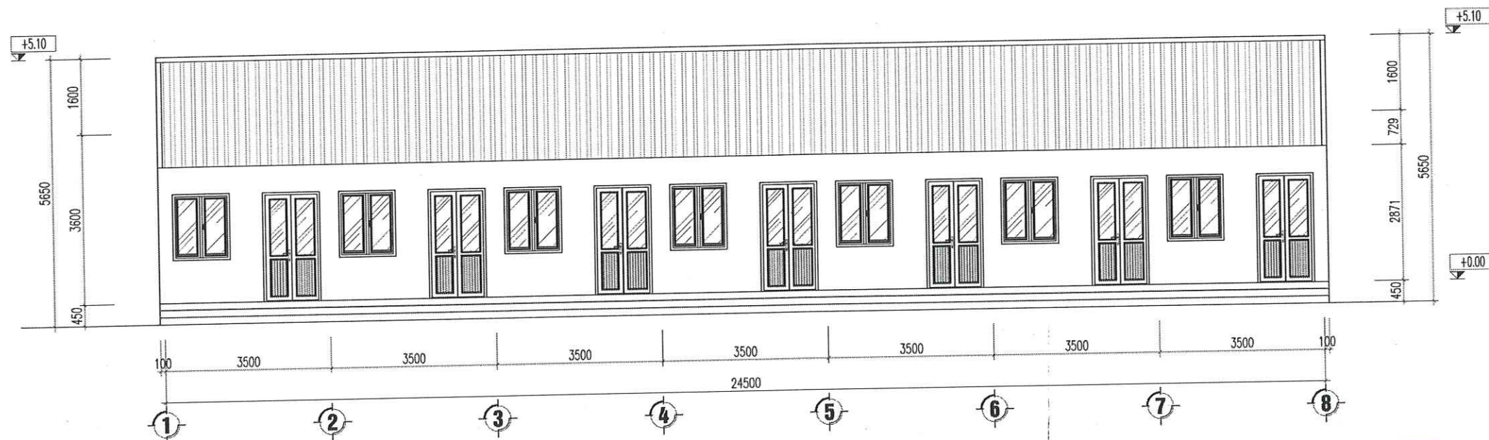
MẶT ĐỨNG TRỰC 1-8
