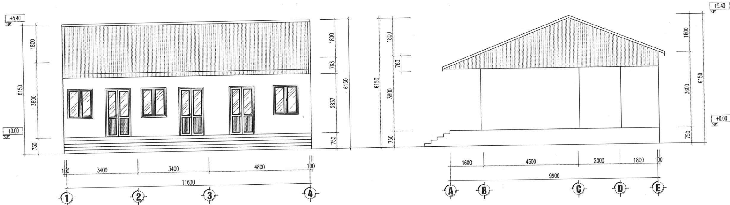
MẶT ĐỨNG TRỰC A-E
