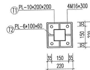
CẮT 1-1
