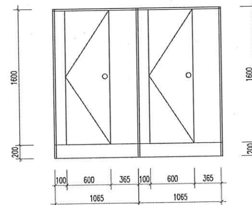
MẶT ĐÚNG VÁCH NGĂN WC NAM
