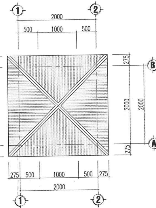
MẶT BẰNG MÁI NHÀ BẢO VỆ
