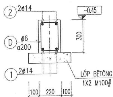
DẦM GM1 (SL= 02, L= 23.02M)
