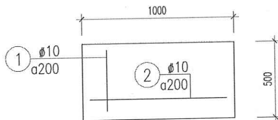
THÉP TẮM ĐẠN NẮP BỂ TỰ HOẠI (SL= 08)
