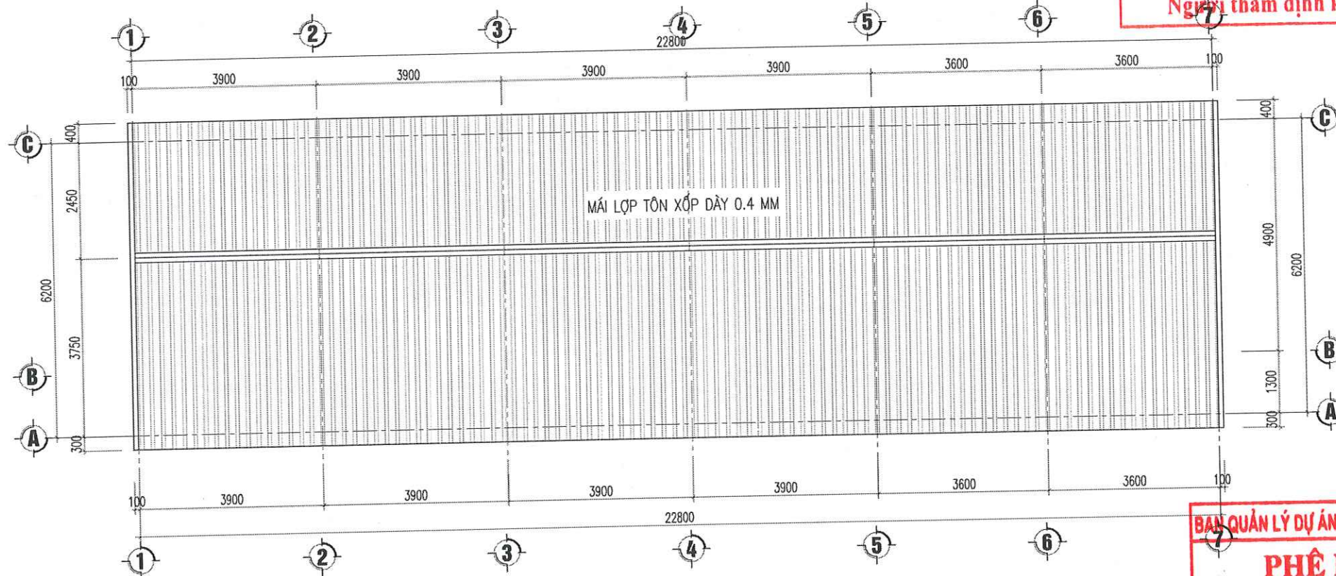
MẶT BẰNG MÁI NHÀ D
