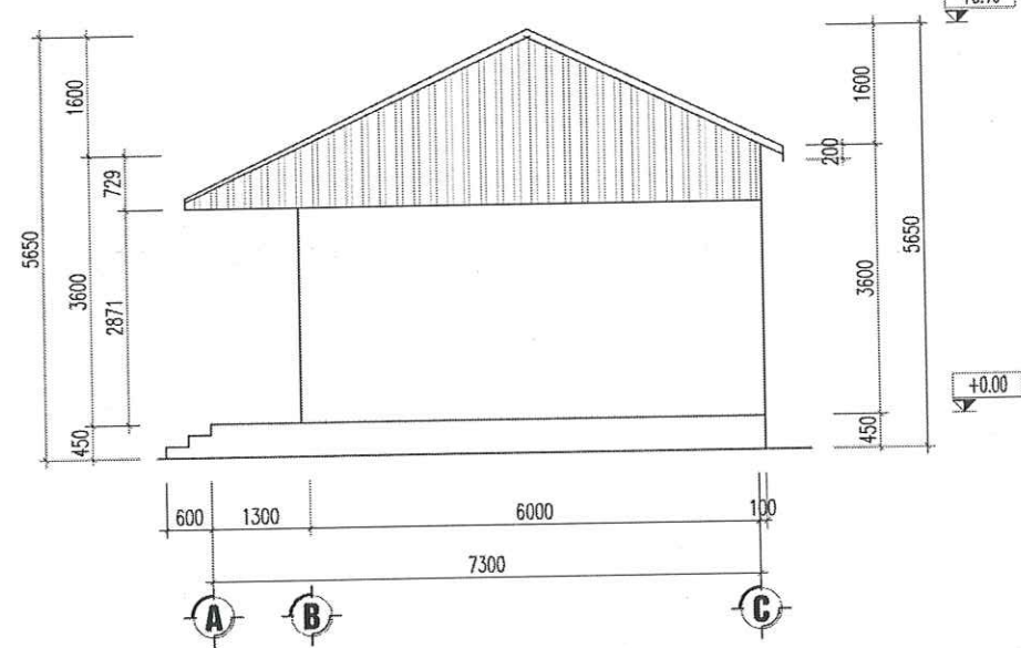
MẶT ĐỨNG TRỰC A-C
