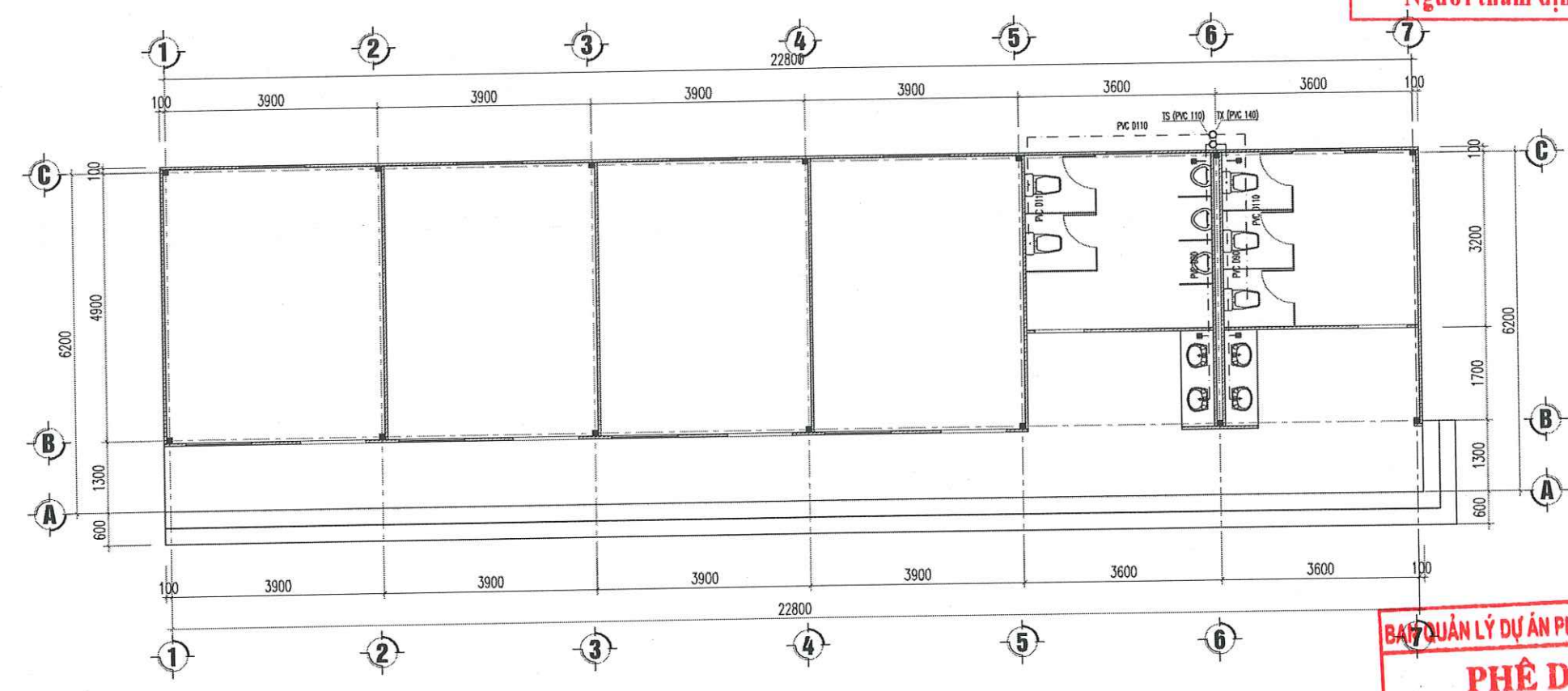
MẶT BẰNG THOÁT NƯỚC NHÀ D
