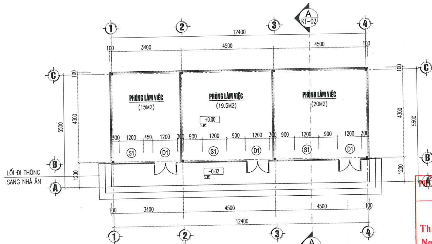
MẶT BẰNG NHÀ B
