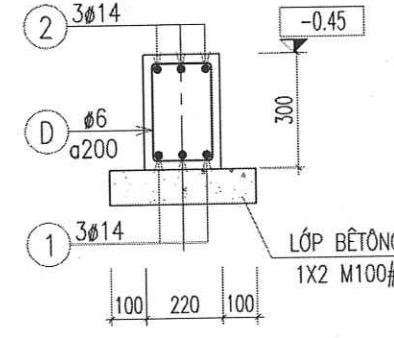
DẦM GM2 (SL= 07, L= 6.42M)
