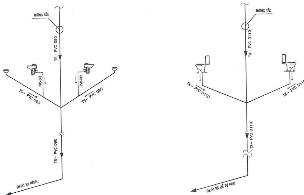
SƠ ĐỒ NGUYÊN LÝ THOÁT NƯỚC
