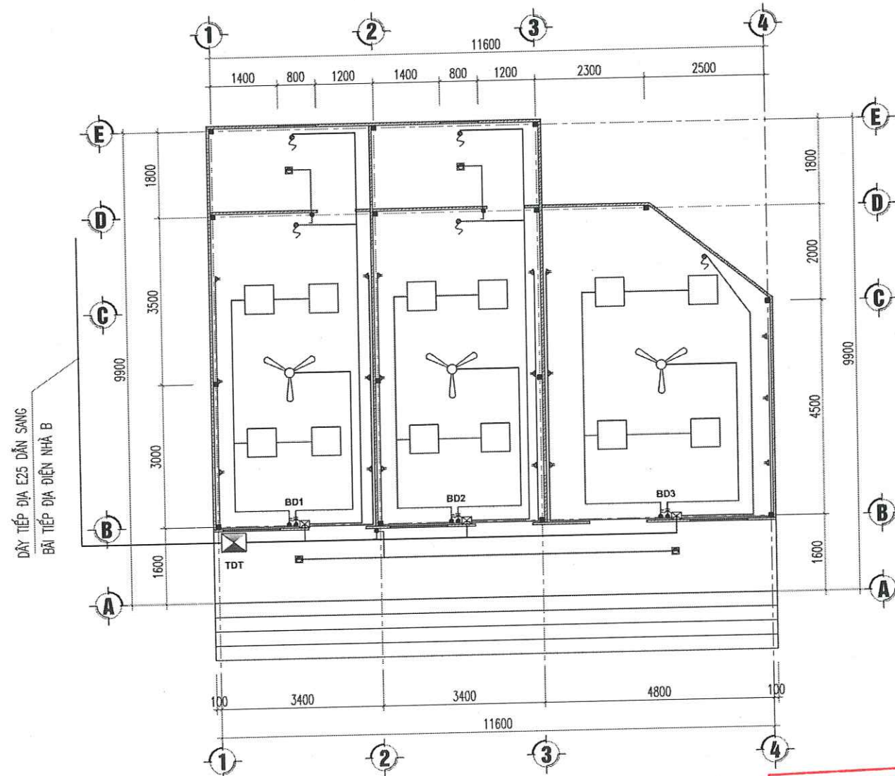
MẶT BẰNG ĐIỆN NHÀ A
