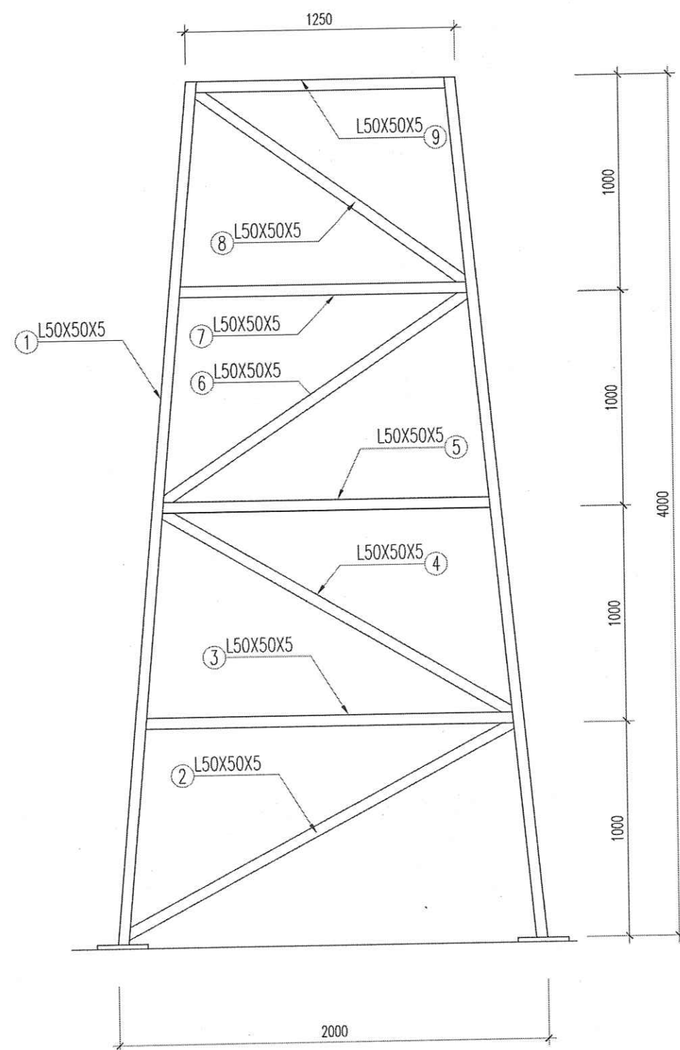
MẶT ĐỨNG KHUNG ĐỖ TẾC NƯỚC (SL= 01 BỘ)
