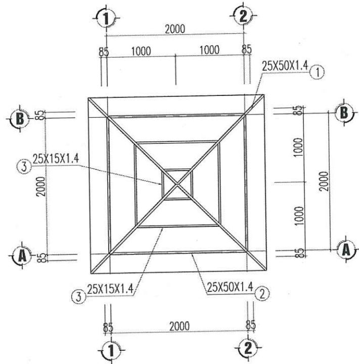
MẶT BẰNG KHUNG NHÀ BẢO VỆ
