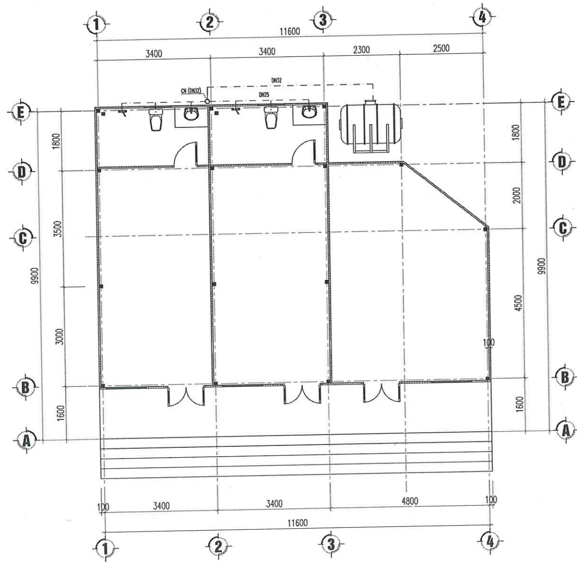
MẶT BẰNG CẤP NƯỚC NHÀ A
