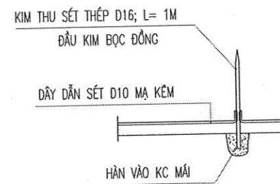
KIM THU SÉT (SỐ LƯỢNG= 04)
