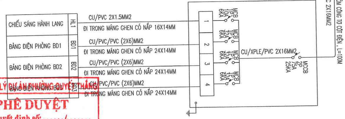
SƠ ĐỒ TỦ ĐIỆN TỔNG
