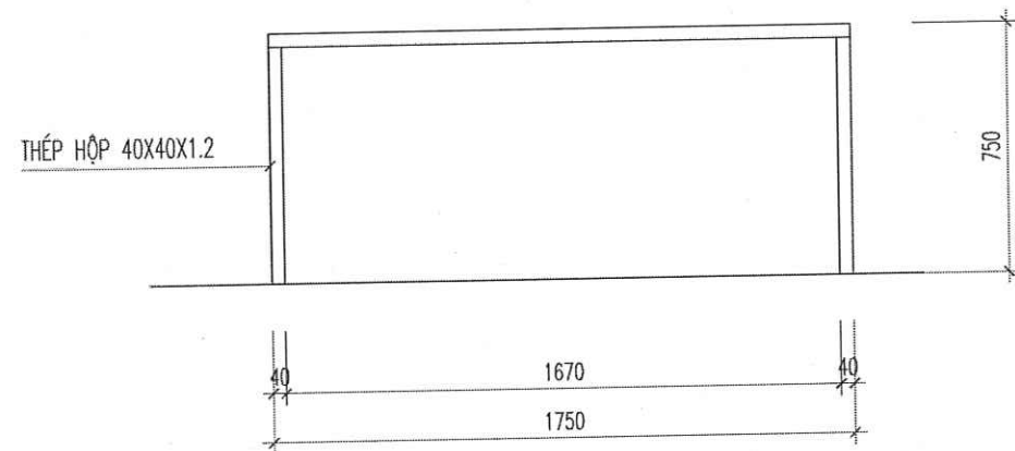
MẶT ĐỨNG KHUNG ĐỖ BÀN ĐÁ (SL= 02 CÁI)
