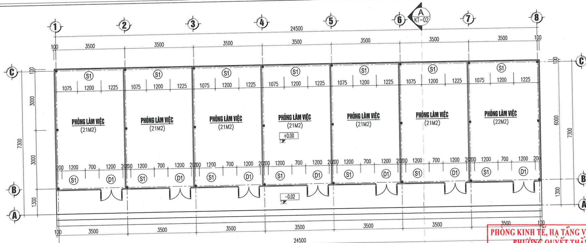
MẶT BẰNG NHÀ C
