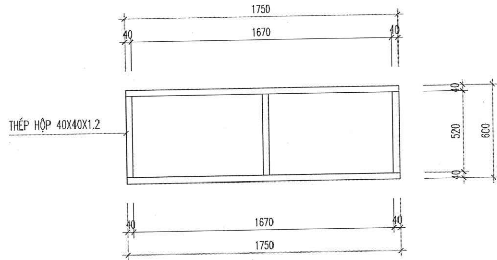
MẶT BẰNG KHUNG ĐỖ BÀN ĐÁ (SL= 02 CÁI)
