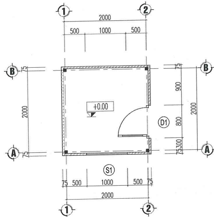
MẶT BẰNG NHÀ BẢO VỆ
