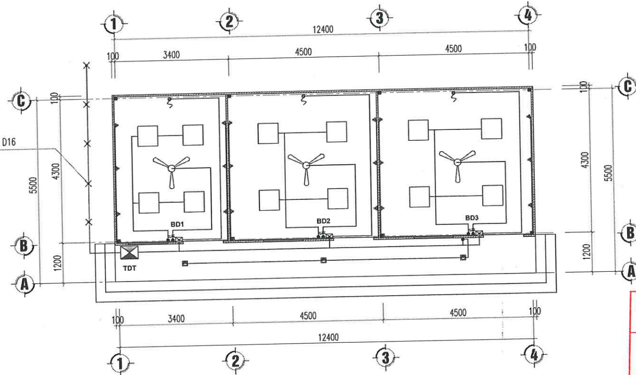
MẶT BẰNG CẤP ĐIỆN NHÀ B
