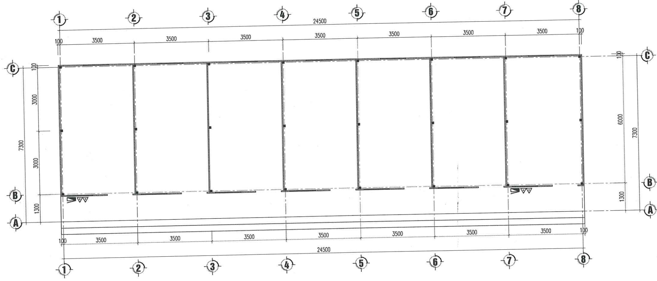
MẶT BẰNG PCCC TẠI CHỖ
