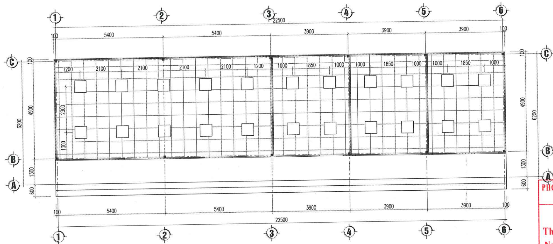
MẶT BẰNG TRẦN ĐÈN NHÀ E
