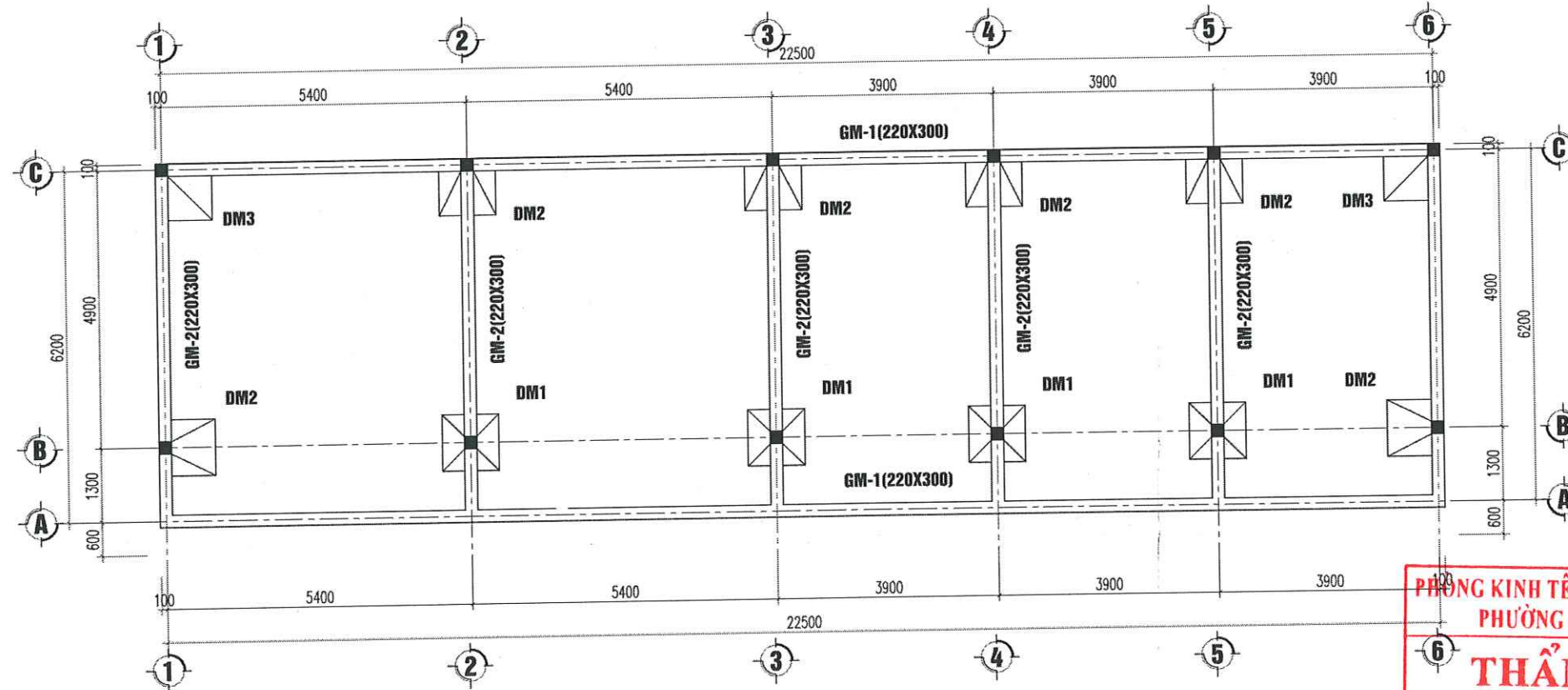
MẶT BẰNG MÓNG NHÀ E
