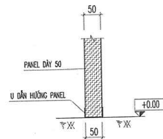
CHI TIẾT CHÂN VÁCH PANEL
