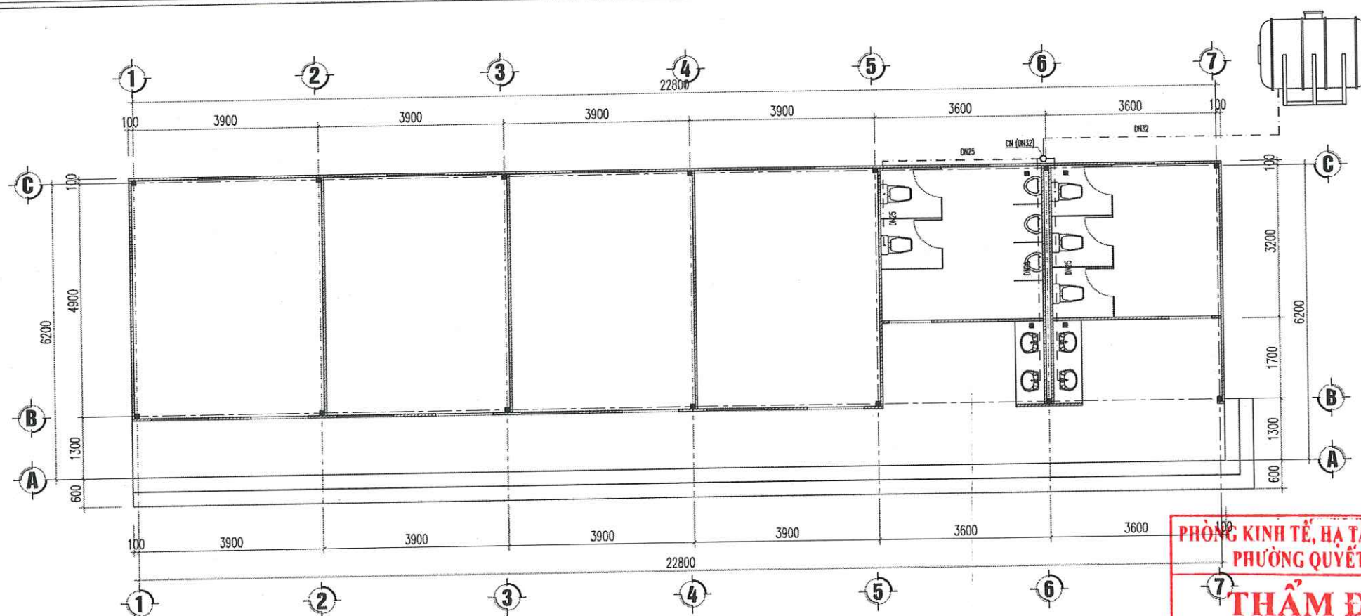
MẶT BẰNG CẤP NƯỚC NHÀ D
