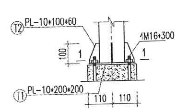
CHI TIẾT CHÂN CỘT C1
