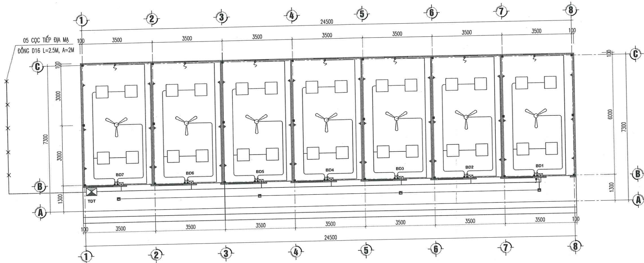
MẶT BẰNG CẤP ĐIỆN NHÀ C
