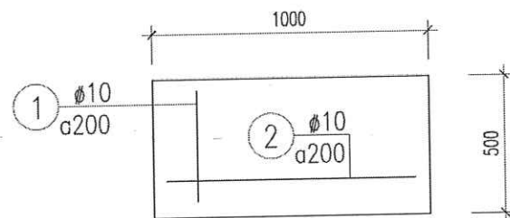
THÉP TẮM ĐAN NẮP BỂ TỰ HOẠI (SL= 08 BỘ)
