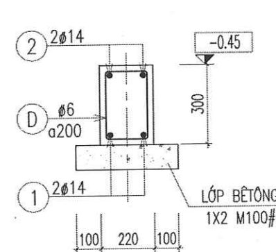
DẦM GM1 (SL= 02, L= 22.72M)
