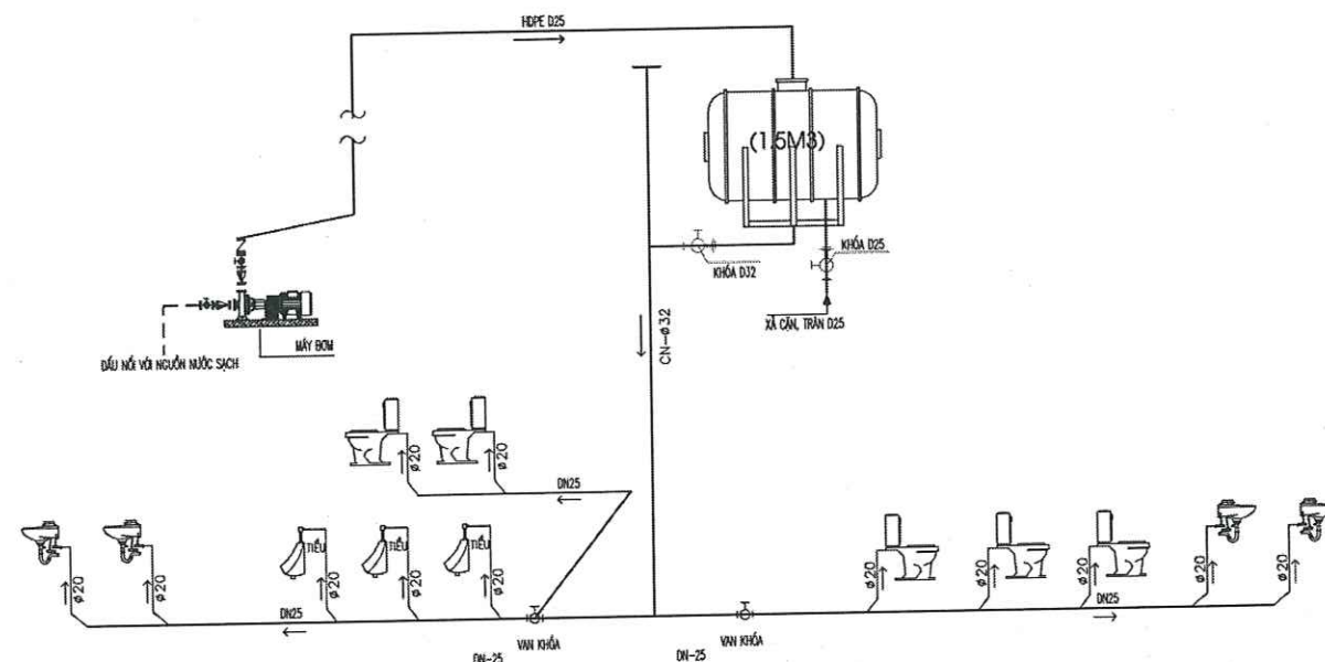
SƠ ĐỒ NGUYÊN LÝ CẤP NƯỚC
