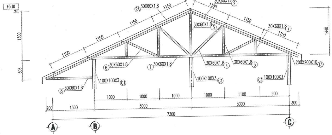
CHI TIẾT VÌ KÈO VK1 (SỐ LƯỢNG=08)
