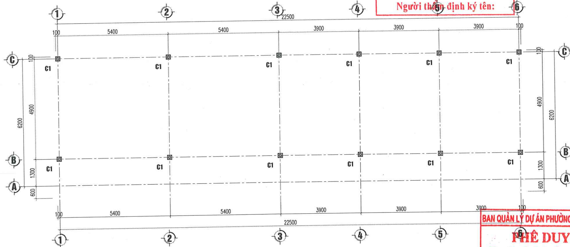
MẶT BẰNG ĐỊNH VỊ CỘT NHÀ E
