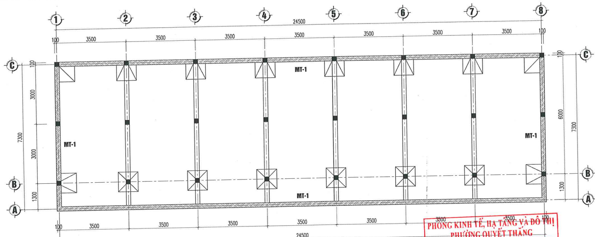
MẶT BẰNG XÂY TƯỜNG MÓNG NHÀ C
