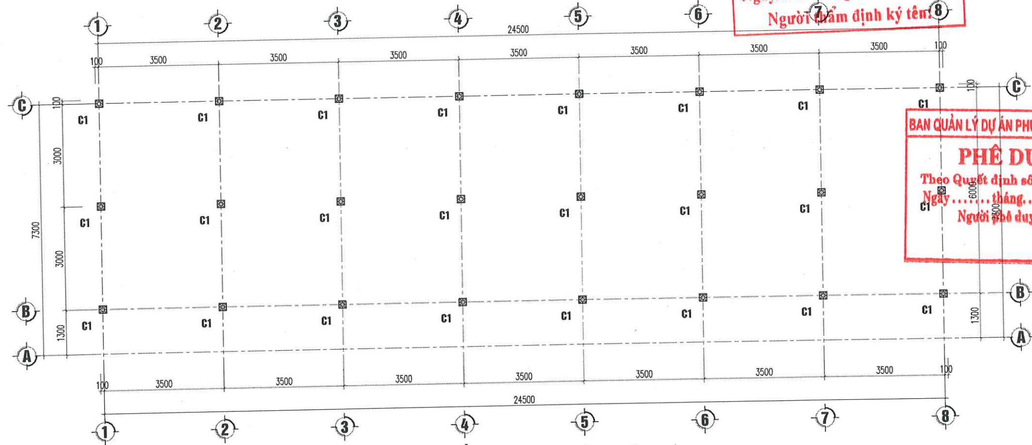
MẶT BẰNG ĐỊNH VỊ CỘT NHÀ C
