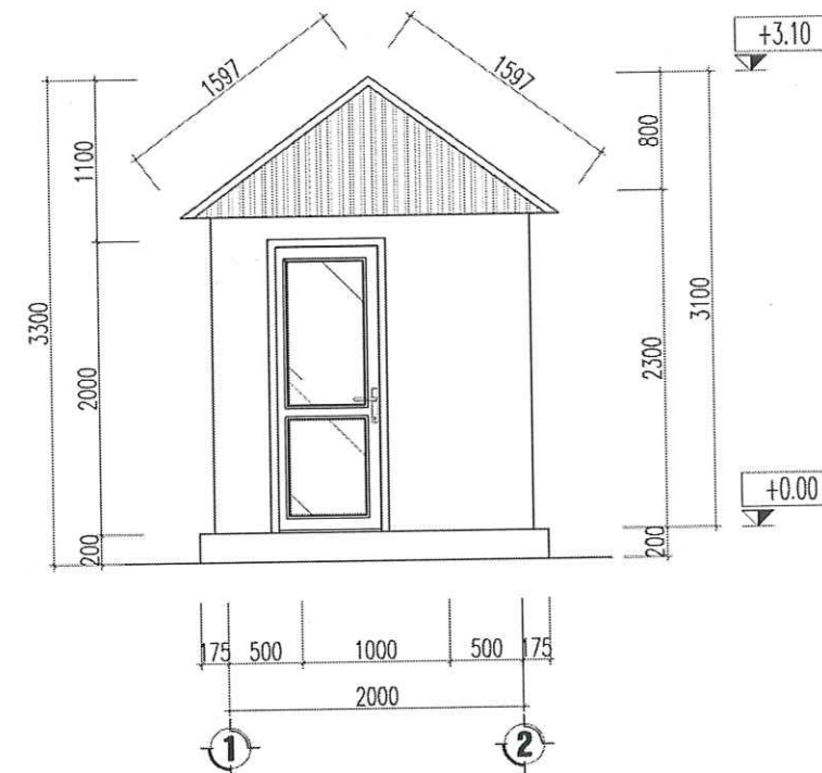
MẶT ĐỨNG A-B
