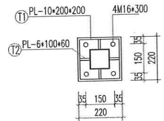
CẮT 1-1
