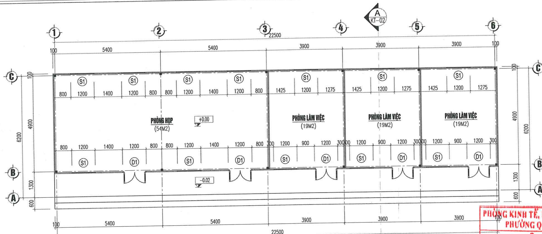
MẶT BẰNG NHÀ E
