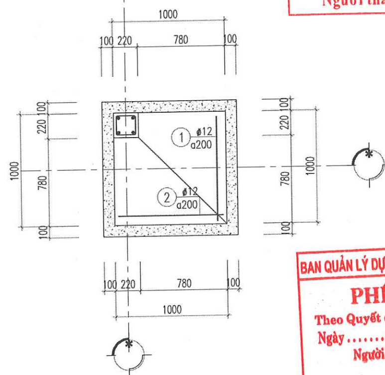
CHI TIẾT MÓNG DM3 (SỐ LƯỢNG= 02)
