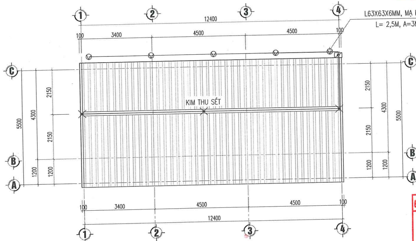
MẶT BẰNG TIẾP ĐỊA NHÀ B
