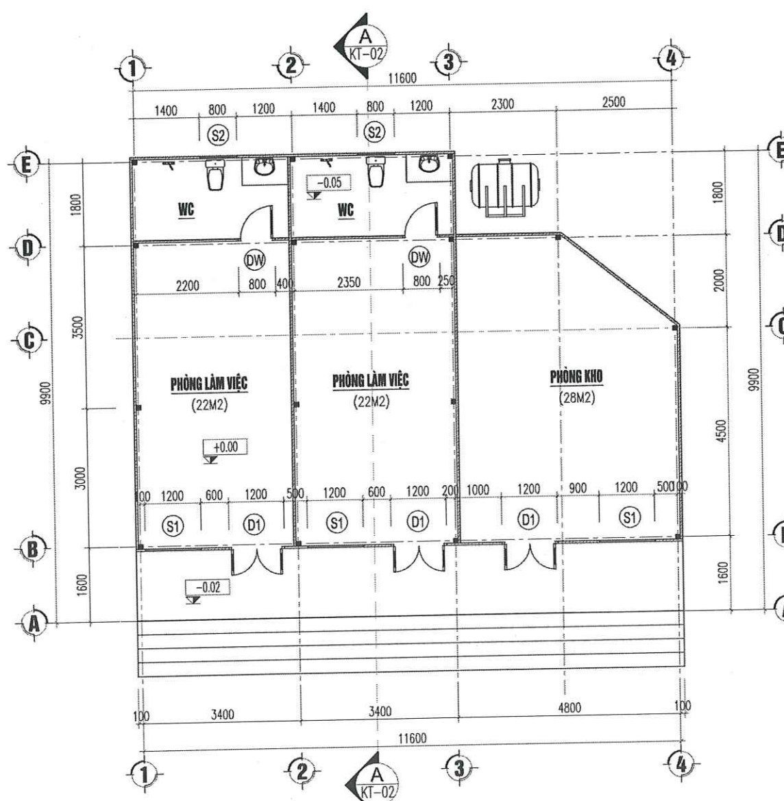
MẶT BẰNG NHÀ A
