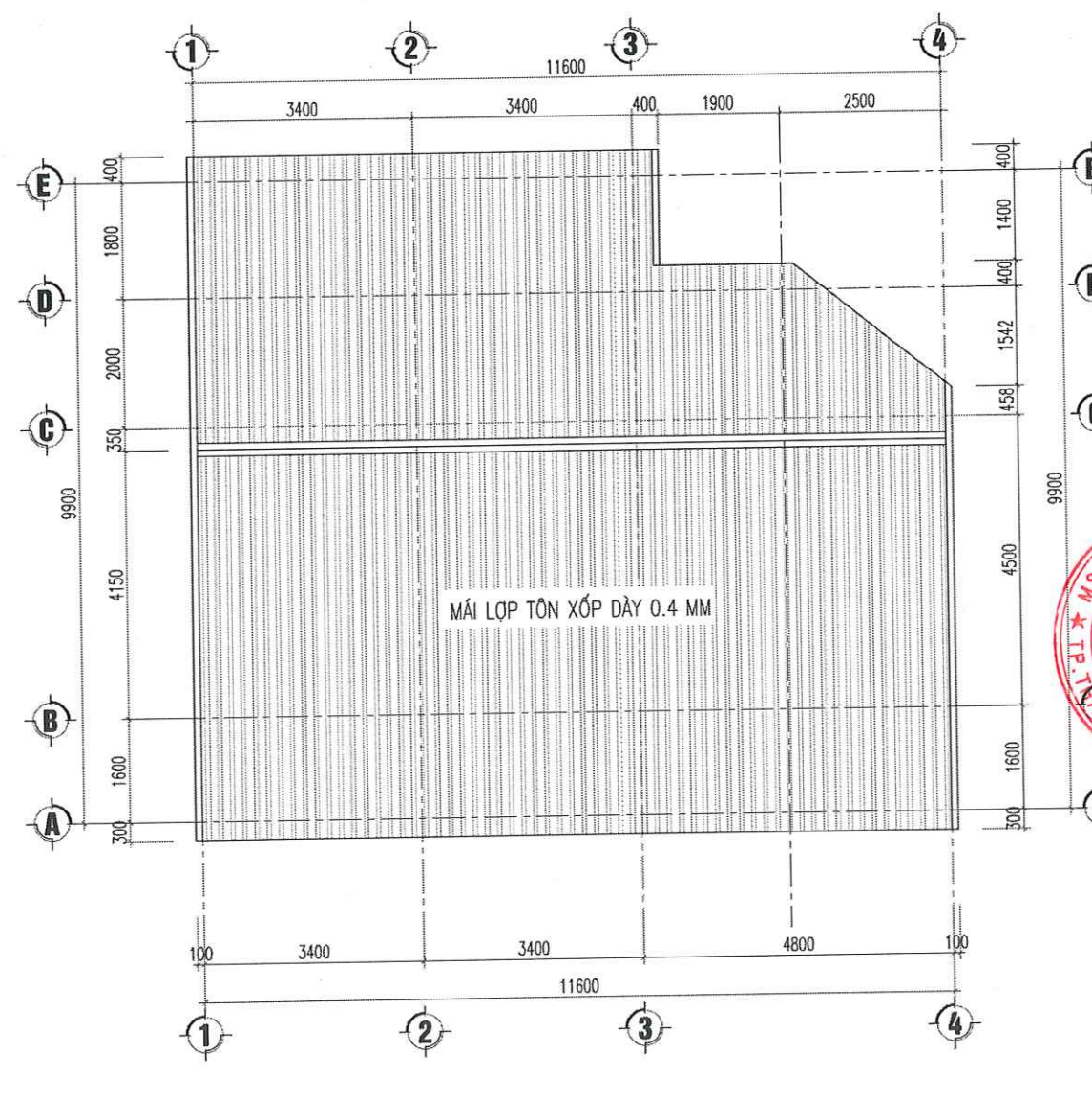
MẶT BẰNG MÁI NHÀ A
