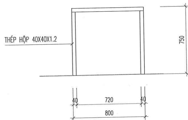
MẶT ĐỨNG KHUNG ĐỖ BÀN ĐÁ (SL= 02 BỘ)
