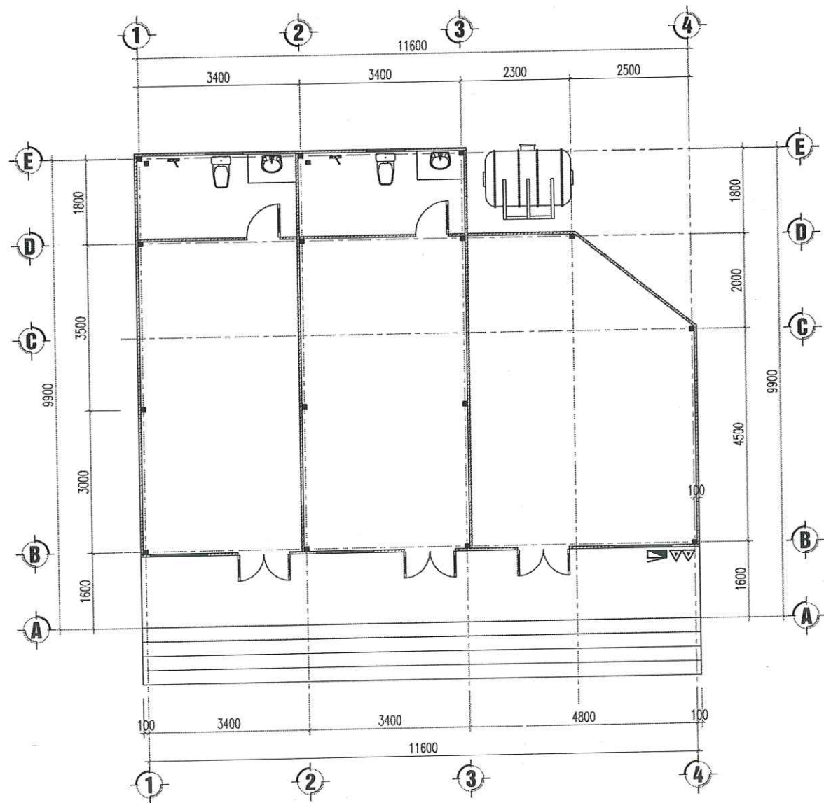
MẶT BẰNG PCCC TẠI CHỖ
