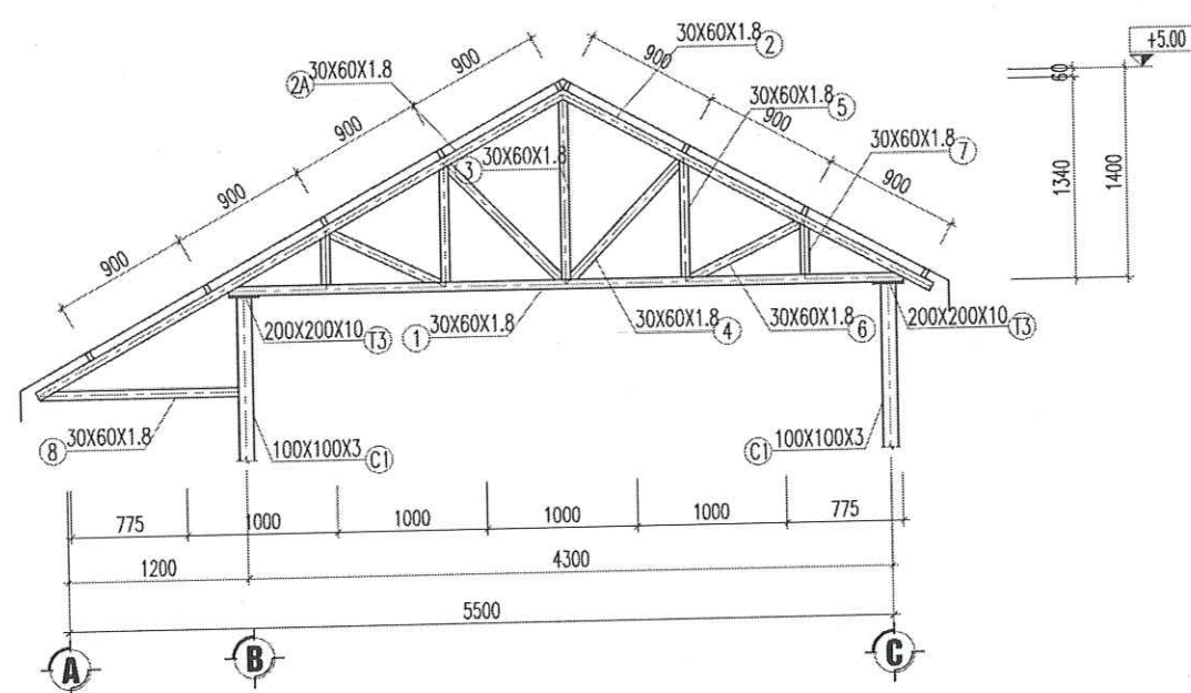
CHI TIẾT VÌ KÈO VK1
