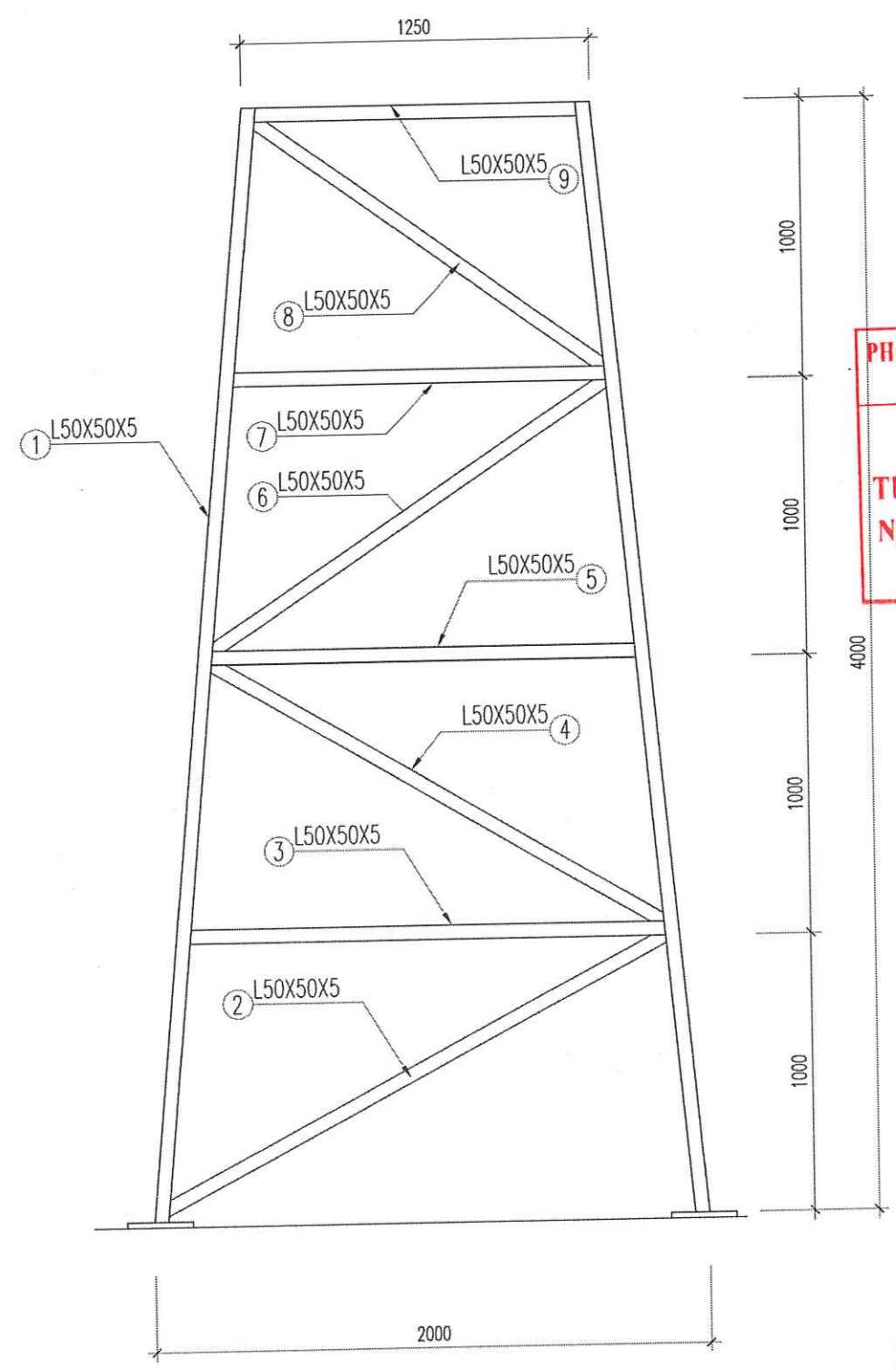
MẶT ĐỨNG KHUNG ĐỒ TẾC NƯỚC (SL= 01 BỘ)
