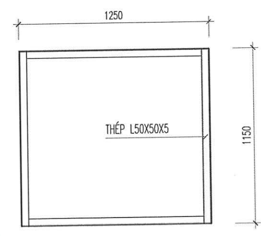
ĐỈNH KHUNG ĐỒ TẾC NƯỚC
