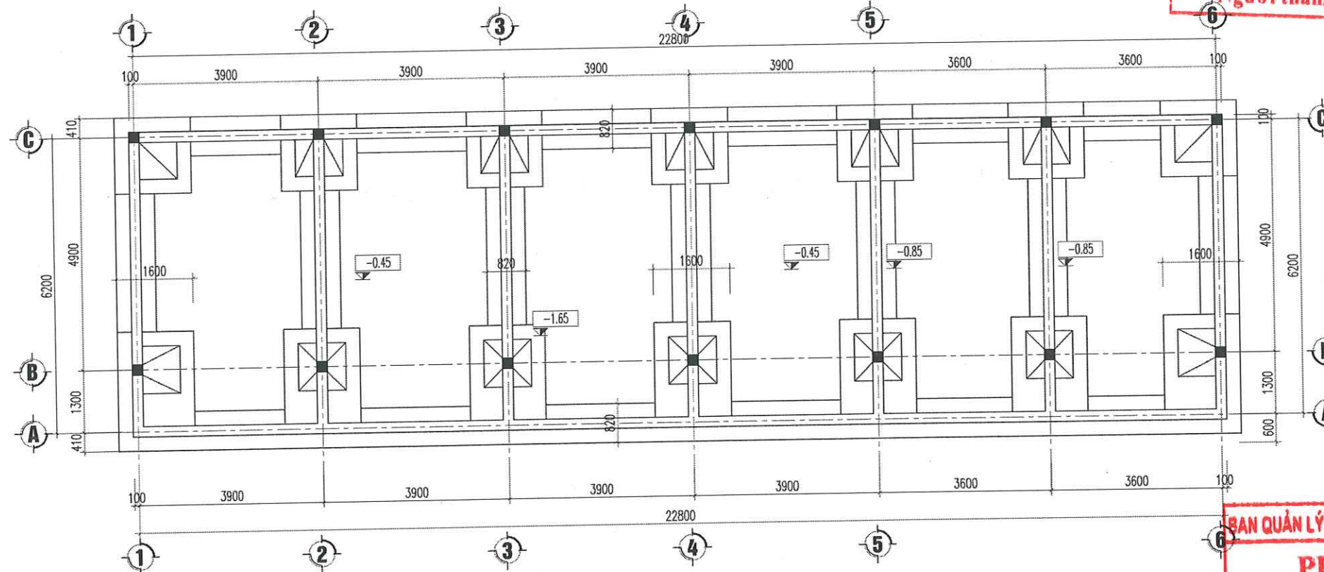
MẶT BẰNG ĐỊNH HƯỚNG ĐÀO MÓNG NHÀ D
