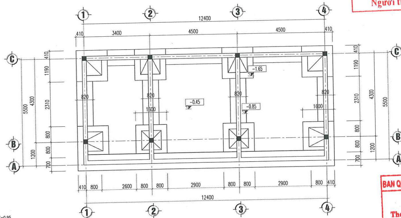
MẶT BẰNG ĐỊNH HƯỚNG ĐÀO MÓNG NHÀ B
