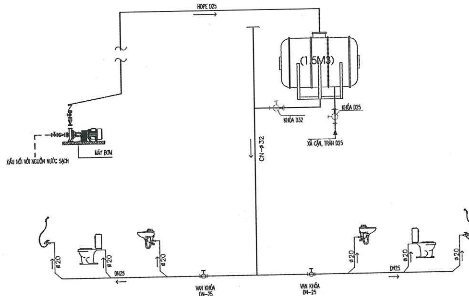
SƠ ĐỒ NGUYÊN LÝ CẤP NƯỚC
