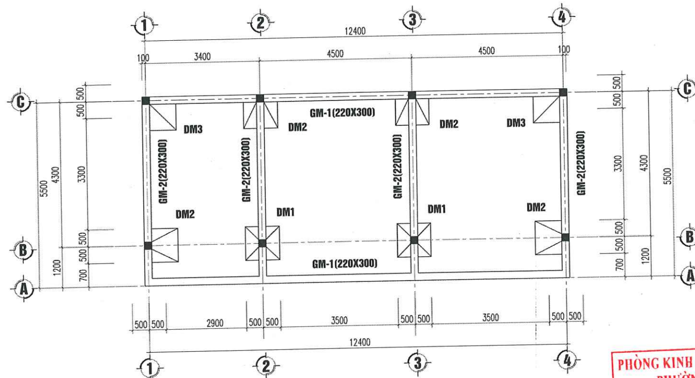
MẶT BẰNG MÓNG NHÀ B
