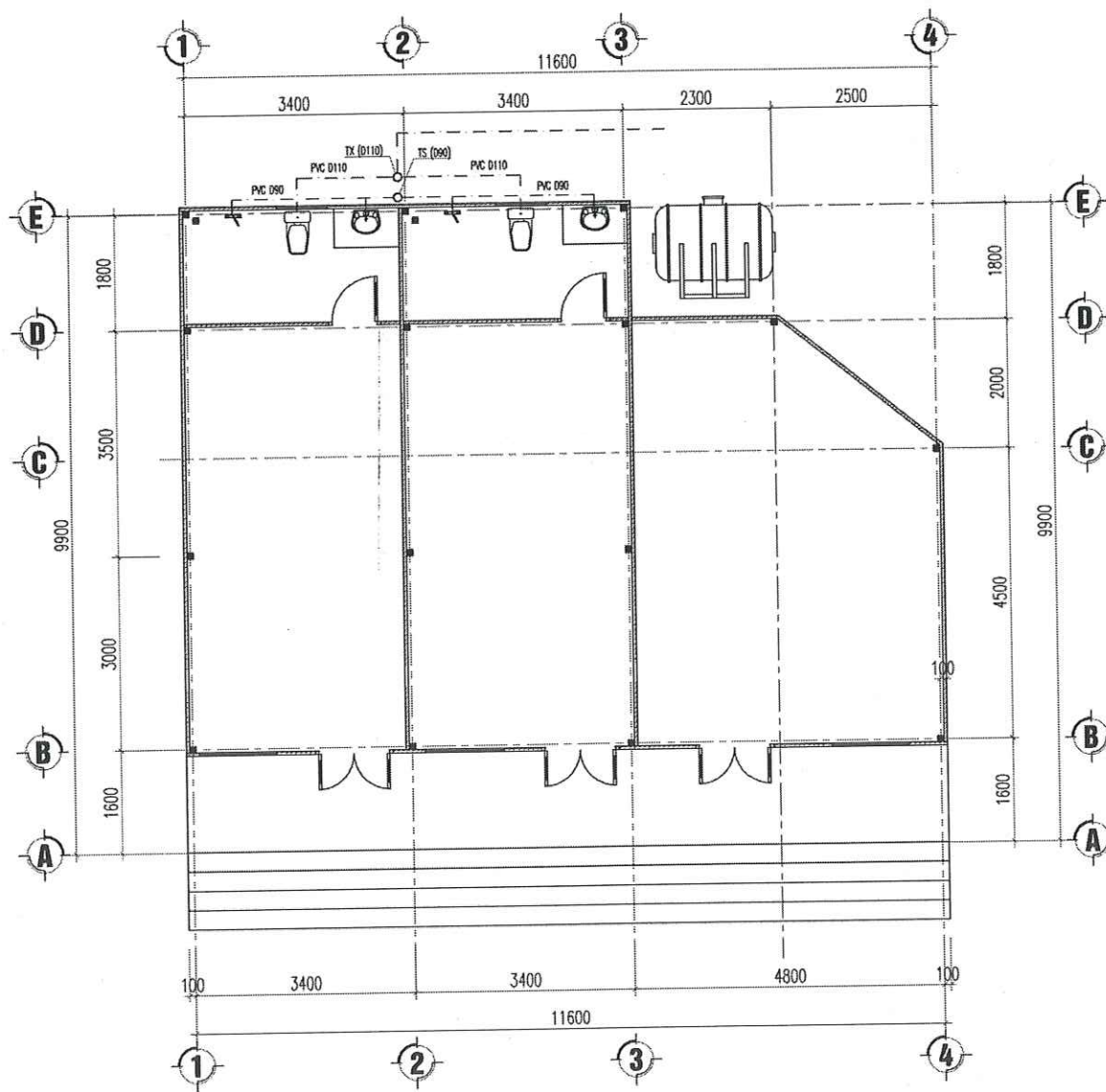
MẶT BẰNG THOÁT NƯỚC NHÀ A
