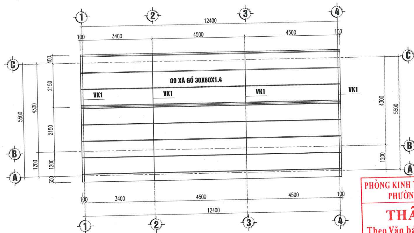
MẶT BẰNG VÌ KÈO+ XÀ GỖ NHÀ B
