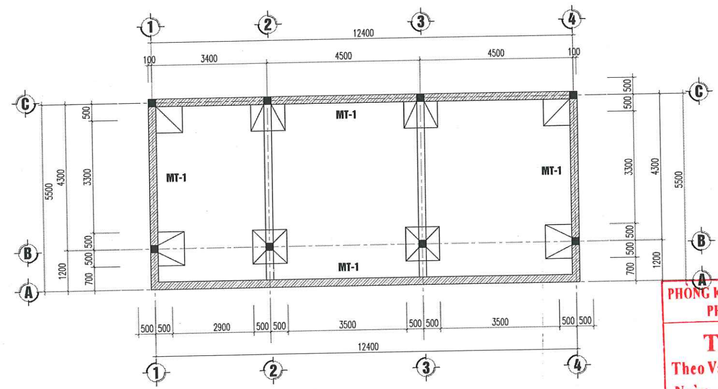
MẶT BẰNG XÂY MÓNG NHÀ B
