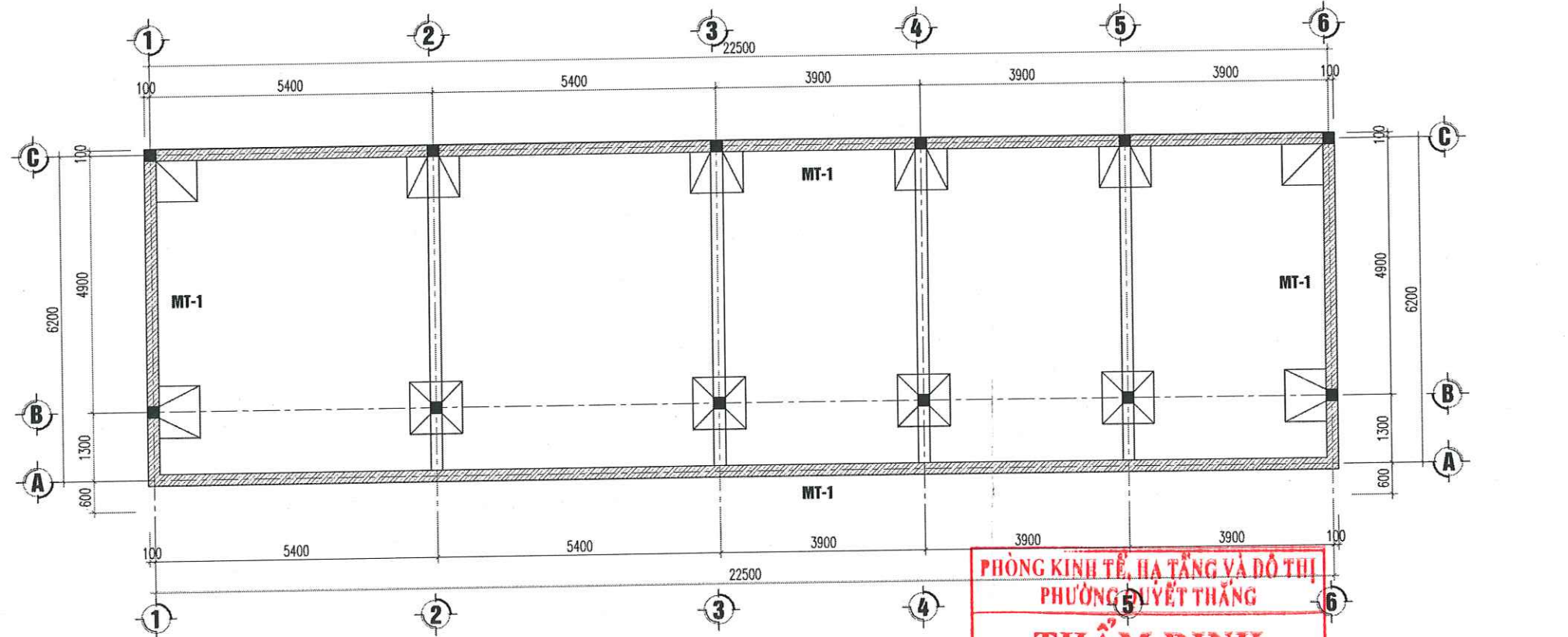
MẶT BẰNG XÂY TƯỜNG MÓNG NHÀ E
