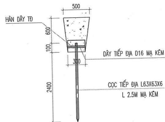
CỌC TIẾP ĐỊA (SỐ LƯỢNG= 08)
