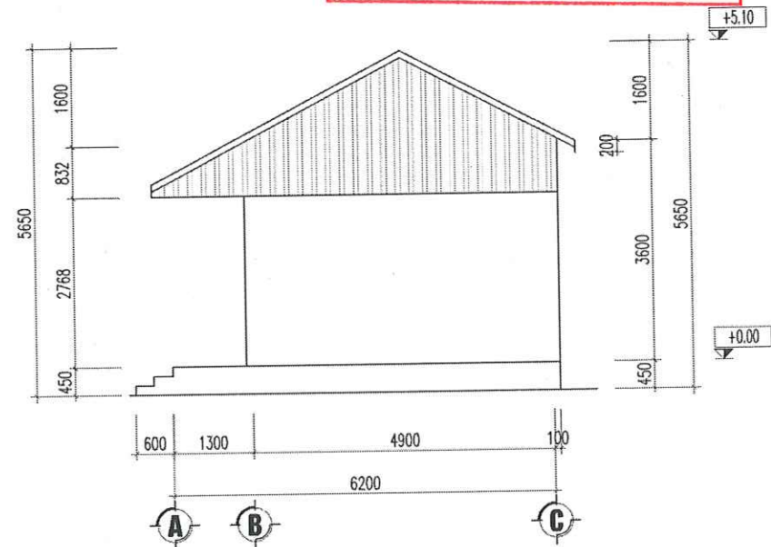
MẶT ĐỨNG TRỰC A-C
