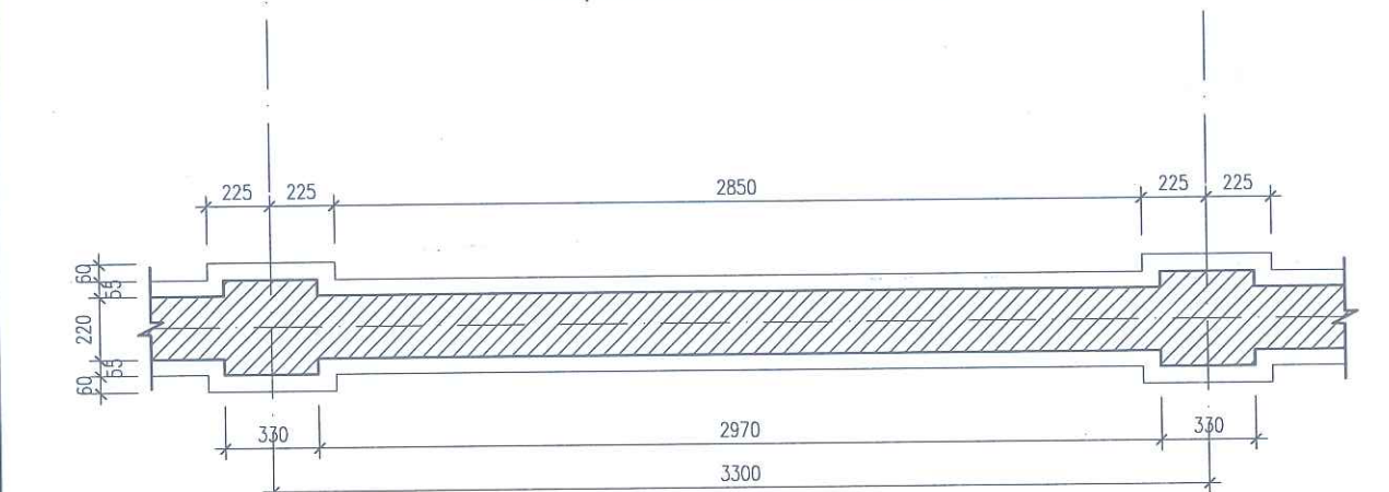
MẶT CẮT 1-1
