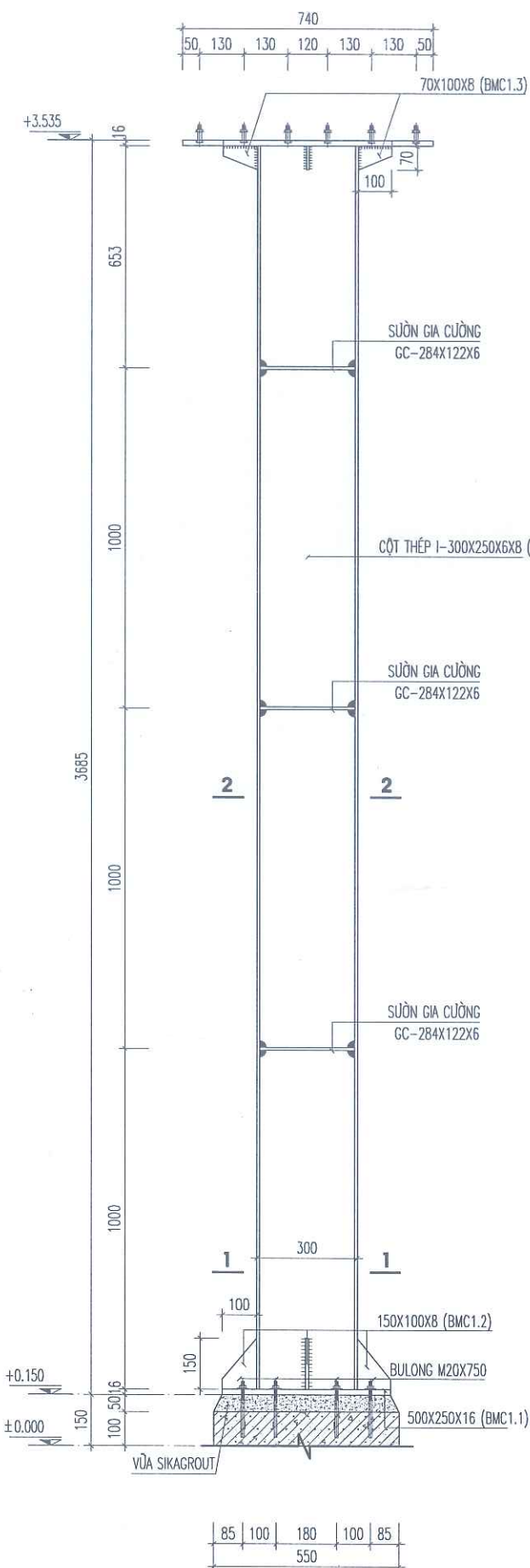
CHI TIẾT CỘT THÉP C1 ( SL : 02 C.KIỆN )
