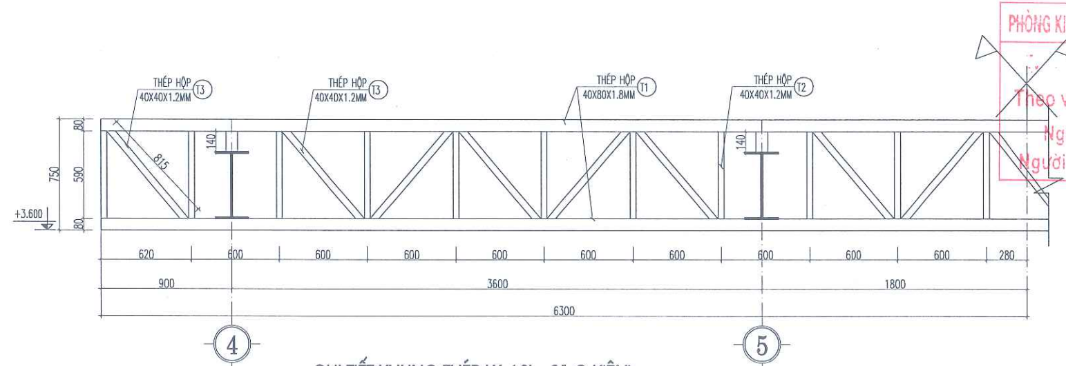
CHI TIẾT KHUNG THÉP K6 ( SL : 01 C.KIỆN)
