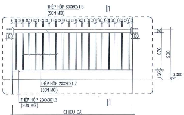
CHI TIẾT LAN CAN ĐIỂN HÌNH TẦNG 1 L=28.66M
