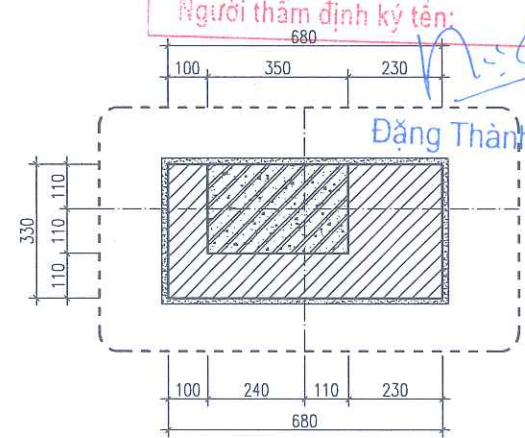
CHI TIẾT 3
