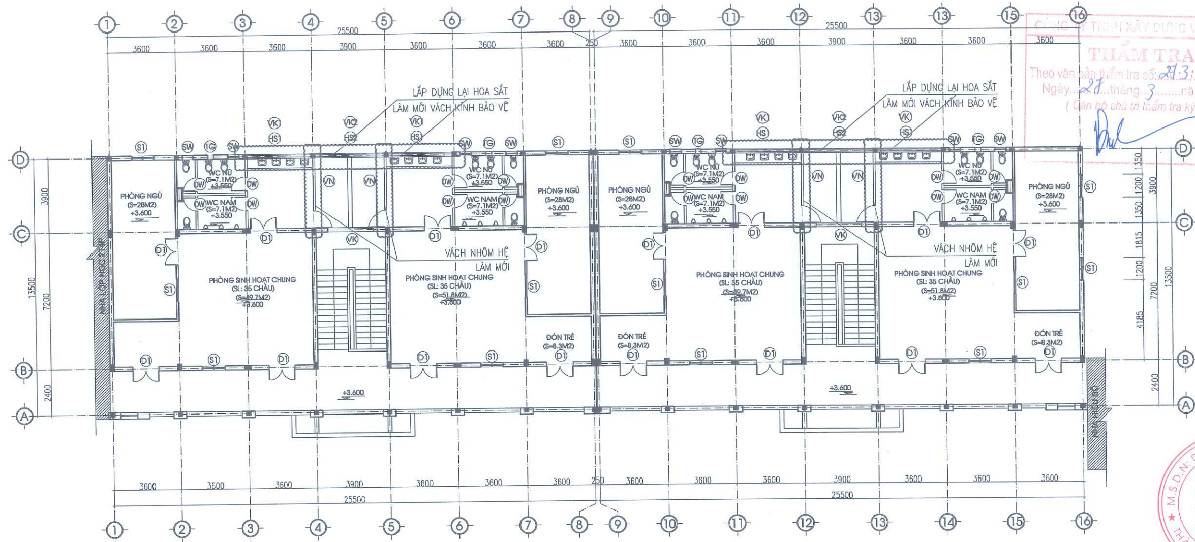
MẶT BẰNG CỦA TẦNG 1
