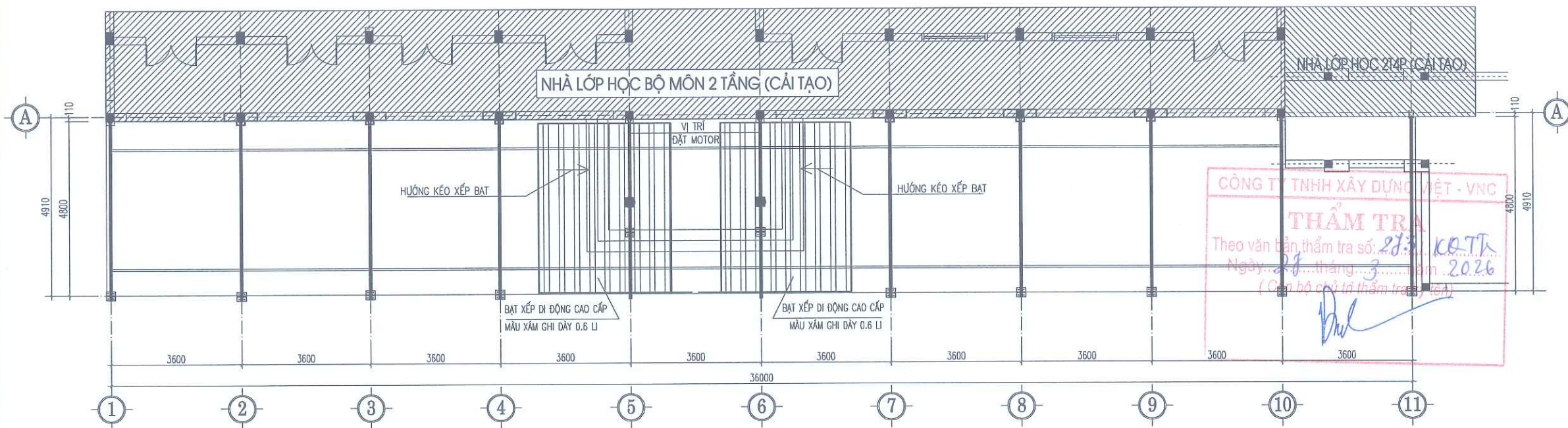
MẶT BẰNG KẾT CẤU MÁI BẠT CHE
