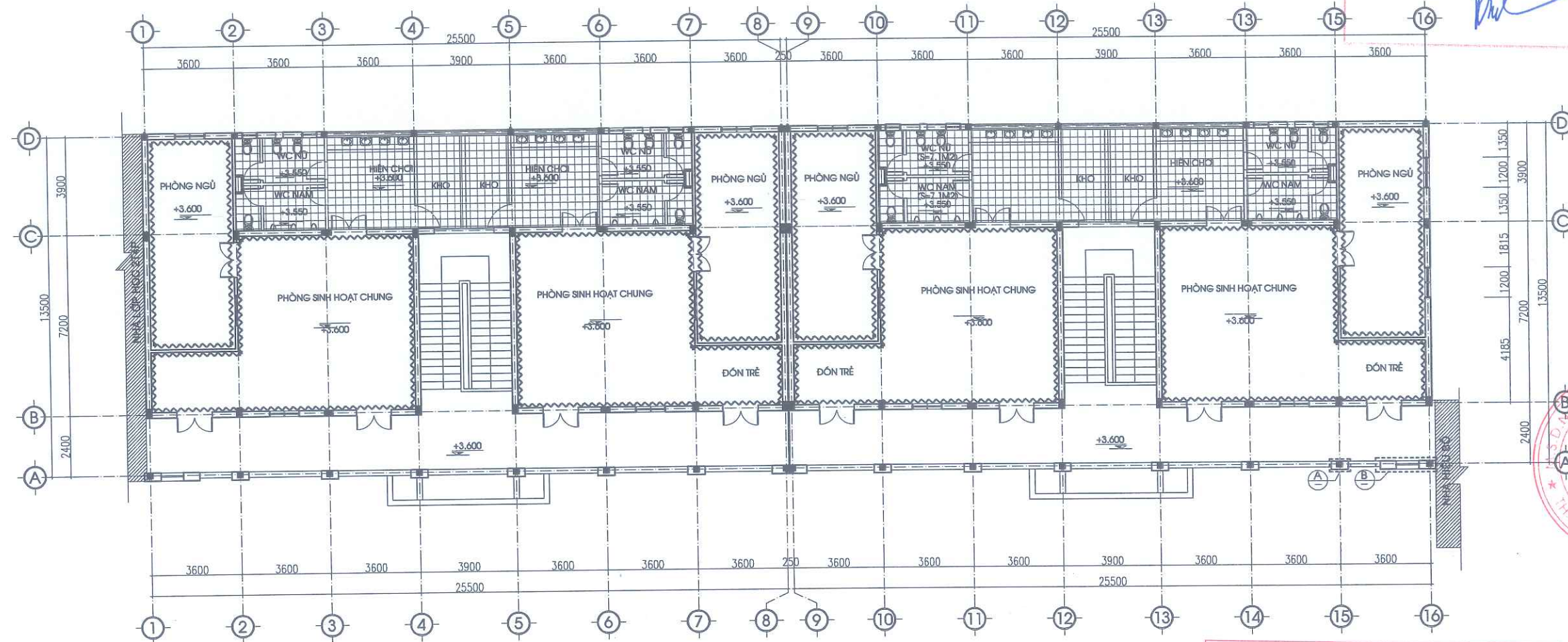
MẶT BẰNG LÁT SÀN TẦNG 2
