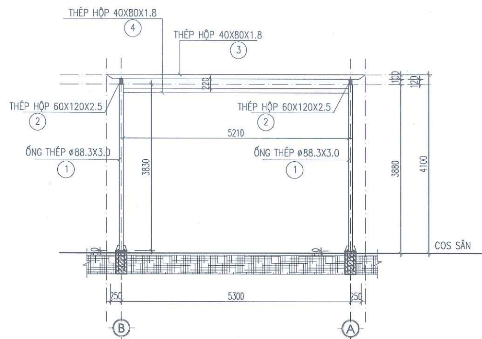
MẶT ĐỨNG TRỤC B-A
