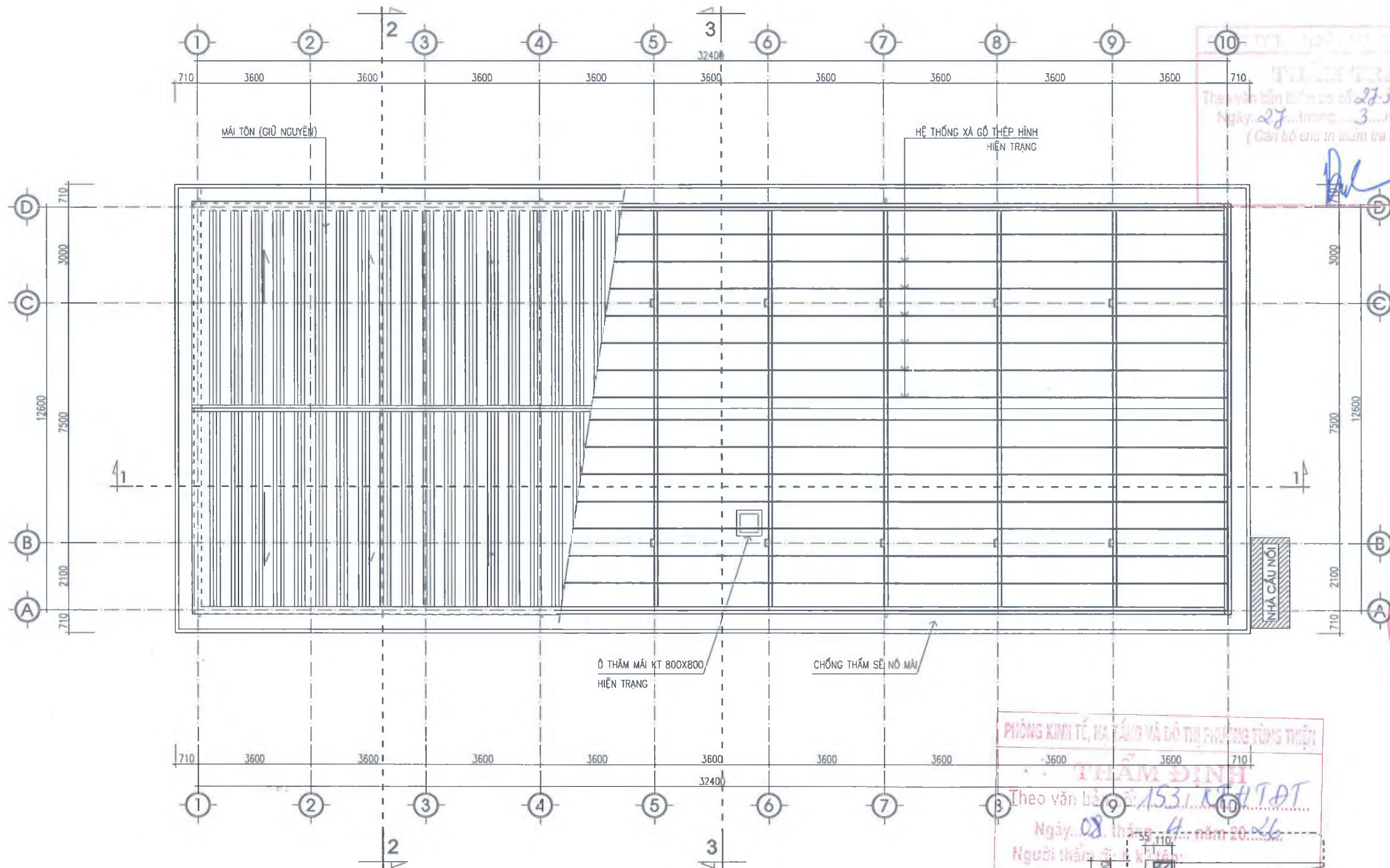
MẶT BẰNG MÁI
