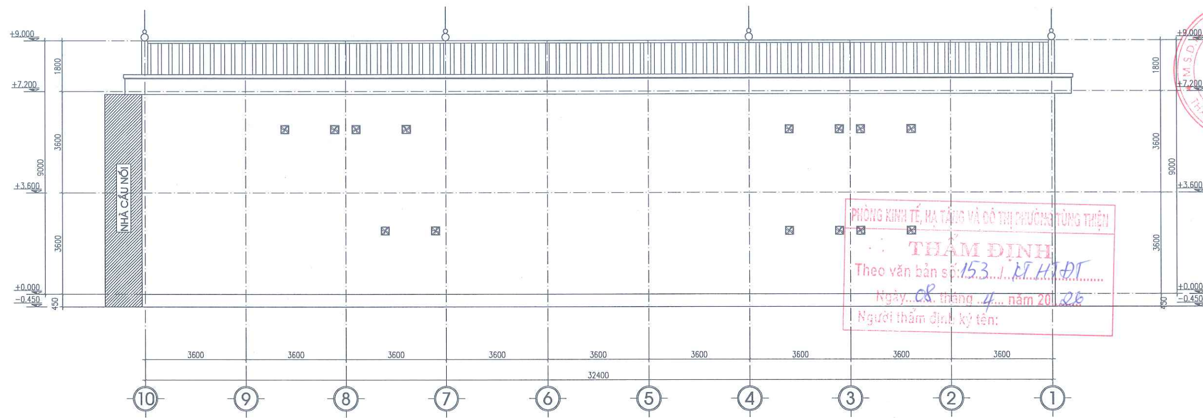
MẶT ĐỨNG TRỰC 10-1
