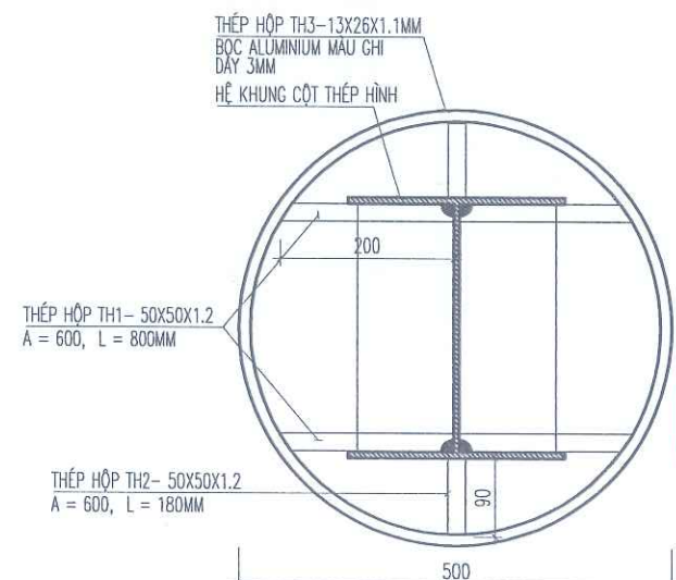
CHI TIẾT BỌC ALUMINIUM CỘT
