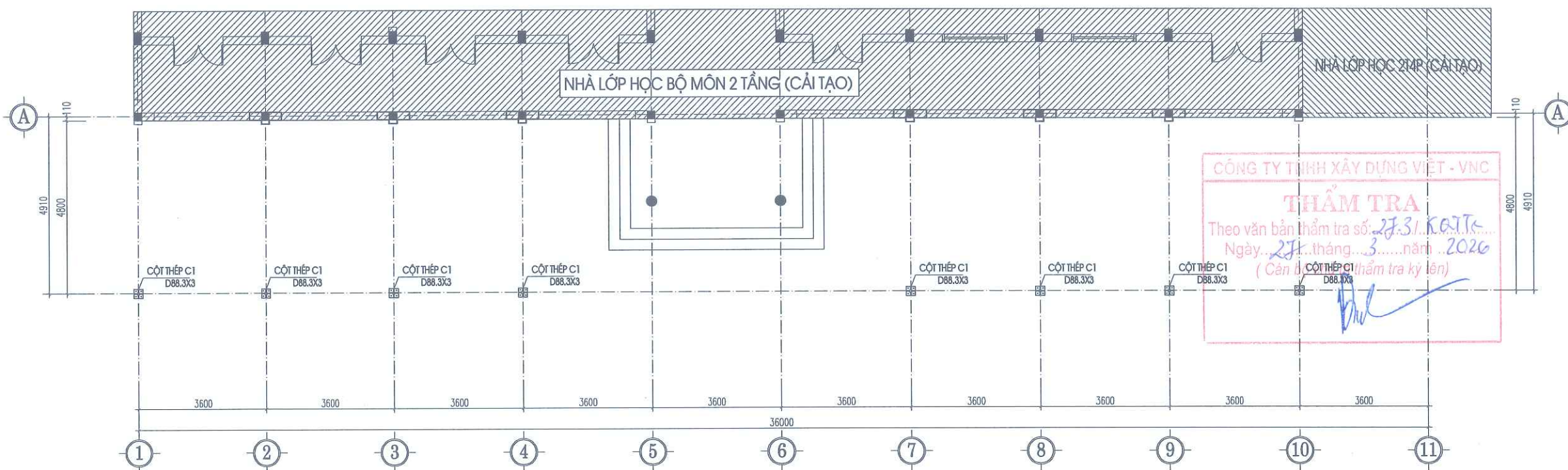
MẶT BẰNG ĐỊNH VỊ CỘT KHUNG THÉP MÁI CHE
