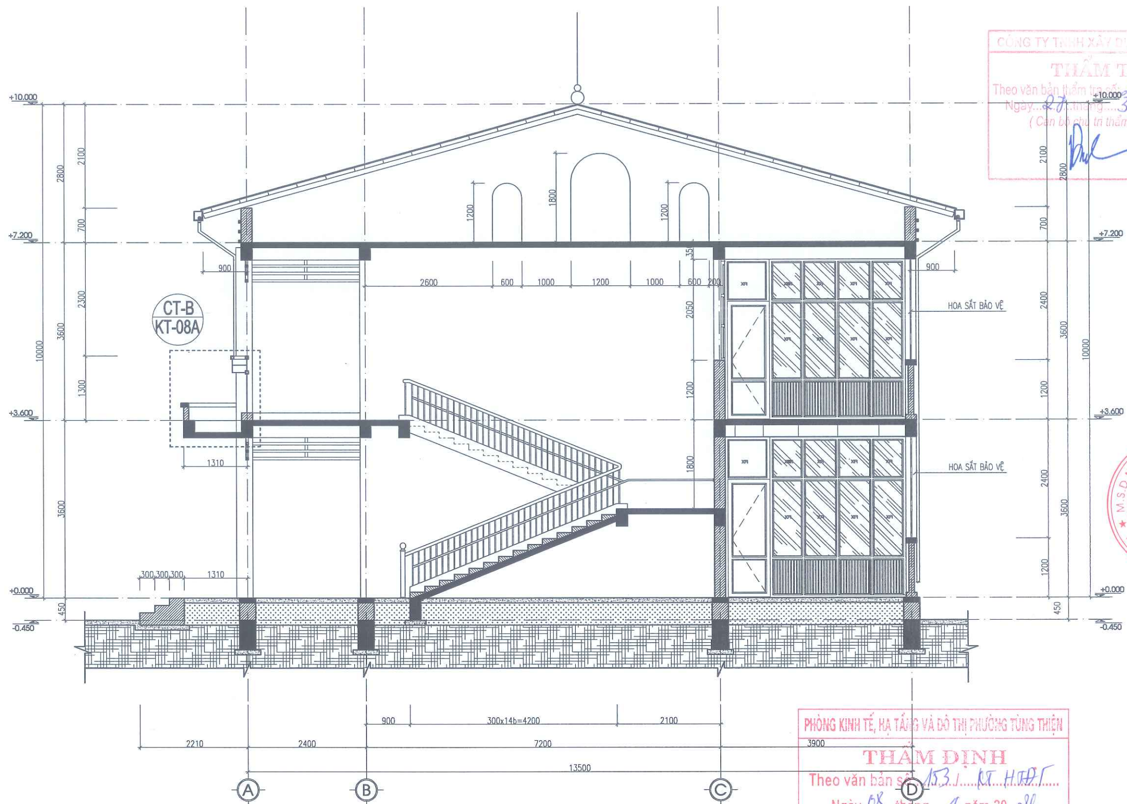
MẶT CẮT 1-1
