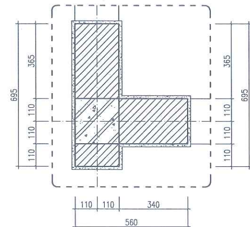
CHI TIẾT 3
