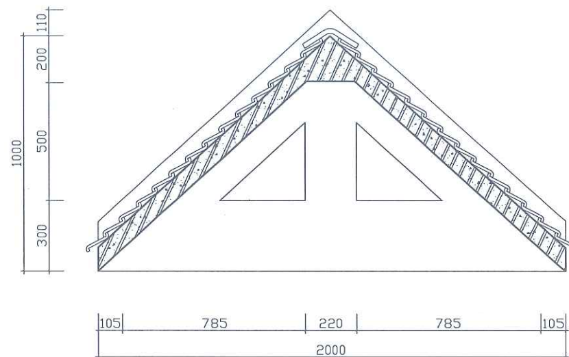
CHI TIẾT CT03
