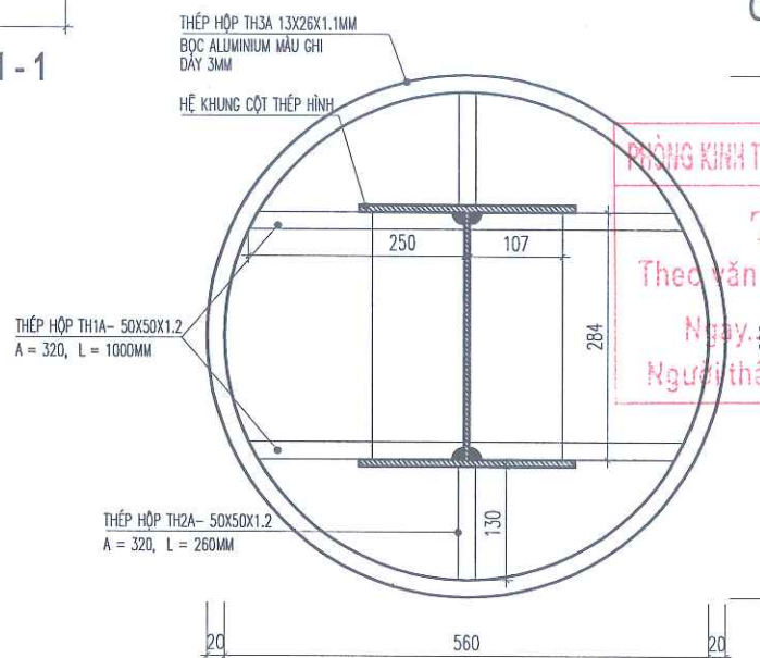
CHI TIẾT BỌC ALUMINIUM CHÂN CỘT
