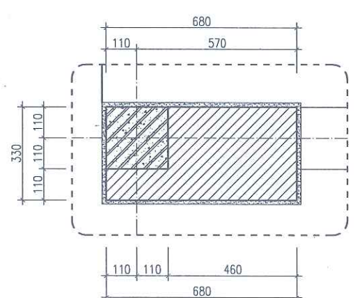
CHI TIẾT 1
