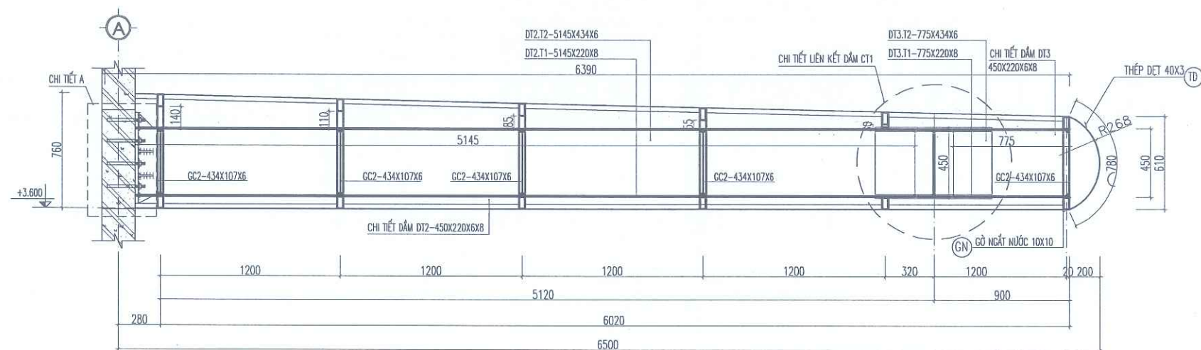
CHI TIẾT DẦM DT2-450X220X6X8(SL : 04 C.KIỆN), DT3-450X220X6X8 (SL : 04 C.KIỆN)
