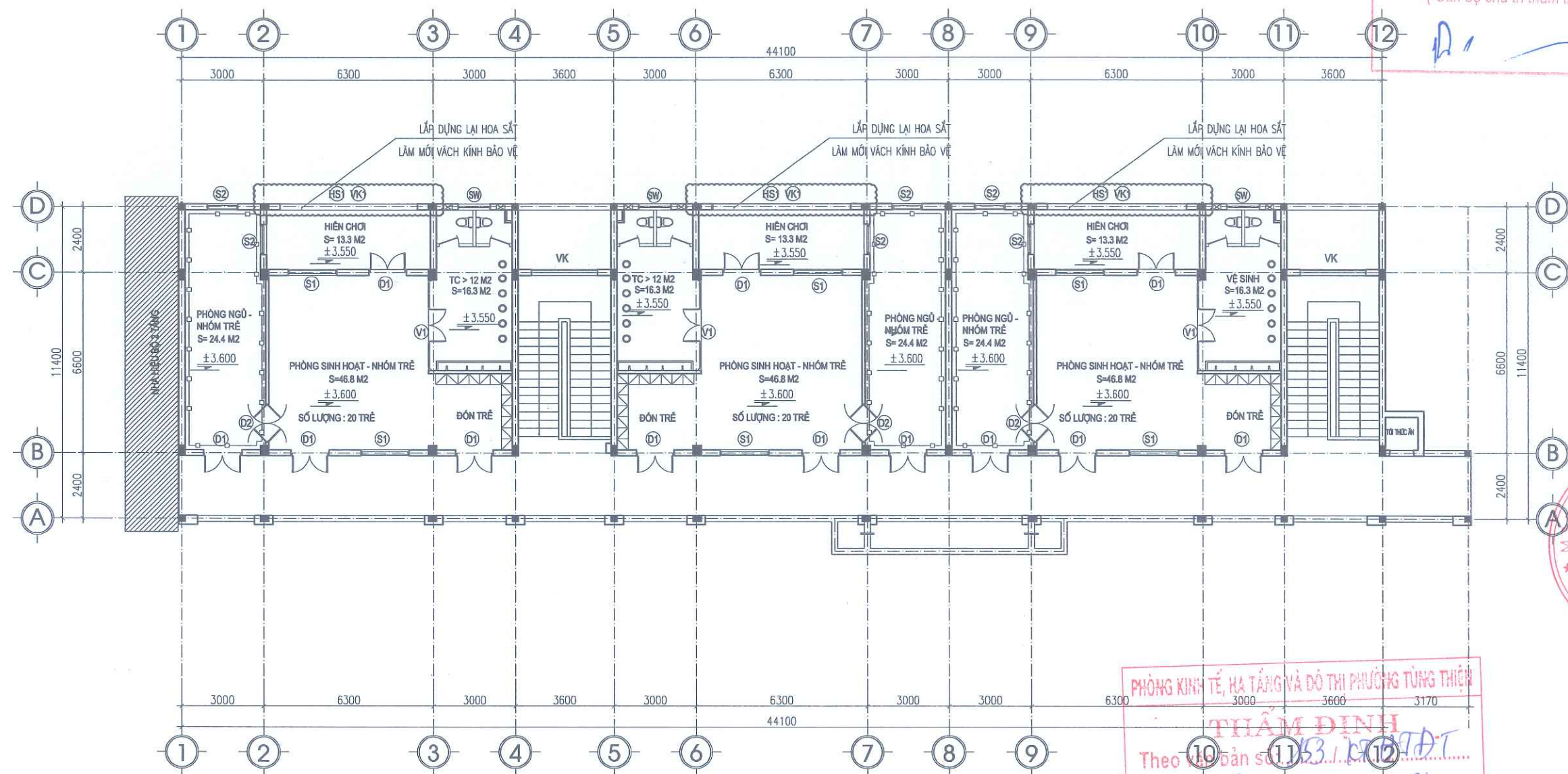
MẶT BẰNG CỦA TẦNG 1
