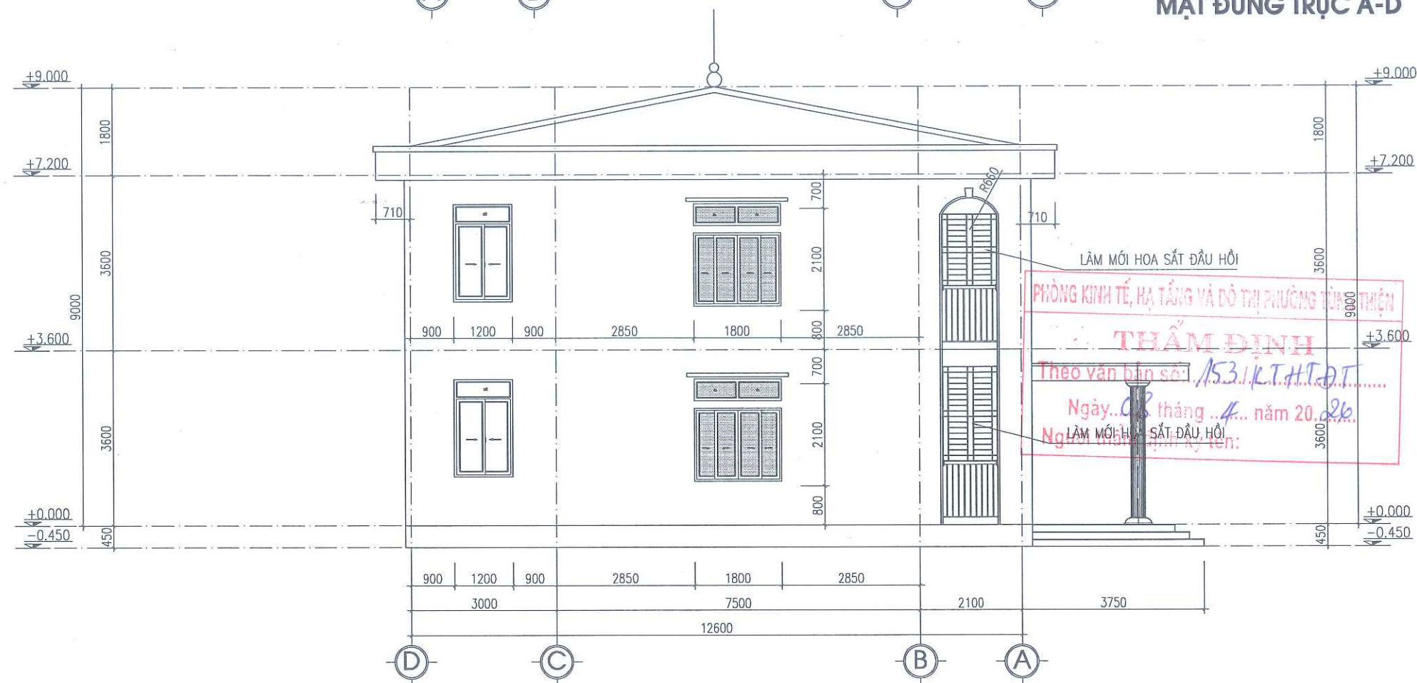
MẶT ĐỨNG TRỰC D-A
