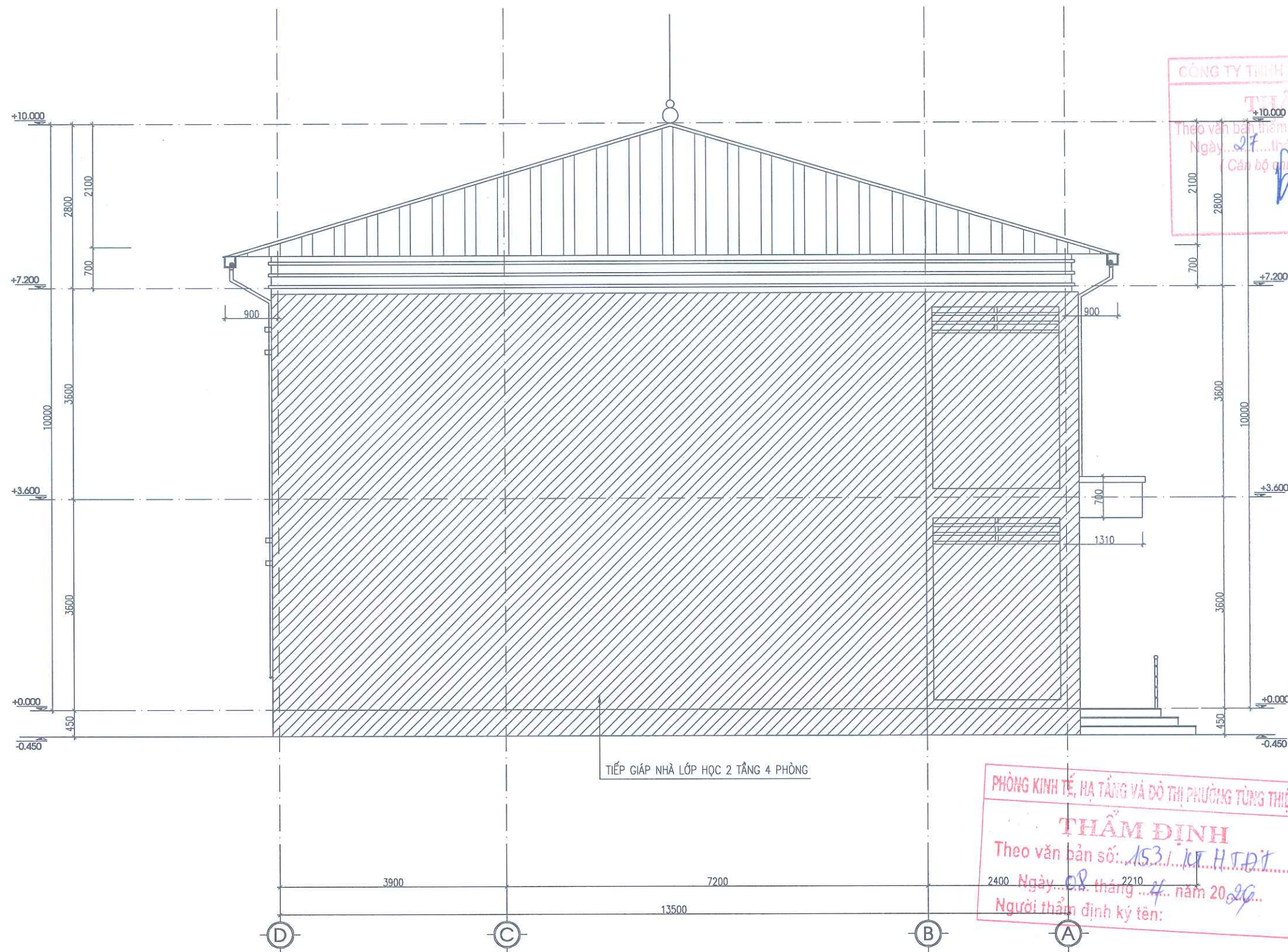
MẶT ĐÚNG TRỤC D-A
