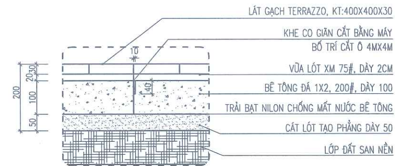
MẶT CẮT ĐIỂN HÌNH SÂN LÁT GẠCH LOẠI 1, SÂN S1 LÁT TRÊN NỀN BÊ TÔNG MỚI, BÊN TRONG TRƯỜNG Y TRỊNH XÂY DỰNG VIỆT - VIỆT DIỆN TÍCH : S = 197.8 M2
