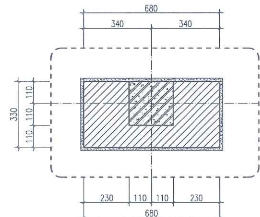
CHI TIẾT 2
