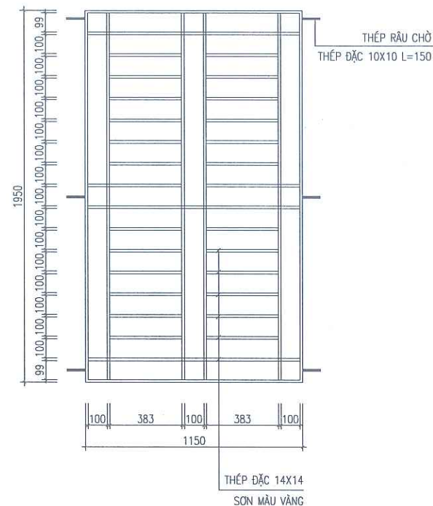
HOA SẮT V1 - TẦNG 1 (KT=1150X1950, SL=01 BỘ)
