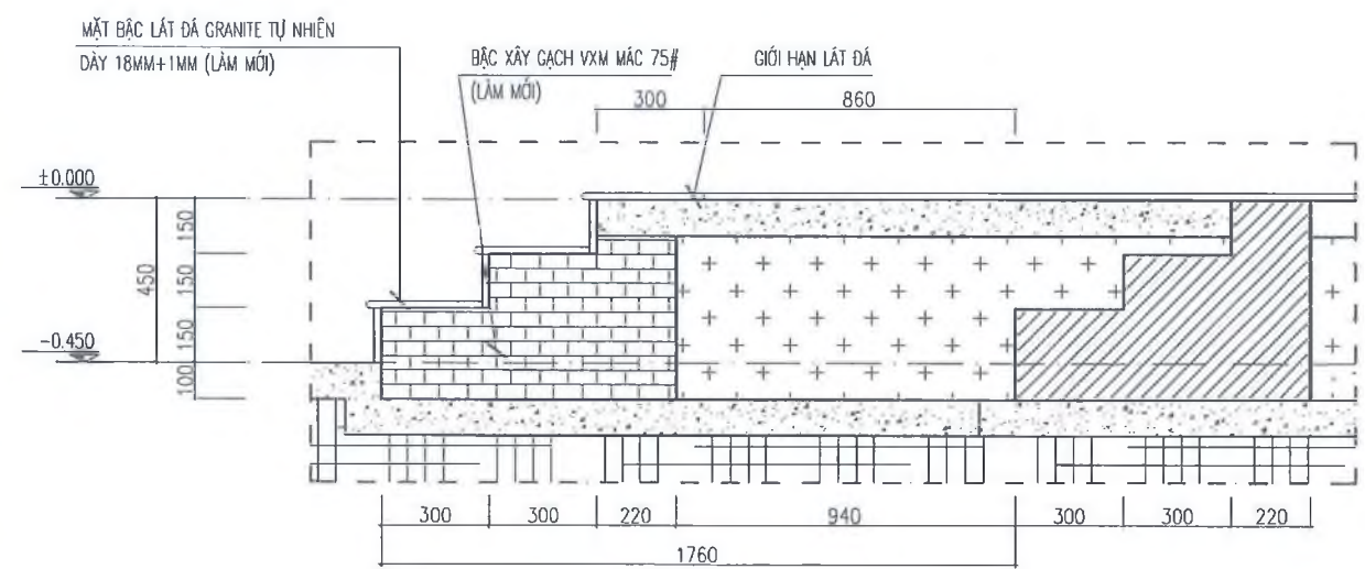
MẶT CẮT 2-2
