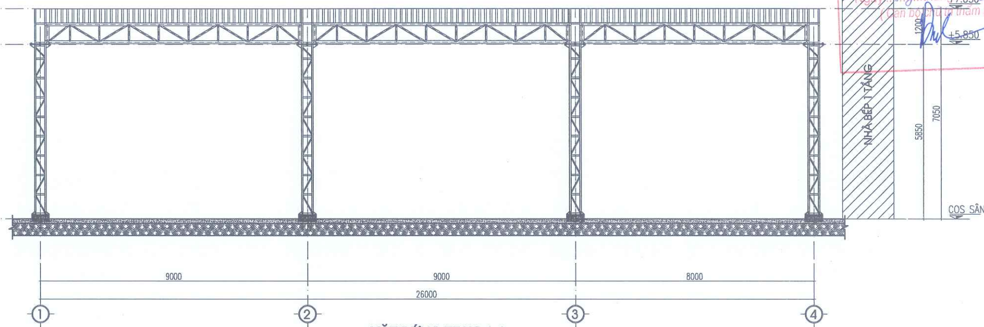
MẶT ĐỨNG TRỰC 1-4
