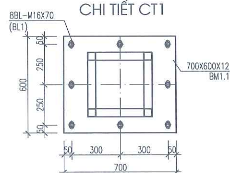
CHI TIẾT BẢN MÃ BM1.1
