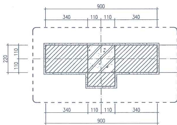
CHI TIẾT 4
