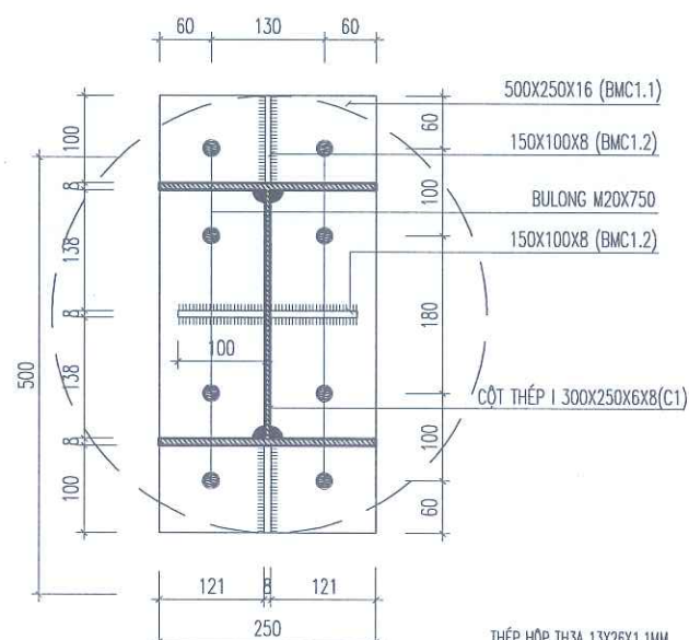
MẶT CẮT 1-1
