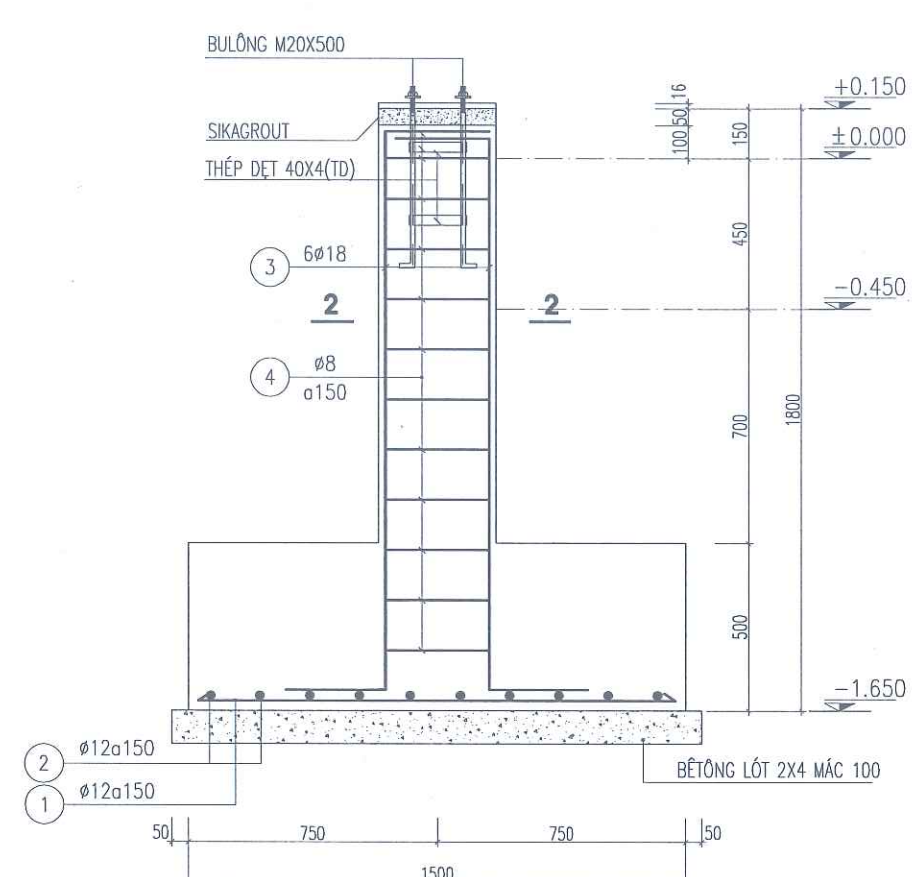
MẶT CẮT 1 - 1
