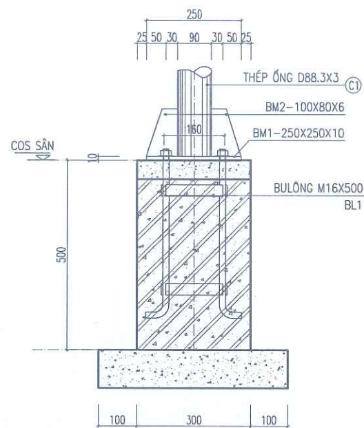
CHI TIẾT MÓNG CHÂN CỘT C1 (MÓNG VUÔNG 300X300; SL= 08 CK)
