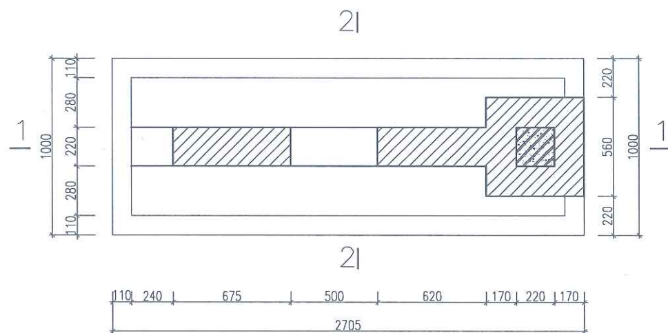
CHI TIẾT 01
