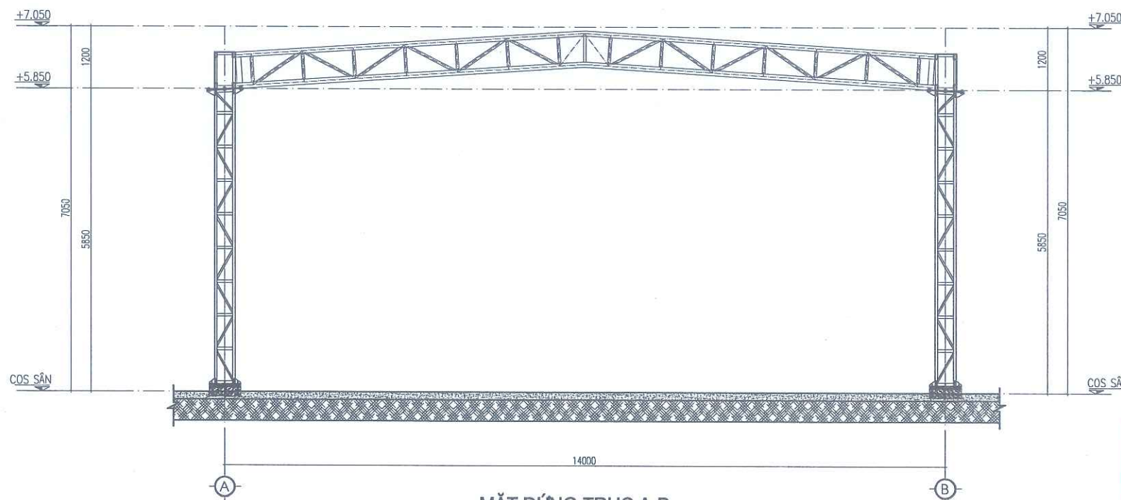
MẶT ĐỨNG TRỤC A-B
