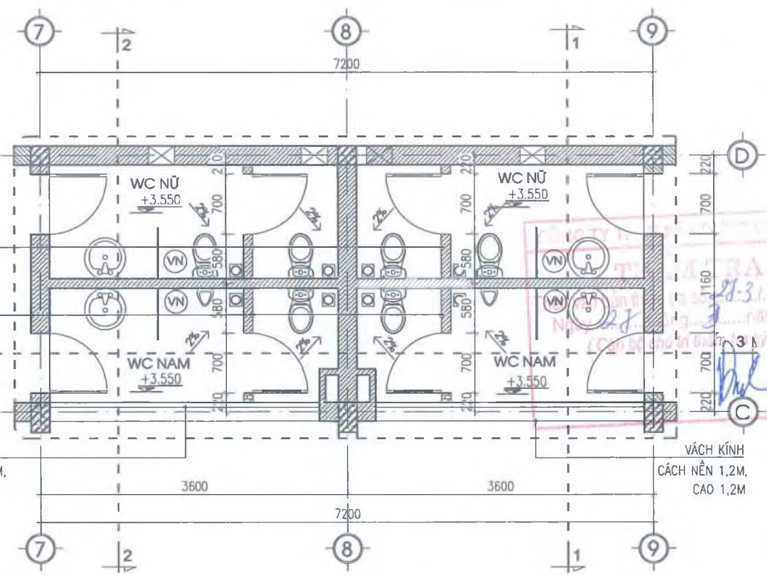
MẶT BẰNG VỆ SINH TẦNG 2 SỐ 2
