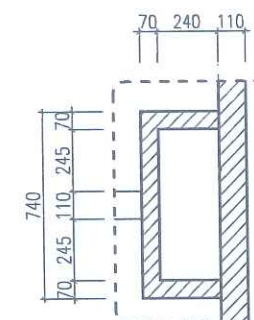
CHI TIẾT HỘP KỸ THUẬT
