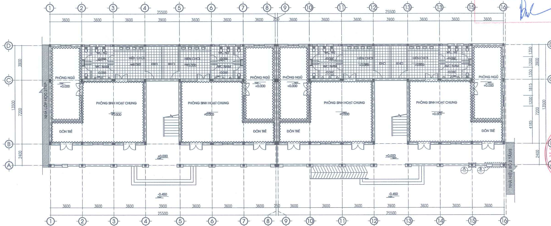
MẶT BẰNG LÁT NỀN TẦNG 1
