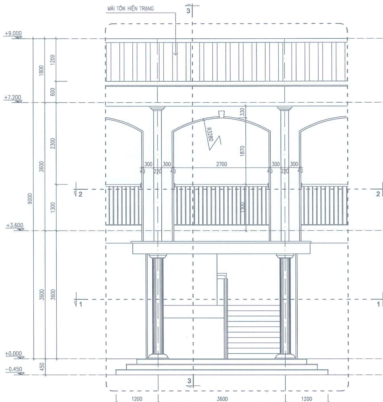
CHI TIẾT SẴNH CHÍNH
