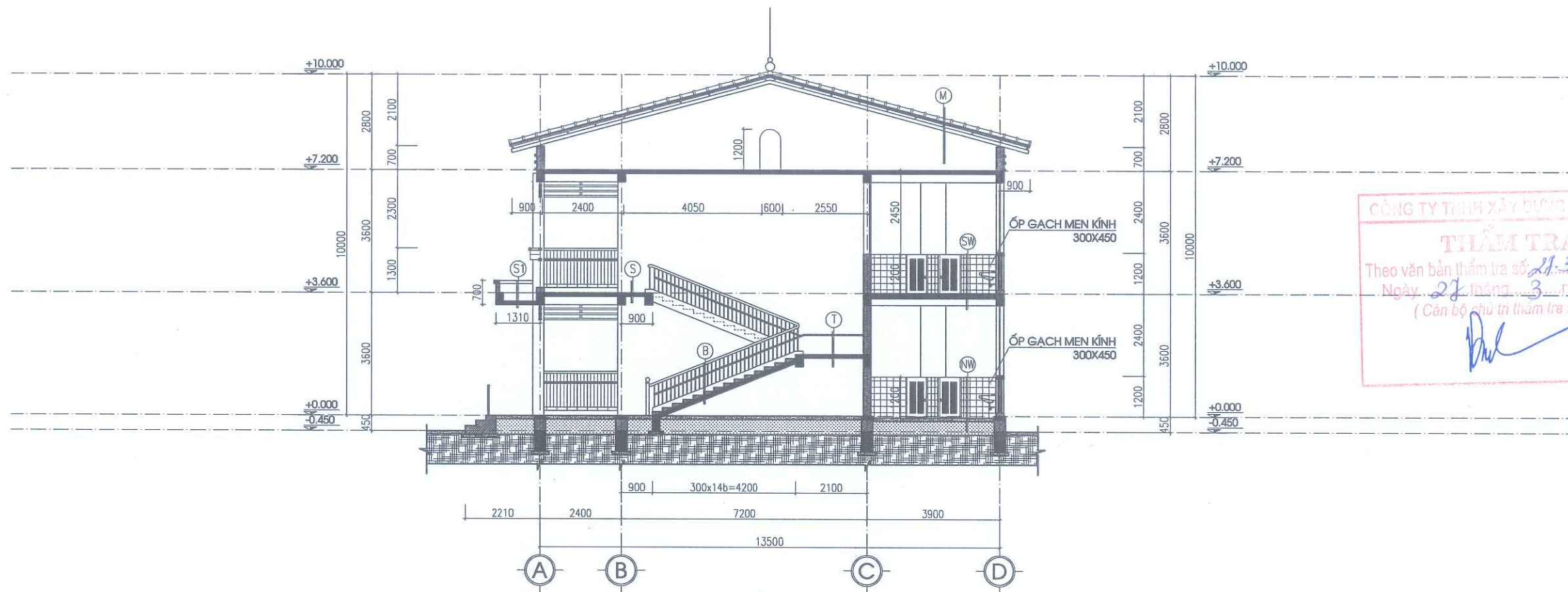
MẶT CẮT 1-1
