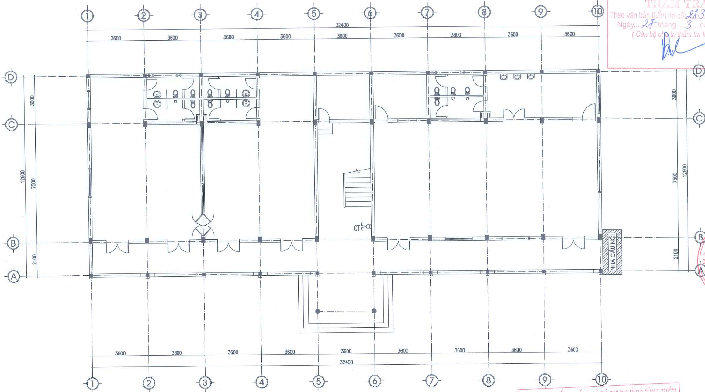
MẶT BẰNG CẢI TẠO ĐIỆN TẦNG 1
