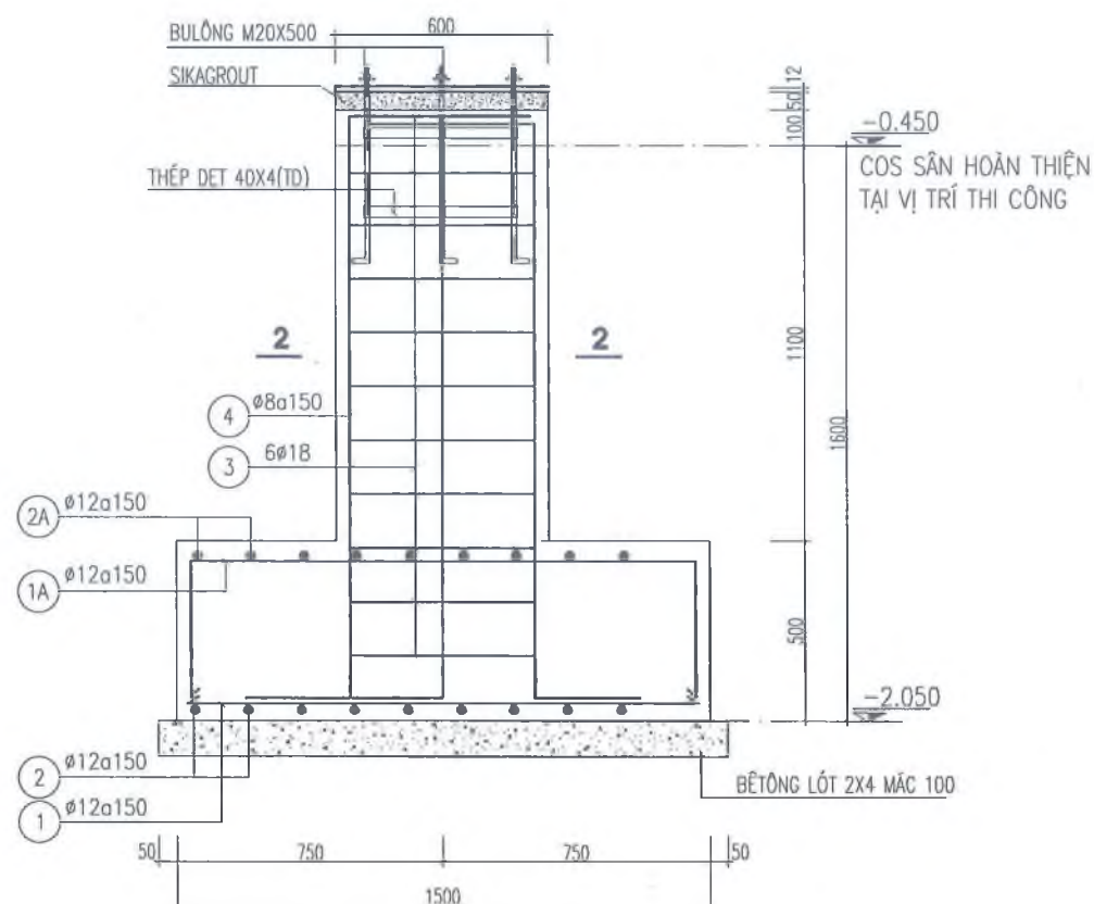
MẶT CẮT 1 - 1
