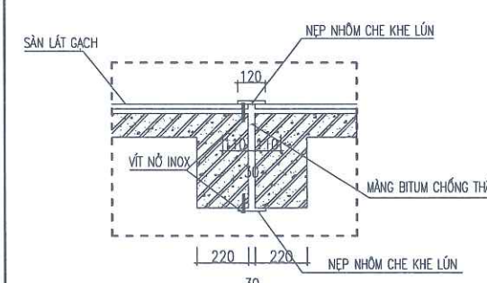
CHI TIẾT CHE KHE TIẾP GIÁP SÀN TẦNG VỊ TRÍ TRỤC 8-9; L= 2.18 M
