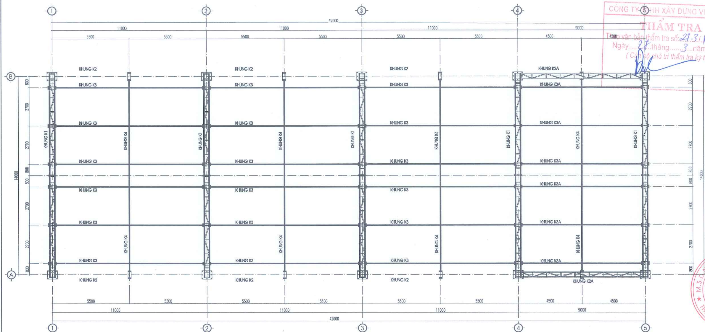
MẶT BẰNG KẾT CẤU KHUNG THÉP MÁI
