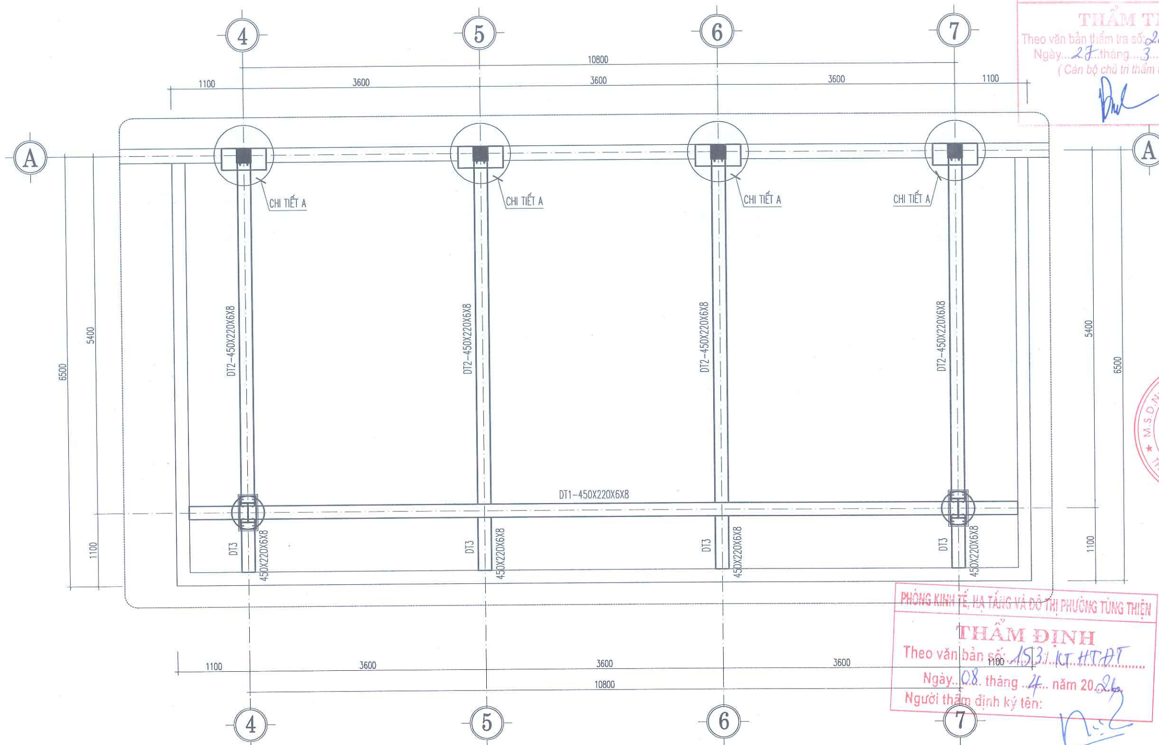
MẶT BẰNG KẾT CẤU MÁI SẢNH
