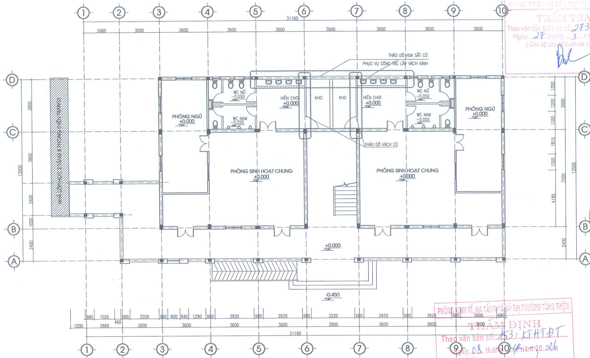
MẶT BẰNG PHÁ DỠ TẦNG 1
