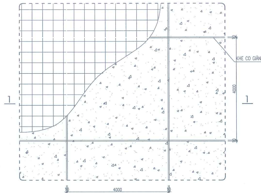
MẶT BẰNG ĐIỂN HÌNH SÂN BÊ TÔNG/ LÁT GẠCH LÀM MỚI
