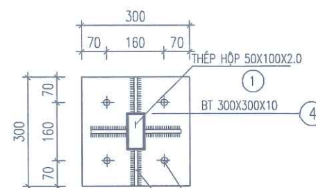
KHUNG MÓNG K1
