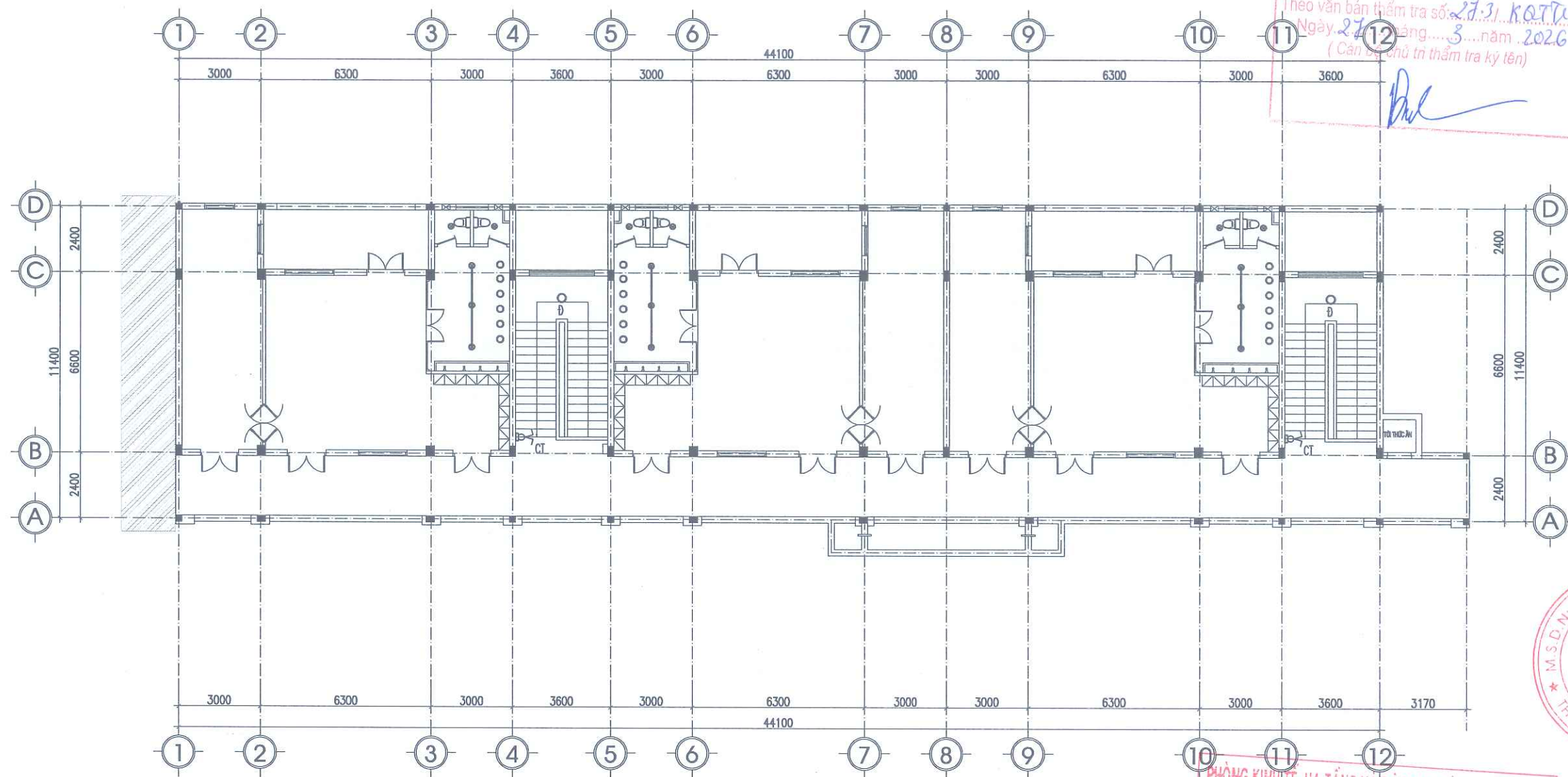
MẶT BẰNG CẢI TẠO ĐIỆN TẦNG 2
