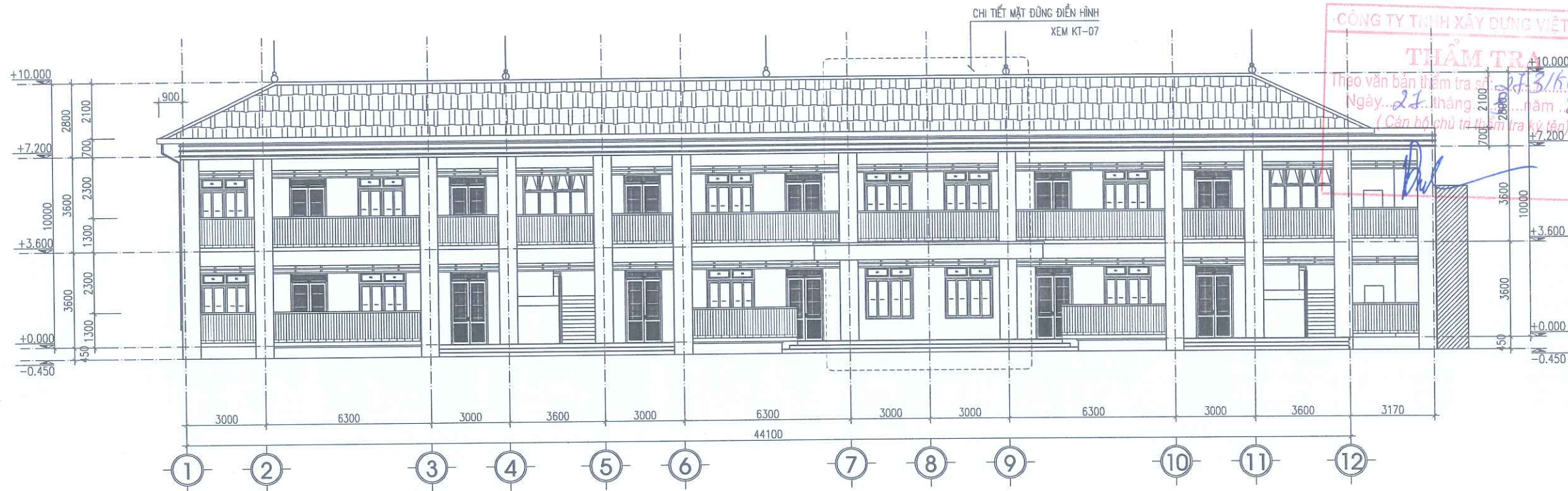
MẶT ĐÚNG TRỤC 1-12
