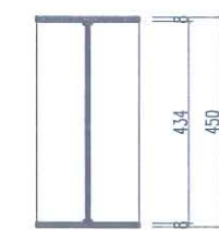
MẶT CẮT 1-1
