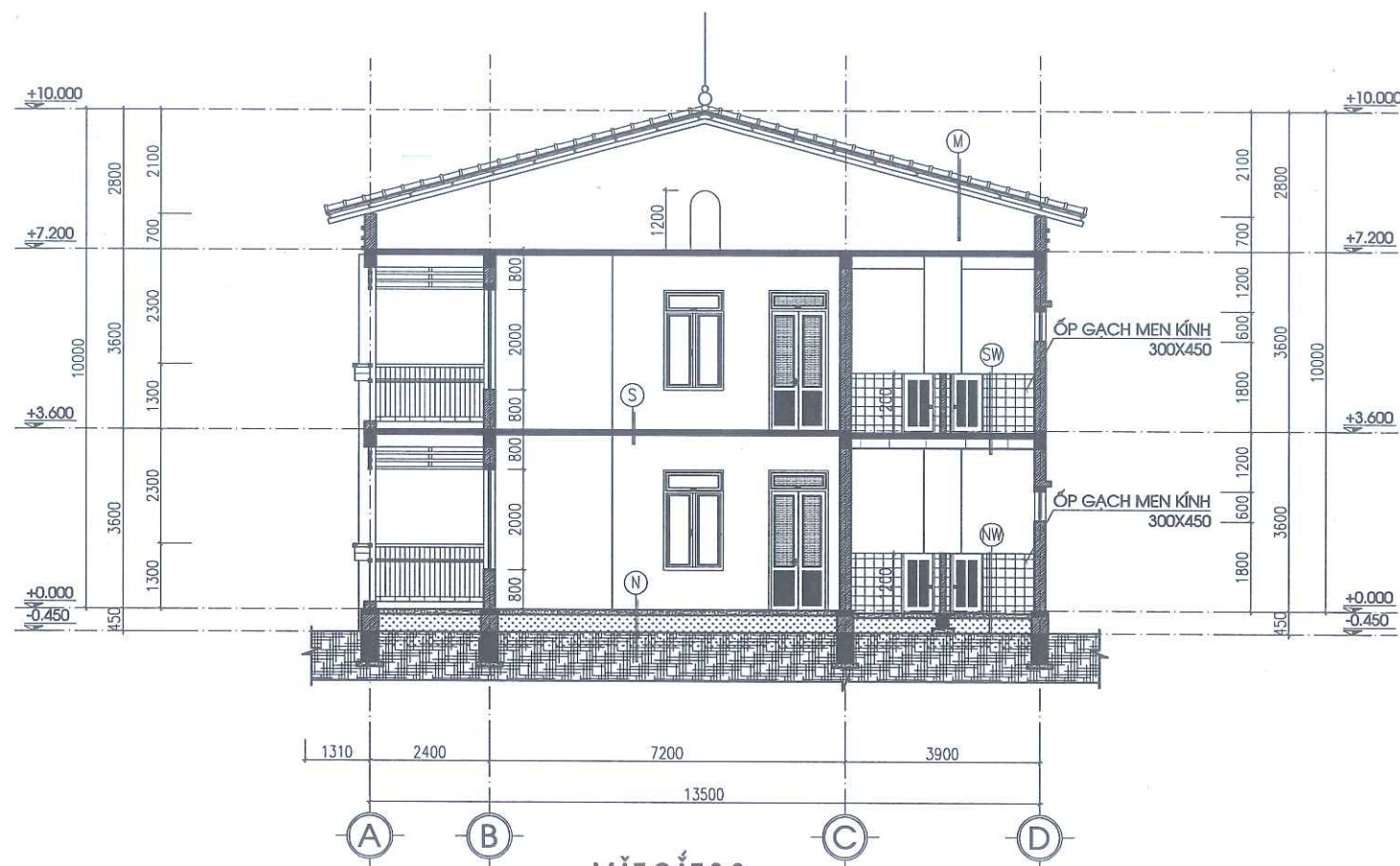
MẶT CẮT 2-2
