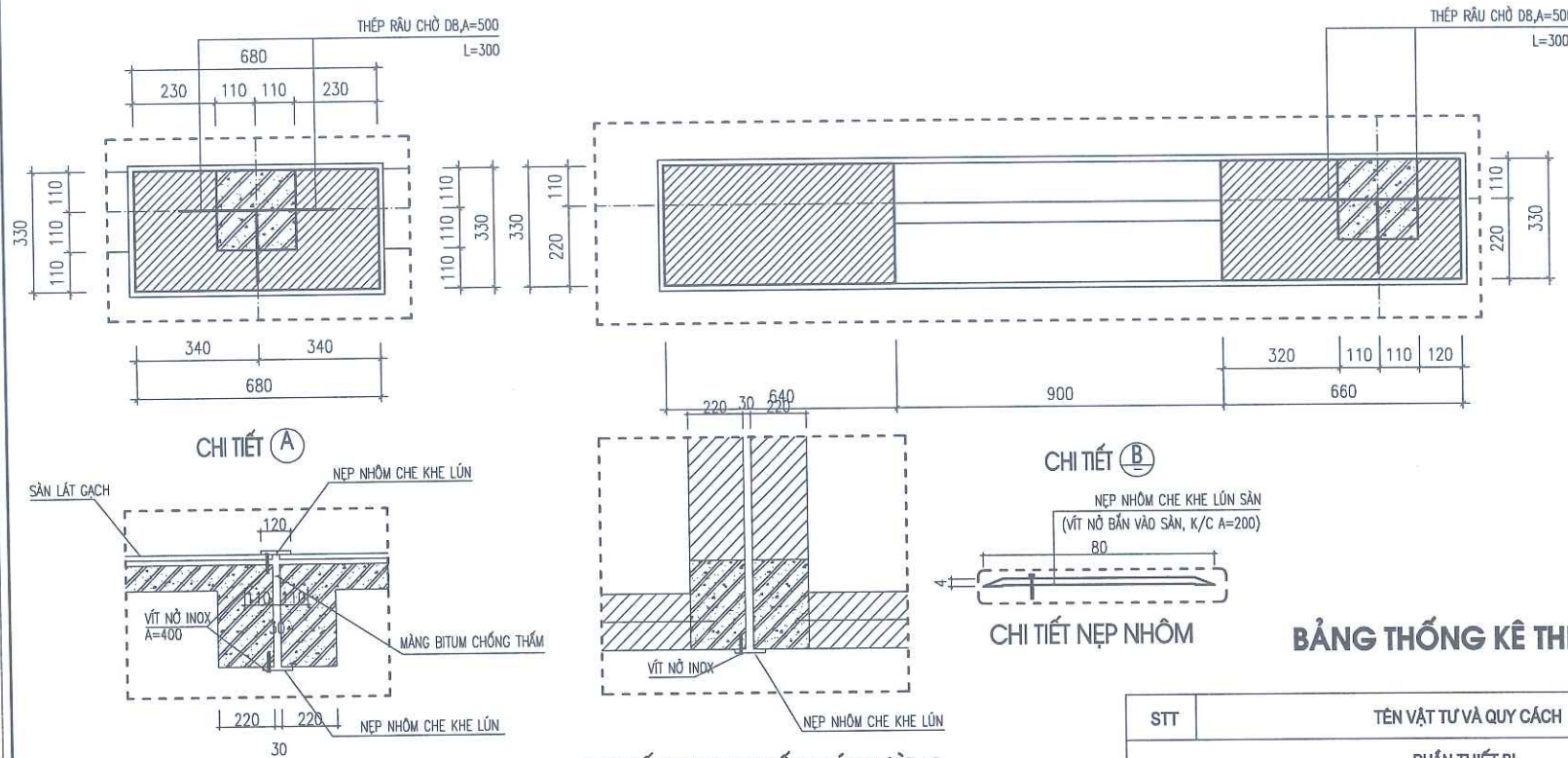
CHI TIẾT CHE KHE TIẾP GIÁP SÀN TẦNG VỊ TRÍ TRỤC 8-9; L= 2.18 M
