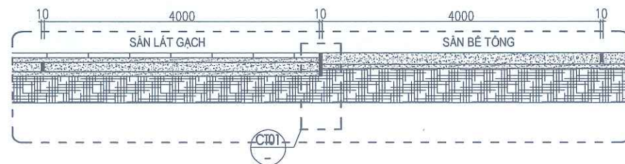
MẶT BẰNG ĐIỂN HÌNH SÂN BÊ TÔNG/ LÁT GẠCH LÀM MỚI
