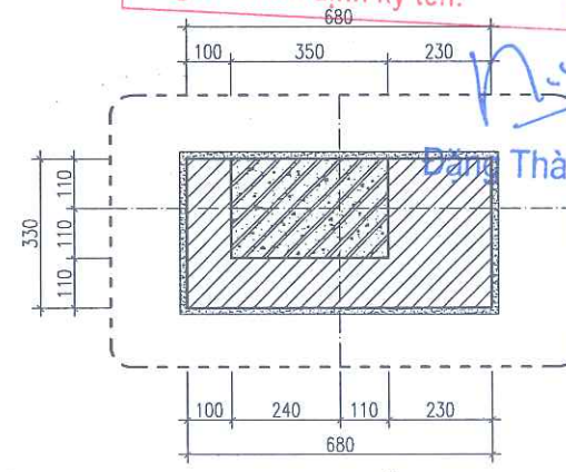
CHI TIẾT 3
