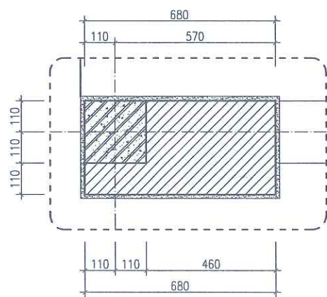
CHI TIẾT 1
