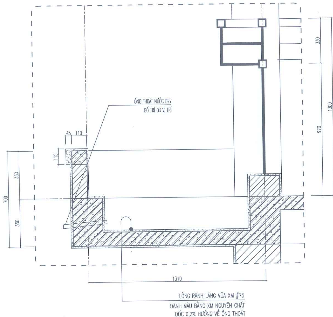
CHI TIẾT MÁI SẢNH (CHI TIẾT B)
