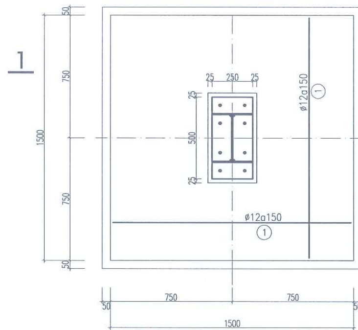
CHI TIẾT MÓNG MĐ1 (SL : 02 C.KIỆN)
