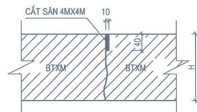
CHI TIẾT KHE CO GIÂN
