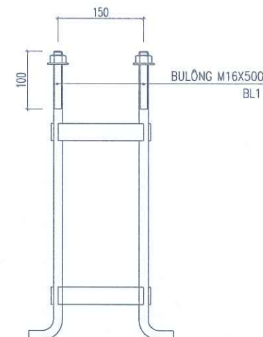
KHUNG THÉP CHÂN MÓNG
