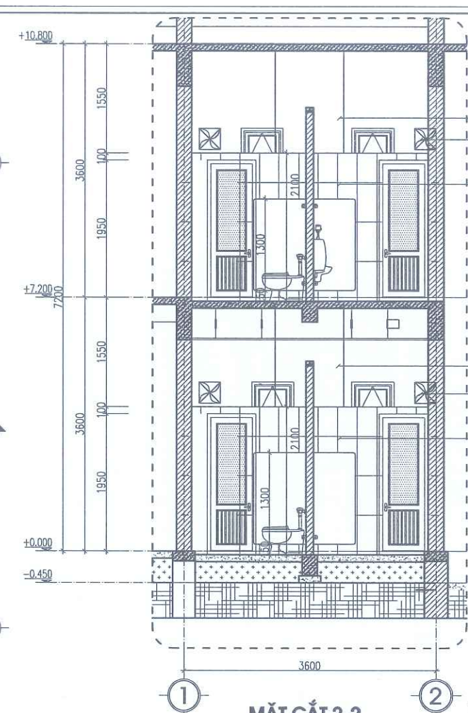
MẶT CẮT 2-2
