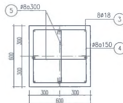
MẶT CẮT 2 - 2
