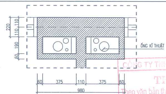
CHI TIẾT HỘP KỸ THUẬT
