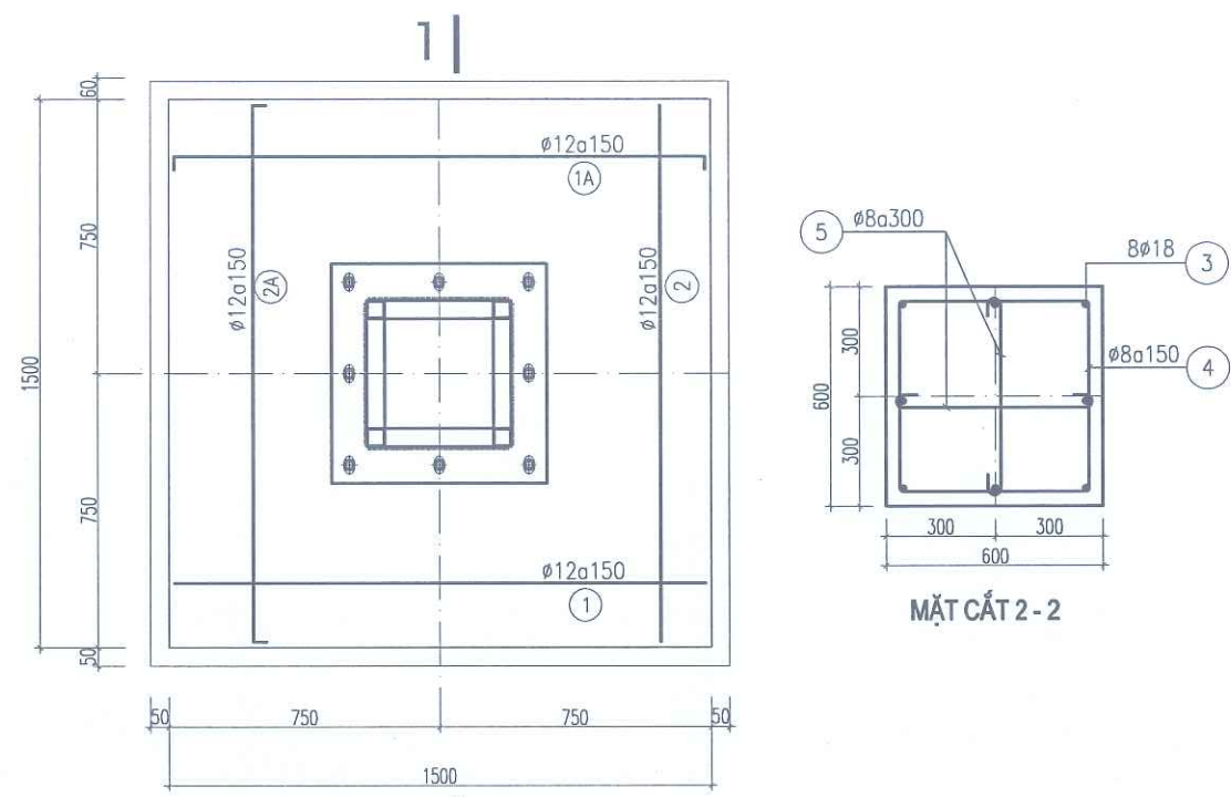
MÓNG MĐ1 (SL : 03 C.KIỆN)
