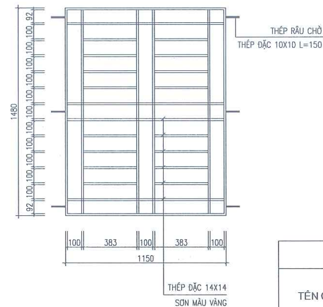
HOA SẮT V1 - TẦNG 2 (KT=1150X1480, SL=01 BỘ)
