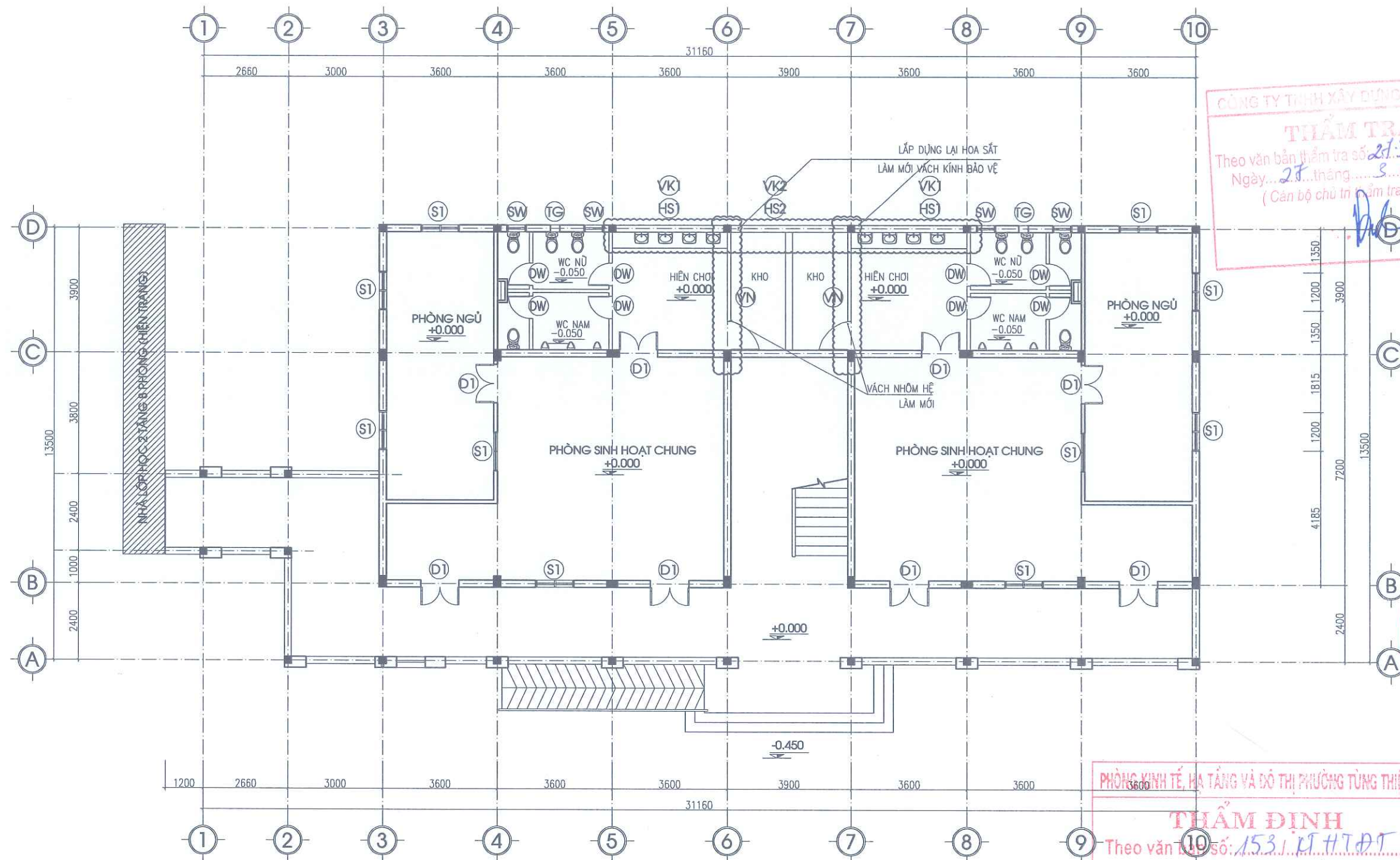
MẶT BẰNG CỦA TẦNG 1
