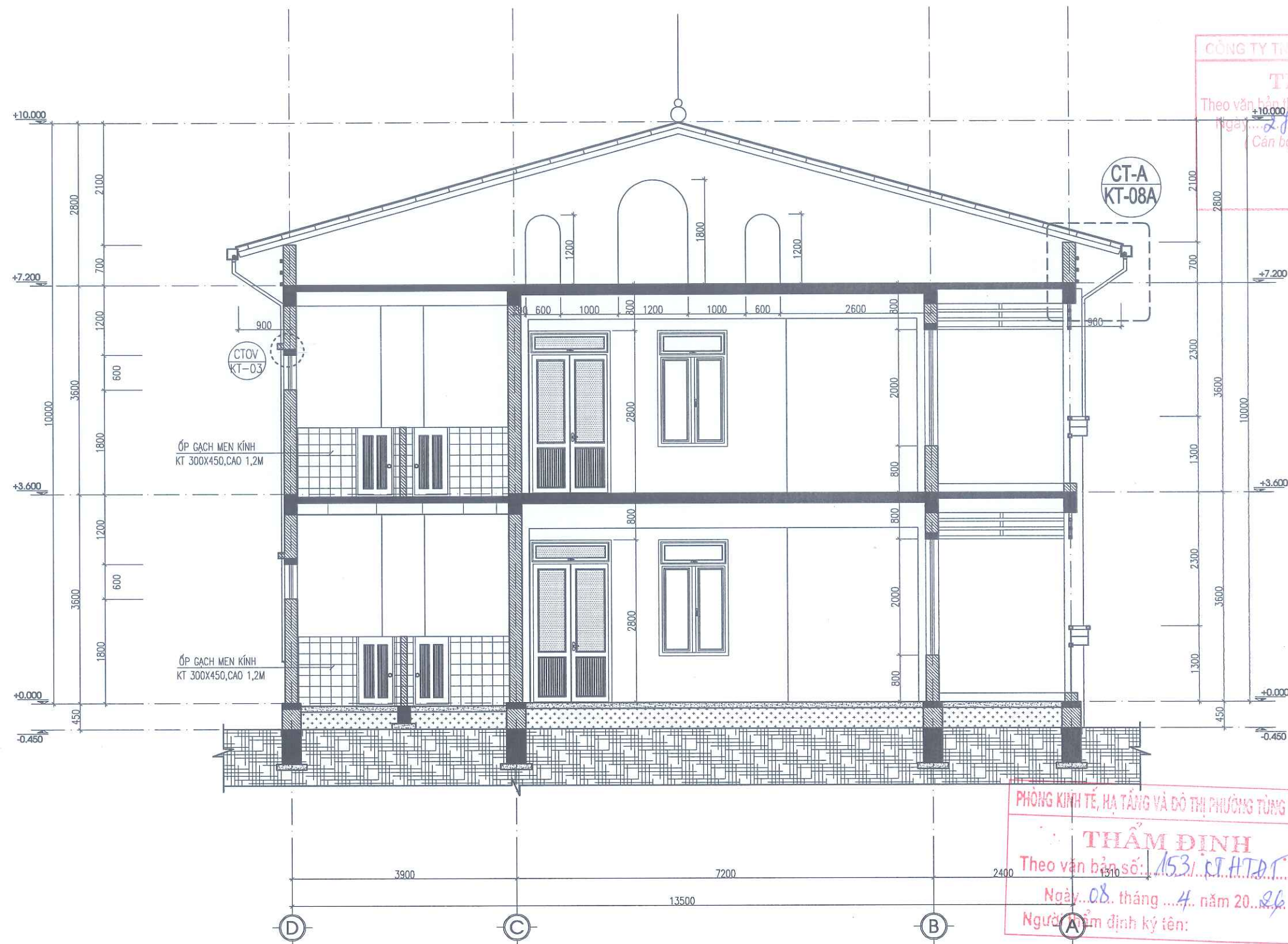
MẶT CẮT 2-2
