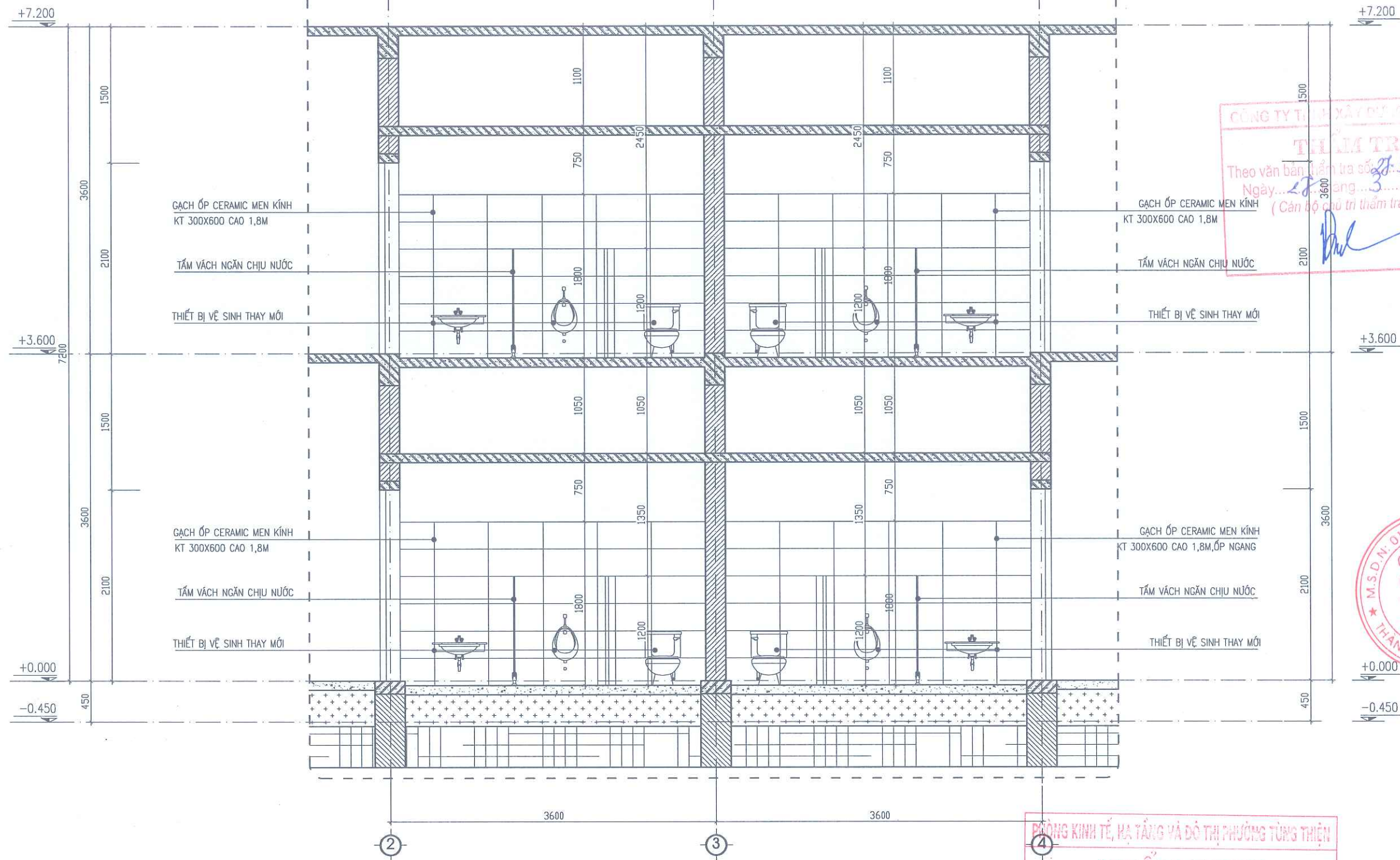
MẶT CẮT 3-3
