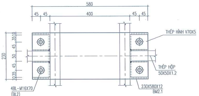
MẶT CẮT 2-2
