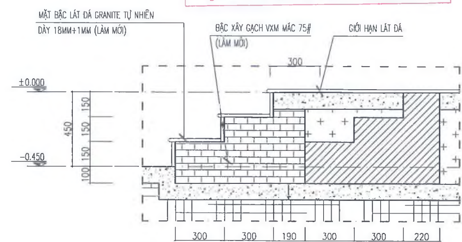
MẶT CẮT 1-1
