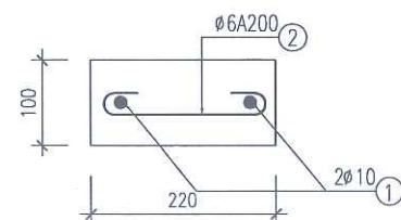
CHI TIẾT GIẺNG ĐÌNH (L=5.1M)
