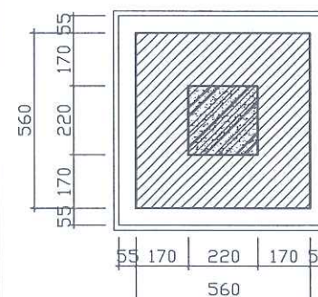
CẮT 2-2
