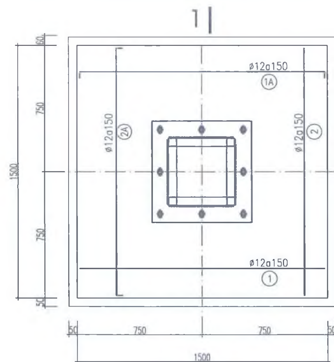
MÓNG MĐ1 (SL : 10 C.KIỆN)
