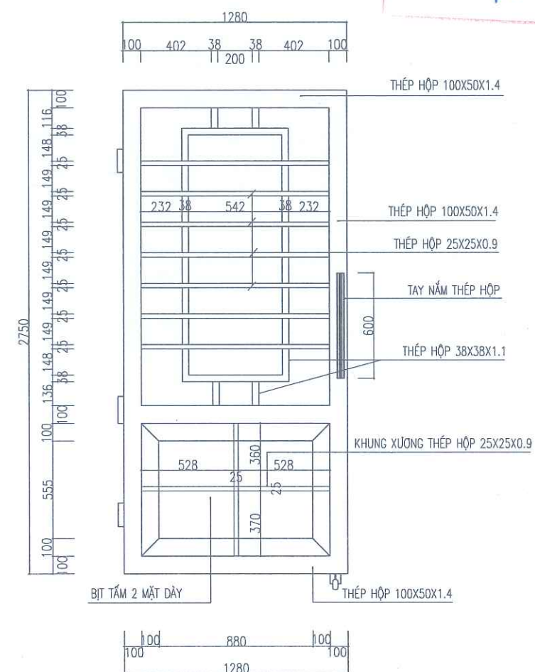
CHI TIẾT CẢNH CỔNG PHỤ (SL=02CK)
