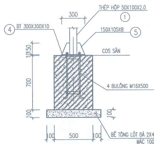
CHI TIẾT MÓNG (MÓNG VUÔNG 500X500X700) (SL : 09 CK)
