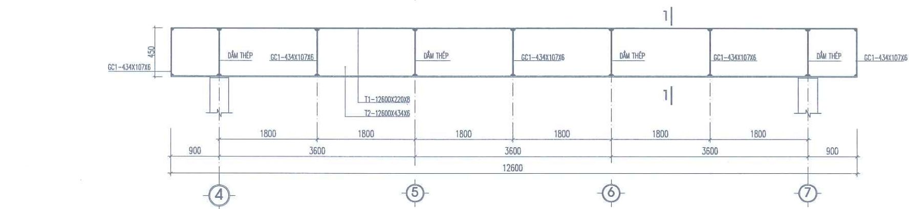
CHI TIẾT DẦM DT1-450X220X6X8 (SL : 01 C.KIỆN)
