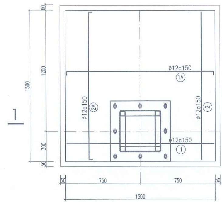
MÓNG MĐ2 (SL : 05 C.KIỆN)
