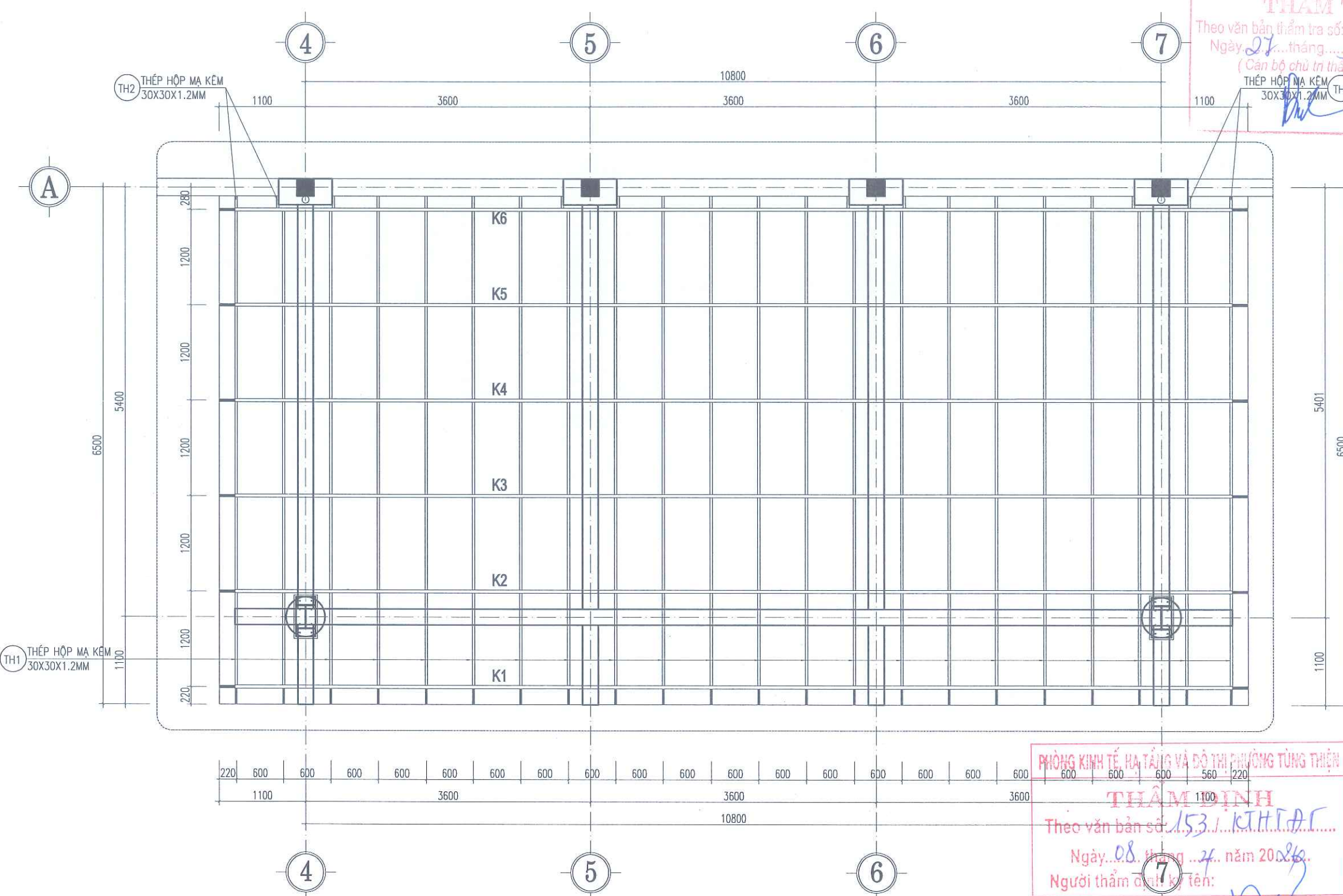
MẶT BẰNG KẾT CẤU MÁI SẴN
