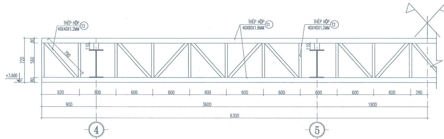
CHI TIẾT KHUNG THÉP K5 ( SL : 01 C.KIỆN)
