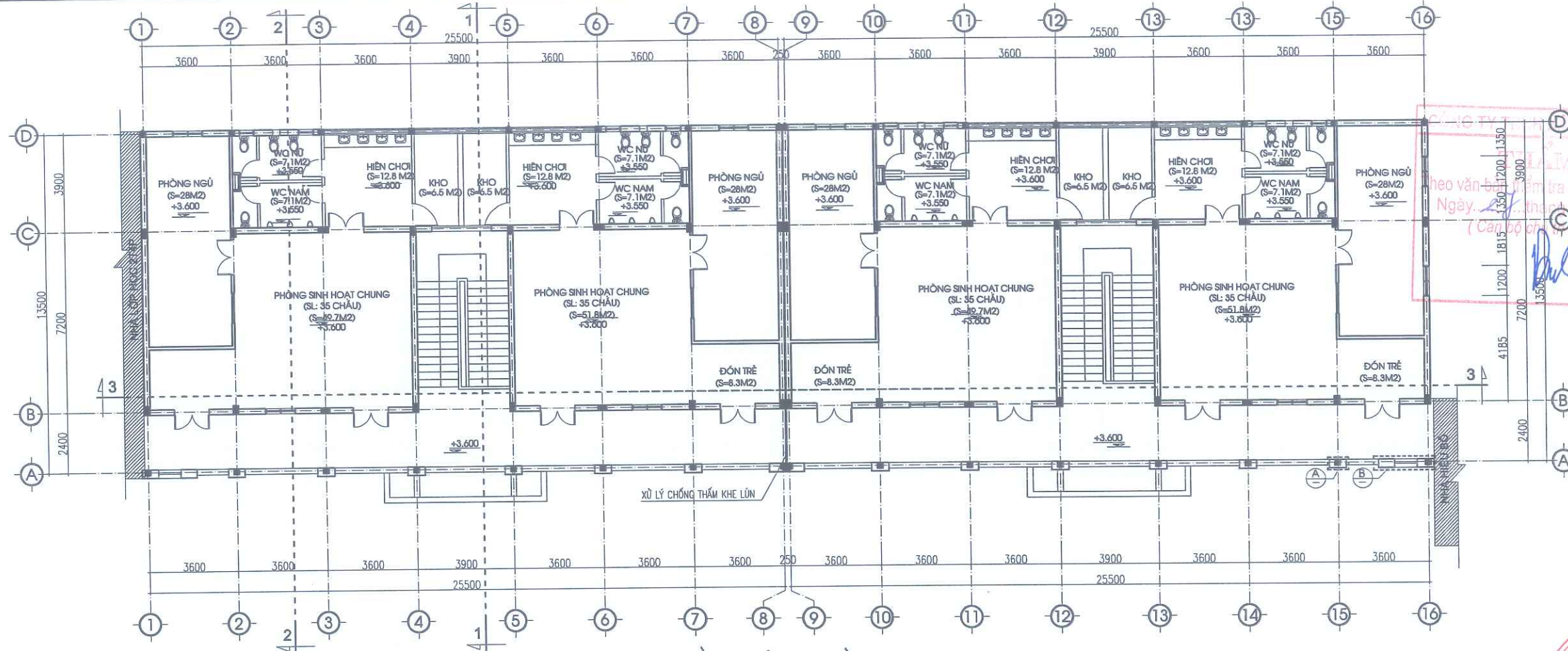
MẶT BẰNG CẢI TẠO TẦNG 2
