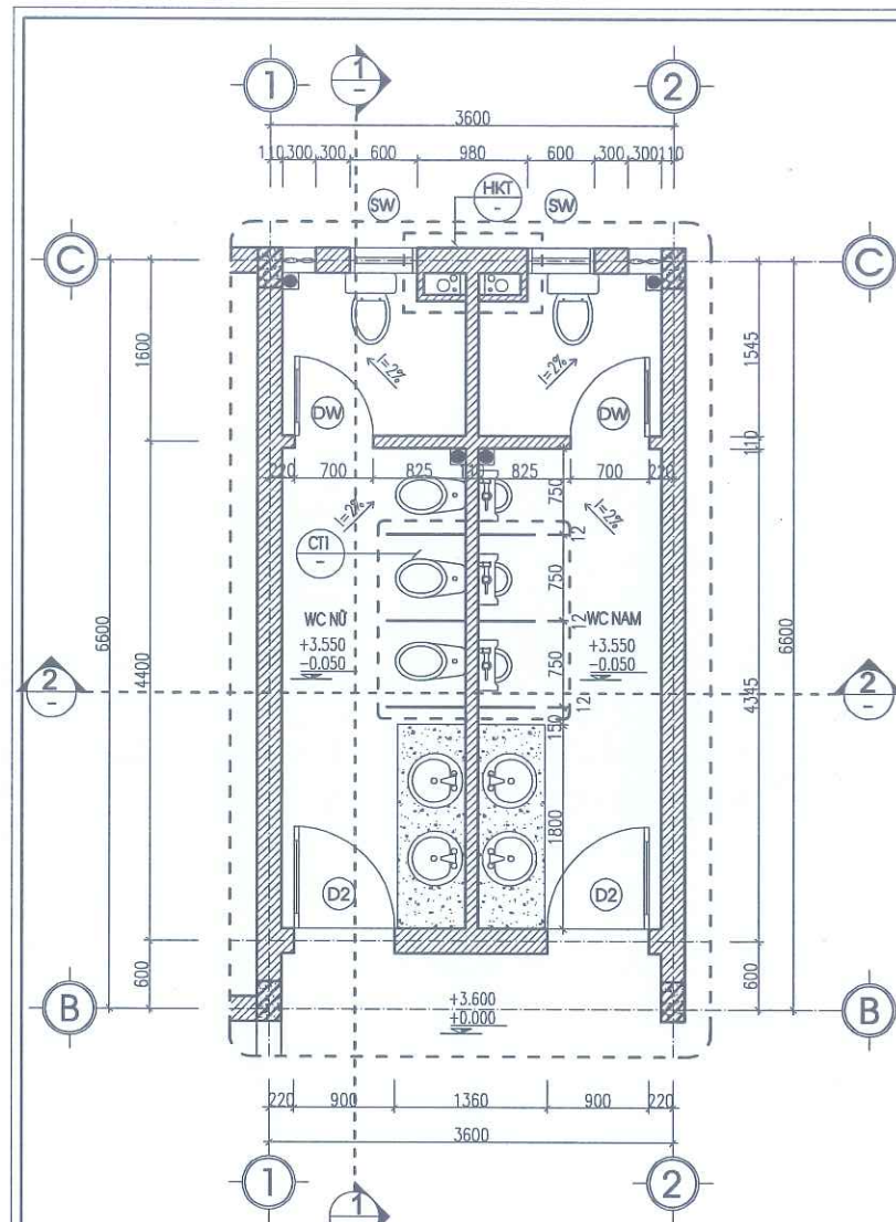
MẶT BẰNG VỆ SINH ĐIỂN HÌNH
