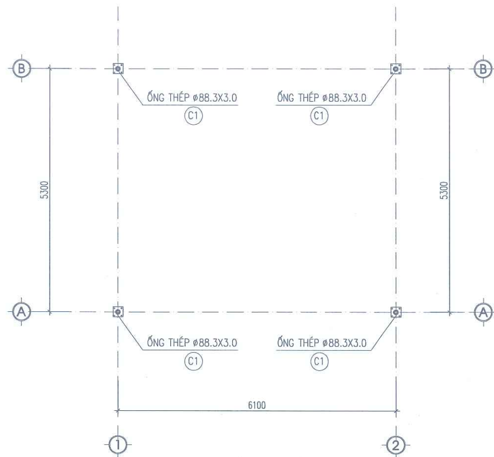
MẶT BẰNG CỘT THÉP SL= 02 CK
