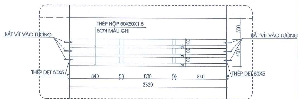
CHI TIẾT THÉP HỘP TRANG TRÍ ĐIỂN HÌNH
