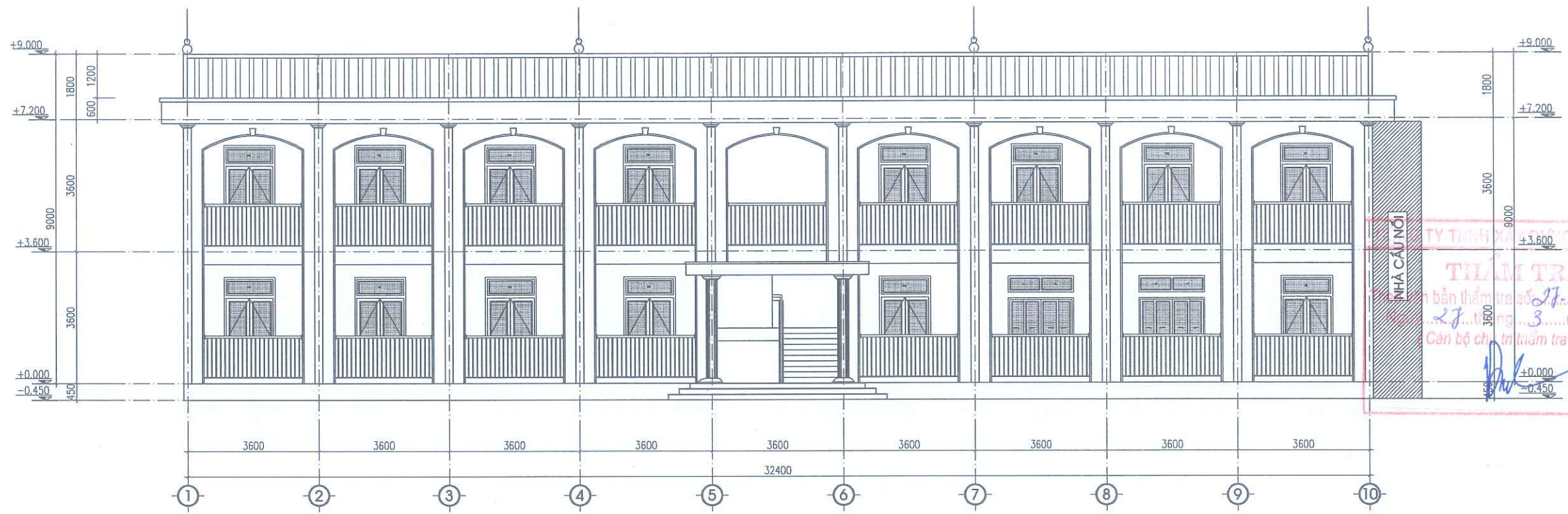
MẶT ĐỨNG TRỰC 1-10
