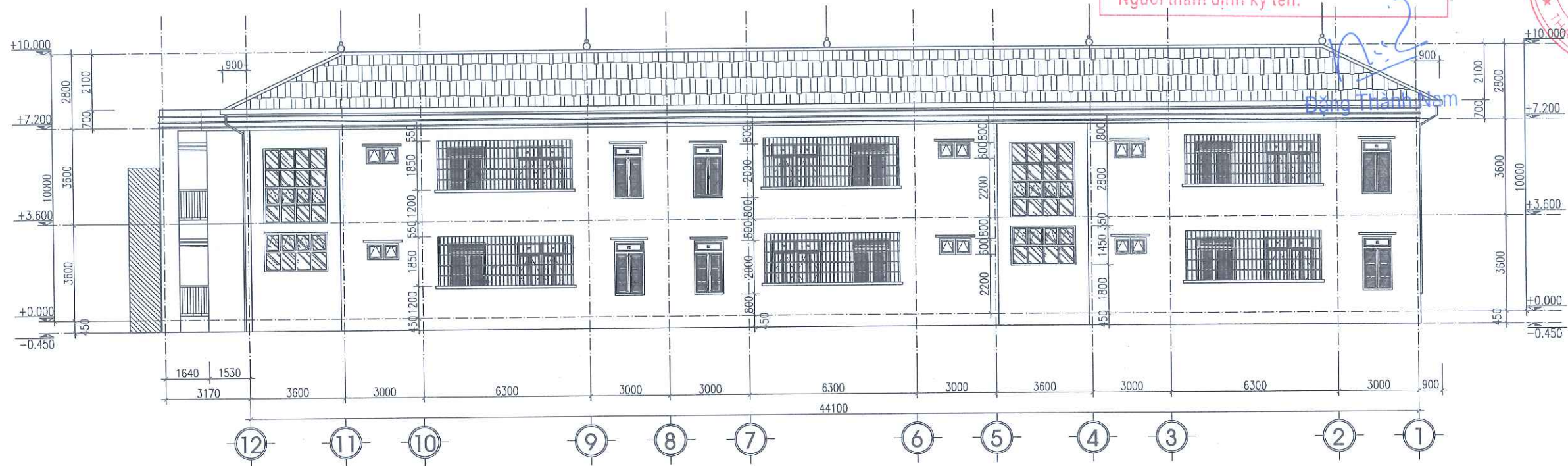
MẶT ĐÚNG TRỤC 12-1
