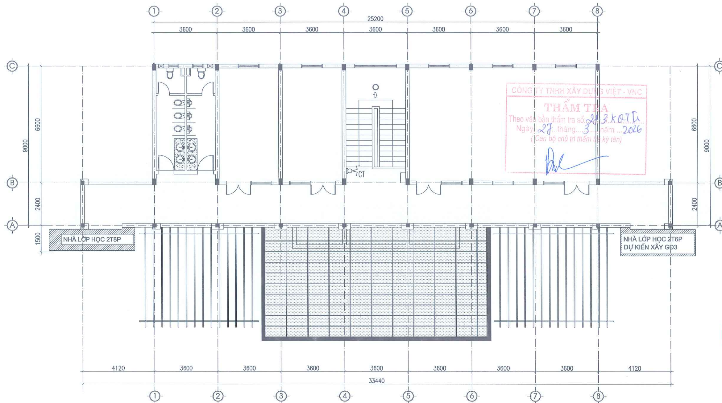
MẶT BẰNG CẢI TẠO ĐIỆN TẦNG 2
