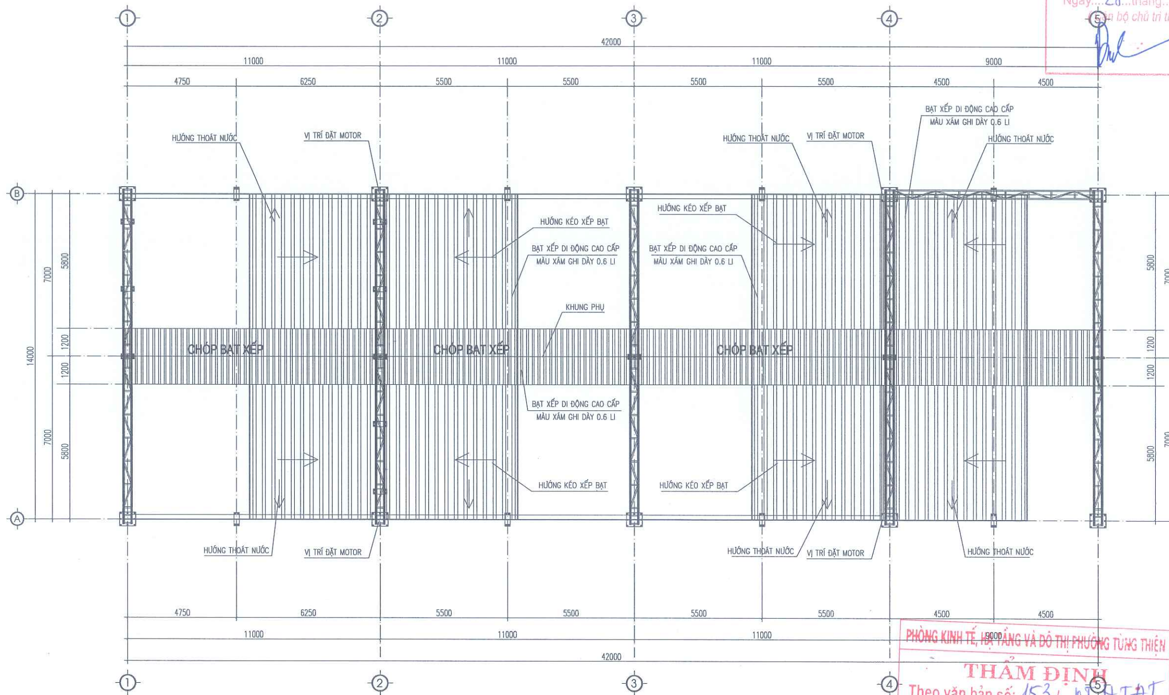
MẶT BẰNG MÁI BẠT CHE
