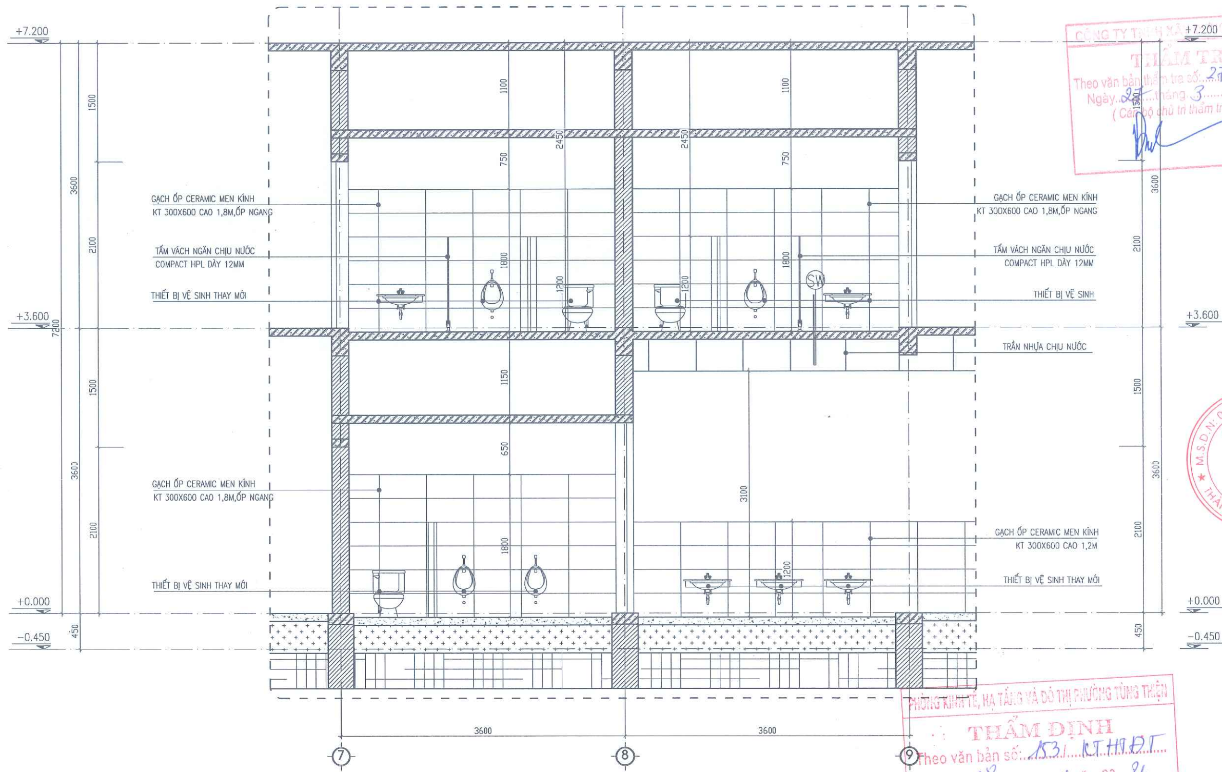
MẶT CẮT 3-3
