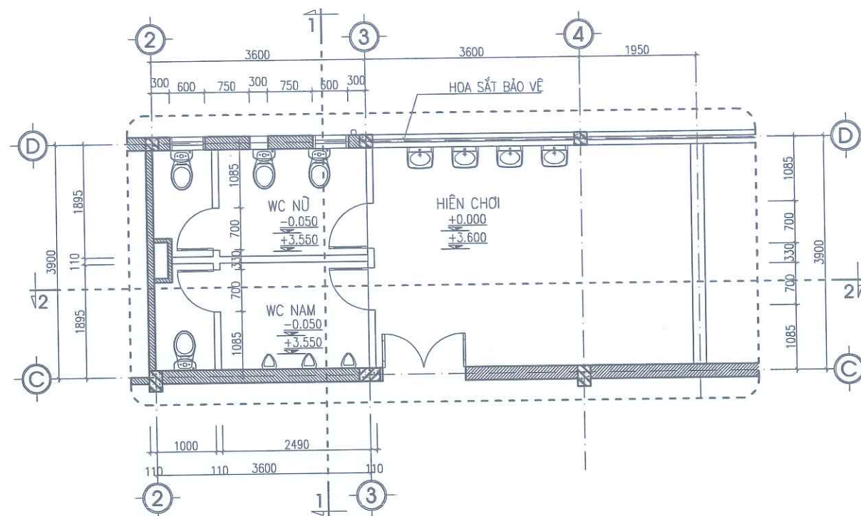
MẶT BẰNG ĐIỂN HÌNH KHU VỆ SINH
