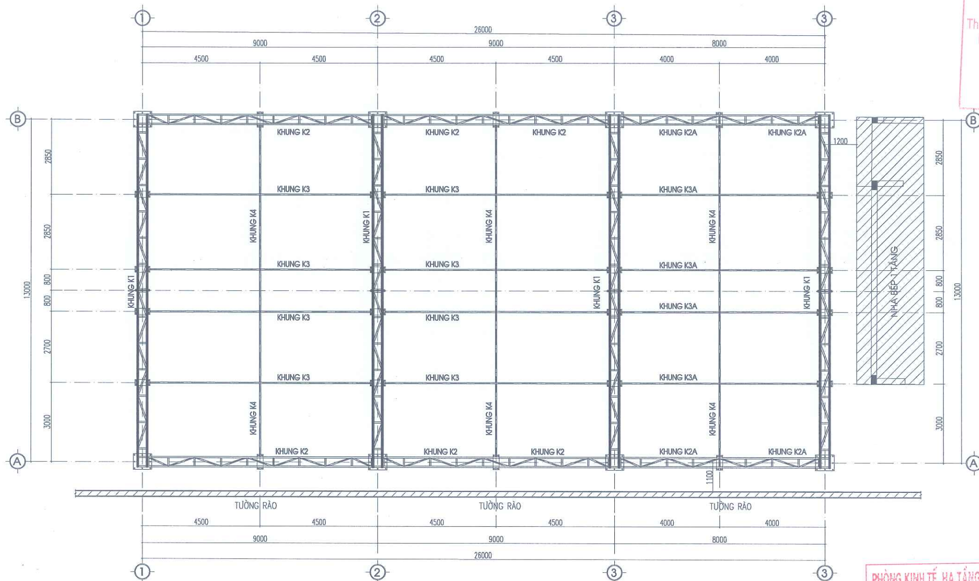
MẶT BẰNG KẾT CẤU KHUNG THÉP MÁI
