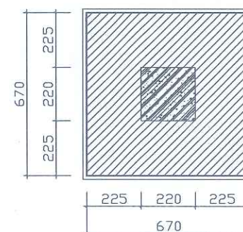
CẮT 1-1
