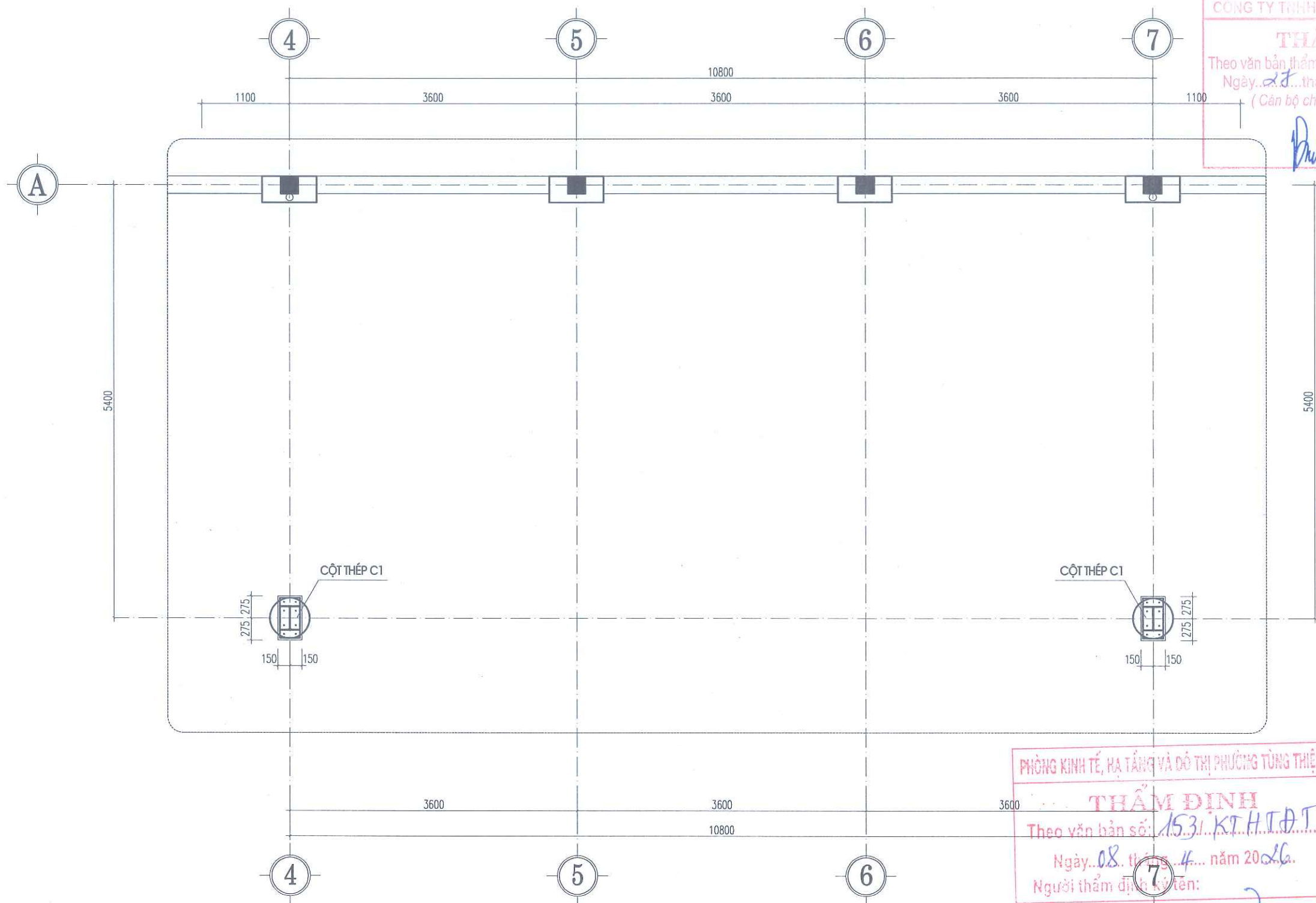
MẶT BẰNG ĐỊNH VỊ CỘT THÉP
