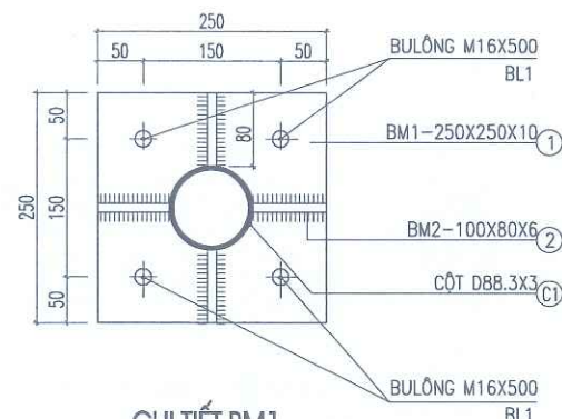
CHI TIẾT BM1
