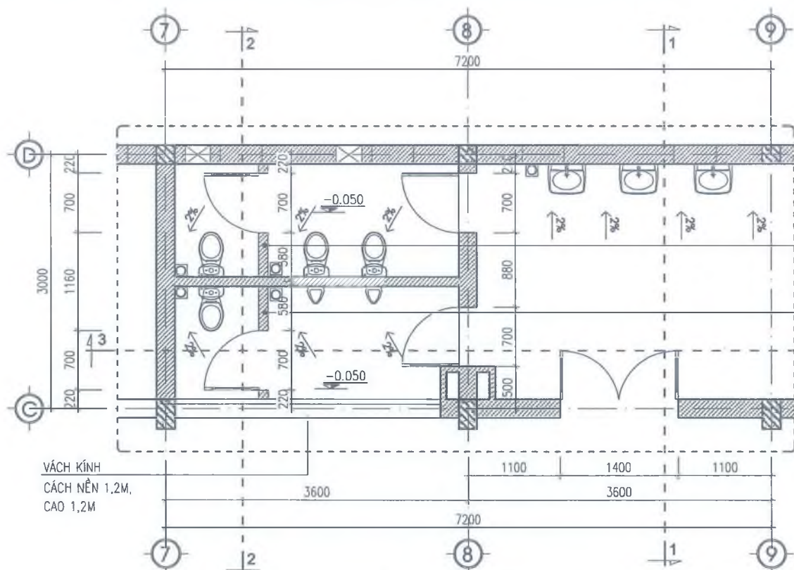
MẶT BẰNG VỆ SINH TẦNG 1 SỐ 2
