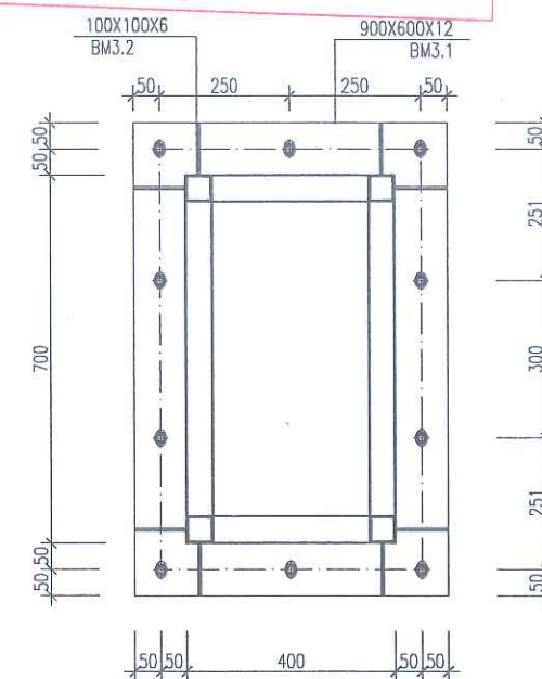
CHI TIẾT BẢN MÃ BM3.1
