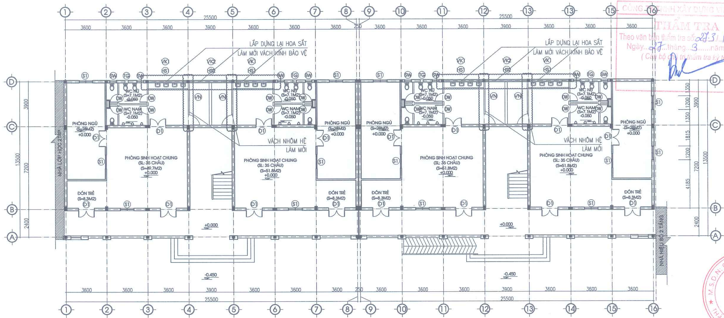
MẶT BẰNG CỦA TẦNG 1
