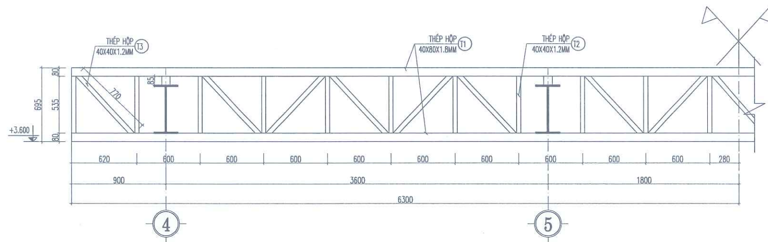
CHI TIẾT KHUNG THÉP K4 ( SL : 01 C.KIỆN)
