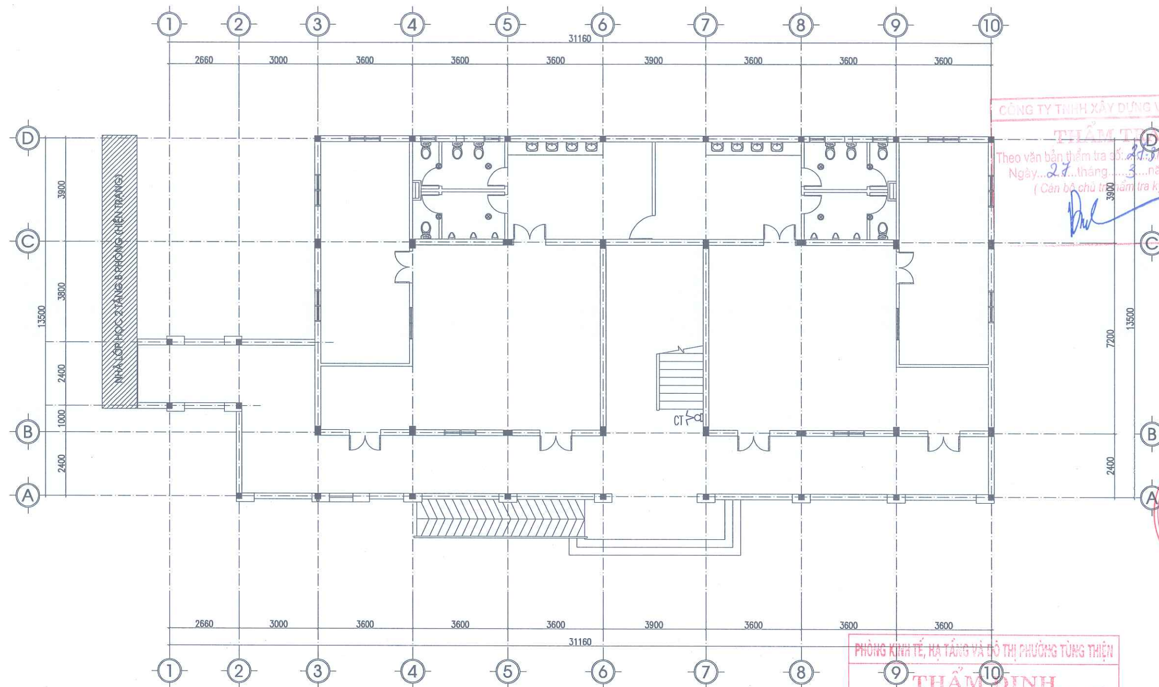
MẶT BẰNG CẢI TẠO ĐIỆN TẦNG 1
