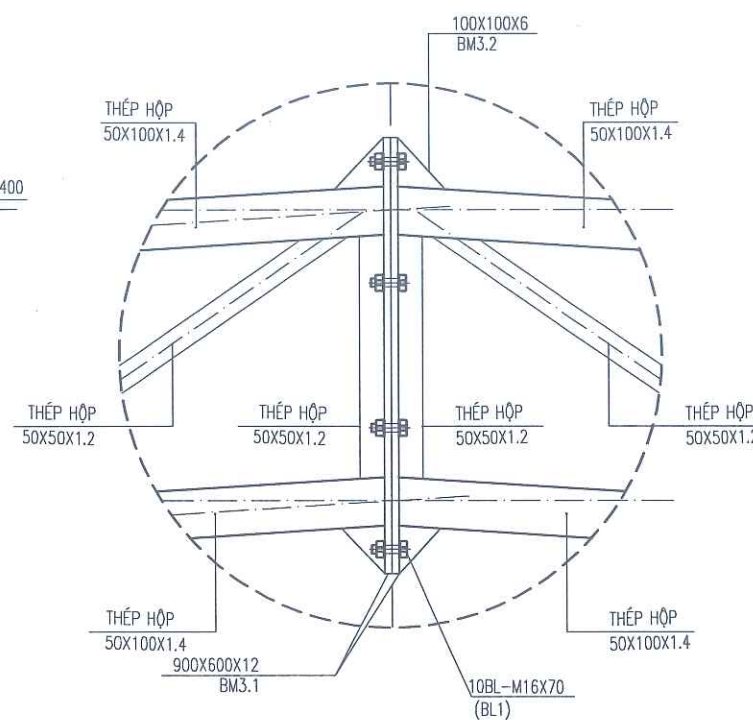
CHI TIẾT CT3
