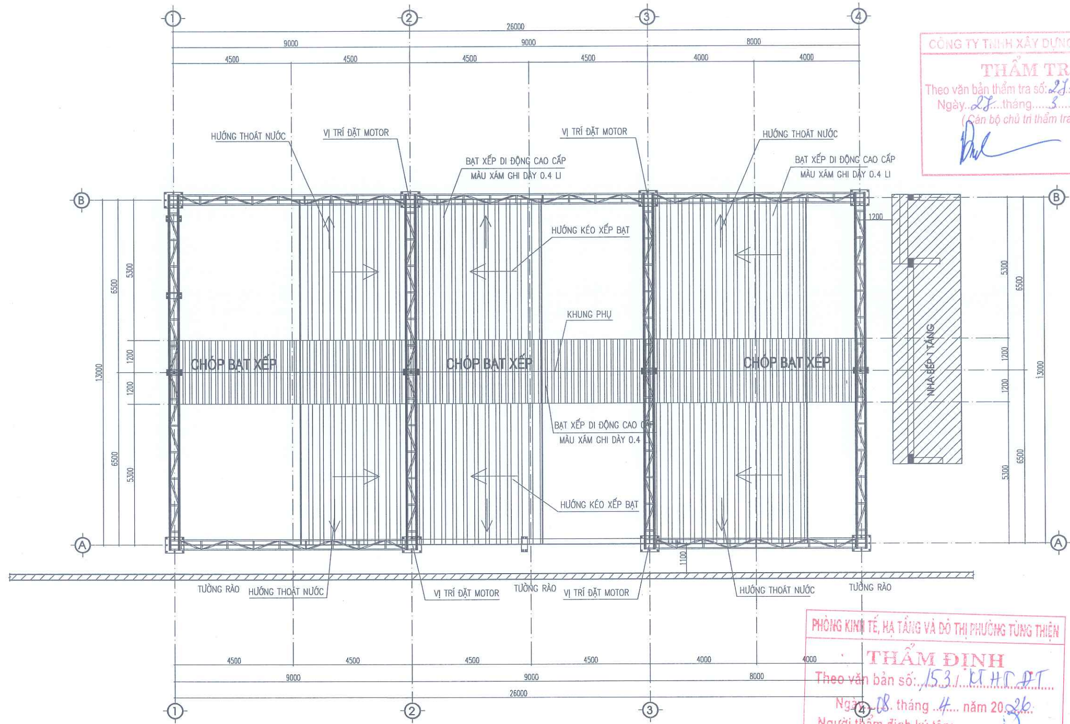
MẶT BẰNG MÁI BẠT CHE
