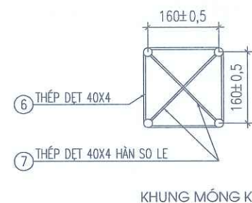
KHUNG MÓNG K1
