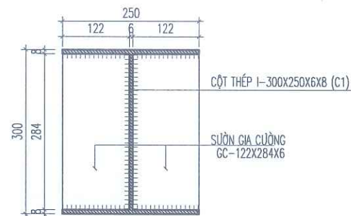
MẶT CẮT 2-2
