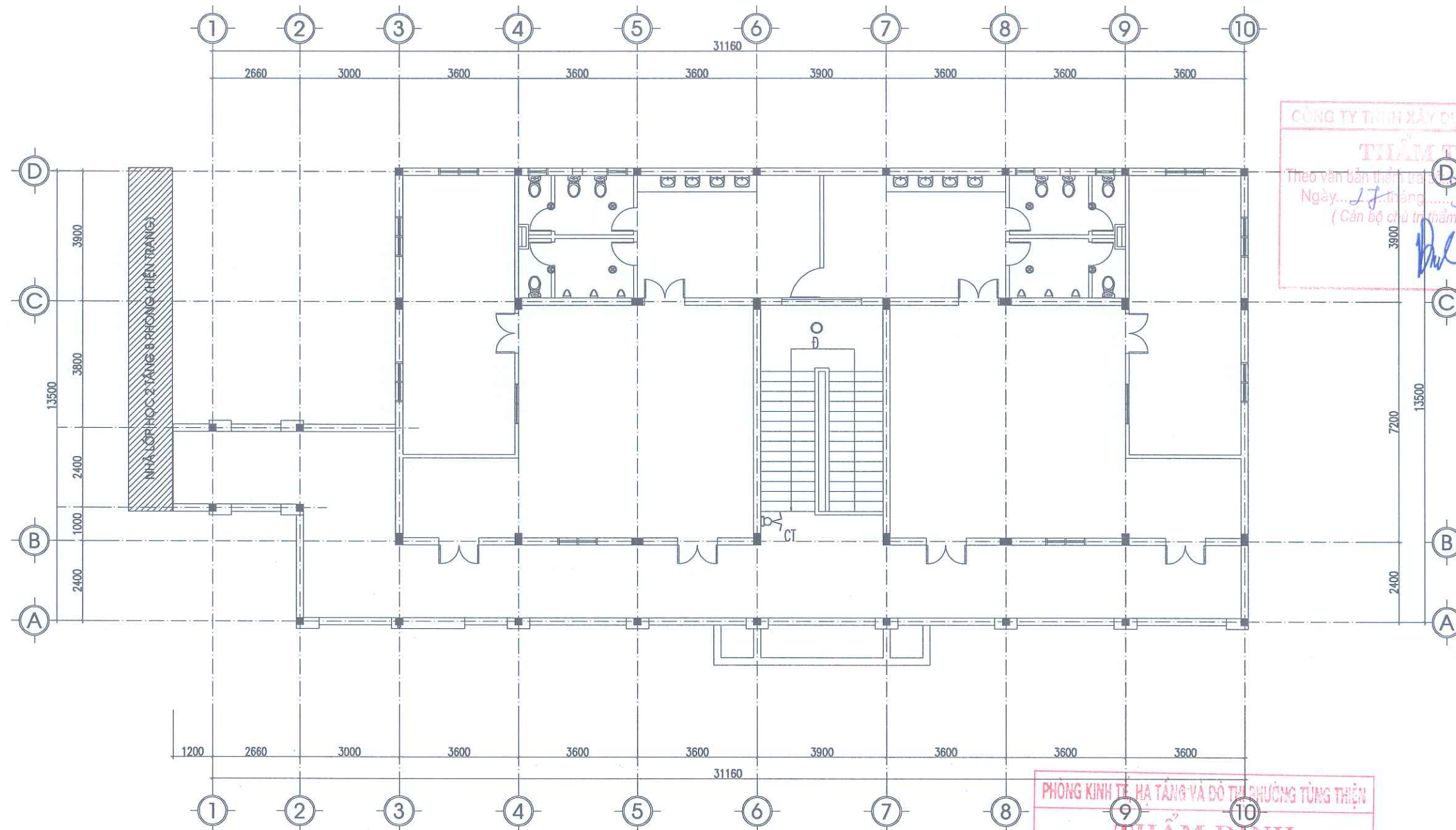
MẶT BẰNG CẢI TẠO ĐIỆN TẦNG 2
