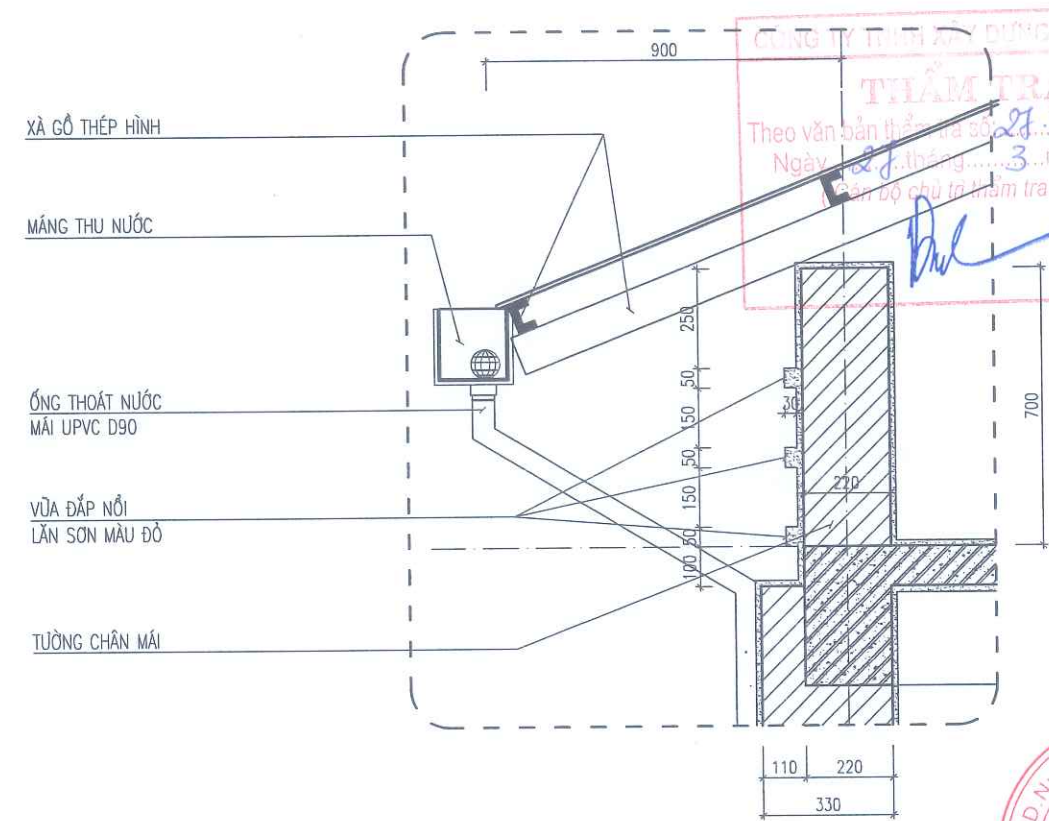
CHI TIẾT MÁNG THU NƯỚC (CHI TIẾT A)
