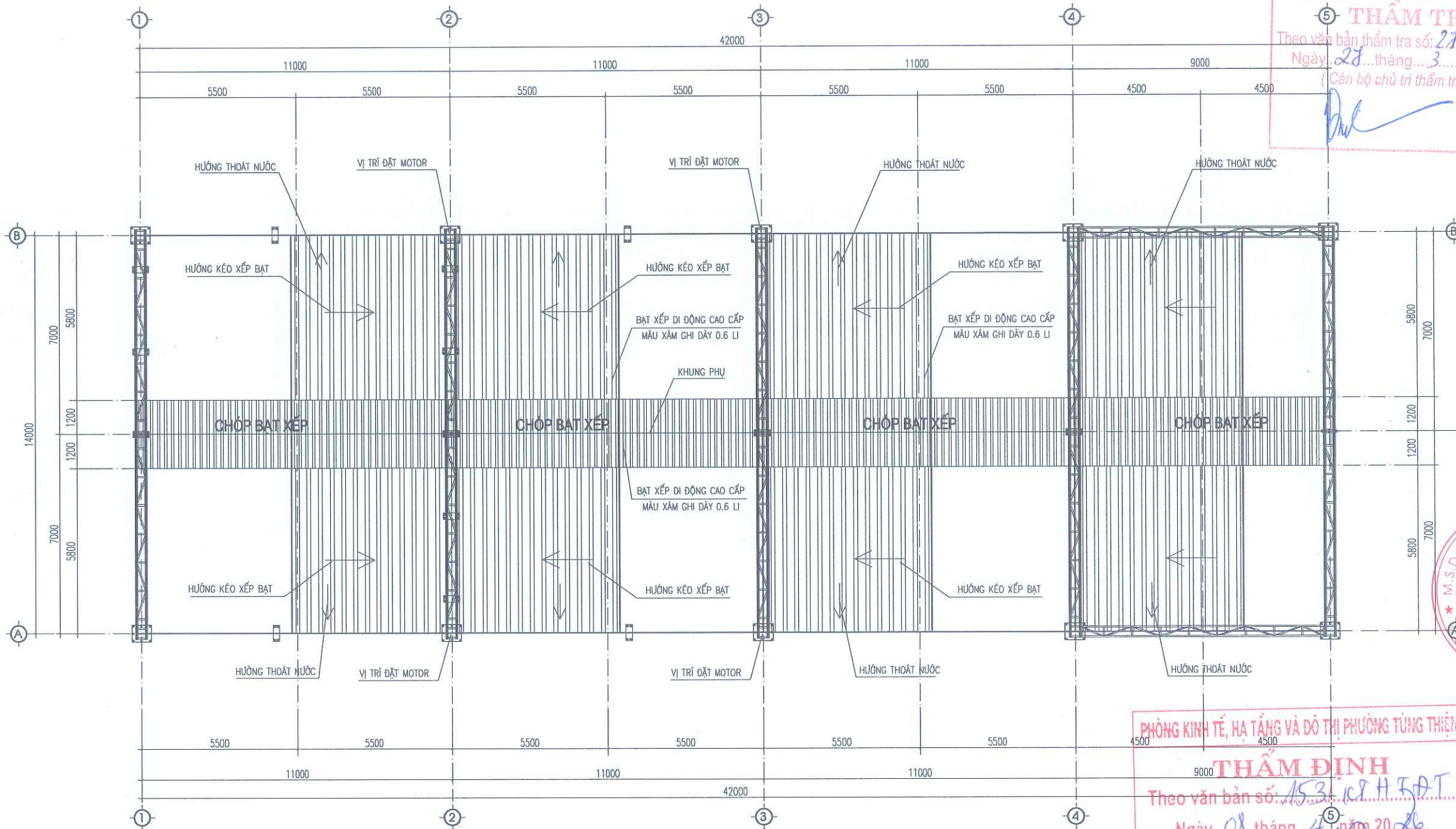
MẶT BẰNG MÁI BẠT CHE
