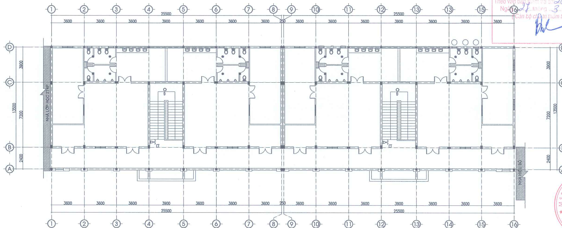
MẶT BẰNG CẢI TẠO ĐIỆN TẦNG 2
