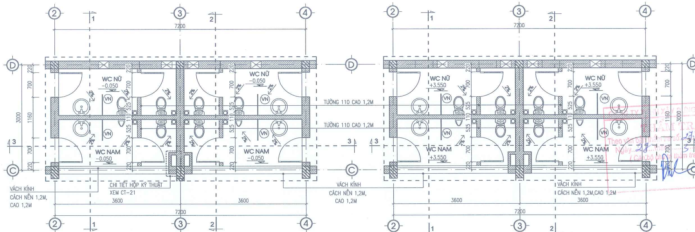
MẶT BẰNG VỆ SINH TẦNG 1 SỐ 1
