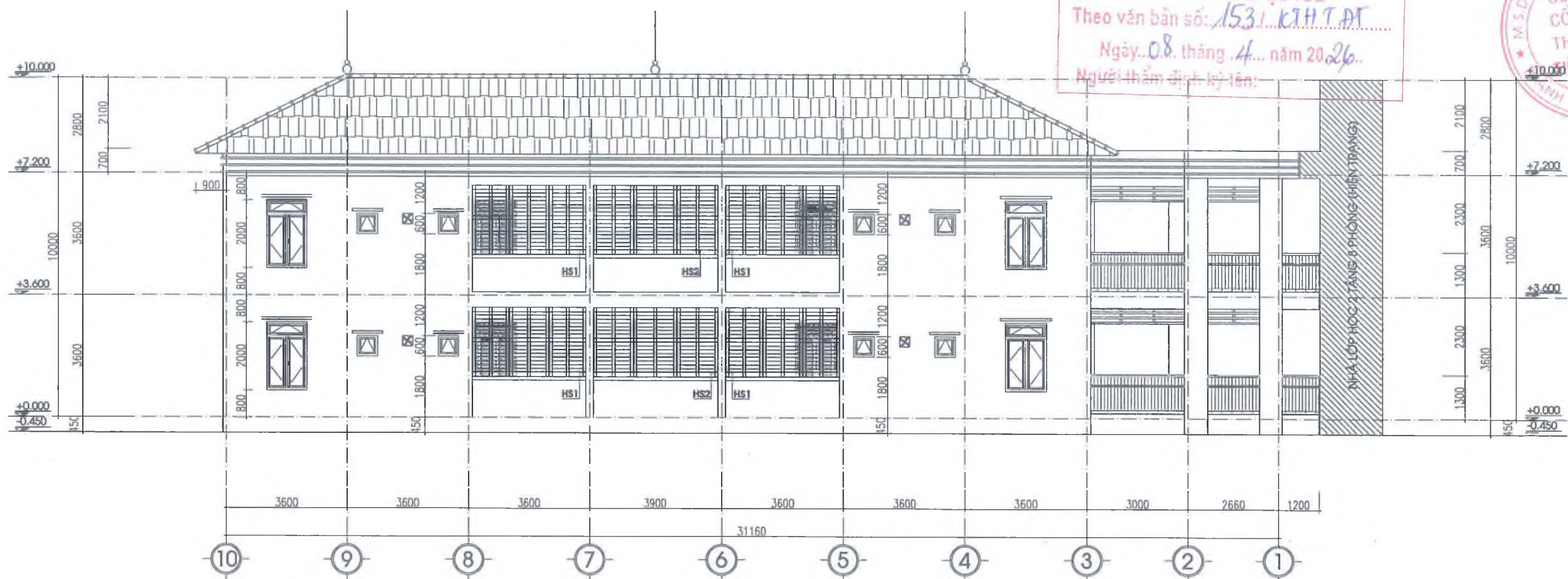
MẶT ĐÚNG TRỰC 1-10
