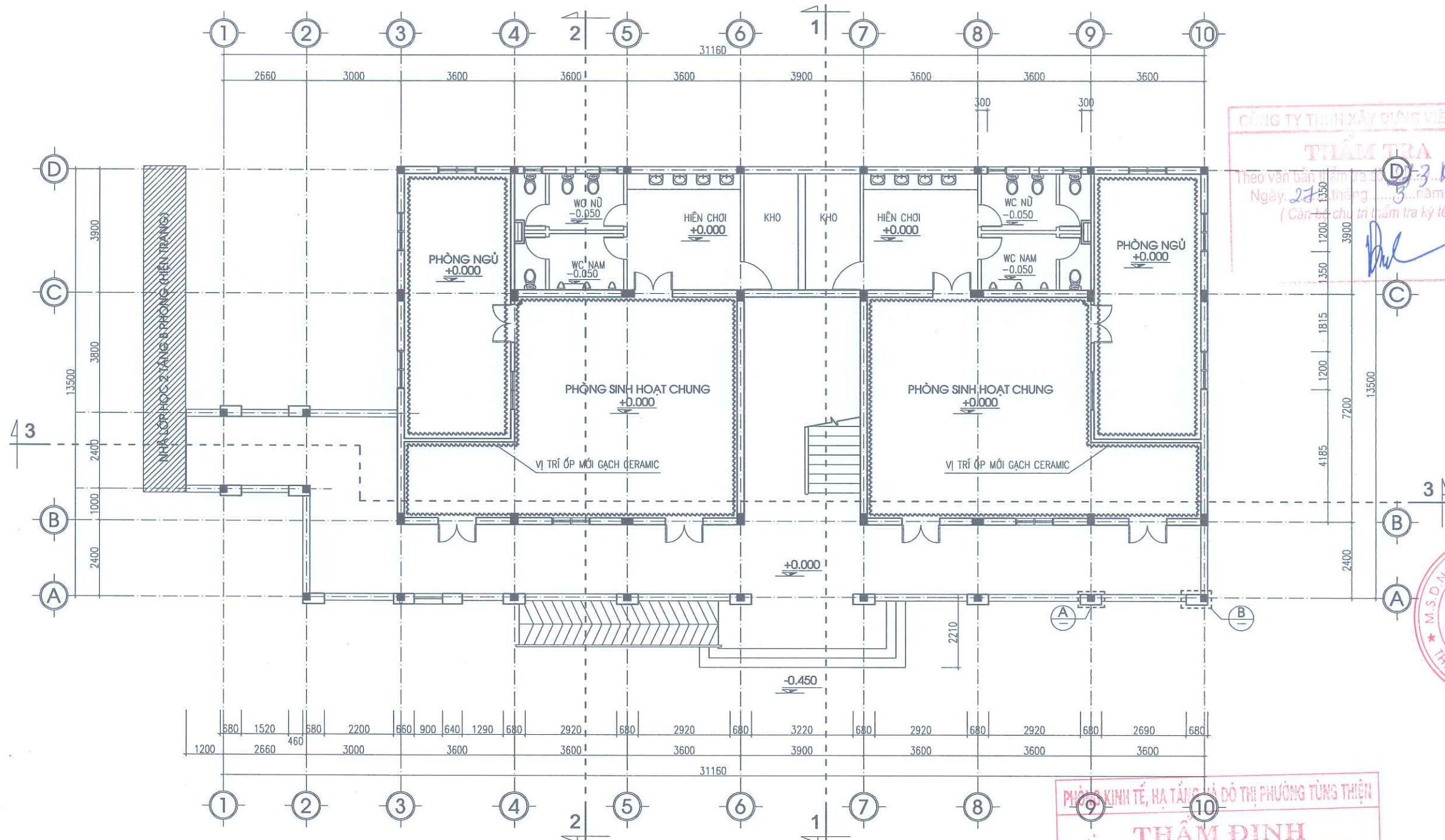
MẶT BẰNG CẢI TẠO TẦNG 1
