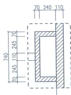
CHI TIẾT HỘP KỸ THUẬT
