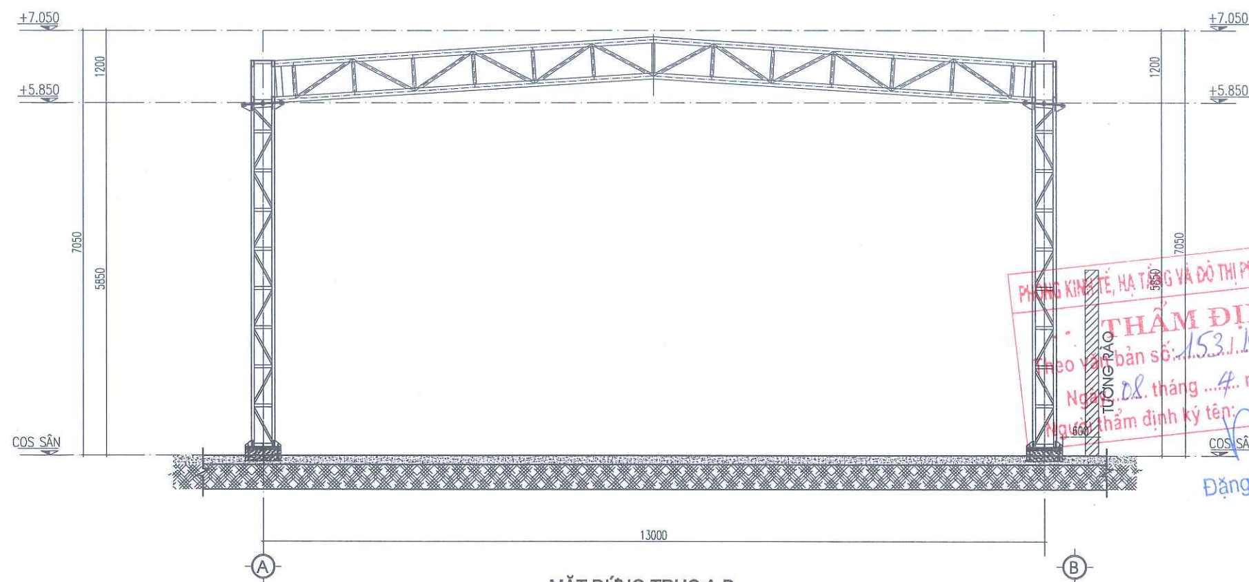
MẶT ĐỨNG TRỰC A-B
