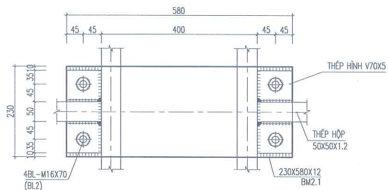
MẶT CẮT 2-2
