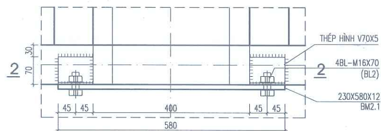
CHI TIẾT CT2
