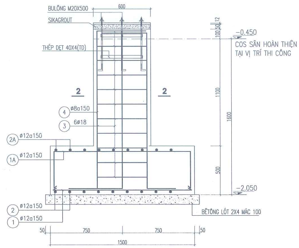
MẶT CẮT 1-1
