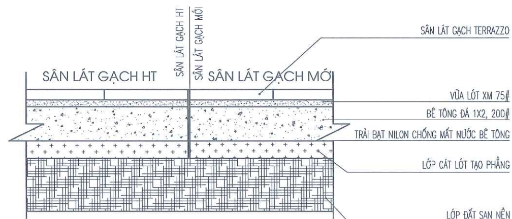
MẶT CẮT VỊ TRÍ TIẾP GIÁP VỚI SÂN BÊ TÔNG (PHÍA TRƯỚC CỔNG)
