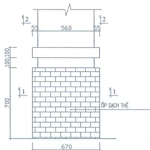
CHI TIẾT 01
