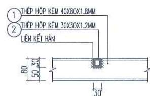
CHI TIẾT LIÊN KẾT THÉP HỘP
