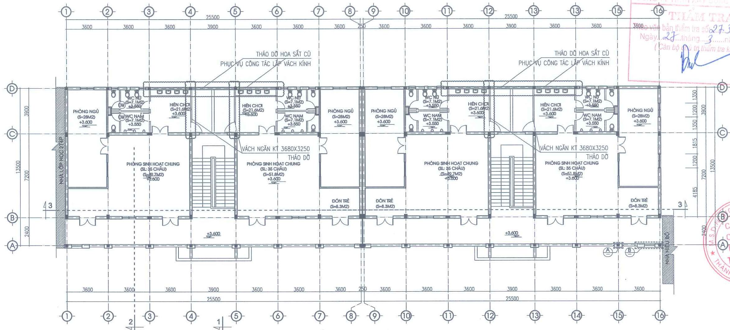
MẶT BẰNG PHÁ DỠ TẦNG 2
