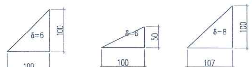
BẢN MẪ T1 BẢN MẪ T2
