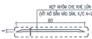
CHI TIẾT NẸP NHÔM
