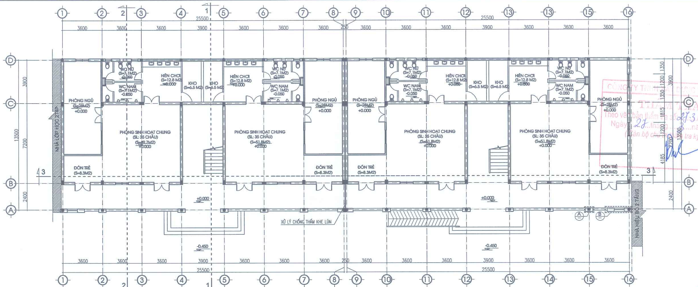
MẶT BẰNG CẢI TẠO TẦNG 1
