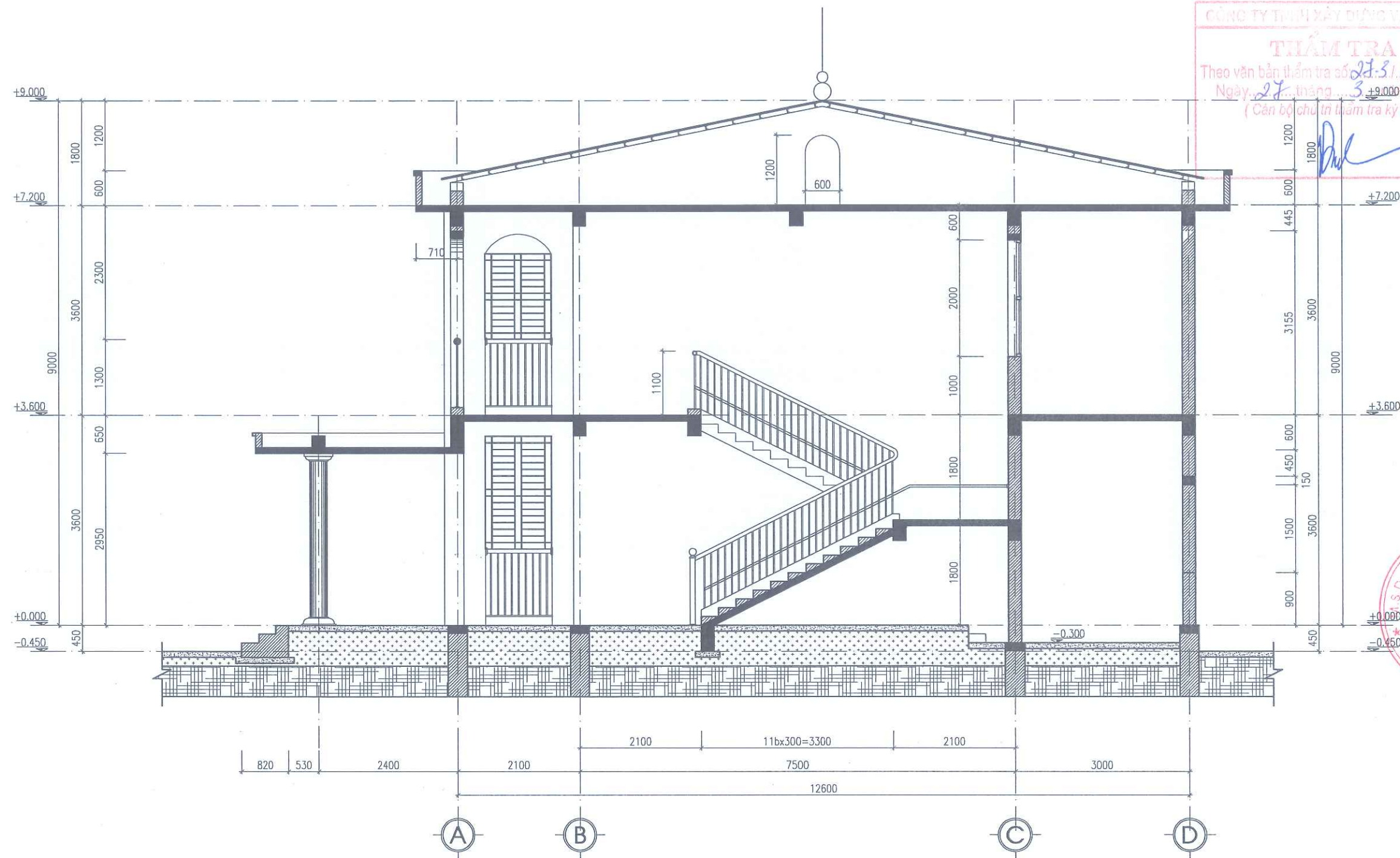
MẶT CẮT 3-3
