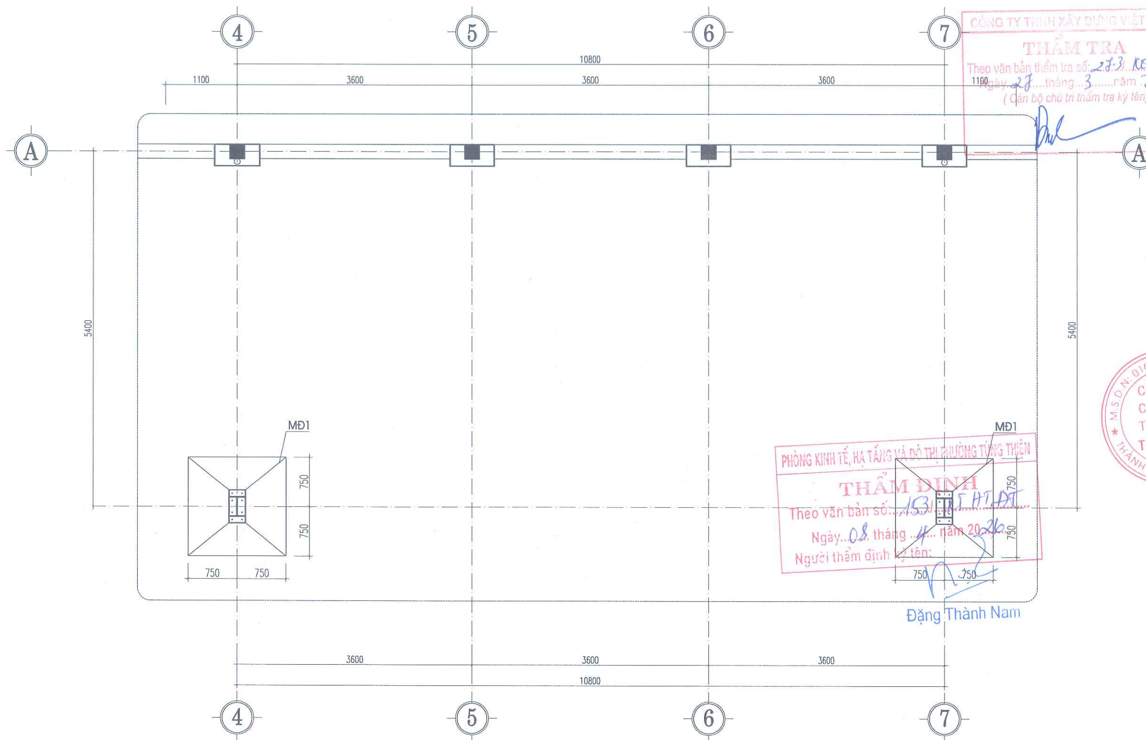
MẶT BẰNG KẾT CẤU MÓNG
