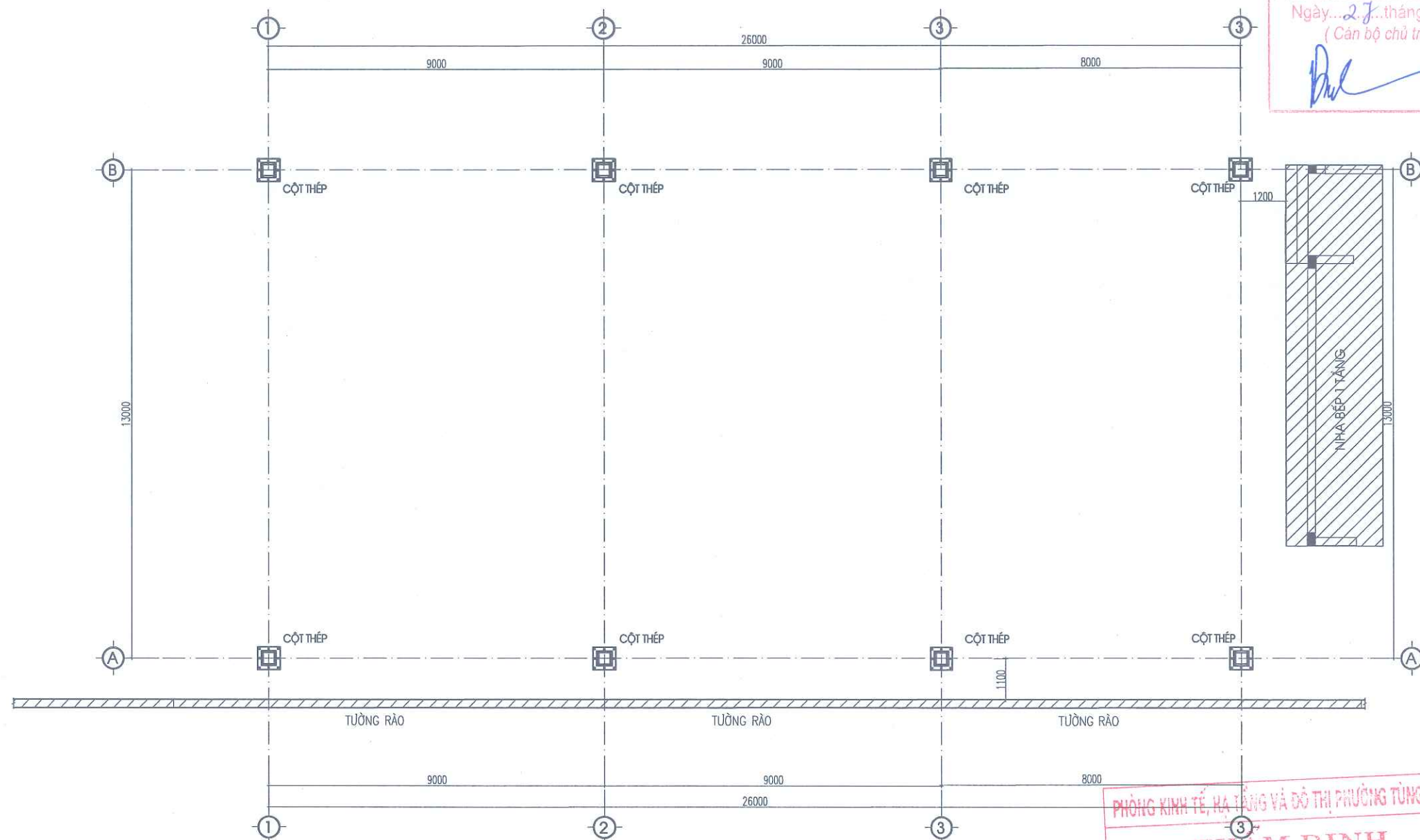
MẶT BẰNG ĐỊNH VỊ CỘT
