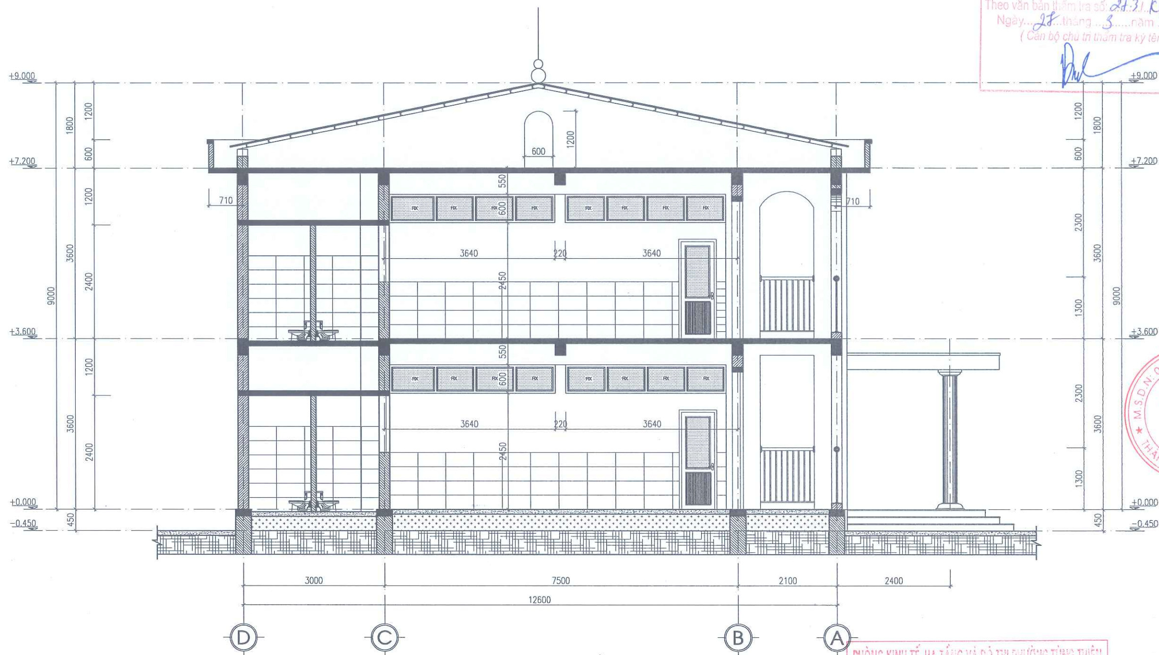
MẶT CẮT 2-2
