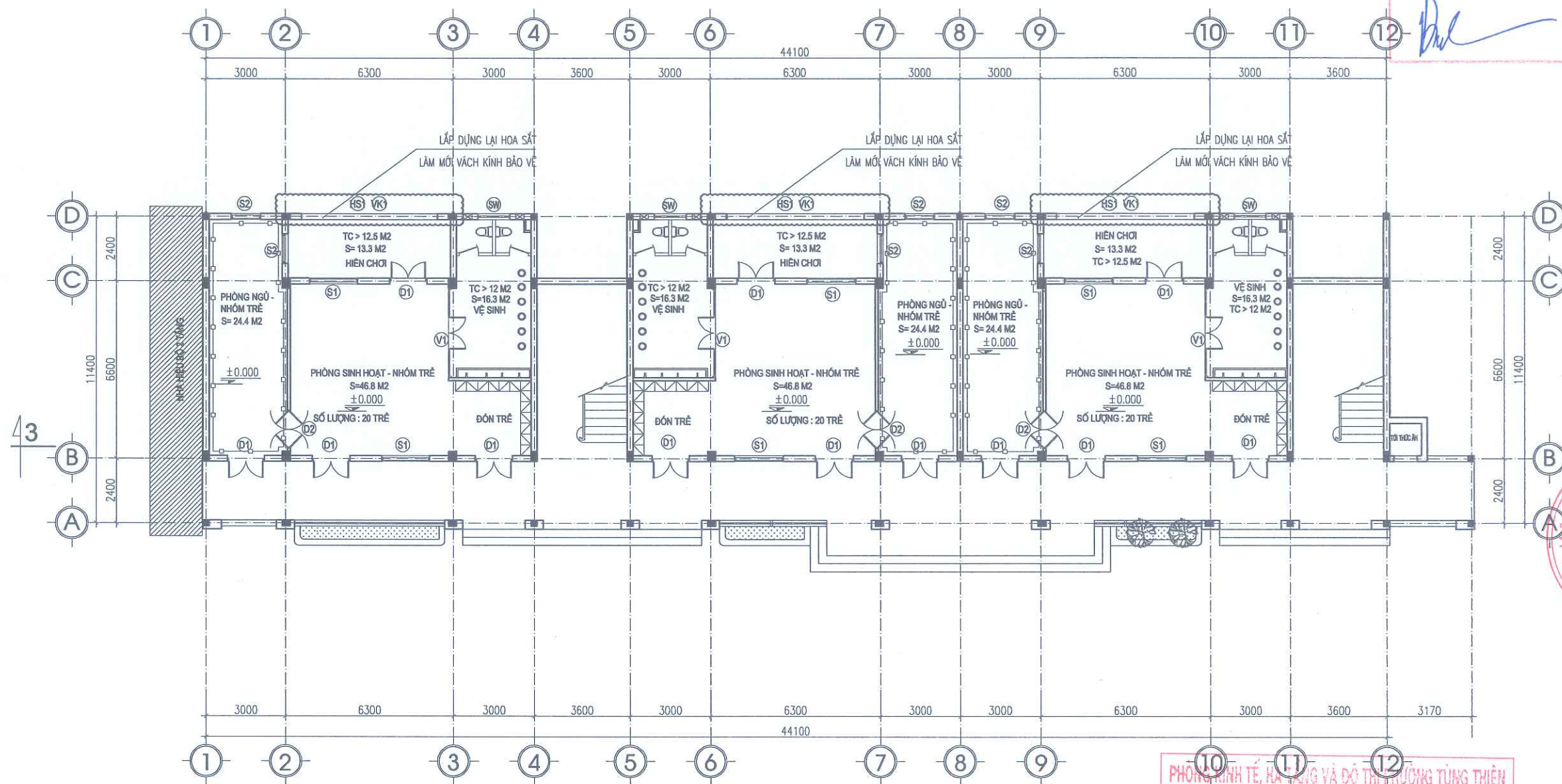
MẶT BẰNG CỦA TẦNG 1
