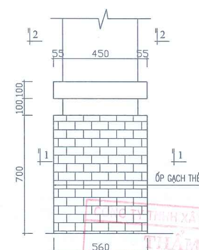
CHI TIẾT 02
