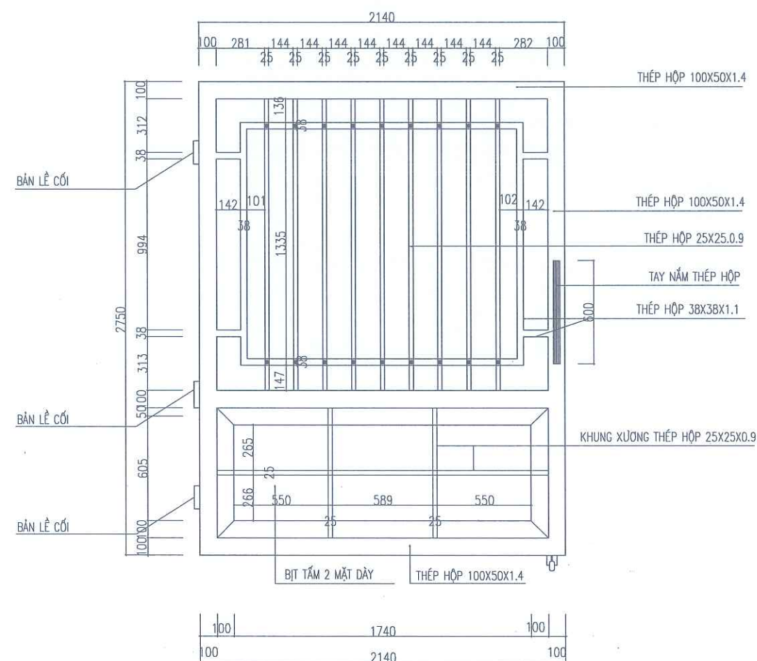
CHI TIẾT CẢNH CỔNG CHÍNH (SL=02CK)
