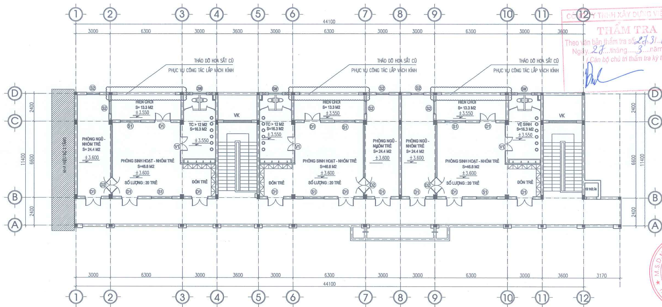
MẶT BẰNG PHÁ DỠ TẦNG 1
