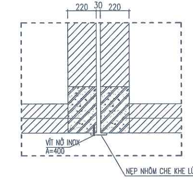
CHI TIẾT CHE KHE TIẾP GIÁP TƯỜNG L= 9.5 M
