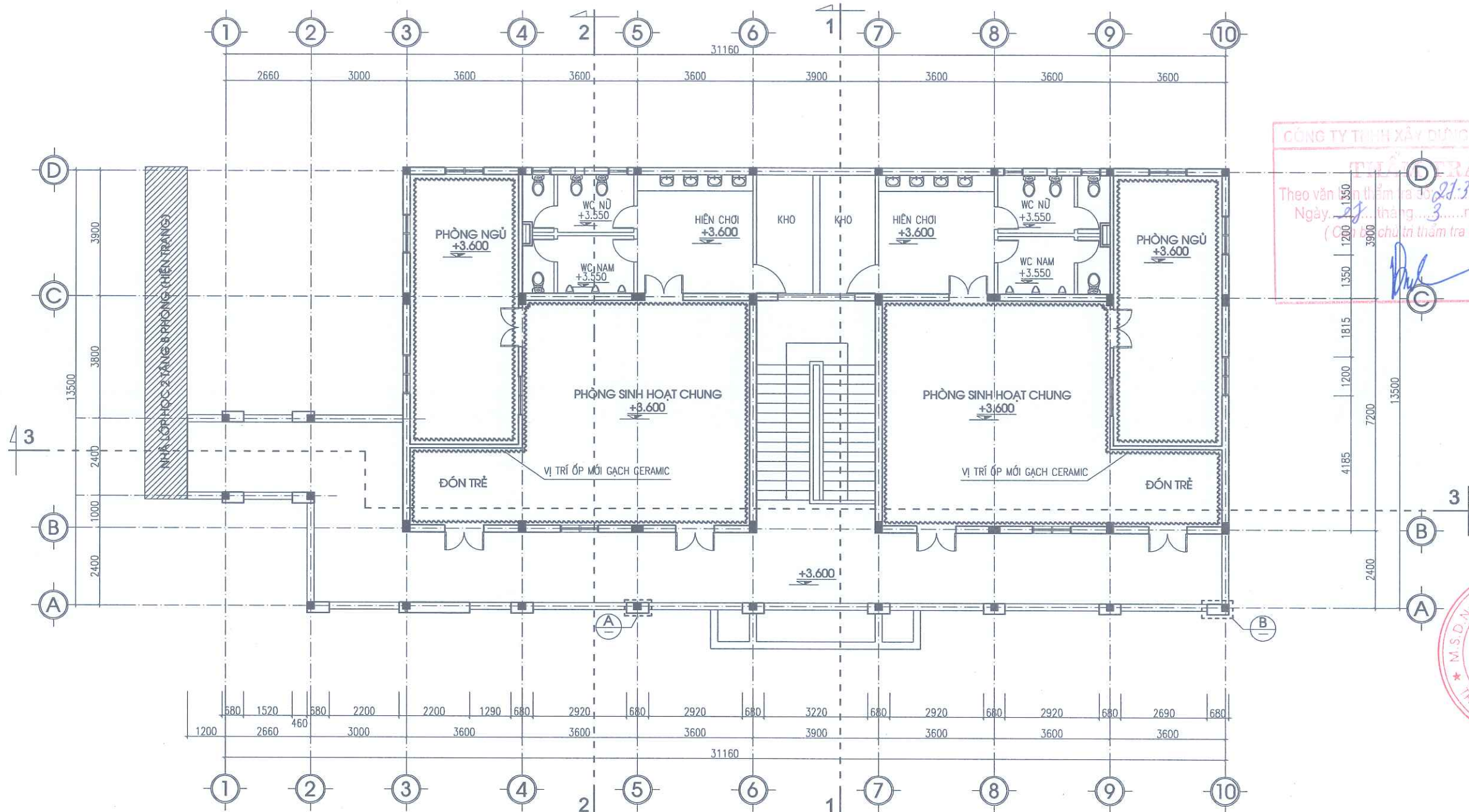
MẶT BẰNG CẢI TẠO TẦNG 2
