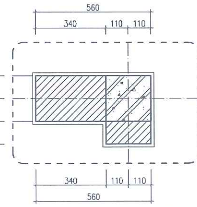
CHI TIẾT 5
