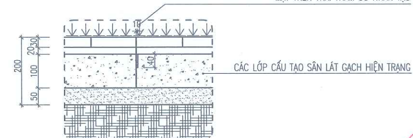
MẶT CẮT ĐIỂN HÌNH SÂN LÁT GẠCH TRẢI THẨM CỎ NHÂN TẠO, SÂN S1 DIỆN TÍCH : SA = 1116.0 M2
