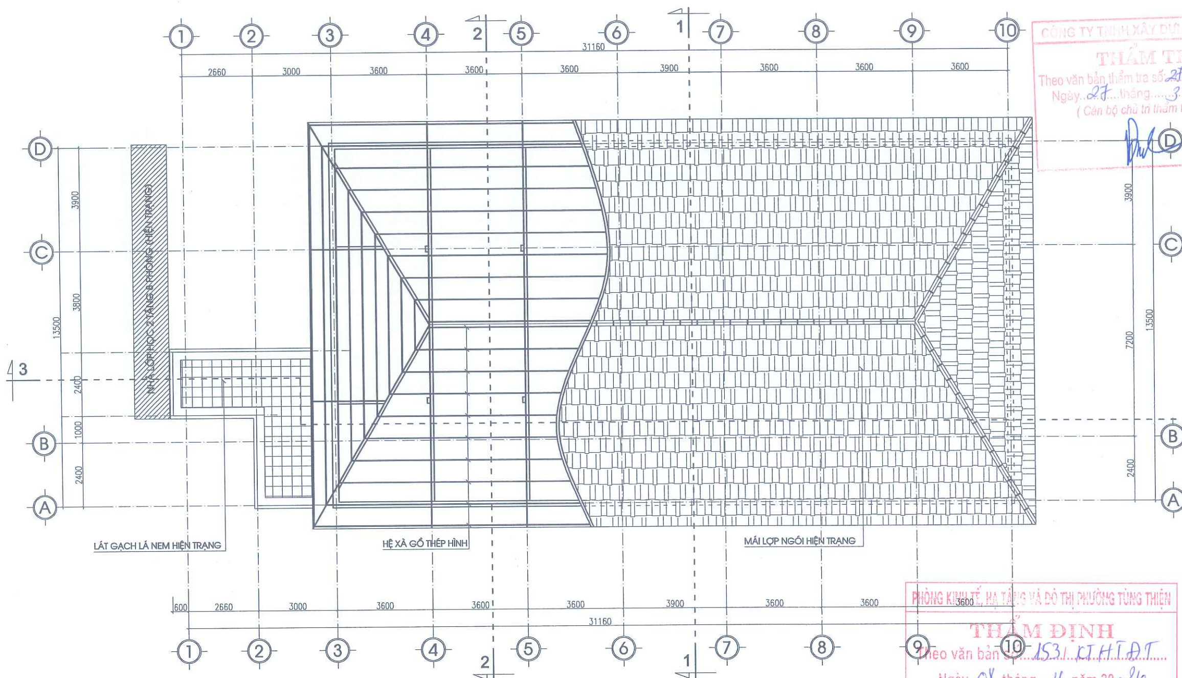
MẶT BẰNG MÁI
