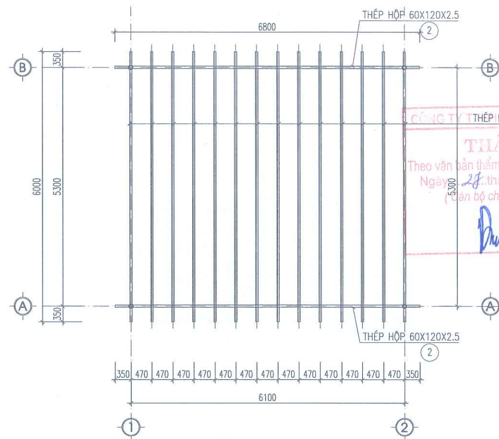
MẶT BẰNG THÉP HỘP COS +4.100 SL= 02 CK
