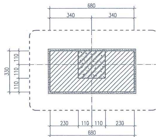
CHI TIẾT 2
