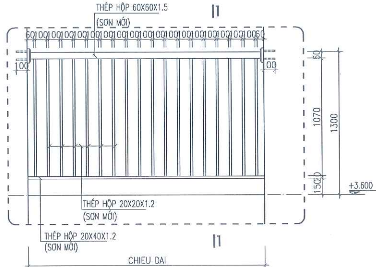
CHI TIẾT LAN CÁN ĐIỂN HÌNH TẦNG 2 L=37.6M
