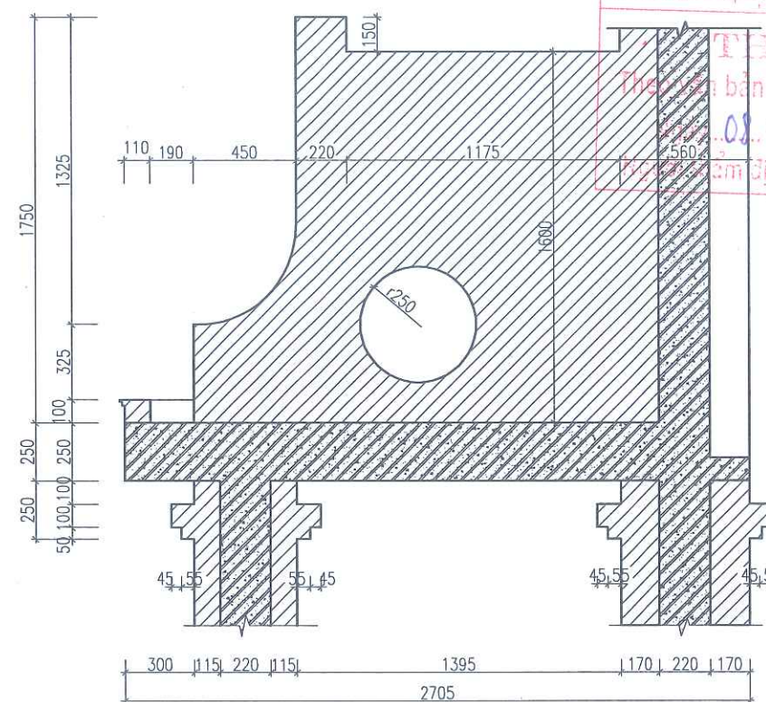
CẮT 1-1
