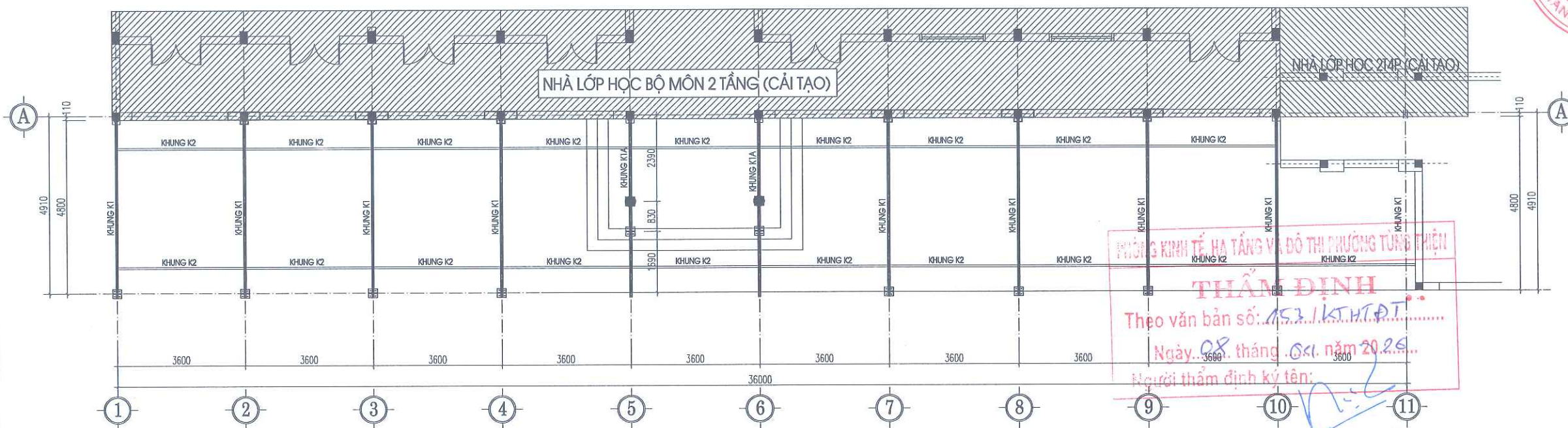
MẶT BẰNG KẾT CẤU KHUNG THÉP MÁI CHE
