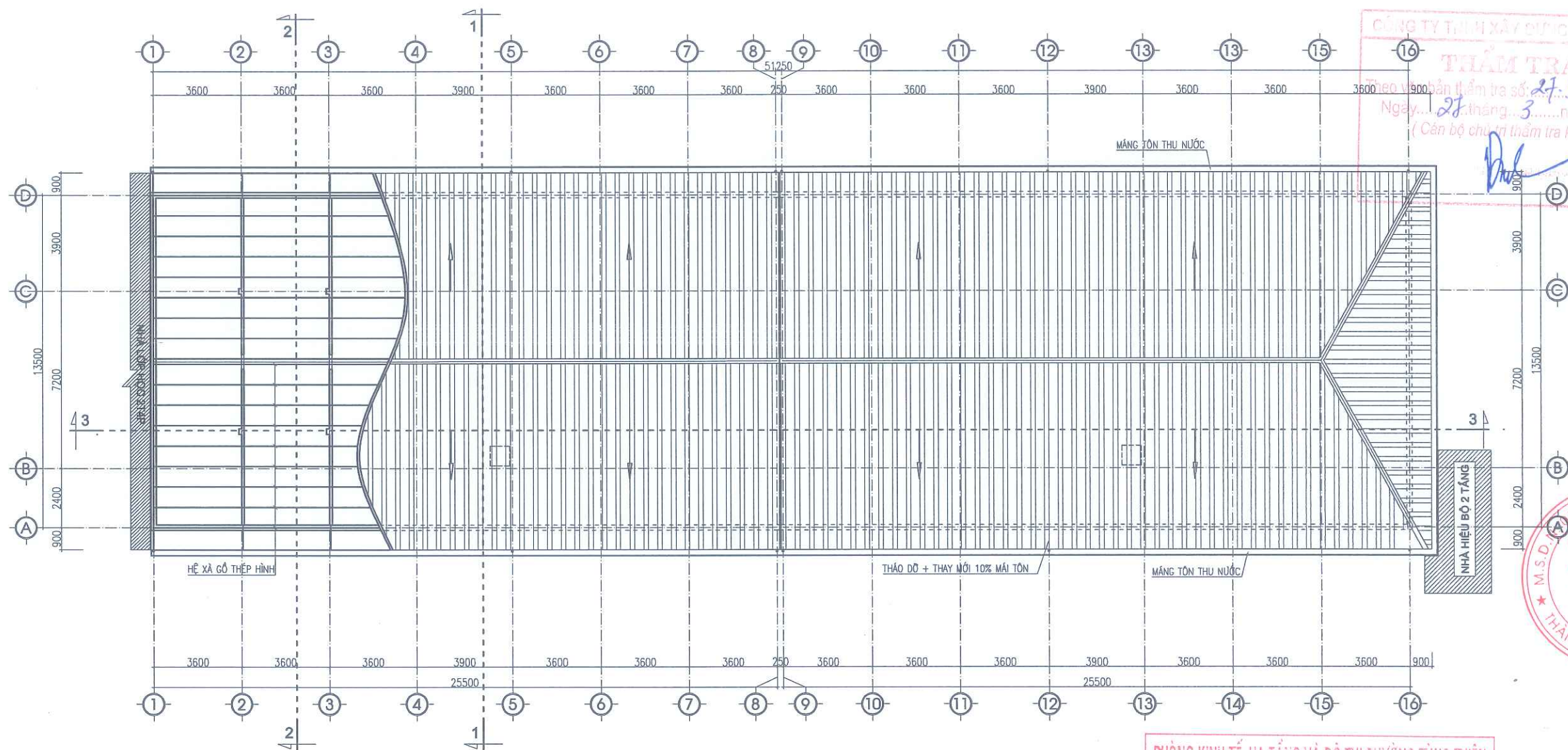
MẶT BẰNG MÁI
