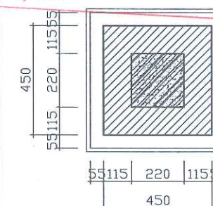
CẮT 2-2
