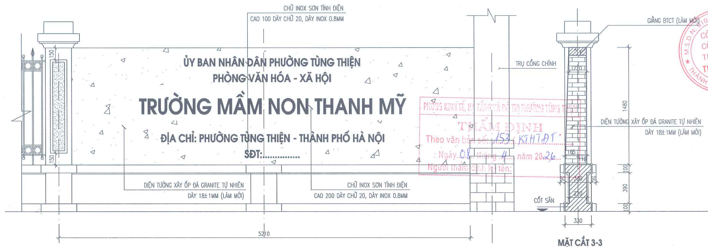
CHI TIẾT TƯỜNG RÀO CẢI TẠO
