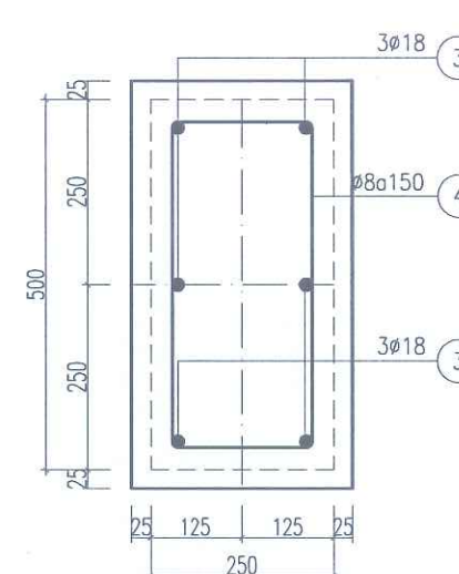
MẶT CẮT 2 - 2
