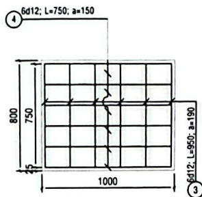
CHI TIẾT CỐT THÉP TẤM ĐAN-LỚP TRÊN TL: 1/25
