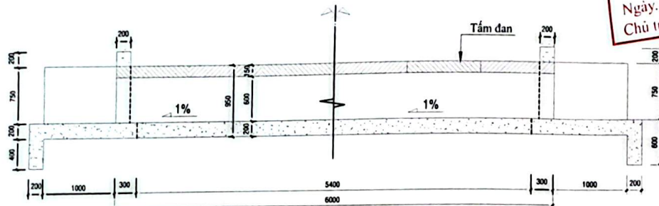
MẶT CẮT A-A TL: 1/50
