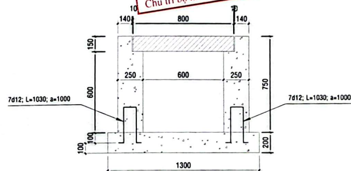
MẶT CẮT B-B TỶ LỆ: 1/25
