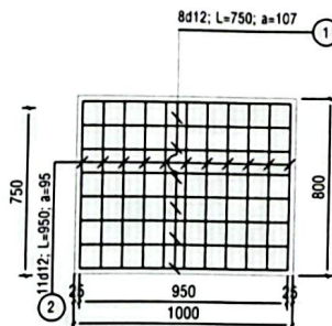
CHI TIẾT CỐT THÉP TẤM ĐAN-LỚP DƯỚI TL: 1/25
