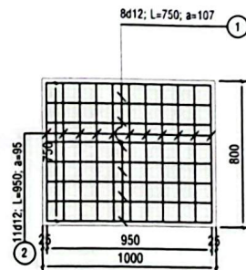
CHI TIẾT CỐT THÉP TẤM ĐAN-LỚP DƯỚI TL: 1/25
