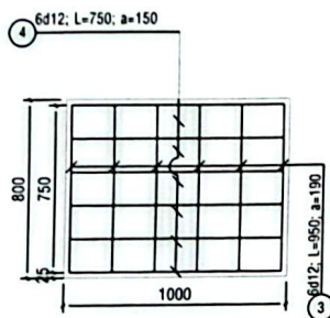
CHI TIẾT CỐT THÉP TẤM ĐAN-LỚP TRÊN TL: 1/25
