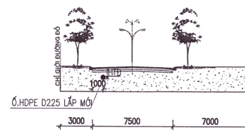
MẶT CẮT 4-4
