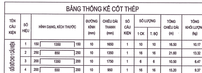
BẢNG THỐNG KÊ THÉP CHO 1 GÓI ĐỒ
