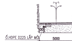
MẶT CẮT 6-6
