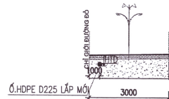
MẮT CẮT 6-6
