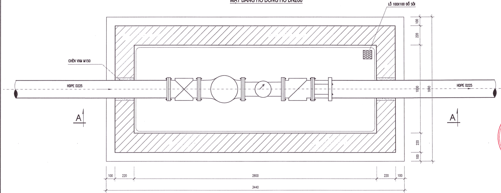
MẶT BẰNG HỐ ĐỒNG HỒ DN200
