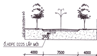
MẶT CẮT 3-3
