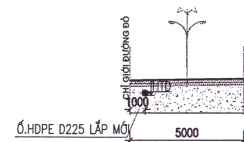
MẶT CẮT 6-6
