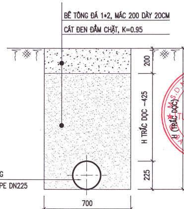
MẶT CẮT MƯƠNG ỐNG DN225 CÓ ỐNG LỒNG DN300 ĐƯỜNG BÊ TÔNG (L=2M)
