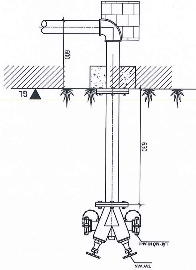
CHI TIẾT LẮP ĐẶT TRỤ NƯỚC CHỮA CHÁY 2 CỬA
