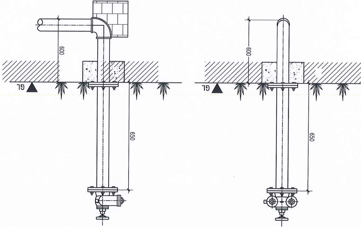
CHI TIẾT LẮP ĐẶT TRỤ NƯỚC TIẾP NƯỚC CHỮA CHÁY 2 CỬA
