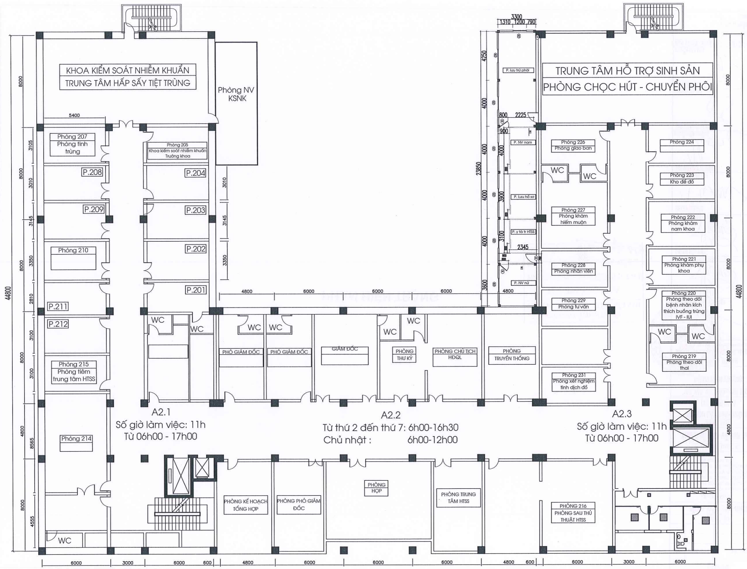
MẶT BẰNG TẦNG 2
