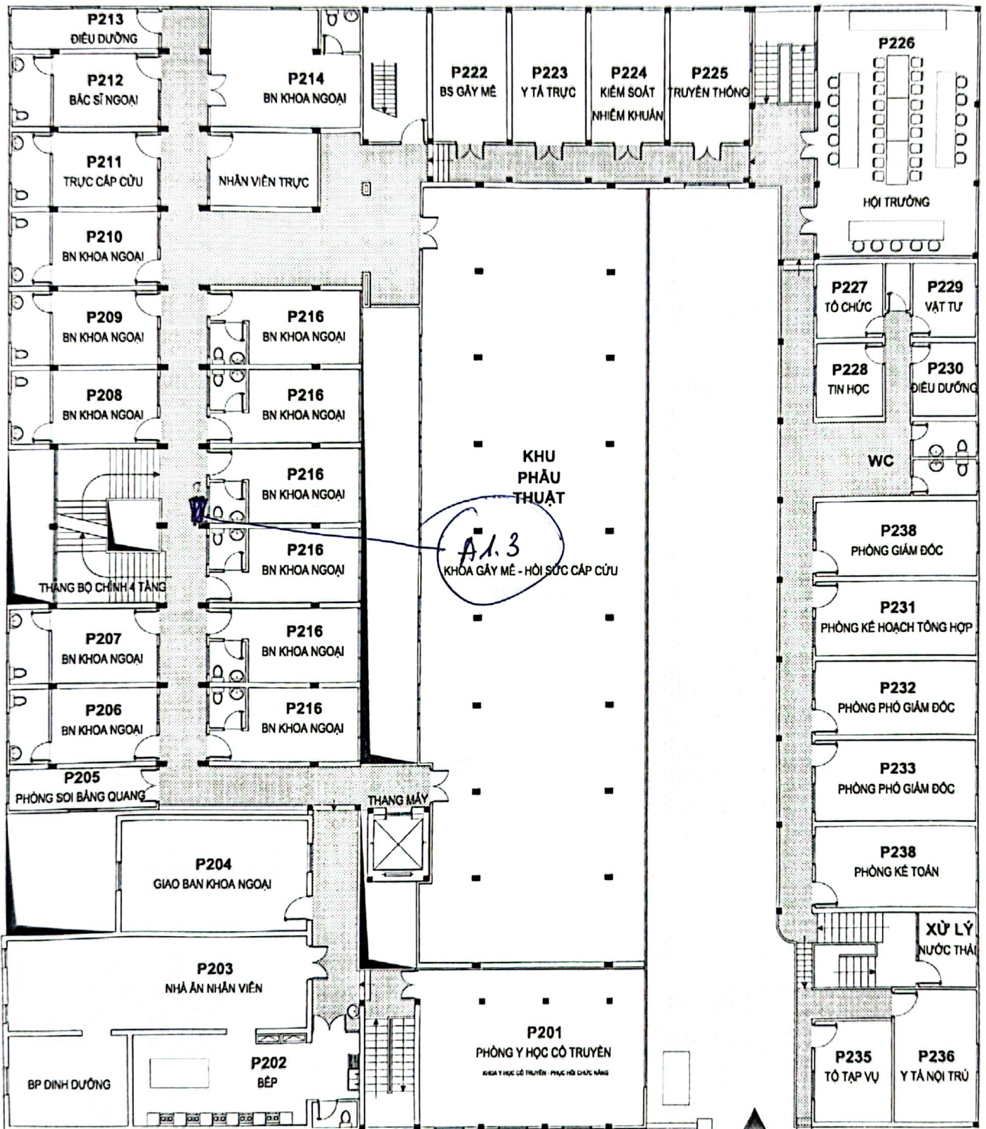
SƠ ĐỒ MẶT BẰNG TẦNG 2
